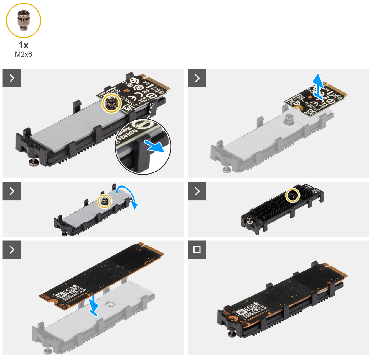
Figure 23. Remplacement du disque SSD M.2 2230 par un disque SSD M.2 2280
