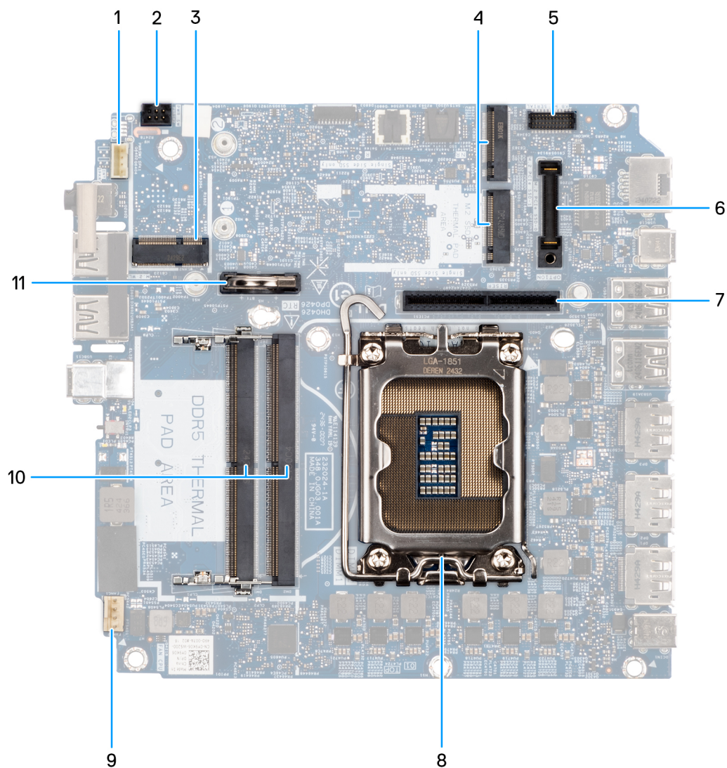
Figure 53. Connecteurs de la carte système
