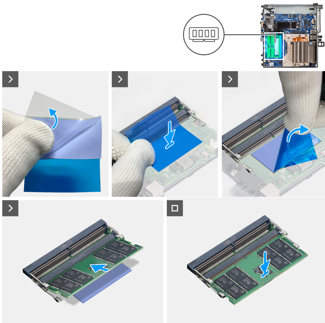
Figure 18. Installation des modules de mémoire
