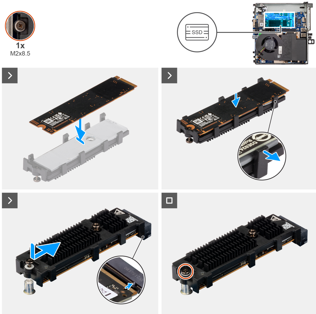
Figure 22. Installation du disque SSD M.2 2280 PCIe (logement 1)
