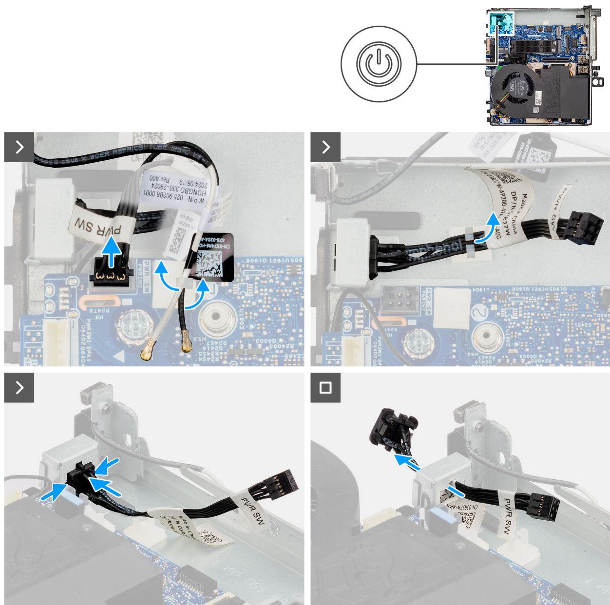
Figure 56. Retrait du bouton d'alimentation
