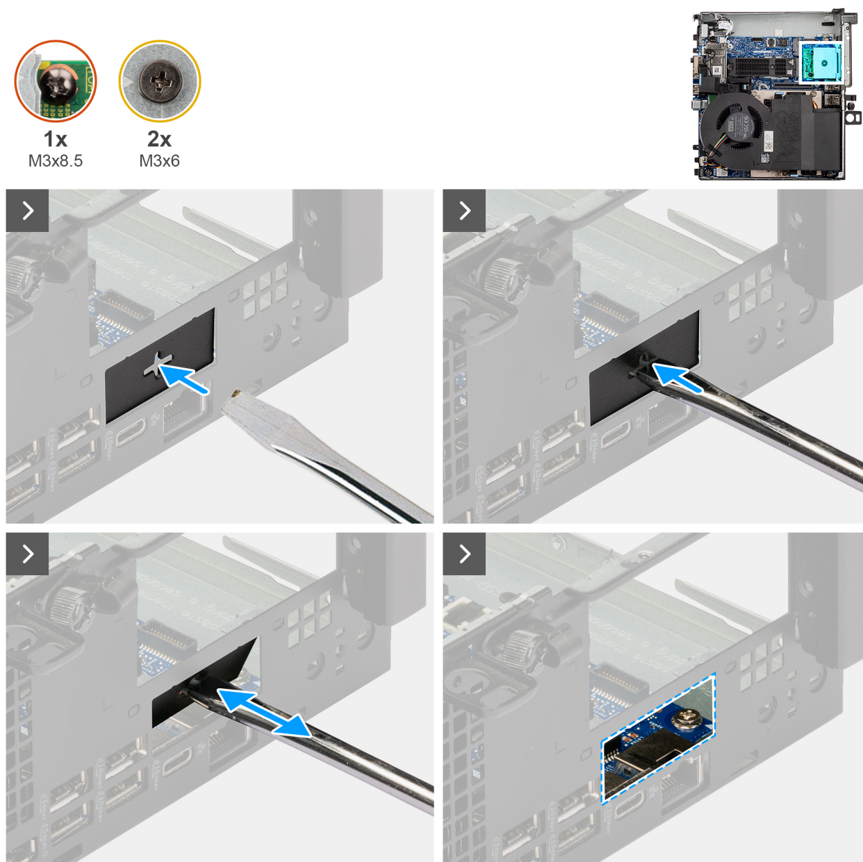
Figure 31. Installation du port fibre optique 5G
