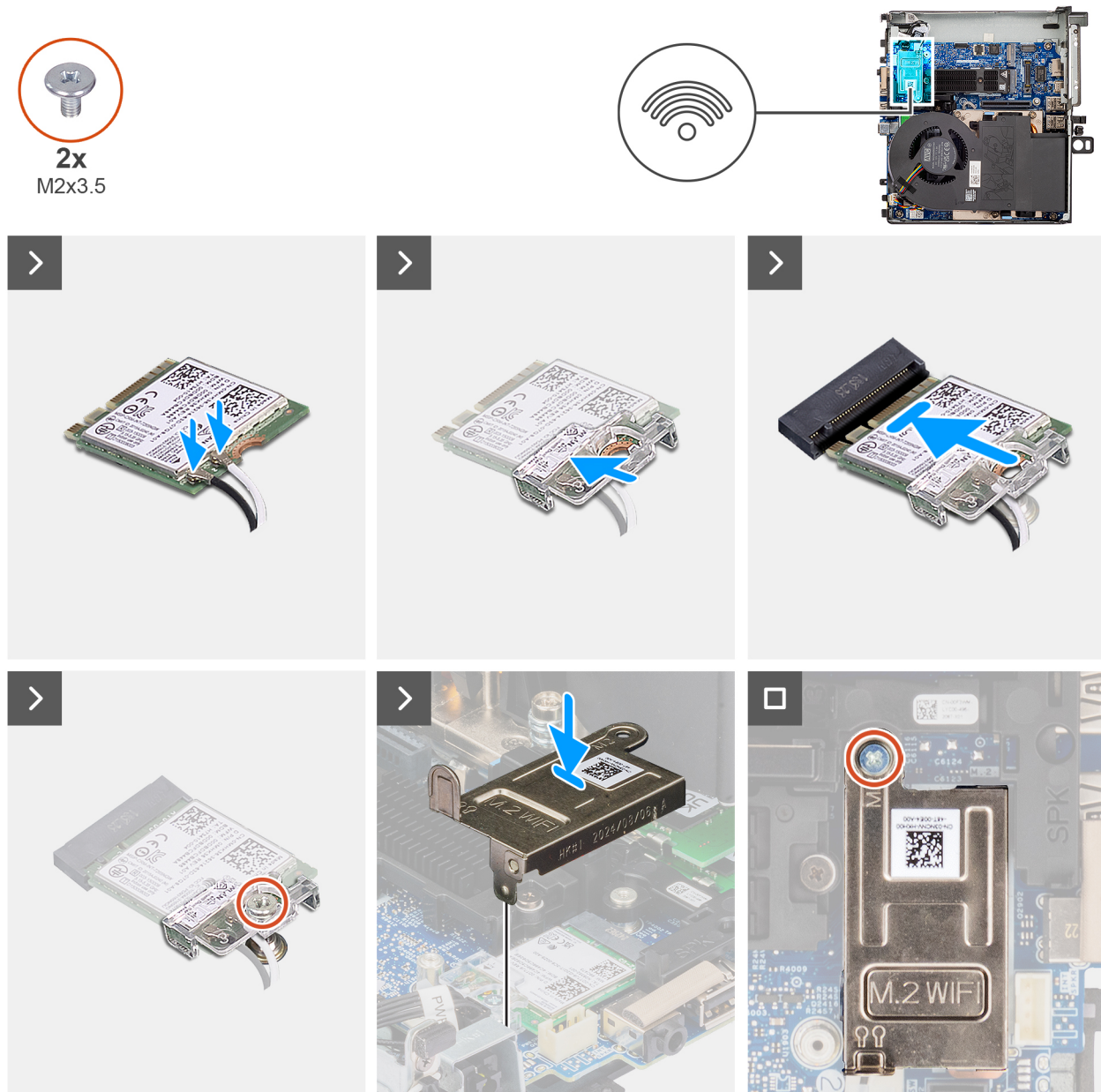
Figure 26. Installation de la carte sans fil
