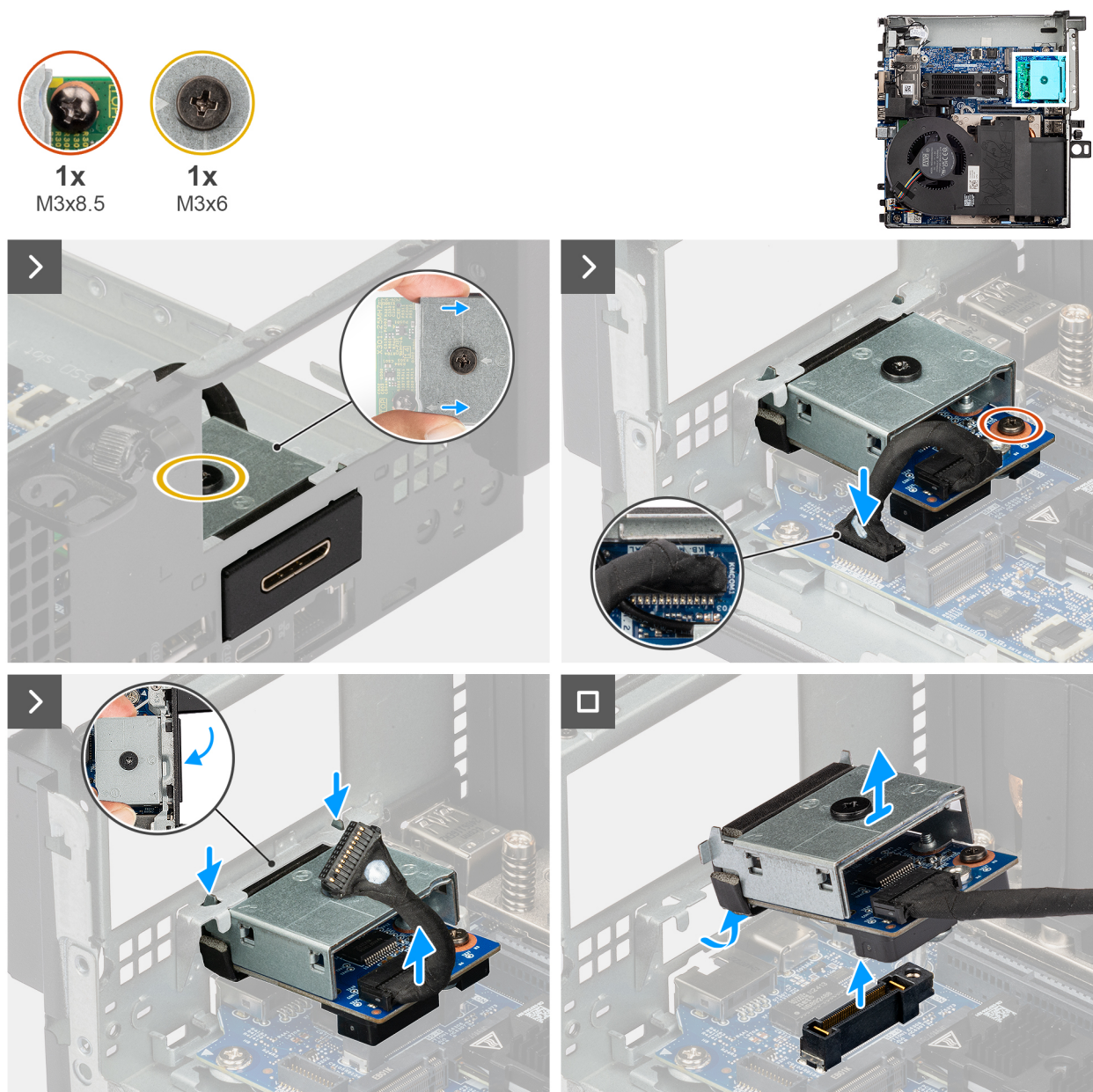
Figure 36. Retrait du port PS2
