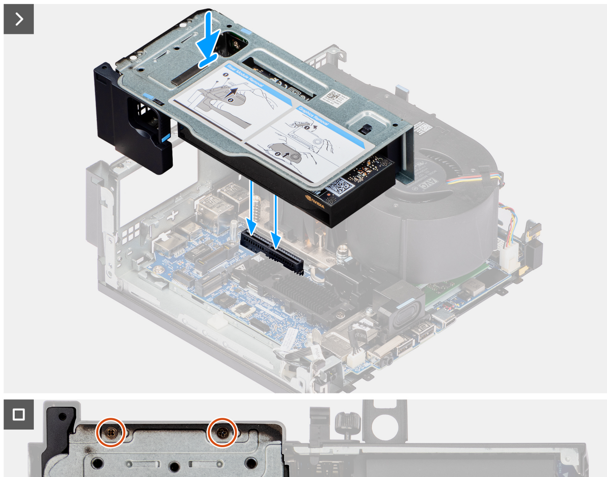
Figure 10. Installation du module de la carte de montage
