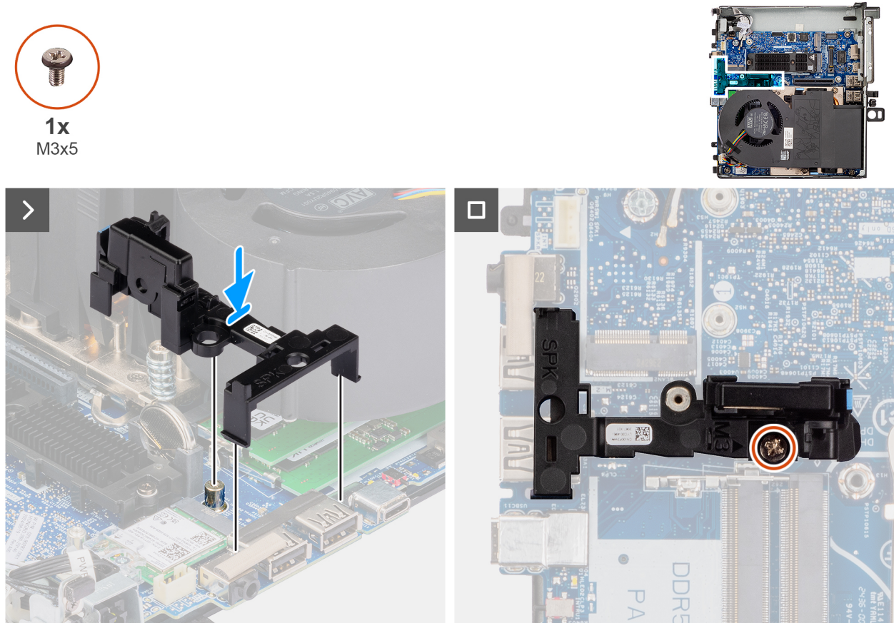
Figure 30. Installation du support de haut-parleur
