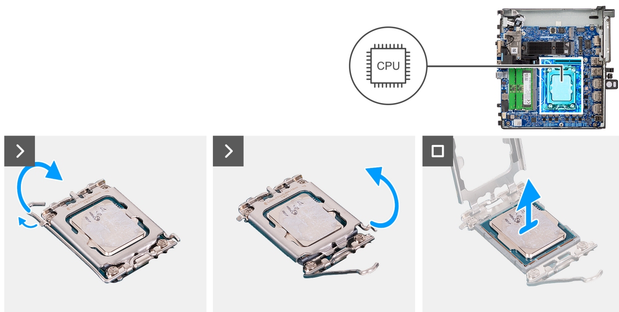
Figure 48. Retrait du processeur
