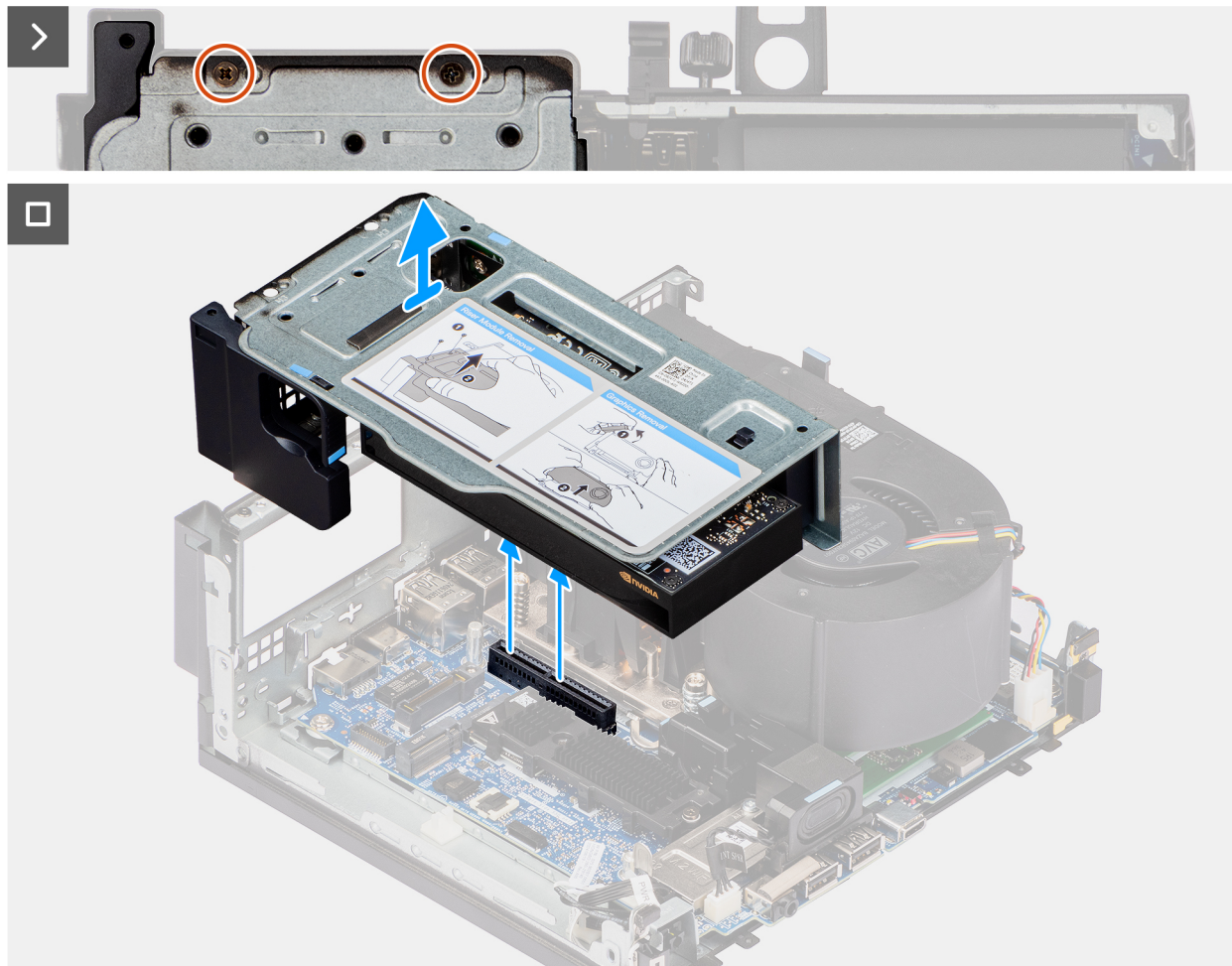
Figure 9. Retrait du module de la carte de montage
