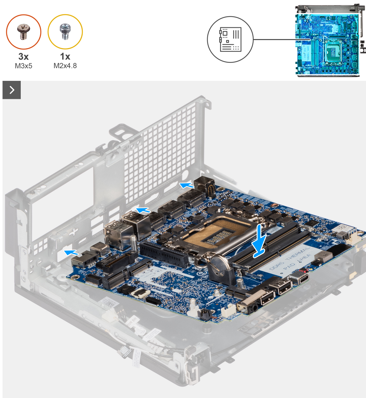
Figure 54. Installation de la carte système
