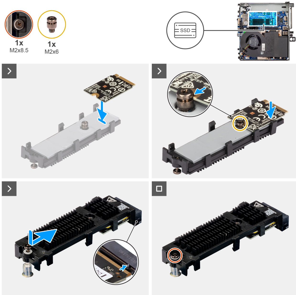
Figure 20. Installation du disque SSD M.2 2230 PCIe (logement 1)
