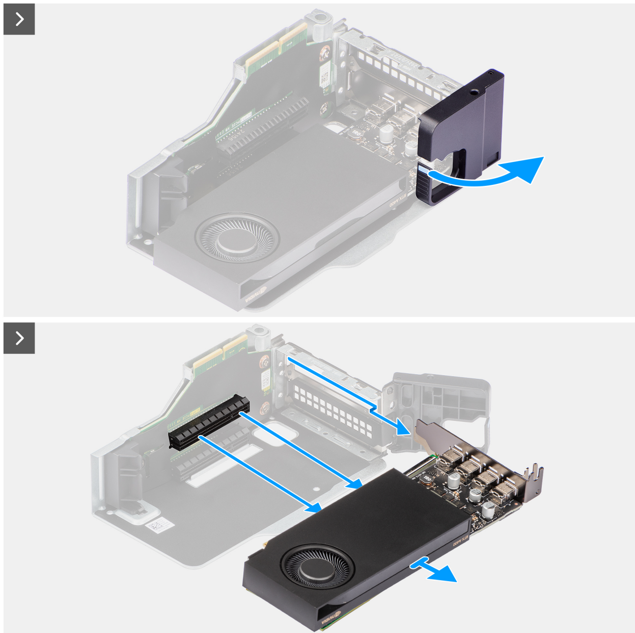
Figure 11. Retrait de la carte graphique
