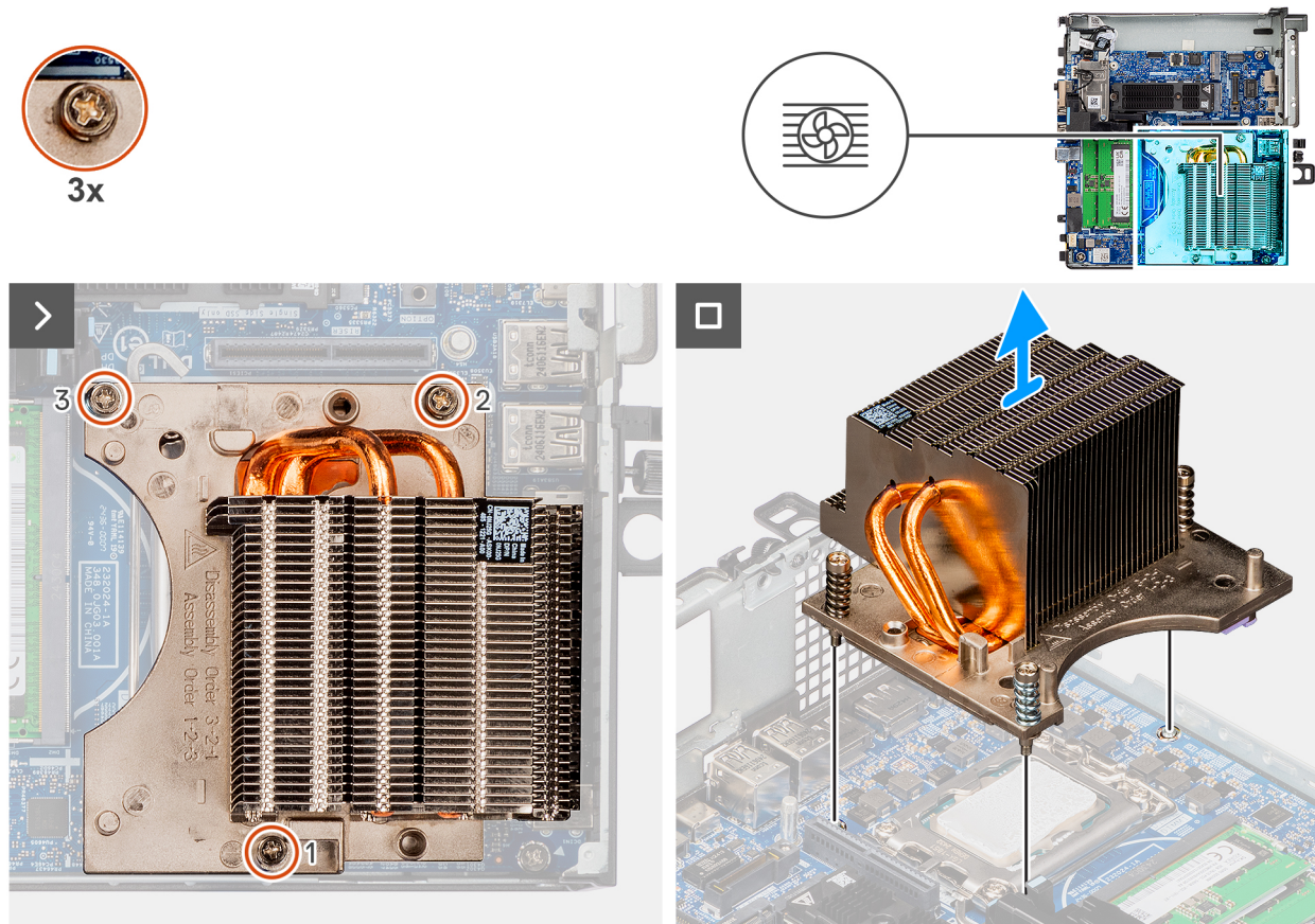
Figure 46. Retrait du dissipateur de chaleur
