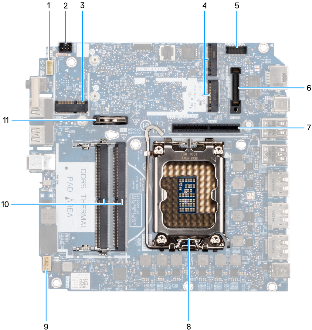
Figure 50. Connecteurs de la carte système
