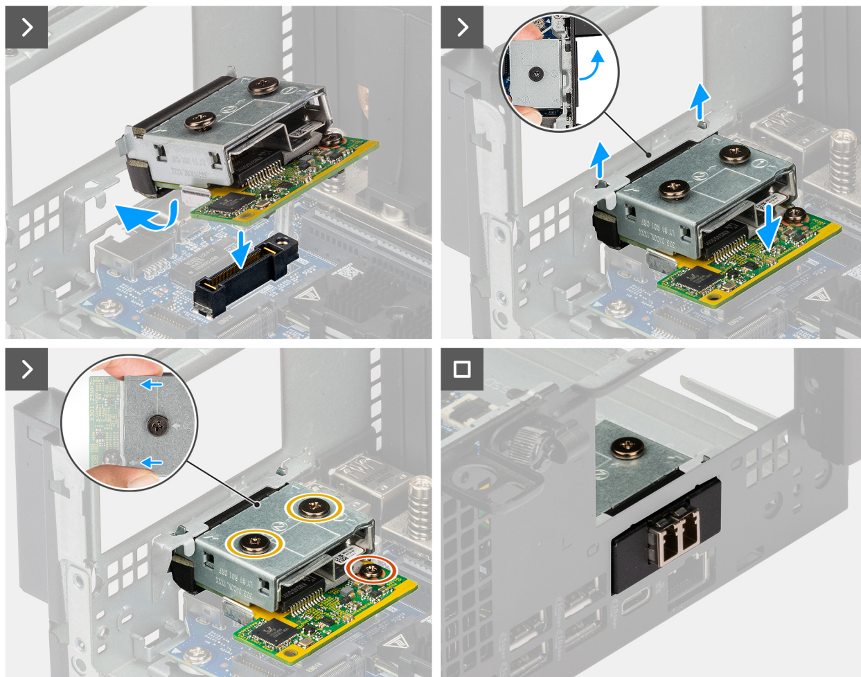
Figure 32. Installation du port fibre optique 5G
