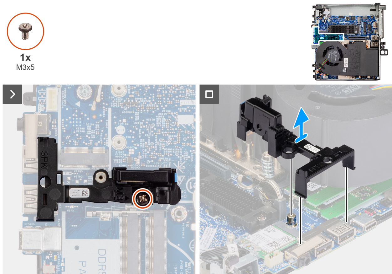
Figure 29. Retrait du support du haut-parleur
