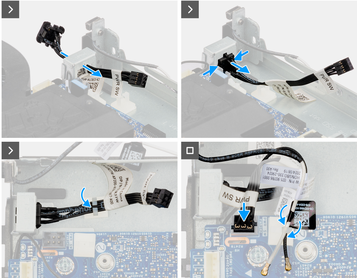
Figure 57. Installation du bouton d'alimentation
