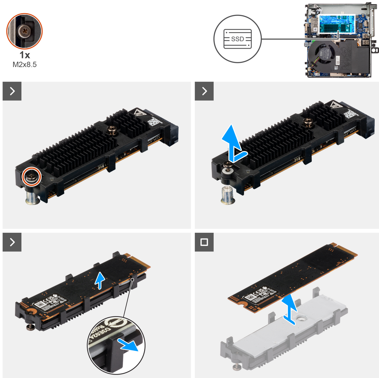
Figure 21. Retrait du disque SSD M.2 2280 PCIe (logement 1)
