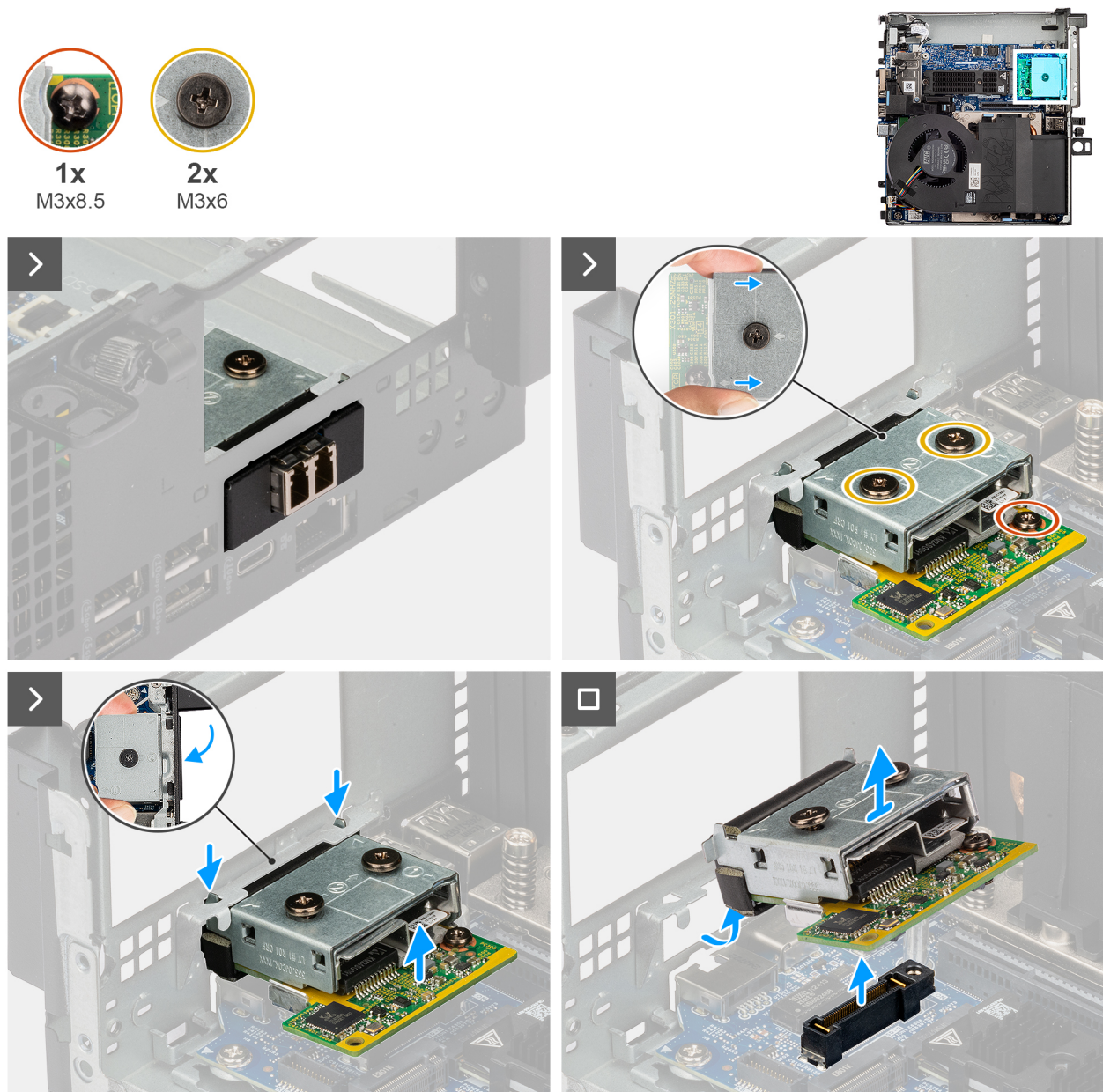
Figure 33. Retrait du port fibre optique 5G
