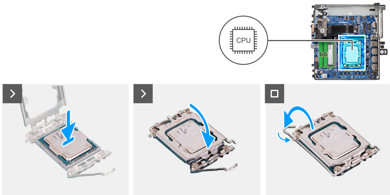
Figure 49. Installation du processeur
