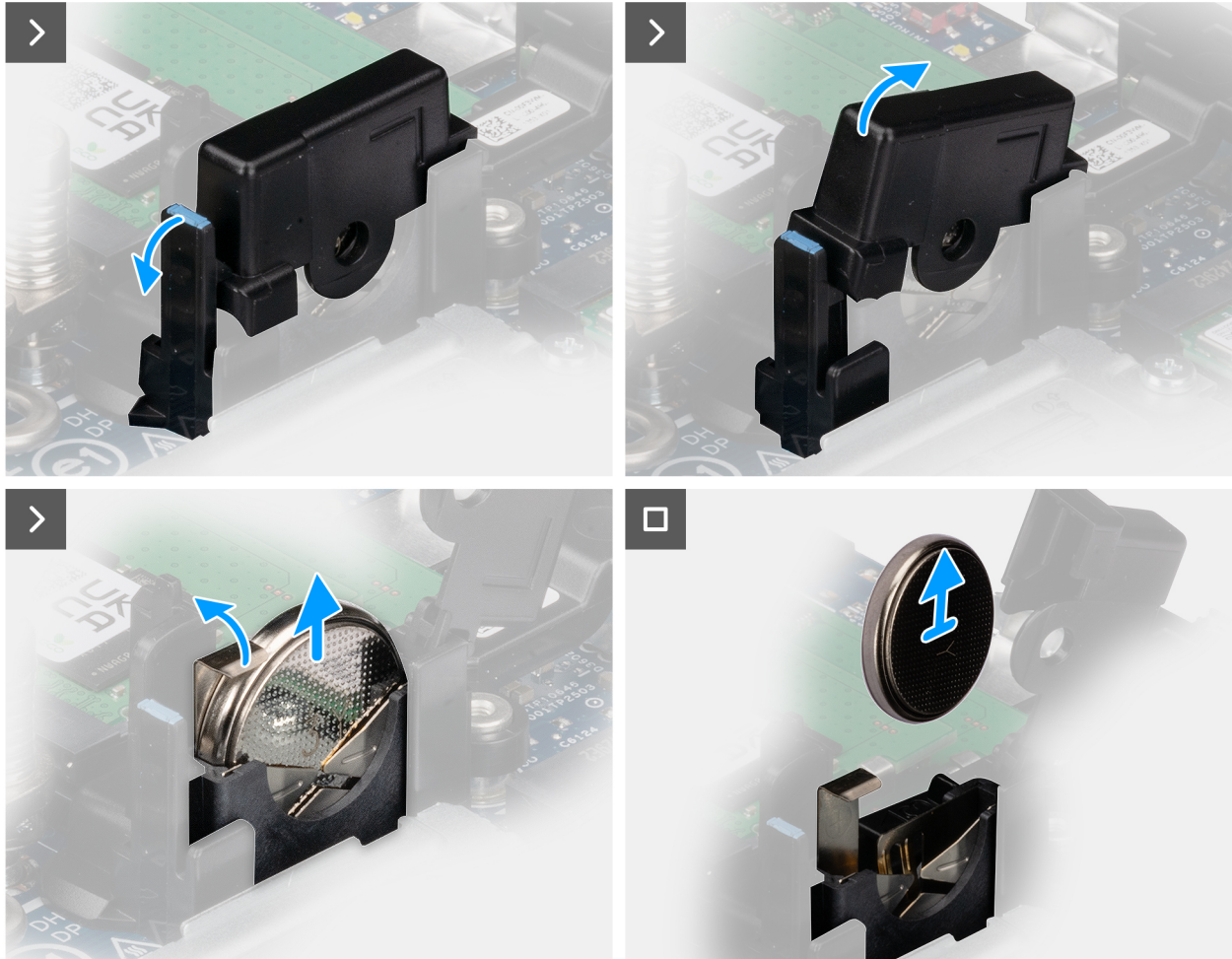
Figure 7. Retrait de la pile bouton
