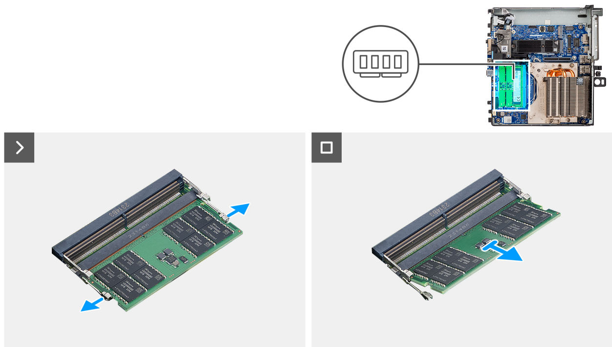
Figure 17. Retrait des modules de mémoire
