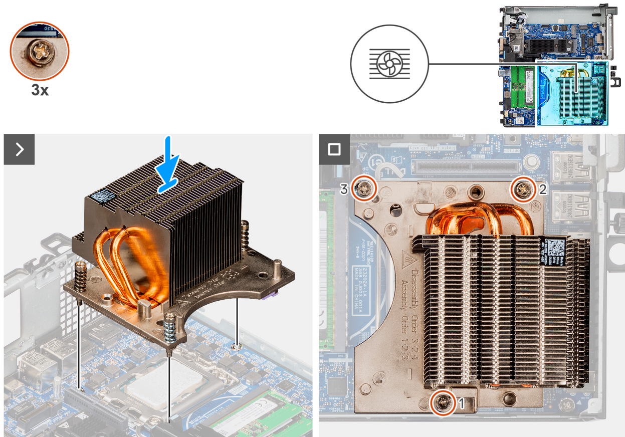
Figure 47. Installation du dissipateur de chaleur
