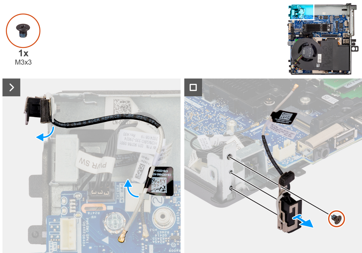
Figure 58. Retrait de l'antenne interne (emplacement 1)
