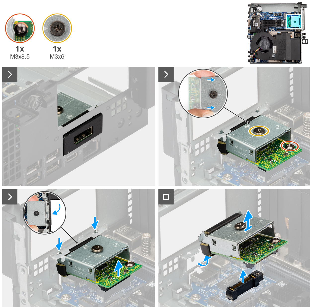
Figure 39. Retrait du port DisplayPort
