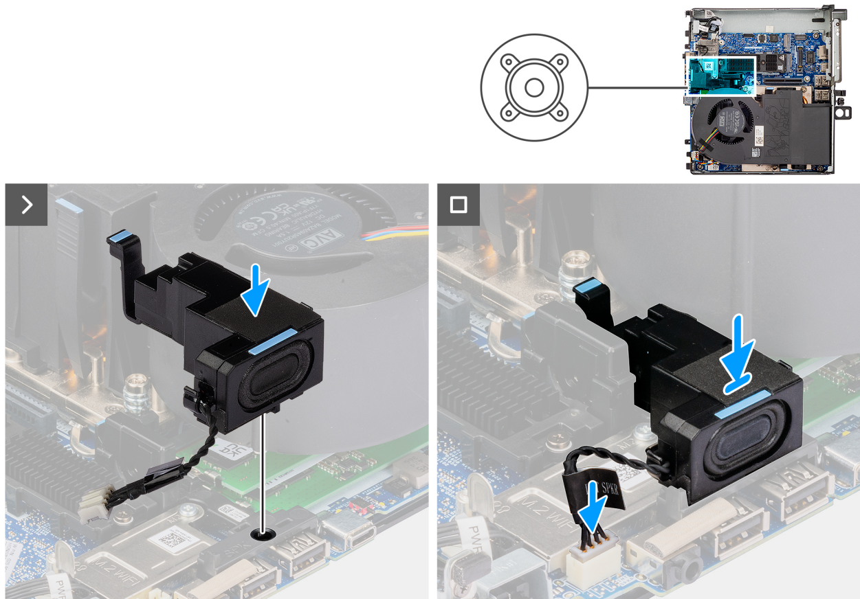
Figure 28. Installation du haut-parleur
