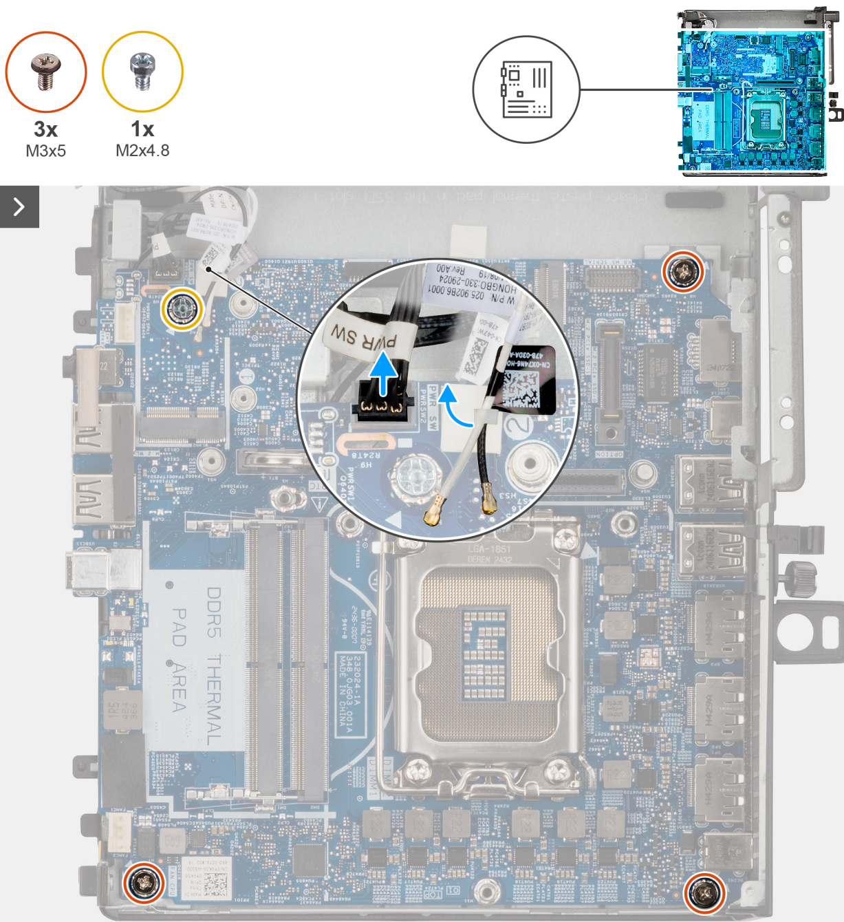
Figure 51. Retrait de la carte système
