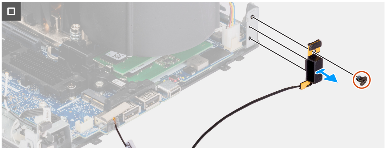
Figure 60. Retrait de l'antenne interne (emplacement 2)
