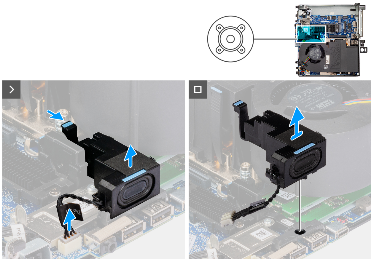
Figure 27. Retrait du haut-parleur
