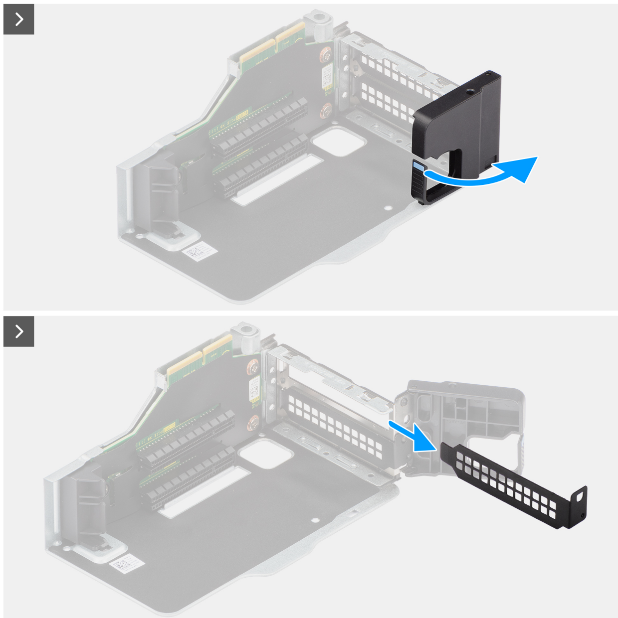
Figure 13. Installation de la carte graphique
