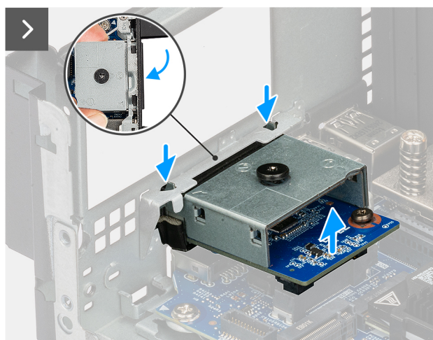
Figure 45. Retrait du port HDMI
