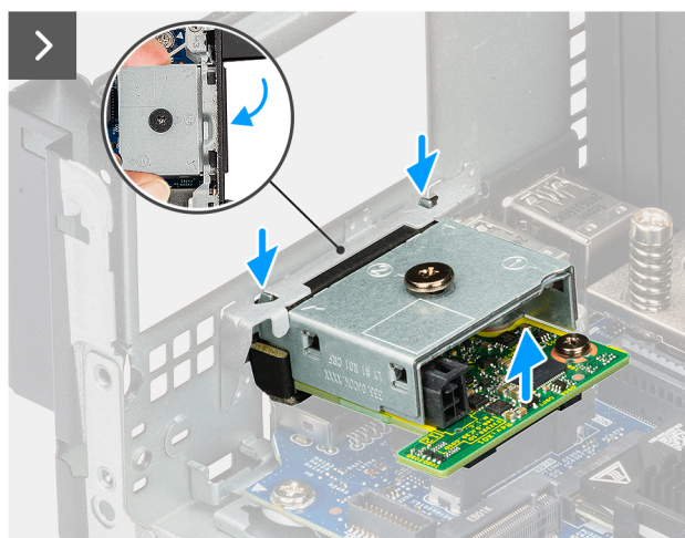
Figure 42. Retrait du port Thunderbolt
