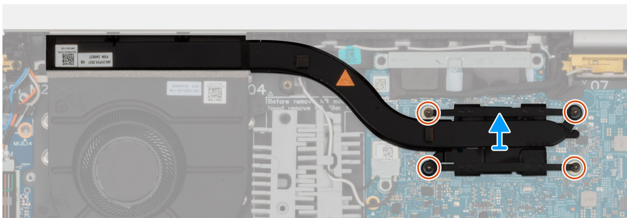
Abbildung 45. Kühlkörper entfernen
