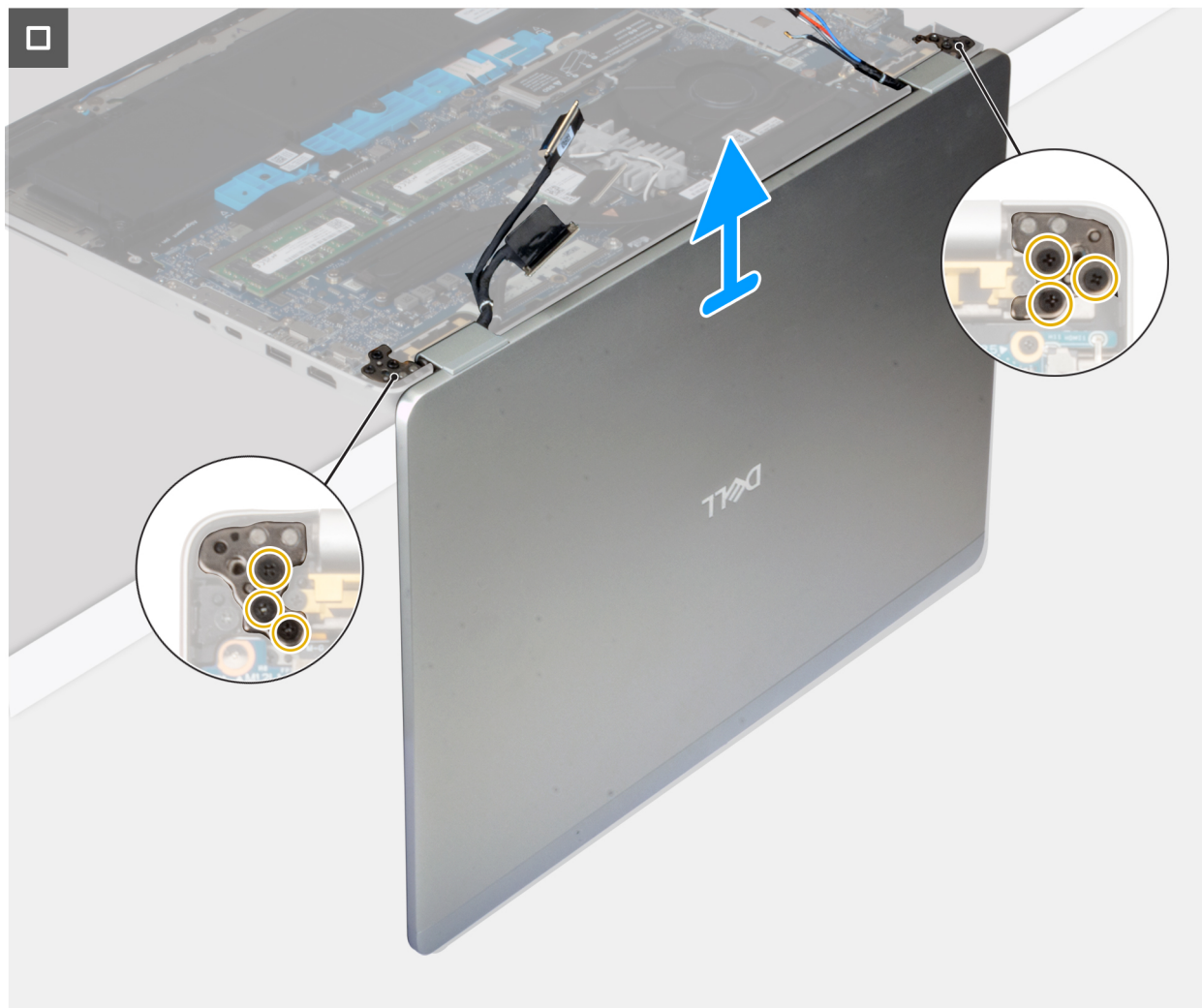
Abbildung 62. Entfernen der Bildschirmbaugruppe
