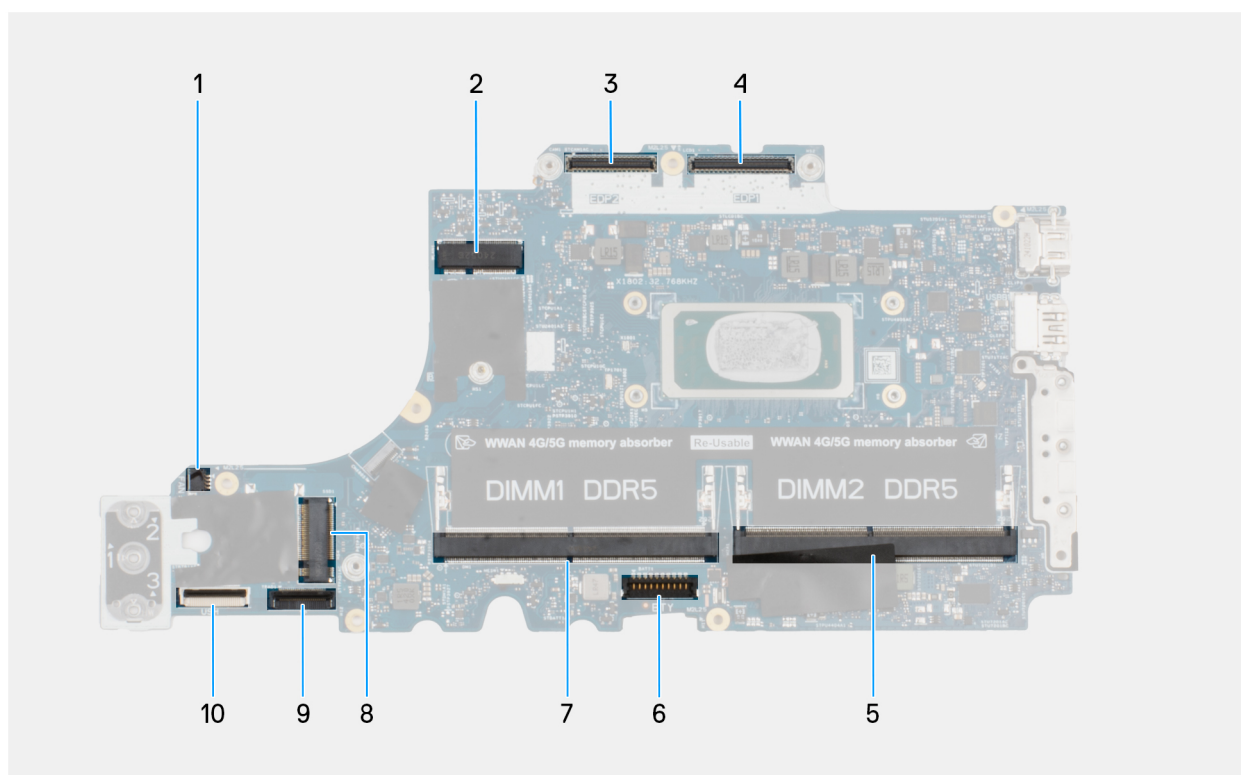
Abbildung 54. Hauptplatinenanschluss
