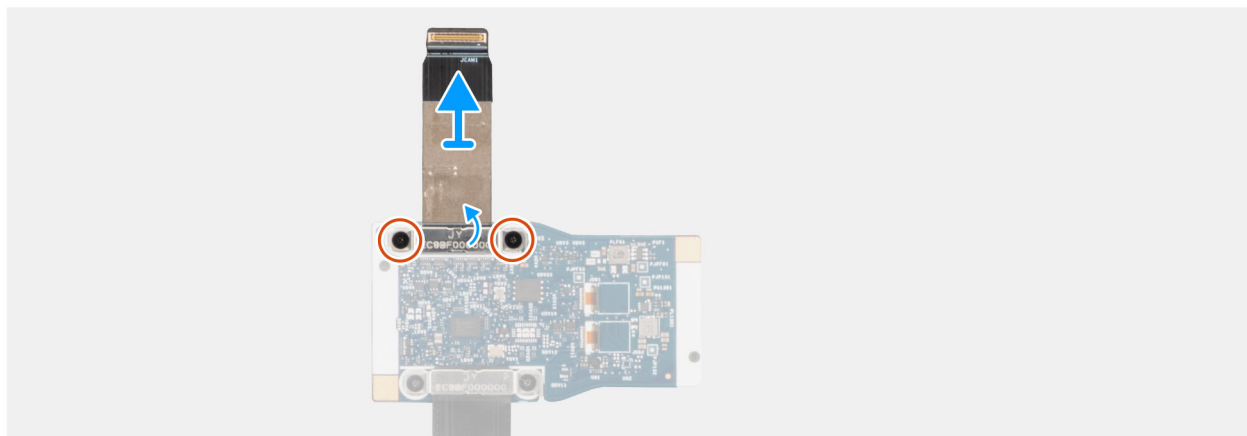
Abbildung 87. Entfernen des Kabels der mittleren Zusatzplatine
