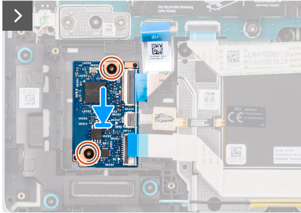
Abbildung 39. Installieren der USH-Zusatzplatine
