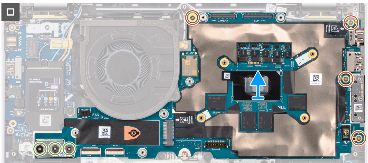
Abbildung 43. Entfernen der Systemplatine
