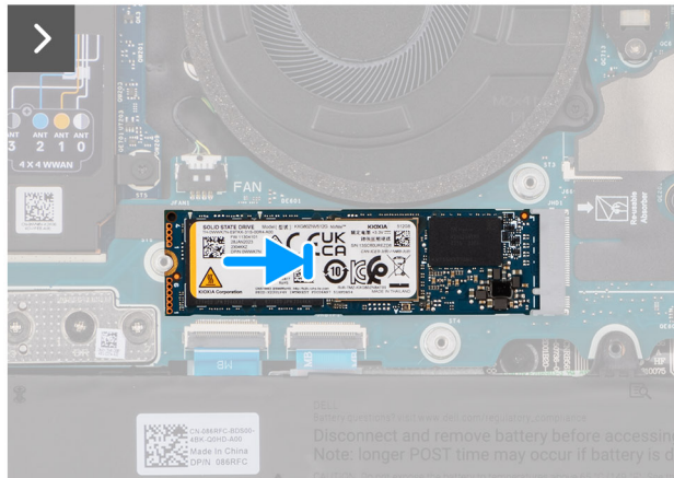
Abbildung 30. Installieren der M.2-2280-SSD
