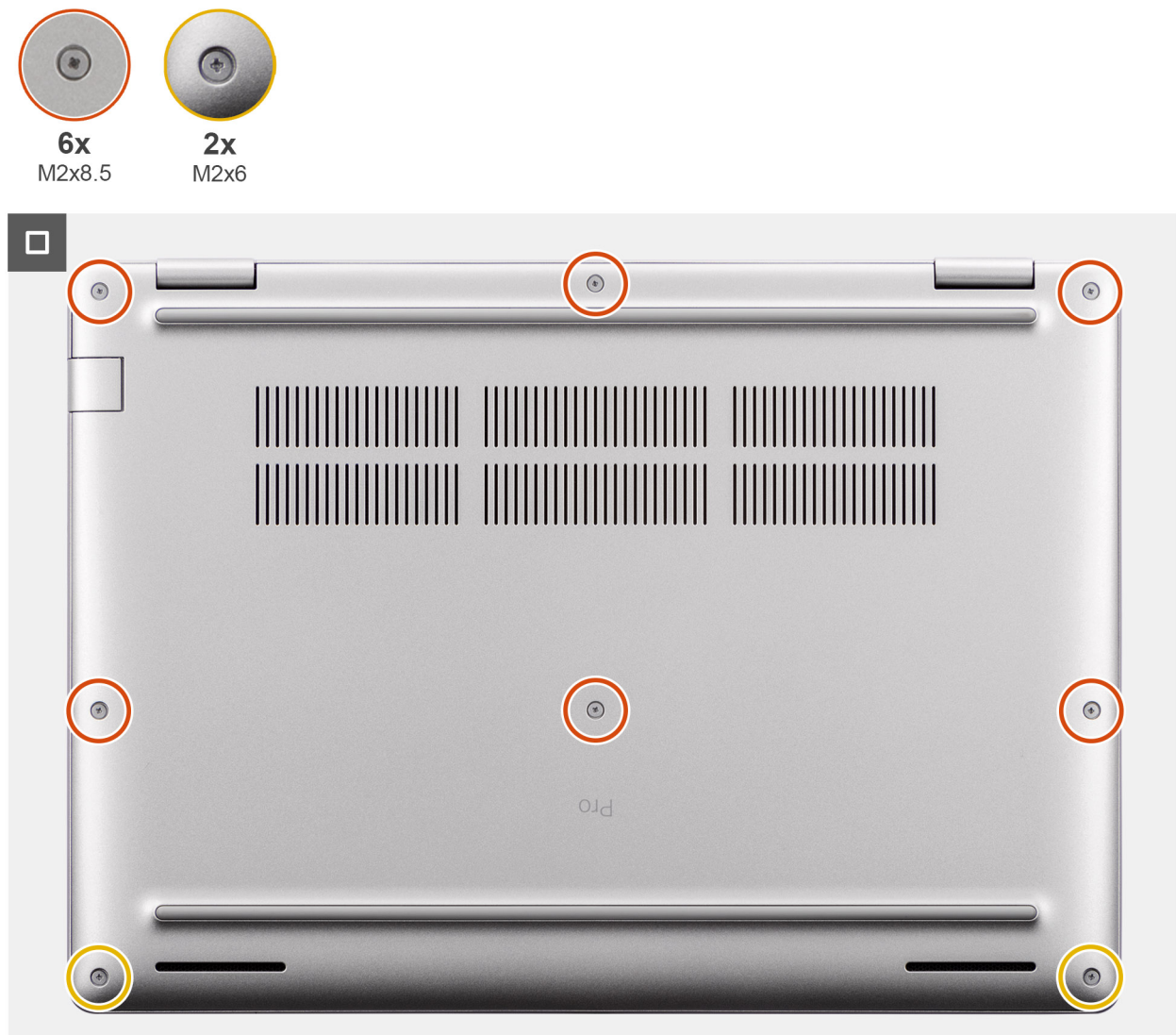
Abbildung 20. Anbringen der Bodenabdeckung
