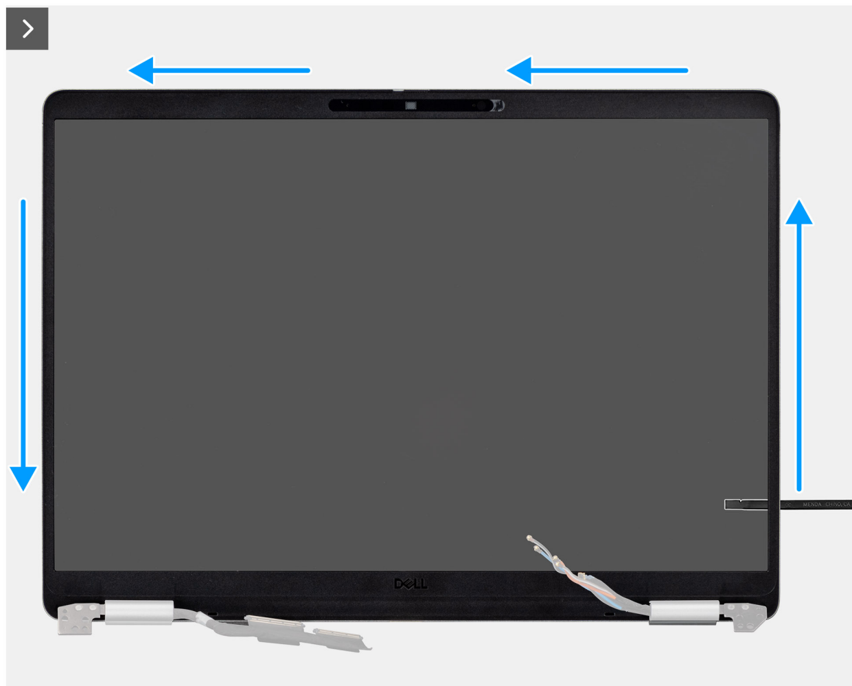
Abbildung 64. Abhebeln der Blende an den Seiten
