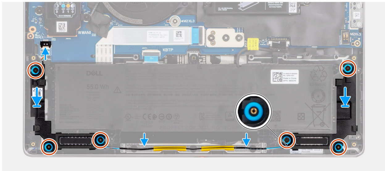
Abbildung 32. Installieren der Lautsprecher
