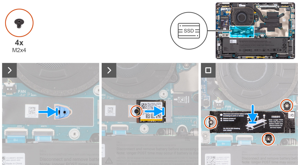
Abbildung 28. Einbauen des M.2-2280-SSD
