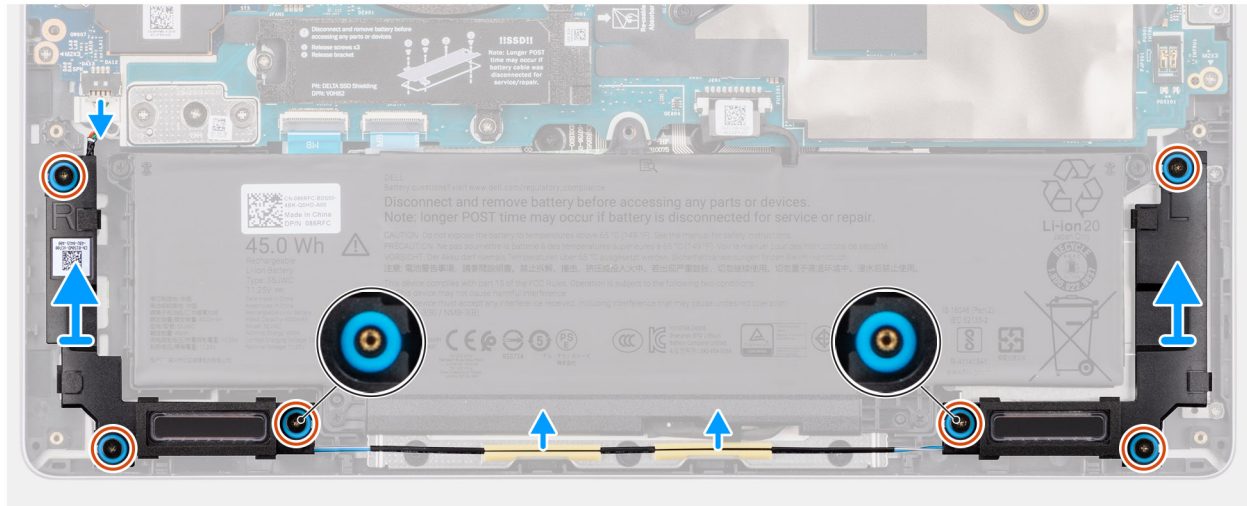
Abbildung 31. Entfernen der Lautsprecher
