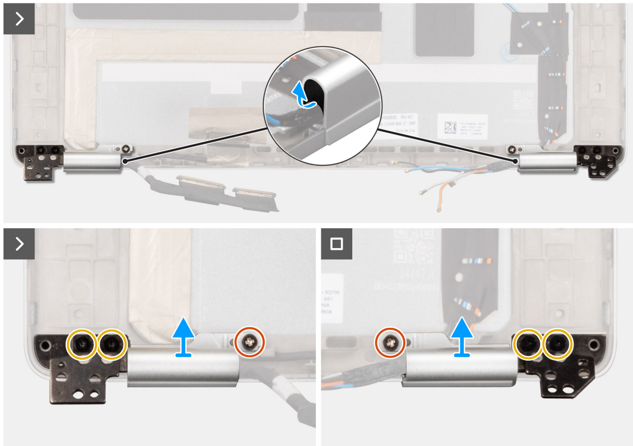
Abbildung 73. Entfernen der Bildschirmscharniere
