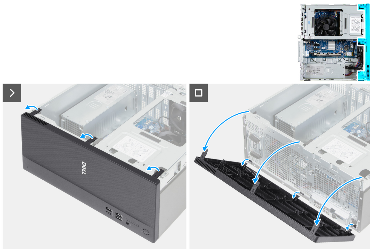
Rysunek 18. Wymontowywanie pokrywy przedniej
