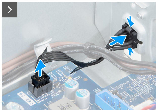
Rysunek 34. Wymontowywanie przycisku zasilania
