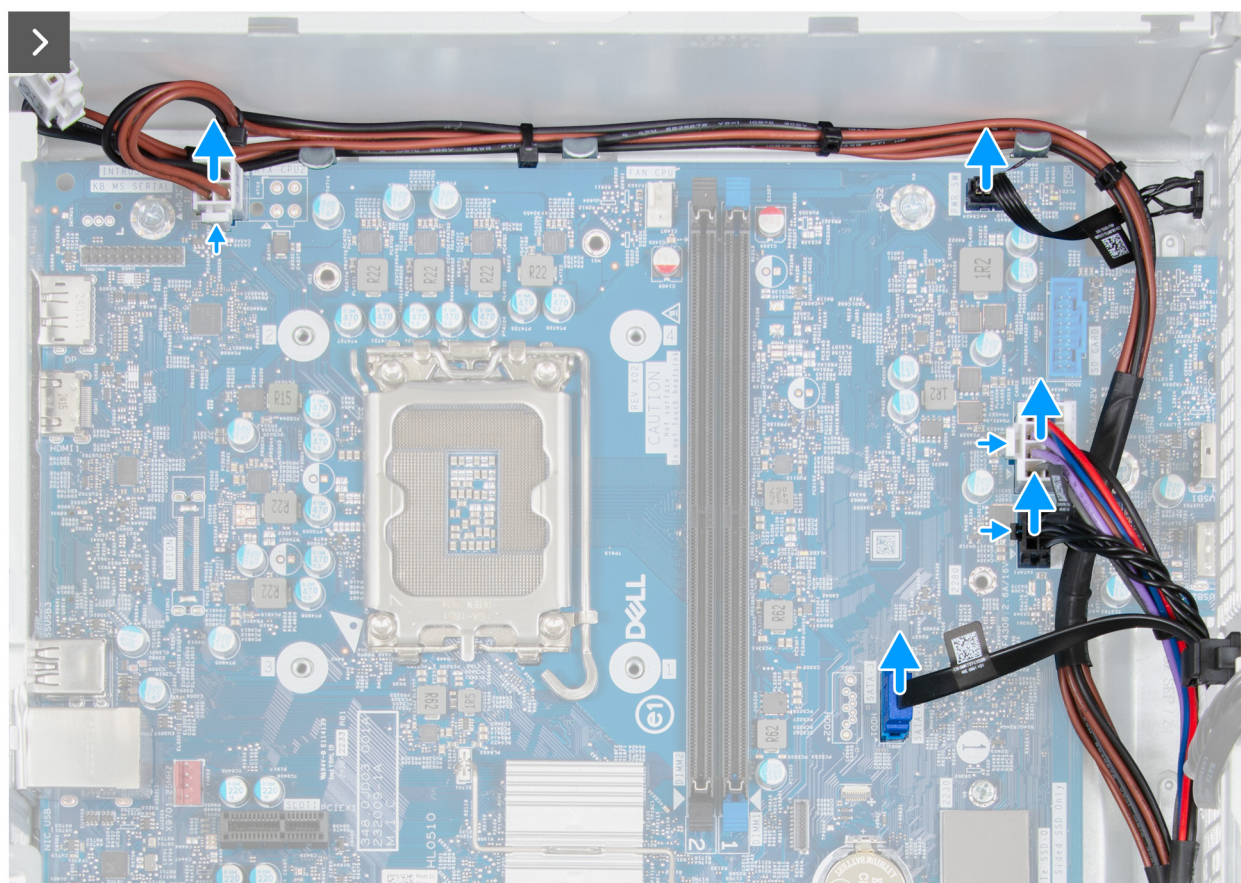
Rysunek 55. Wymontowywanie płyty głównej
