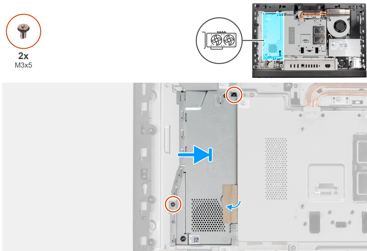
Rysunek 25. Instalowanie zestawu karty graficznej (model z ekranem dotykowym)
