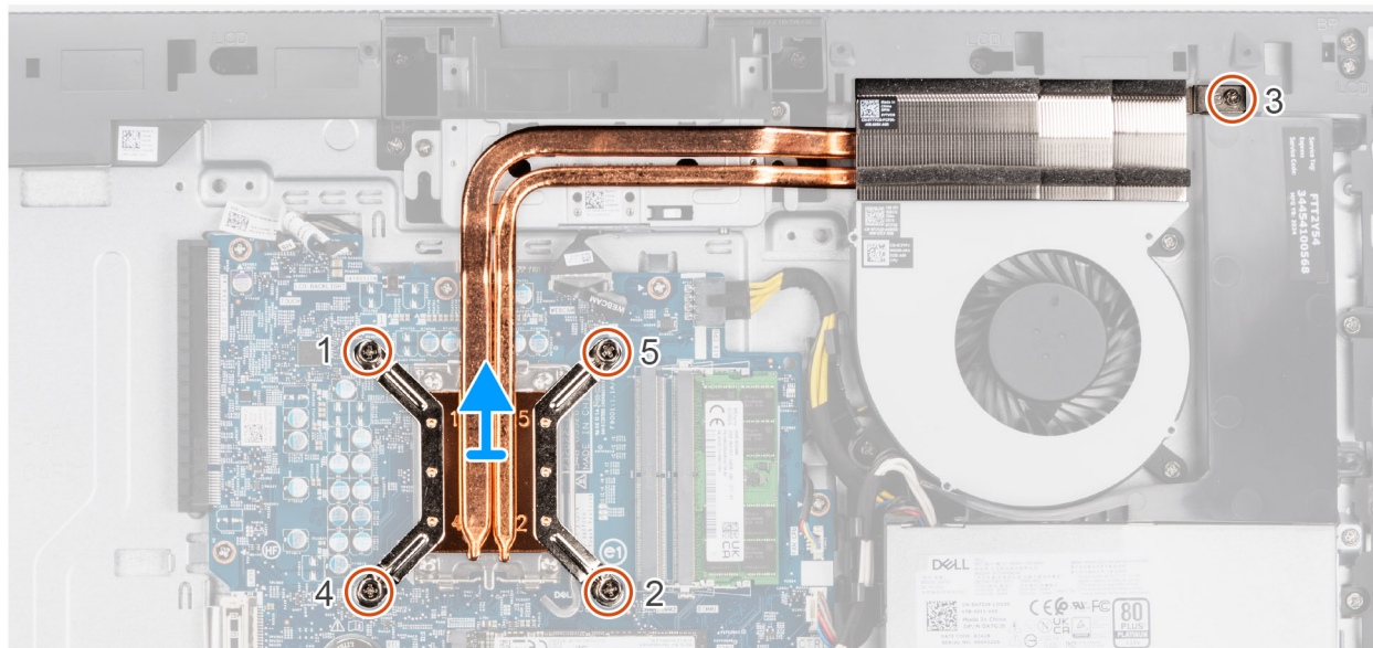
Rysunek 59. Wymontowywanie radiatora
