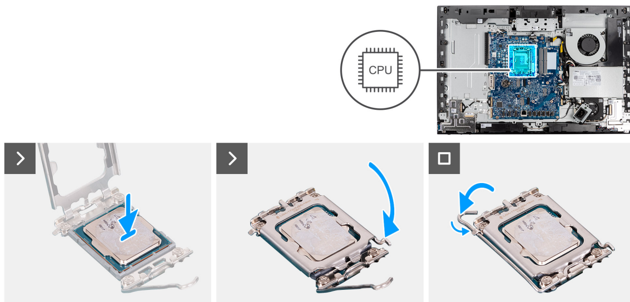
Rysunek 62. Instalowanie procesora
