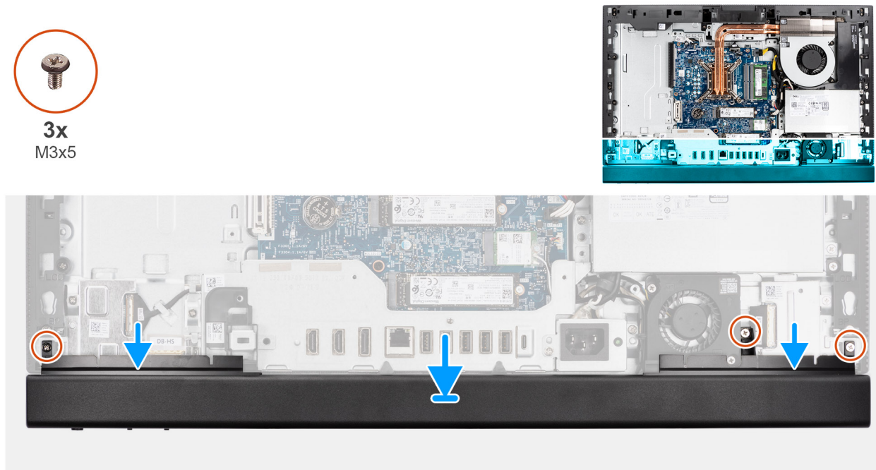
Rysunek 46. Instalowanie pokrywy dolnej
