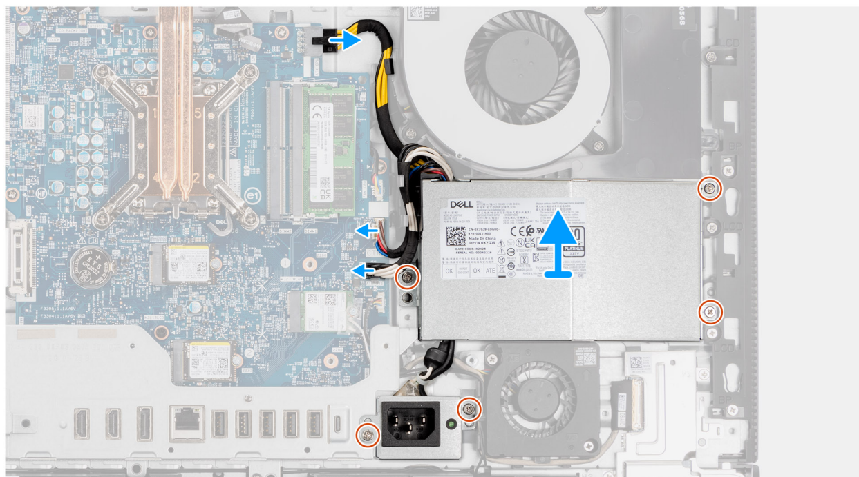
Rysunek 51. Wymontowywanie zasilacza
