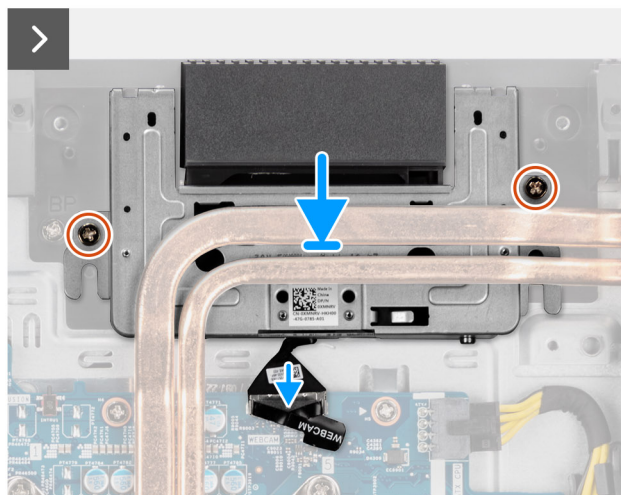
Rysunek 48. Instalowanie zestawu wysuwanej kamery
