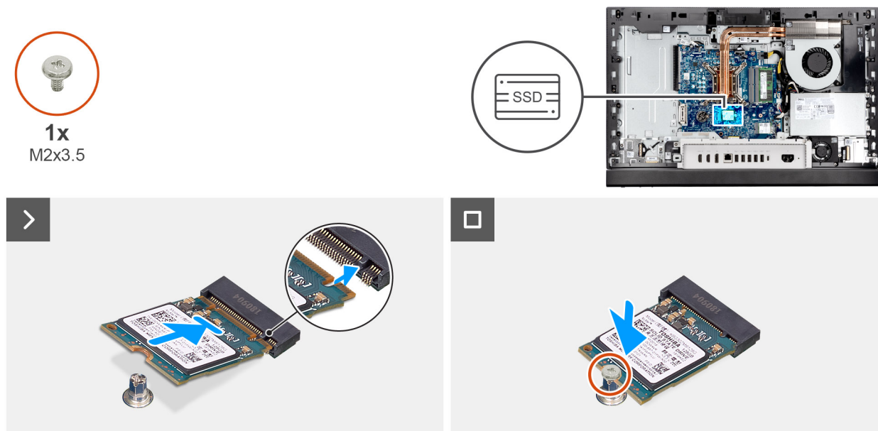
Rysunek 32. Instalowanie dysku SSD M.2 2230 w gnieździe M.2 nr 0
