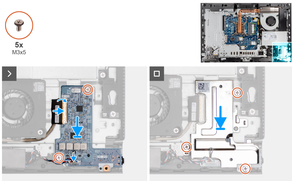
Rysunek 72. Instalowanie karty dźwiękowej
