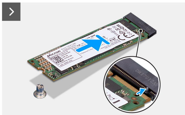
Rysunek 34. Instalowanie dysku SSD M.2 2280 w gnieździe M.2 nr 0
