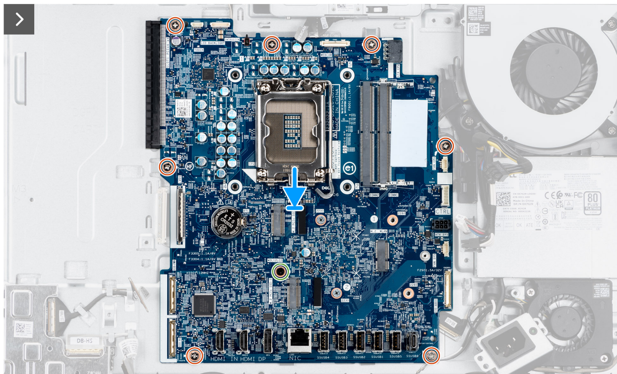
Rysunek 67. Instalowanie płyty głównej
