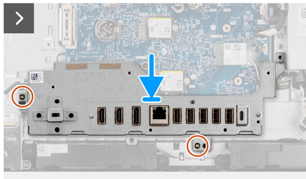
Rysunek 56. Instalowanie panelu we/wy
