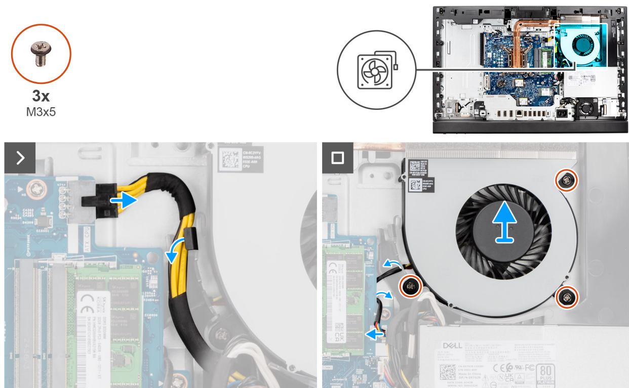
Rysunek 49. Wymontowywanie wentylatora
