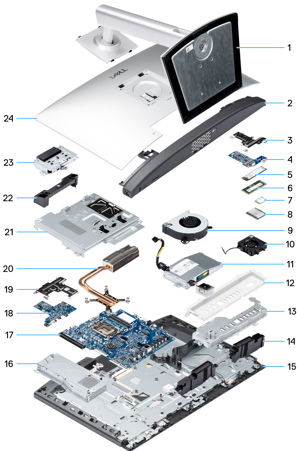
Rysunek 14. Główne elementy komputera Dell Pro 24 All-in-One Plus QB24250
