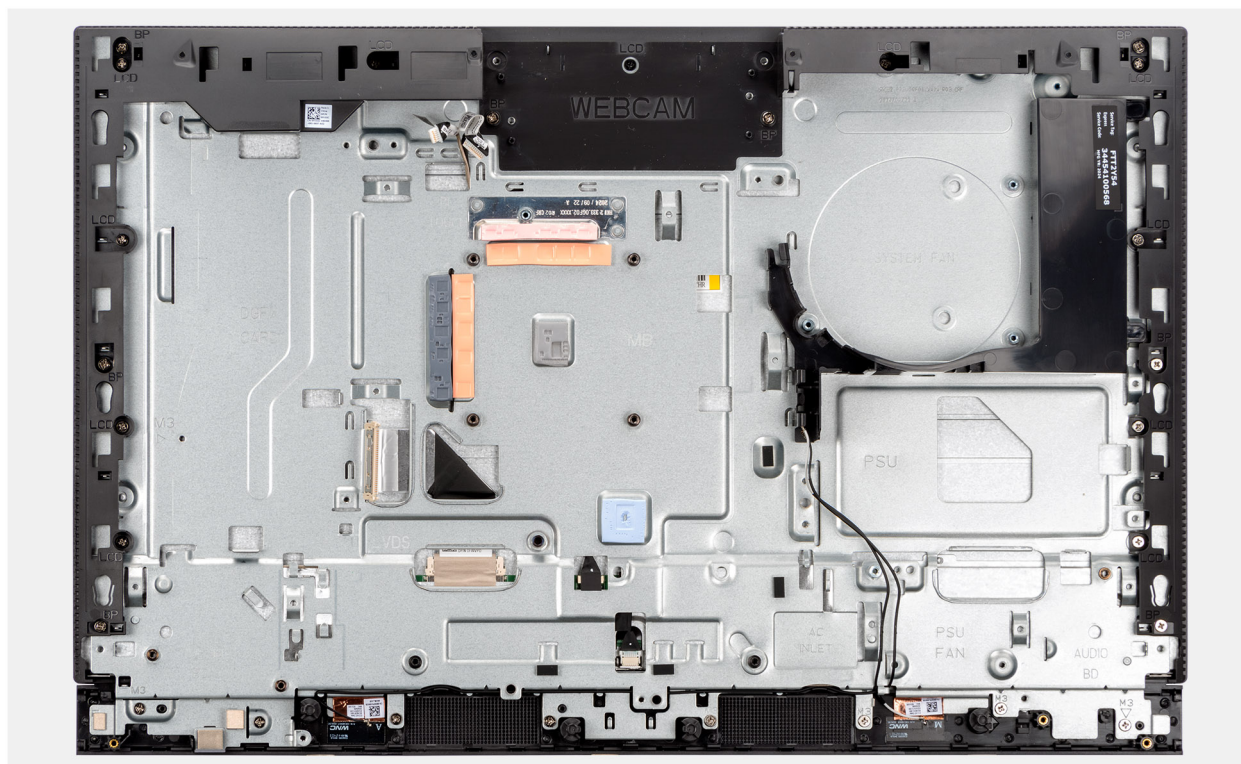
Rysunek 74. Wymontowywanie podstawy zestawu wyświetlacza
