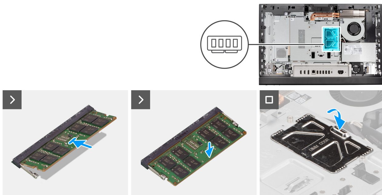
Rysunek 22. Instalowanie modułów pamięci
