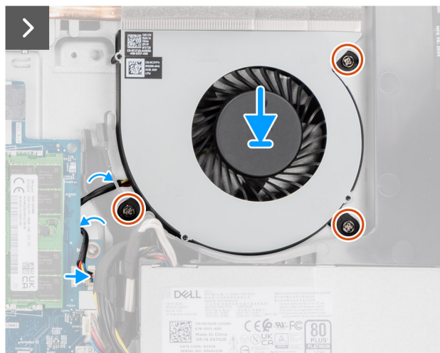
Rysunek 50. Instalowanie wentylatora
