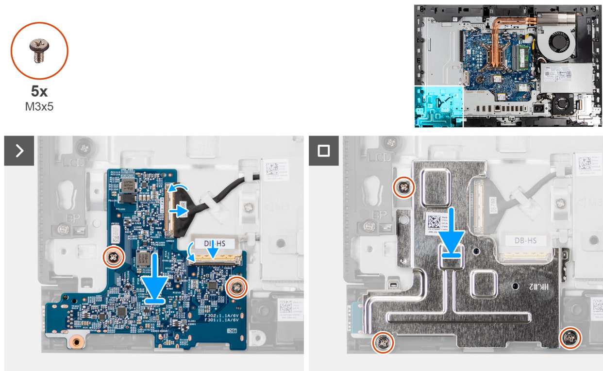
Rysunek 70. Instalowanie płyty przycisku zasilania i złączy we/wy
