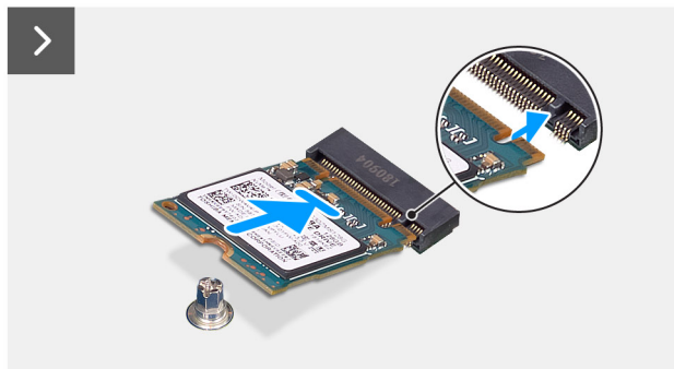
Rysunek 37. Instalowanie dysku SSD M.2 2230 w gnieździe M.2 nr 1
