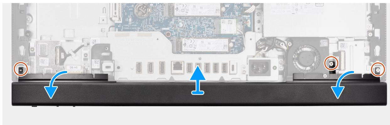
Rysunek 45. Wymontowywanie pokrywy dolnej
