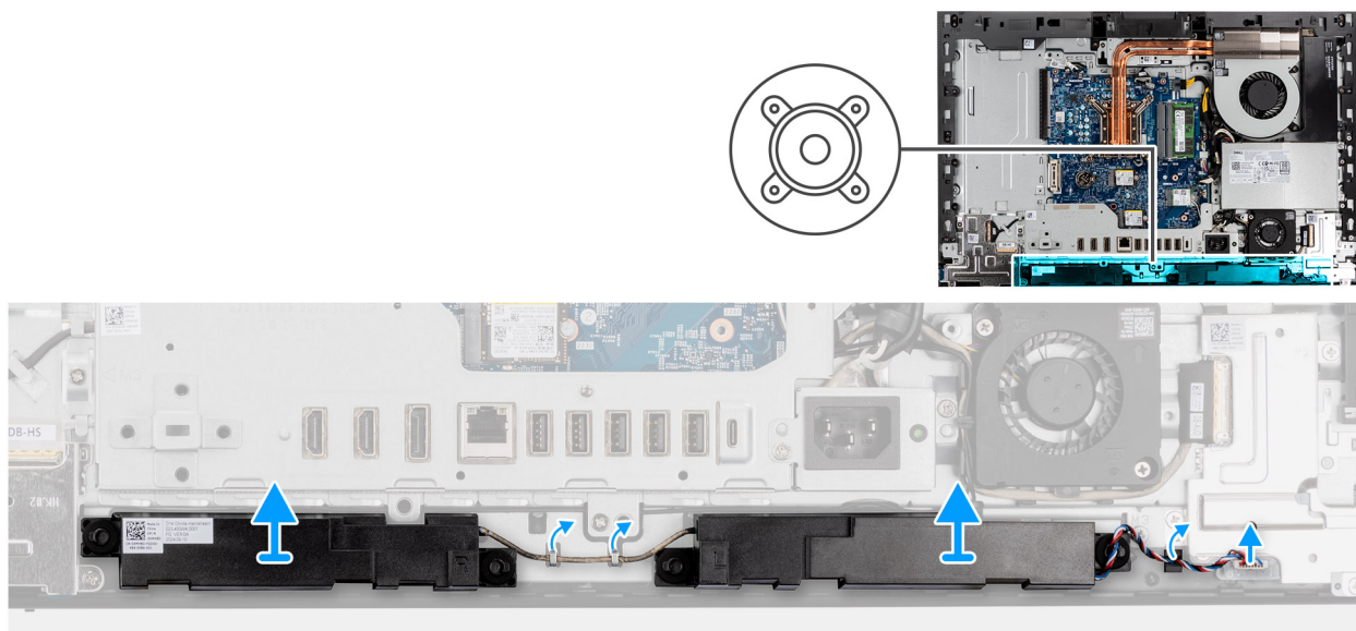
Rysunek 57. Wymontowywanie głośników
