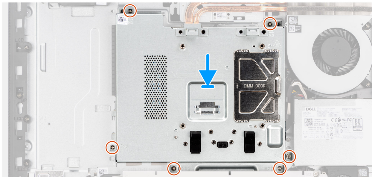
Rysunek 28. Instalowanie osłony płyty głównej
