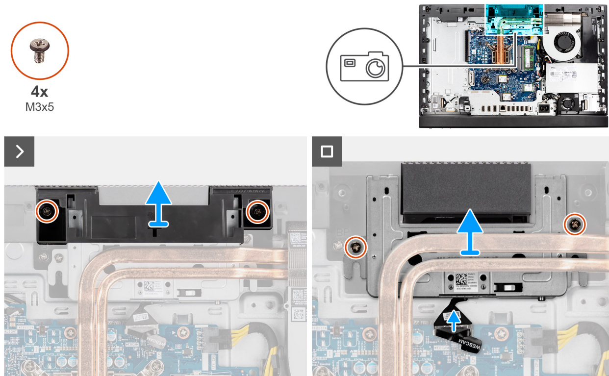
Rysunek 47. Wymontowywanie zestawu wysuwanej kamery
