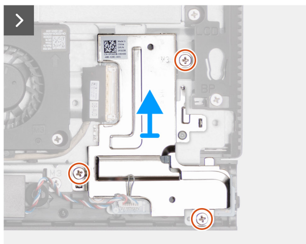
Rysunek 71. Wymontowywanie karty dźwiękowej
