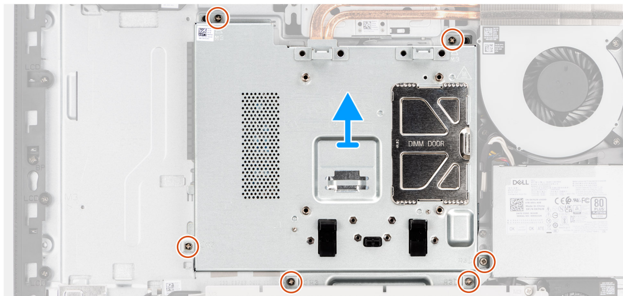
Rysunek 27. Wymontowywanie osłony płyty głównej
