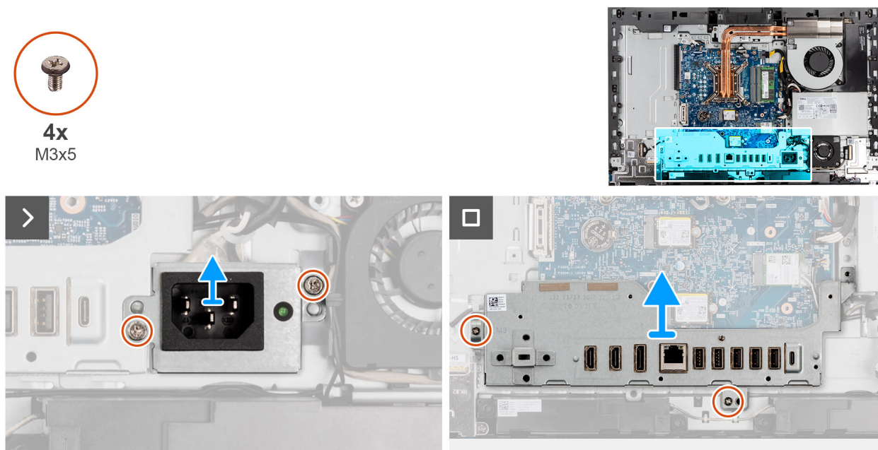
Rysunek 55. Wymontowywanie panelu we/wy
