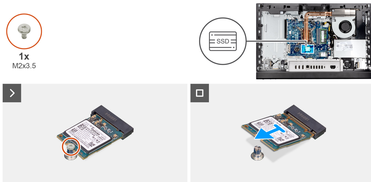
Rysunek 31. Wymontowywanie dysku SSD M.2 2230 z gniazda M.2 nr 0
