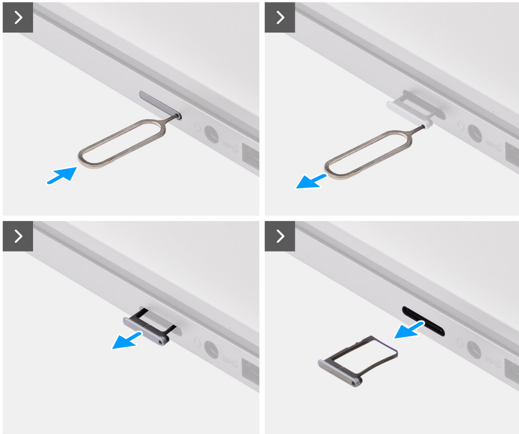
איור 3. הסרת מגש כרטיס ה-SIM מהמחשב
