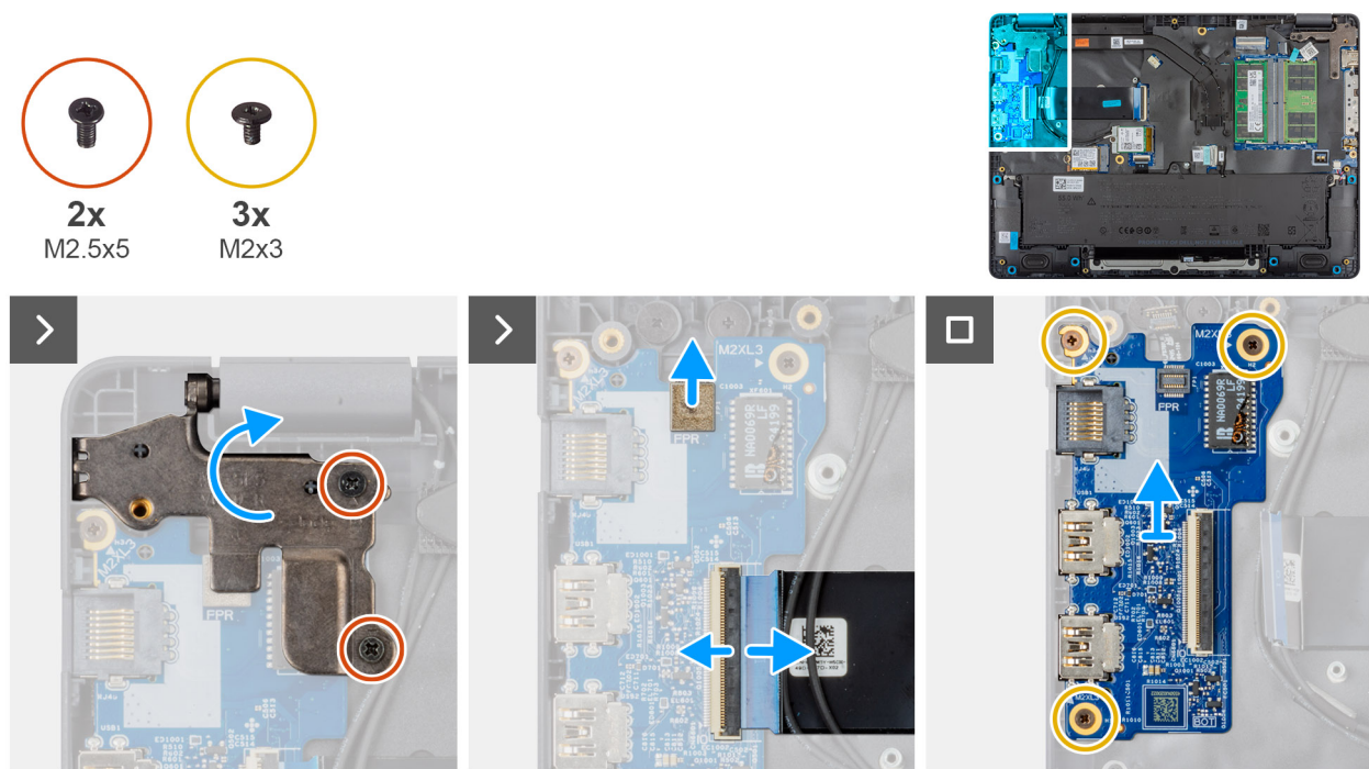
Figura 38. Rimozione della scheda di I/O
