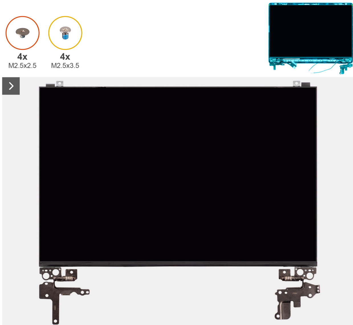
Figura 88. Installazione del gruppo del pannello del display
