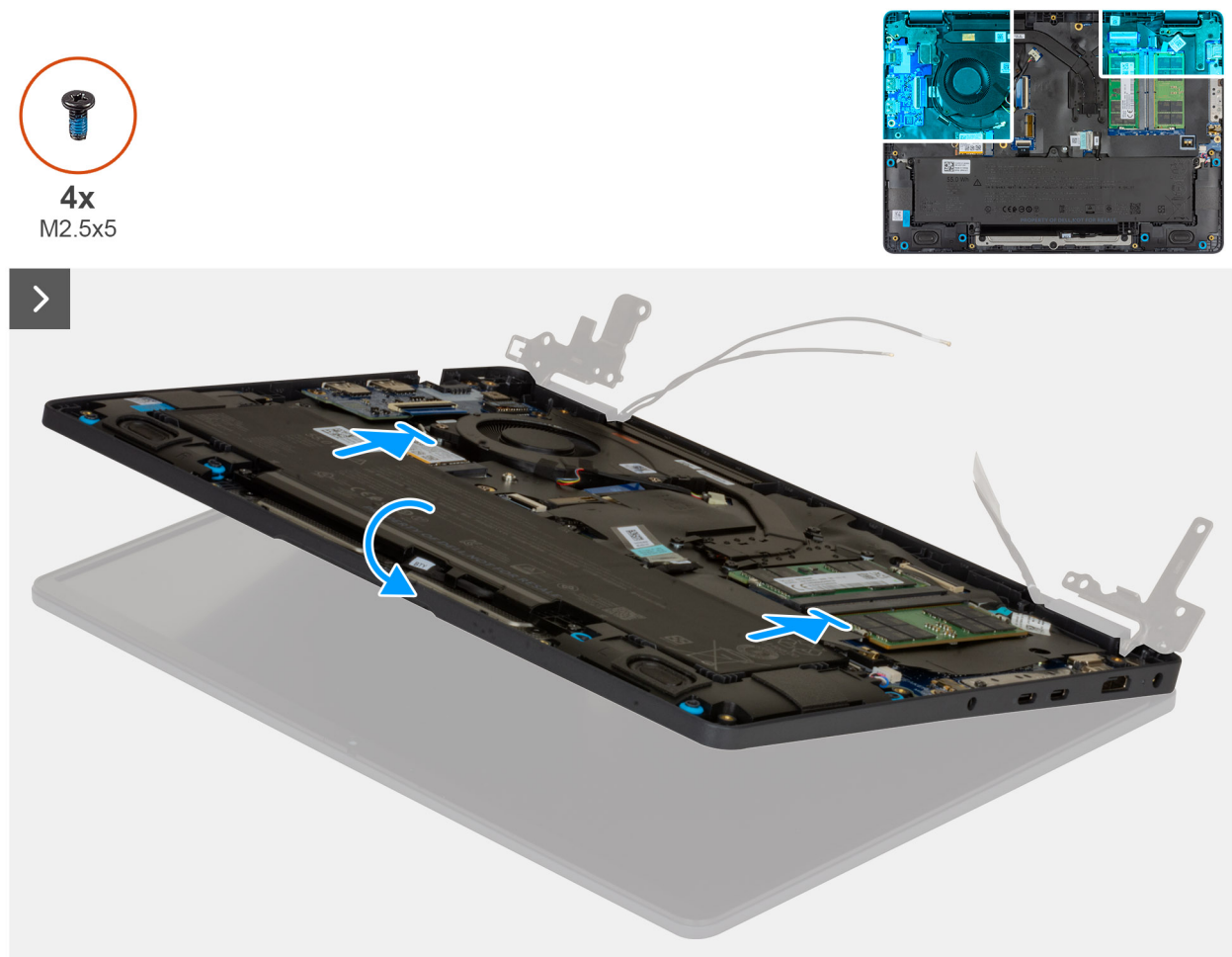
Figura 75. Installazione del gruppo del display
