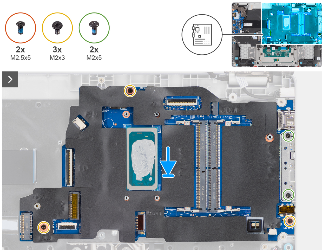
Figura 56. Installazione della scheda di sistema
