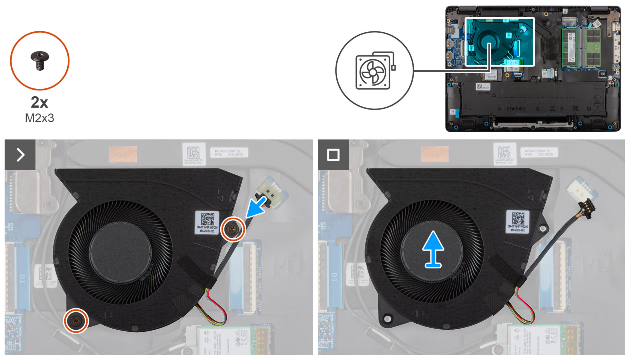
Figura 30. Rimozione della ventola
