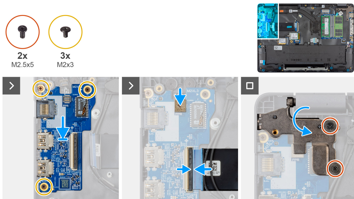
Figura 39. Installazione della scheda di I/O
