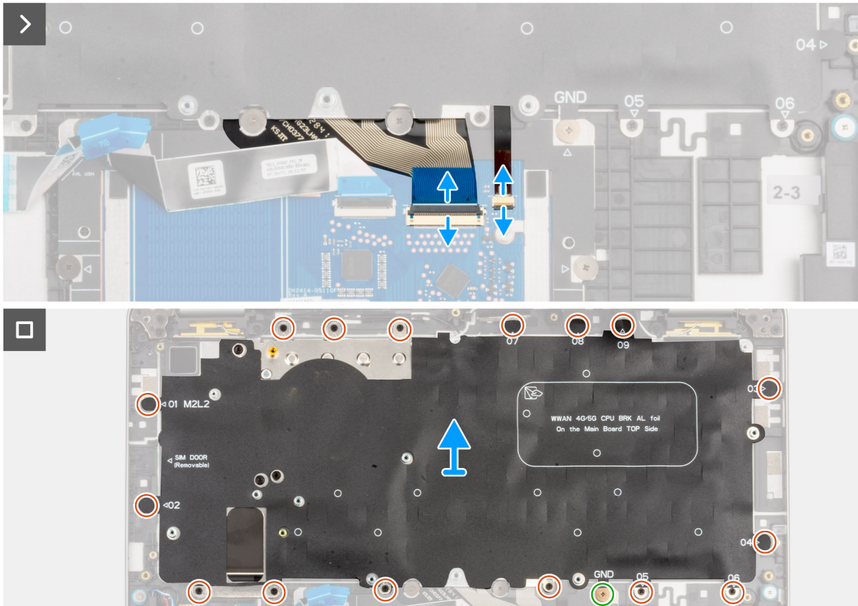
Figure 64. Retrait du clavier
