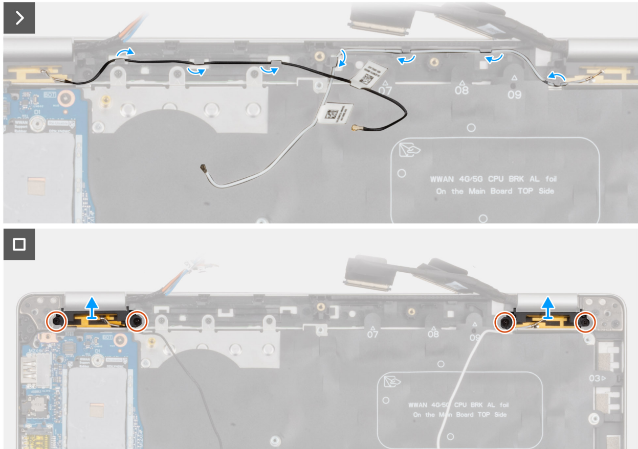
Figure 58. Retrait du module d'antenne sans fil
