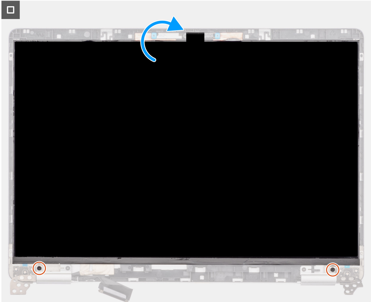
Figure 74. Installation du panneau d'écran
