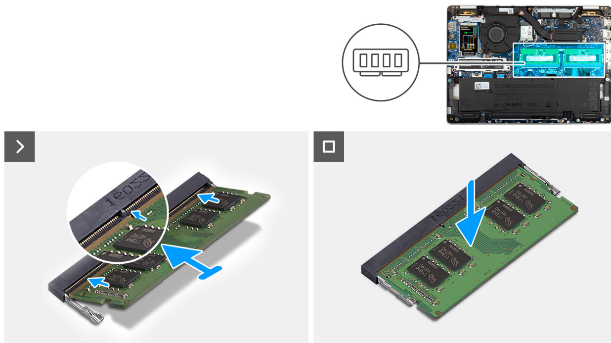
Figure 26. Installation des modules de mémoire
