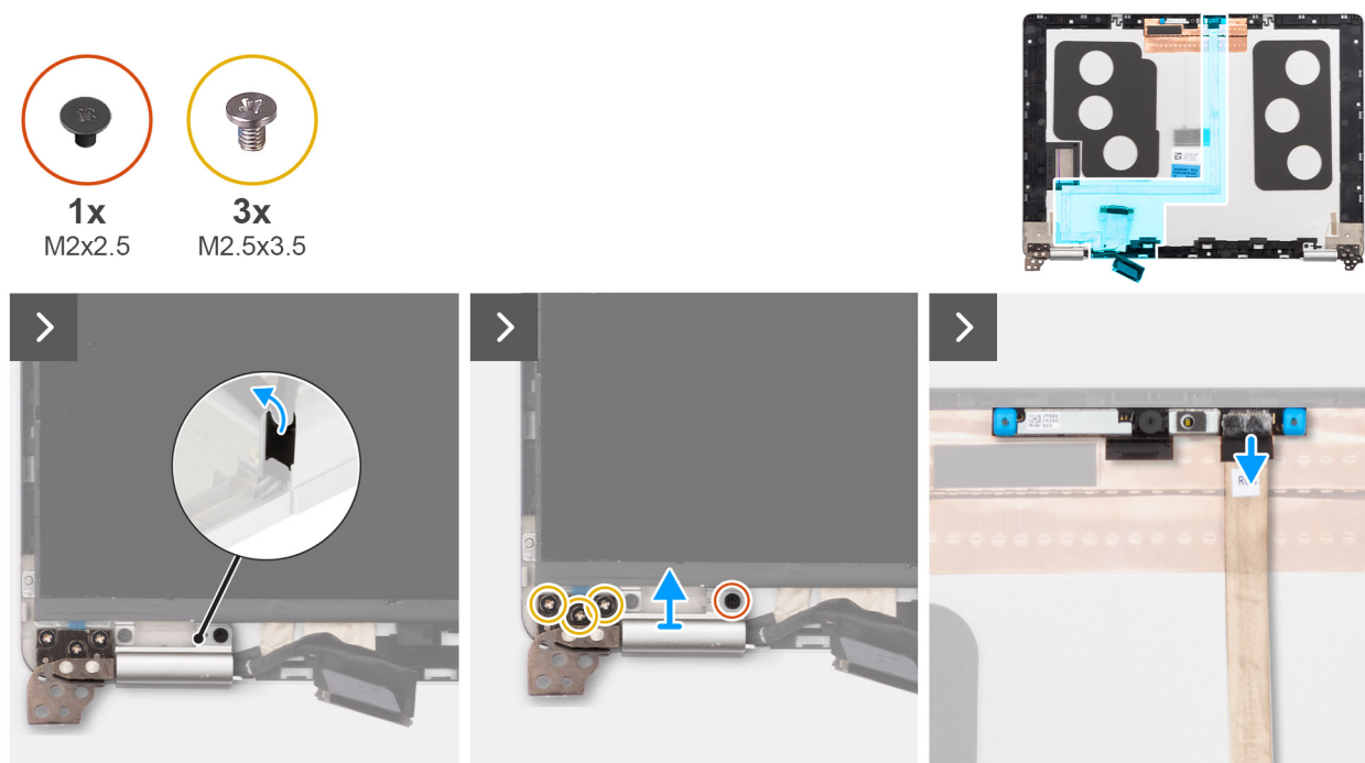
Figure 78. Retrait du câble de l'écran
