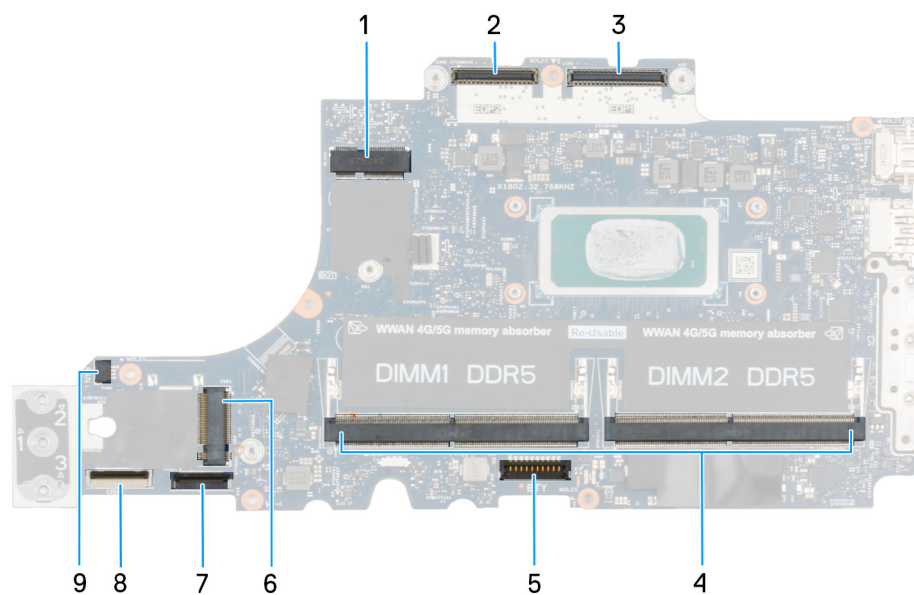
Figure 54. Connecteurs de la carte système
