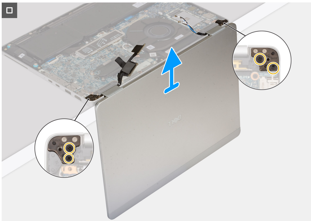
Figure 49. Retrait de l'assemblage d'écran
