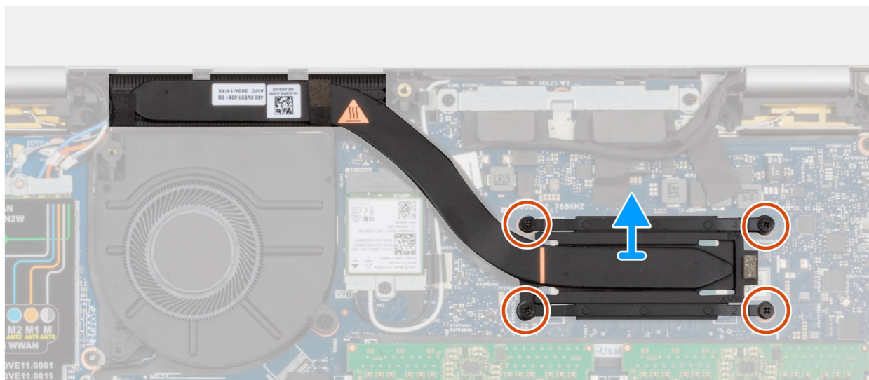
Figure 46. Retrait du dissipateur de chaleur
