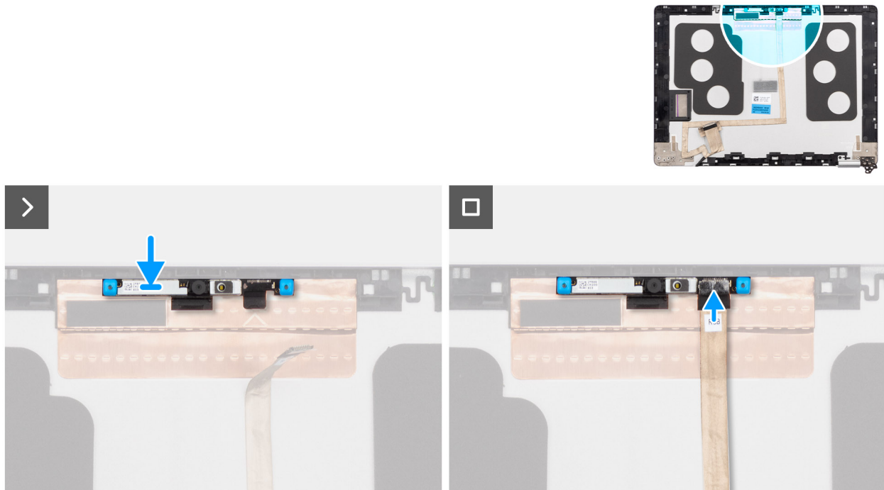
Figure 77. Installation du module de caméra
