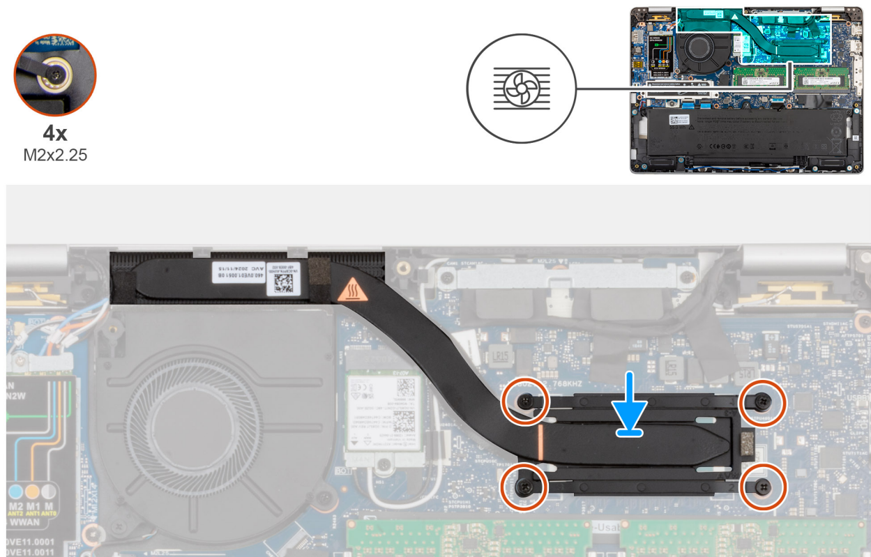
Figure 47. Installation du dissipateur de chaleur
