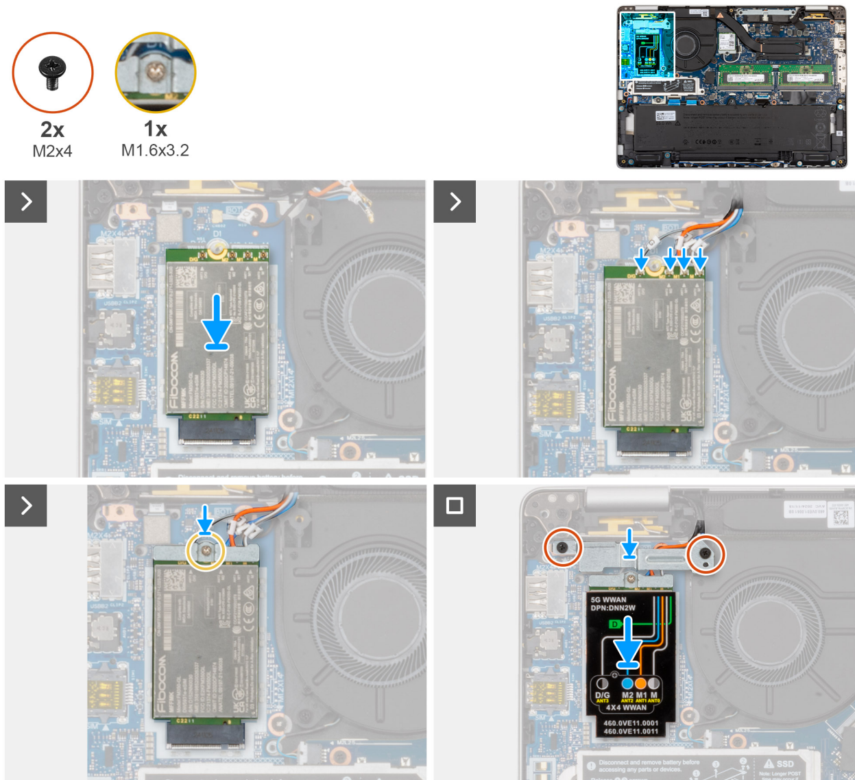
Figure 29. Installation de la carte WWAN 5G
