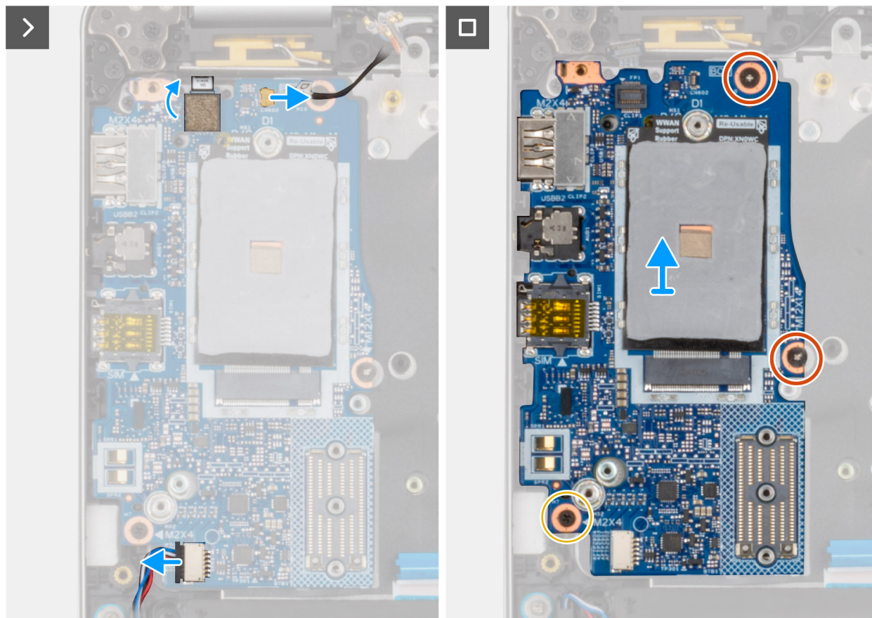
Figure 60. Image : retrait de la carte d'E/S
