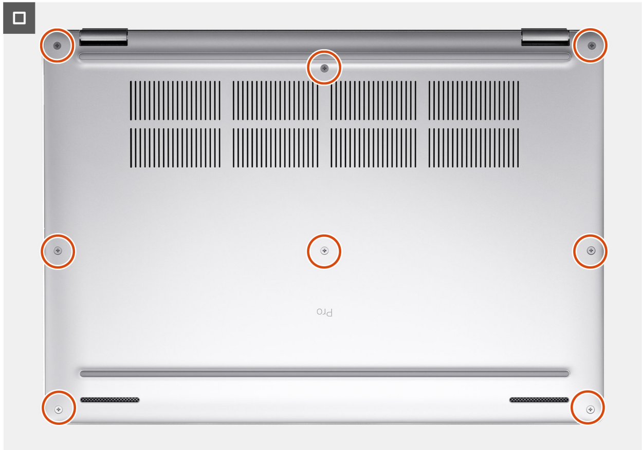
Figure 20. Installation du cache de fond
