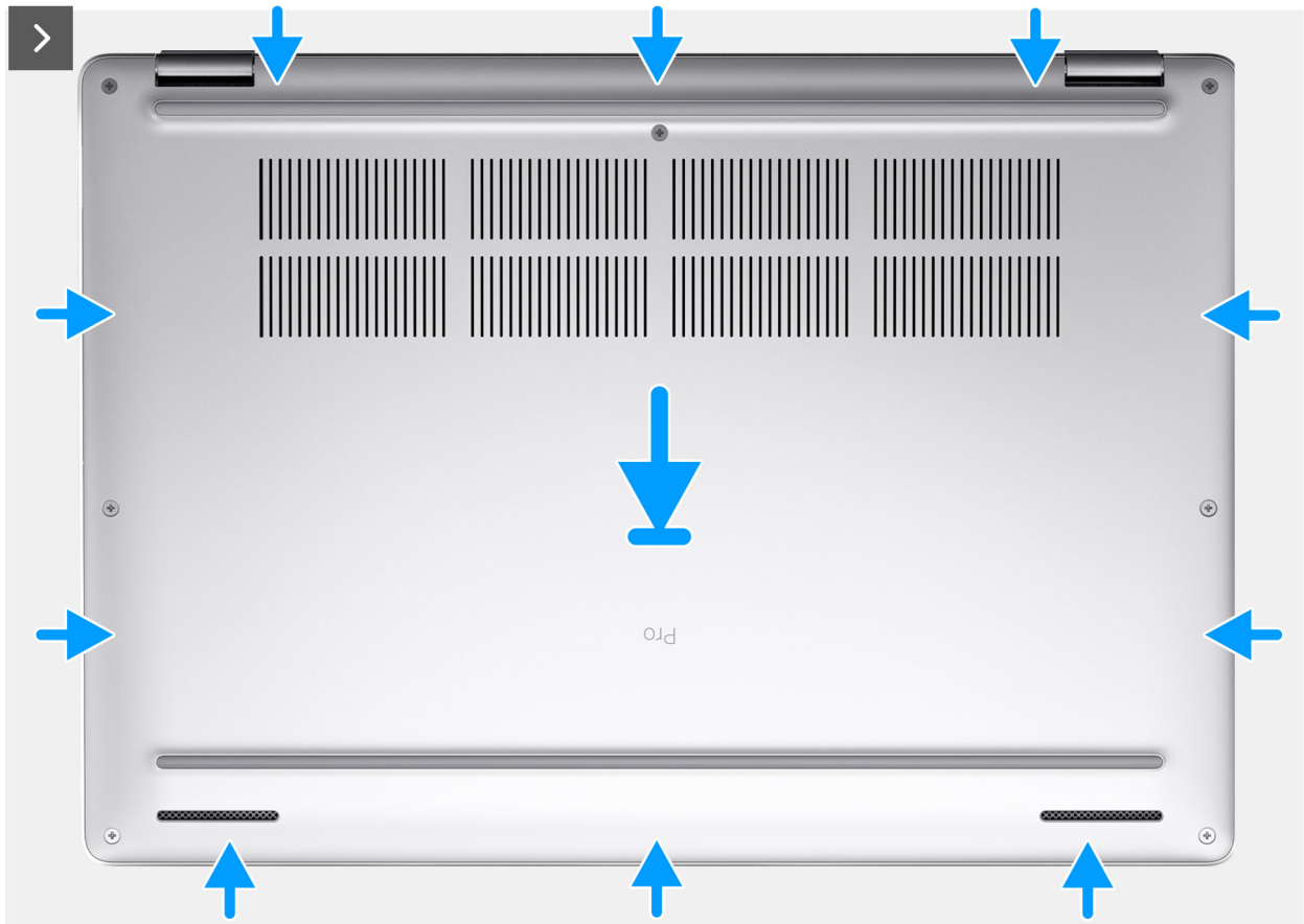
Figure 19. Installation du cache de fond
