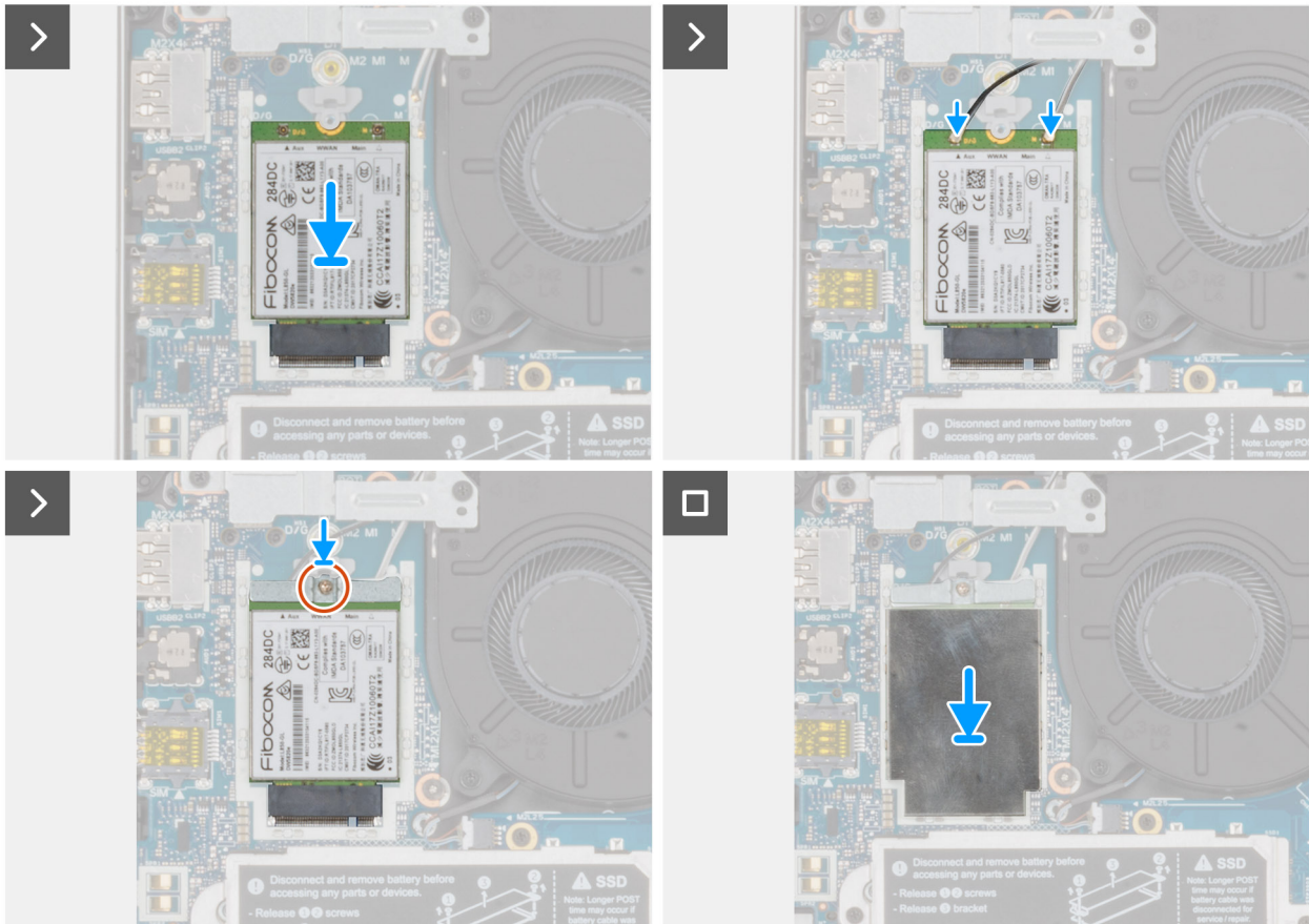
Figure 30. Installation de la carte WWAN 5G
