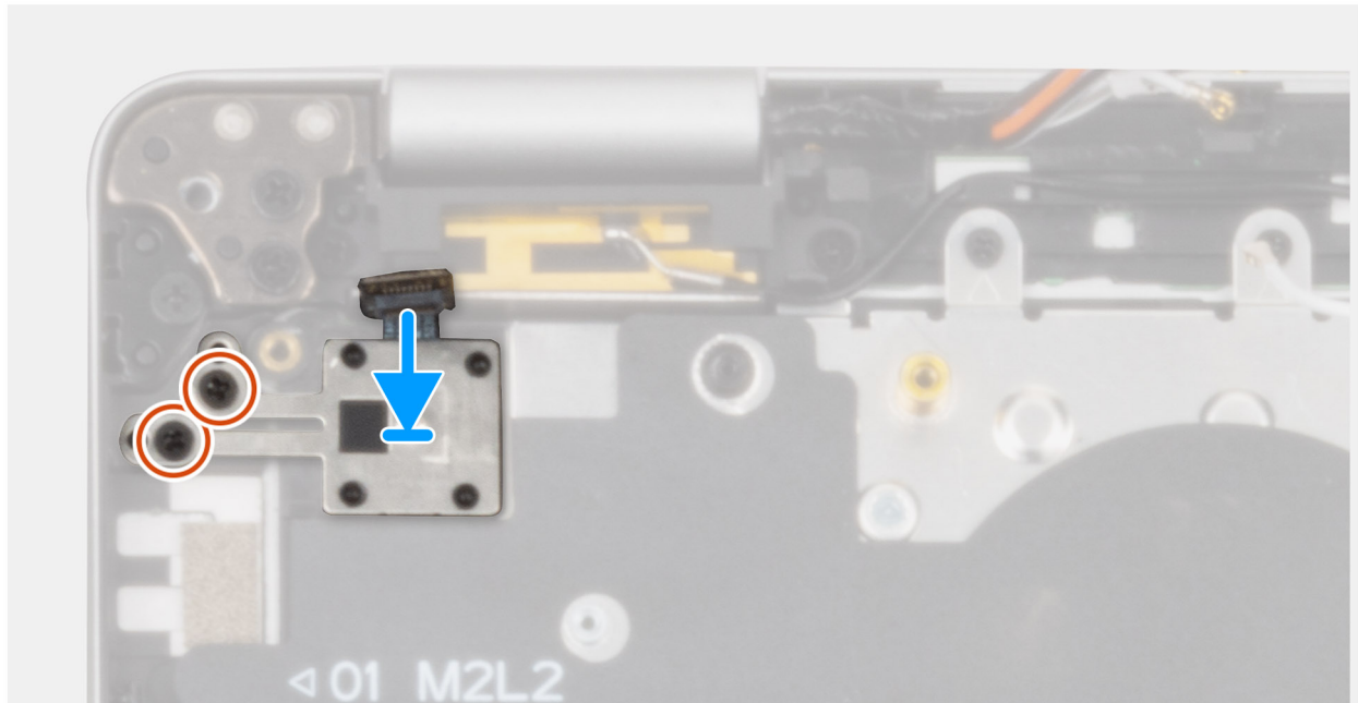
Figure 63. Installation du bouton d'alimentation avec lecteur d'empreintes digitales (en option)
