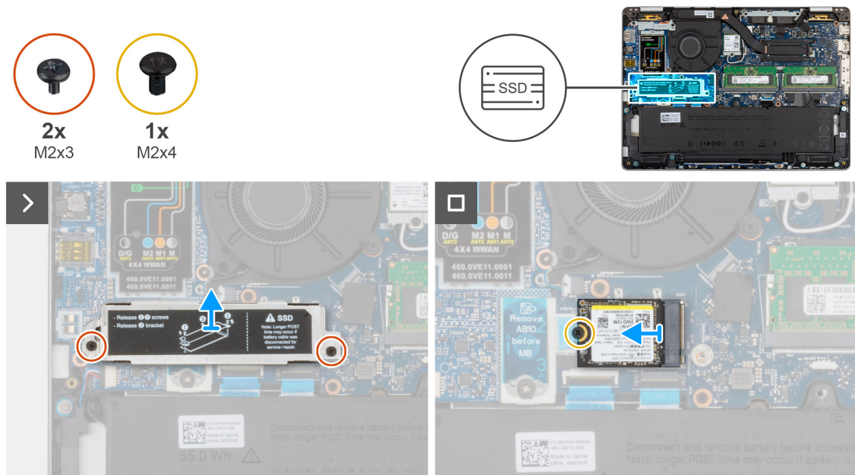
Figure 33. Retrait du disque SSD M.2 2230
