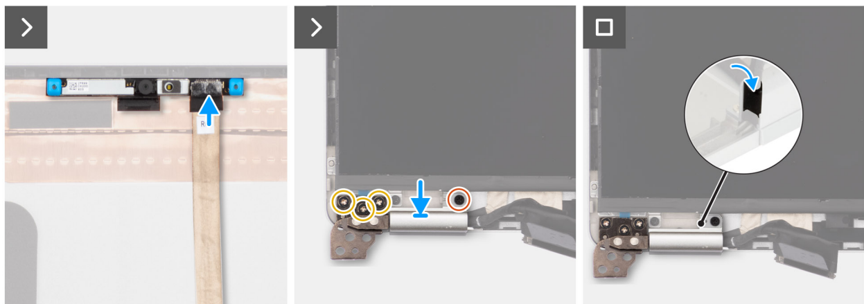
Figure 81. Installation du câble d'écran
