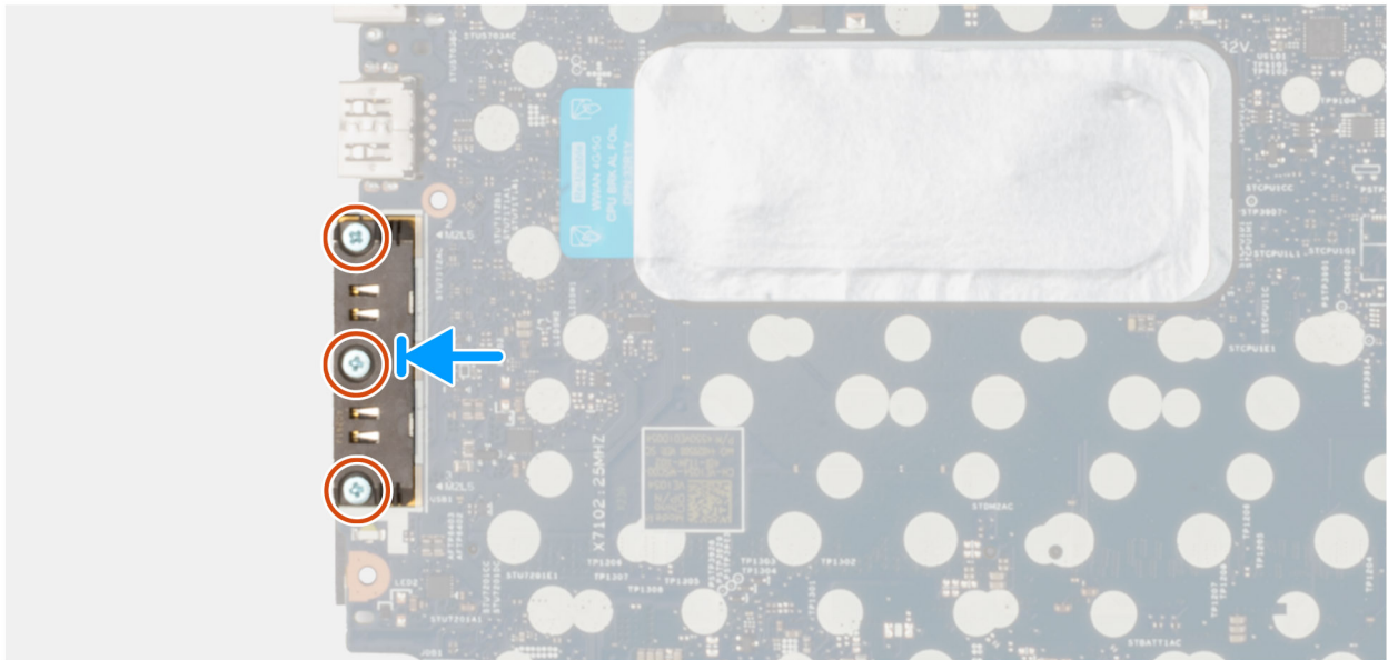
Figure 57. Installation du module de connecteur USB-C
