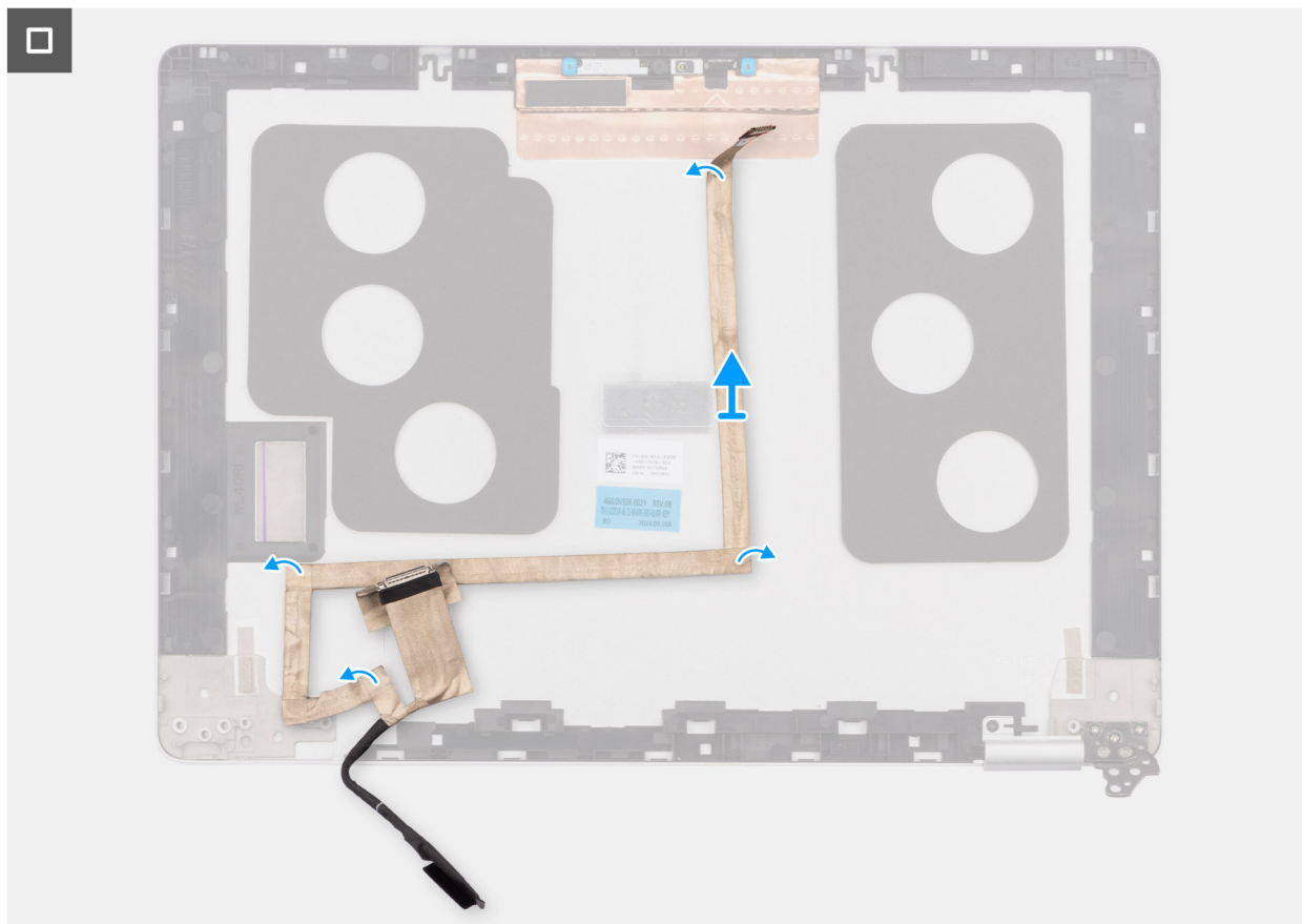
Figure 79. Retrait du câble de l'écran
