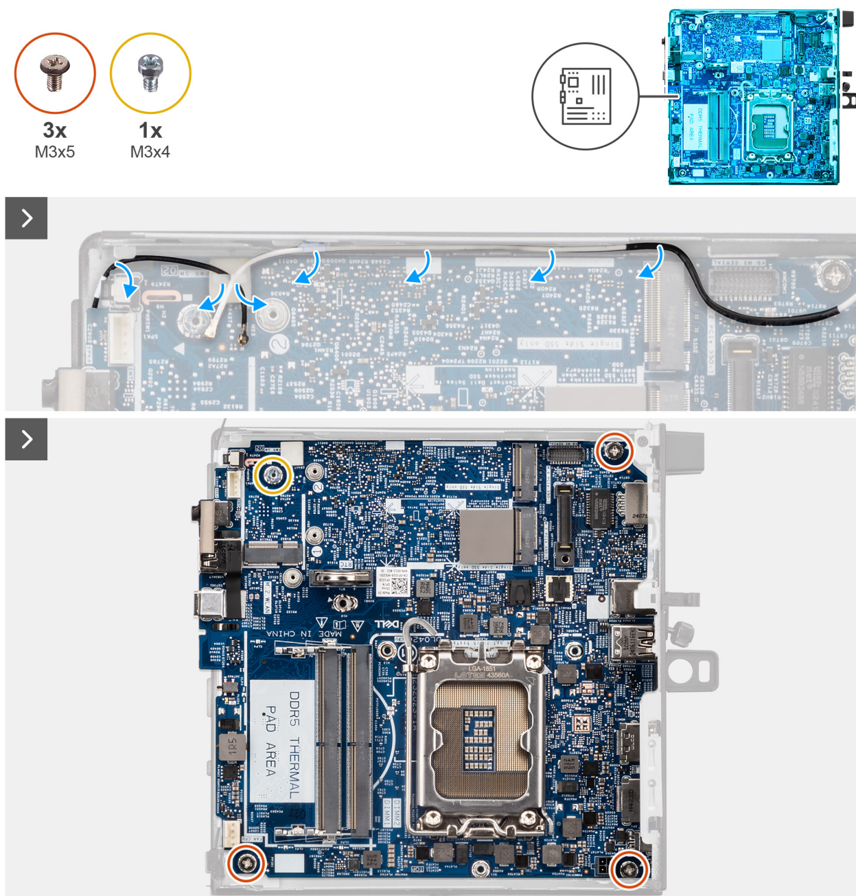
Obrázek 75. Demontáž základní desky
