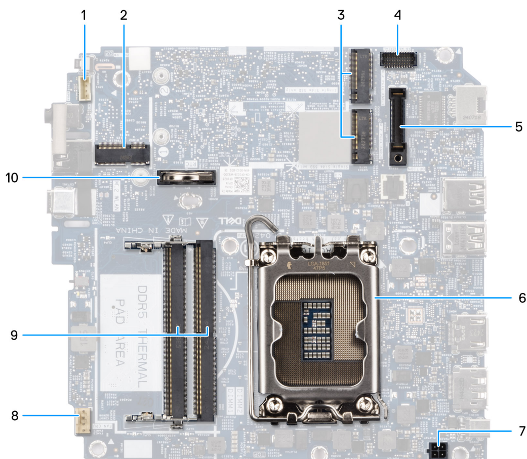
Obrázek 74. Konektory základní desky
