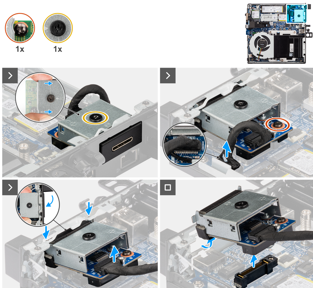
Obrázek 53. Demontáž modulu portu PS2
