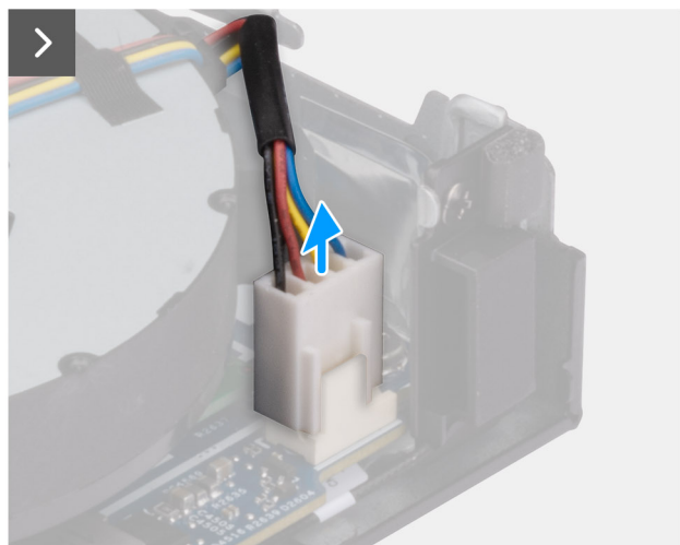
Obrázek 28. Demontáž ventilátoru
