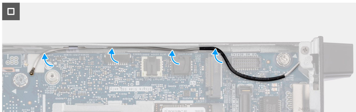
Obrázek 69. Montáž anténního modulu (bílý kabel)
