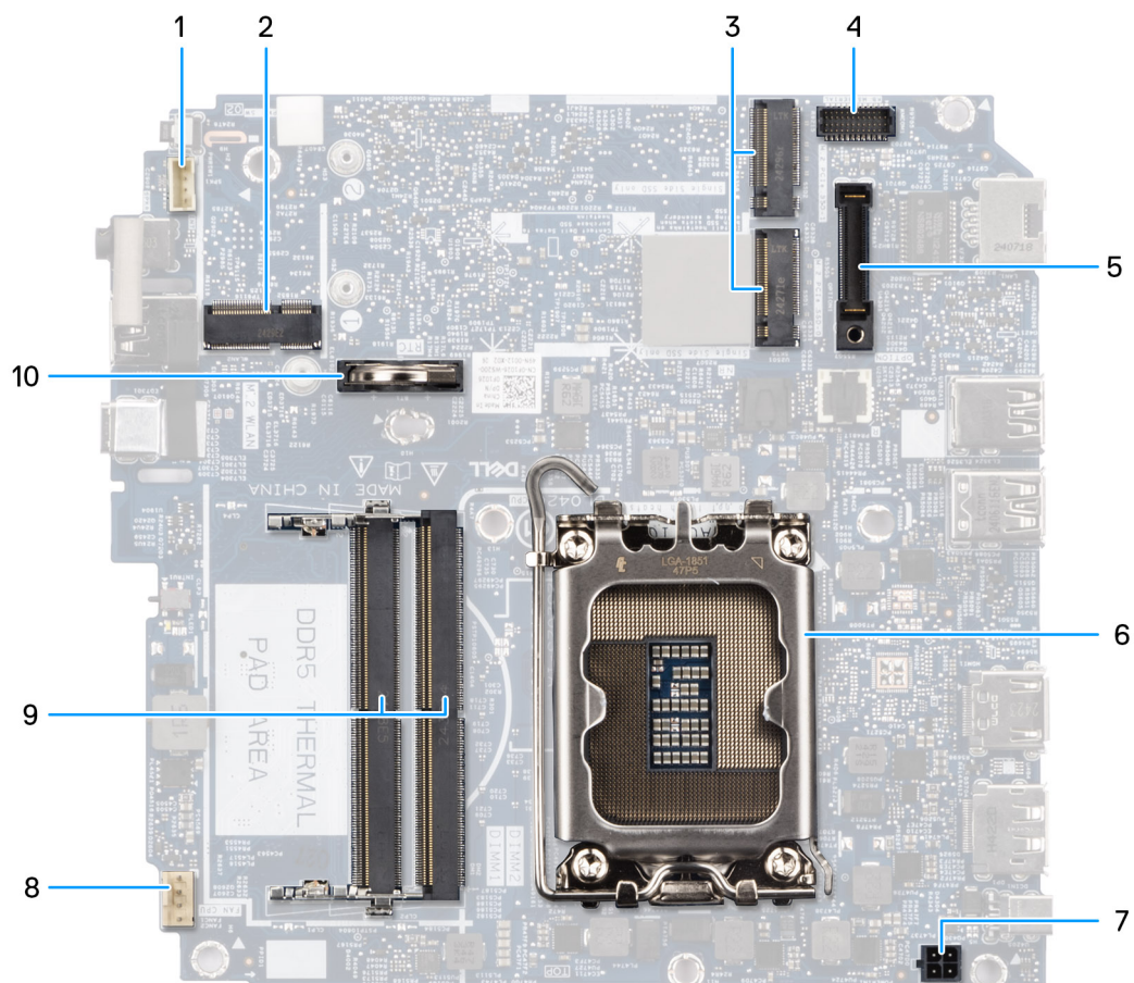
Obrázek 77. Konektory základní desky
