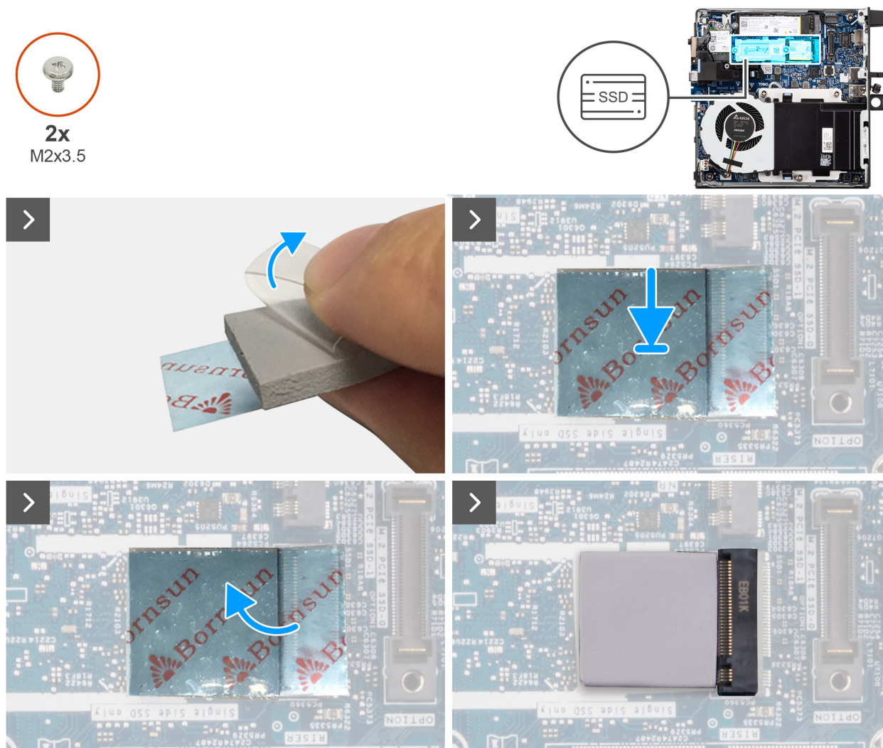
Obrázek 17. Montáž disku SSD 2230
