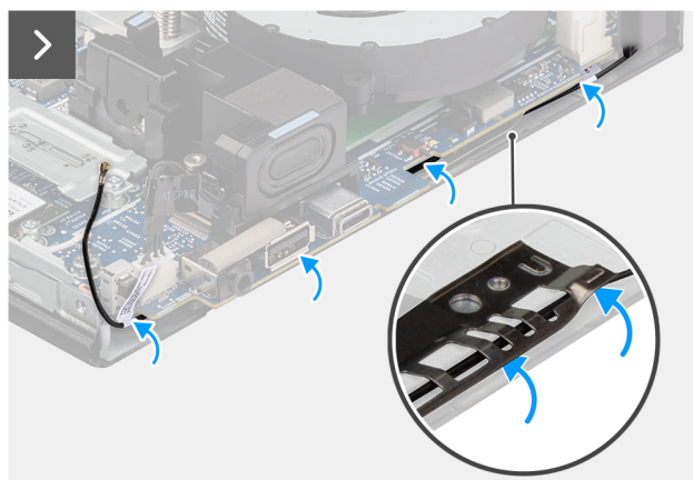
Obrázek 65. Montáž anténního modulu (černý kabel)
