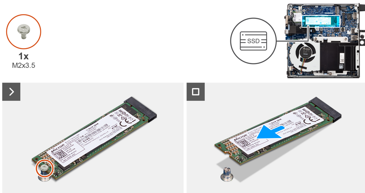
Obrázek 19. Demontáž disku SSD M.2 2280
