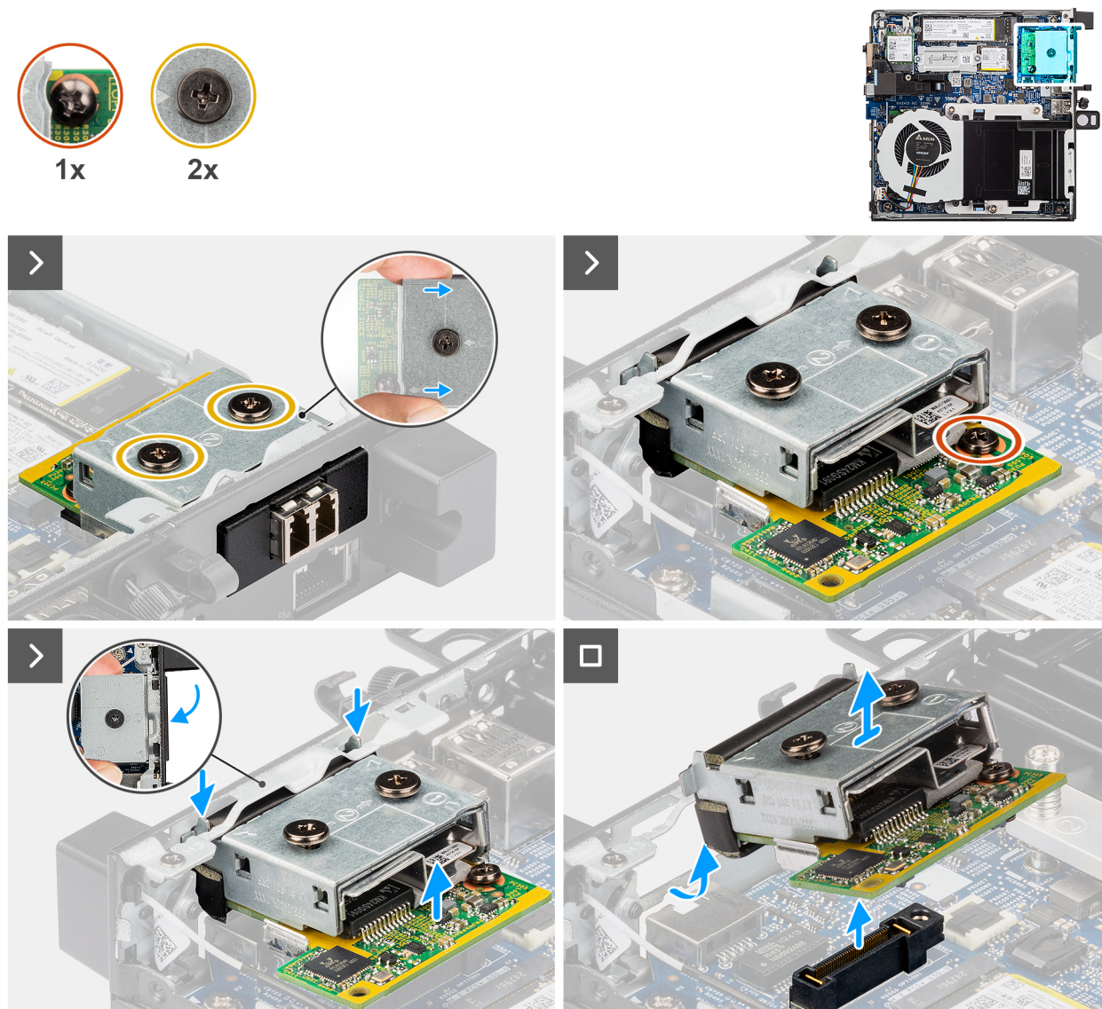
Obrázek 59. Demontáž modulu optického portu
