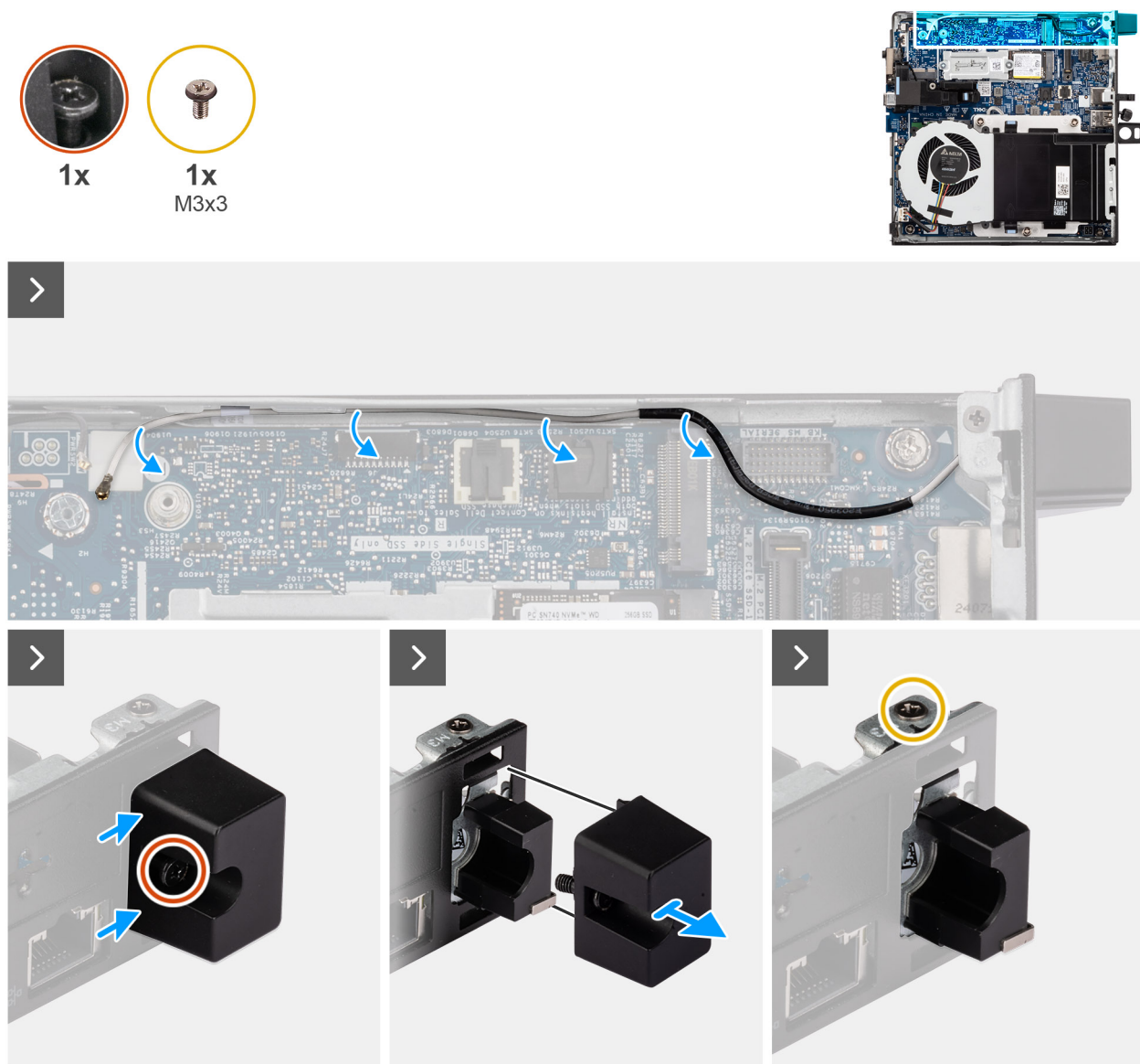
Obrázek 66. Demontáž anténního modulu (bílý kabel)
