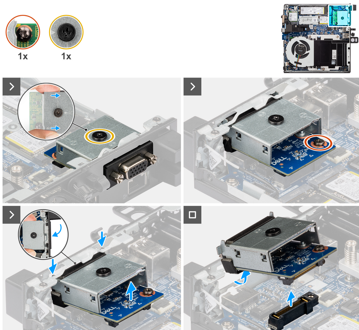
Obrázek 50. Demontáž modulu portu VGA
