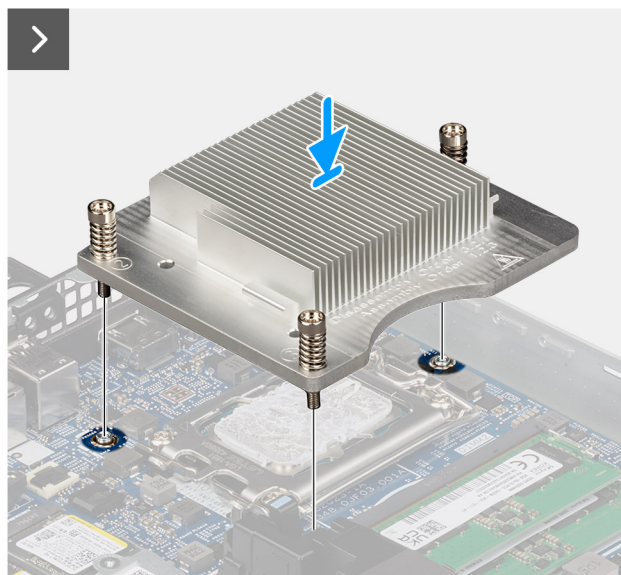
Obrázek 63. Montáž chladiče
