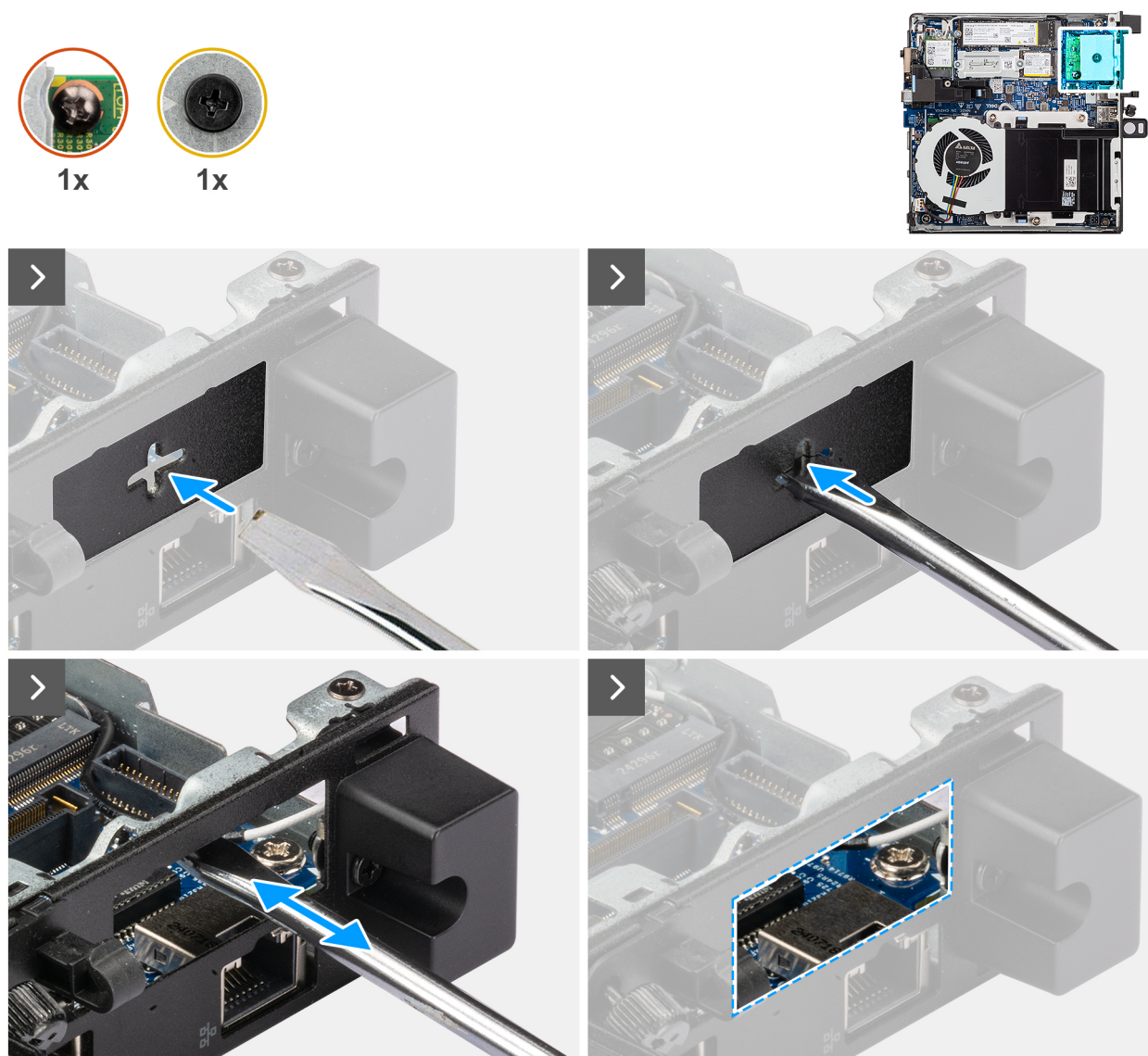
Obrázek 48. Montáž modulu portu HDMI
