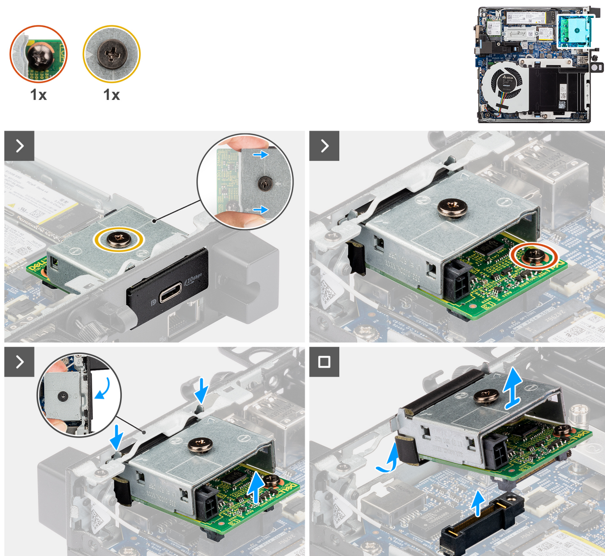
Obrázek 41. Demontáž modulu portu USB Type-C
