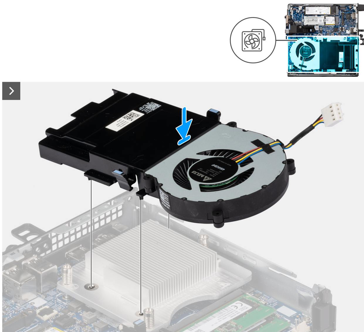
Obrázek 30. Montáž ventilátoru
