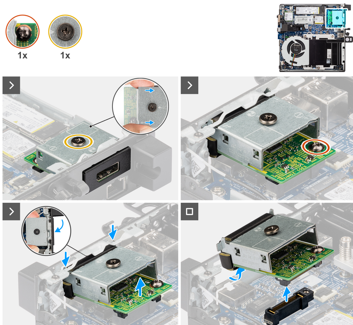
Obrázek 44. Demontáž modulu DisplayPort
