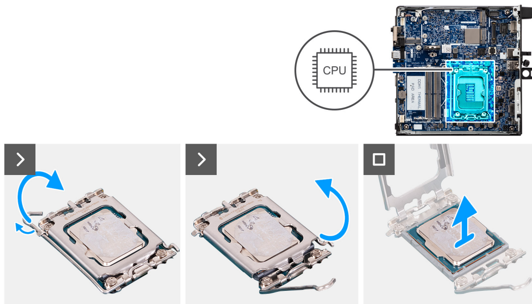
Obrázek 70. Demontáž procesoru
