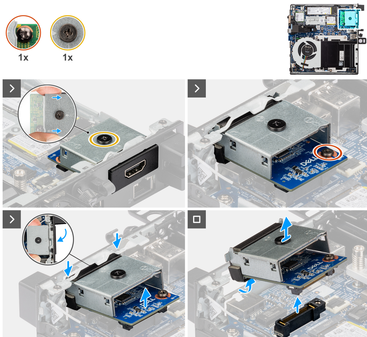
Obrázek 47. Demontáž modulu portu HDMI
