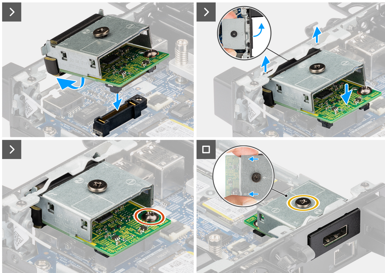
Obrázek 46. Montáž modulu DisplayPort
