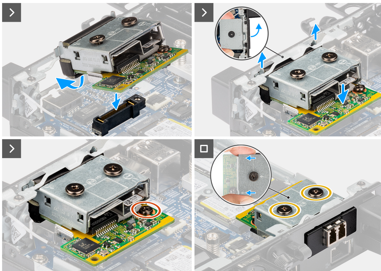
Obrázek 61. Montáž modulu optického portu
