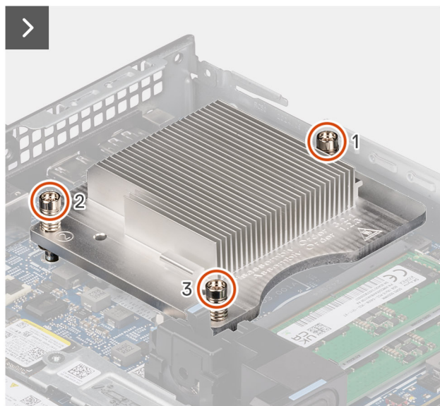
Obrázek 62. Demontáž chladiče
