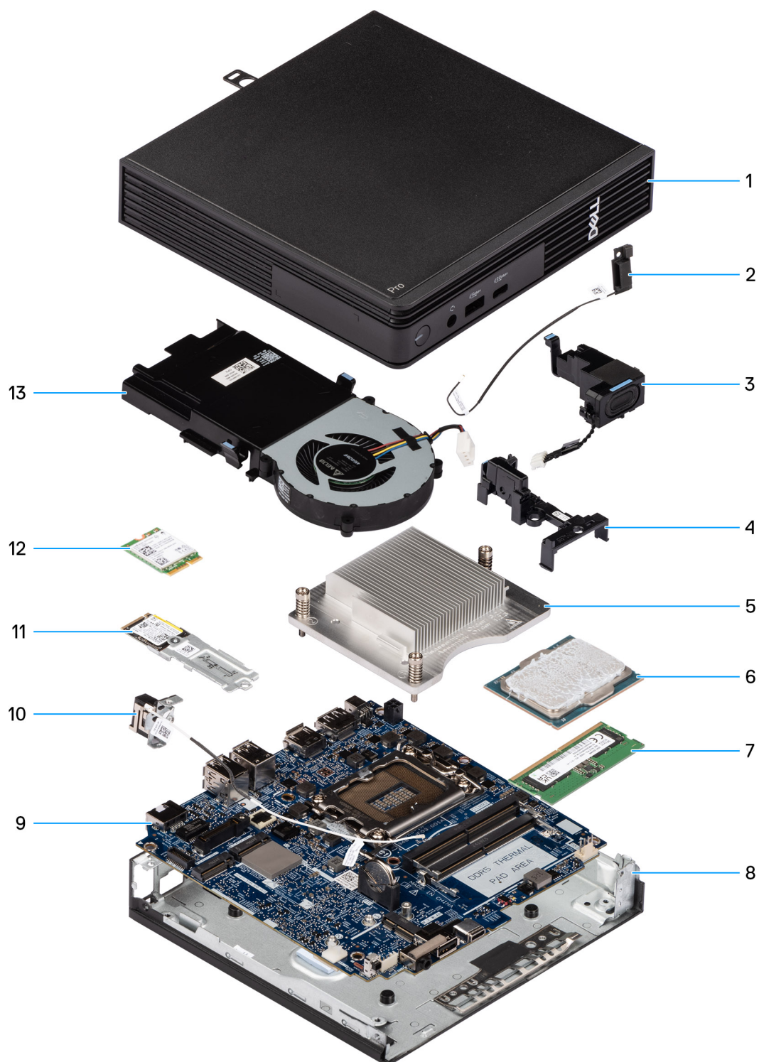
Obrázek 9. Hlavní komponenty počítače Dell Pro Micro QCM1250
