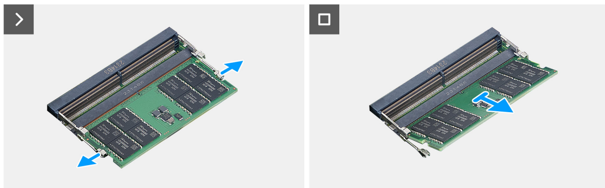
Obrázek 32. Vyjmutí paměťového modulu
