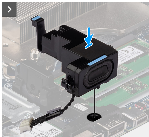
Obrázek 15. Montáž reproduktoru
