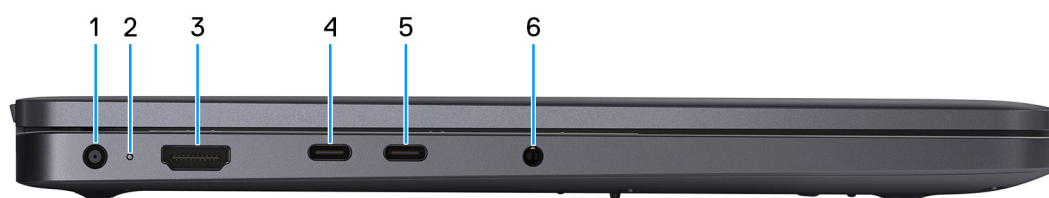
Obrázek 2. Pohled zleva
