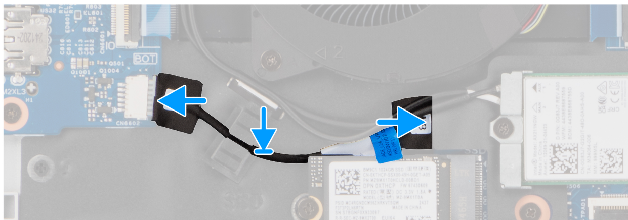
Obrázek 37. Montáž kabelu vPro
