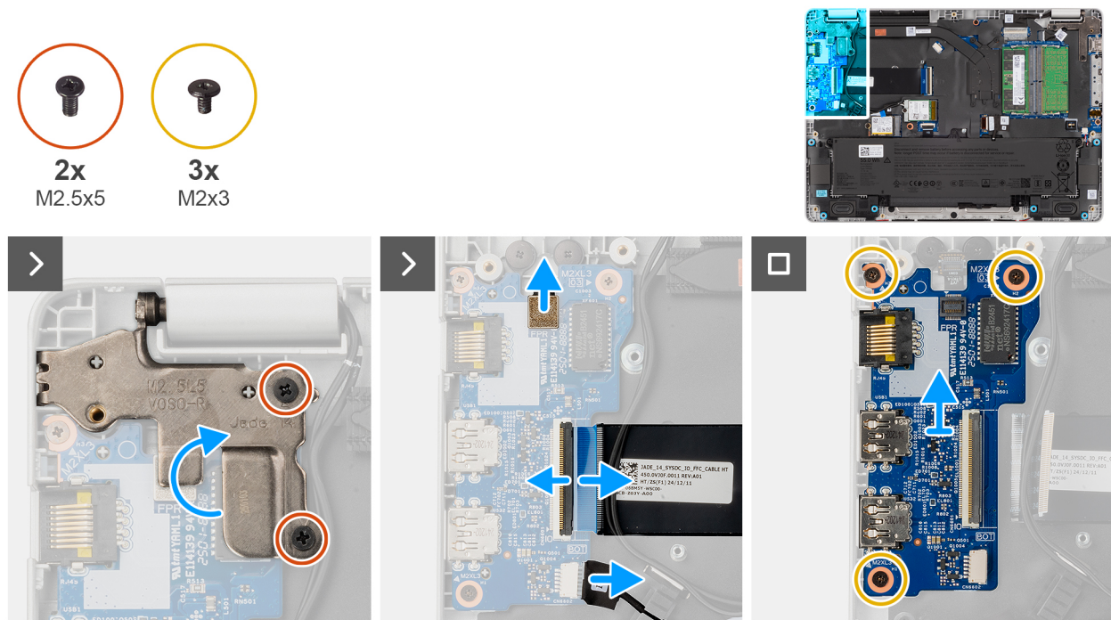
Obrázek 40. Demontáž desky I/O
