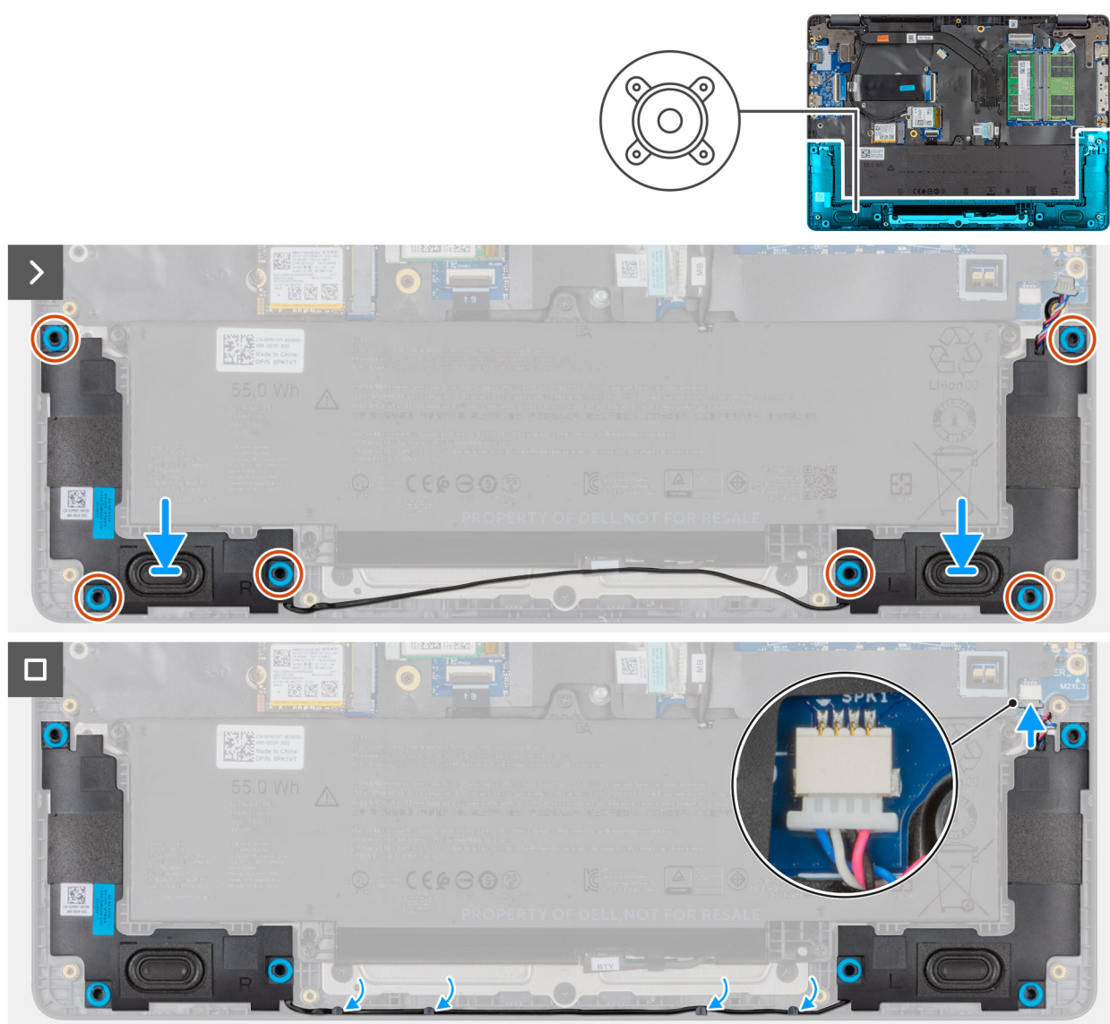
Obrázek 28. Montáž reproduktorů
