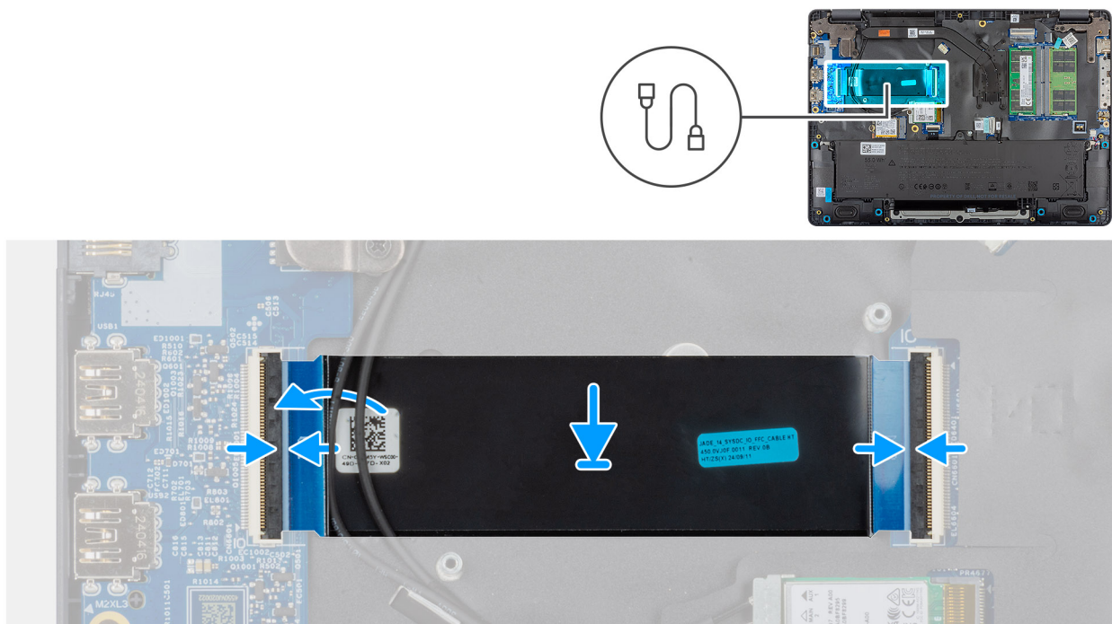
Obrázek 43. Montáž kabelu FPC desky I/O
