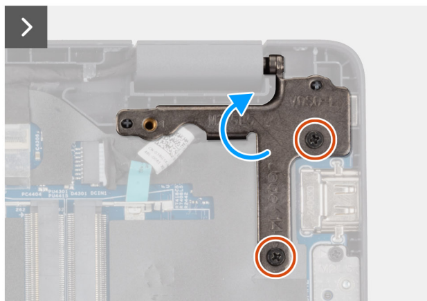
Obrázek 32. Demontáž portu napájecího adaptéru
