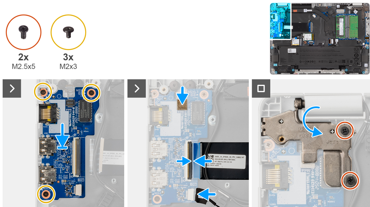
Obrázek 41. Vložení desky I/O
