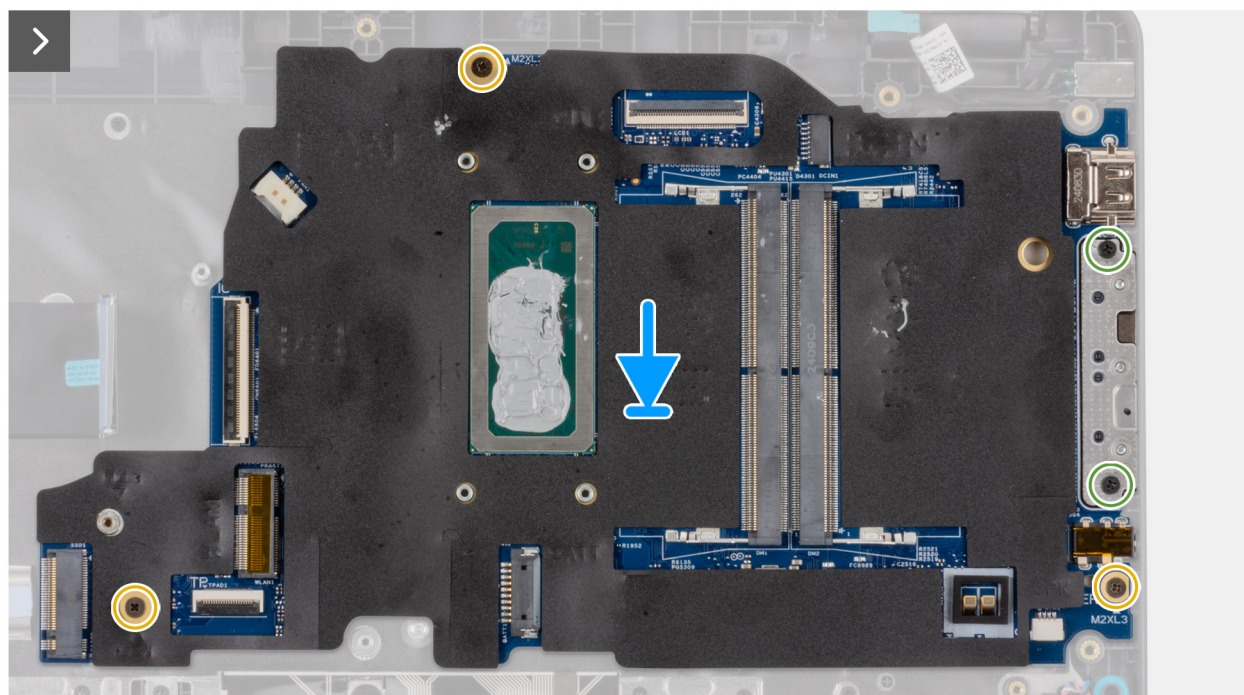
Obrázek 50. Montáž základní desky
