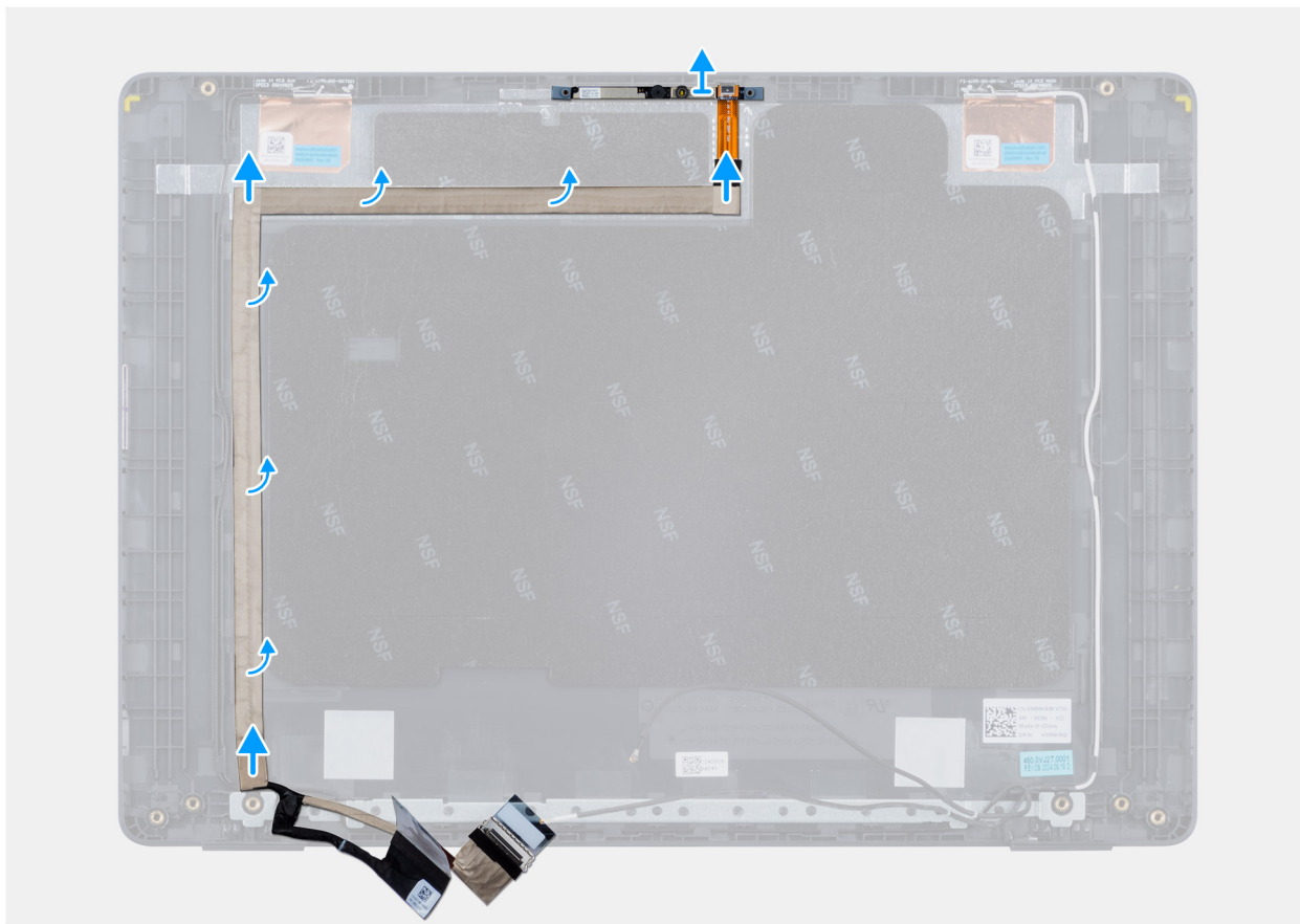
Obrázek 94. Vyjmutí kabelu eDP
