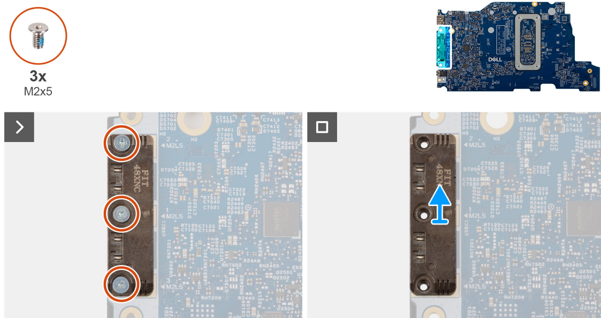
Obrázek 58. Demontáž modulu USB Type-C
