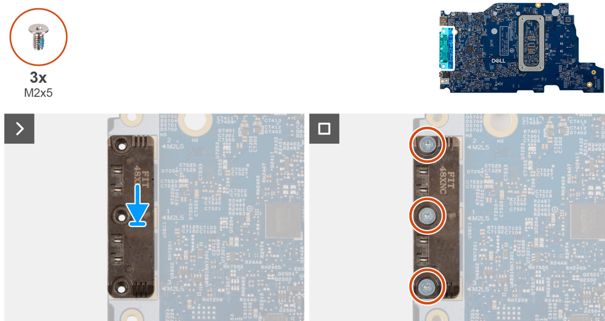
Obrázek 59. Montáž modulu USB Type-C
