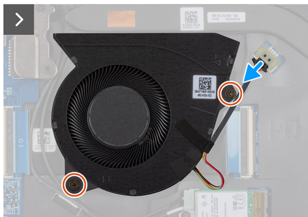
Obrázek 30. Demontáž ventilátoru
