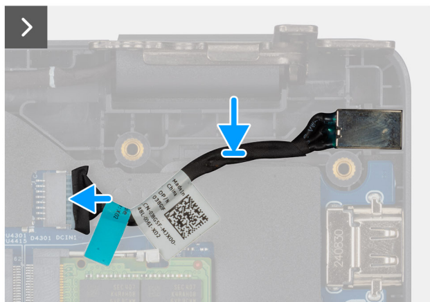
Obrázek 33. Montáž portu napájecího adaptéru
