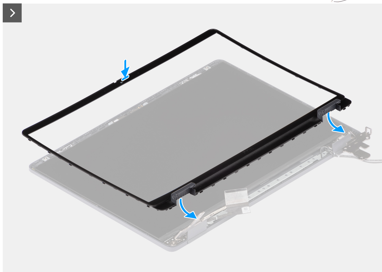
Obrázek 82. Montáž čelního krytu displeje
