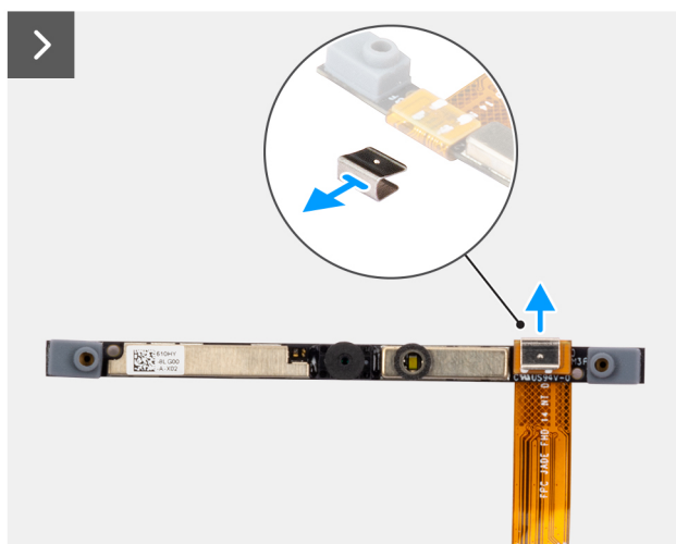
Obrázek 92. Demontáž kamery
