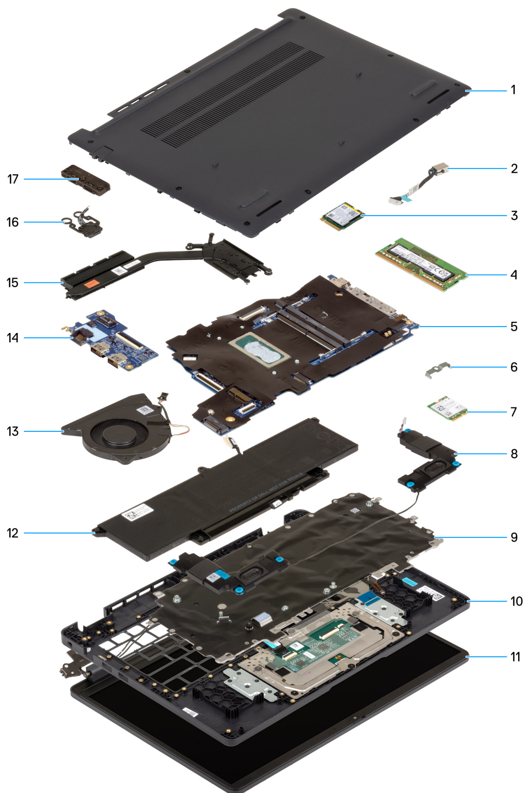
Obrázek 10. Hlavní součásti systému / plné zobrazení
