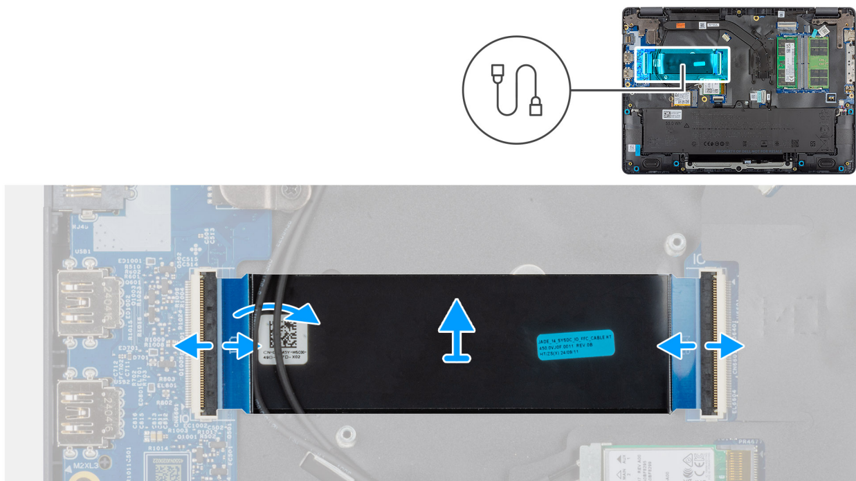
Obrázek 42. Demontáž kabelu FPC desky I/O
