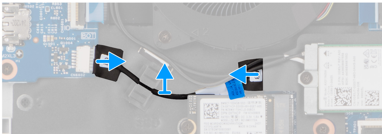
Obrázek 36. Demontáž kabelu vPro
