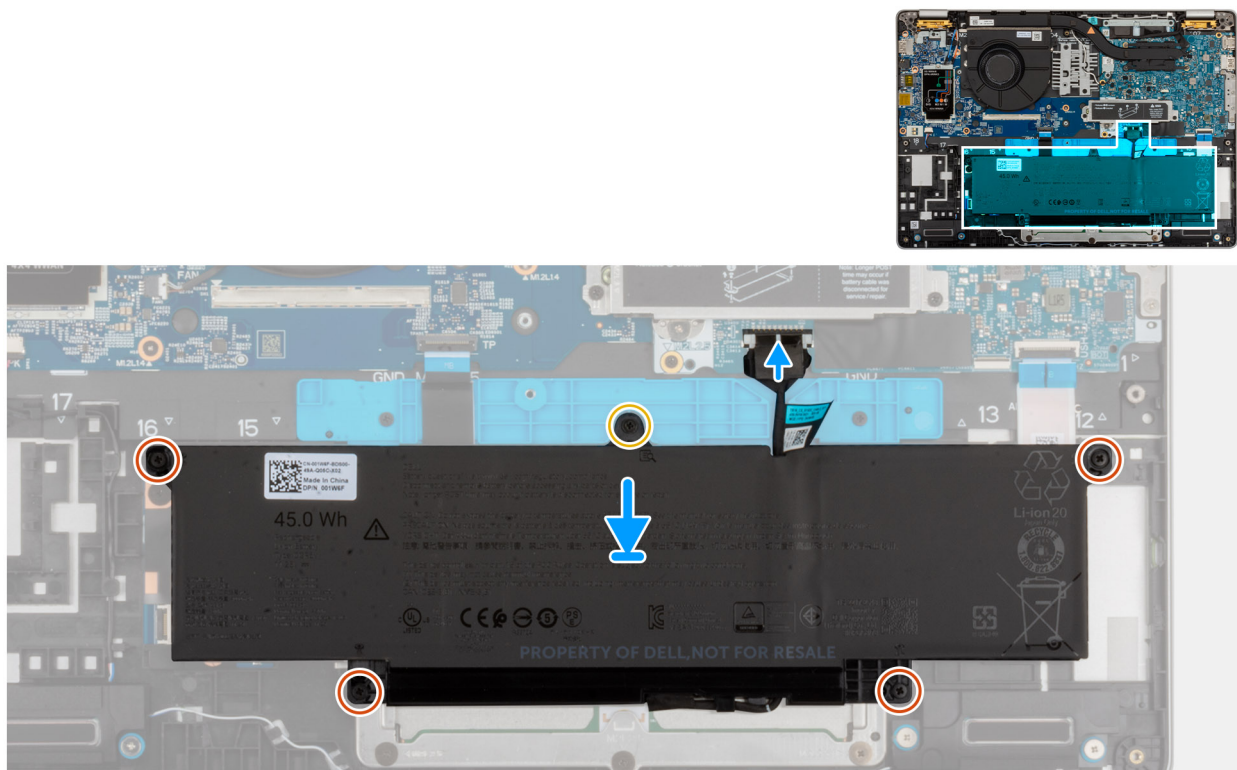
Ilustración 16. Connecting the battery cable
