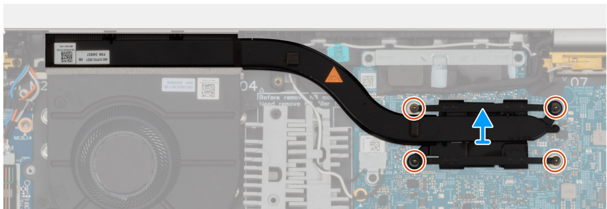
Ilustración 45. Extracción del disipador de calor
