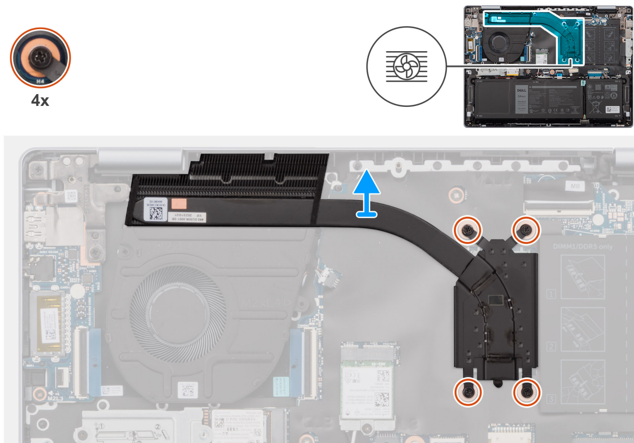
Ilustración 29. Extracción del disipador de calor
