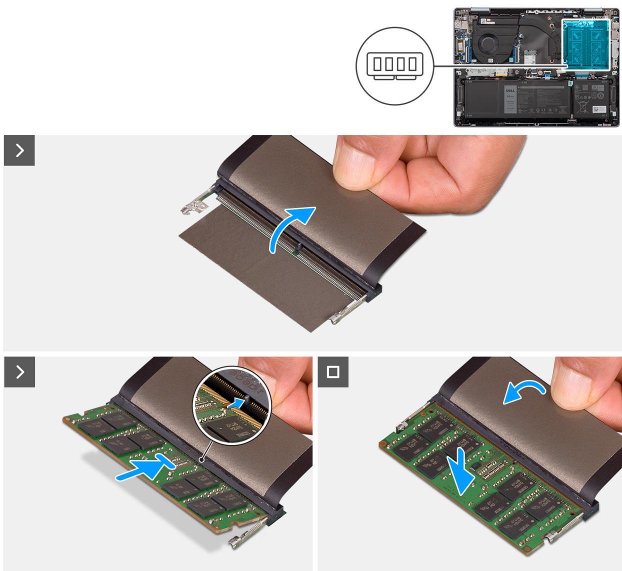
Ilustración 18. Instalación del módulo de memoria
