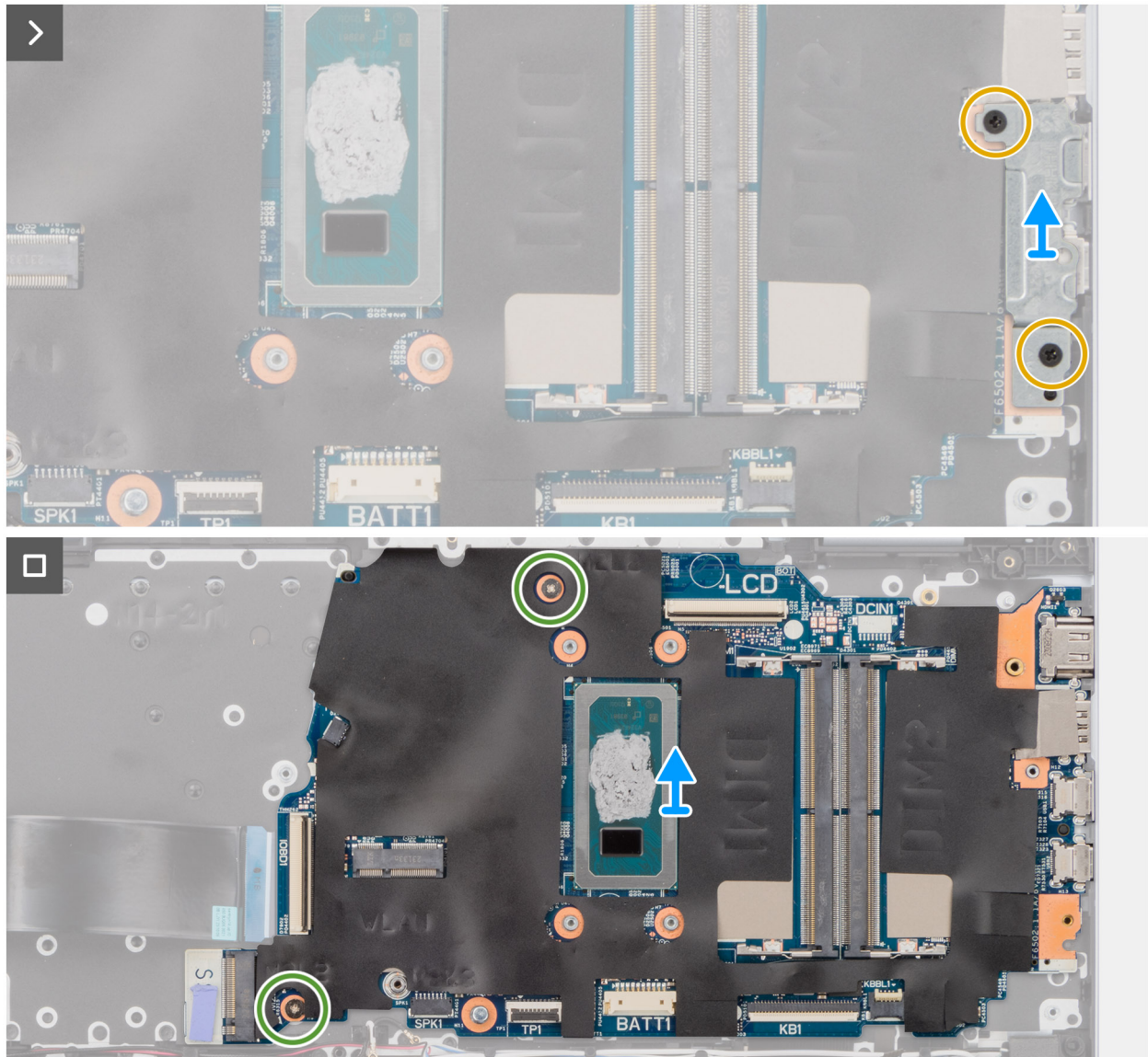
Ilustración 48. Extracción del soporte de USB-C y la tarjeta madre
