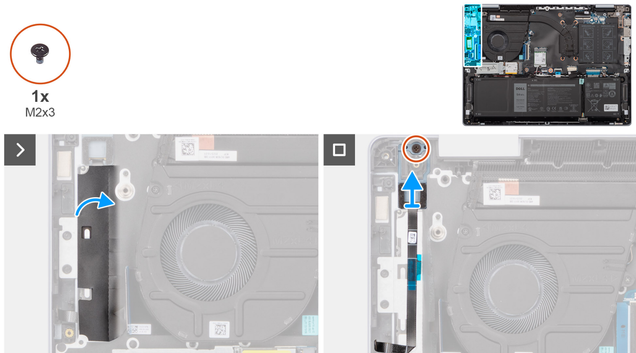
Ilustración 35. Extracción del botón de encendido con lector de huellas digitales
