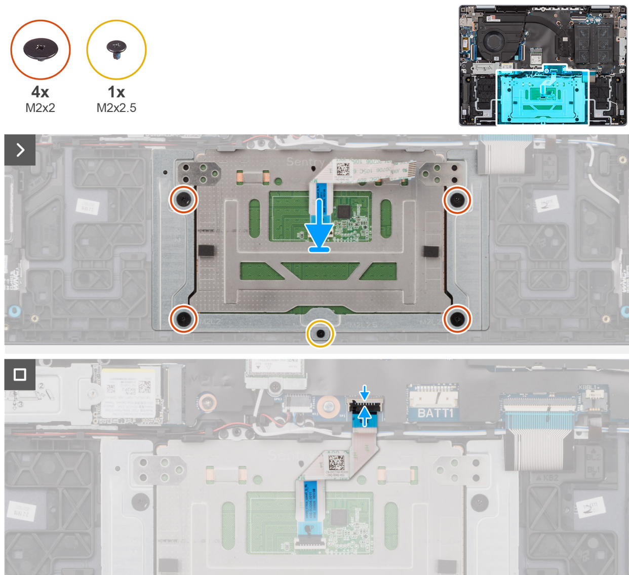
Ilustración 38. Instalación del panel táctil
