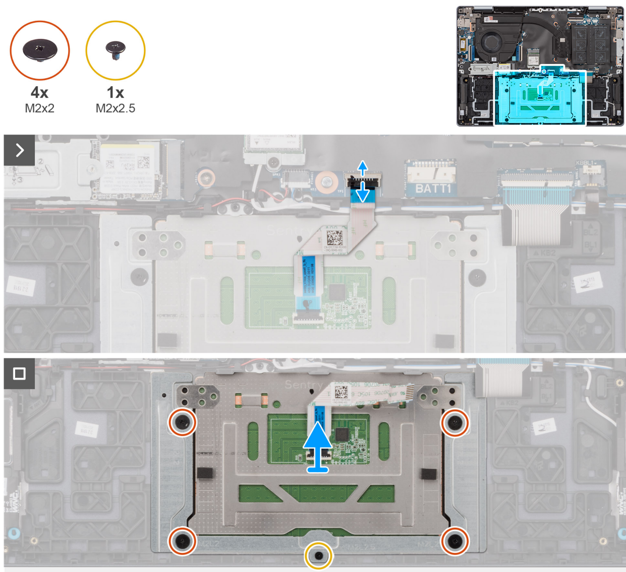
Ilustración 37. Extracción del panel táctil
