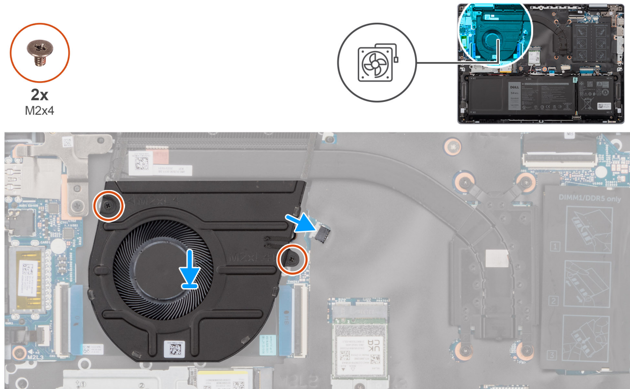
Ilustración 24. Instalación del ventilador
