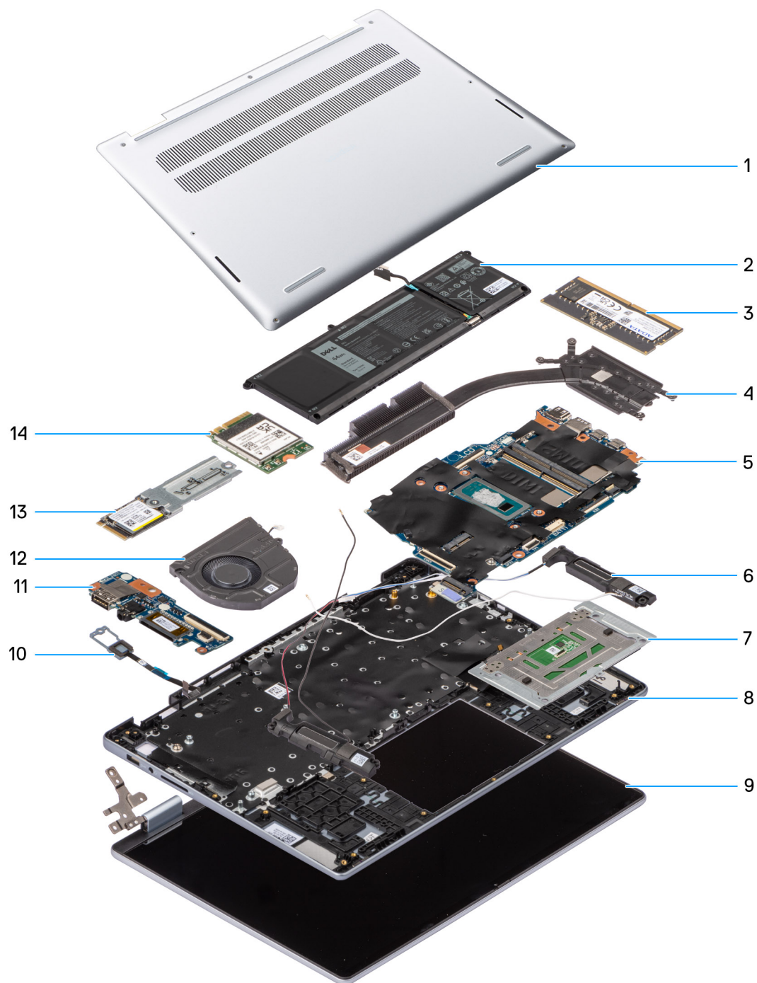
Ilustración 12. Componentes principales del sistema
