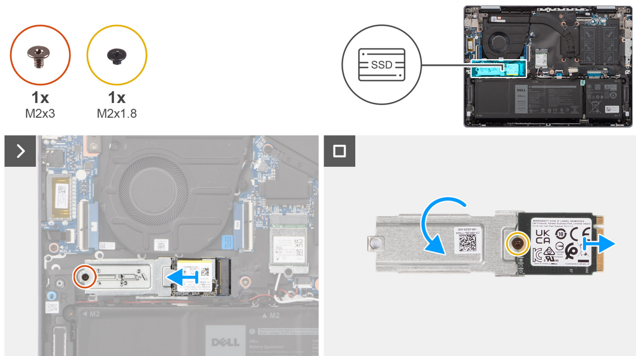
Ilustración 19. Extracción de la unidad de estado sólido
