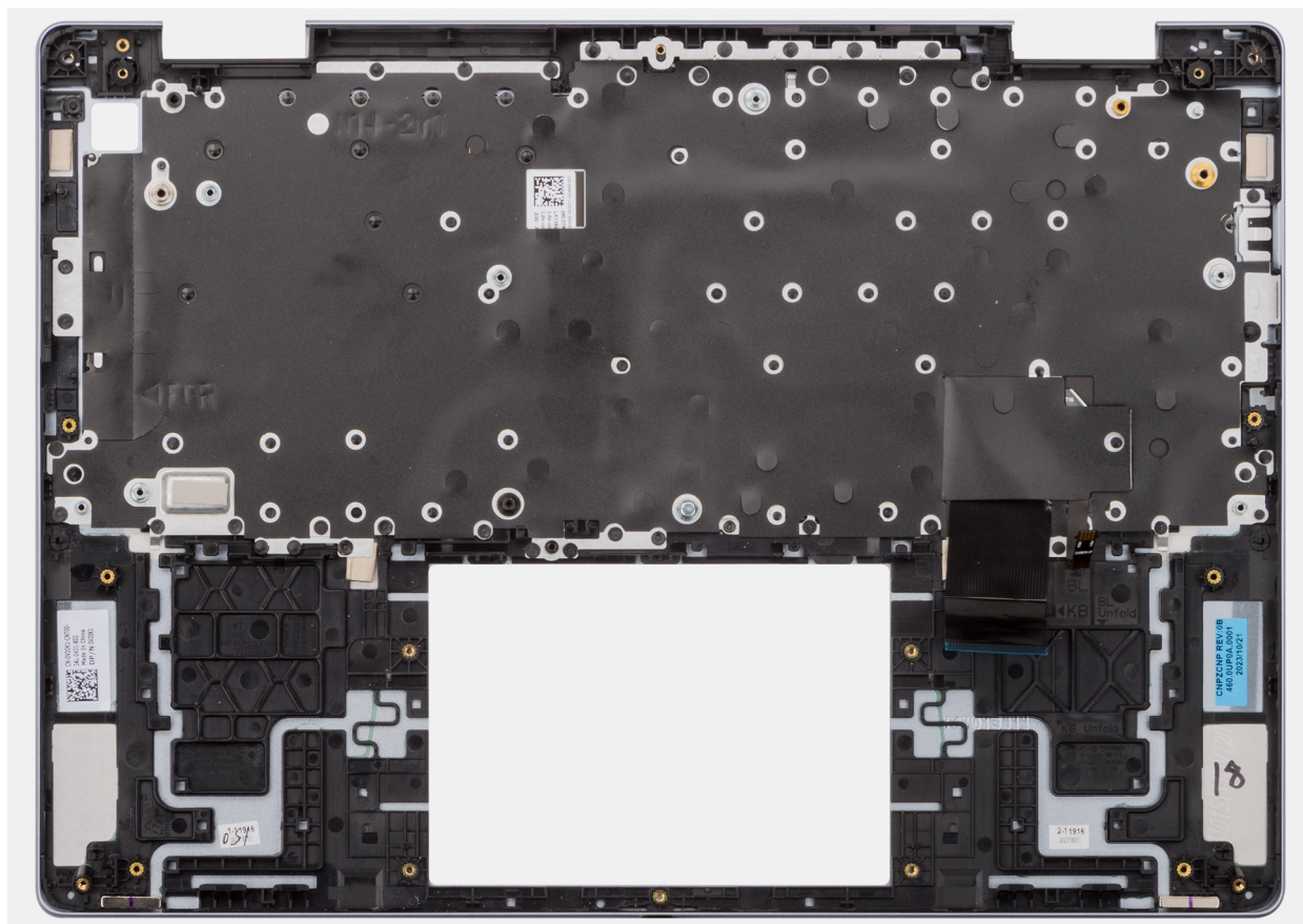
Ilustración 55. Instalación del ensamblaje del teclado y el reposamanos
