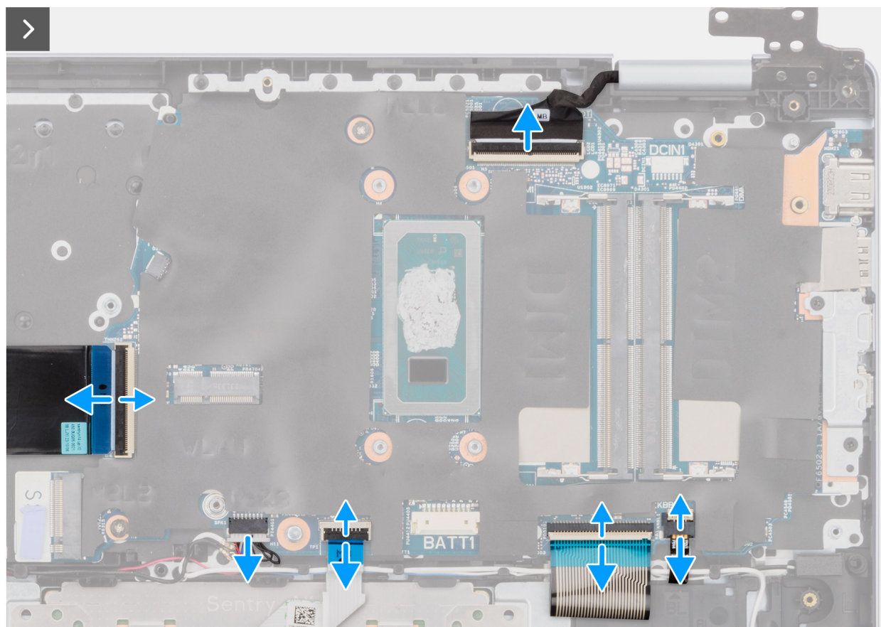
Ilustración 47. Extracción de los conectores de los cables
