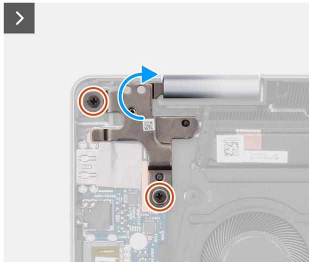
Ilustración 41. Extracción de los tornillos
