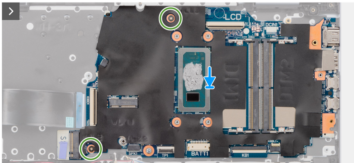
Ilustración 50. Instalación de la tarjeta madre
