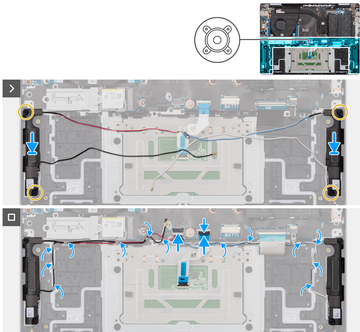
Ilustración 40. Instalación de los parlantes
