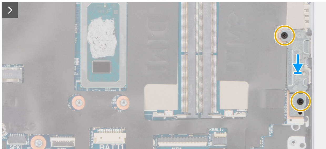
Ilustración 51. Colocación del soporte para USB Type-C
