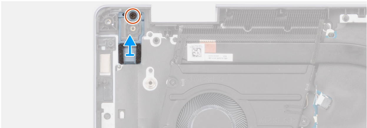
Ilustración 33. Extracción del botón de encendido
