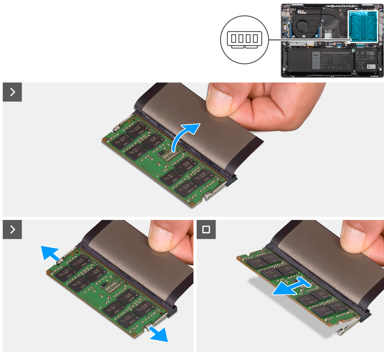
Ilustración 17. Extracción del módulo de memoria
