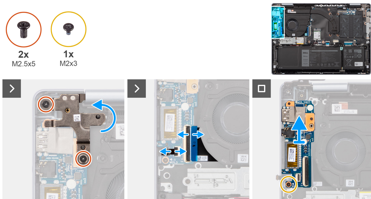
Ilustración 31. Extracción de la placa de I/O
