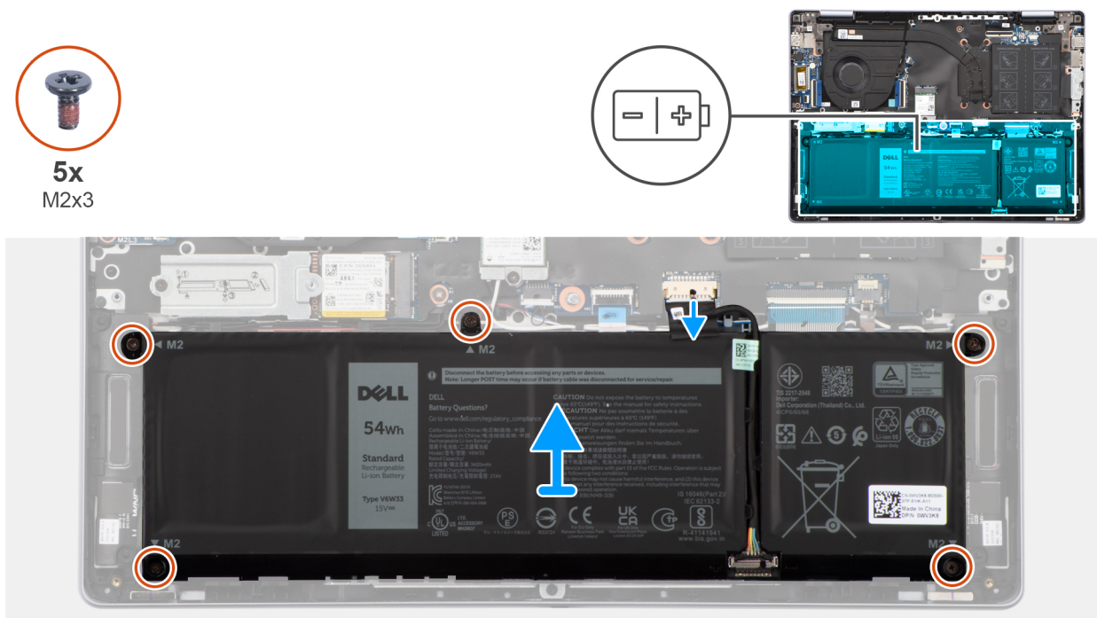
Ilustración 25. Extracción de la batería
