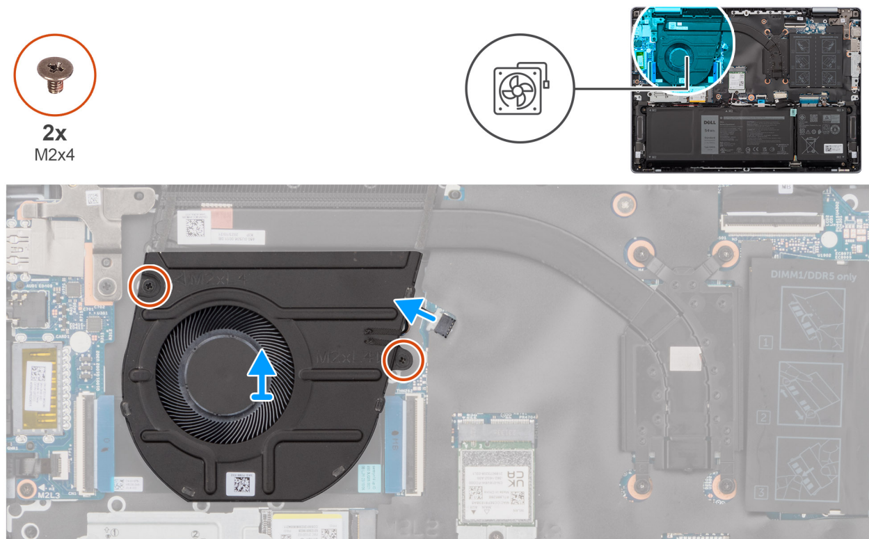
Ilustración 23. Extracción del ventilador
