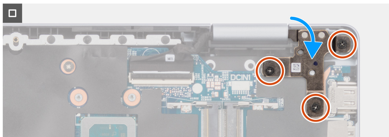
Ilustración 53. Colocación de los tornillos de las bisagras
