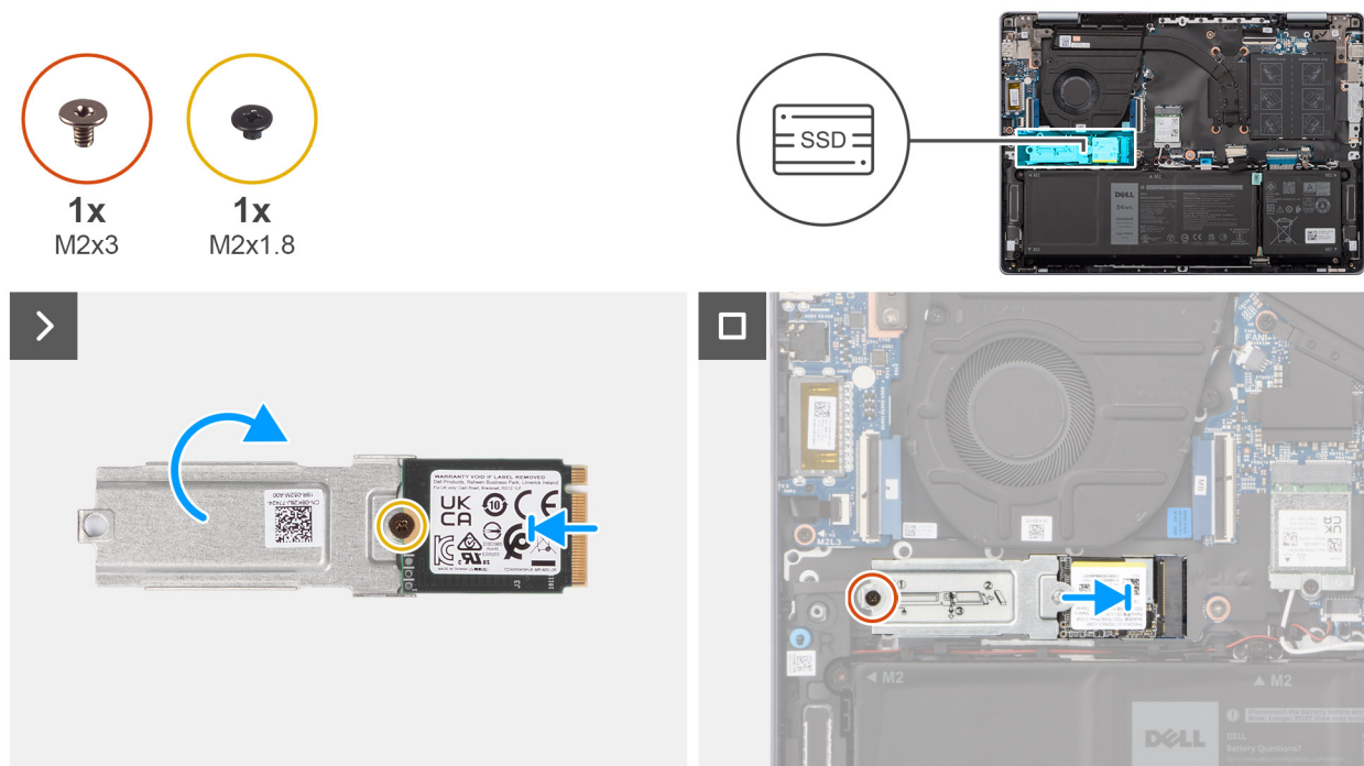
Ilustración 20. Instalación de la unidad de estado sólido
