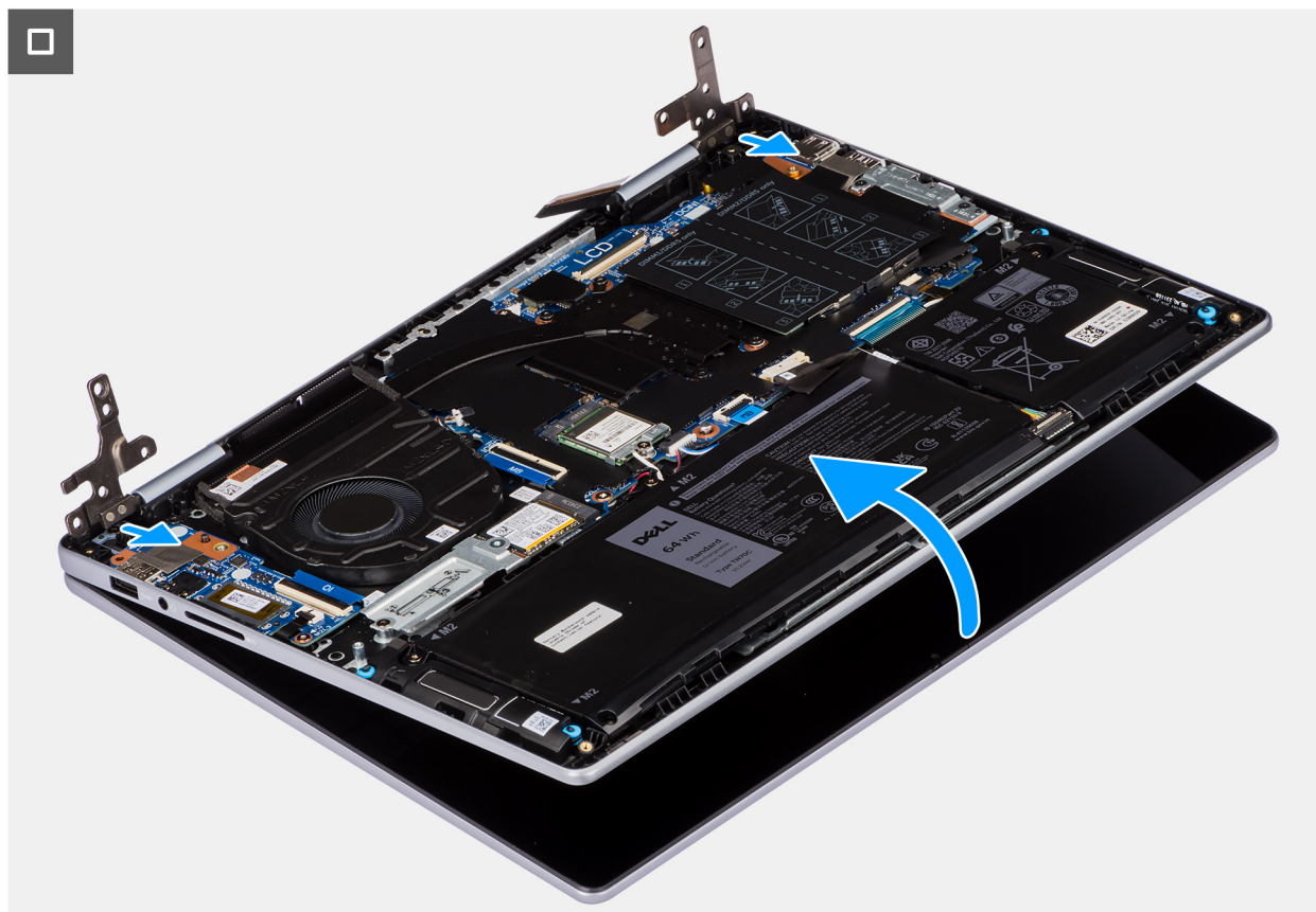
Ilustración 42. Extracción del ensamblaje de la pantalla
