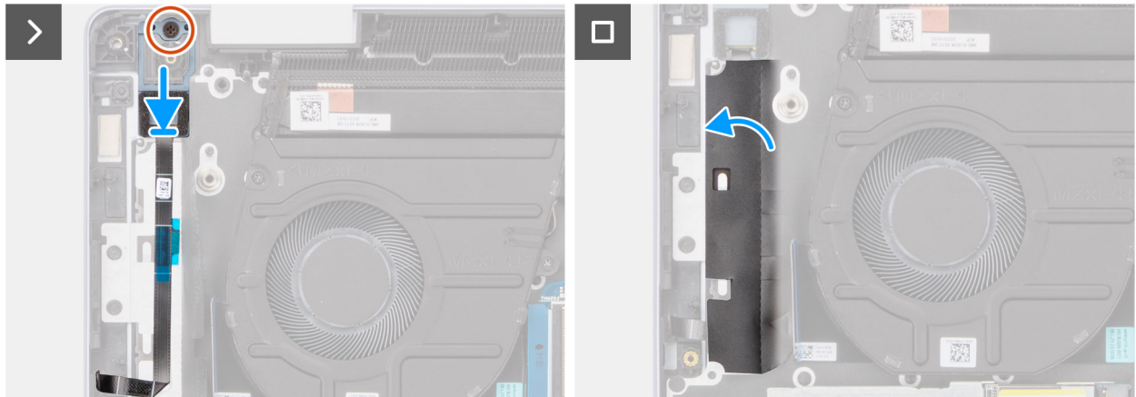
Ilustración 36. Instalación del botón de encendido con lector de huellas digitales
