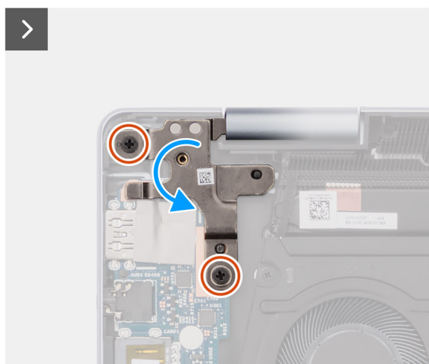
Ilustración 44. Reemplazo de los tornillos
