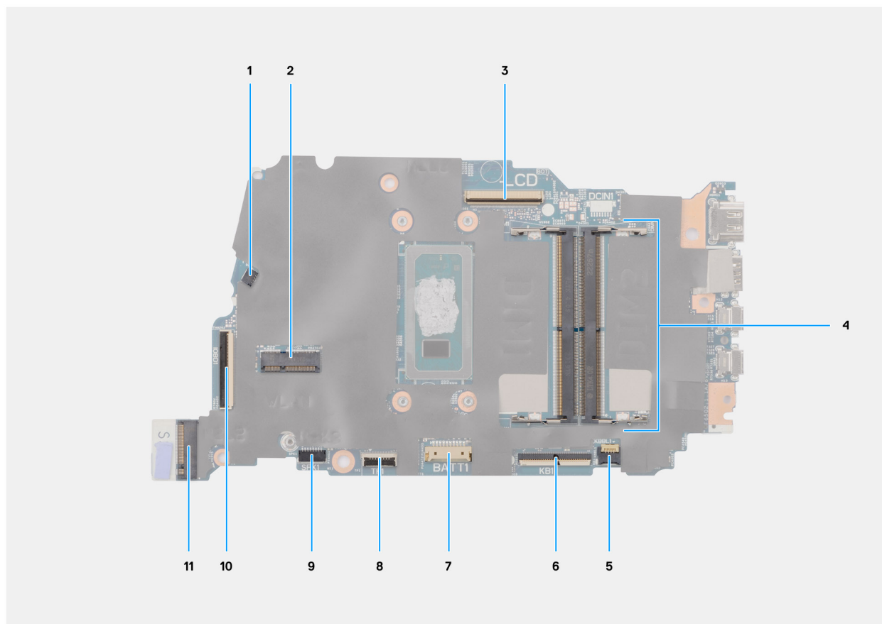
Ilustración 45. Conectores en la tarjeta madre
