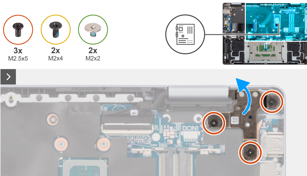
Ilustración 46. Extracción de los tornillos de la bisagra derecha
