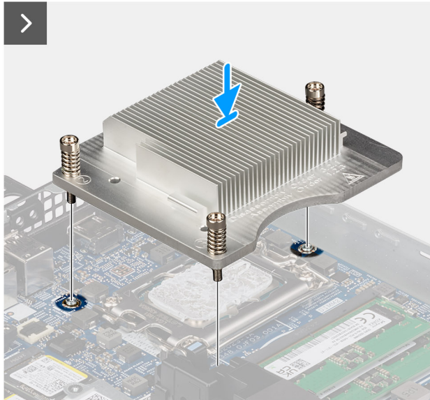
Afbeelding 63. De koelplaat plaatsen
