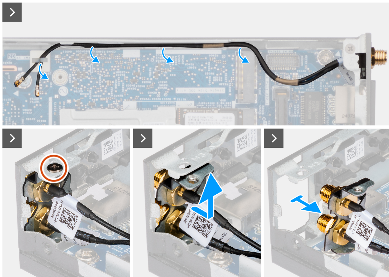
Afbeelding 36. De SMA-antenne verwijderen
