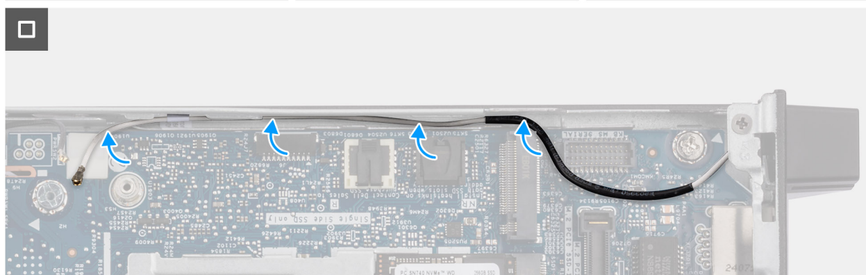
Afbeelding 69. De antennemodule (witte kabel) plaatsen
