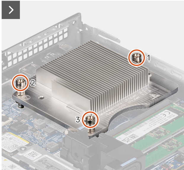
Afbeelding 62. De koelplaat verwijderen
