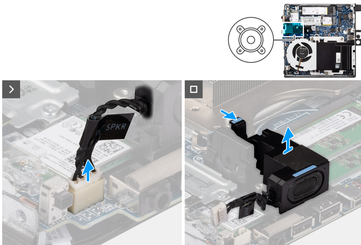
Afbeelding 14. De luidspreker verwijderen
