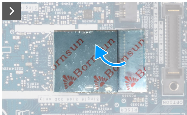
Afbeelding 17. De 2230 SSD installeren
