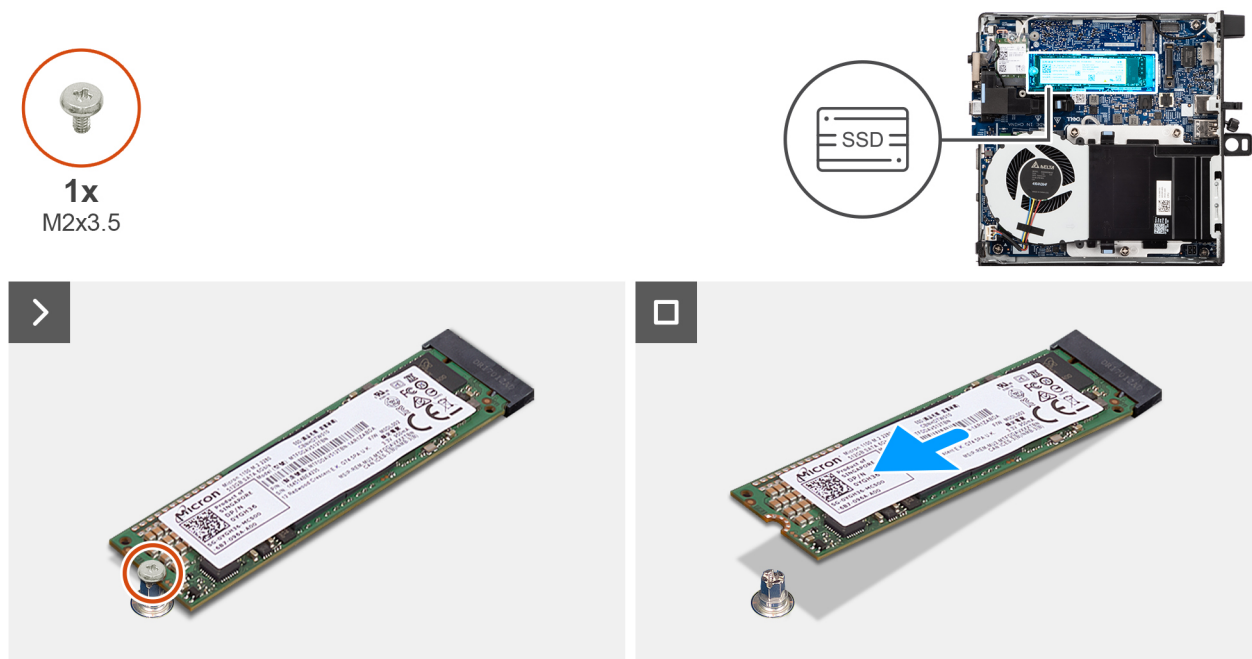
Afbeelding 19. De M.2 2280 SSD verwijderen
