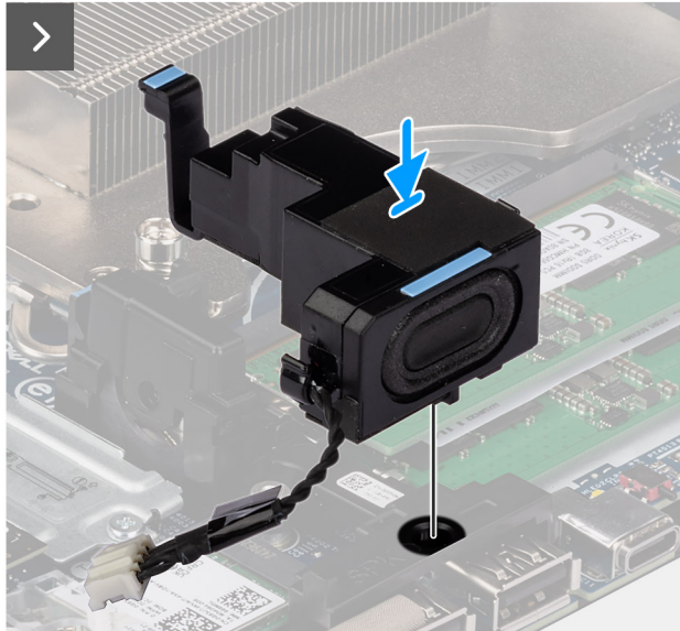
Afbeelding 15. De luidspreker plaatsen
