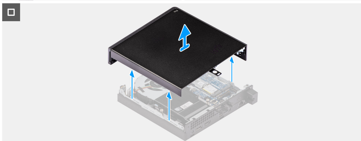
Afbeelding 10. De zijplaat verwijderen
