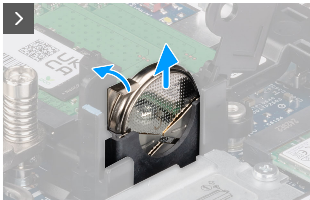
Afbeelding 12. De knoopcelbatterij verwijderen
