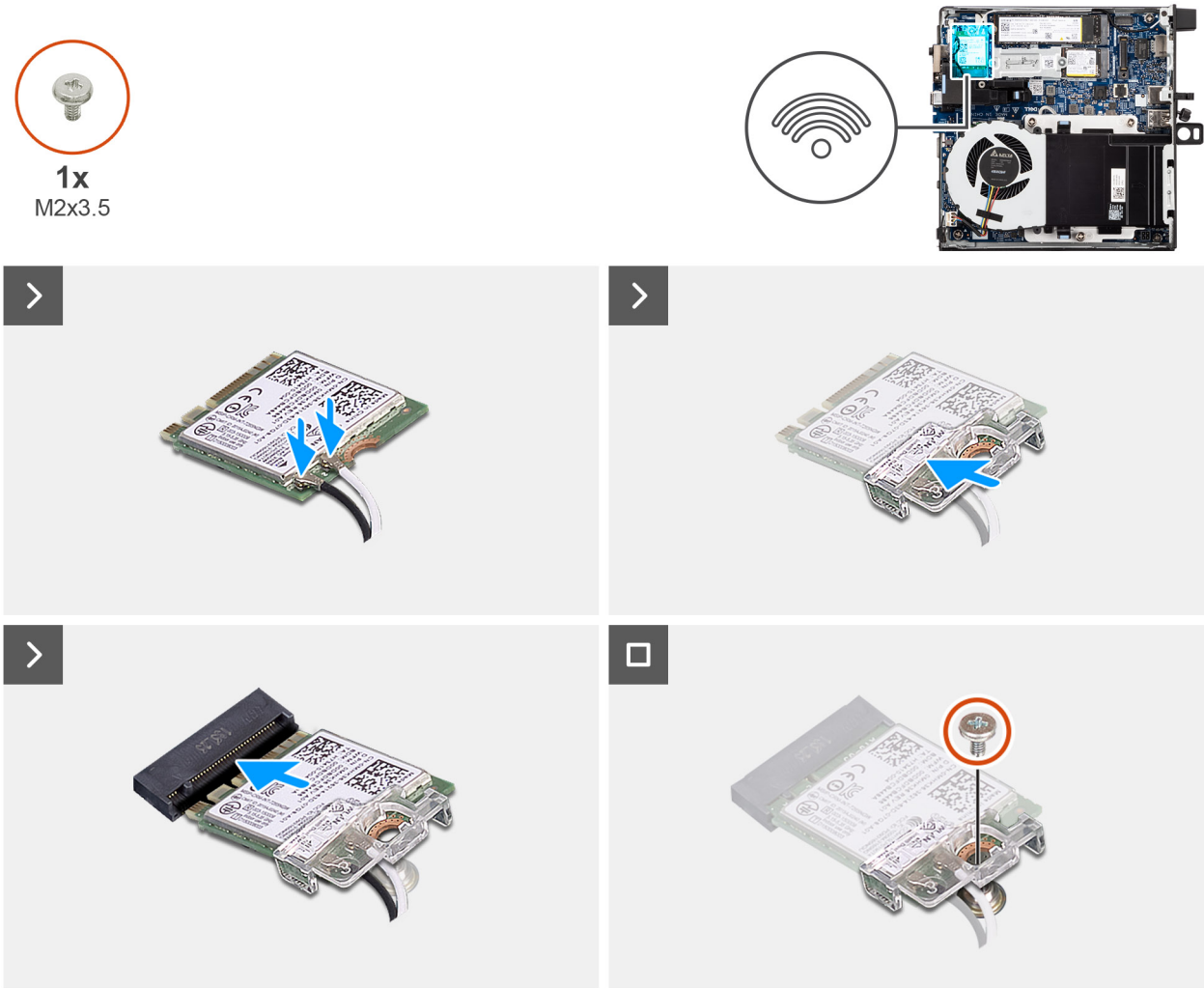
Afbeelding 27. De draadloze kaart plaatsen
