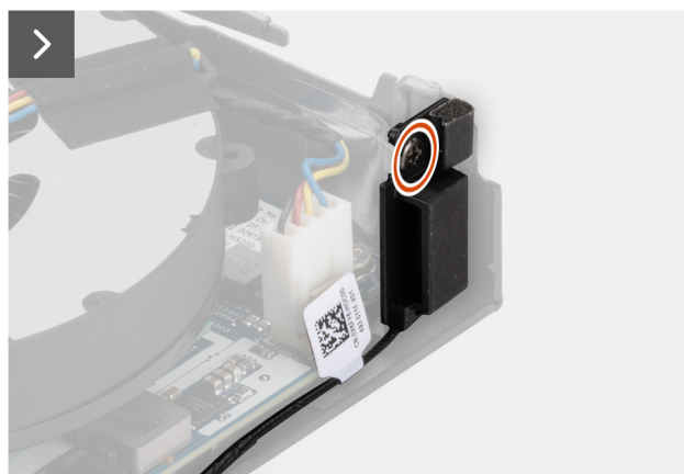
Afbeelding 64. De antennemodule (zwarte kabel) verwijderen
