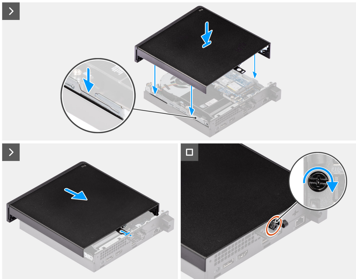
Afbeelding 11. De zijplaat plaatsen
