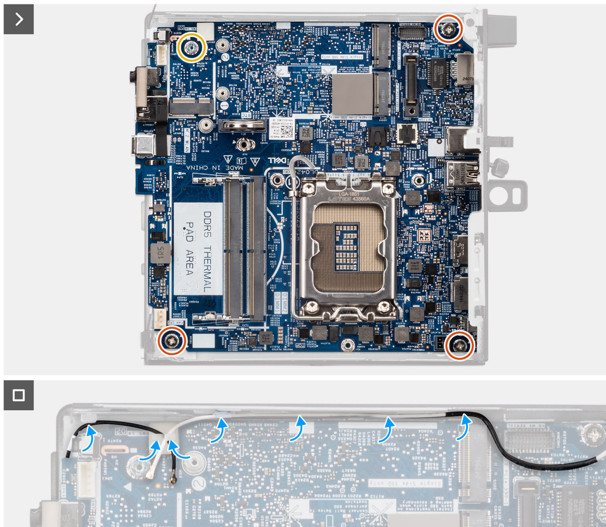
Afbeelding 79. De systeemkaart installeren
