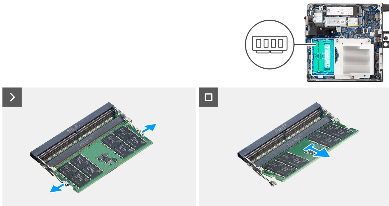
Afbeelding 32. De geheugenmodule verwijderen
