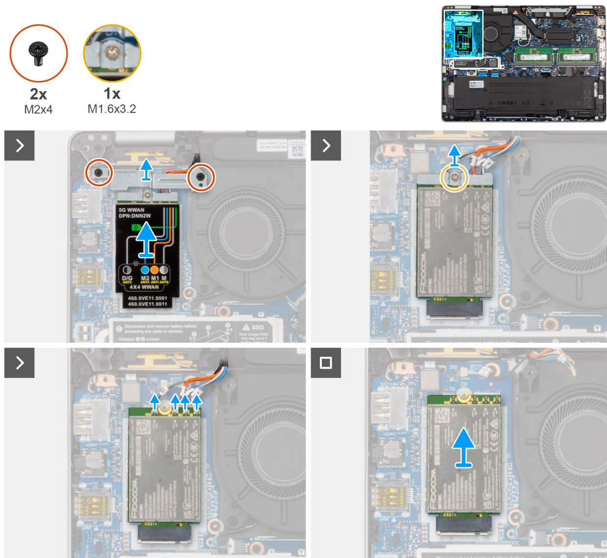
Afbeelding 29. De 5G WWAN-kaart verwijderen
