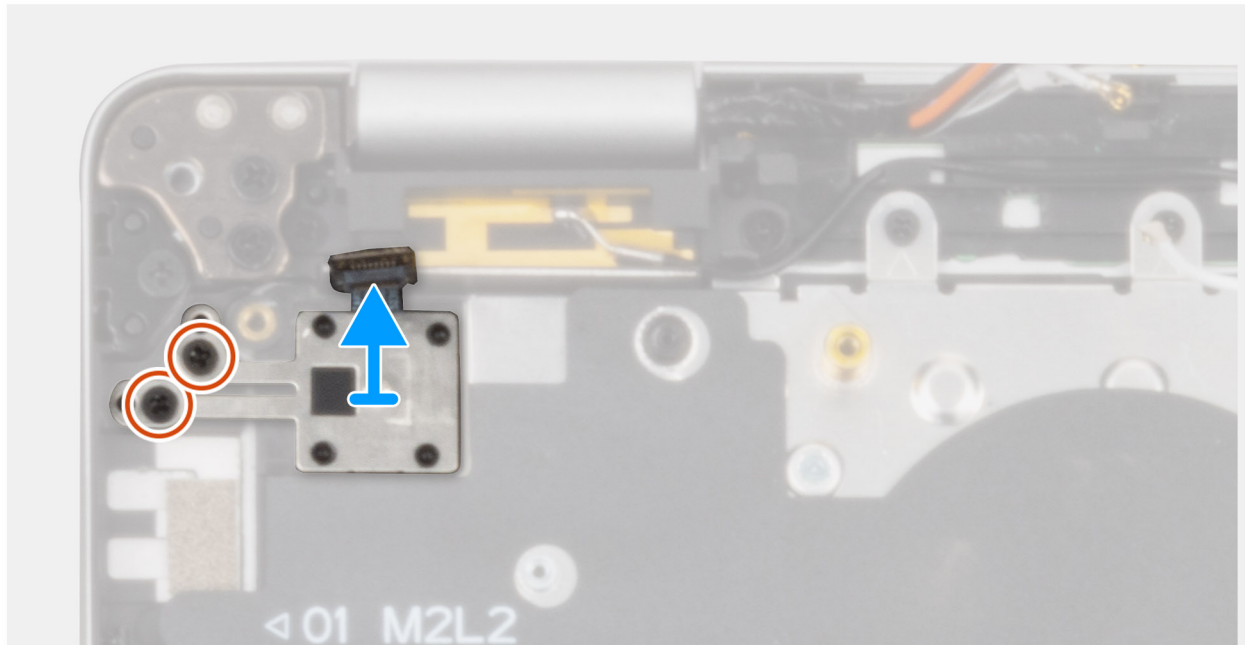
Afbeelding 64. De aan-uitknop met de optionele vingerafdruklezer verwijderen
