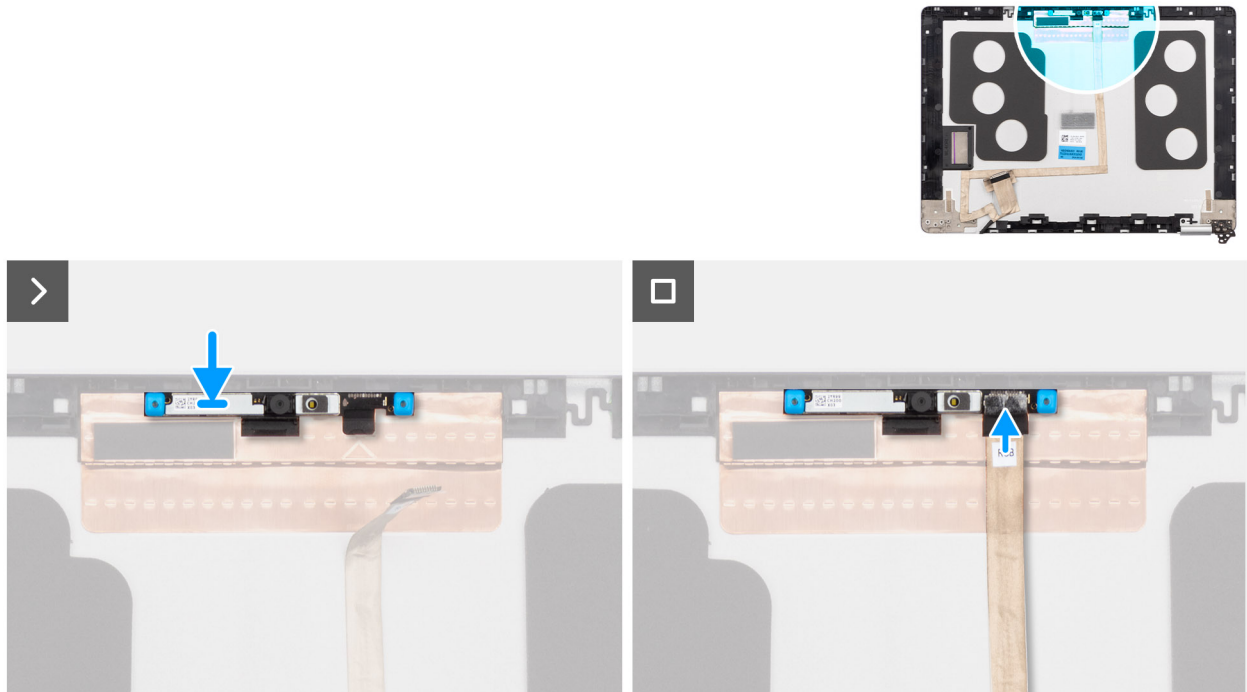
Afbeelding 79. De cameramodule installeren
