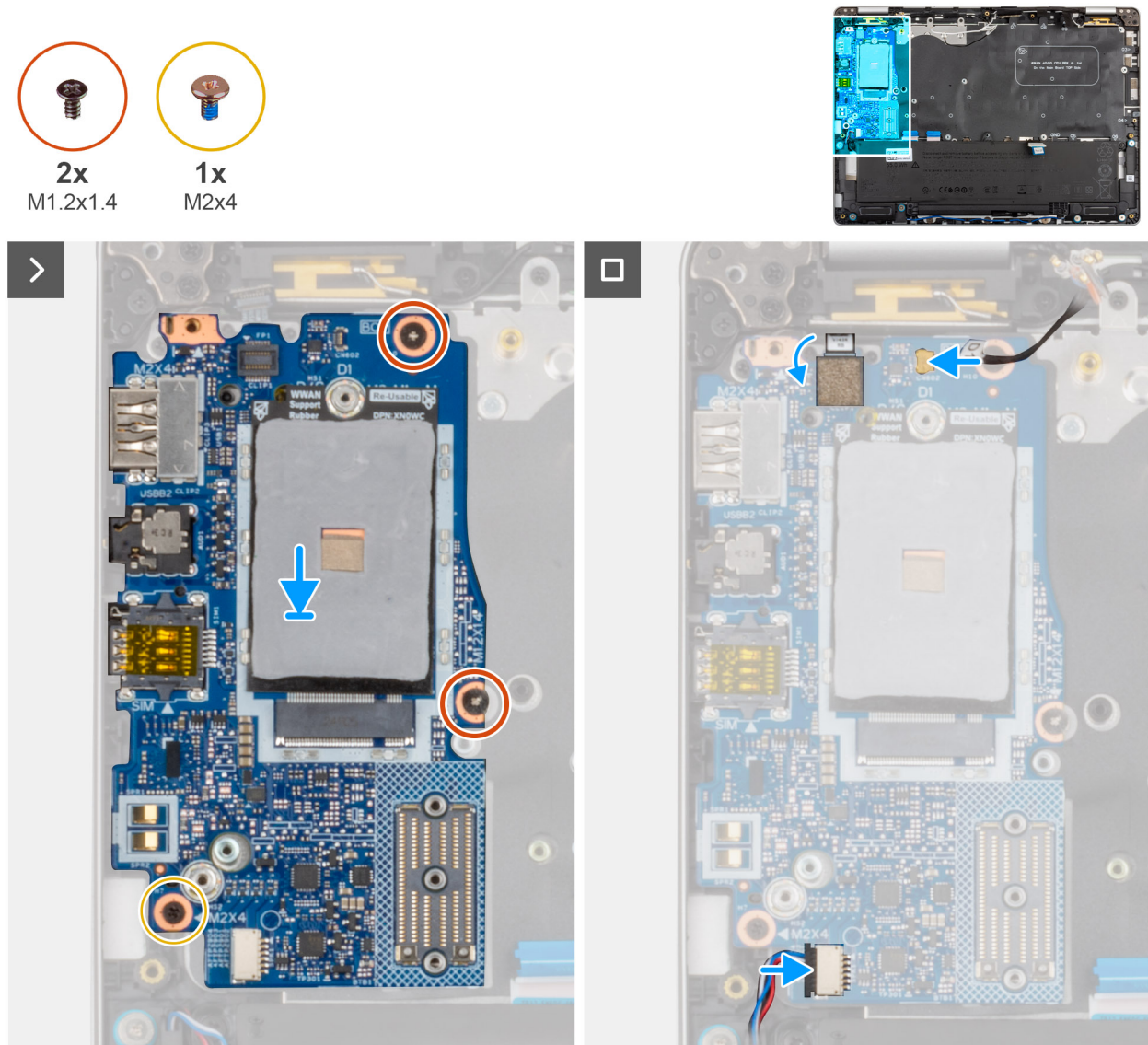
Afbeelding 63. De I/O-kaart installeren
