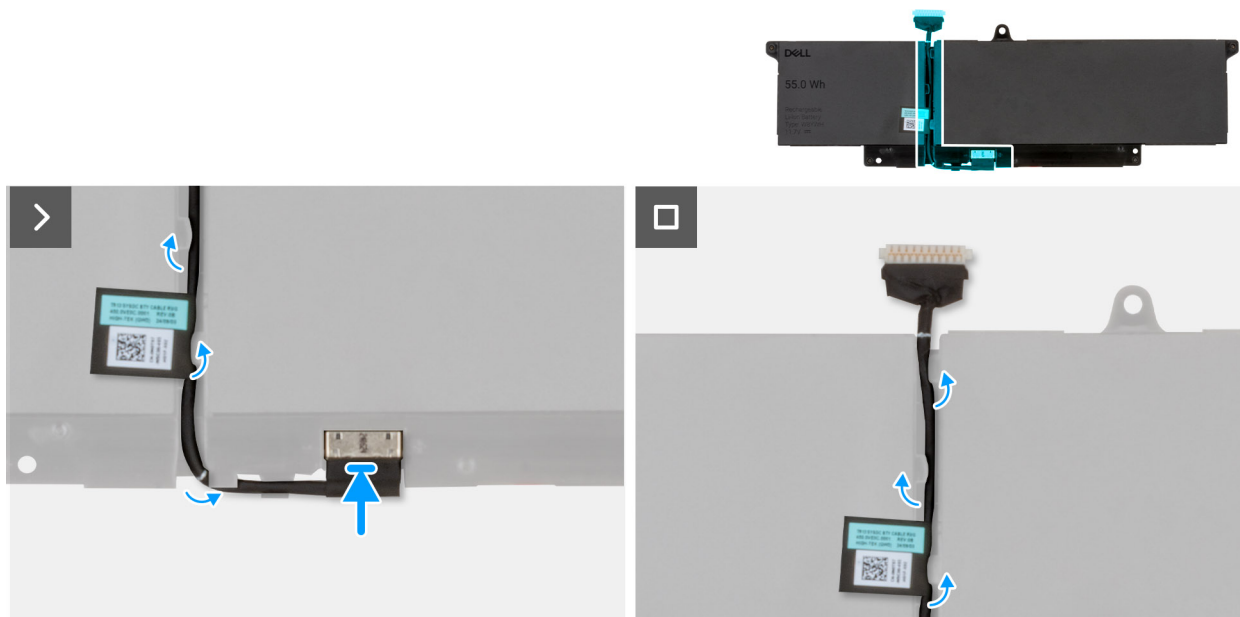
Afbeelding 26. De batterijkabel installeren
