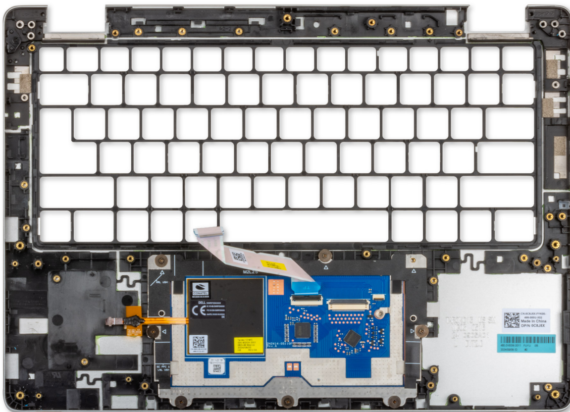
Afbeelding 71. De palmsteuneenheid installeren
