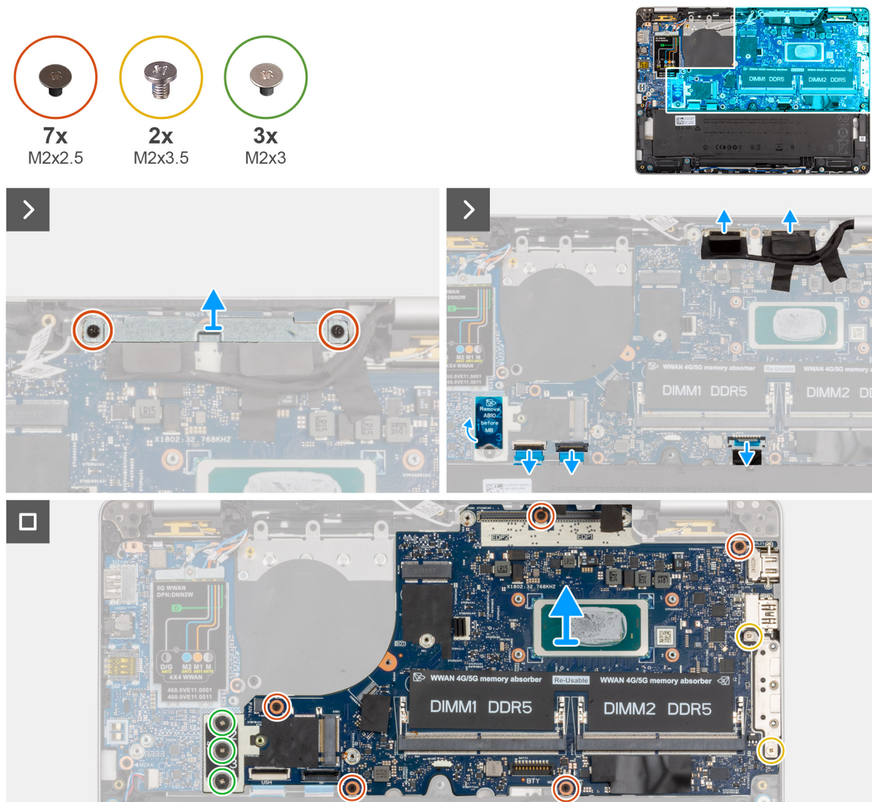
Afbeelding 55. De systeemkaart verwijderen
