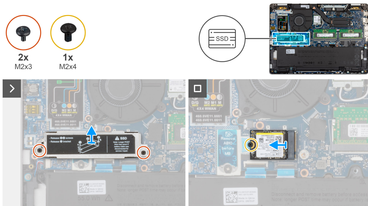
Afbeelding 35. De M.2 2230 SSD verwijderen
