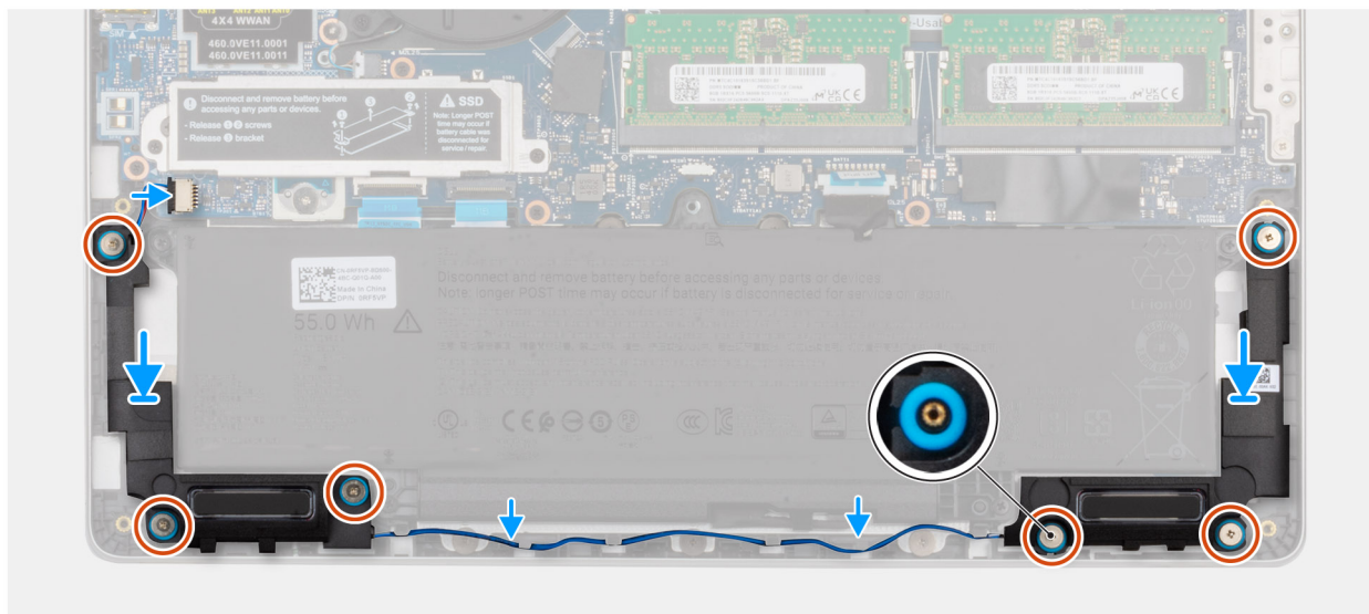
Afbeelding 40. De luidsprekers installeren
