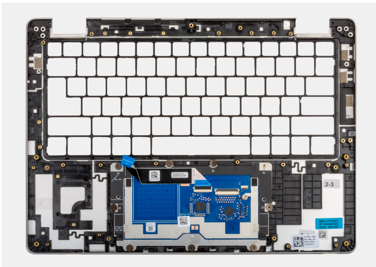
Afbeelding 70. De palmsteuneenheid verwijderen
