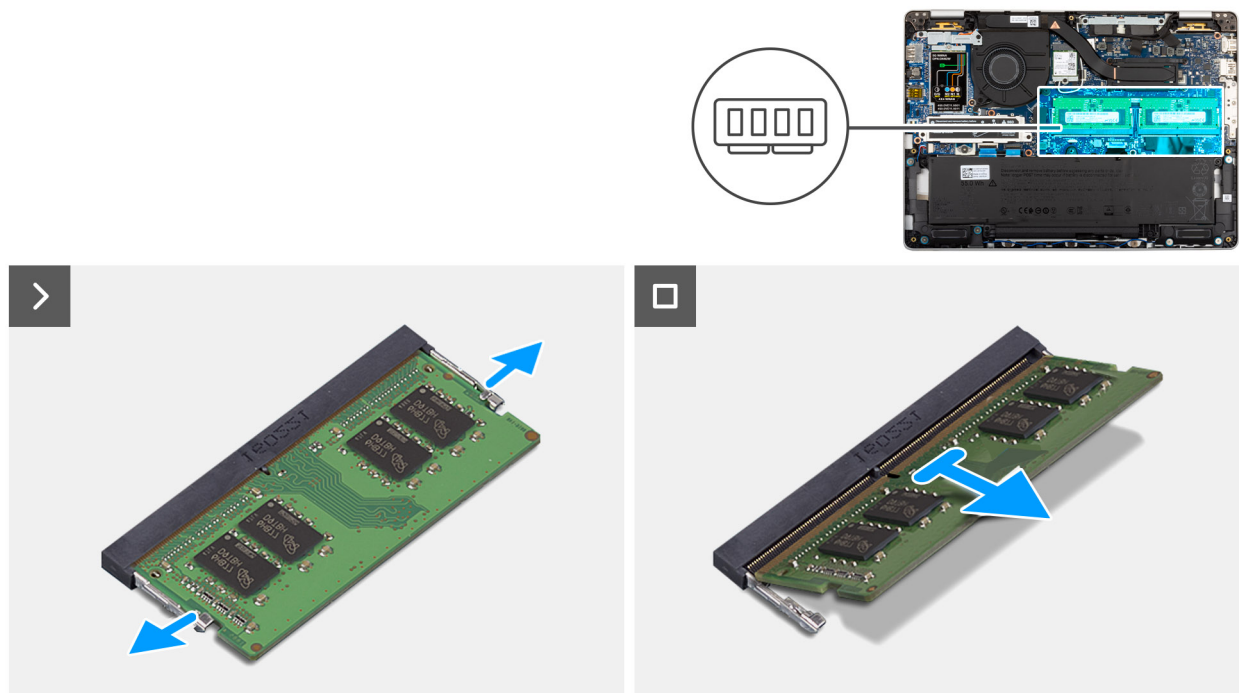
Afbeelding 27. De geheugenmodule verwijderen
