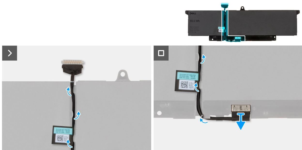
Afbeelding 25. De batterijkabel verwijderen
