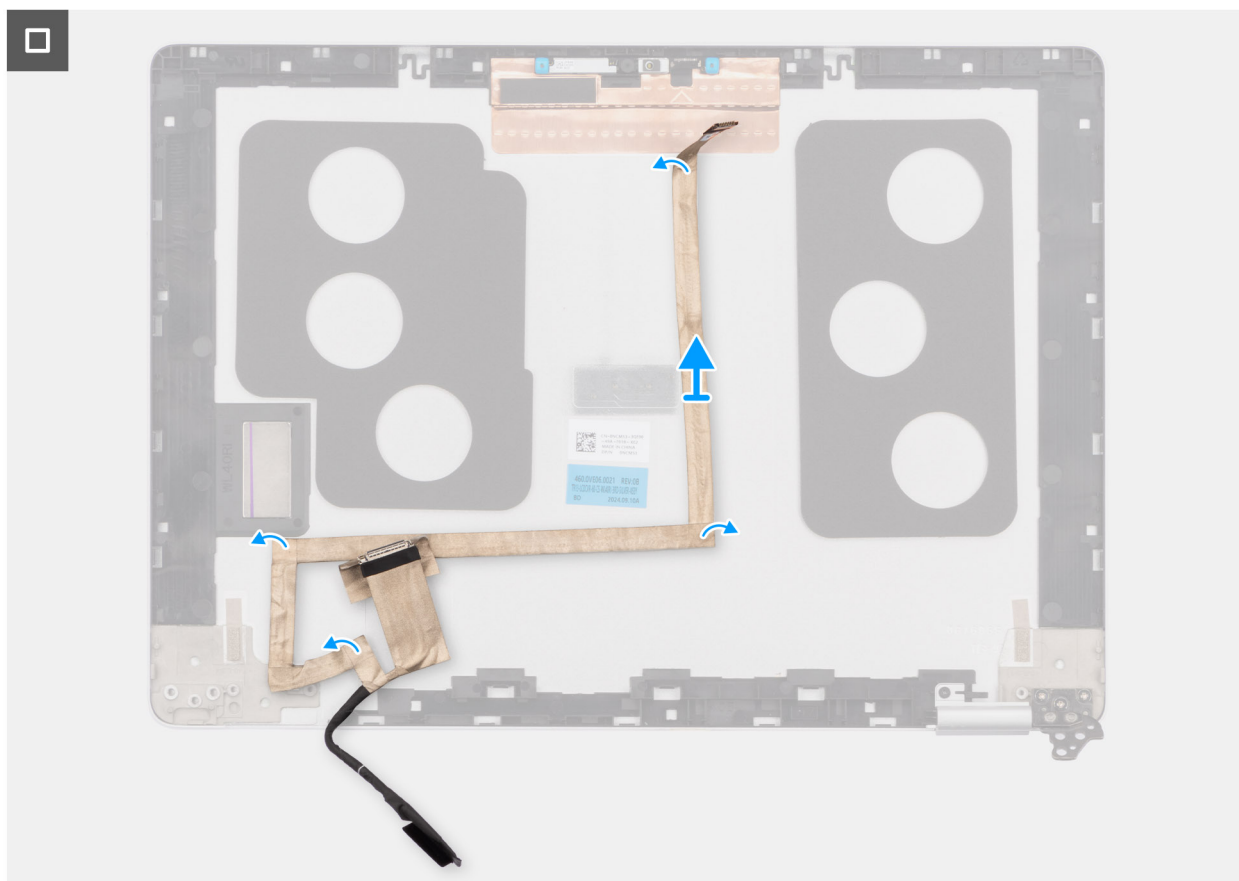
Afbeelding 81. De beeldschermkabel verwijderen
