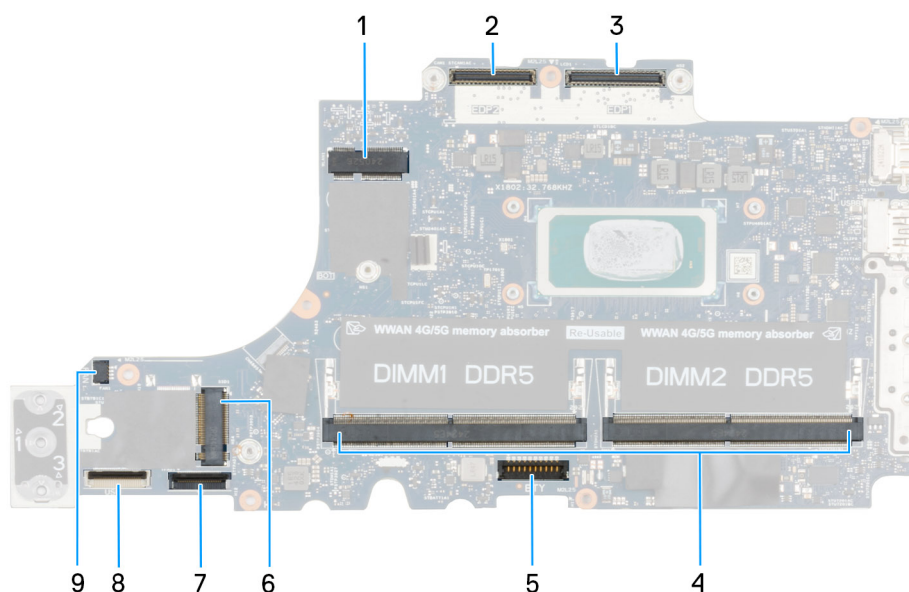
Afbeelding 56. Systeemkaartconnectoren
