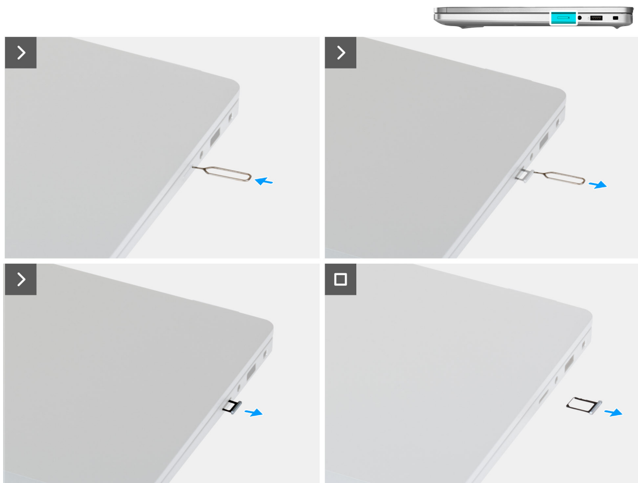
Afbeelding 15. De simkaartlade verwijderen
