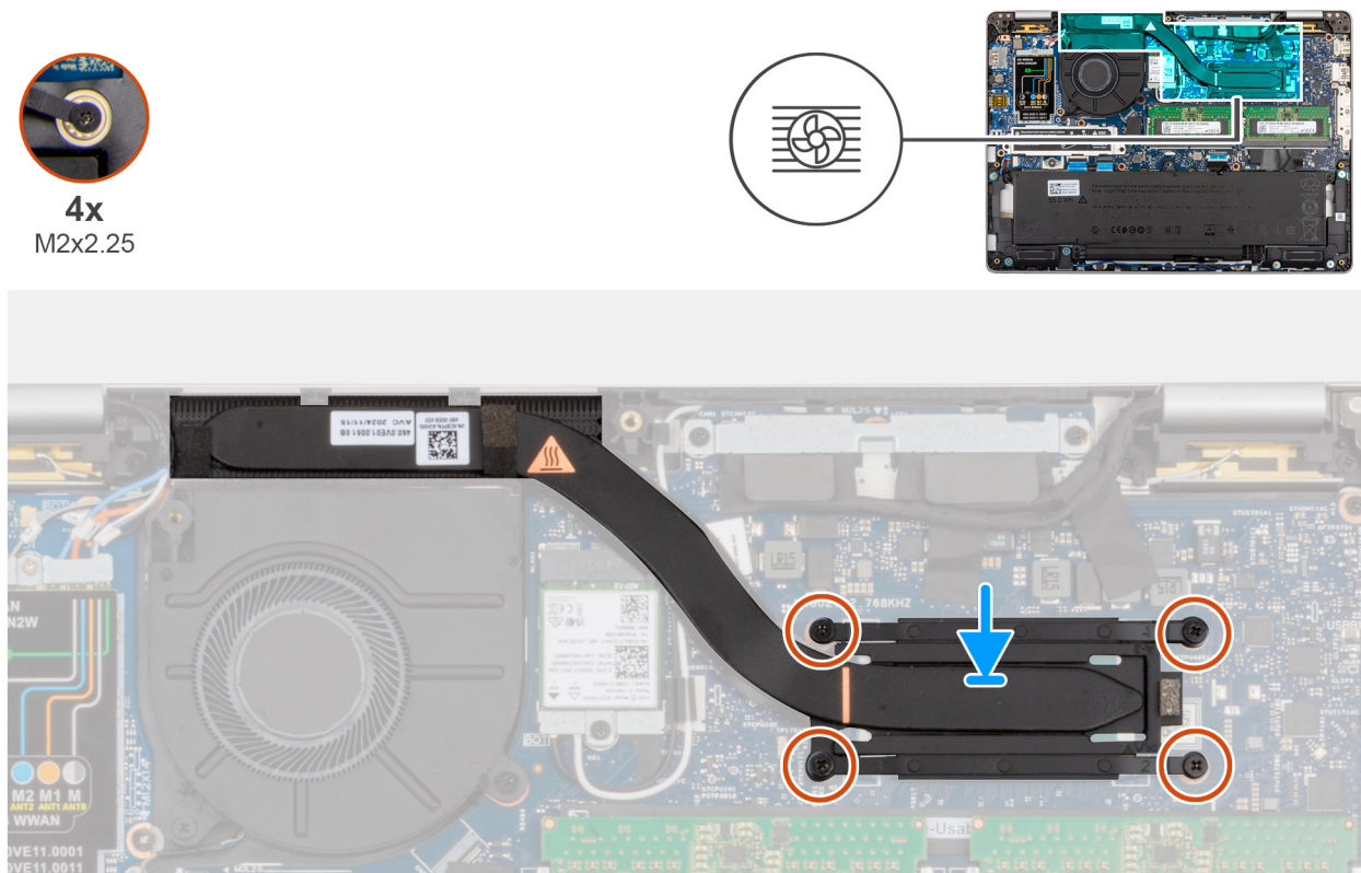
Afbeelding 49. De koelplaat installeren
