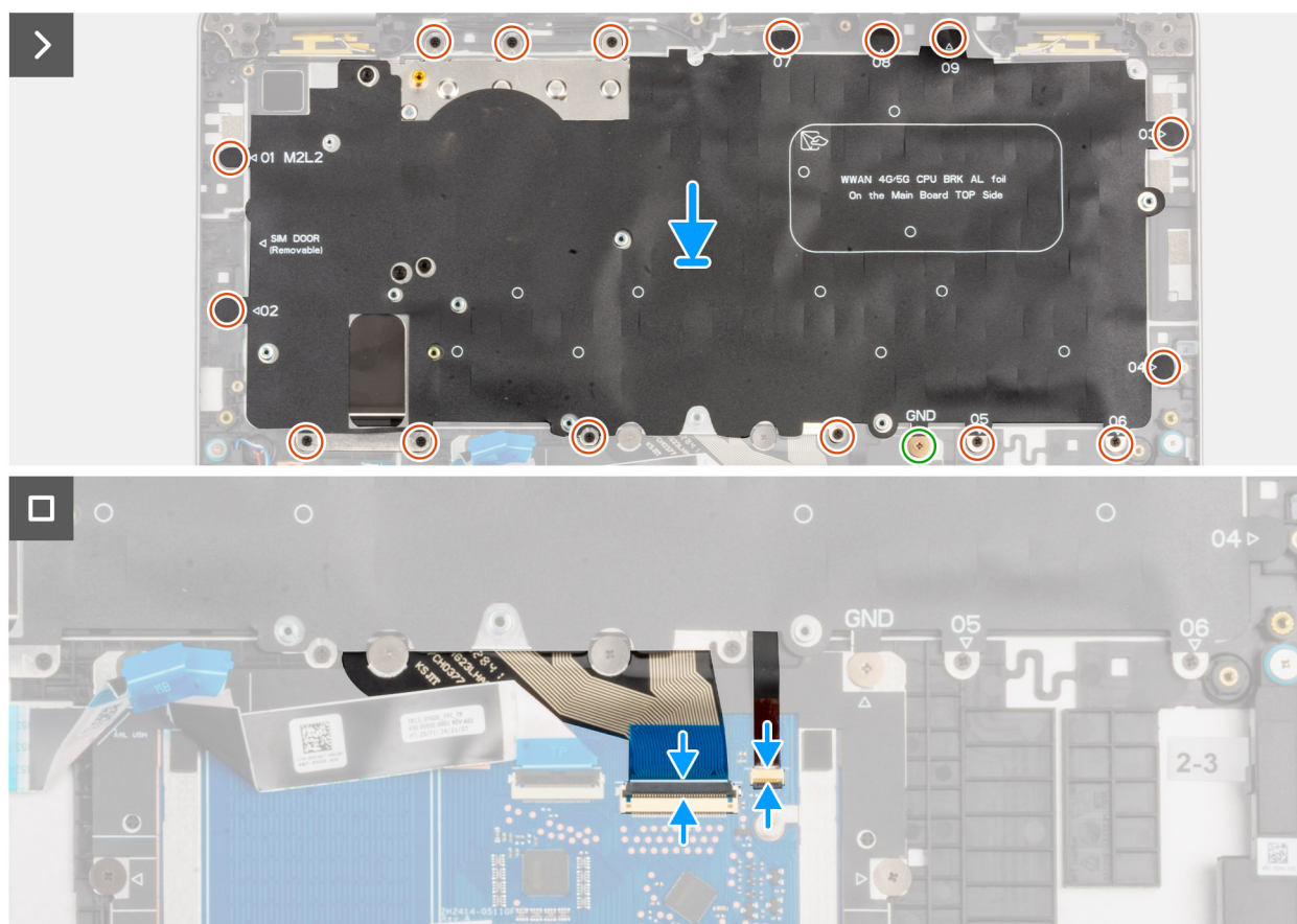
Afbeelding 69. Het toetsenbord installeren
