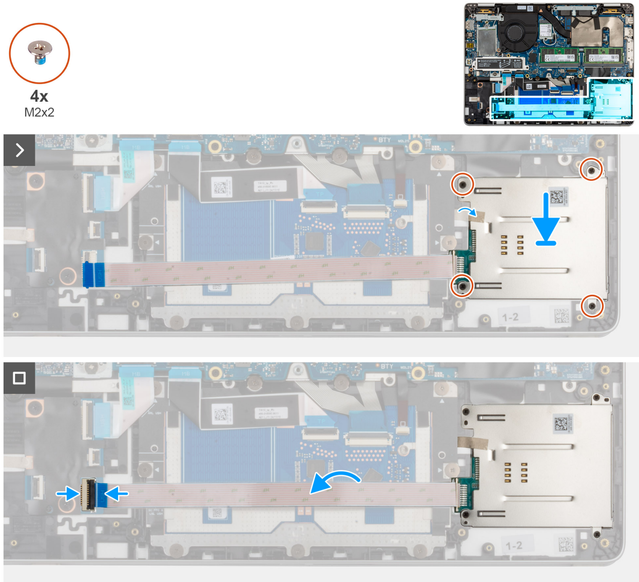
Afbeelding 47. De smartcardlezer installeren
