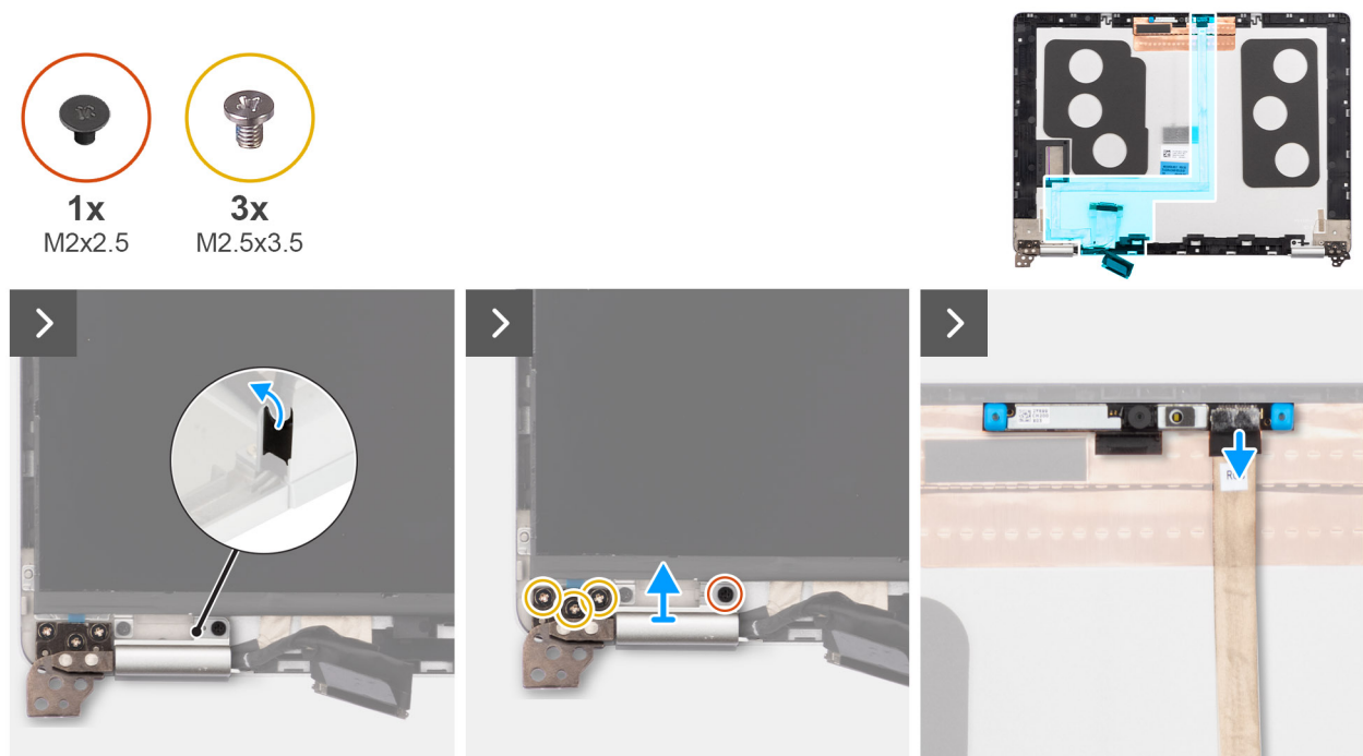
Afbeelding 80. De beeldschermkabel verwijderen
