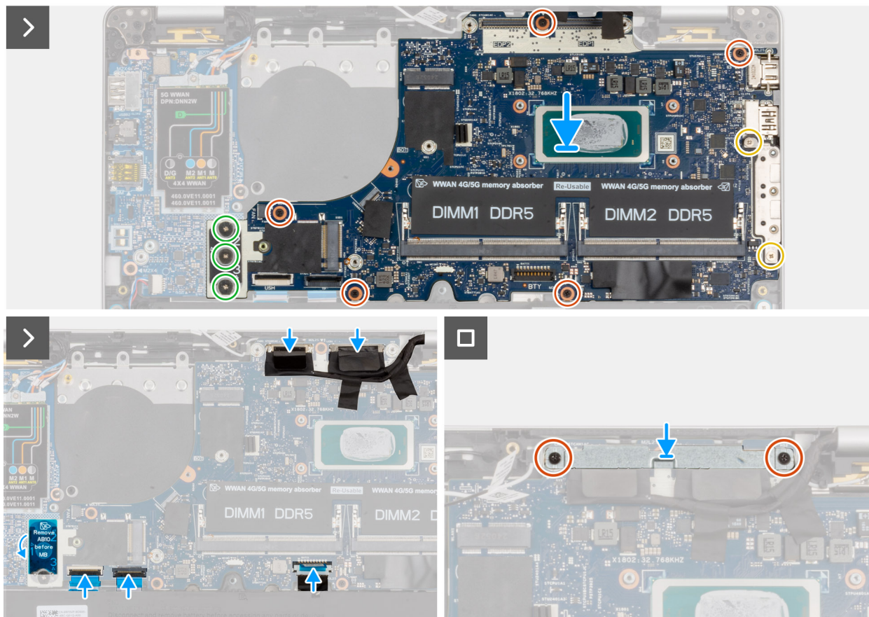
Afbeelding 57. De systeemkaart installeren
