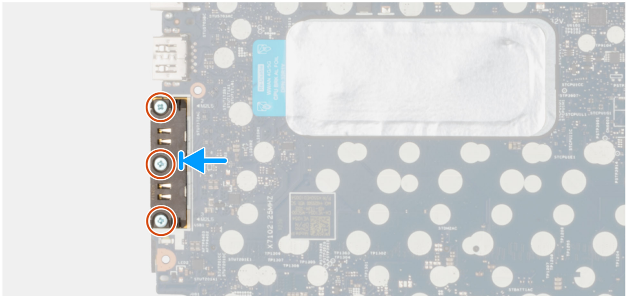
Afbeelding 59. De USB Type-C aansluitingsmodule installeren
