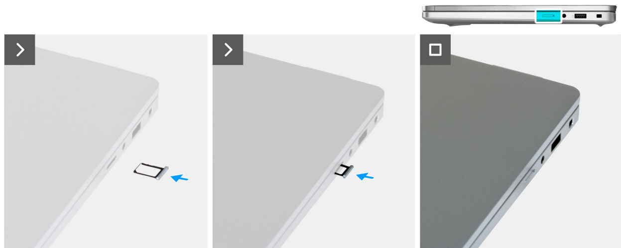
Afbeelding 16. De simkaarthouder installeren
