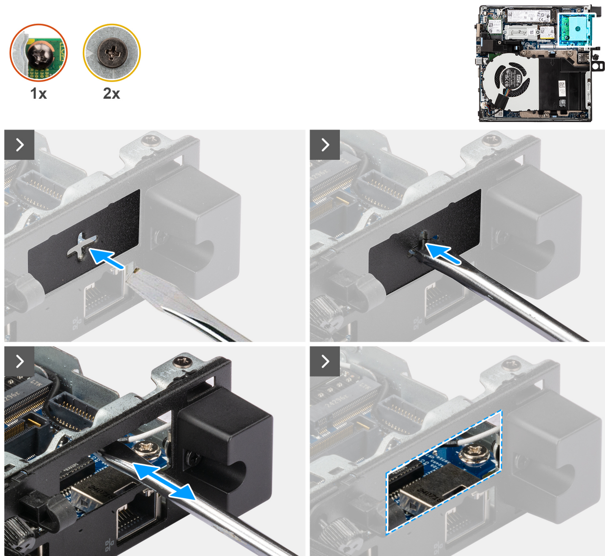
Figure 63. Installation du module de port fibre optique
