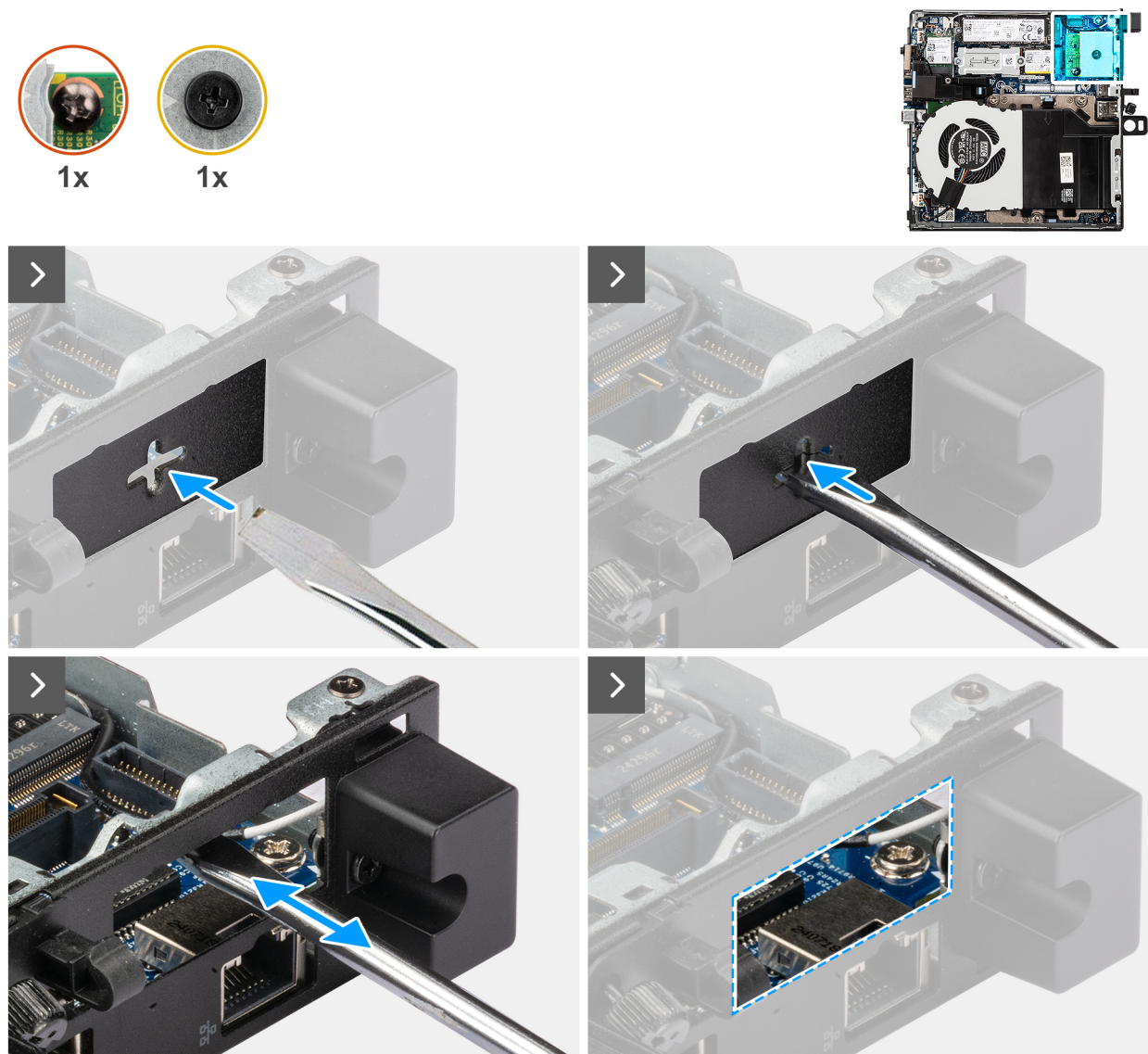
Figure 54. Installation du module de port VGA
