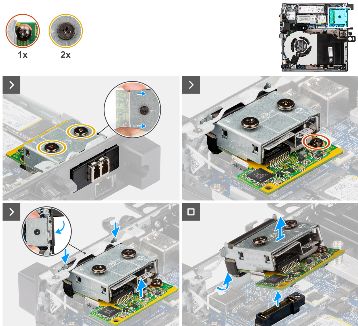
Figure 62. Retrait du module de port fibre optique
