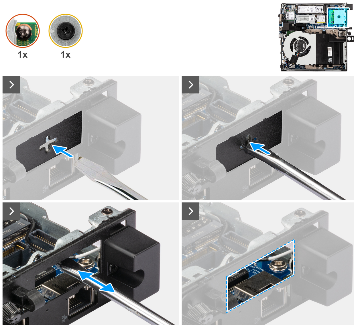
Figure 51. Installation du module de port HDMI
