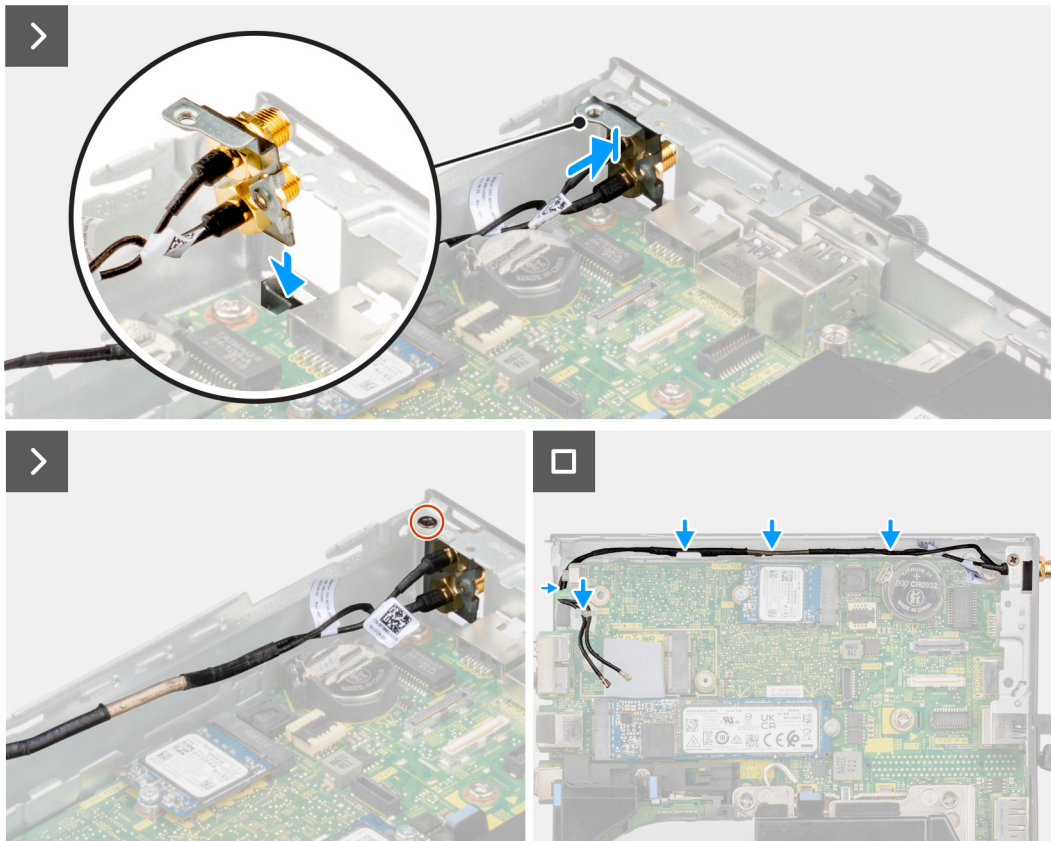
Figure 37. Installation du module d'antenne SMA
