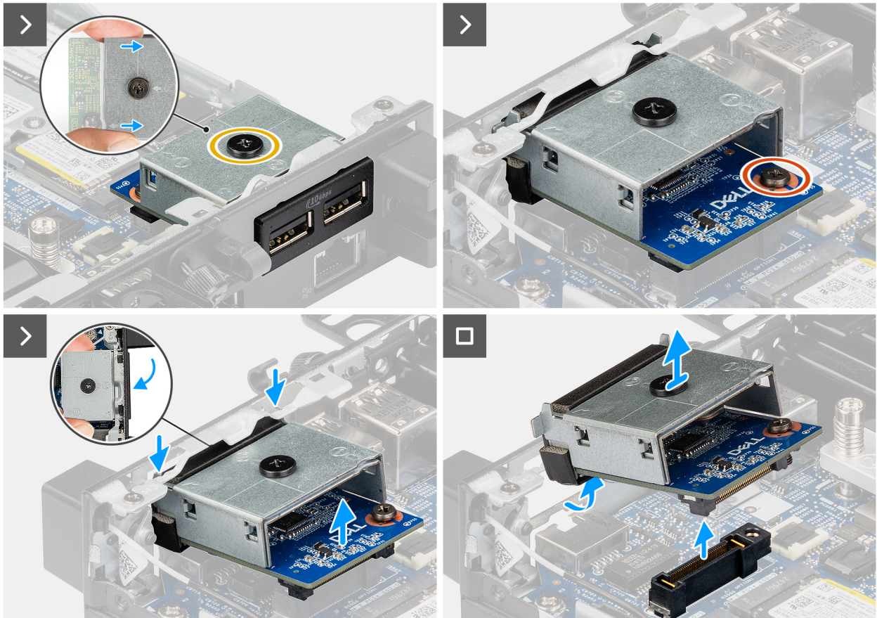
Figure 38. Retrait du module à deux ports USB 3,2 Gen 2
