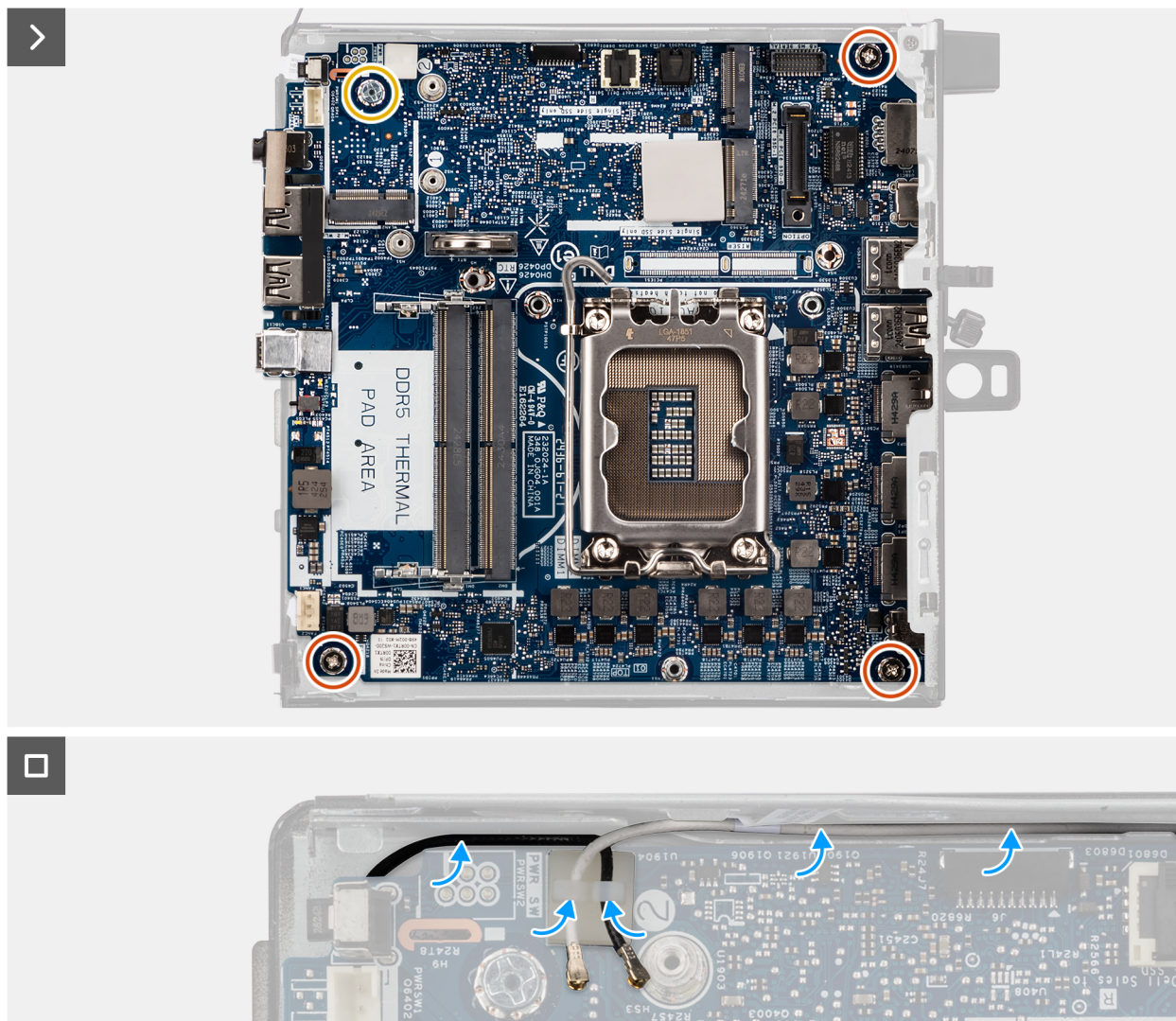
Figure 85. Installation de la carte système
