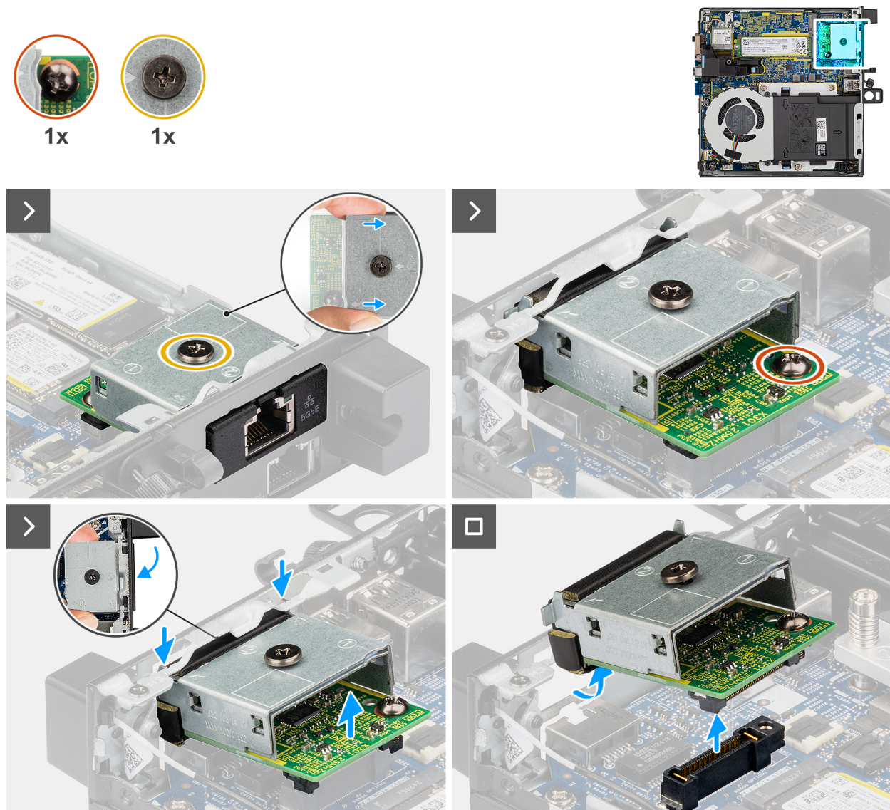
Figure 65. Retrait du module de port ethernet RJ45
