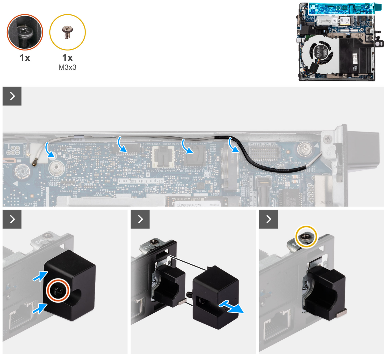
Figure 72. Retrait du module d'antenne (câble blanc)
