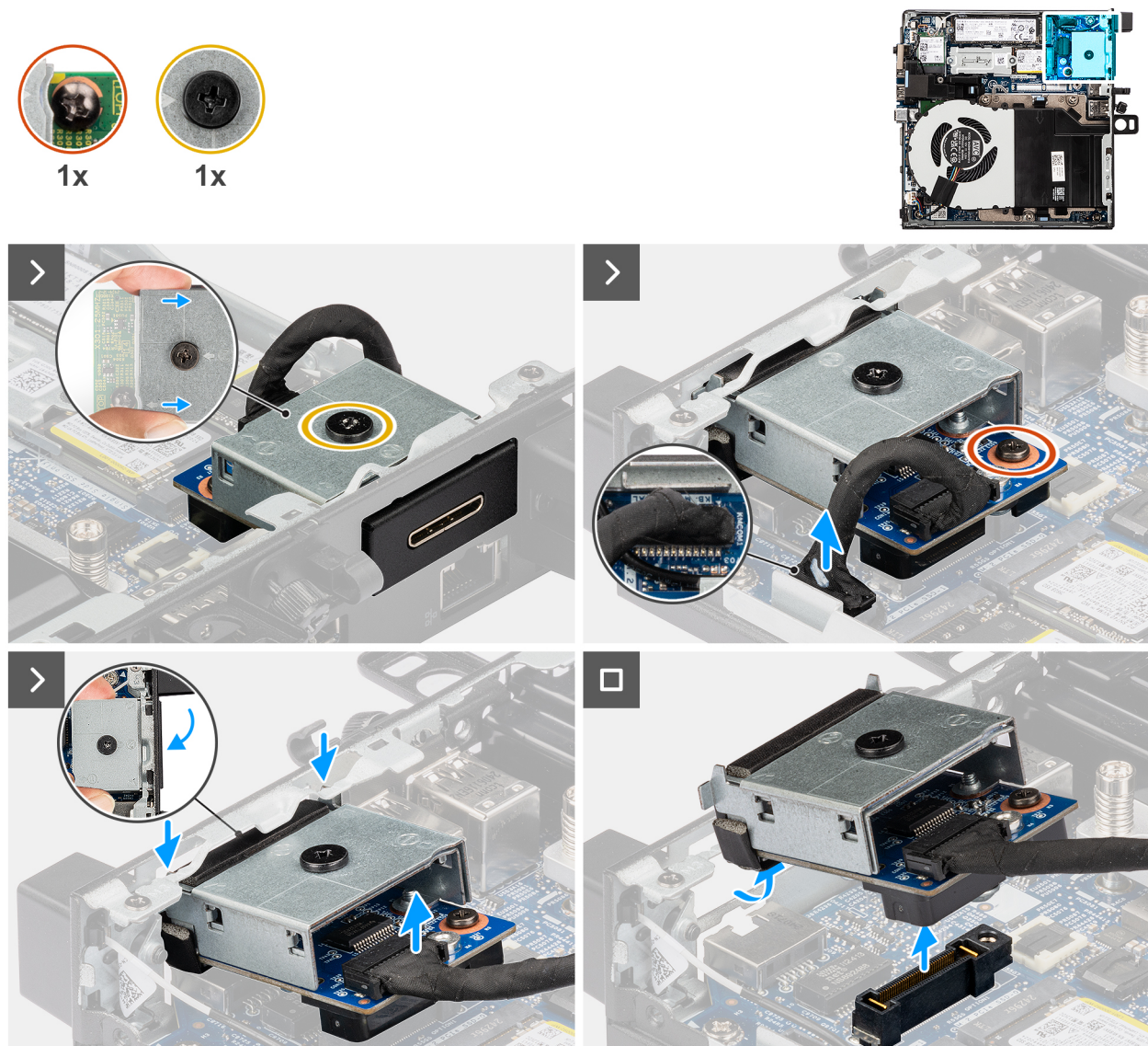
Figure 56. Retrait du module de port PS2
