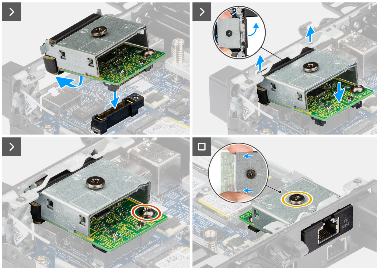
Figure 67. Installation du module de port Ethernet RJ45
