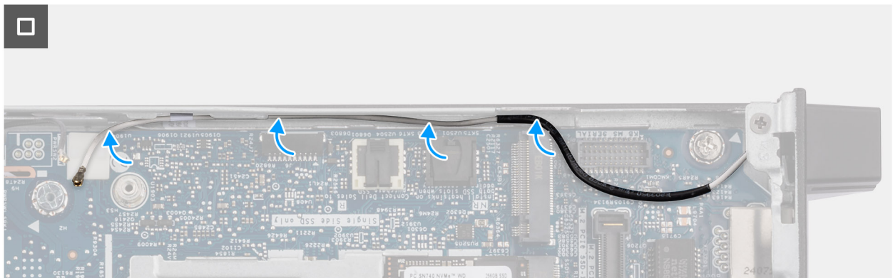
Figure 75. Installation du module d'antenne (câble blanc)
