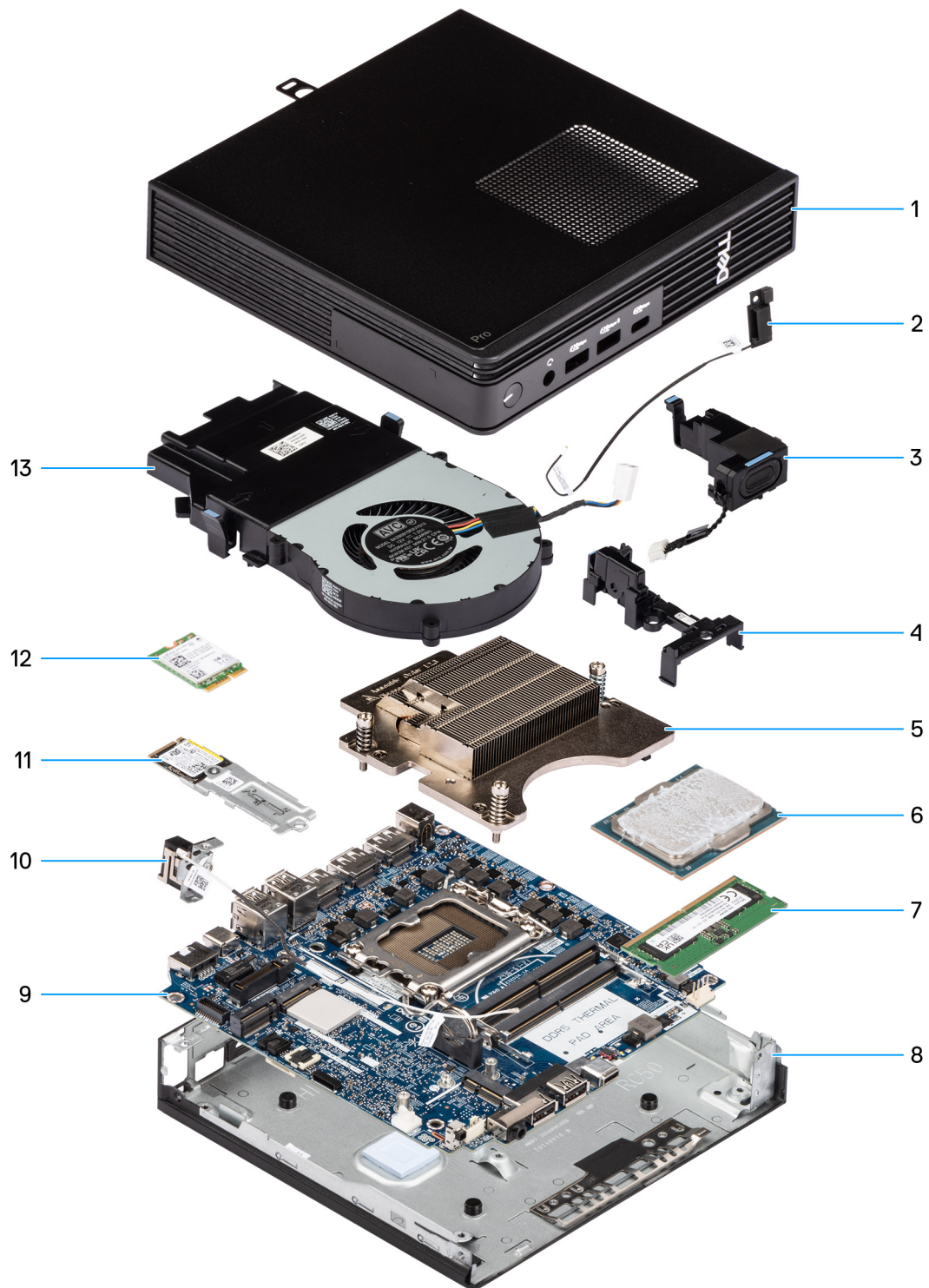
Figure 9. Principaux composants de l'ordinateur Dell Pro Micro Plus GBM1250
