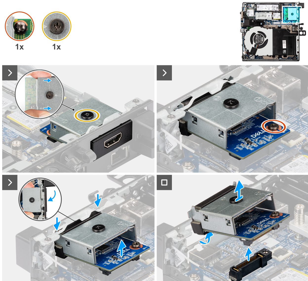
Figure 50. Retrait du module de port HDMI
