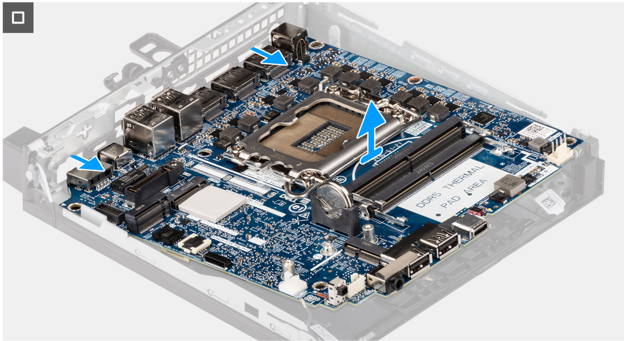
Figure 82. Retrait de la carte système
