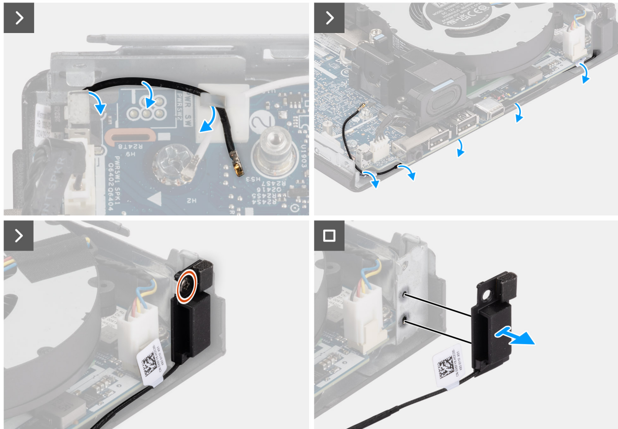
Figure 70. Retrait du module d'antenne (câble noir)
