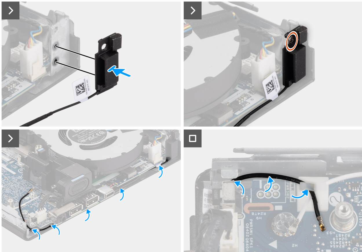
Figure 71. Installation du module d'antenne (câble noir)
