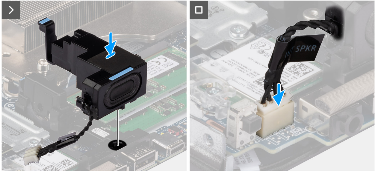
Figure 15. Installation du haut-parleur
