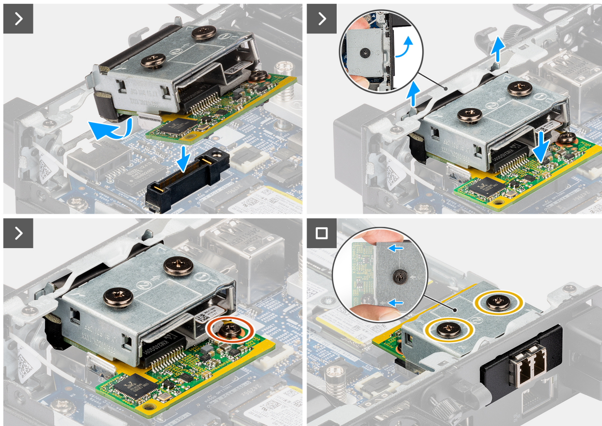
Figure 64. Installation du module de port fibre optique
