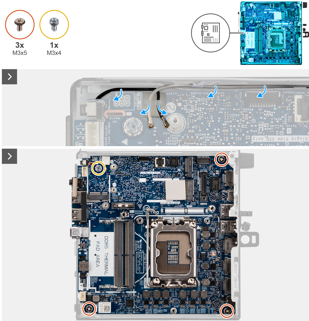
Figure 81. Retrait de la carte système
