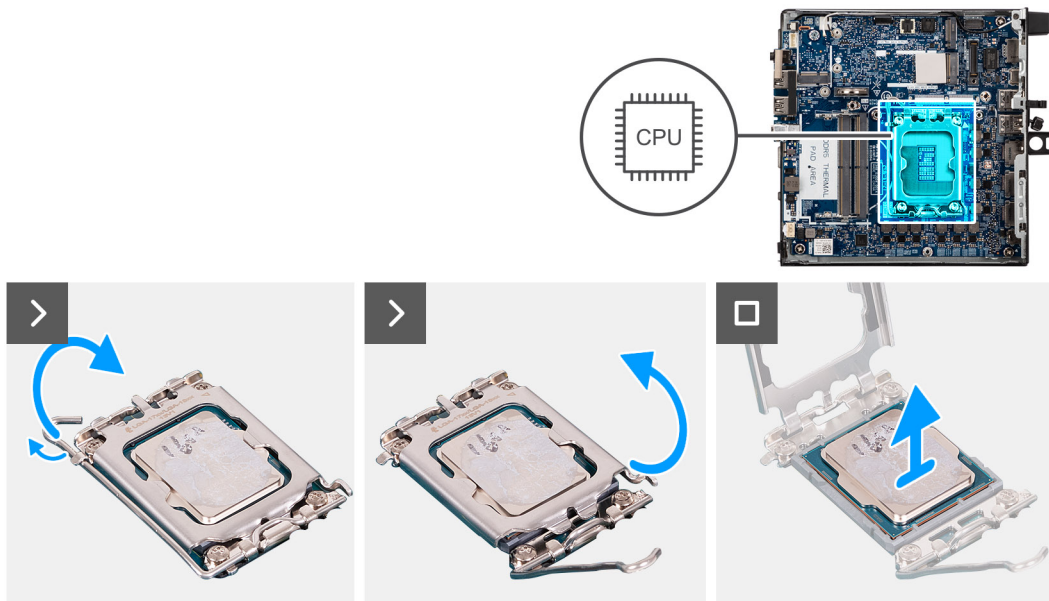
Figure 76. Retrait du processeur
