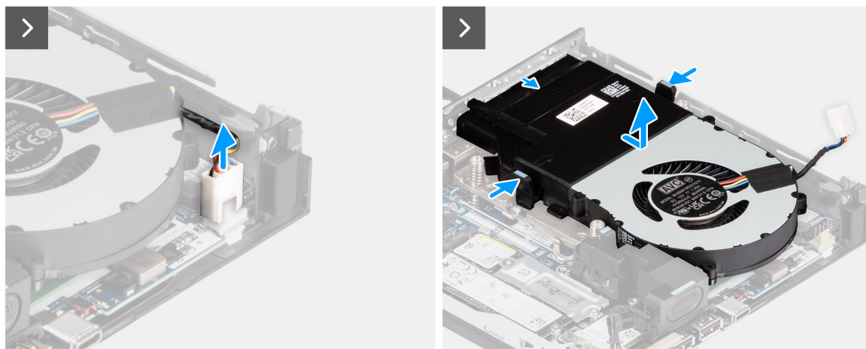
Figure 28. Retrait du ventilateur
