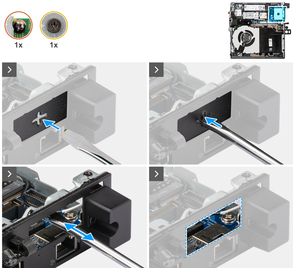
Figure 45. Installation du port Thunderbolt et du module de port USB type-C.
