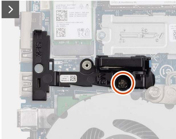
Figure 78. Retrait du support de haut-parleur
