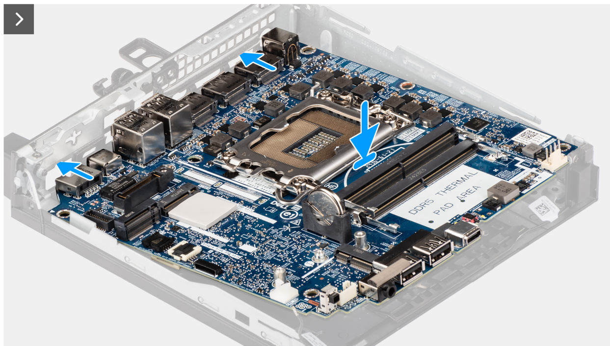
Figure 84. Installation de la carte système
