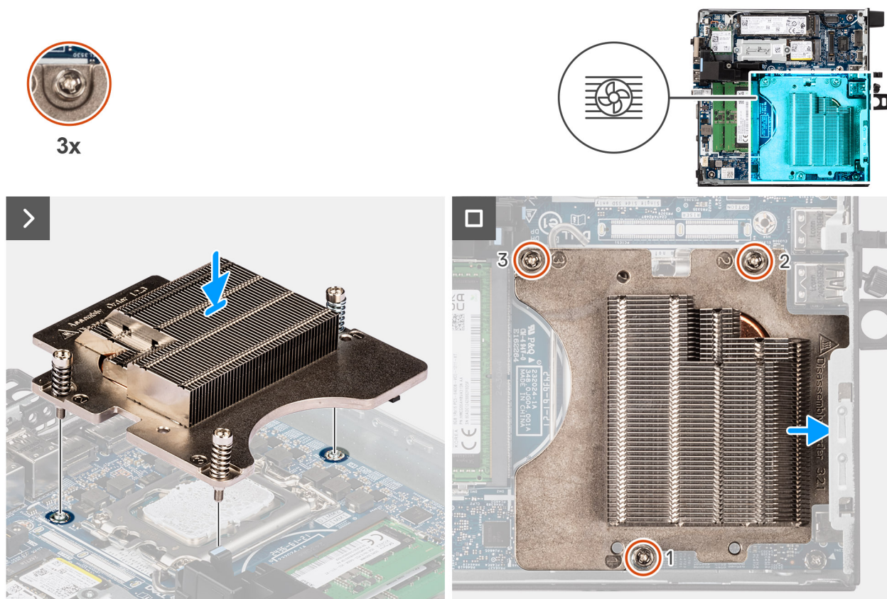
Figure 69. Installation du dissipateur de chaleur
