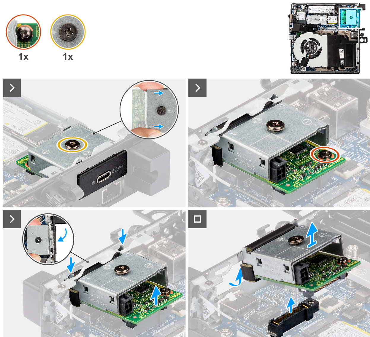
Figure 41. Installation du module de port USB-C
