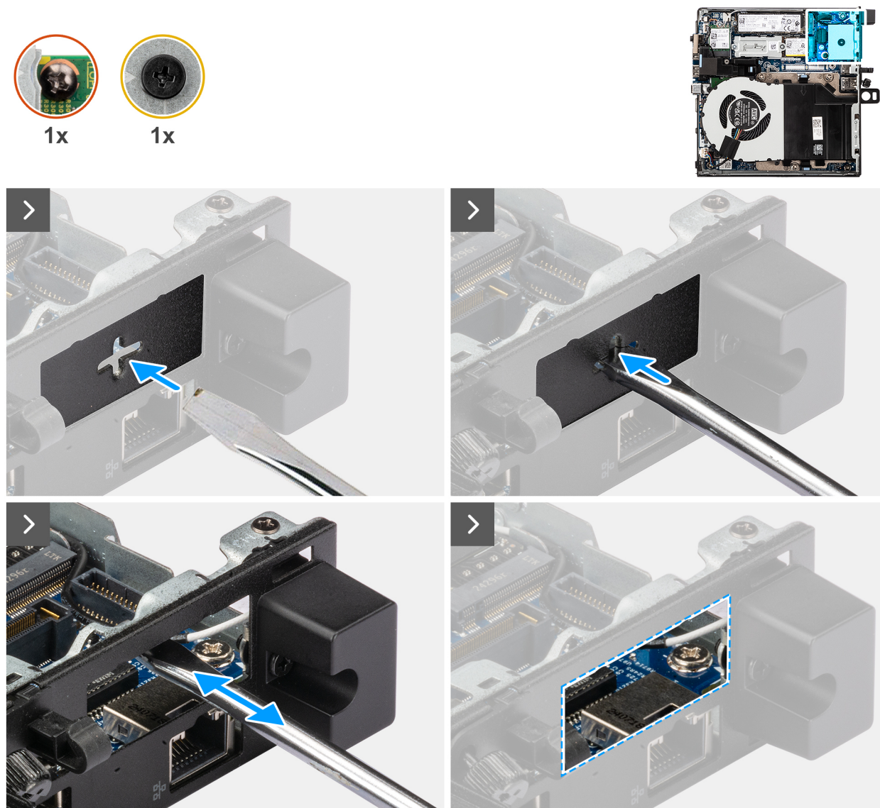
Figure 60. Installation du module de port série
