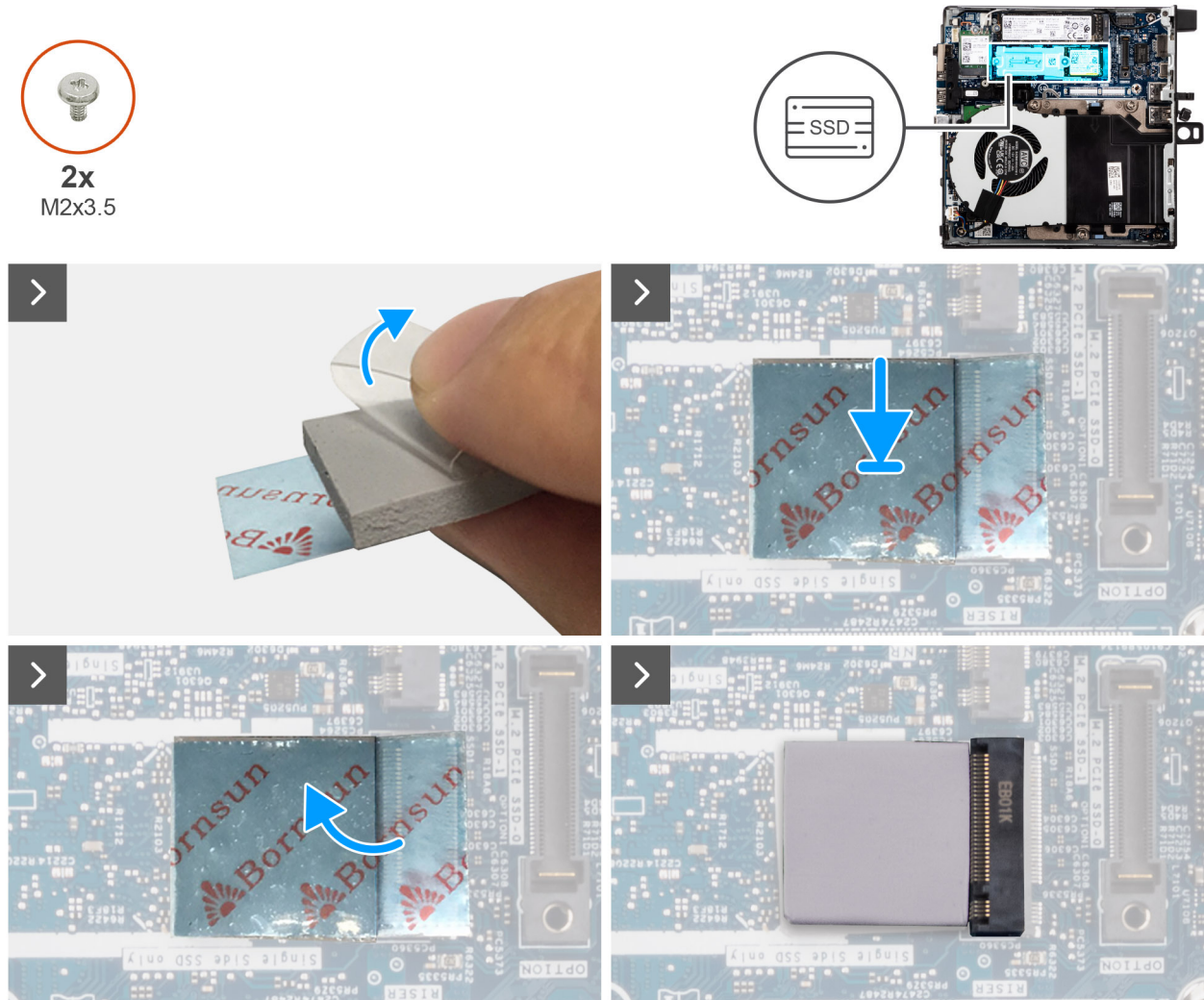
Figure 17. Installation du disque SSD 2230
