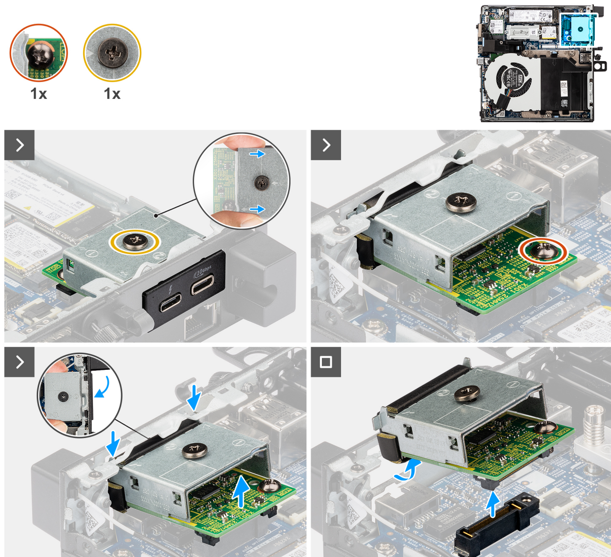
Figure 44. Retrait du port Thunderbolt et du module de port USB type-C.
