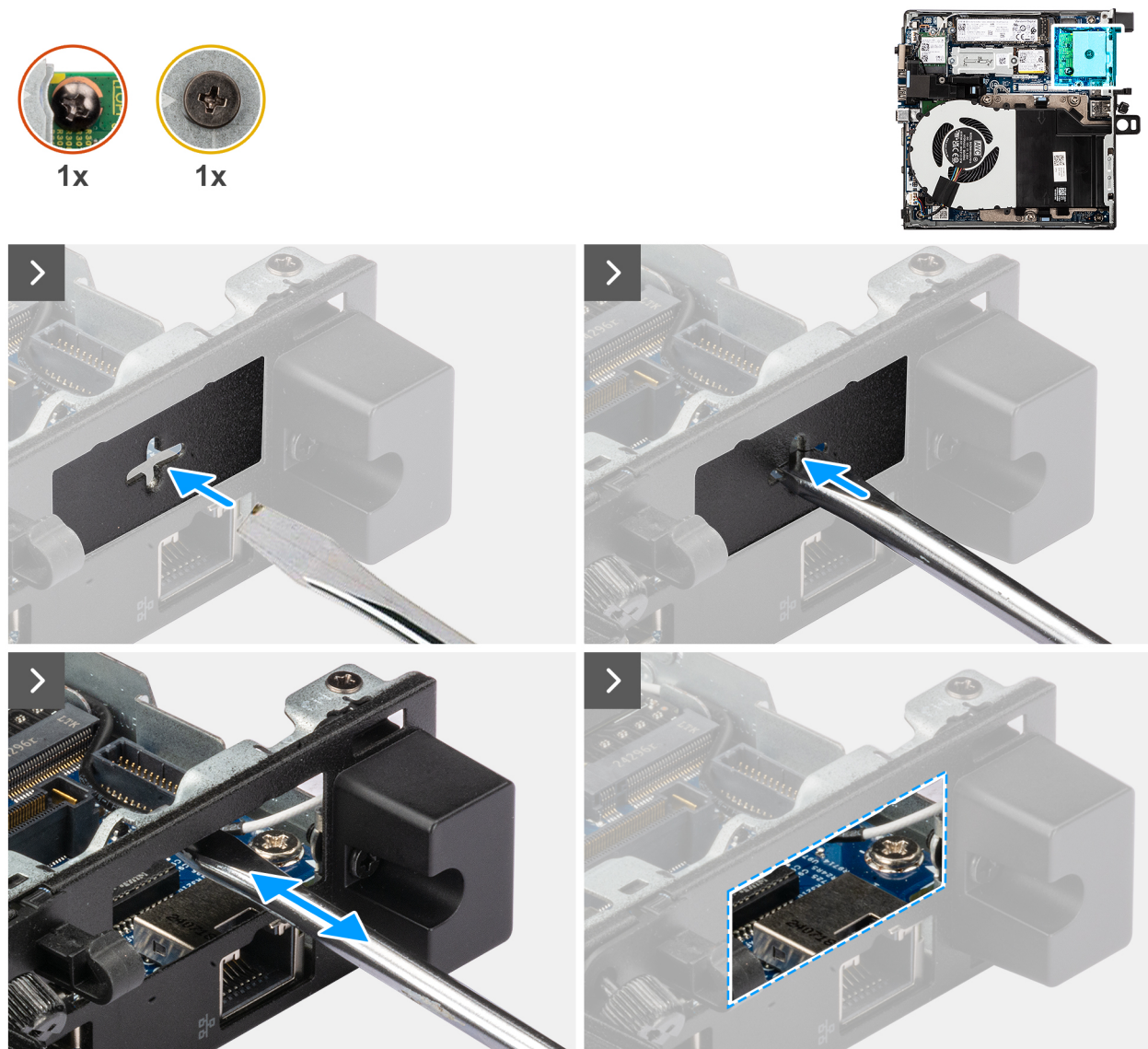
Figure 48. Installation du module DisplayPort
