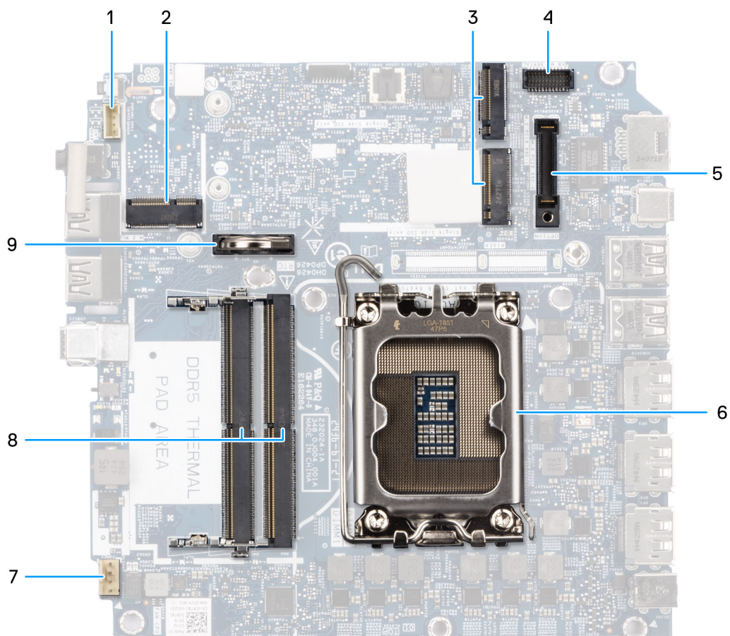
Figure 80. Connecteurs de la carte système
