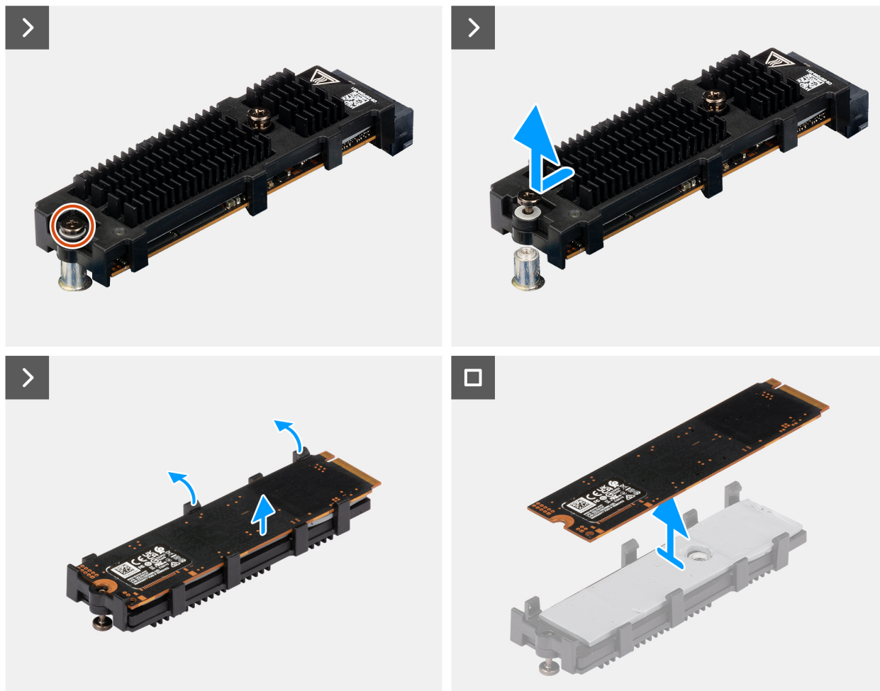
Figure 24. Retrait du disque SSD M.2 2280 PCIe
