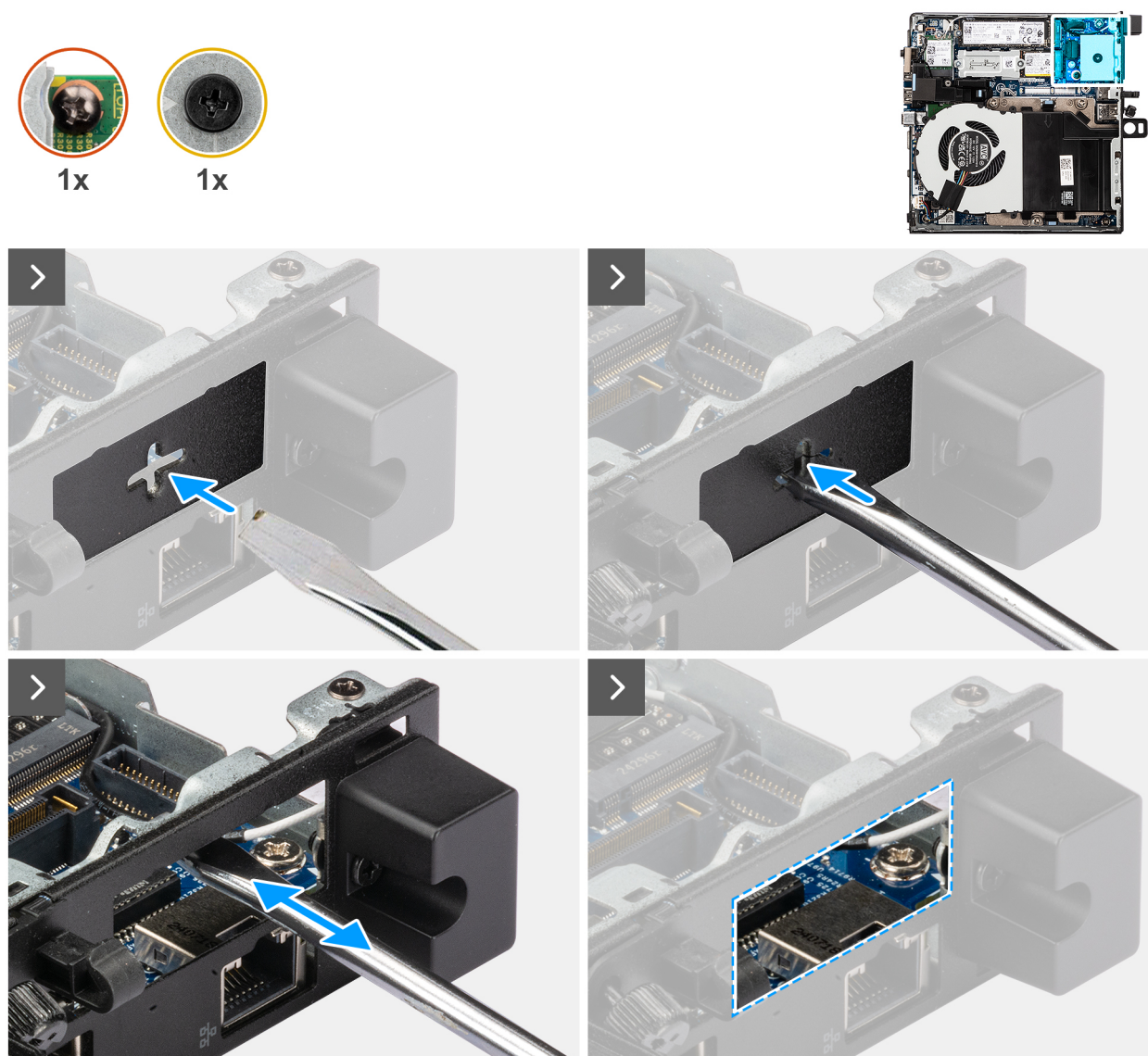
Figure 57. Installation du module de port PS2
