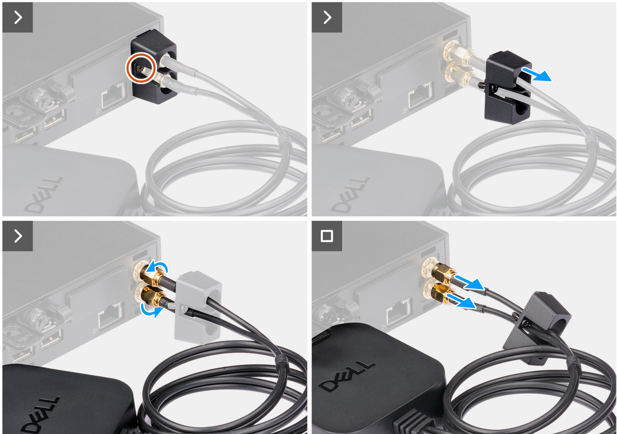
Figure 34. Retrait de l'antenne Puck externe
