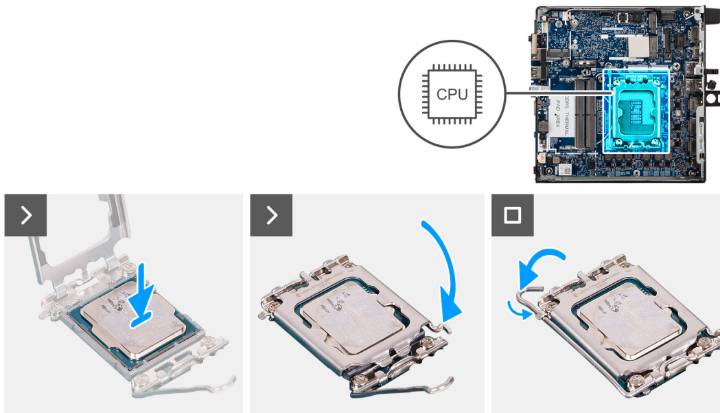
Figure 77. Installation du processeur
