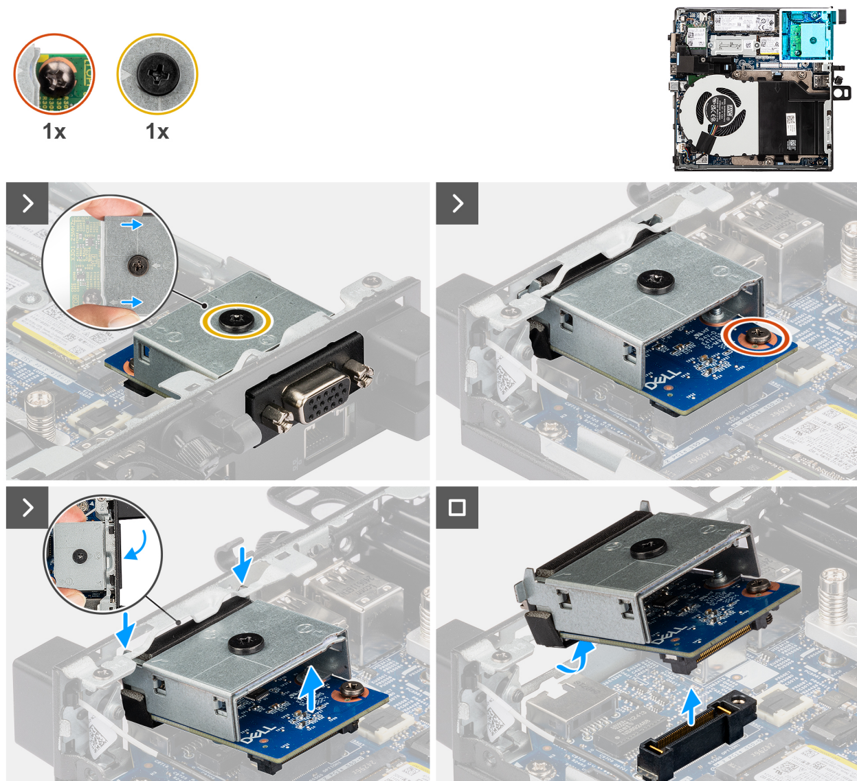
Figure 53. Retrait du module de port VGA
