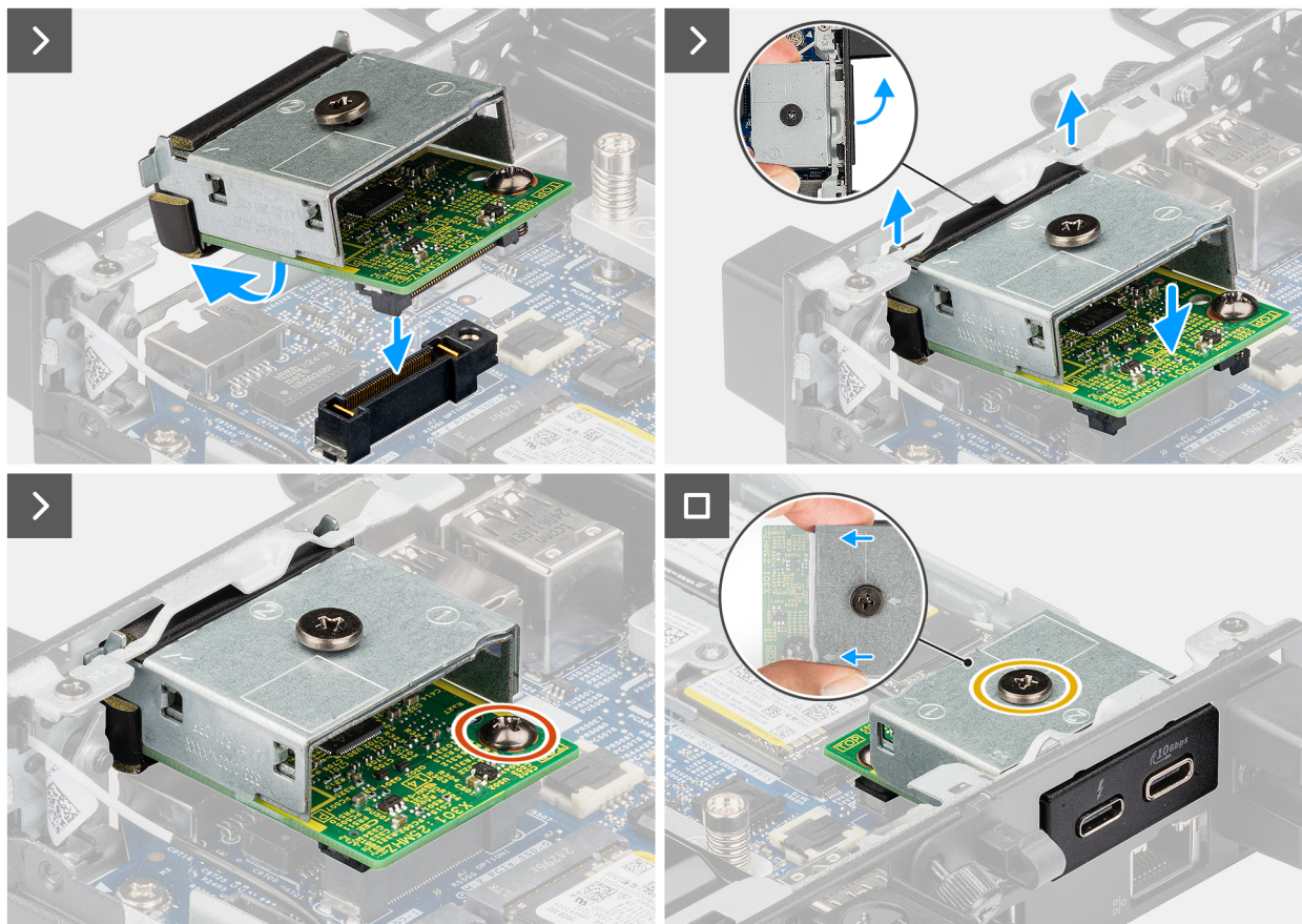
Figure 46. Installation du port Thunderbolt et du module de port USB type-C.
