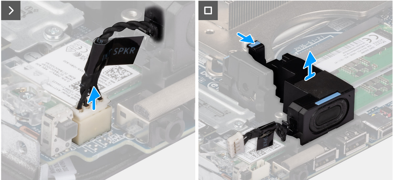
Figure 14. Retrait du haut-parleur
