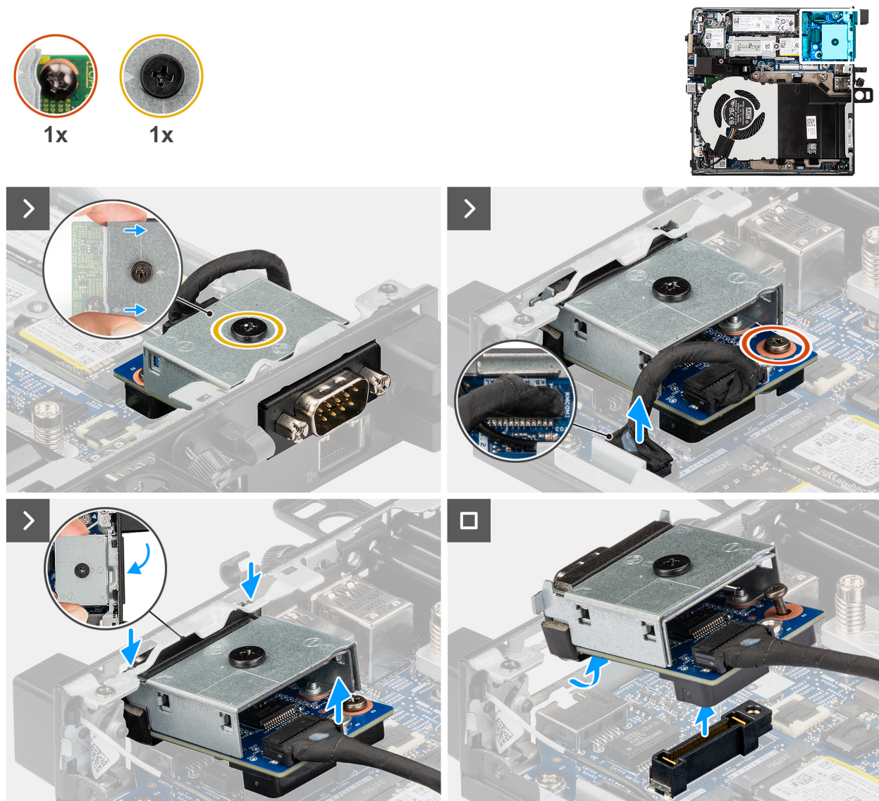
Figure 59. Retrait du module de port série
