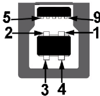
Abbildung 6. USB 5Gbps Type-B Upstream-Port
