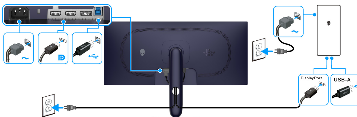
Abbildung 24. DisplayPort Verbindung
