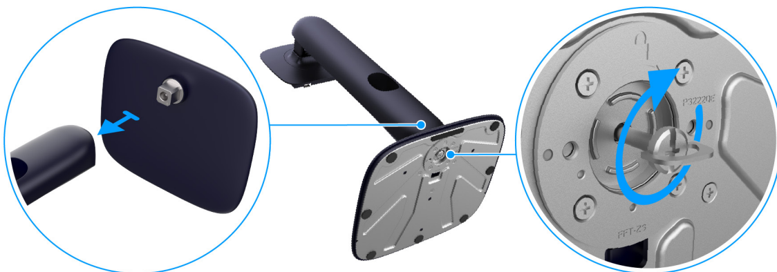
Abbildung 15. Ständerarm am Ständersockel befestigen
