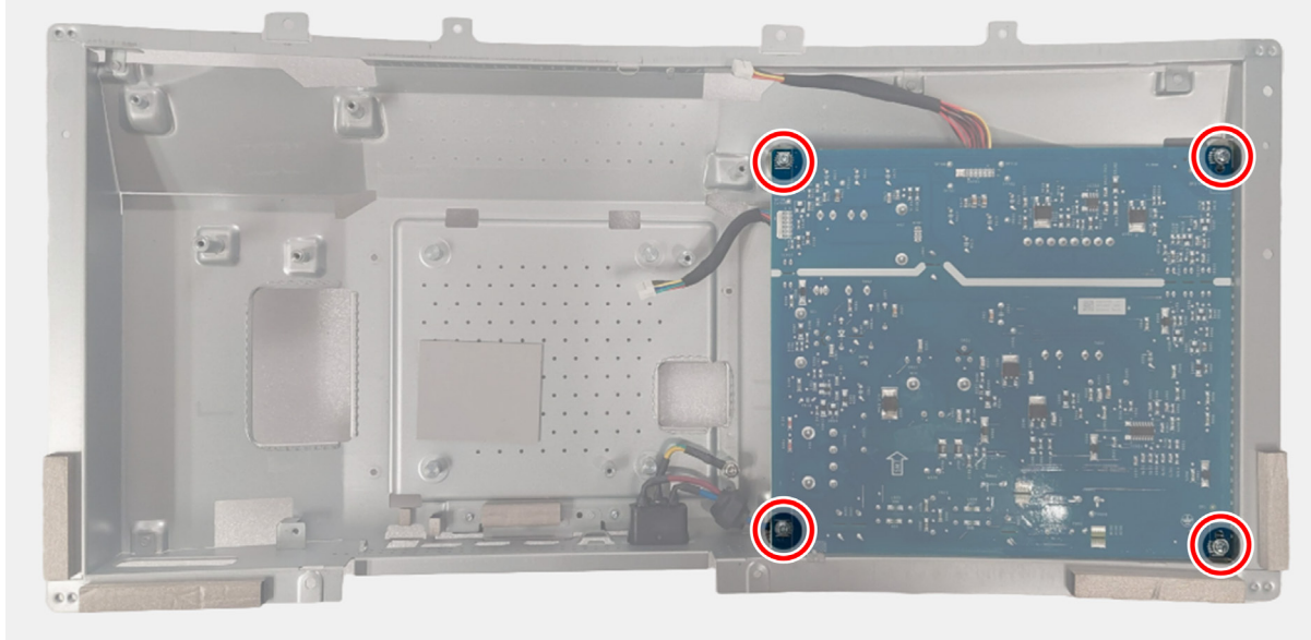
Obrázek 34. Instalace napájecí desky
