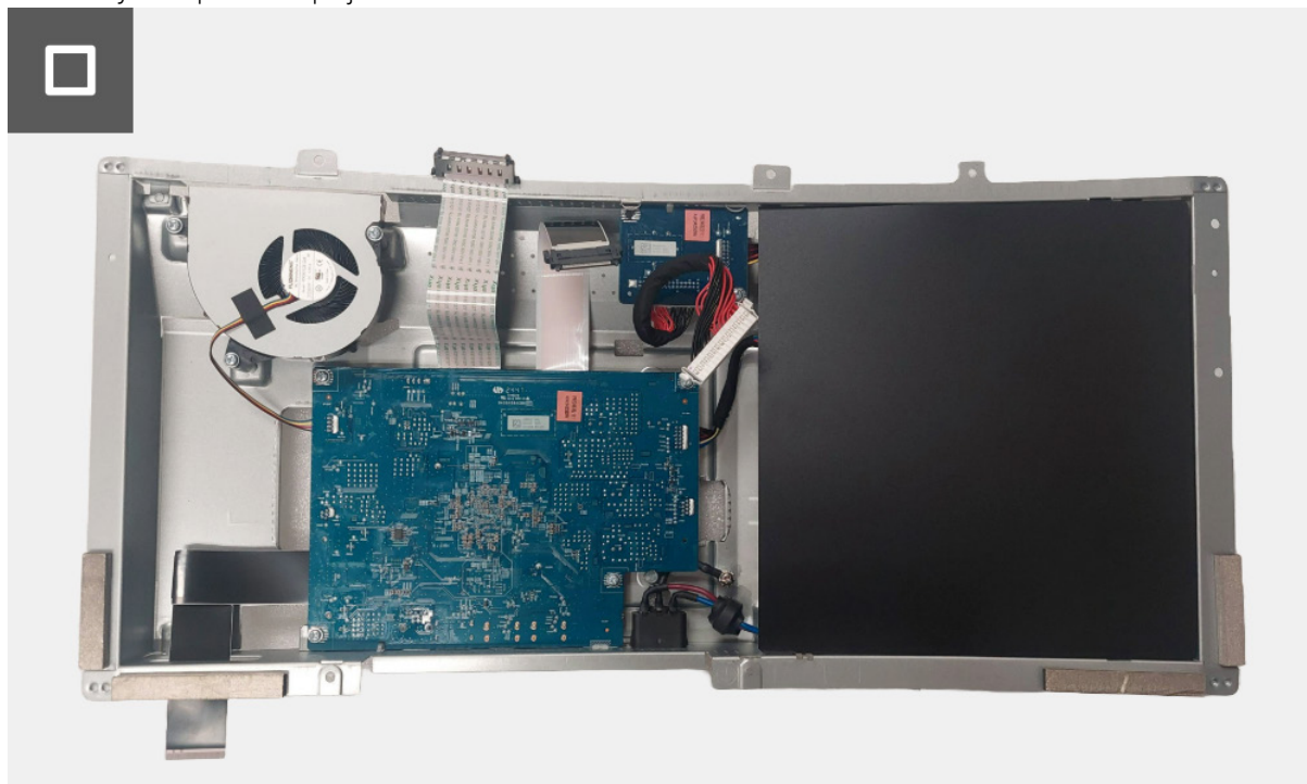
Obrázek 13. Demontáž kovového štítu
