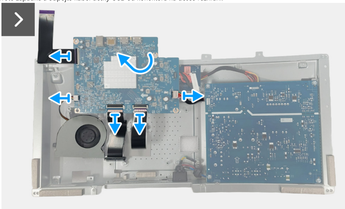
Obrázek 19. Demontáž desky rozhraní
