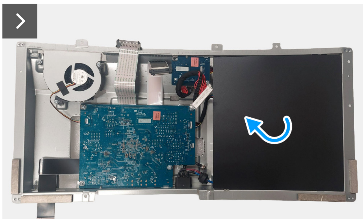
Obrázek 17. Demontáž desky rozhraní
