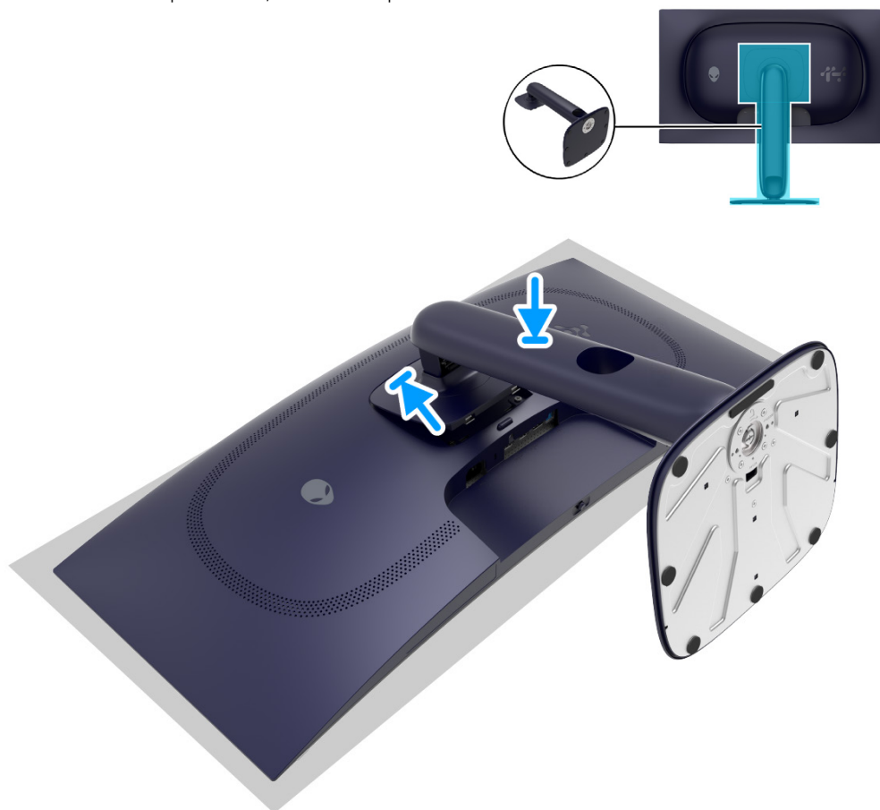
Obrázek 3. Instalace podstavce
