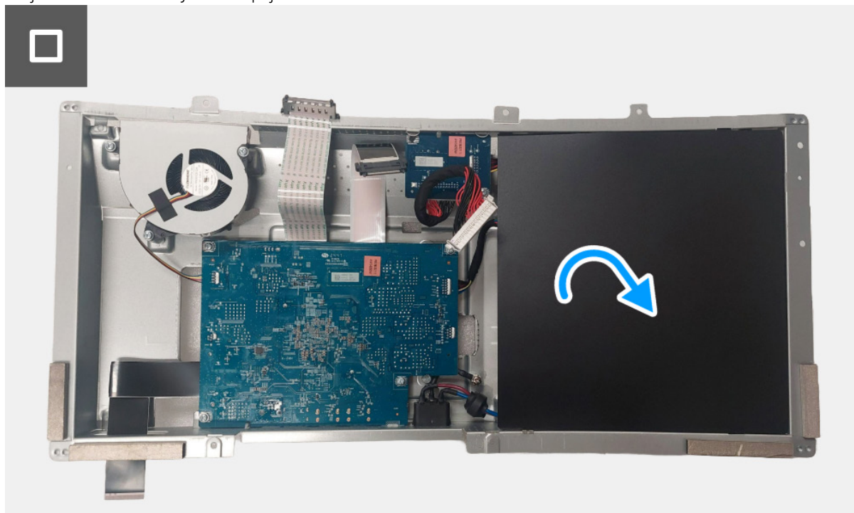
Obrázek 24. Instalace desky rozhraní
