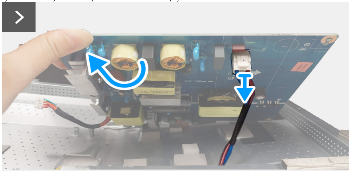
Obrázek 30. Demontáž napájecí desky
