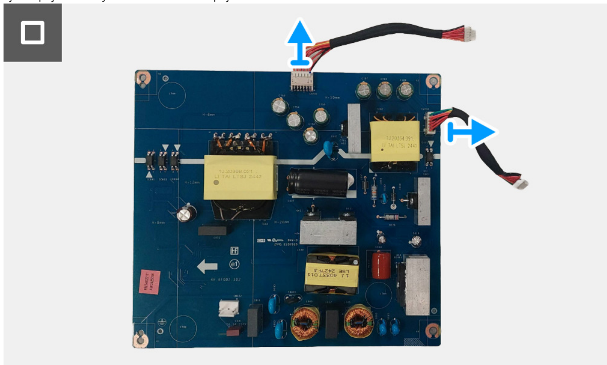
Obrázek 31. Demontáž napájecí desky
