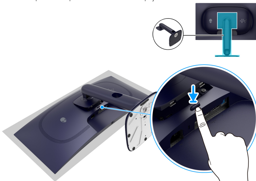
Obrázek 1. Demontáž podstavce
