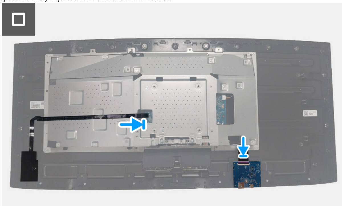
Obrázek 16. Instalace kovového štítu
