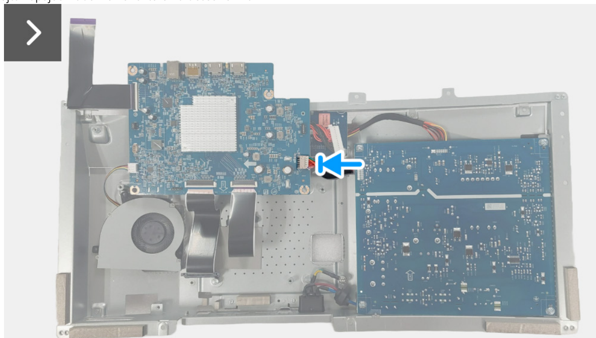
Obrázek 22. Instalace desky rozhraní
