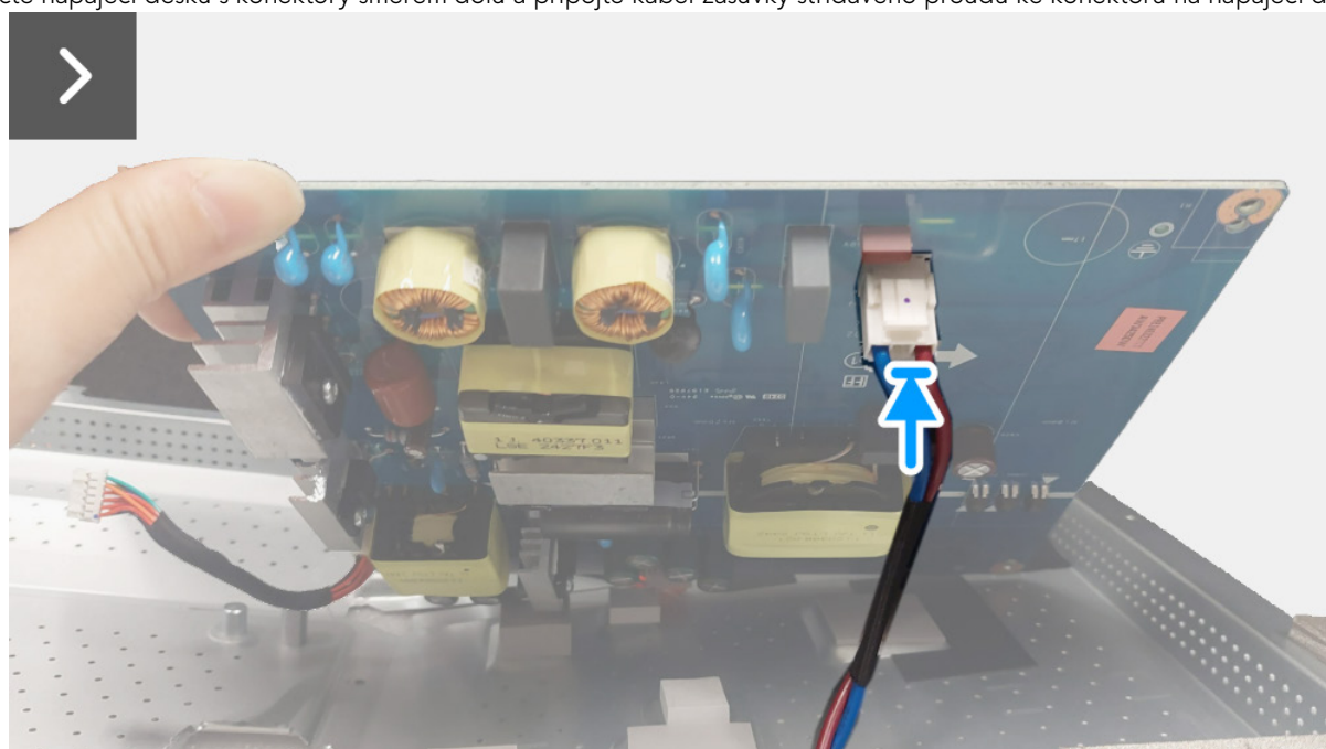
Obrázek 33. Instalace napájecí desky
