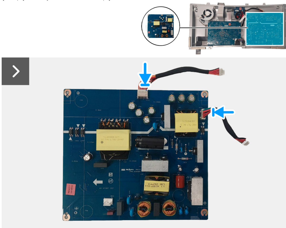
Obrázek 32. Instalace napájecí desky
