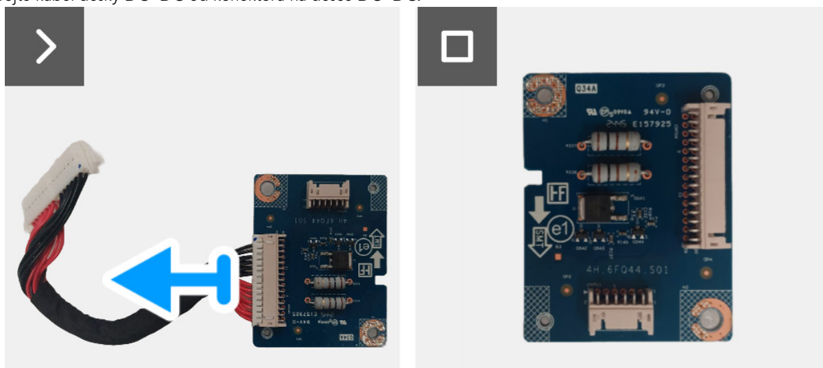
Obrázek 26. Demontáž desky DC-DC
