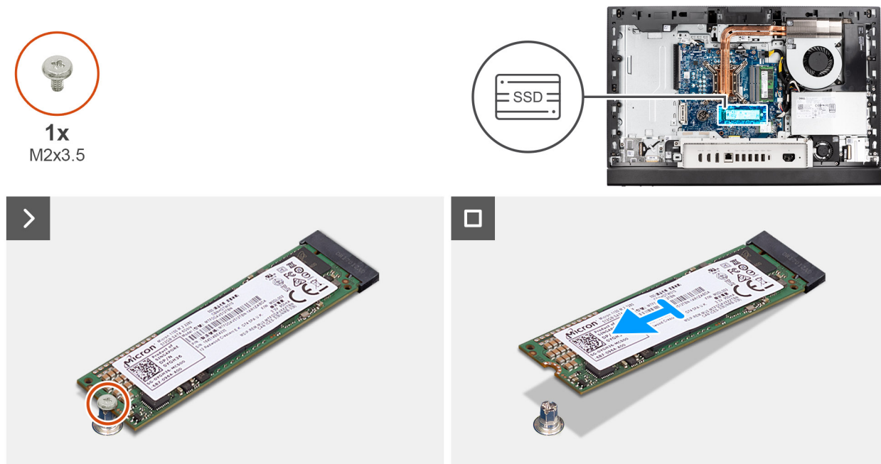
Figure 35. Retrait du disque SSD M.2 2280 du logement M.2 0
