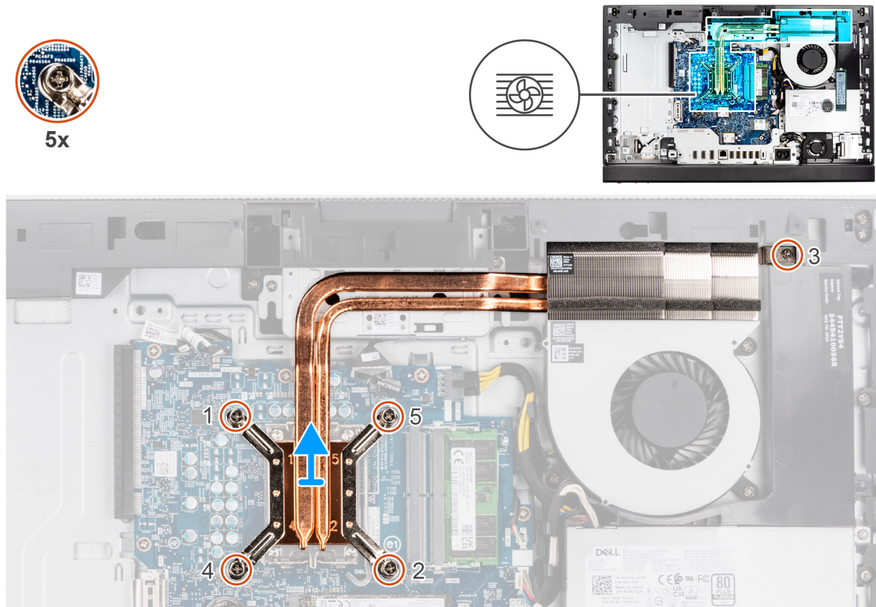
Figure 61. Retrait du dissipateur de chaleur
