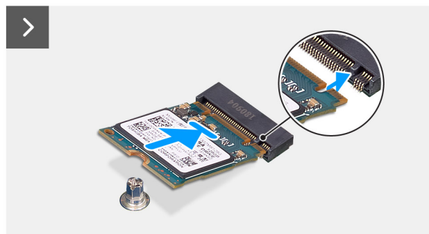
Figure 39. Installation du disque SSD M.2 2230 dans le logement M.2 1
