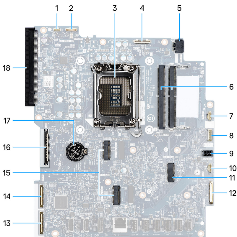
Figure 65. Légendes de la carte système
