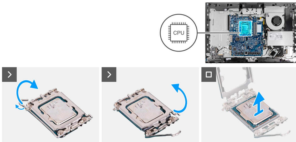
Figure 63. Retrait du processeur
