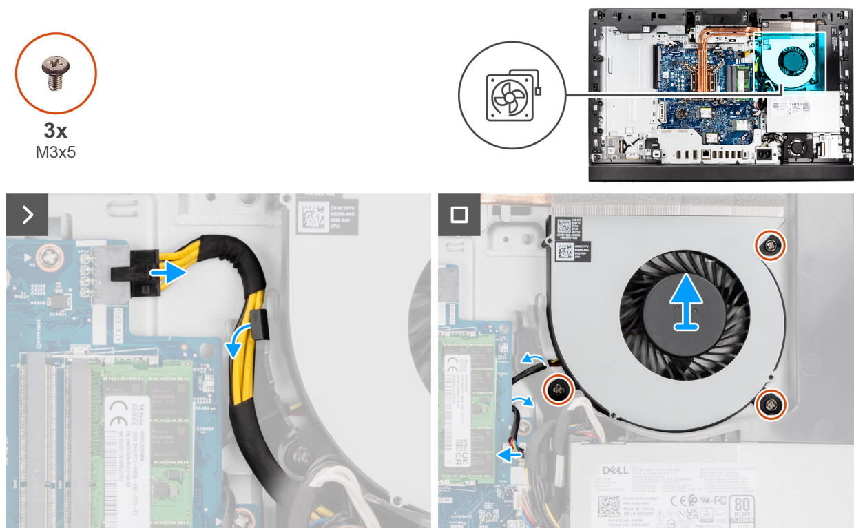
Figure 51. Retrait du ventilateur
