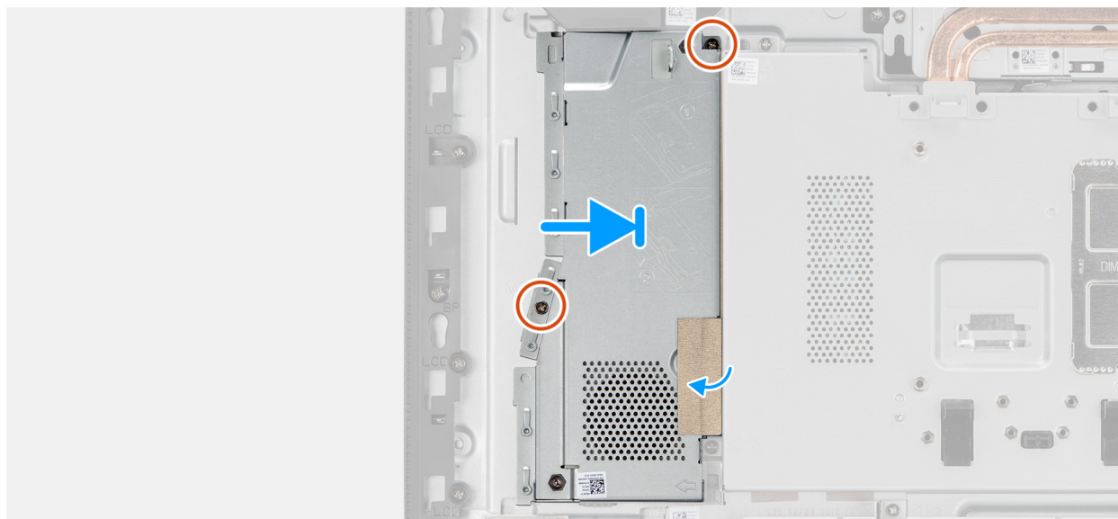
Figure 28. Installation de l'assemblage de carte graphique (modèle non tactile)
