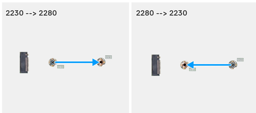
Figure 37. Déplacement du support de vis du Disque SSD pour le logement M.2 0
