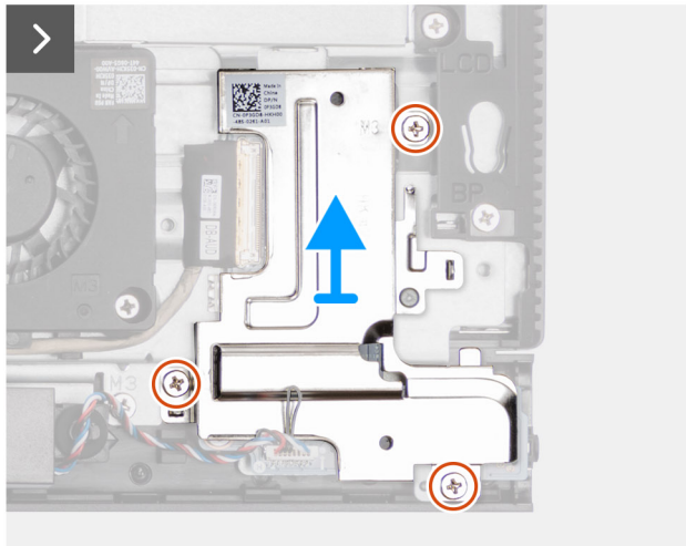
Figure 73. Retrait de la carte audio
