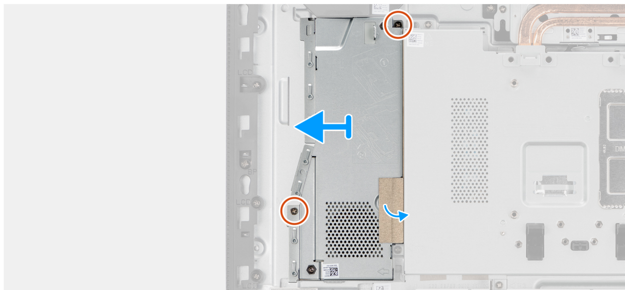
Figure 25. Retrait de l'assemblage de carte graphique (modèle tactile)
