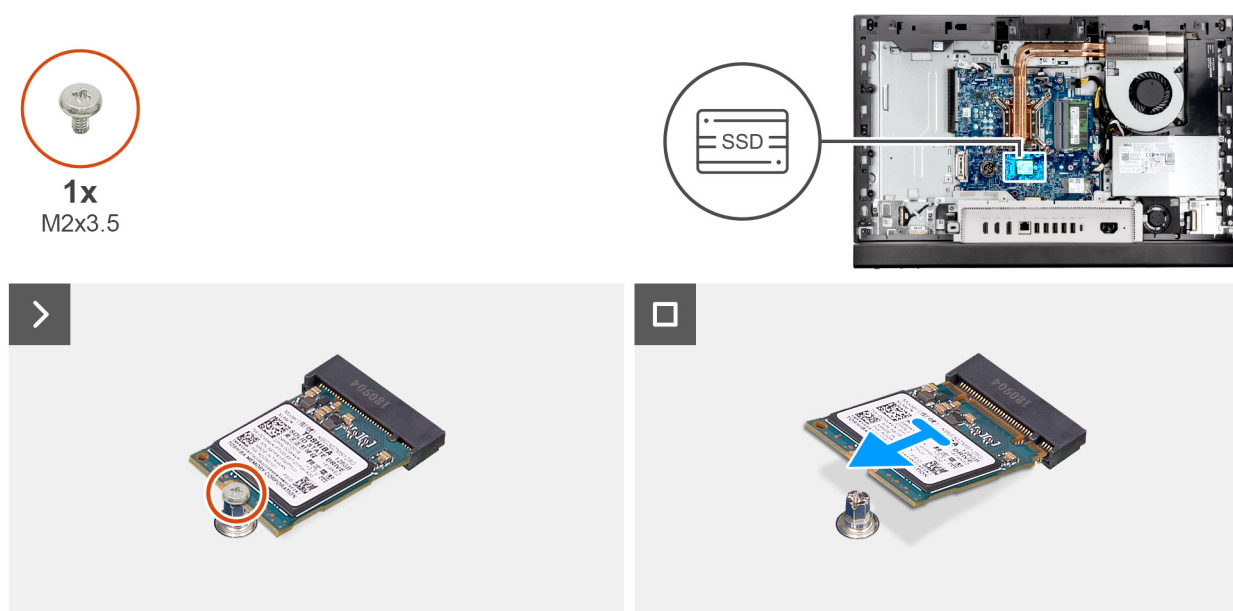
Figure 33. Retrait du disque SSD M.2 2230 du logement M.2 0
