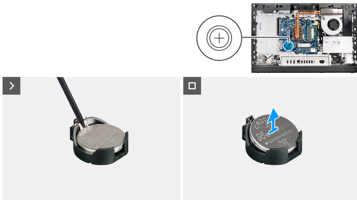
Figure 43. Retrait de la pile bouton
