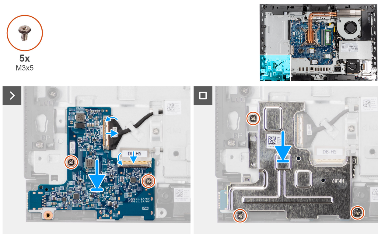
Figure 72. Installation du bouton d'alimentation et de la carte d'E/S
