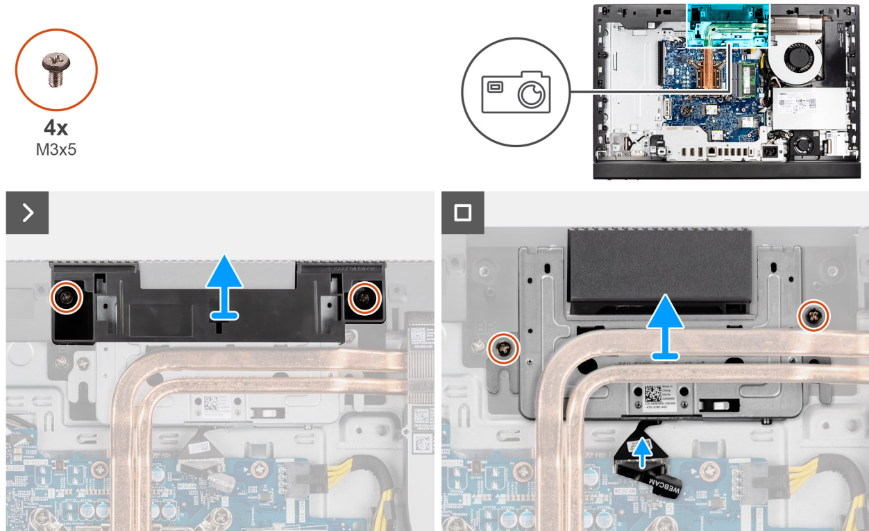
Figure 49. Retrait de l'assemblage de la caméra escamotable
