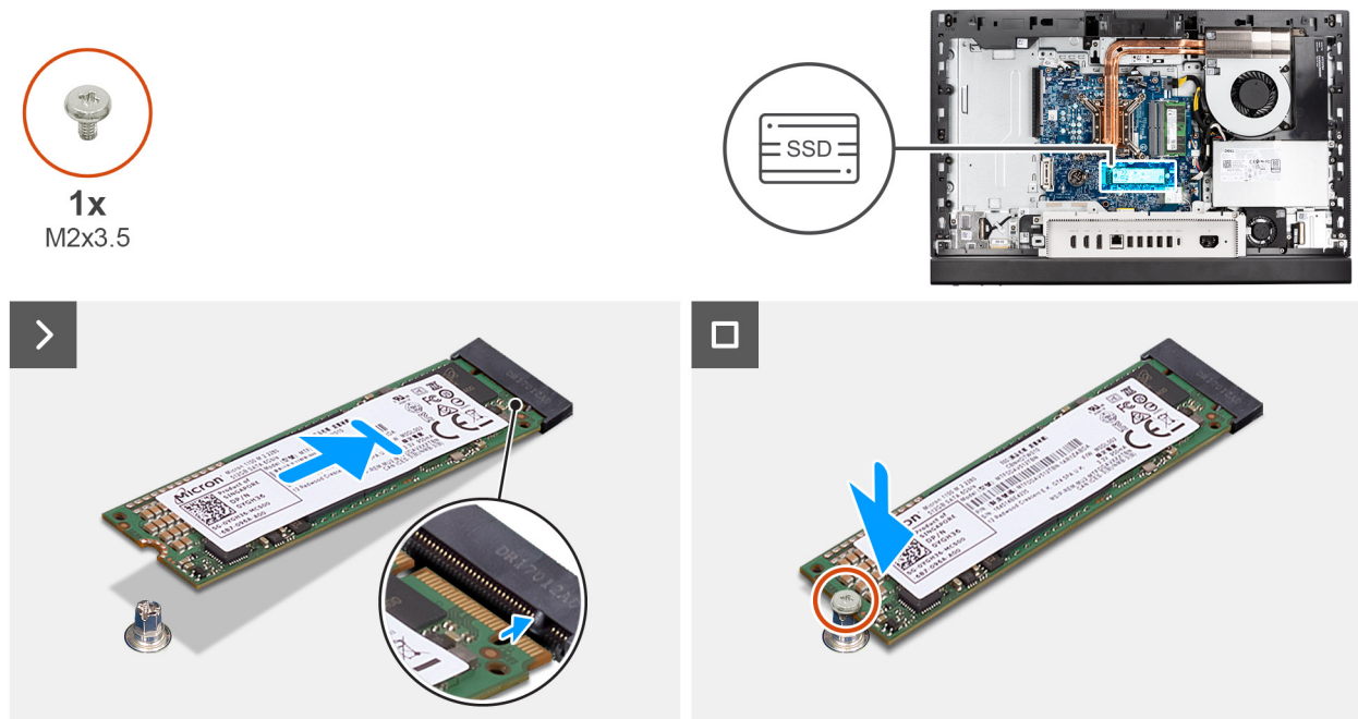
Figure 36. Installation du disque SSD M.2 2280 dans le logement M.2 0
