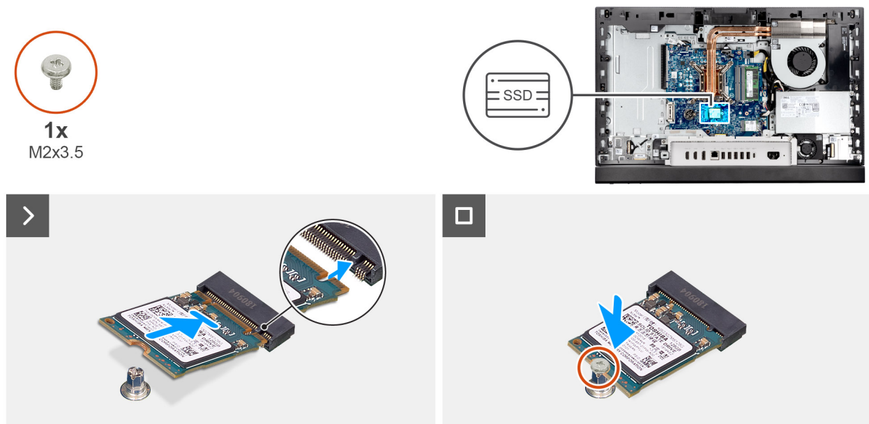
Figure 34. Installation du disque SSD M.2 2230 dans le logement M.2 0
