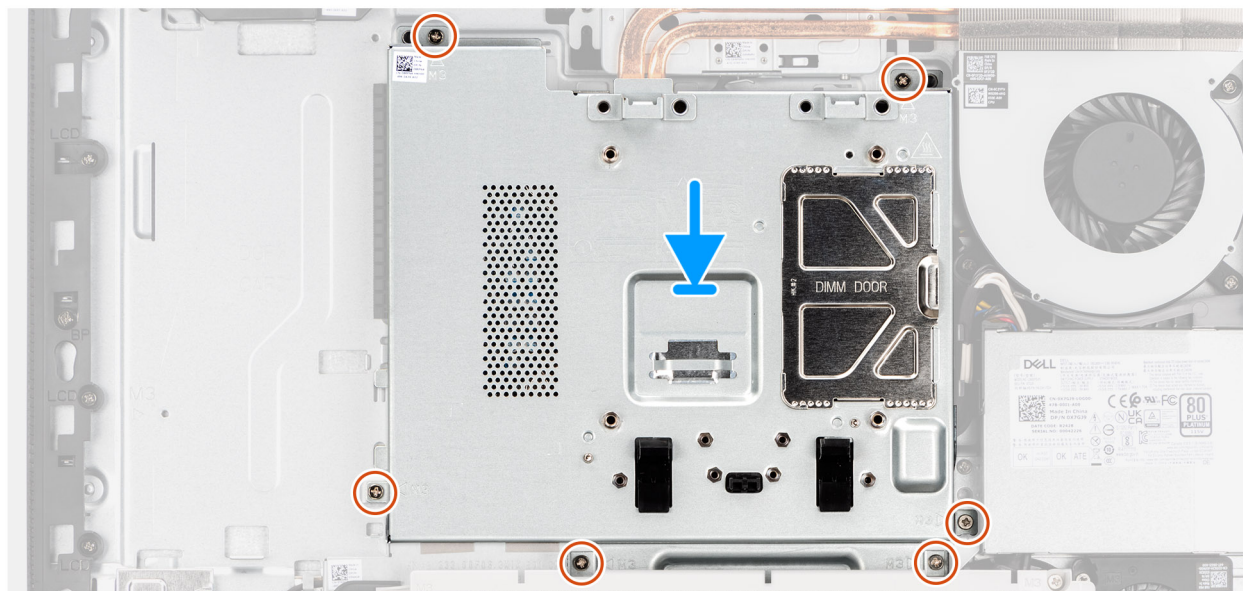
Figure 30. Pose de la protection de la carte système
