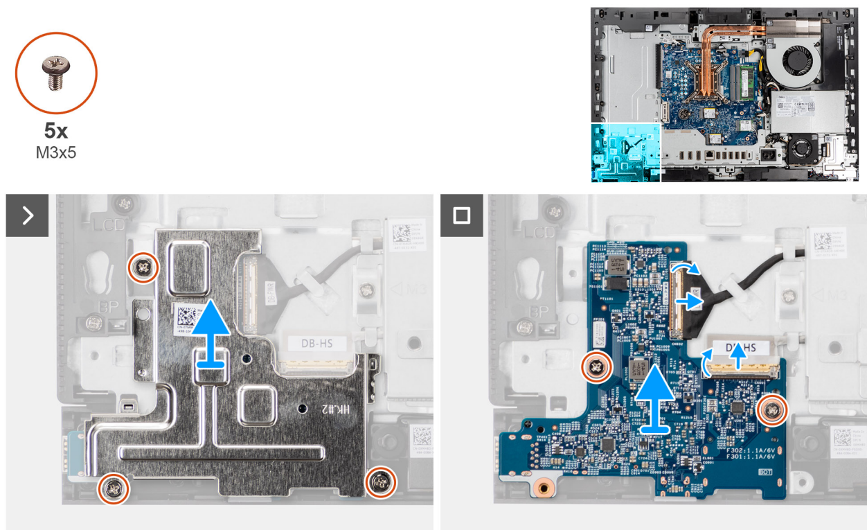
Figure 71. Retrait de la carte du bouton d'alimentation et de la carte d'E/S
