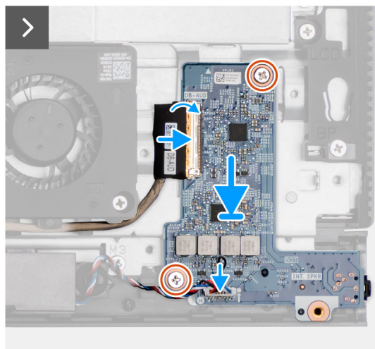
Figure 74. Installation de la carte audio
