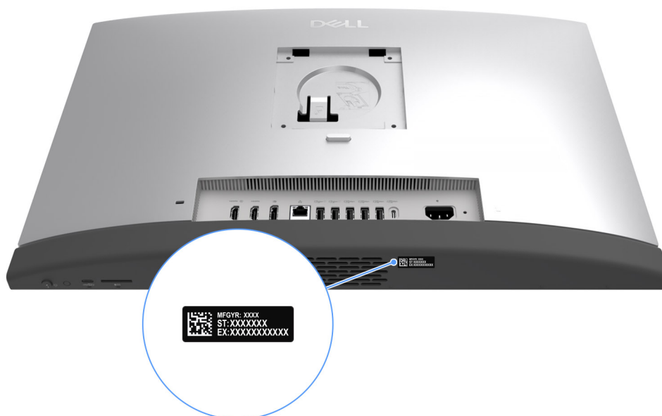
Figure 9. Emplacement de l'étiquette de service de votre ordinateur Tout-en-un Dell Pro 24 plus QB24250
