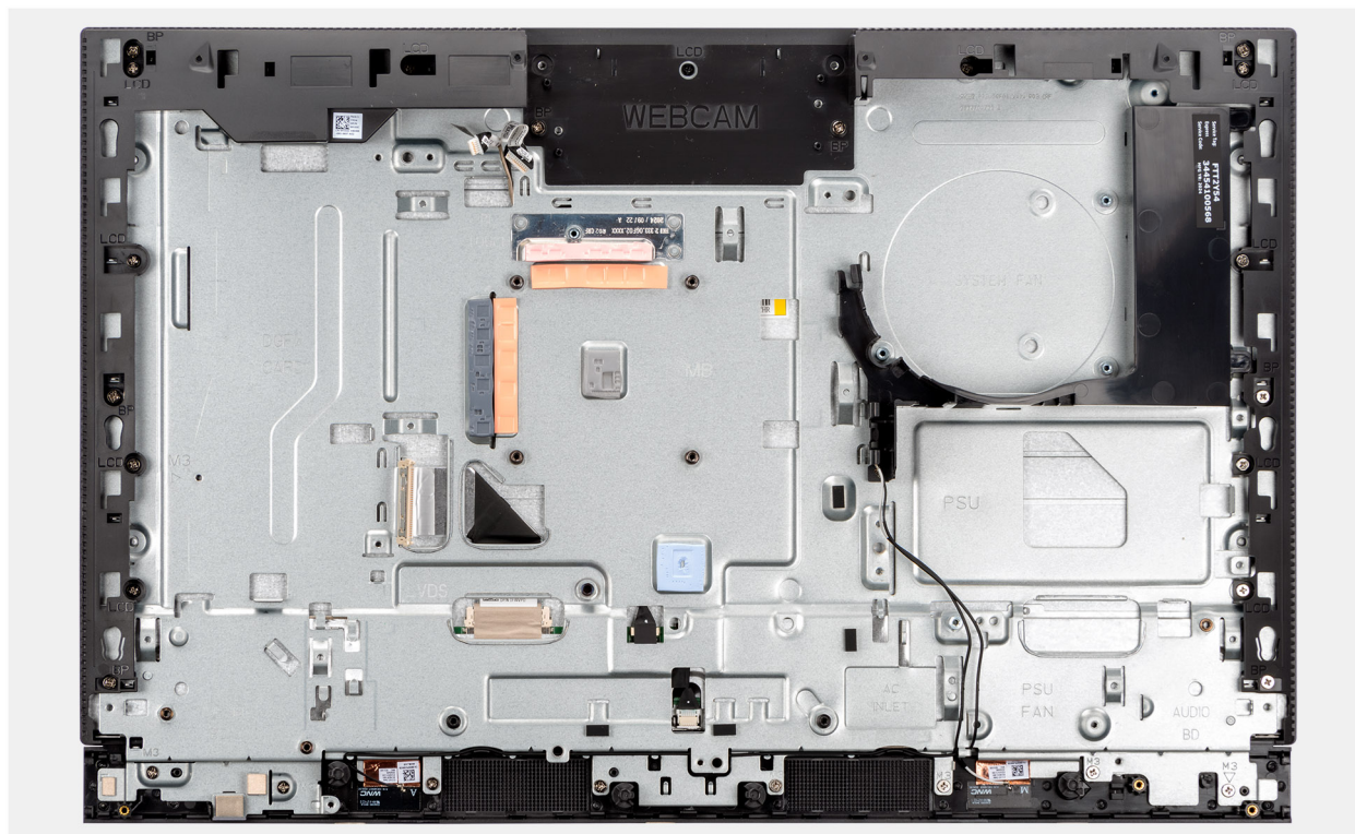
Figure 75. Retrait de la base de l'assemblage d'écran
