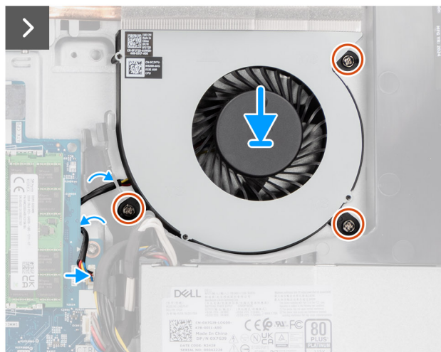
Figure 52. Installation du ventilateur
