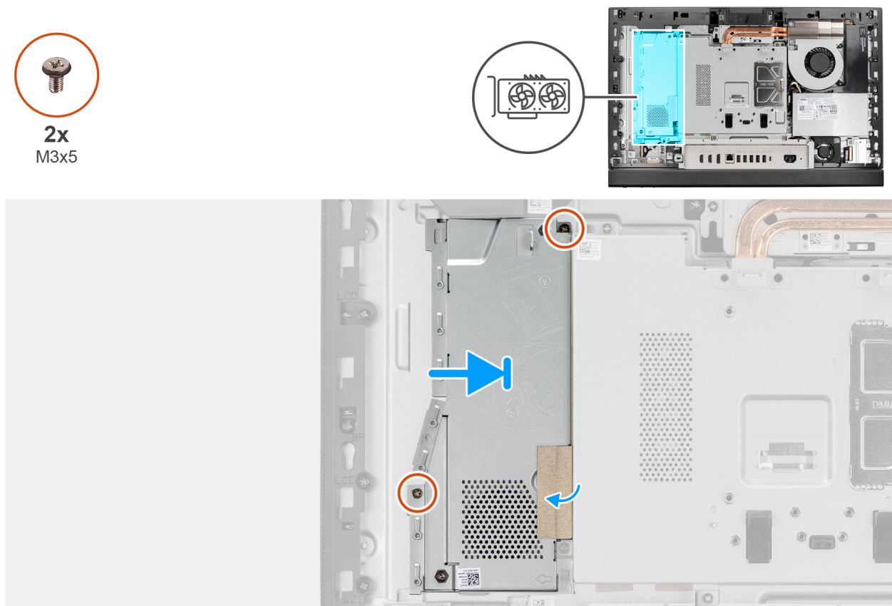
Figure 27. Installation de l'assemblage de carte graphique (modèle tactile)
