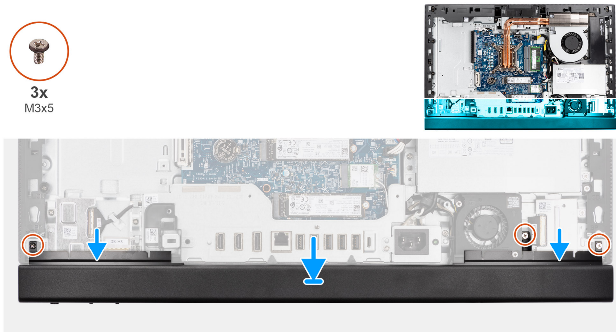
Figure 48. Installation du capot inférieur
