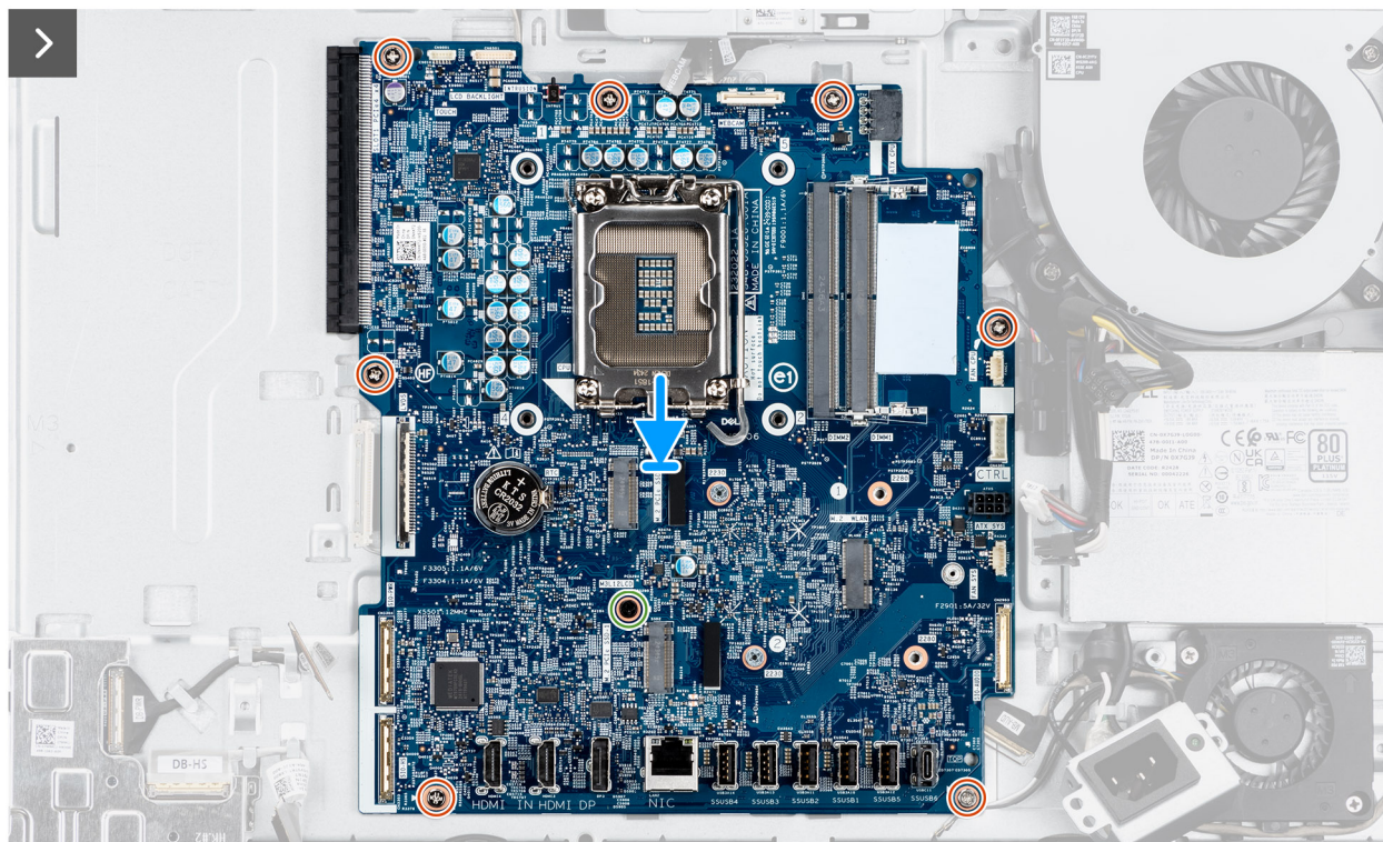
Figure 69. Installation de la carte système
