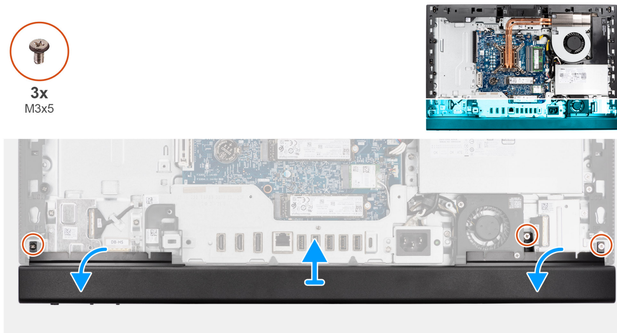
Figure 47. Retrait du cache inférieur
