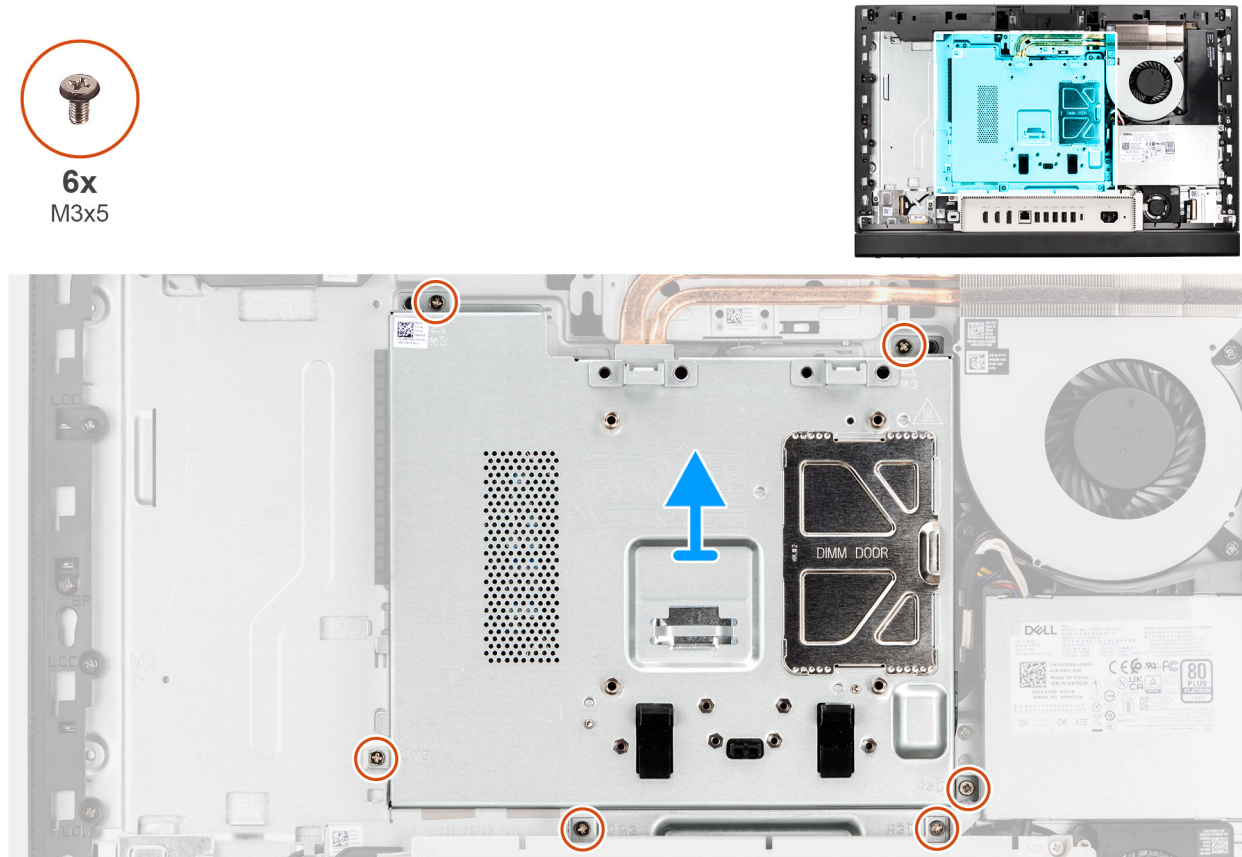
Figure 29. Retrait de la protection de la carte système
