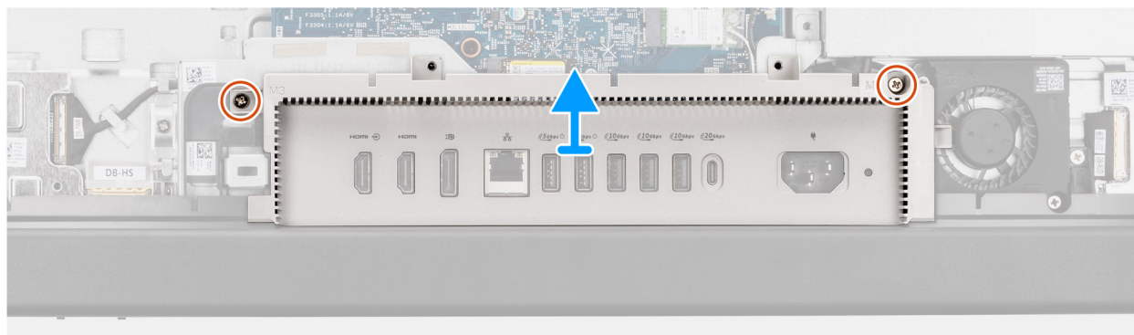
Figure 45. Retrait du cache d'E/S
