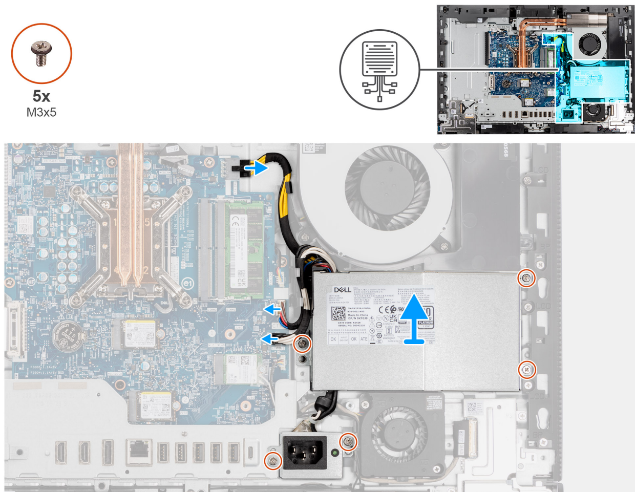
Figure 53. Retrait du bloc d'alimentation
