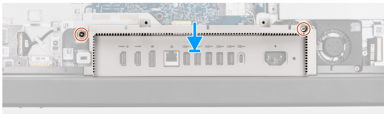
Figure 46. Installation du cache d'E/S
