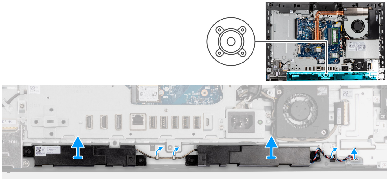
Figure 59. Retrait des haut-parleurs
