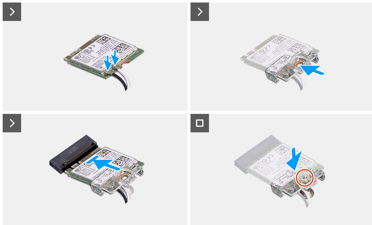
Figure 32. Installation de la carte sans fil
