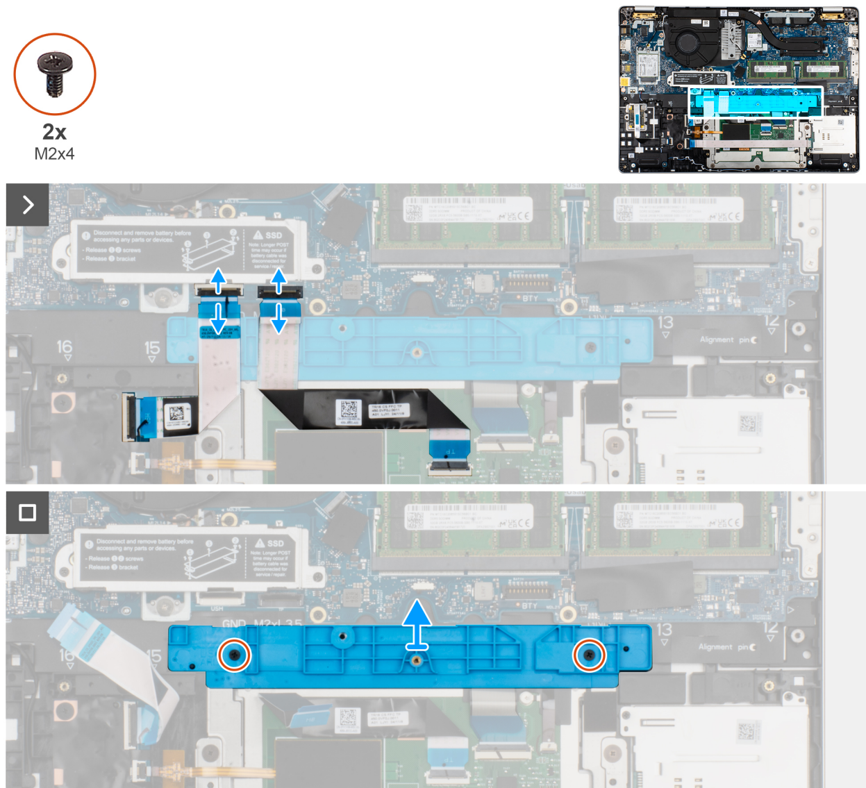
Figure 45. Retrait du support de la batterie
