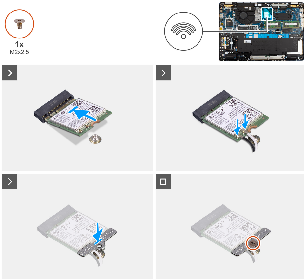
Figure 34. Installation de la carte WLAN
