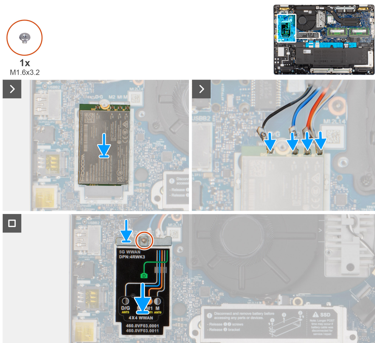
Figure 32. Installation de la carte WWAN 5G
