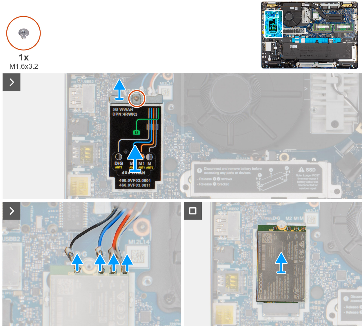
Figure 30. Retrait de la carte WWAN 5G
