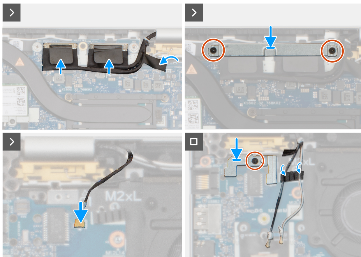
Figure 44. Installation de l'antenne WLAN
