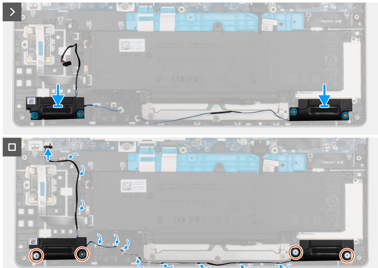
Figure 37. Installation des haut-parleurs
