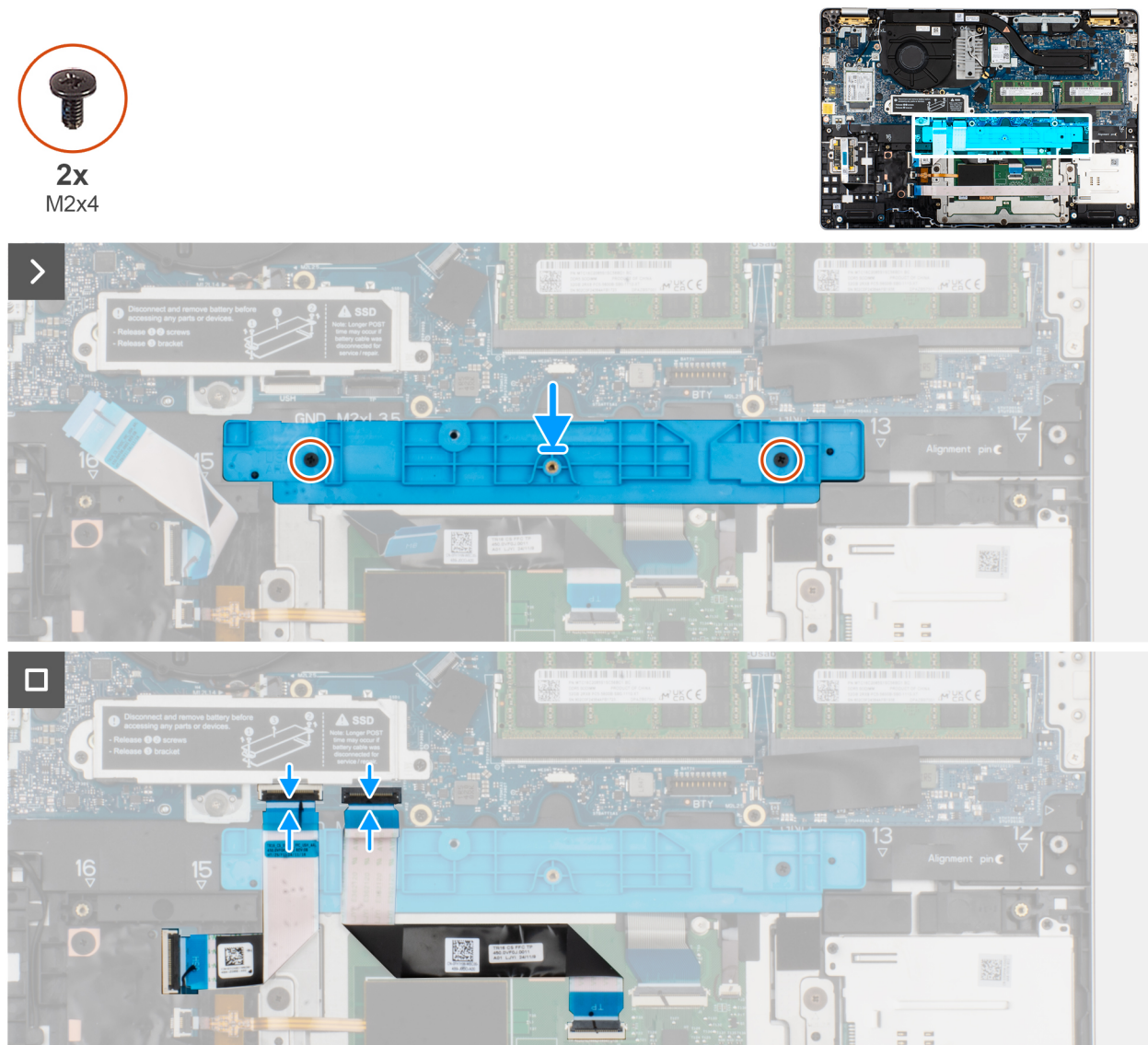
Figure 46. Installation du support de la batterie
