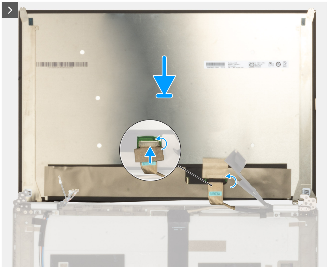
Figure 69. Installation du panneau d'écran
