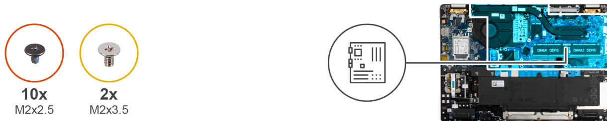
Figure 50. Retrait de la carte
