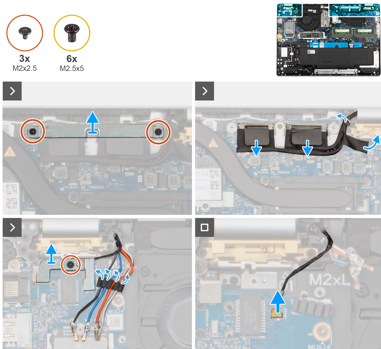
Figure 58. Retrait de l'assemblage d'écran
