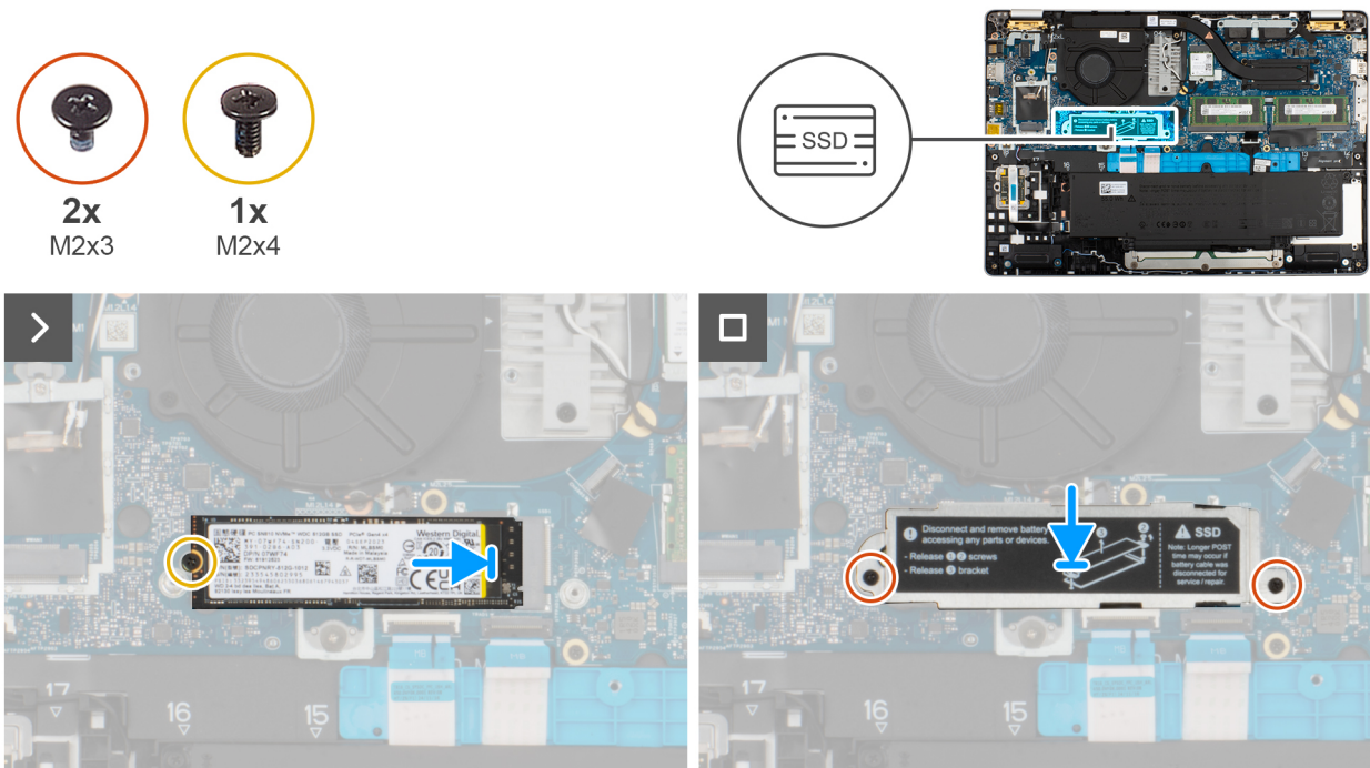
Figure 28. Installation du disque SSD M.2230
