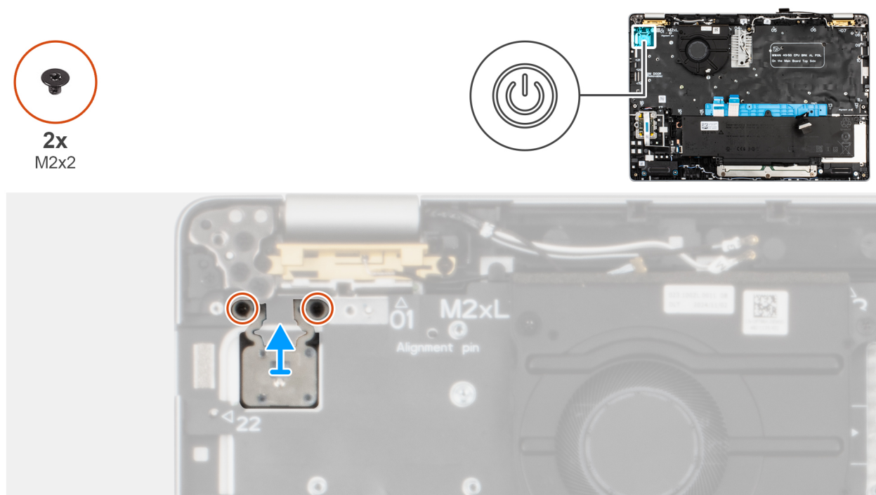
Figure 56. Installation du bouton d'alimentation avec lecteur d'empreintes digitales (en option)
