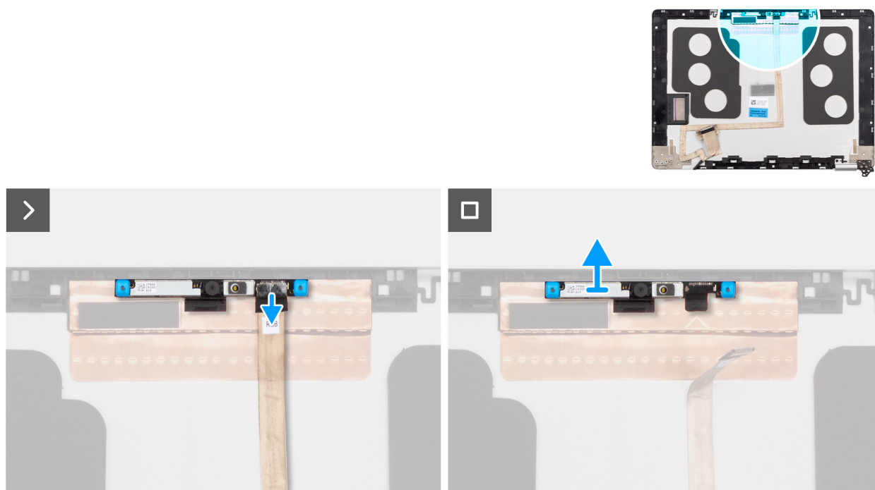
Figure 75. Retrait du module de caméra
