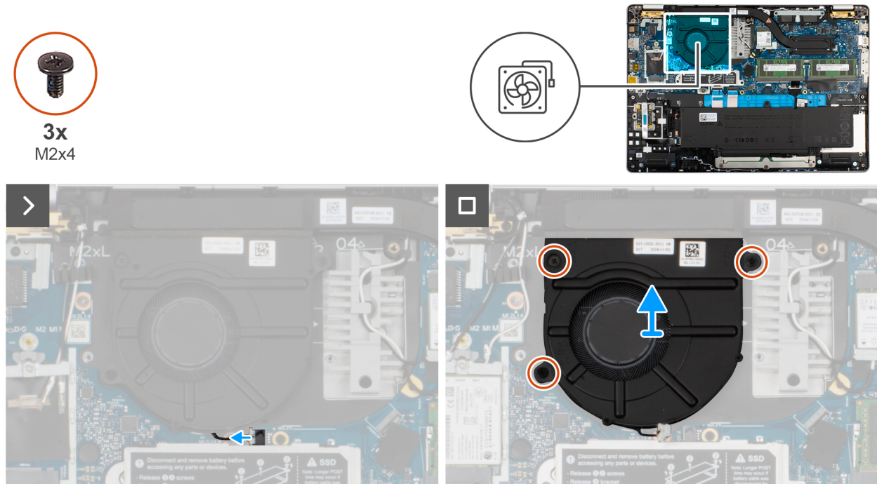
Figure 35. Retrait du ventilateur
