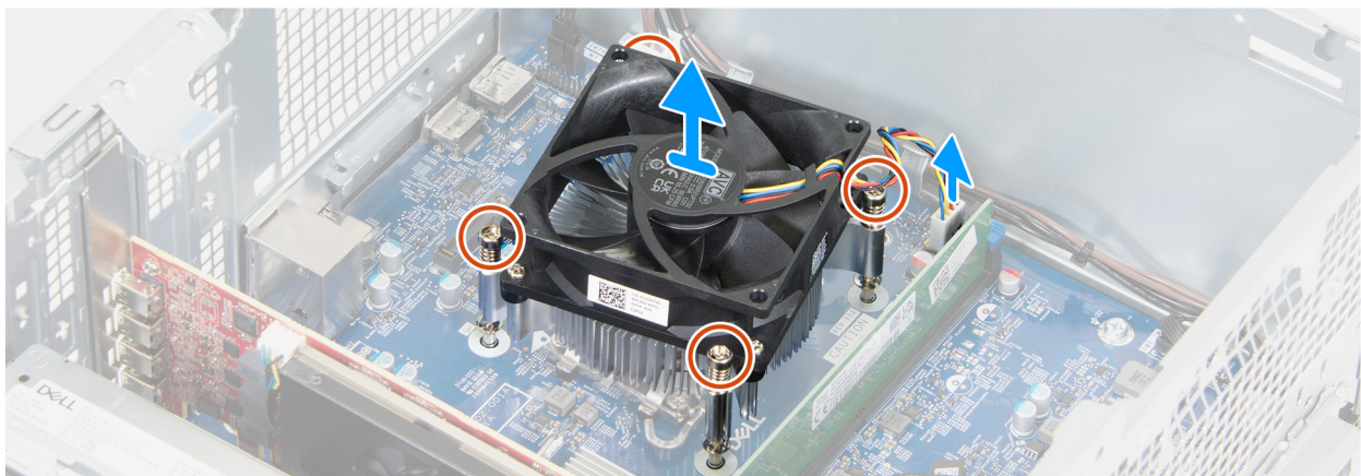
Abbildung 65. Entfernen des Prozessorlüfters und der Kühlkörperbaugruppe
