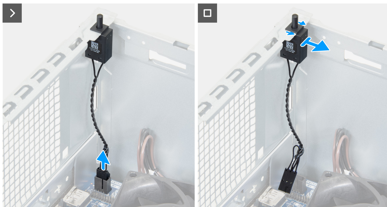
Abbildung 47. Entfernen des Eingriffsschalters
