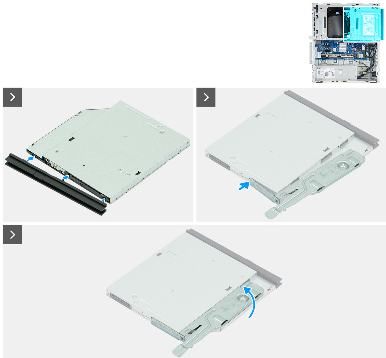
Abbildung 39. Installieren des optischen Laufwerks
