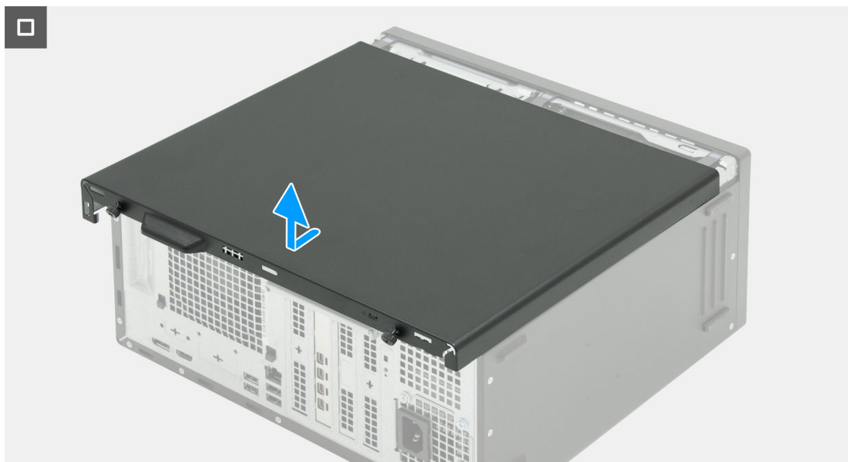
Abbildung 13. Entfernen der linken Abdeckung
