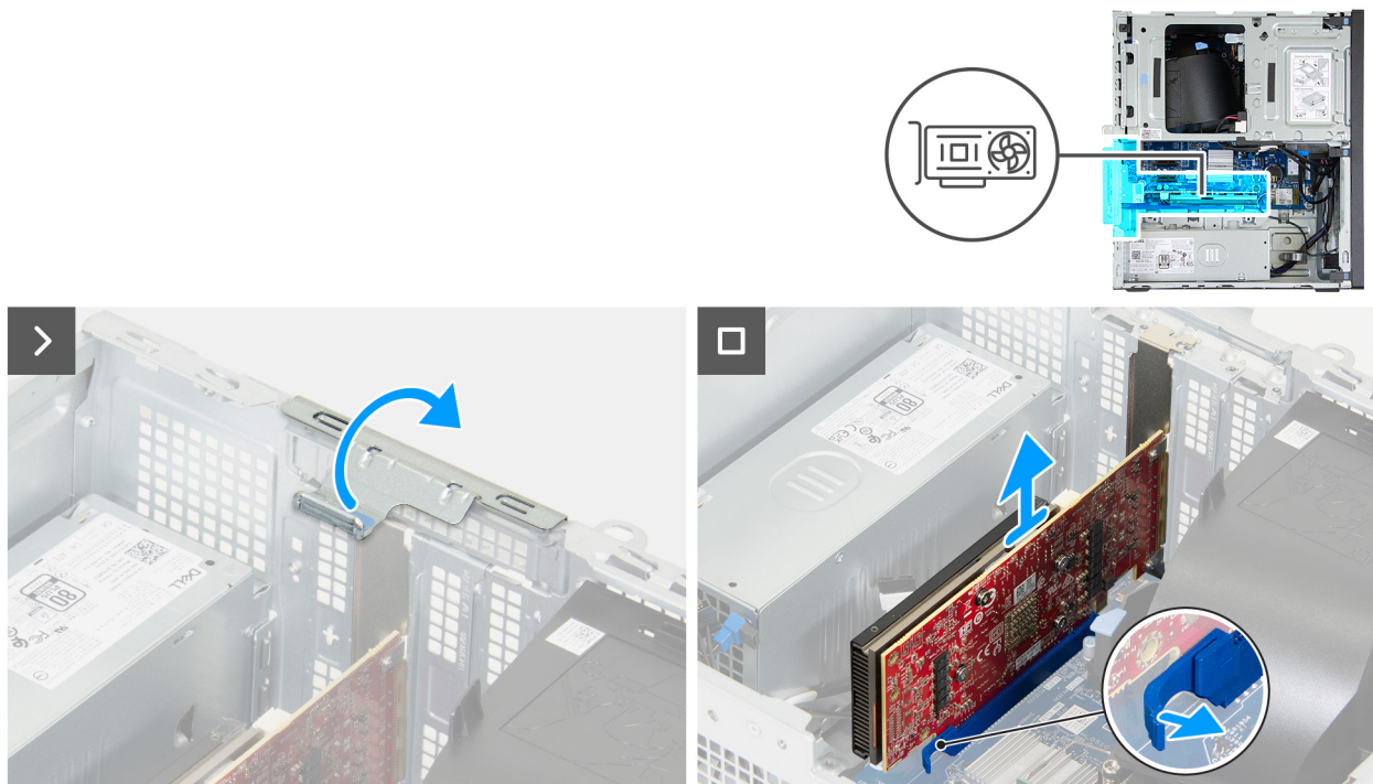
Abbildung 33. Entfernen der Grafikkarte
