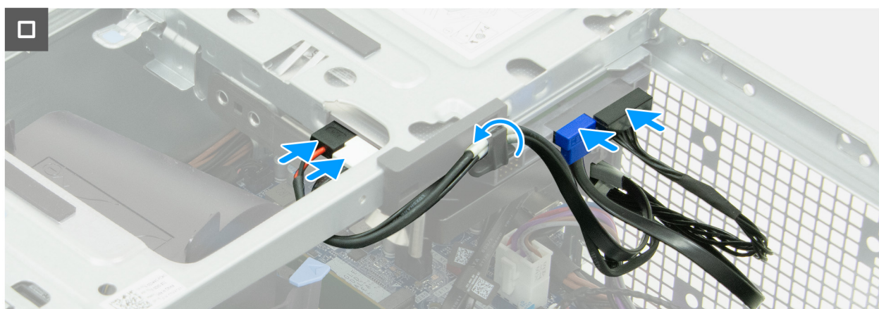
Abbildung 44. Installieren des Laufwerksschachts
