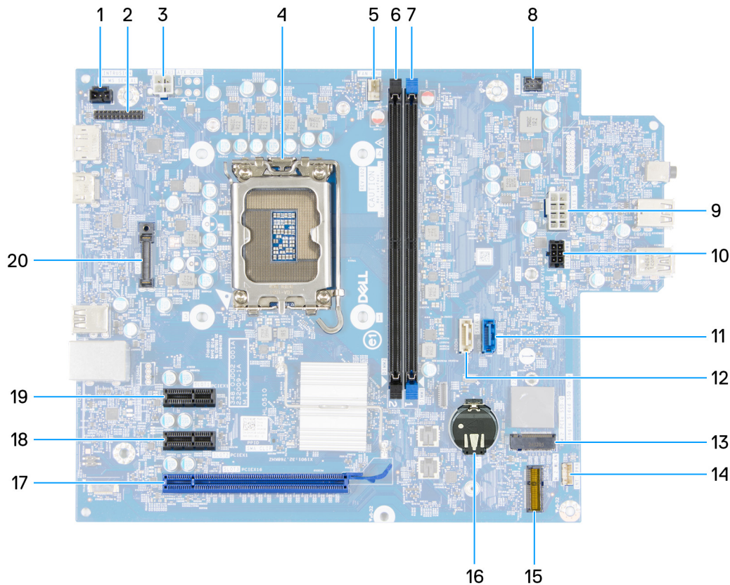
Abbildung 74. Systemplatinenbeschriftung
