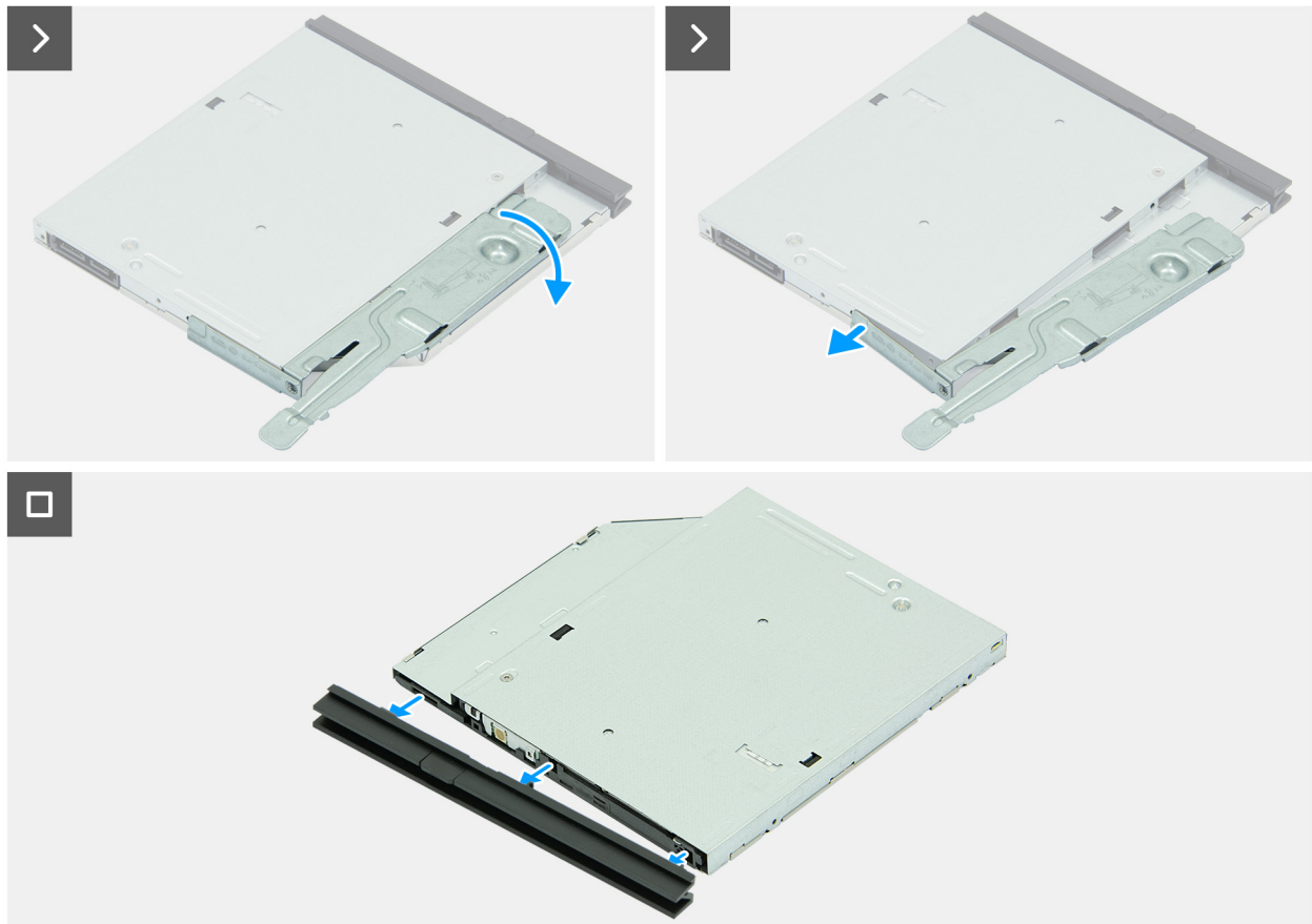
Abbildung 38. Entfernen des optischen Laufwerks
