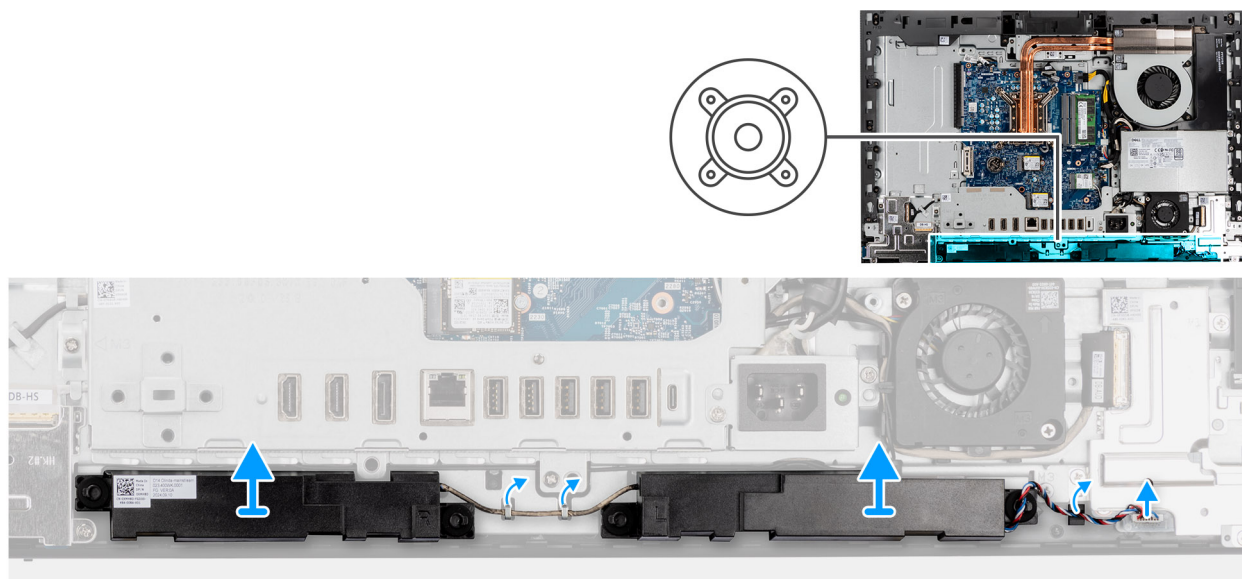
Figura 47. Rimozione degli altoparlanti
