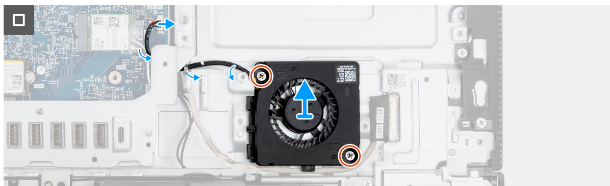
Figura 43. Rimozione della ventola di alimentazione
