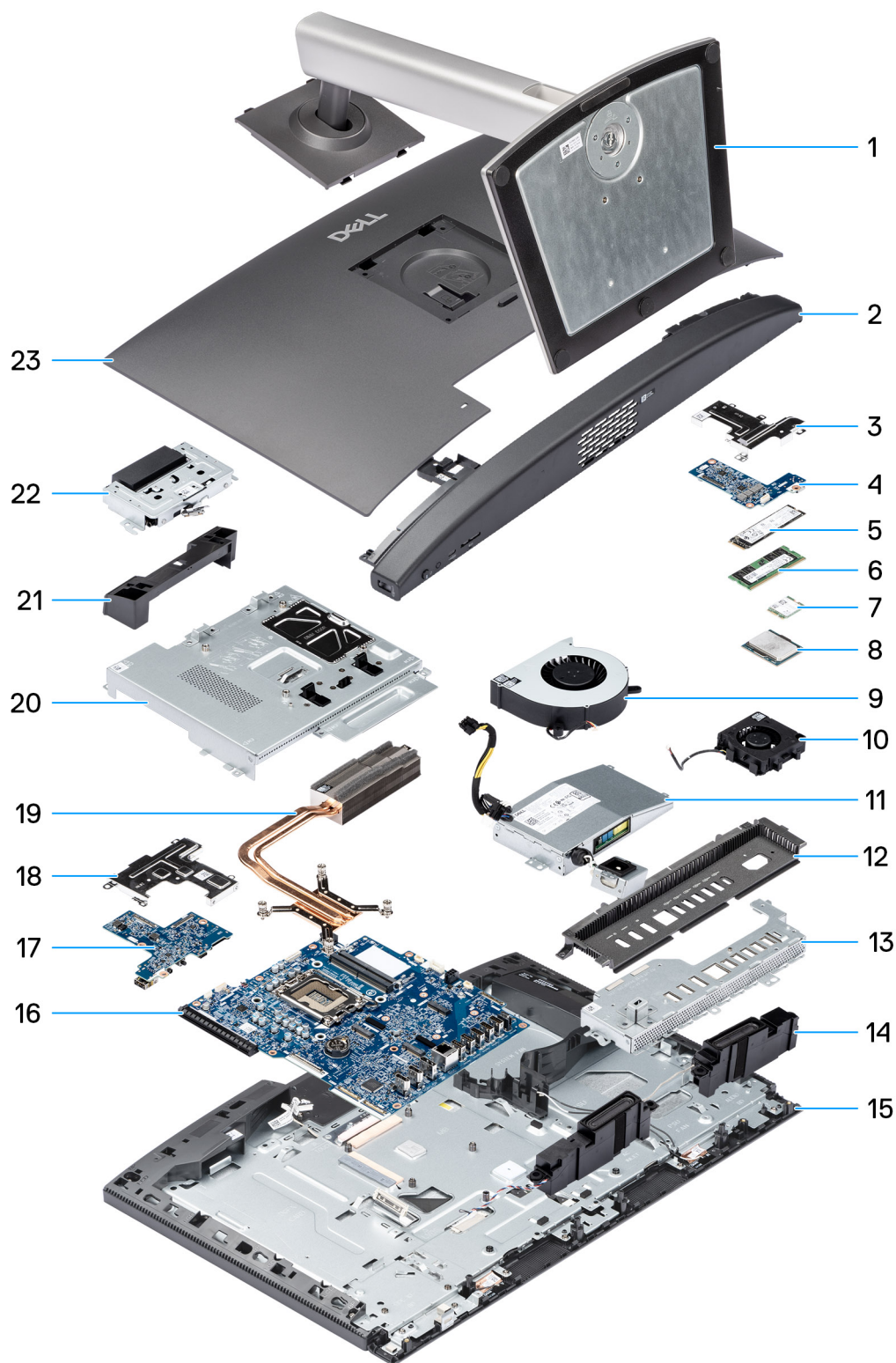
Figura 12. Componenti principali di Dell Pro 24 All-in-One QC24250
