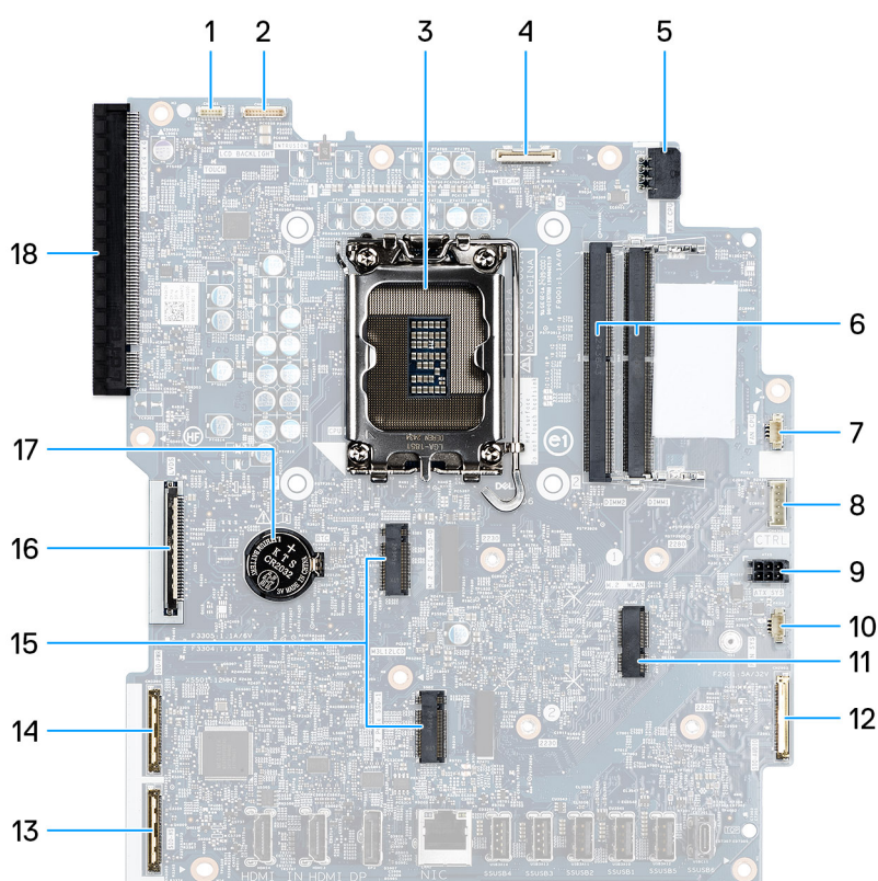
Figura 53. Callout della scheda di sistema
