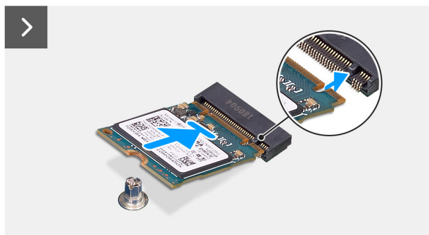
Figura 29. Installazione dell'unità SSD M.2 2230 nello slot M.2 1
