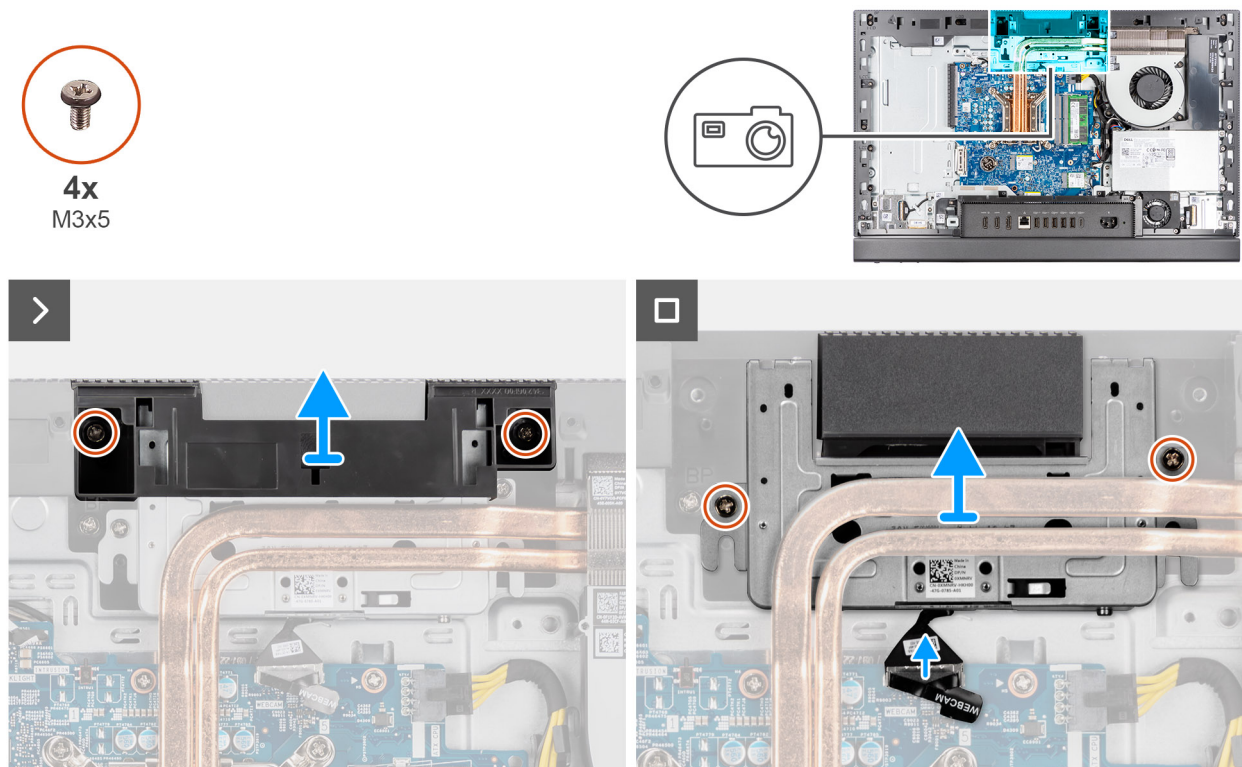
Figura 37. Rimozione del gruppo della fotocamera retraibile
