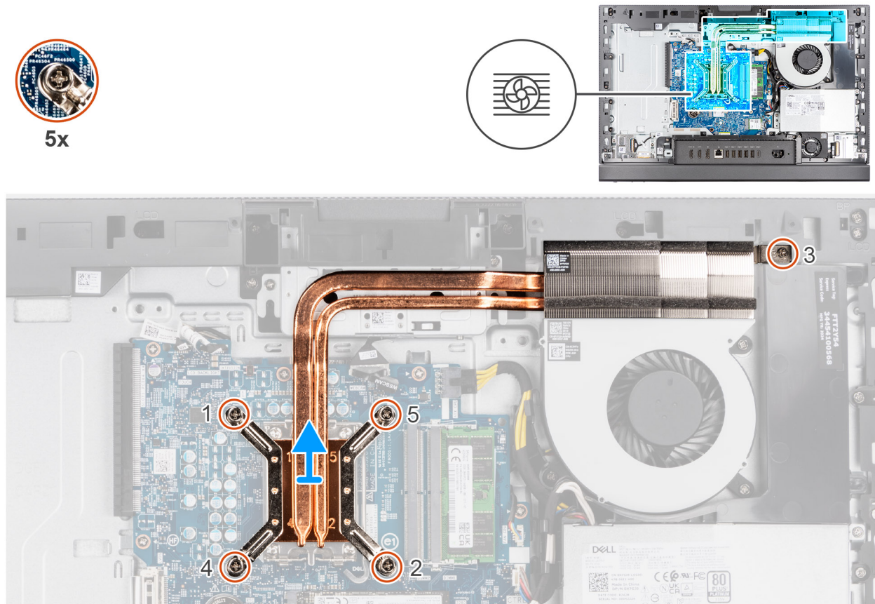
Figura 49. Rimozione del dissipatore di calore
