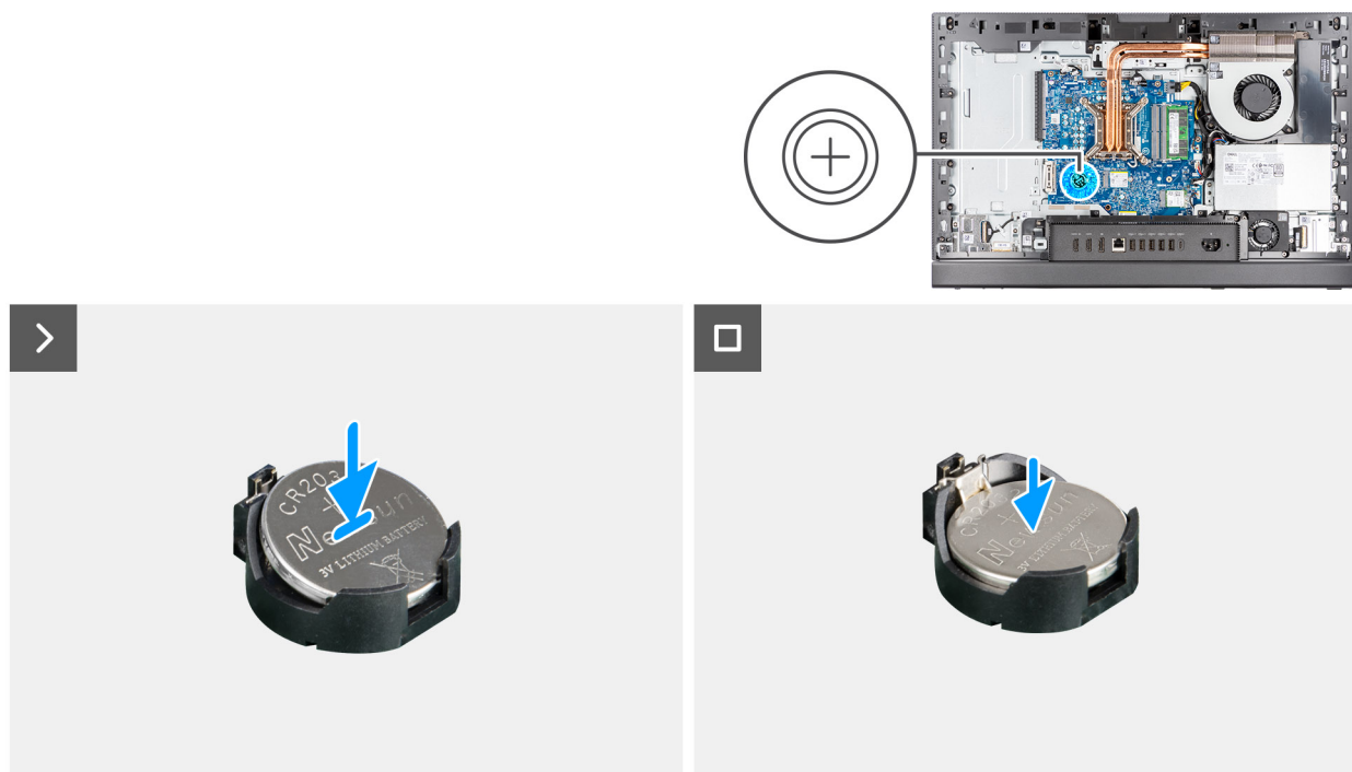
Figura 32. Installazione della batteria a bottone
