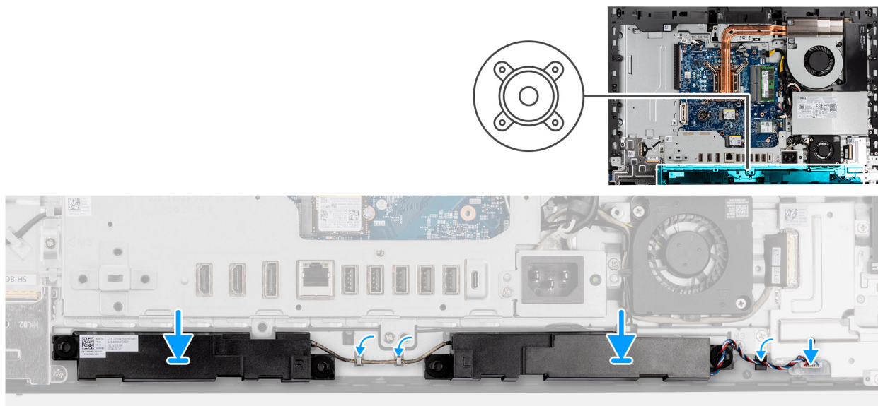
Figura 48. Installazione degli altoparlanti
