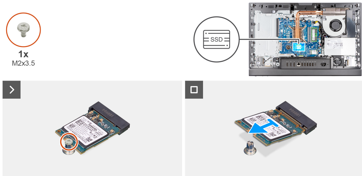
Figura 25. Rimozione dell'unità SSD M.2 2230 dallo slot M.2 0
