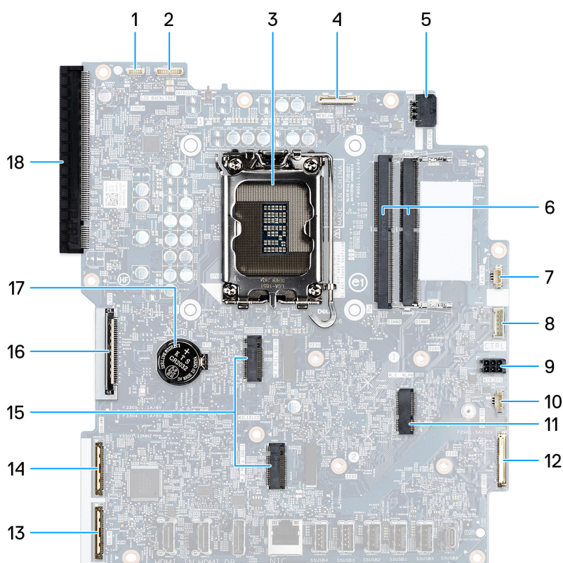
Figura 56. Callout della scheda di sistema
