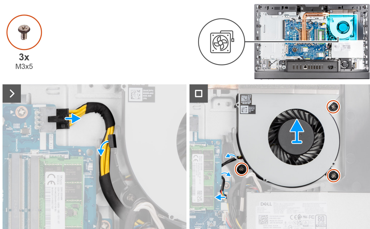
Figura 39. Rimozione della ventola
