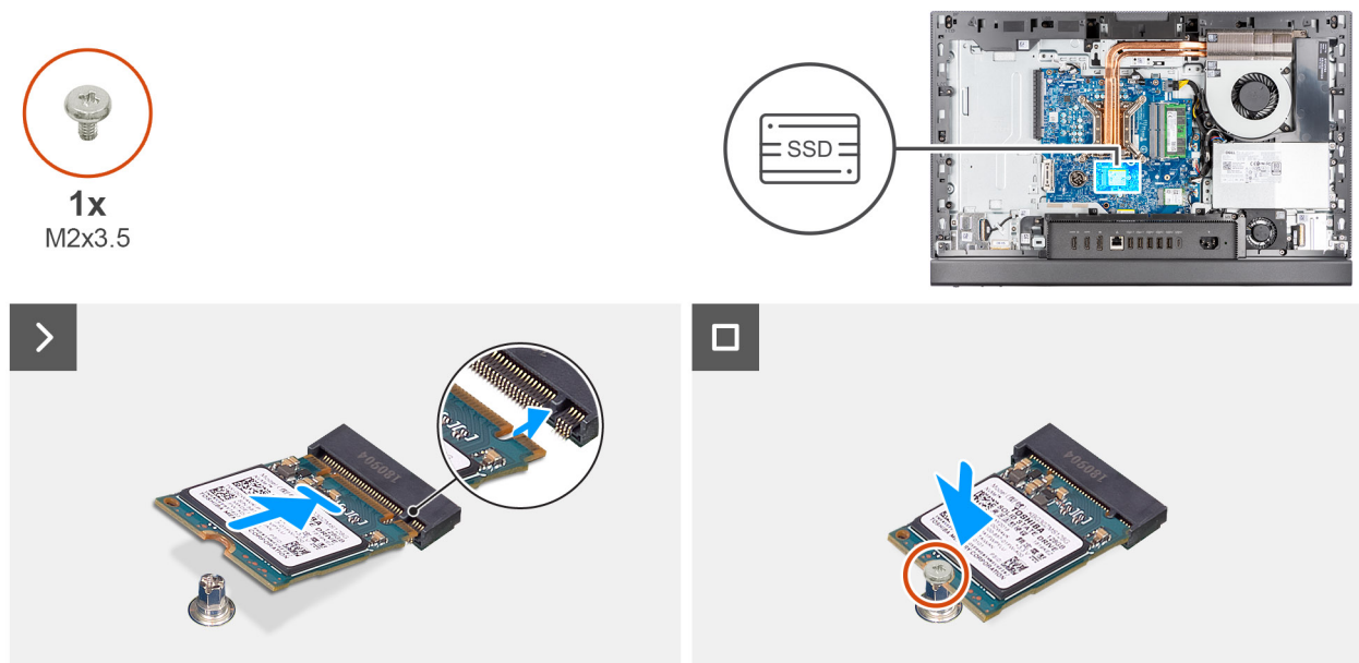
Figura 26. Installazione dell'unità SSD M.2 2230 nello slot M.2 0
