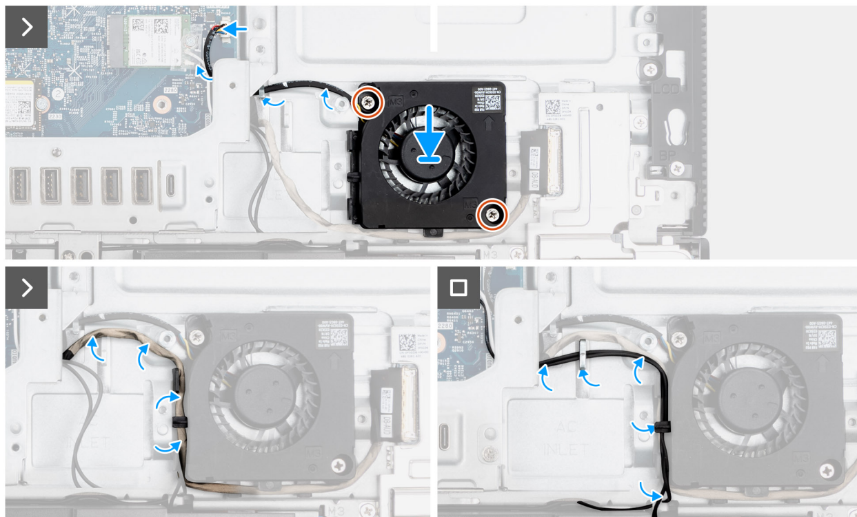
Figura 44. Installazione della ventola dell'alimentatore
