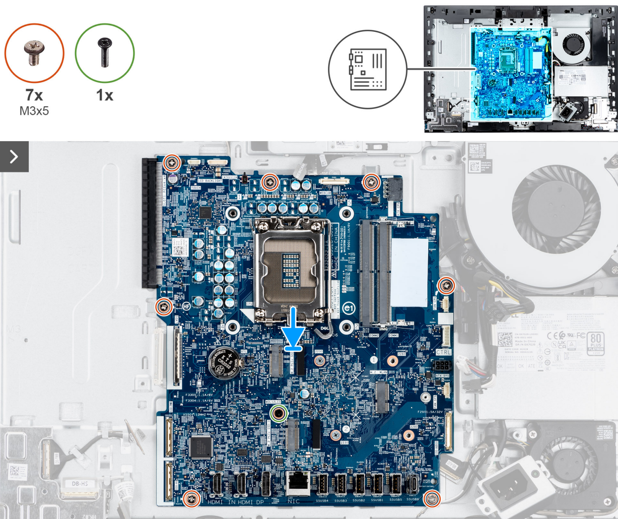
Figura 57. Installazione della scheda di sistema
