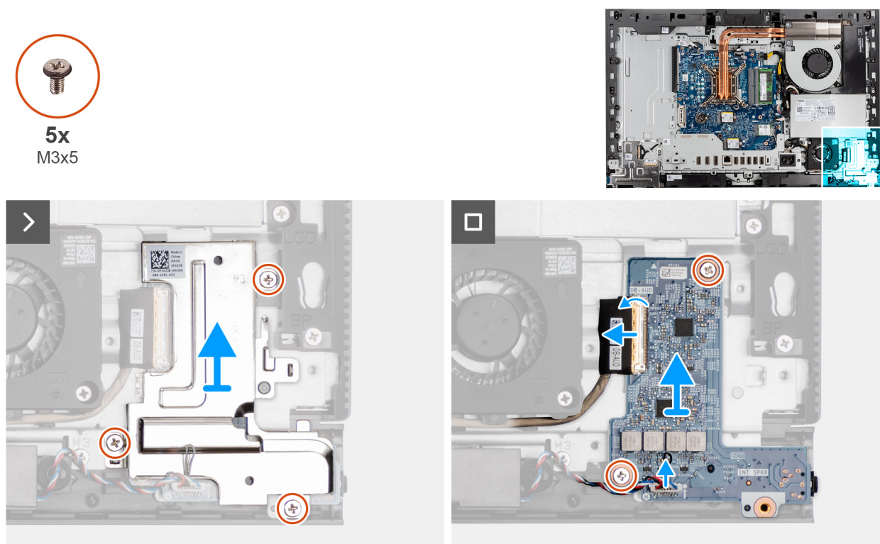
Figura 61. Rimozione della scheda audio
