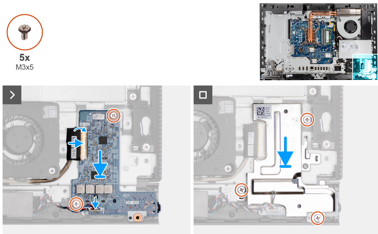
Figura 62. Installazione della scheda audio
