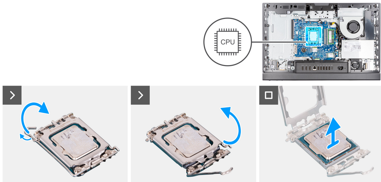
Figura 51. Rimozione del processore
