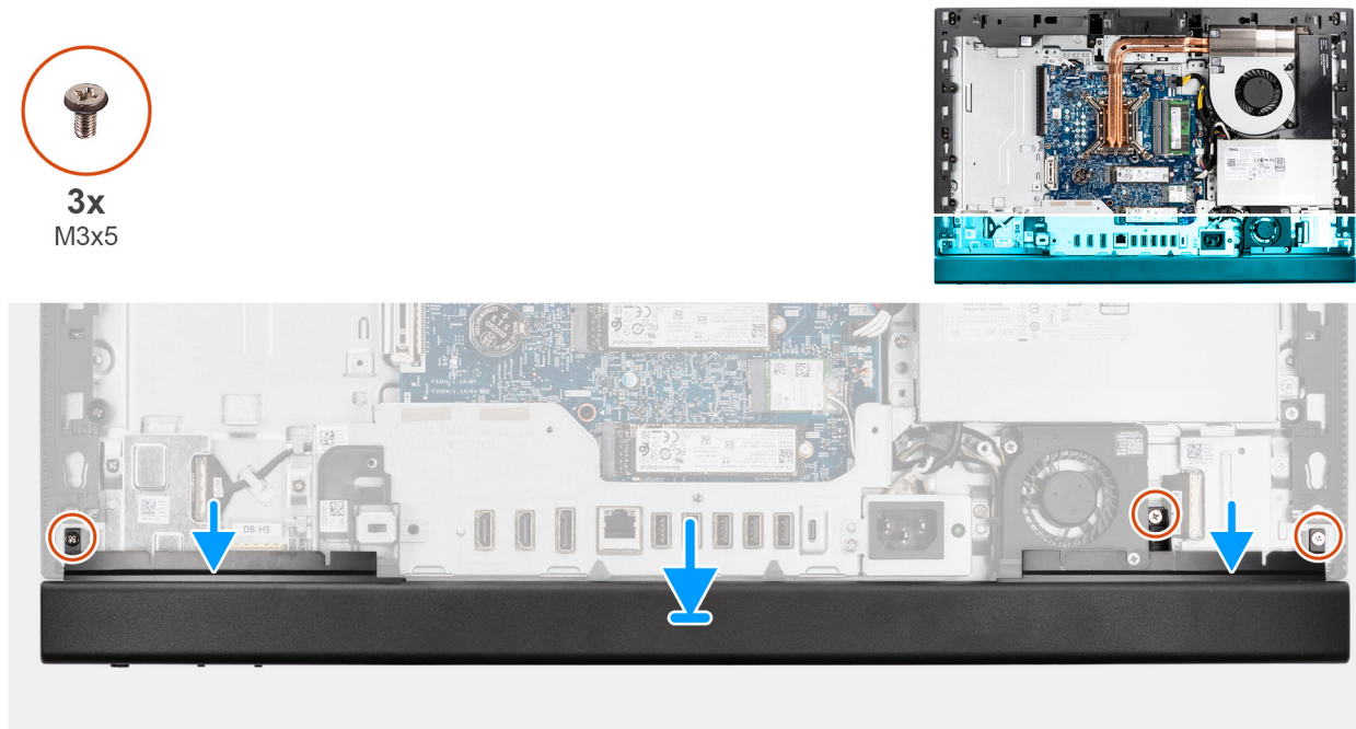
Figura 36. Installazione del coperchio inferiore
