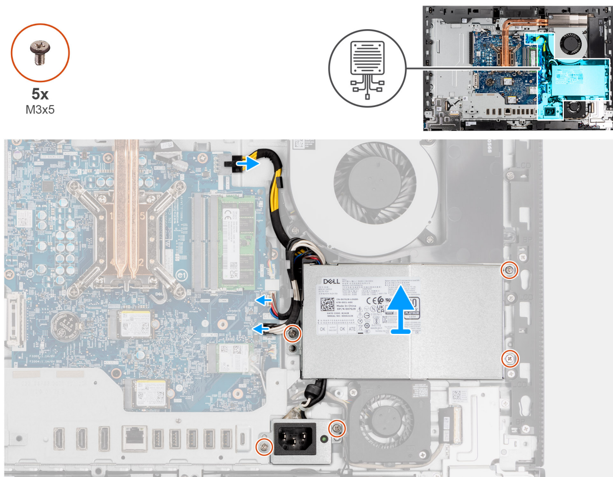
Figura 41. Rimozione dell'unità di alimentazione
