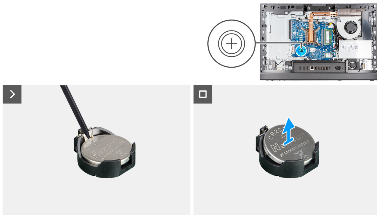
Figura 31. Rimozione della batteria a bottone
