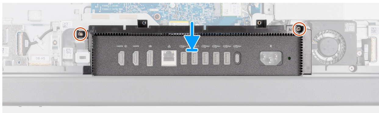
Figura 34. Installazione del coperchio di I/O
