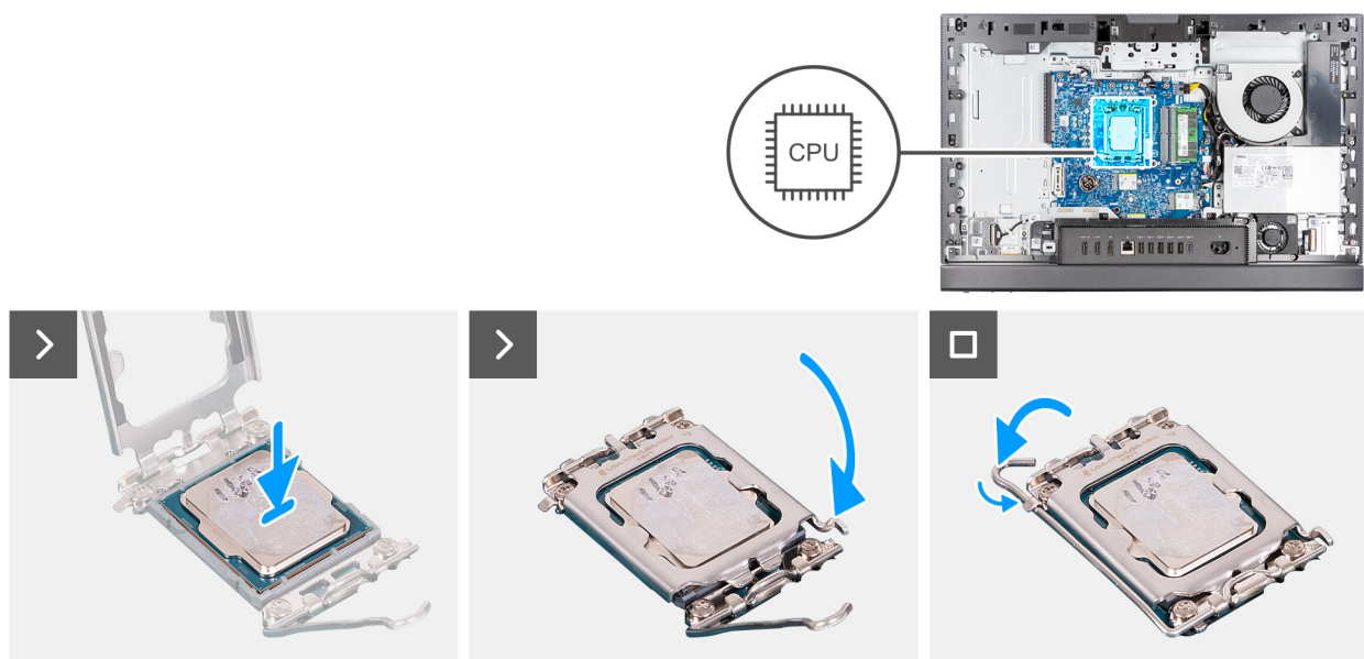
Figura 52. Installazione del processore
