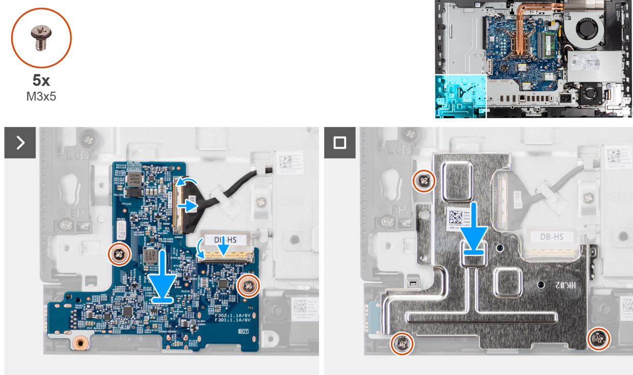
Figura 60. Installazione della scheda del pulsante di accensione e di I/O
