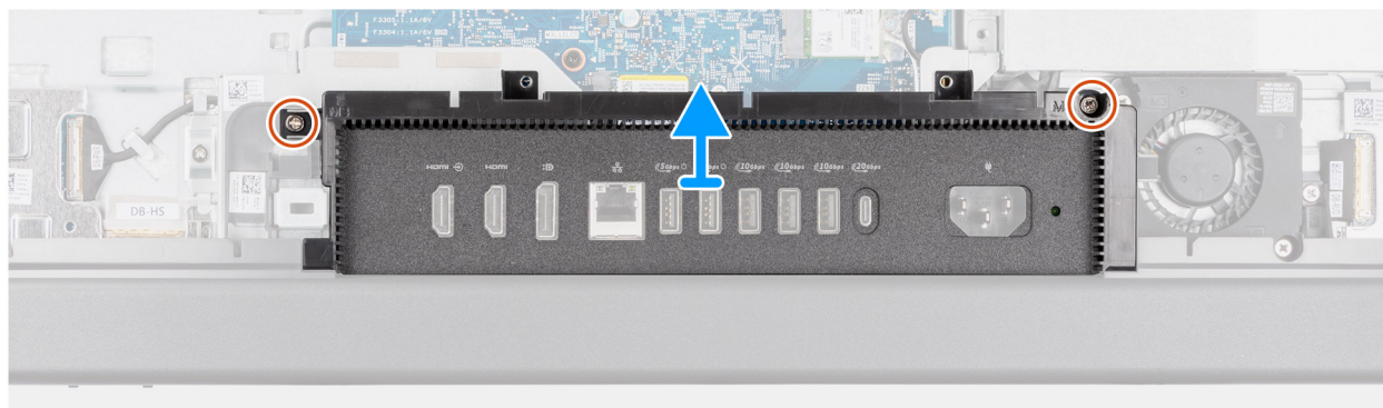
Figura 33. Rimozione del coperchio di I/O
