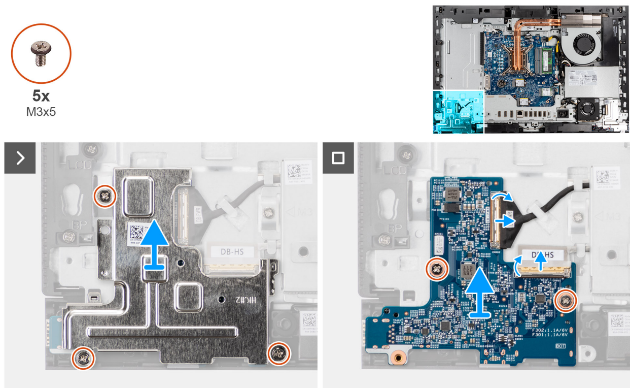
Figura 59. Rimozione della scheda del pulsante di accensione e di I/O
