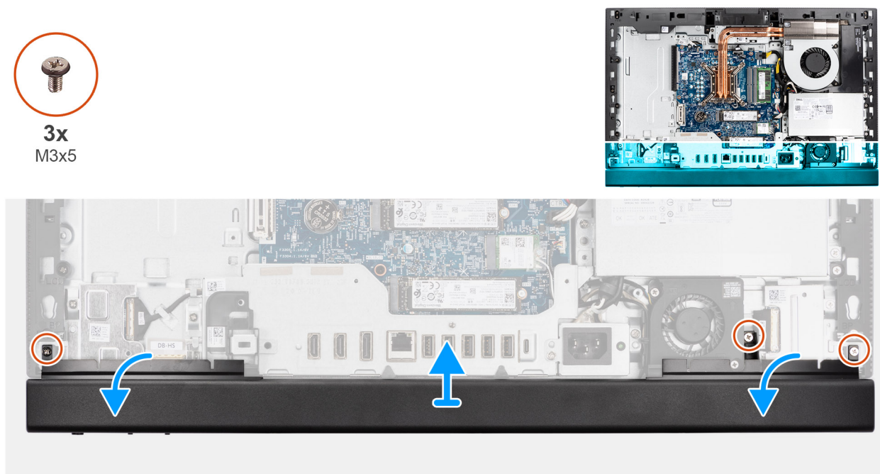
Figura 35. Rimozione del coperchio inferiore
