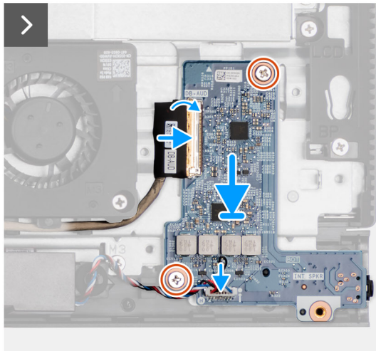
Abbildung 62. Einbauen der Audioplatine
