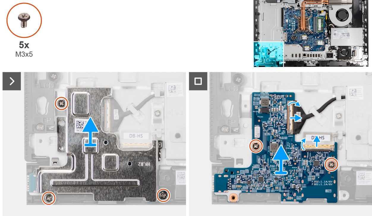
Abbildung 59. Entfernen des Netzschalters und der E/A-Platine
