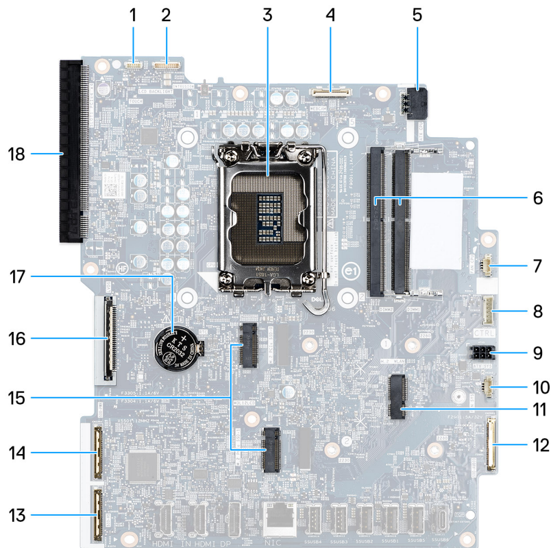
Abbildung 56. Systemplatinenbeschriftung
