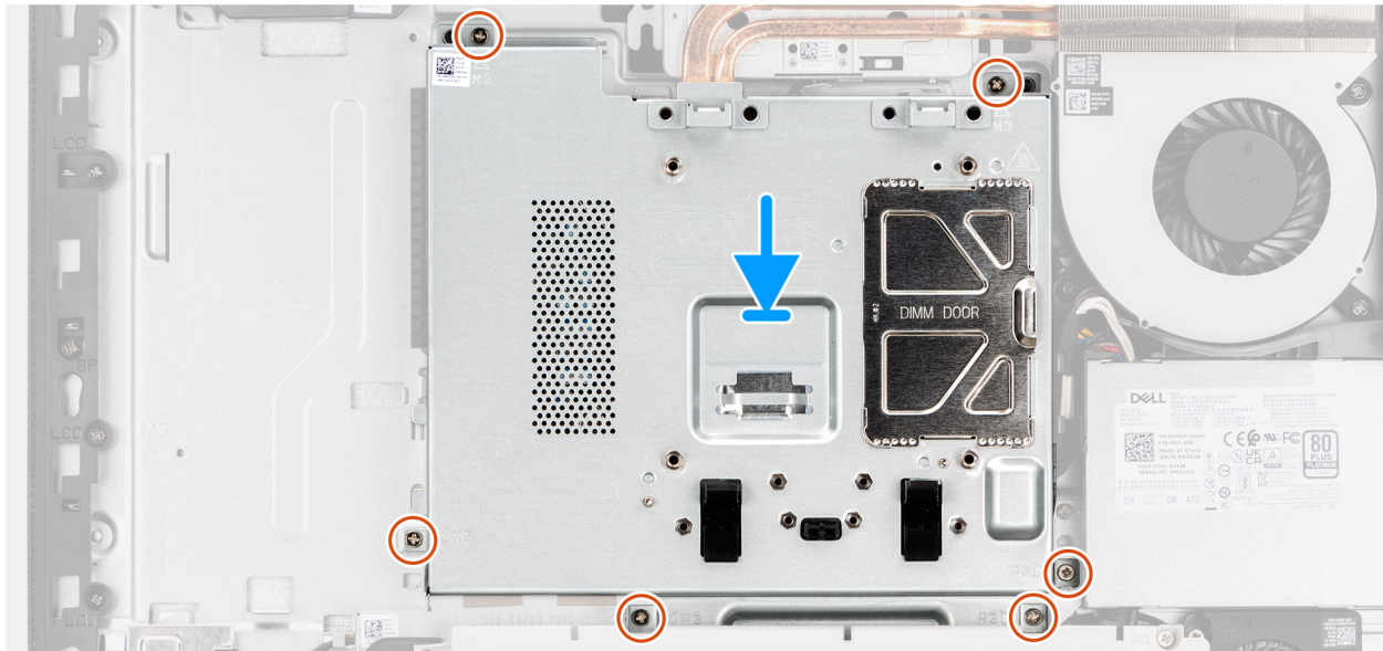
Abbildung 22. Einbauen der Abdeckung der Systemplatine
