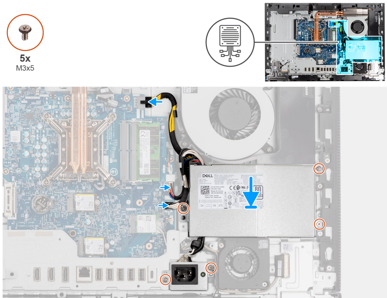
Abbildung 42. Installieren der Stromversorgungseinheit
