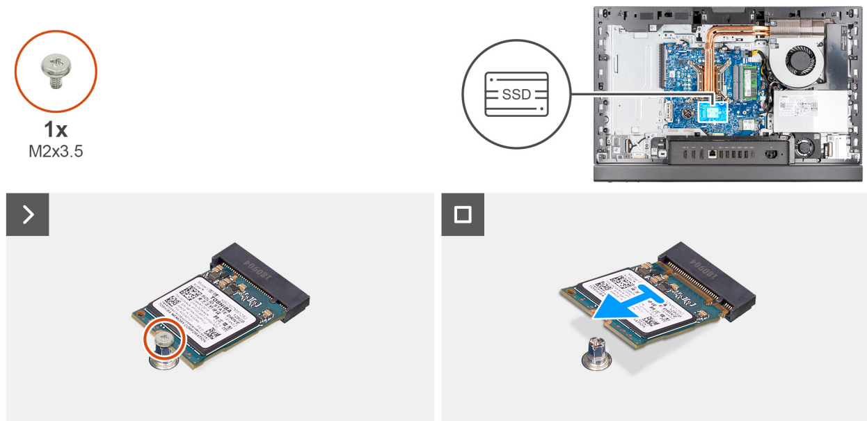
Abbildung 25. Entfernen des M.2 2230-SSD-Laufwerks aus M.2-Steckplatz 0
