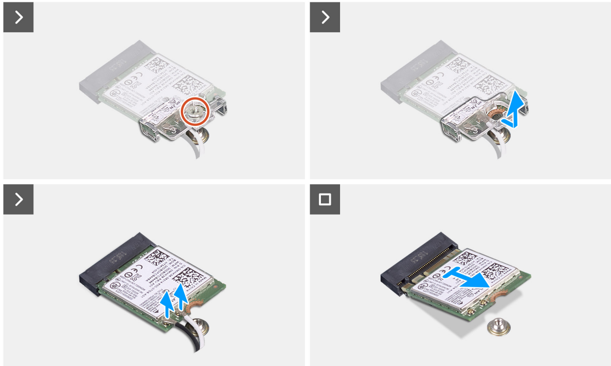
Abbildung 23. Entfernen der Wireless-Karte
