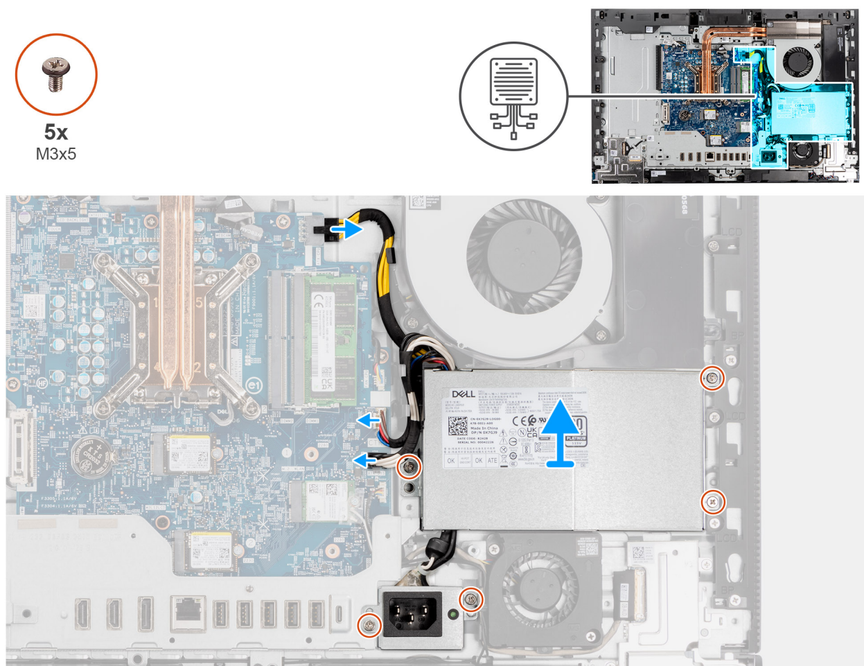
Abbildung 41. Entfernen der Stromversorgungseinheit
