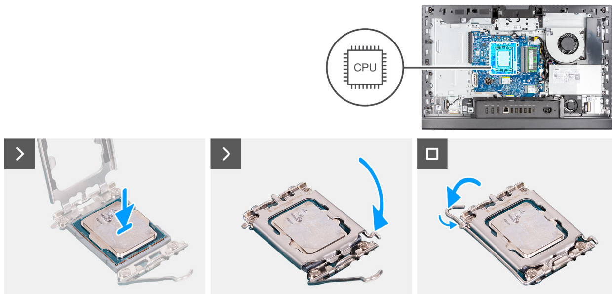
Abbildung 52. Einbauen des Prozessors
