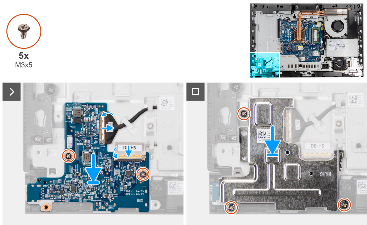
Abbildung 60. Einbauen der Netzschalter- und E/A-Platine
