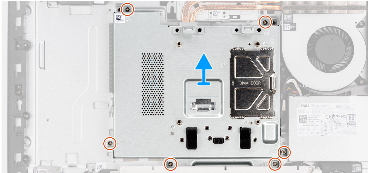
Abbildung 21. Entfernen der Abdeckung der Systemplatine
