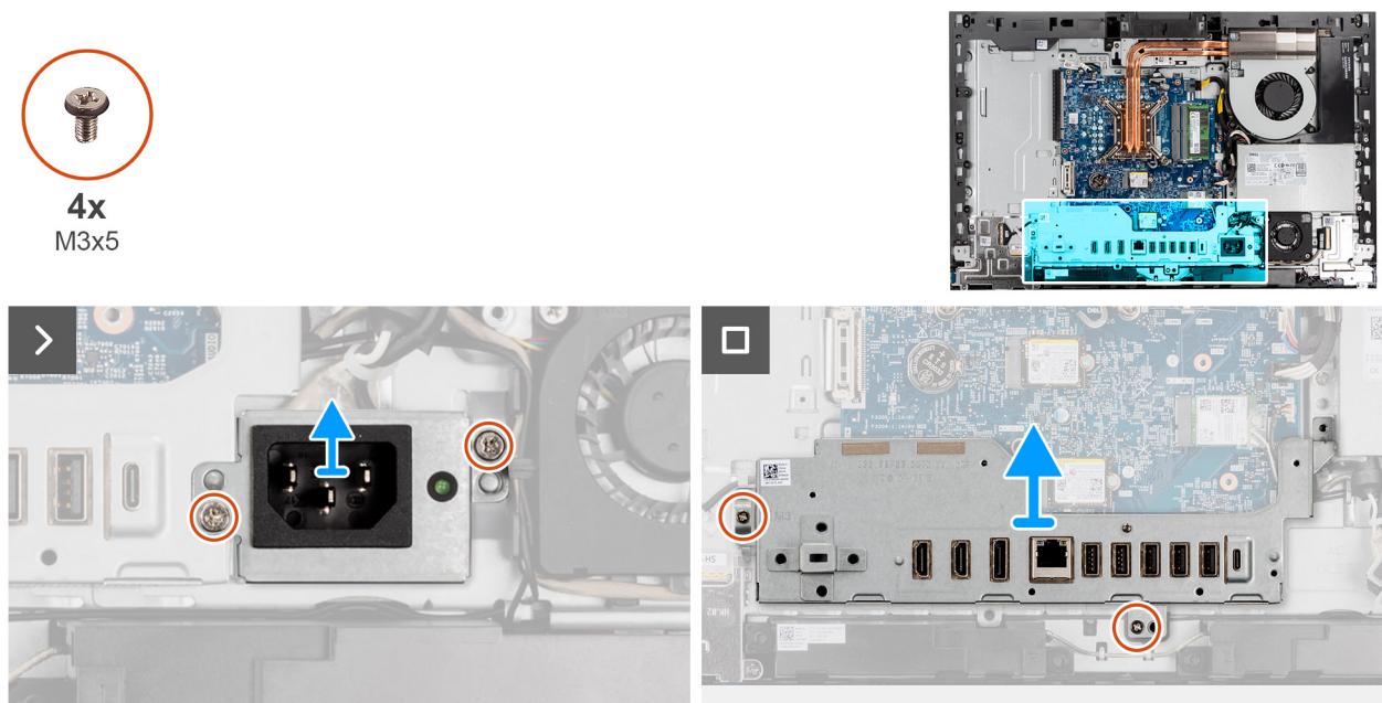
Abbildung 45. Entfernen der E/A-Halterung
