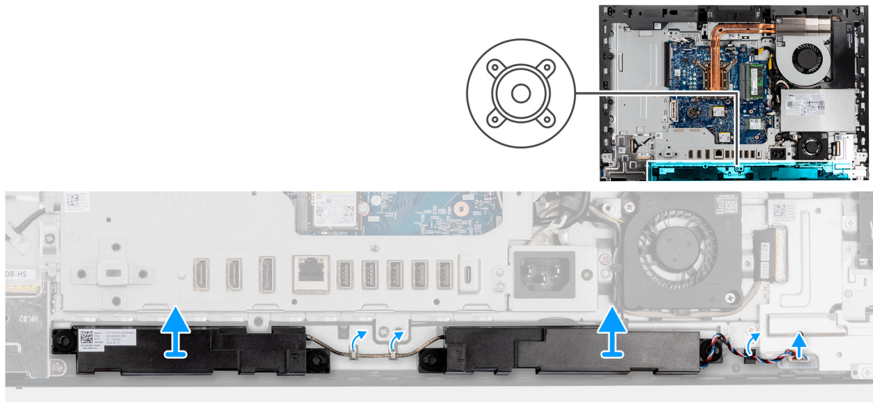
Abbildung 47. Entfernen der Lautsprecher
