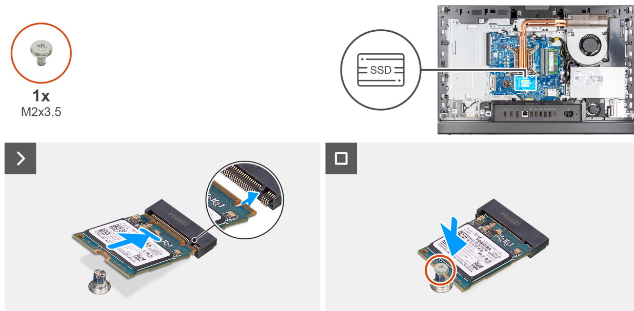
Abbildung 26. Installieren des M.2-2230-SSD-Laufwerks in M.2-Steckplatz 0
