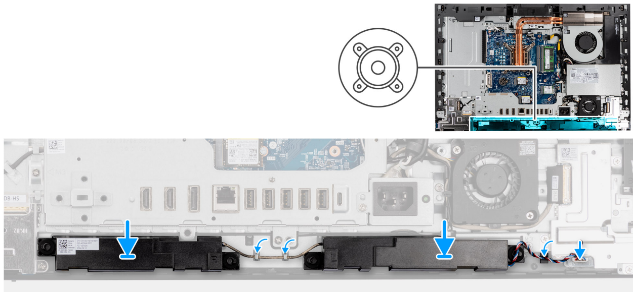
Abbildung 48. Installieren der Lautsprecher
