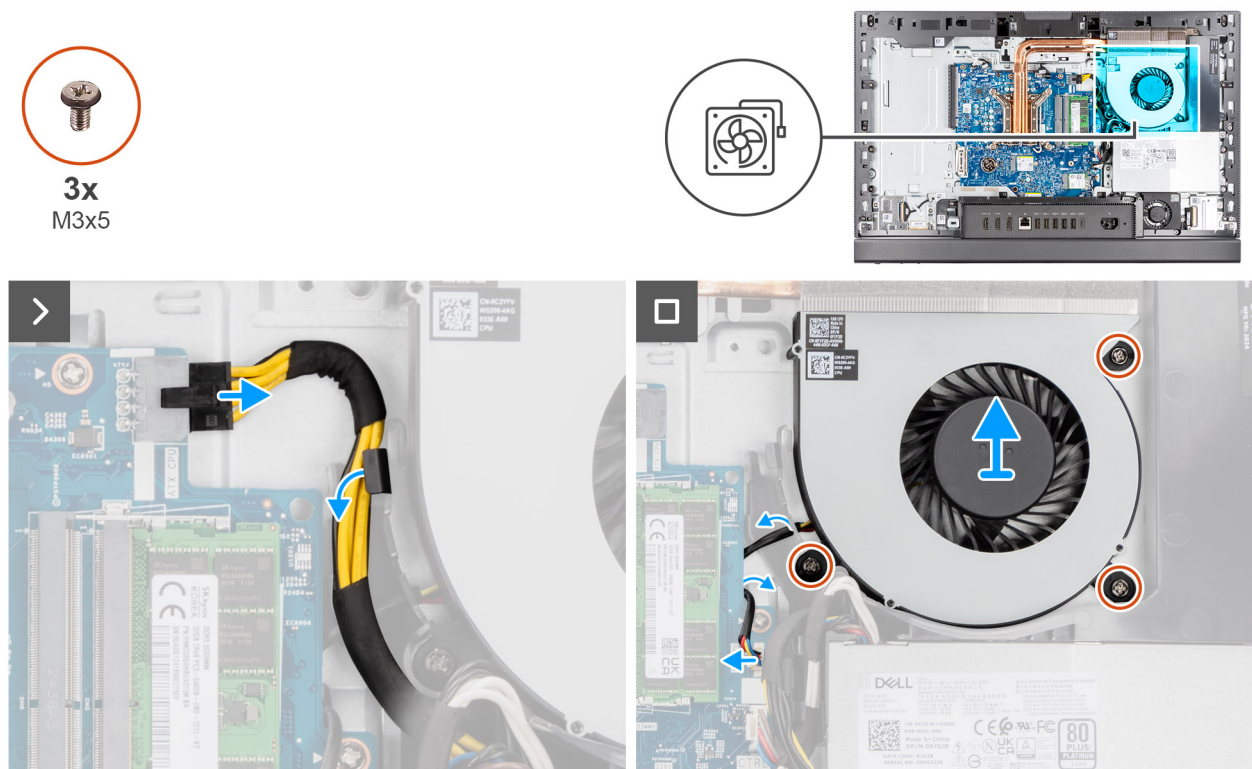
Abbildung 39. Entfernen des Lüfters
