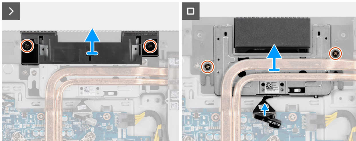
Abbildung 37. Entfernen der einziehbaren Kamerabaugruppe
