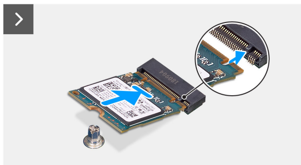
Abbildung 29. Installieren des M.2-2230-SSD-Laufwerks in M.2-Steckplatz 1
