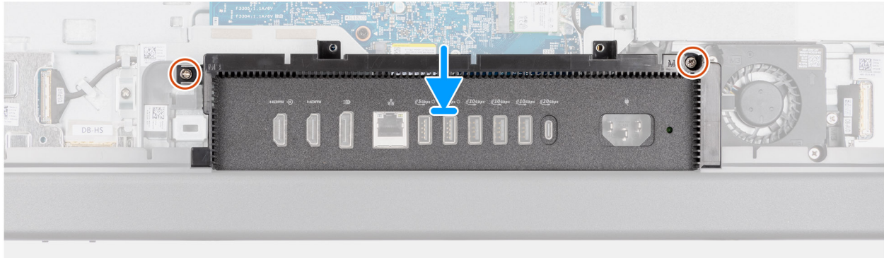
Abbildung 34. Einbauen der E/A-Abdeckung
