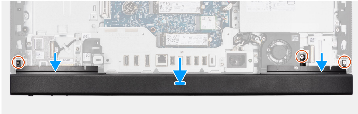
Abbildung 36. Anbringen der unteren Abdeckung
