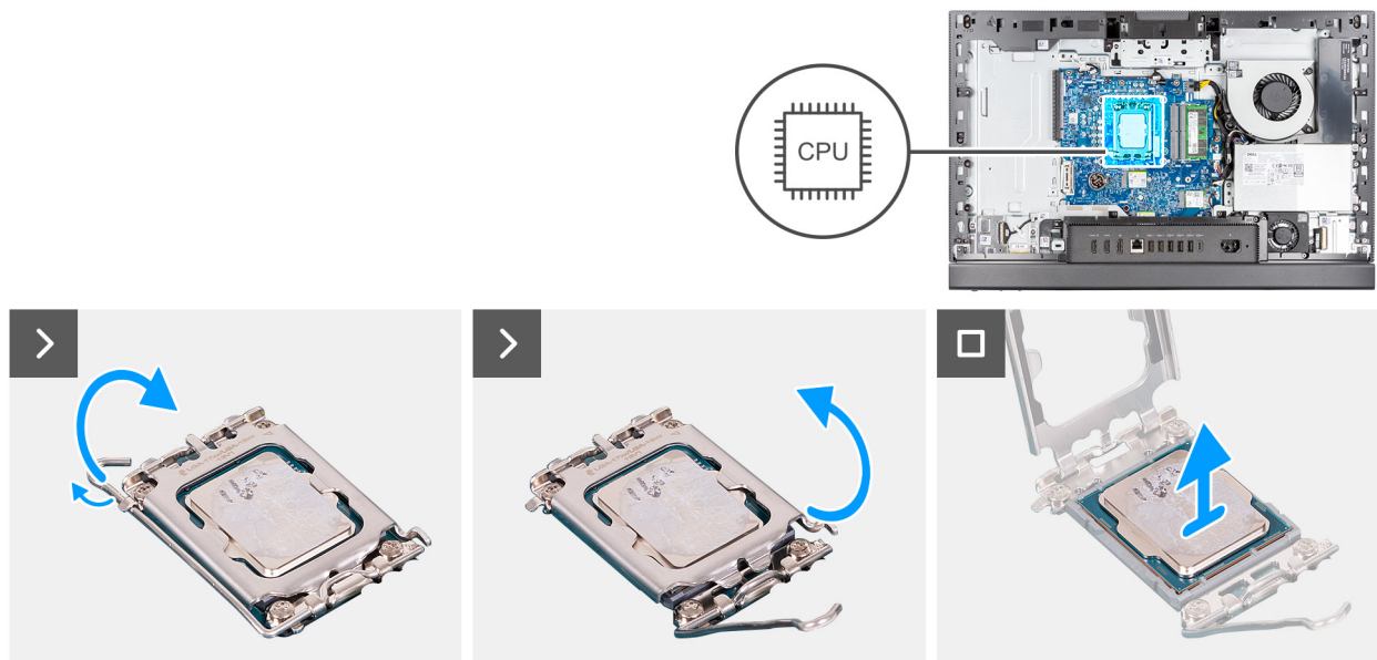
Abbildung 51. Entfernen des Prozessors
