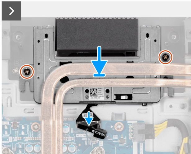
Abbildung 38. Installieren der einziehbaren Kamerabaugruppe
