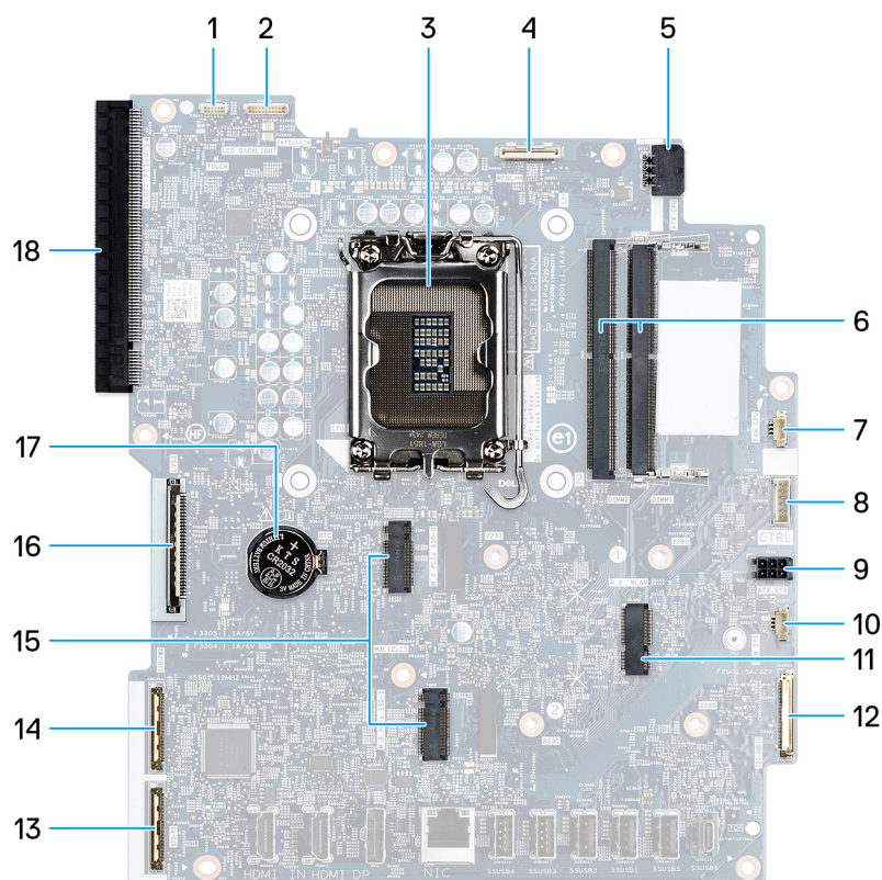
Abbildung 53. Systemplatinenbeschriftung
