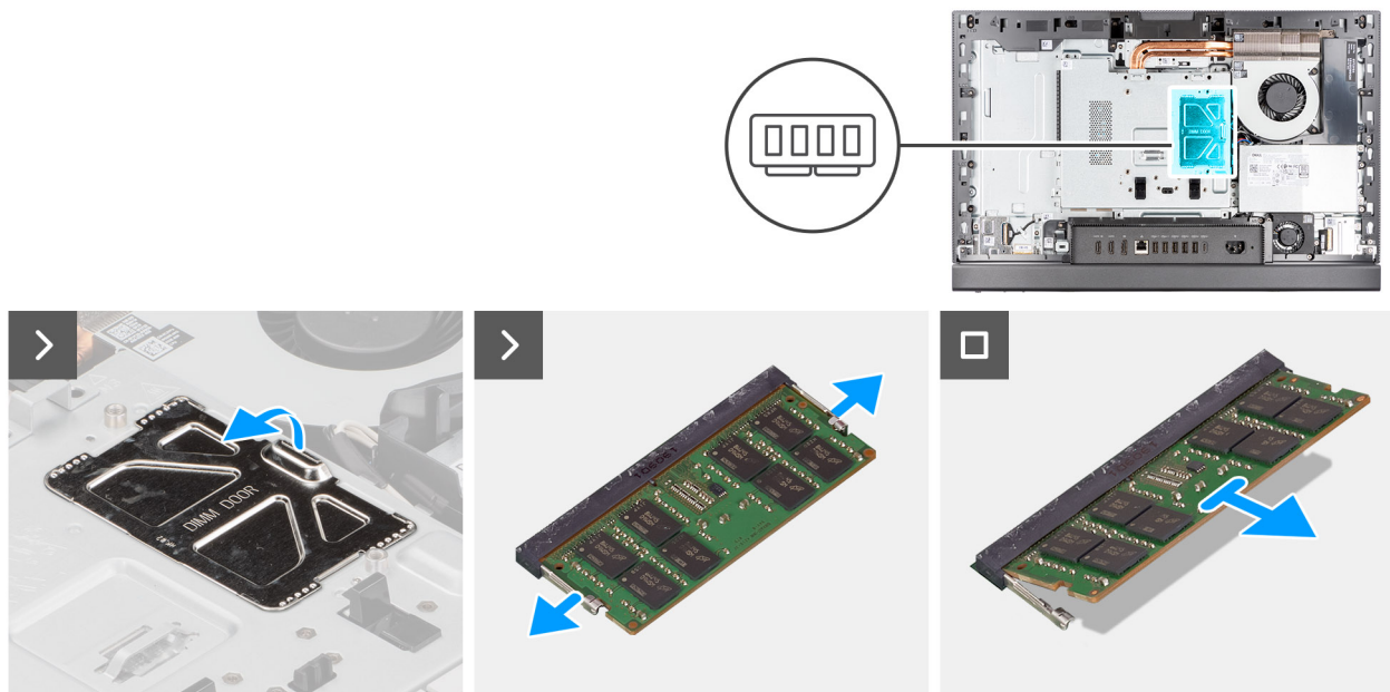
Abbildung 19. Entfernen des Speichers
