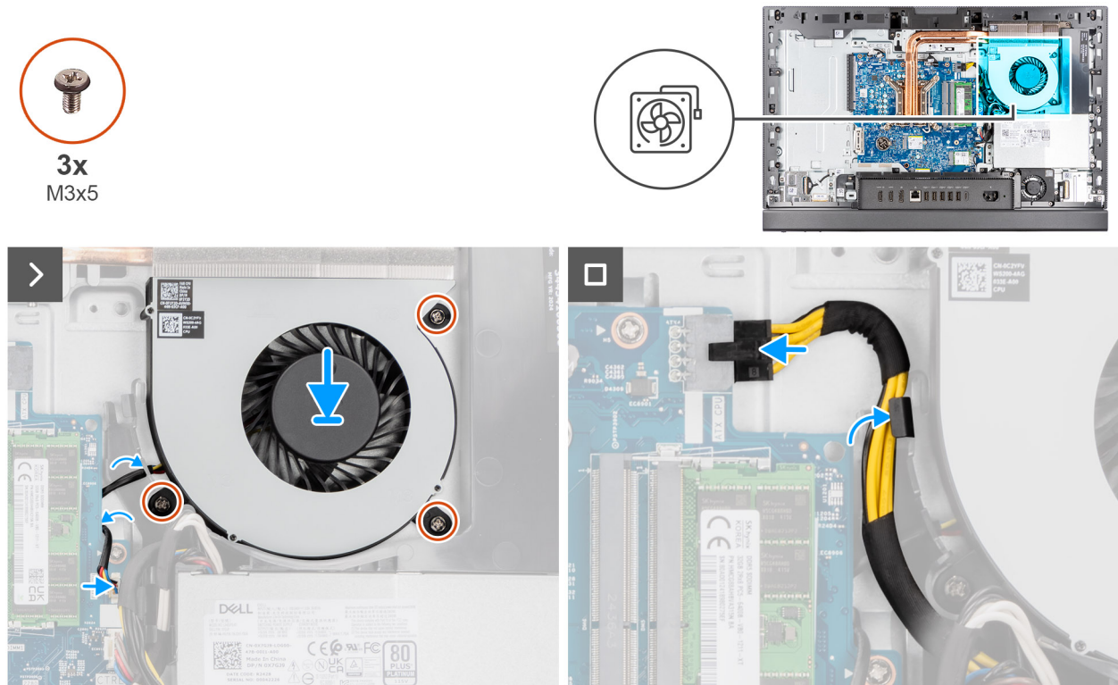
Abbildung 40. Einbauen des Lüfters
