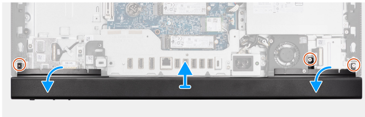
Abbildung 35. Entfernen der unteren Abdeckung
