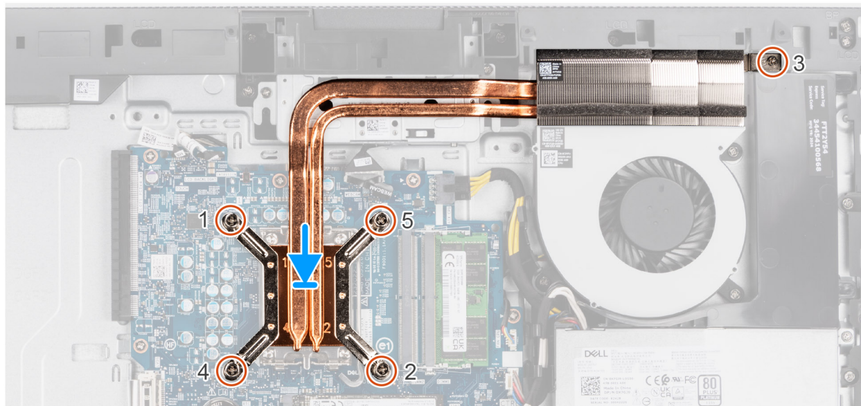
Abbildung 50. Einsetzen des Kühlkörpers
