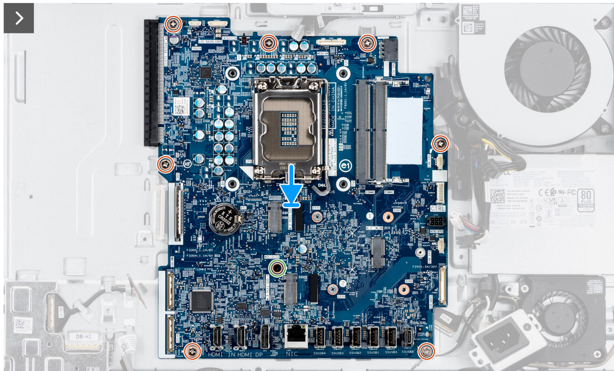
Abbildung 57. Einbauen der Systemplatine
