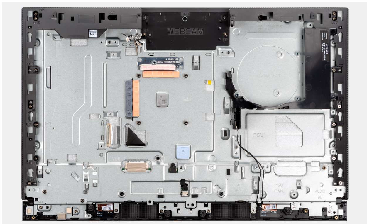
Abbildung 63. Entfernen der Grundplatte der Bildschirmbaugruppe
