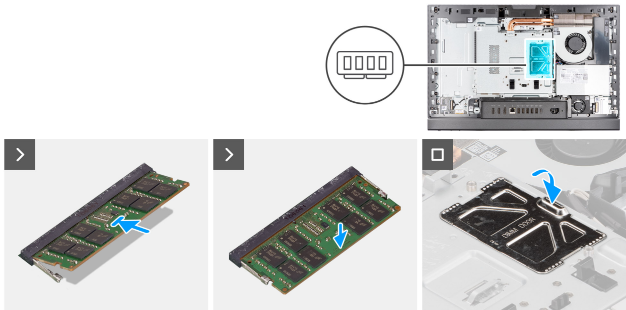
Abbildung 20. Einbauen des Speichers
