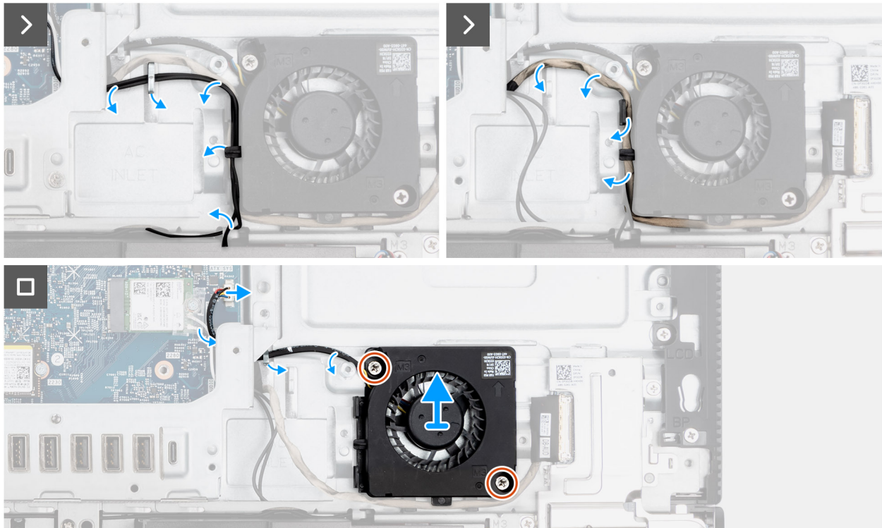
Abbildung 43. Entfernen des Netzteil­lüfters
