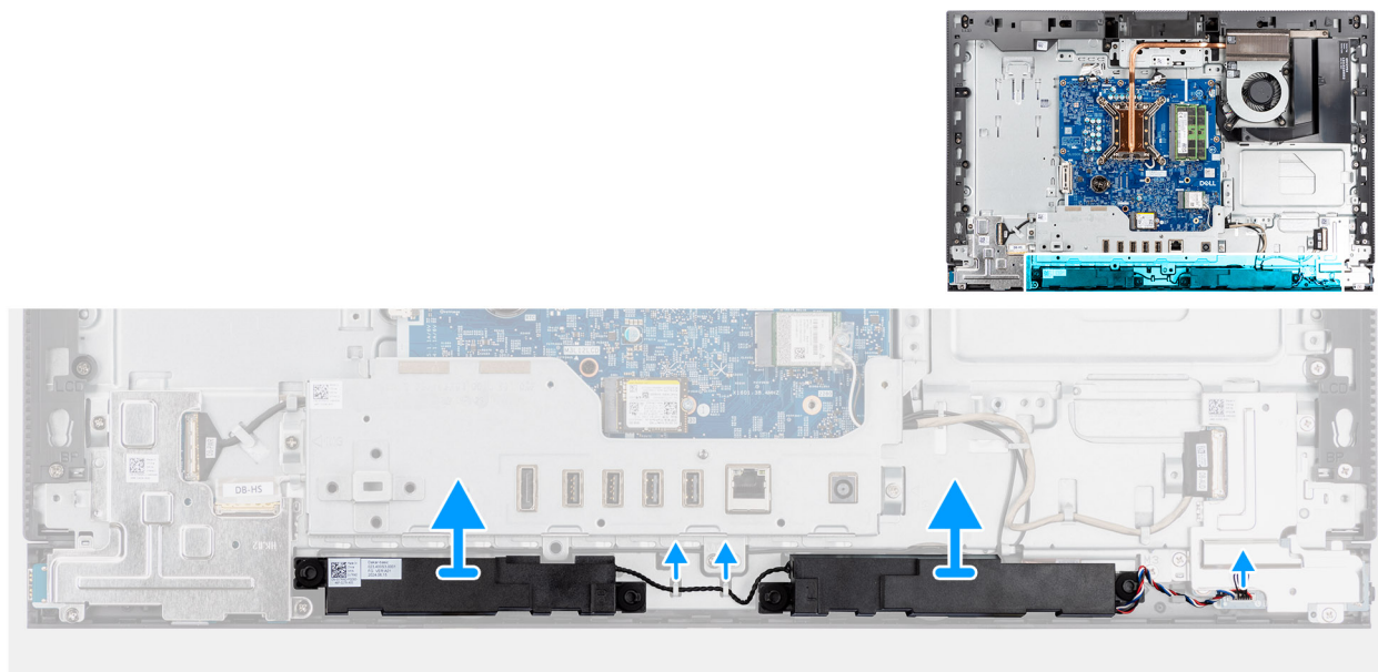
Figura 40. Rimozione degli altoparlanti
