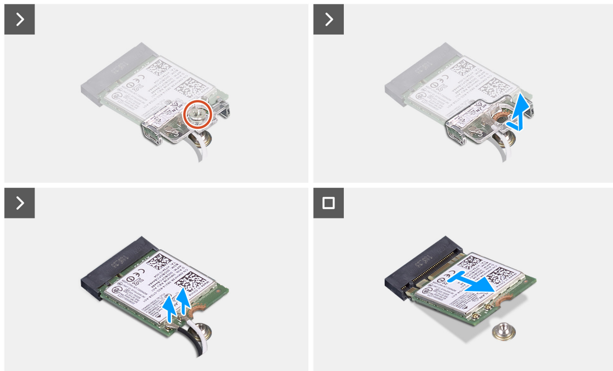
Figura 23. Rimozione della scheda wireless
