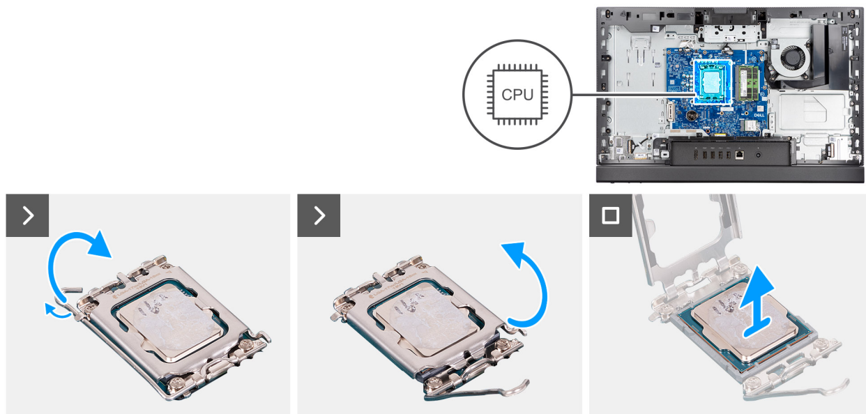
Figura 44. Rimozione del processore
