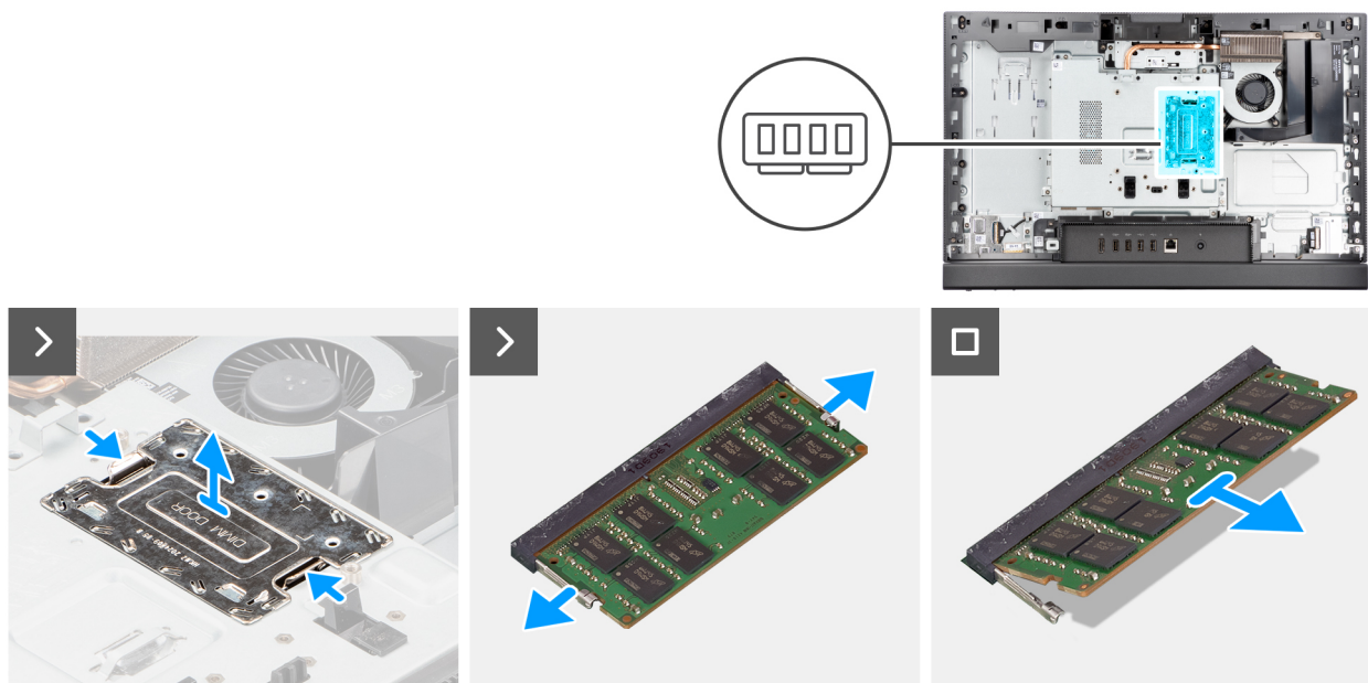
Figura 19. Rimozione della memoria
