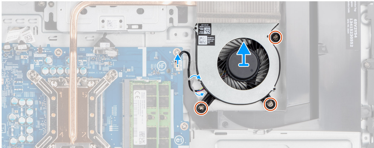
Figura 36. Rimozione della ventola
