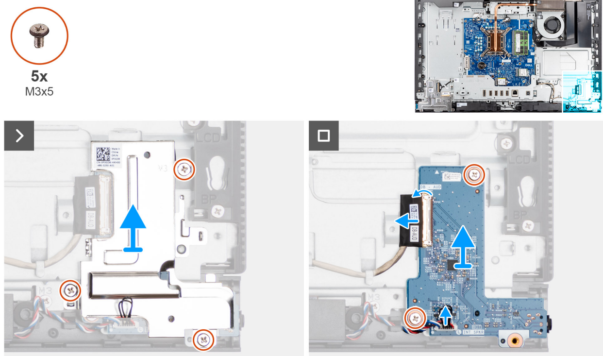
Figura 54. Rimozione della scheda audio
