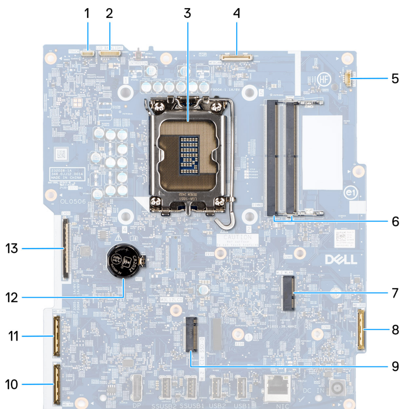
Figura 49. Callout della scheda di sistema
