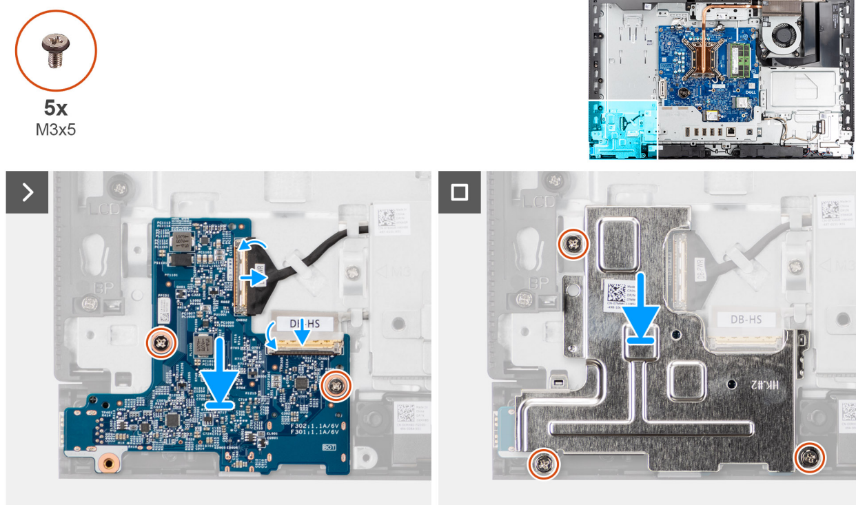
Figura 53. Installazione della scheda del pulsante di accensione e di I/O
