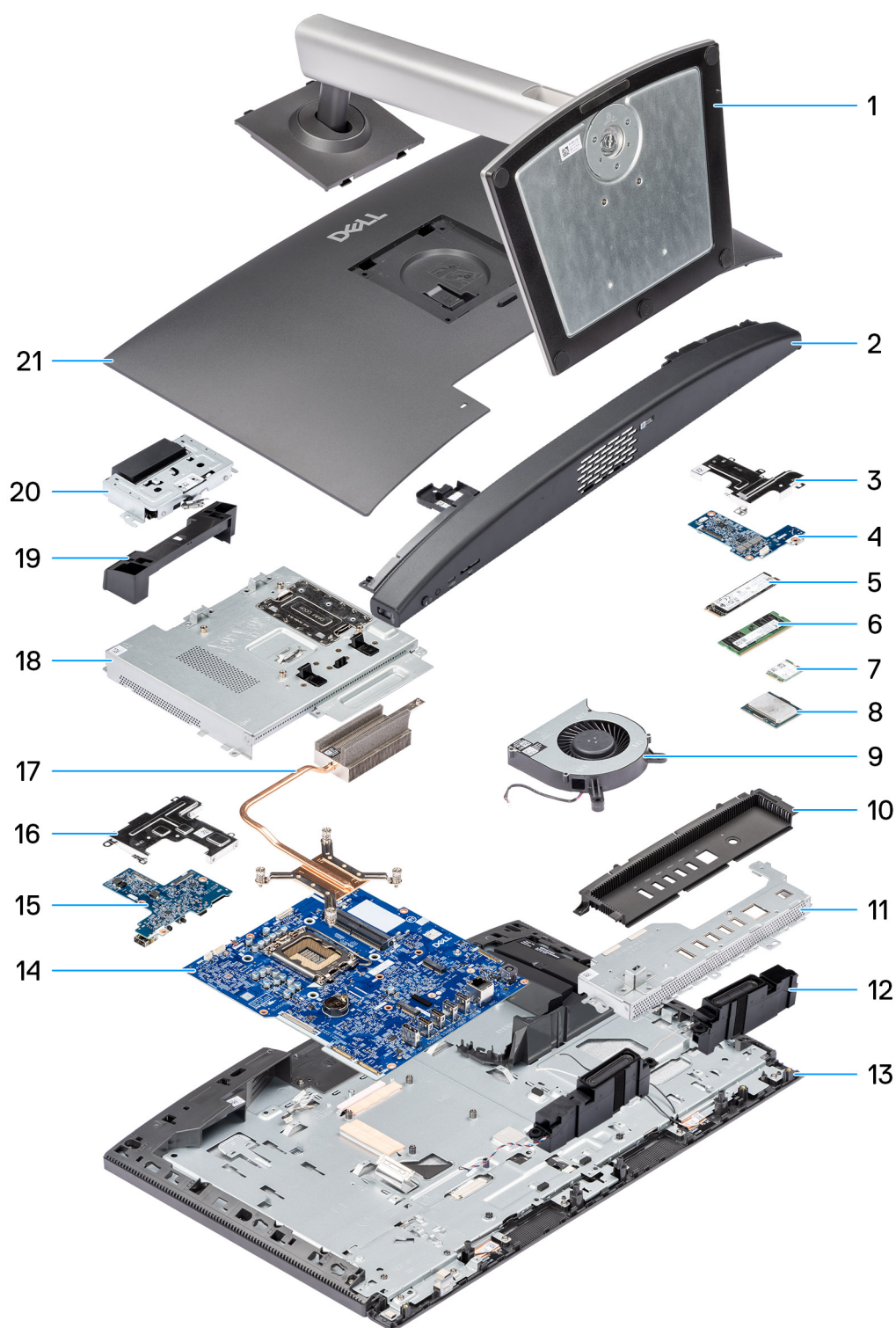
Figura 12. Componenti principali di Dell Pro 24 All-in-One QC24251
