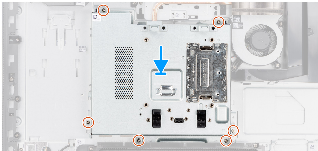
Figura 22. Installazione della protezione della scheda di sistema
