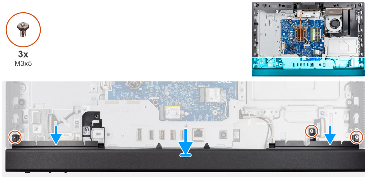
Figura 33. Installazione del coperchio inferiore
