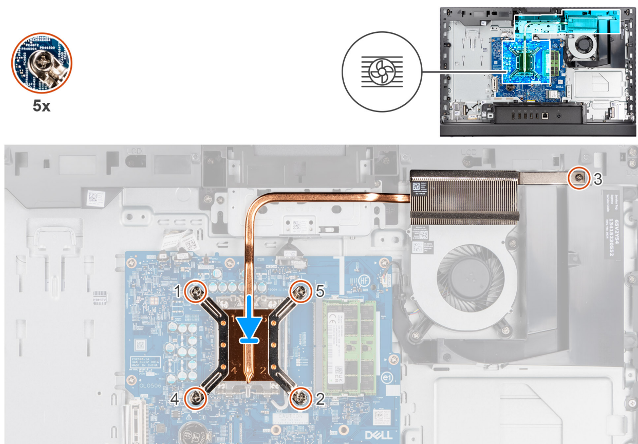
Figura 43. Installazione del dissipatore di calore
