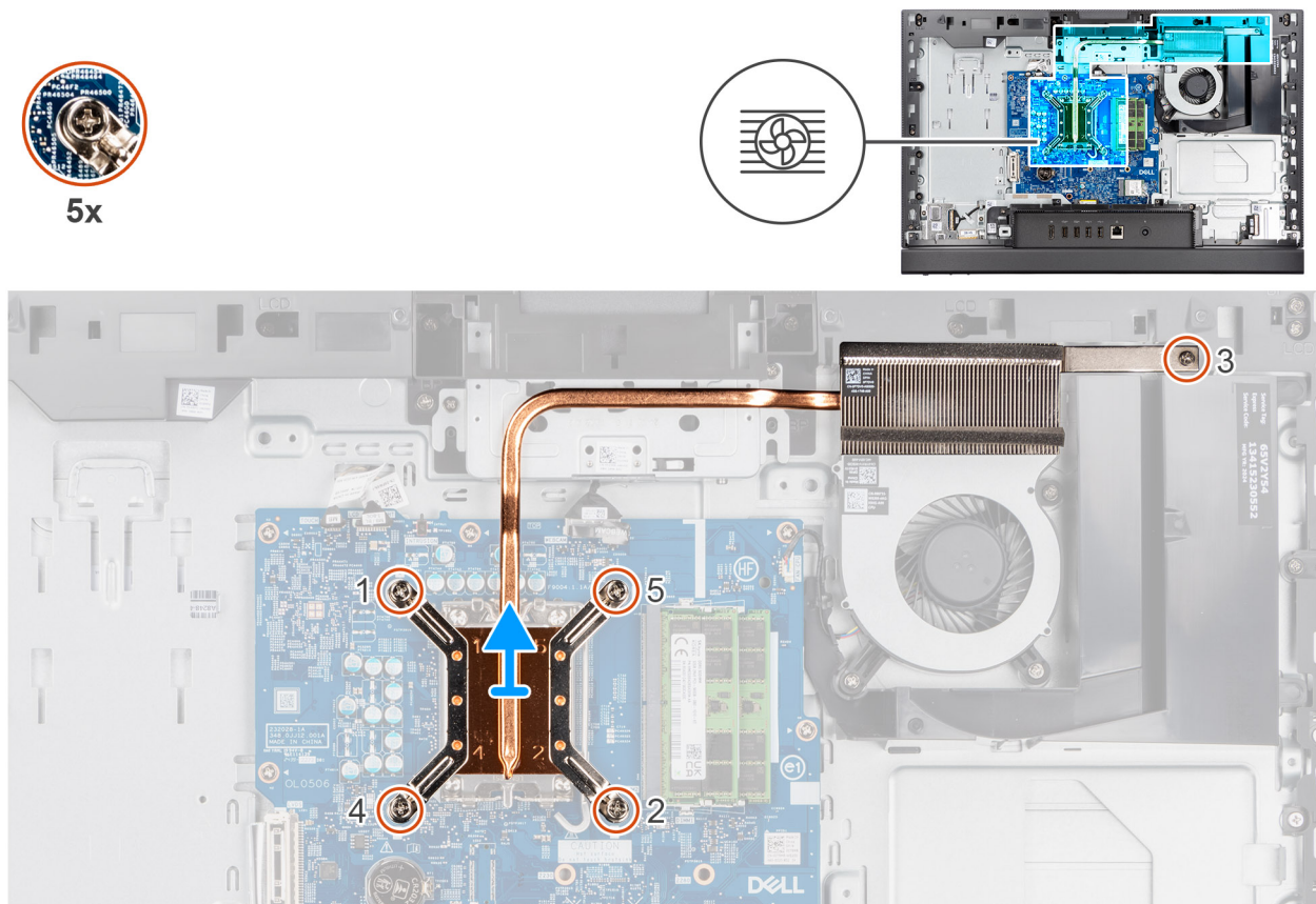
Figura 42. Rimozione del dissipatore di calore
