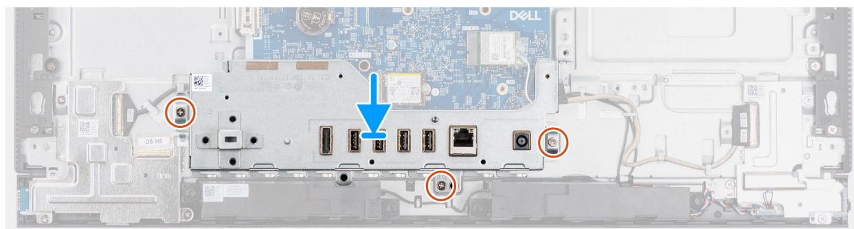
Figura 39. Installazione della staffa di I/O
