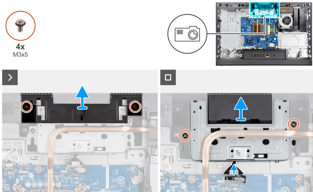
Figura 34. Rimozione del gruppo della fotocamera retraibile
