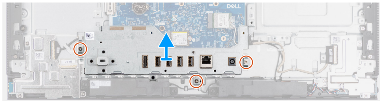
Figura 38. Rimozione della staffa di I/O
