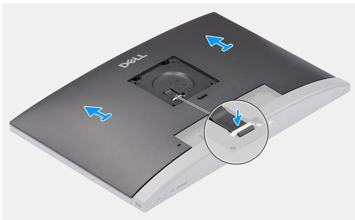
Figura 17. Rimozione del coperchio posteriore
