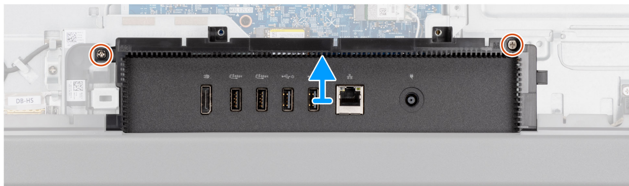
Figura 30. Rimozione del coperchio di I/O
