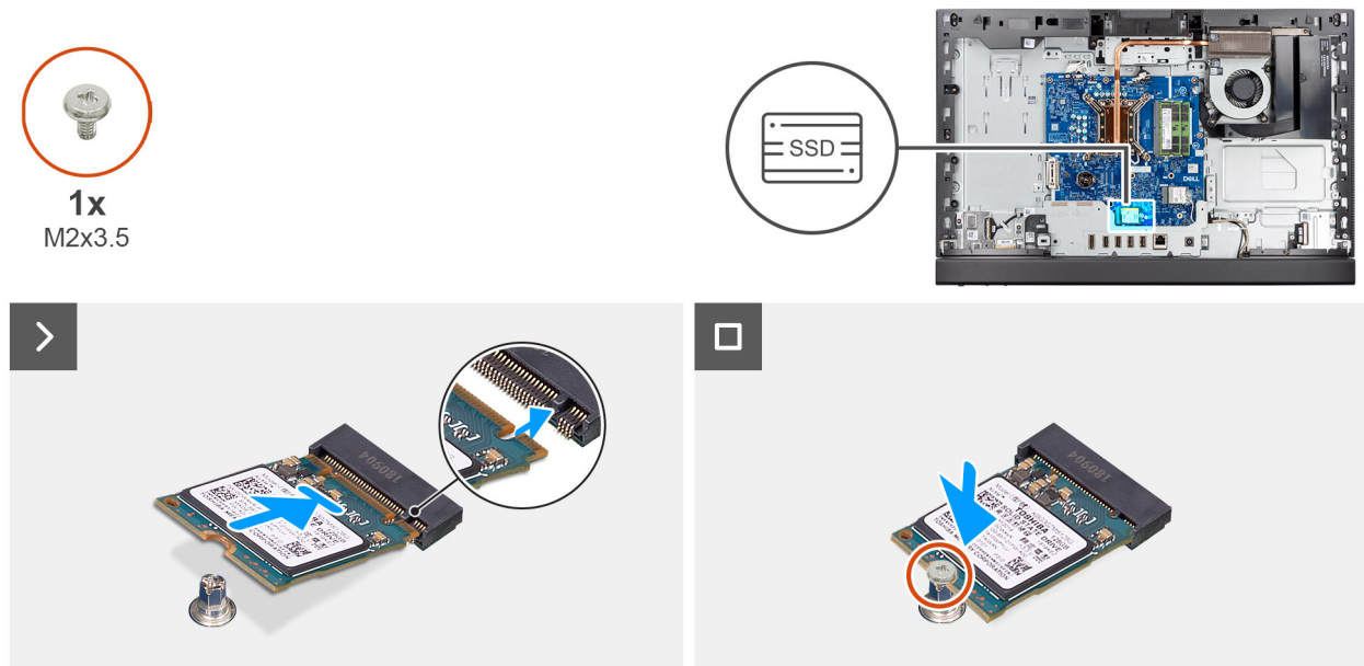
Figura 26. Installazione dell'unità SSD M.2 2230
