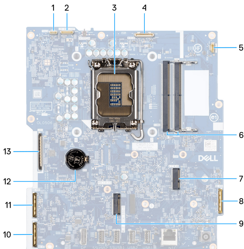
Figura 46. Callout della scheda di sistema
