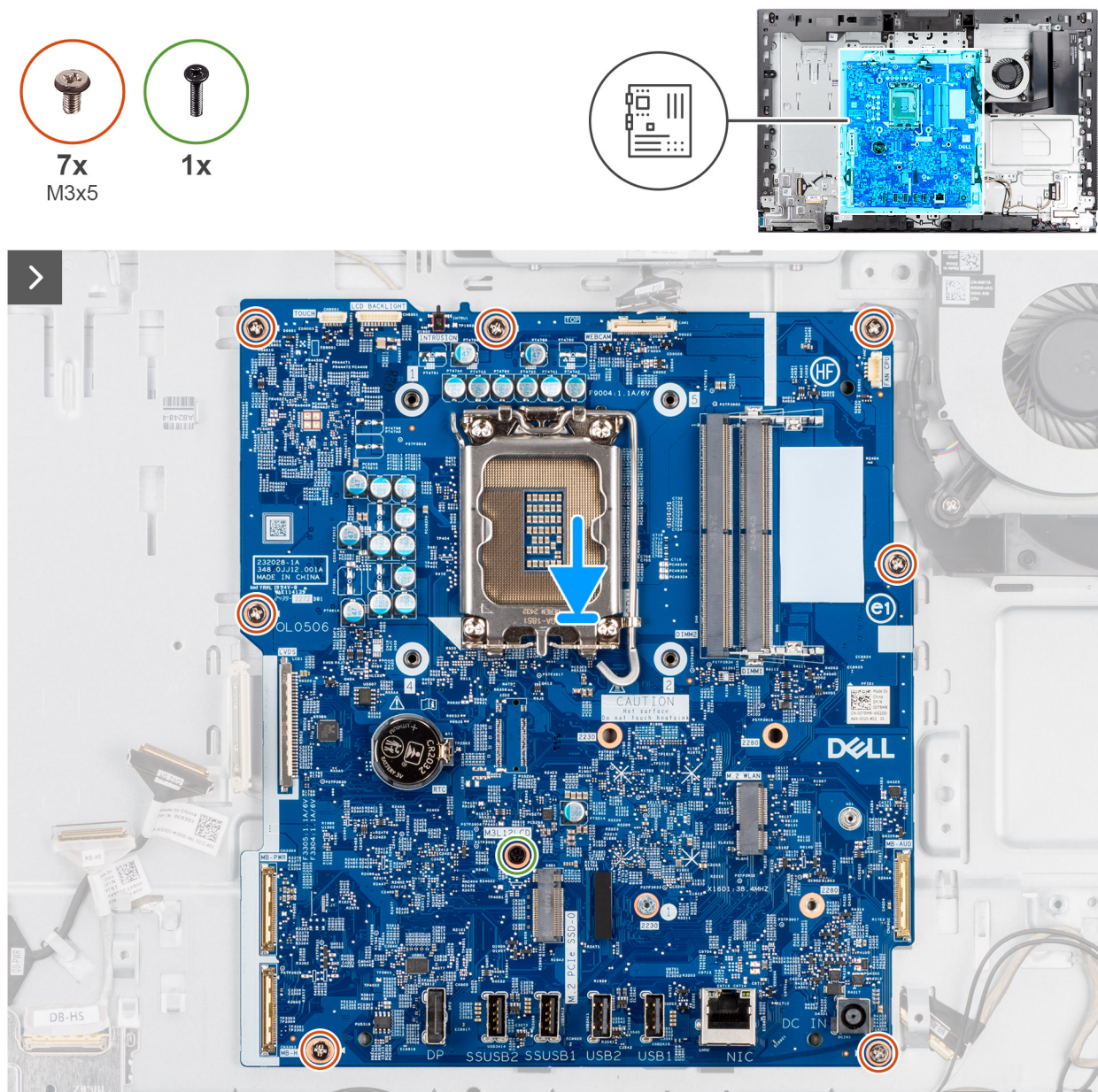
Figura 50. Installazione della scheda di sistema
