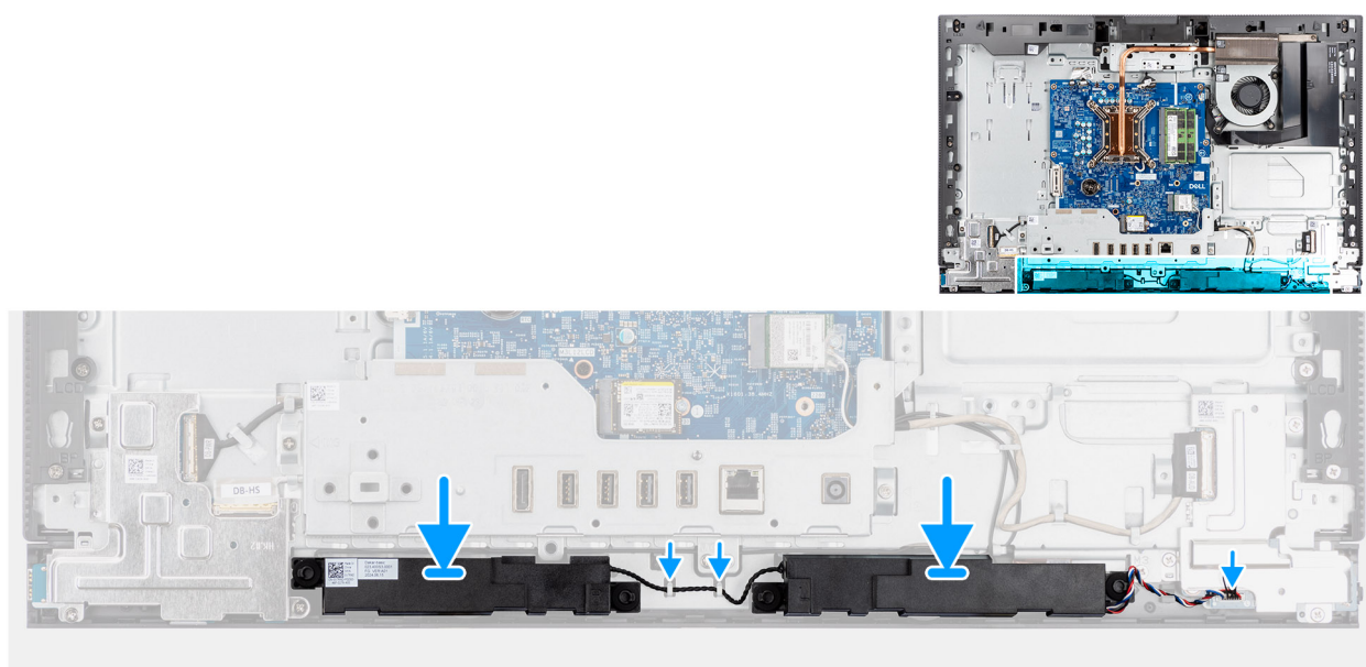
Figura 41. Installazione degli altoparlanti
