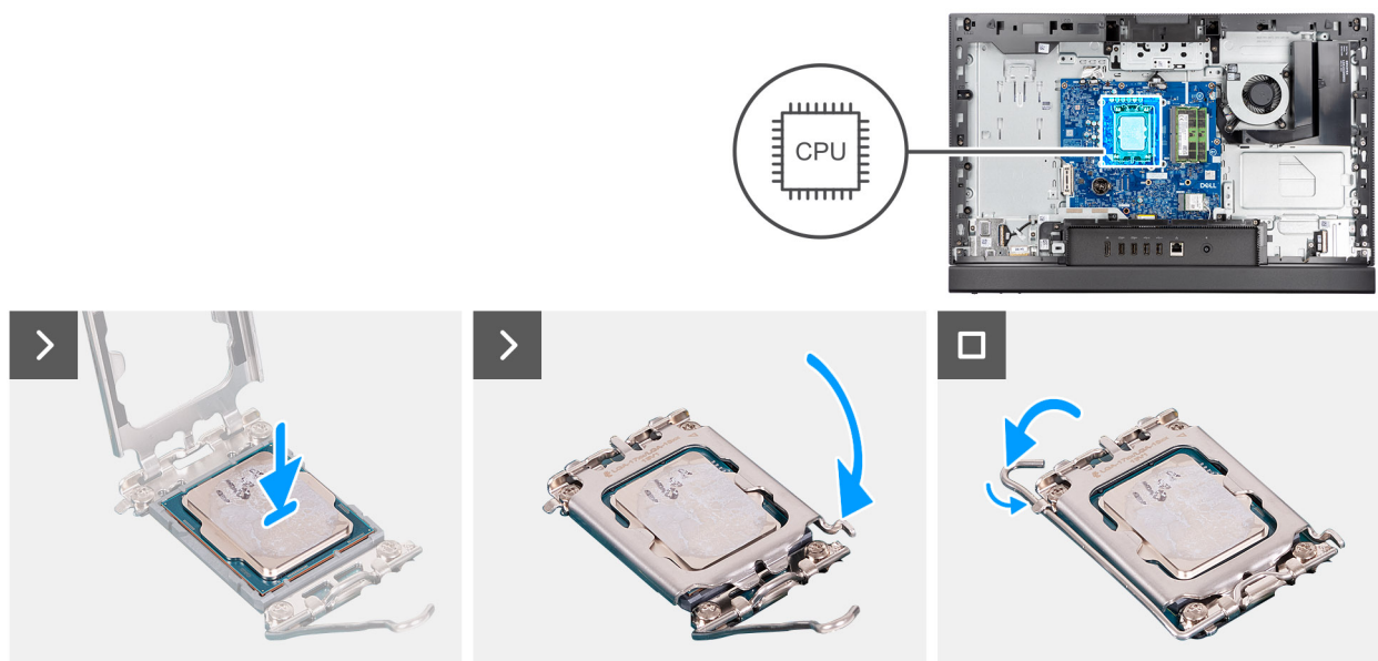
Figura 45. Installazione del processore
