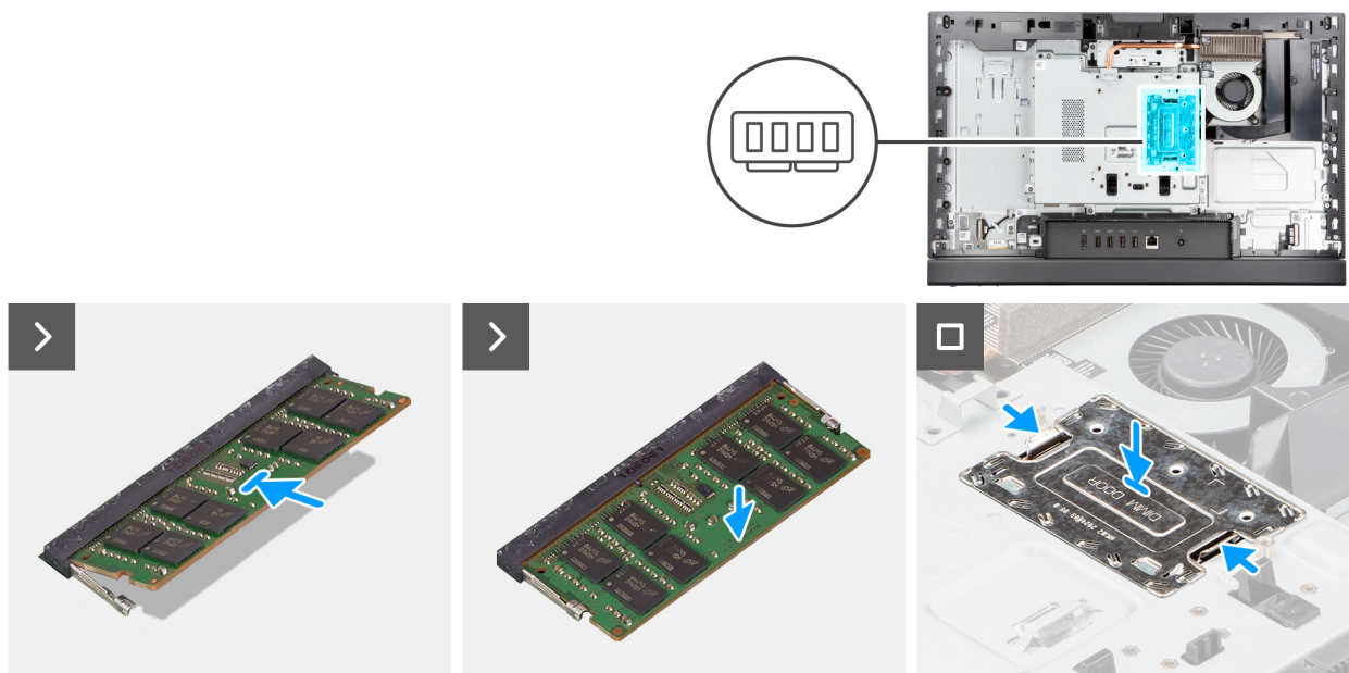
Figura 20. Installazione della memoria
