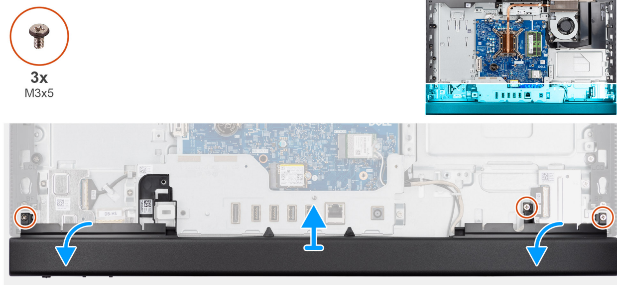
Figura 32. Rimozione del coperchio inferiore
