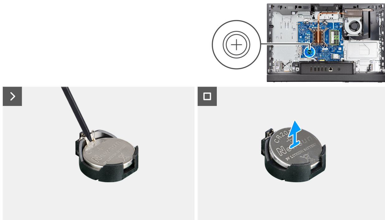
Figura 28. Rimozione della batteria a bottone
