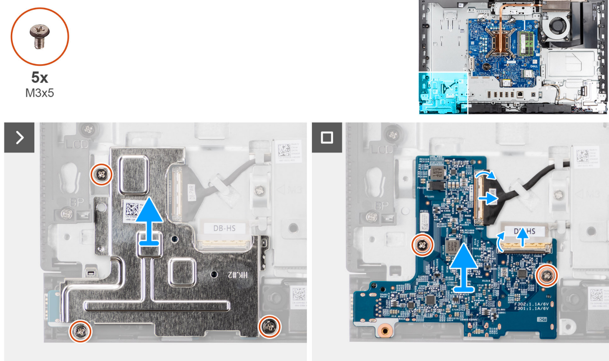
Figura 52. Rimozione della scheda del pulsante di accensione e di I/O
