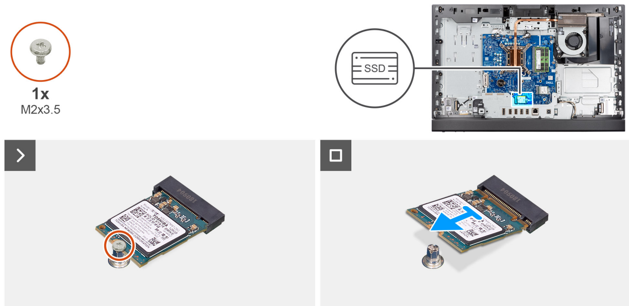
Figura 25. Rimozione dell'unità SSD M.2 2230
