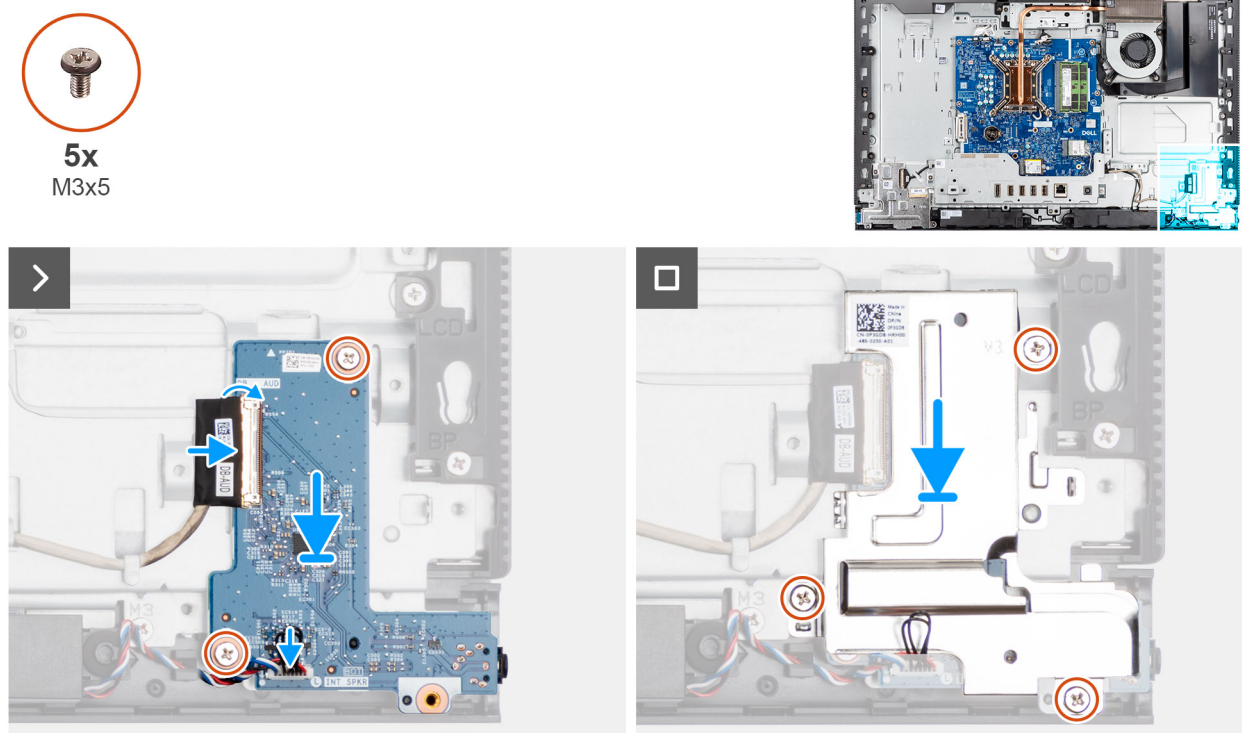
Figura 55. Installazione della scheda audio
