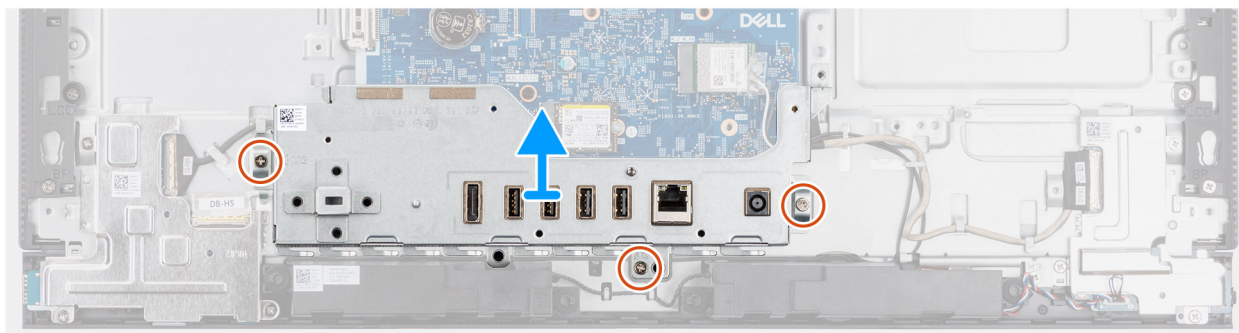
Figure 38. Retrait du support d'E/S
