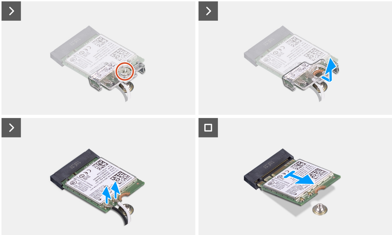
Figure 23. Retrait de la carte sans fil
