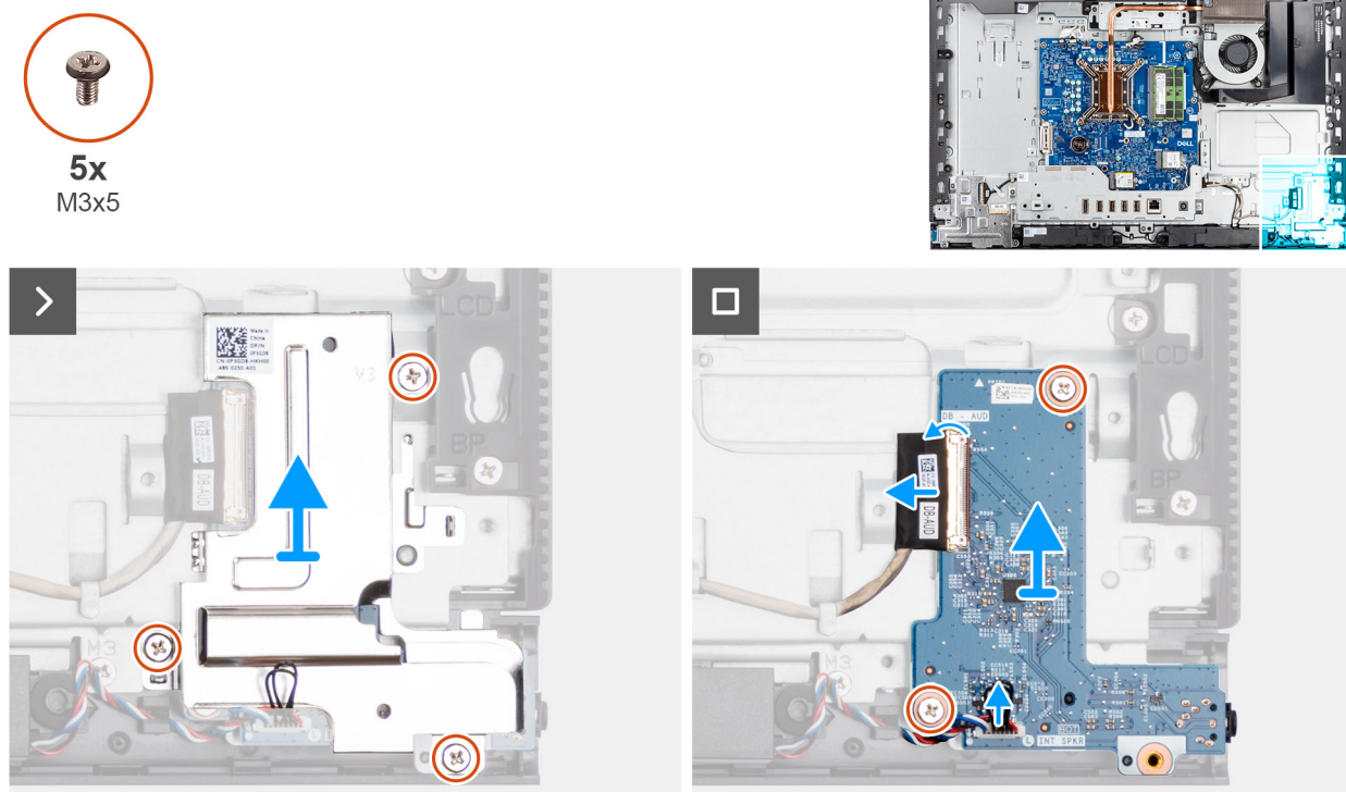
Figure 54. Retrait de la carte audio
