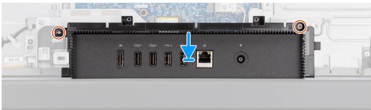
Figure 31. Installation du cache d'E/S
