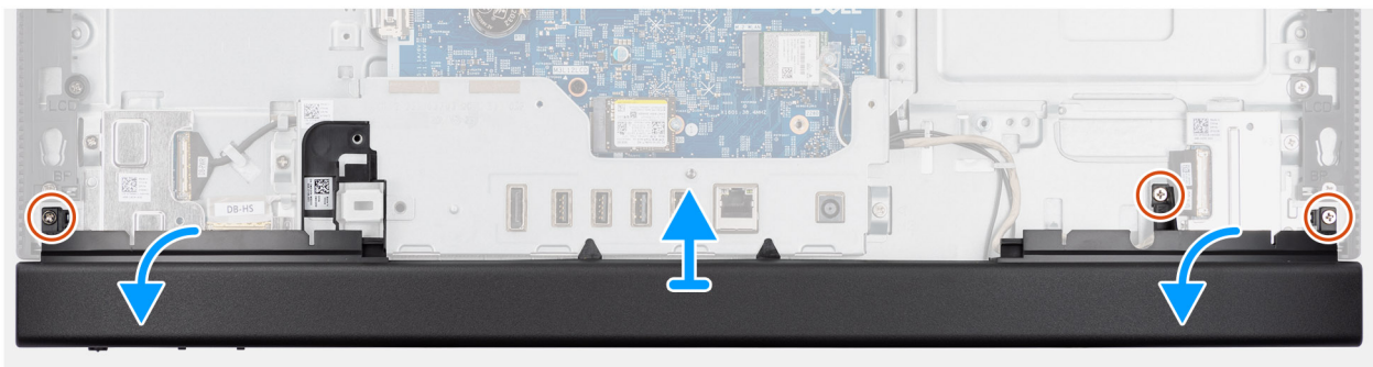
Figure 32. Retrait du cache inférieur
