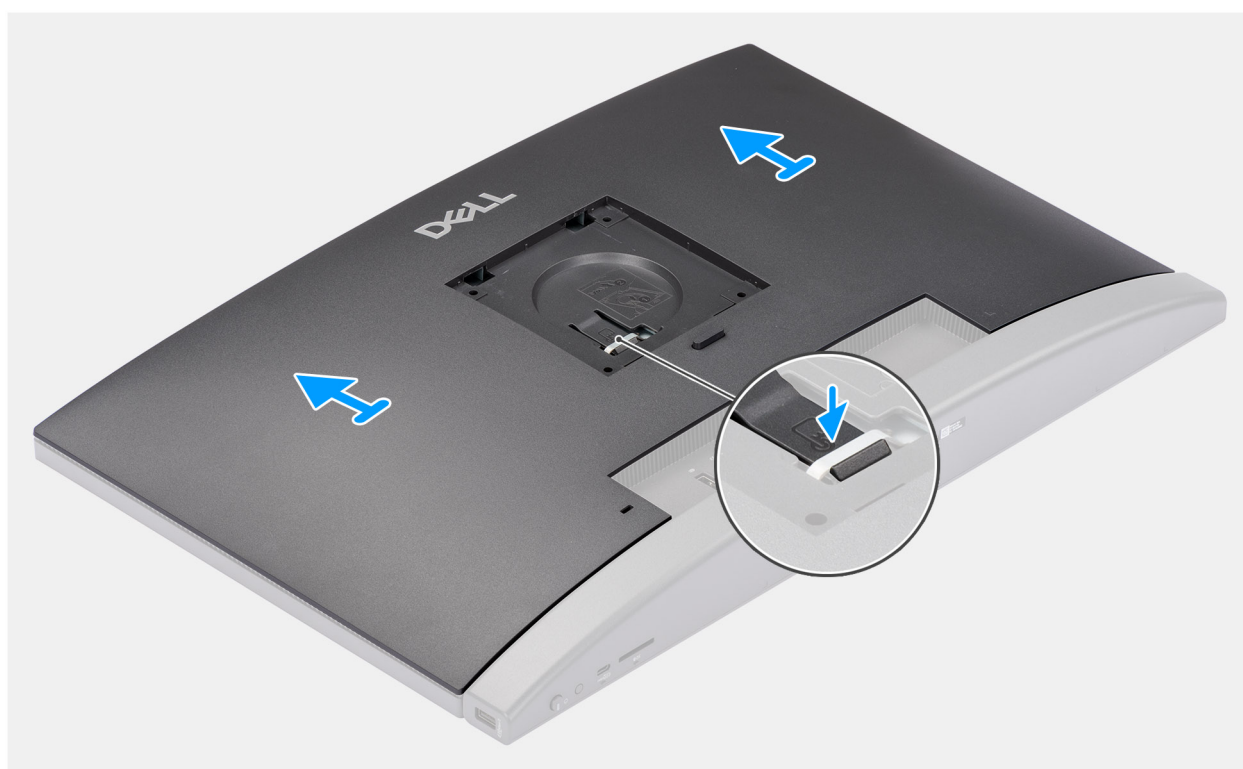
Figure 17. Retrait du capot arrière
