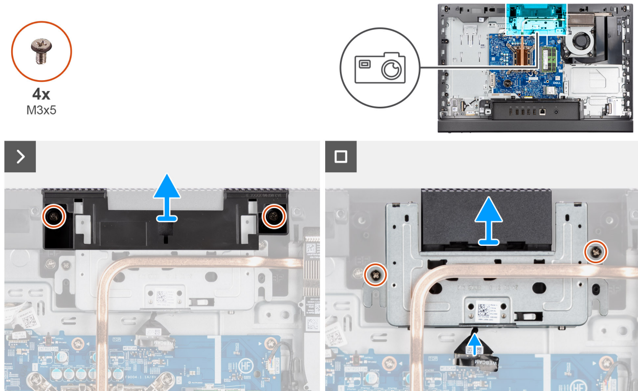
Figure 34. Retrait de l'assemblage de la caméra escamotable
