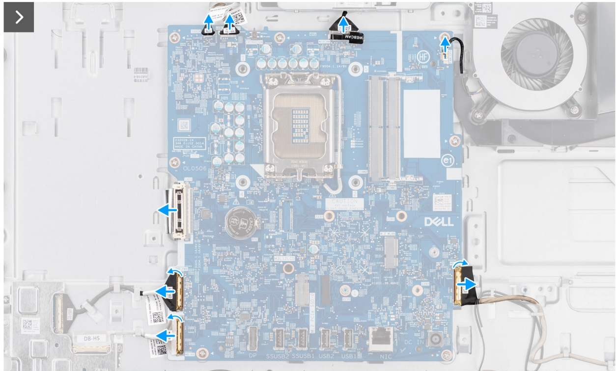
Figure 47. Retrait de la carte système
