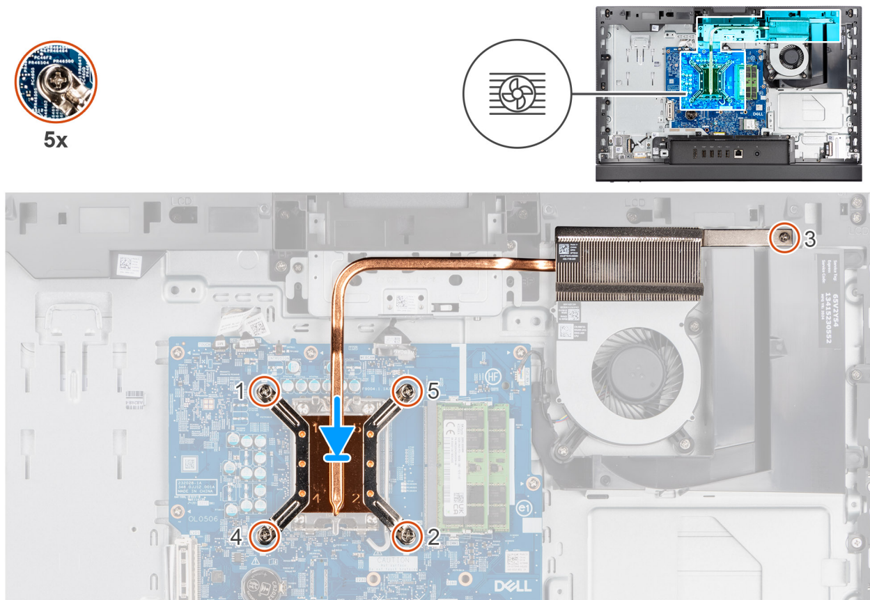
Figure 43. Installation du dissipateur de chaleur
