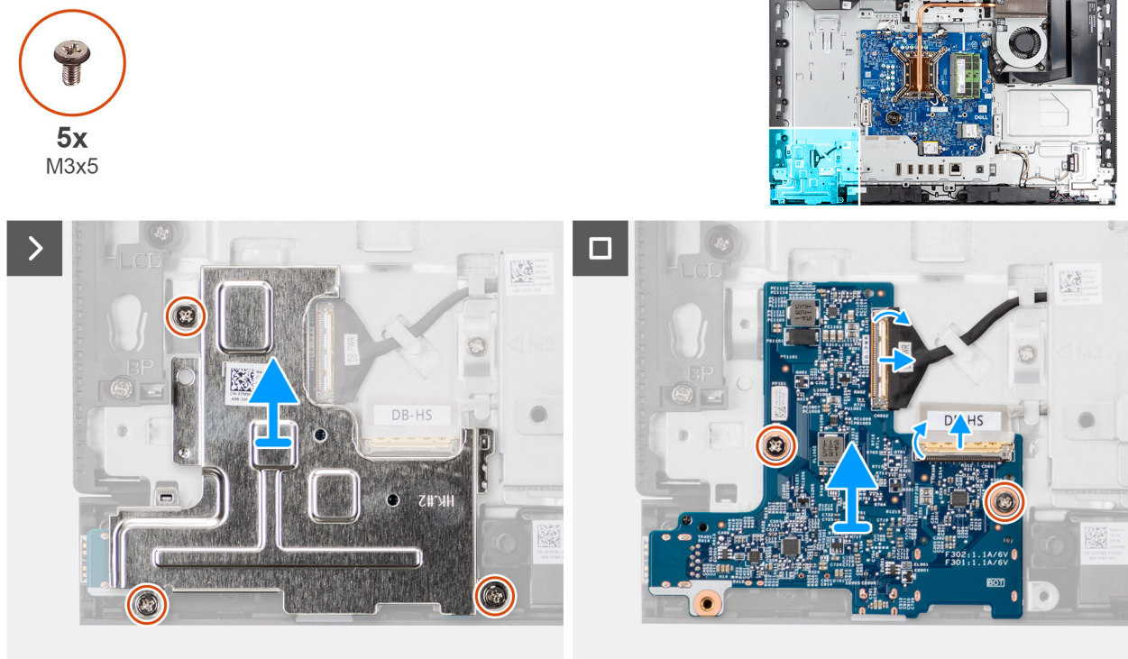
Figure 52. Retrait de la carte du bouton d'alimentation et de la carte d'E/S
