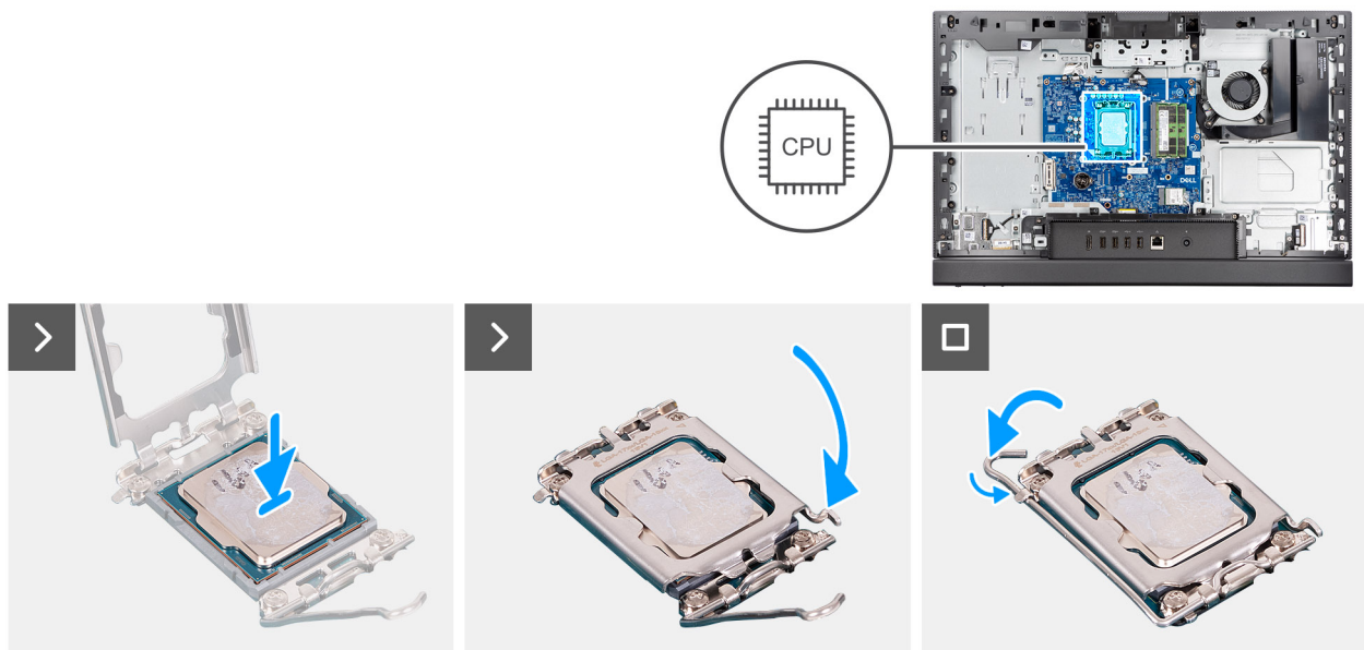
Figure 45. Installation du processeur
