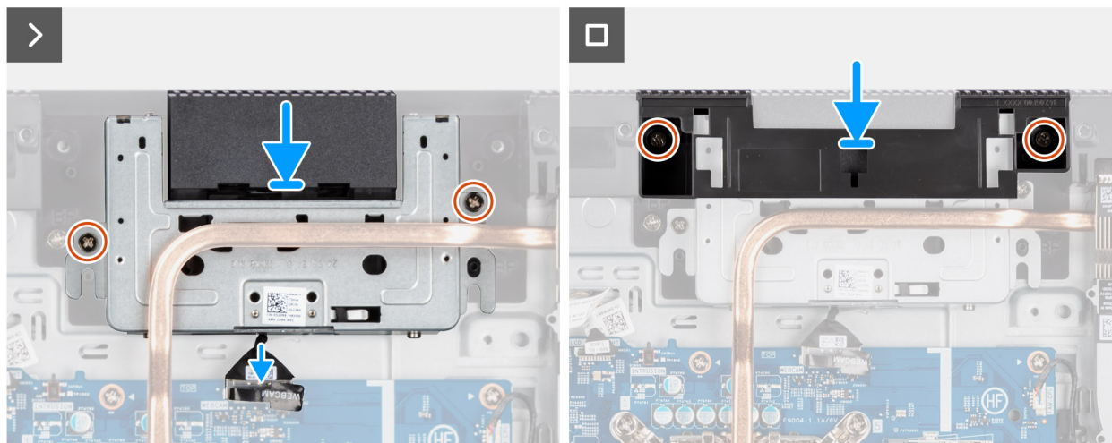
Figure 35. Installation de l'assemblage de la caméra escamotable
