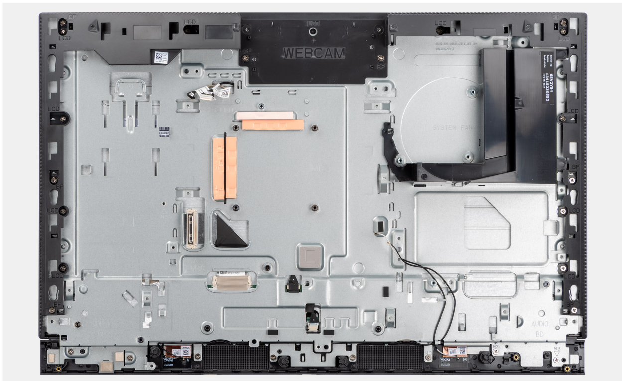
Figure 57. Retrait de la base de l'assemblage d'écran
