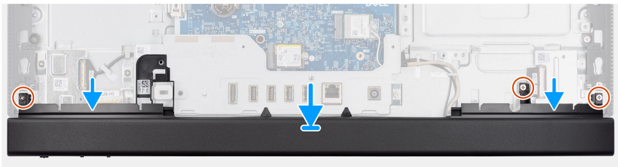
Figure 33. Installation du capot inférieur
