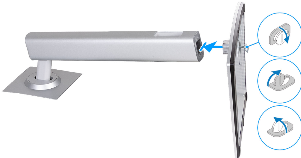
Figure 8. Installation de la base du socle
