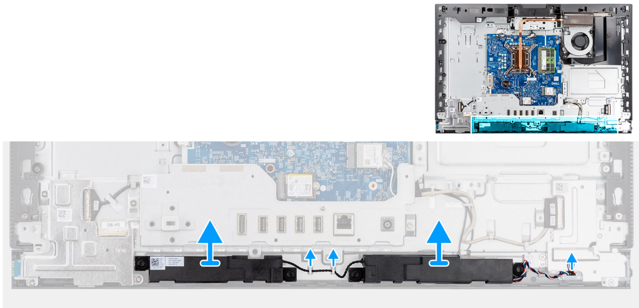
Figure 40. Retrait des haut-parleurs
