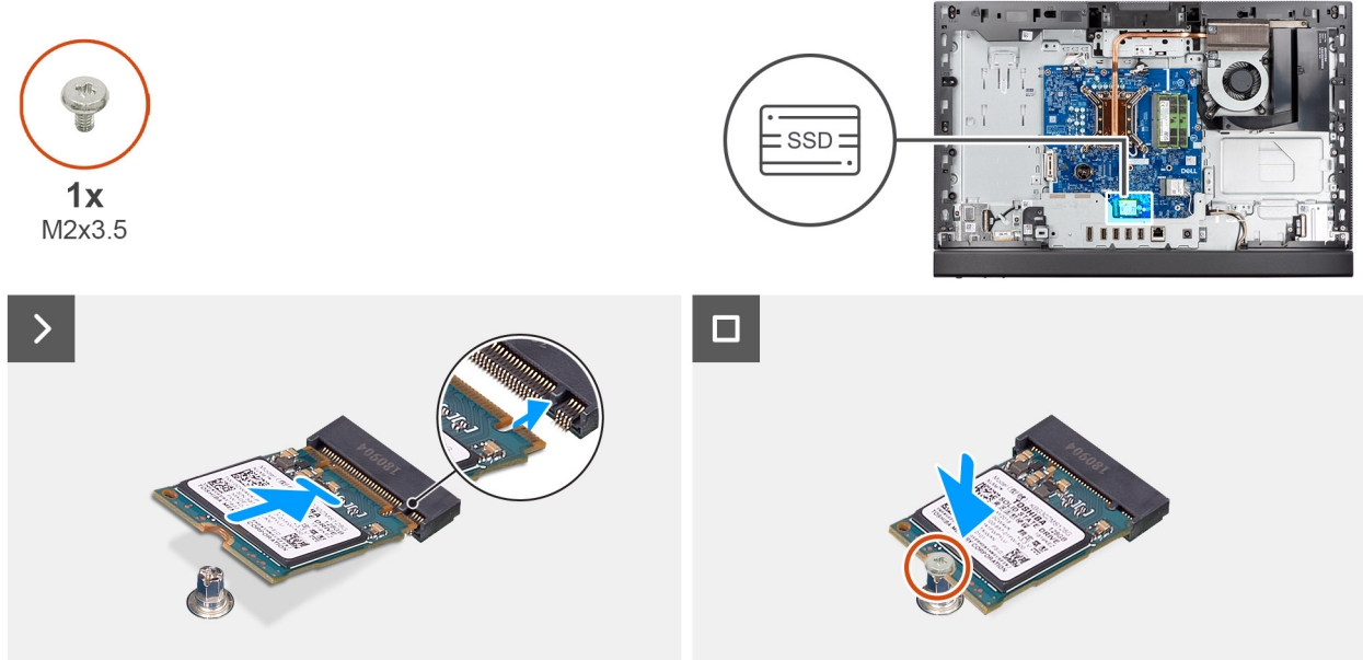
Figure 26. Installation du disque SSD M.2 2230
