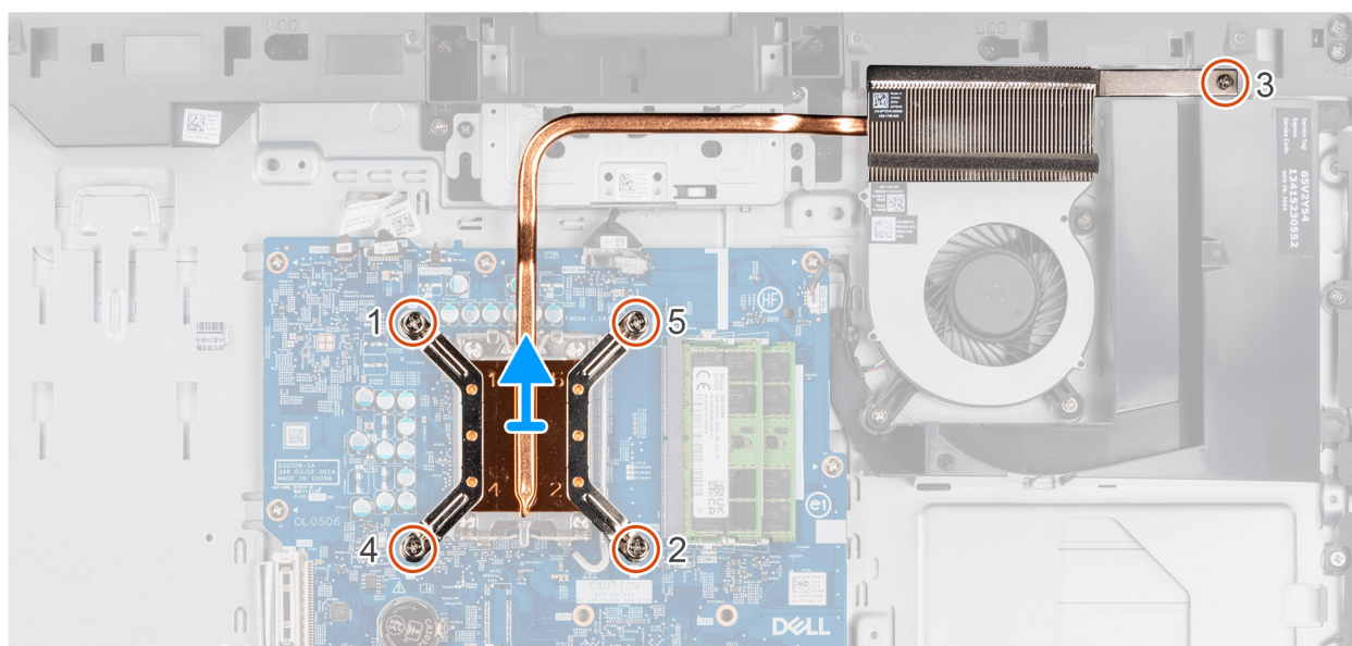
Figure 42. Retrait du dissipateur de chaleur
