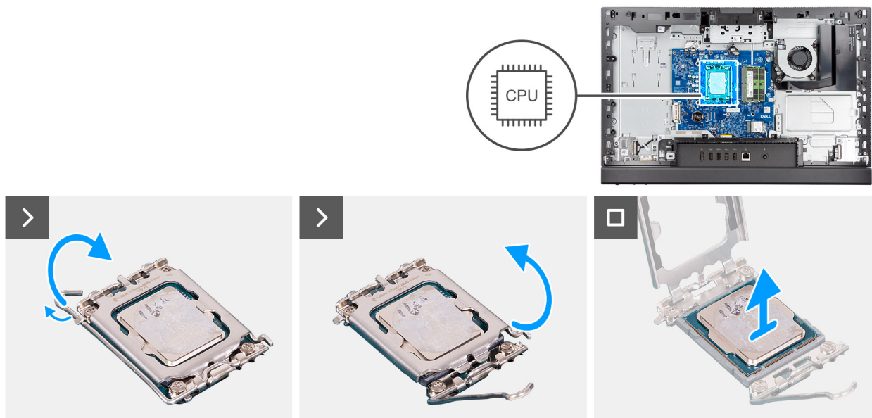
Figure 44. Retrait du processeur
