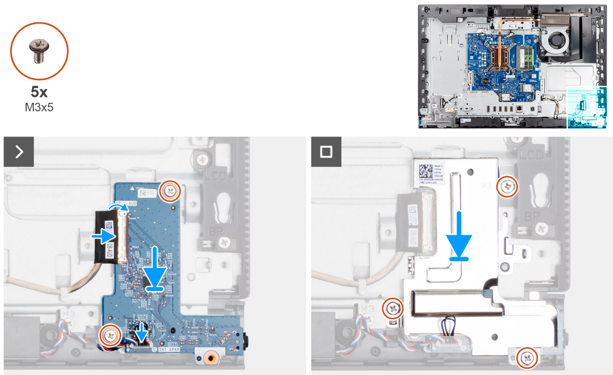
Figure 55. Installation de la carte audio
