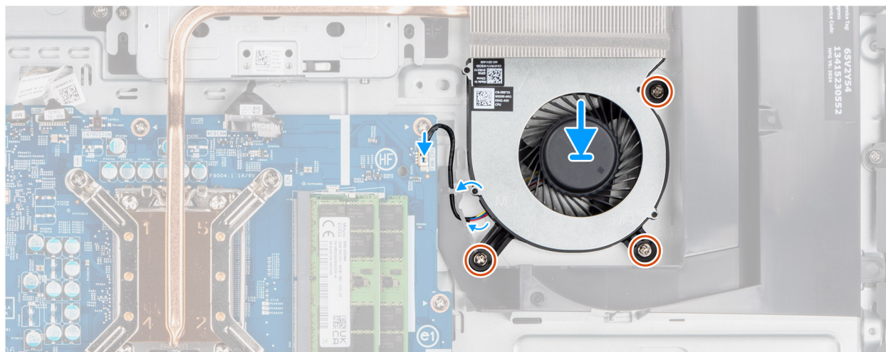
Figure 37. Installation du ventilateur
