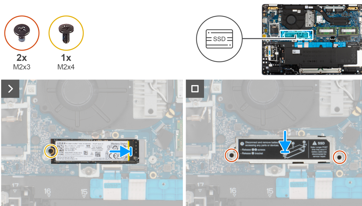
Figura 28. Installazione dell'SSD M.2230
