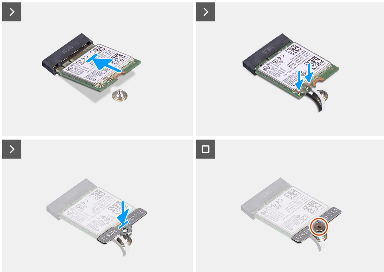
Figura 34. Installazione della scheda WLAN
