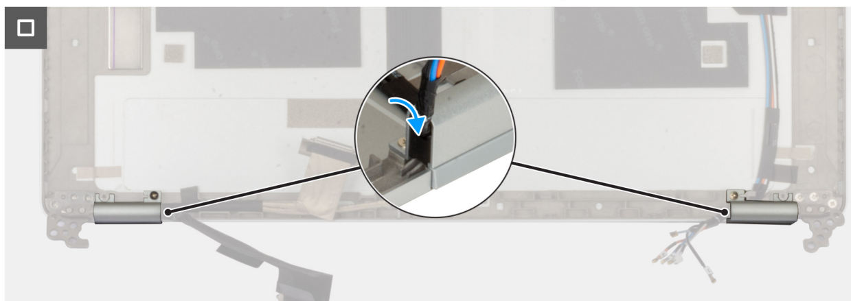
Ilustración 70. Instalación de la tapa de la bisagra de la pantalla
