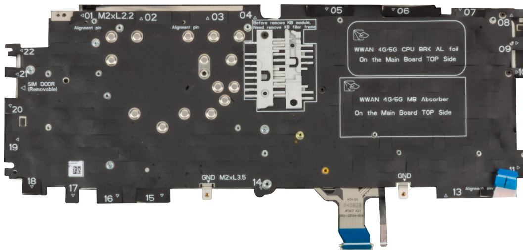
Ilustración 84. Instalación del relleno del teclado
