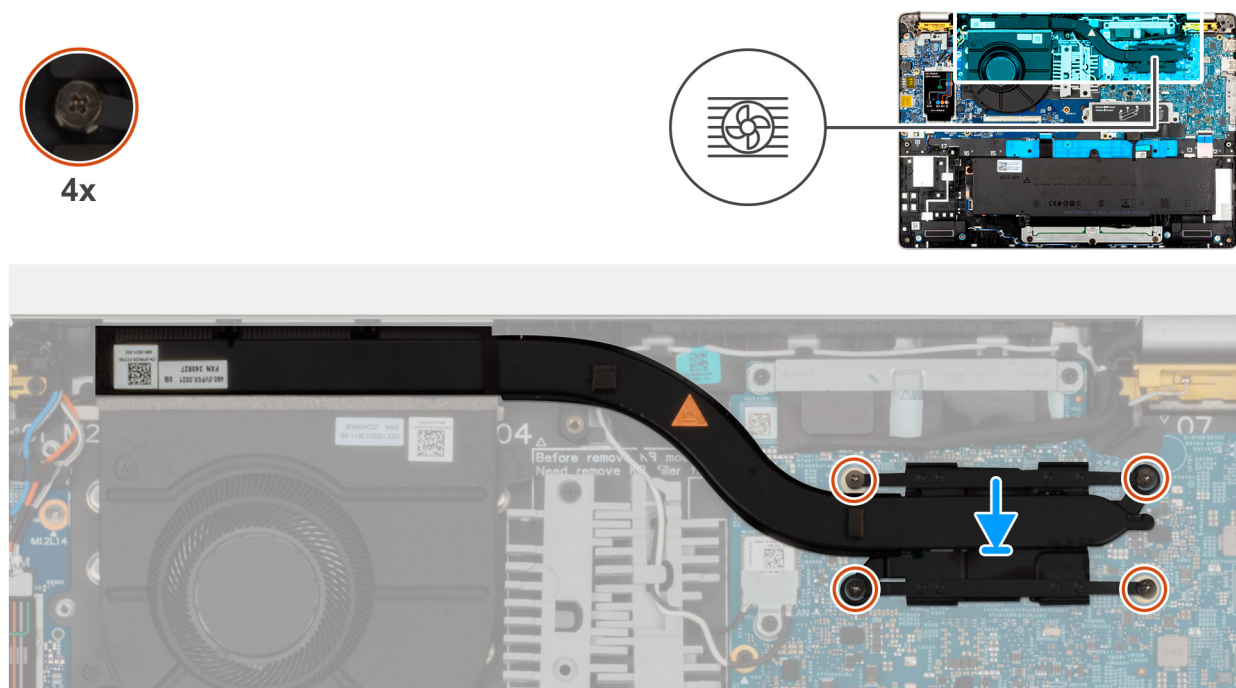
Ilustración 46. Instalación del dissipador de calor
