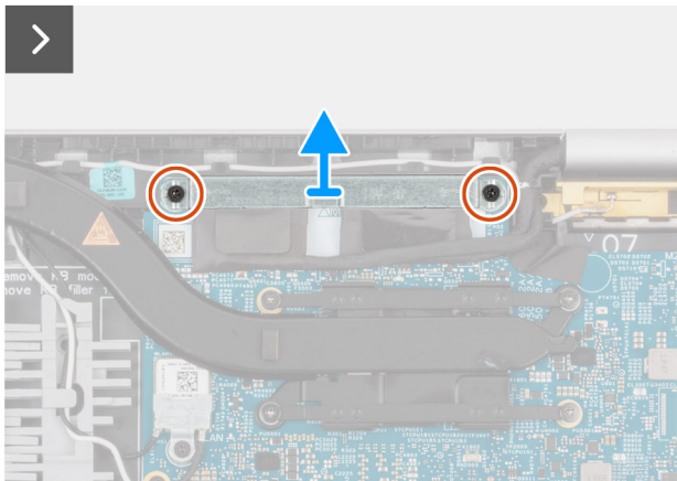
Ilustración 55. Extracción del ensamblaje de la pantalla
