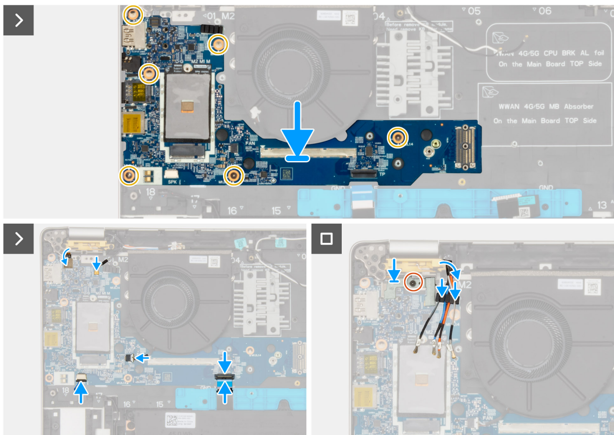
Ilustración 52. Instalación de la placa de I/O
