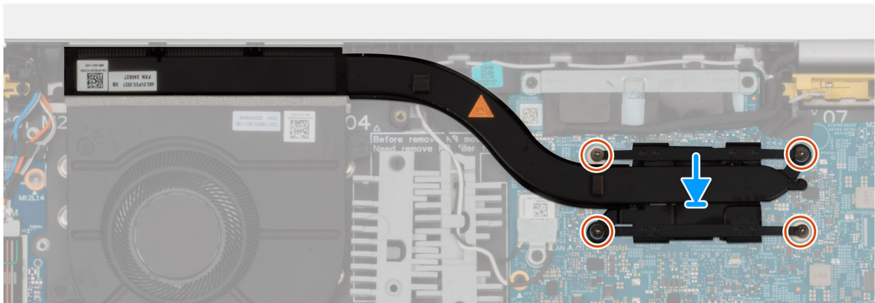
Ilustración 46. Instalación del disipador de calor
