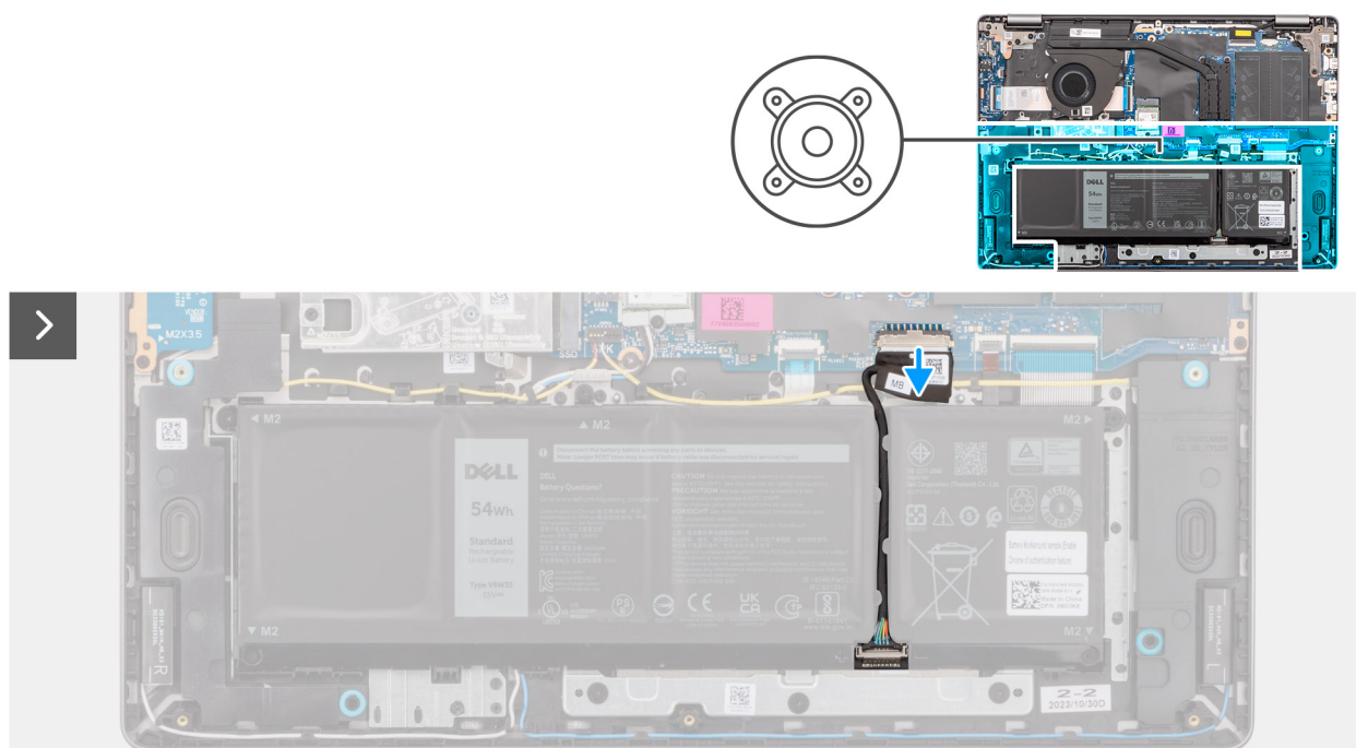
Rysunek 29. Odłączanie kabla baterii
