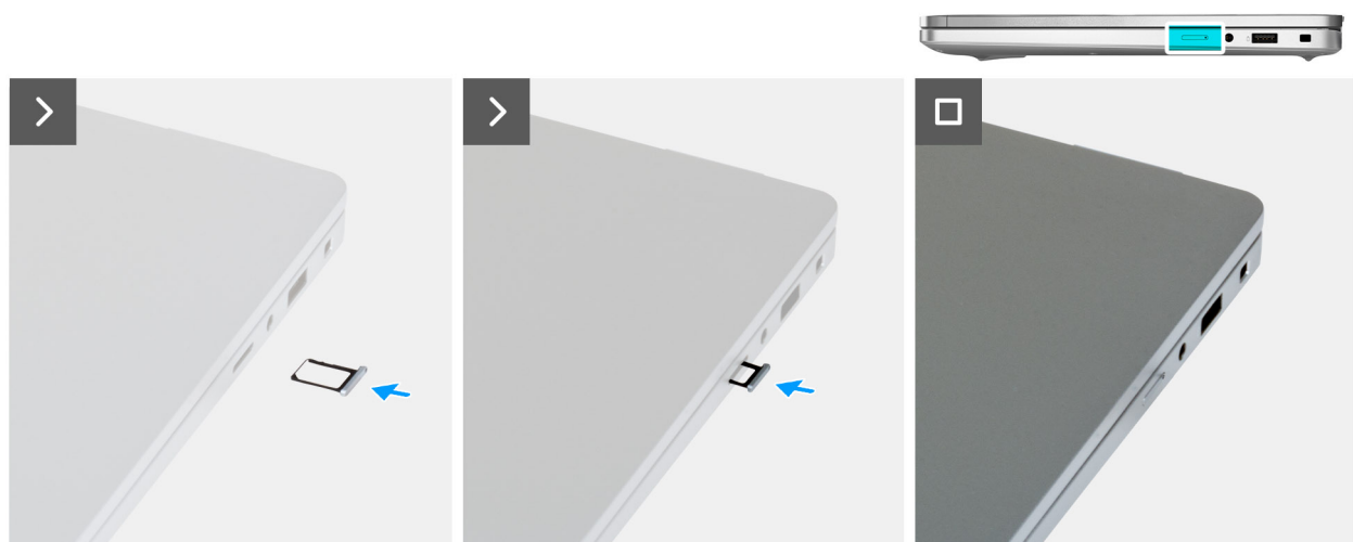
איור 16. התקנת מגש כרטיס ה-SIM
