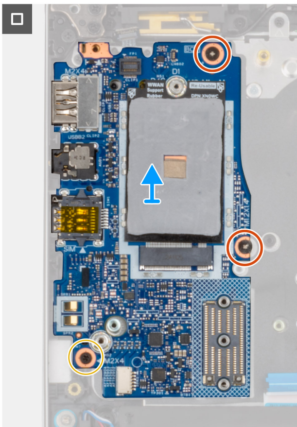
איור 62. תמונה: הסרת לוח הקלט/פלט
