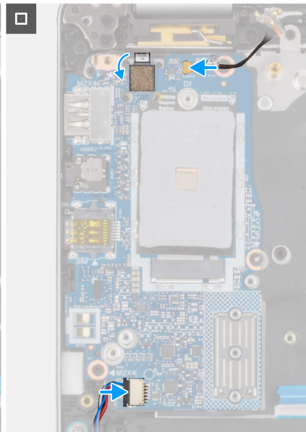
איור 63. התקנת לוח הקלט/פלט
