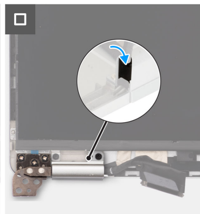
איור 83. התקנת כבל הצג
