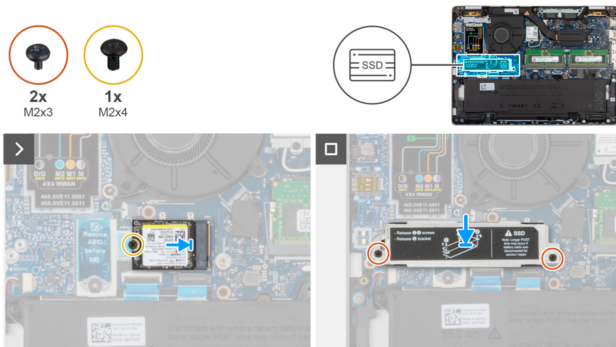
איור 36. התקנת ה-SSD מסוג M.2 2230
