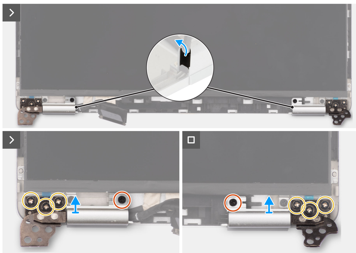
איור 73. הסרת צירי הצג
