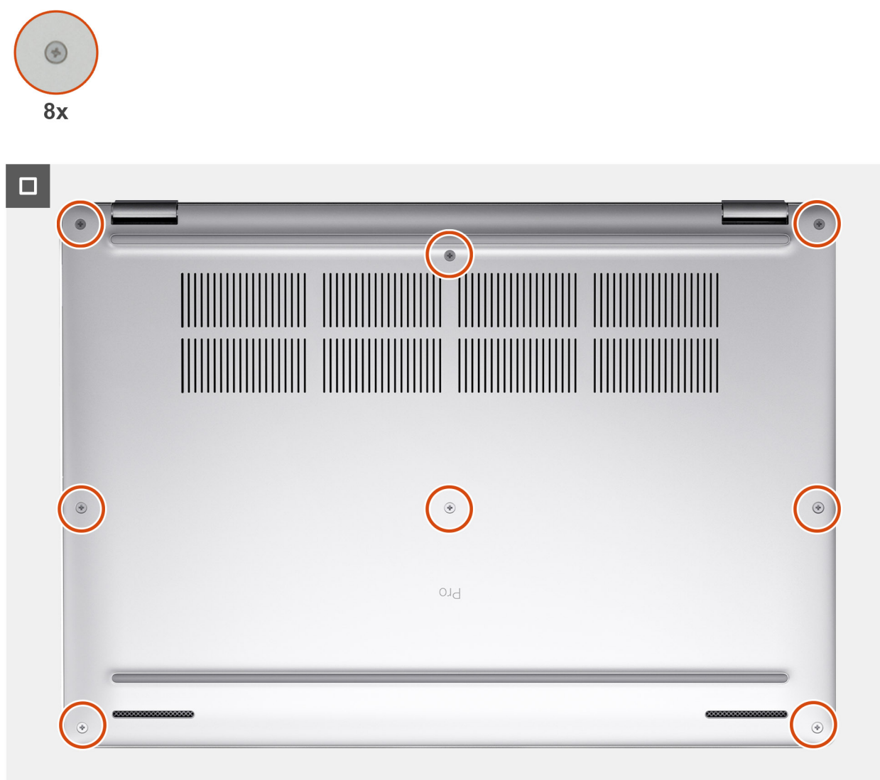
איור 22. התקנת כיסוי הבסיס
