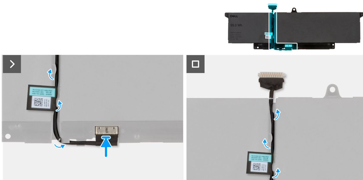
איור 26. התקנת כבל הסוללה
