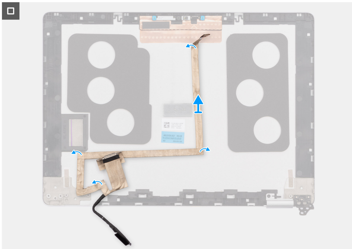
איור 81. הסרת כבל הצג
