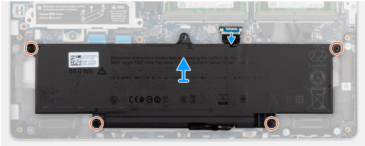
איור 19. ניתוק כבל הסוללה
