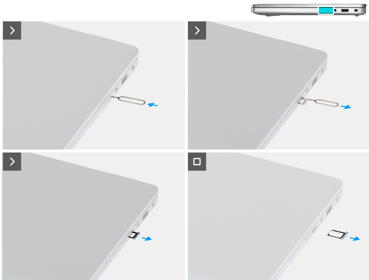
איור 15. הסרת מגש כרטיס ה-SIM
