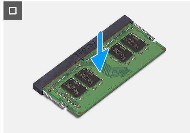
איור 28. התקנת מודולי הזיכרון
