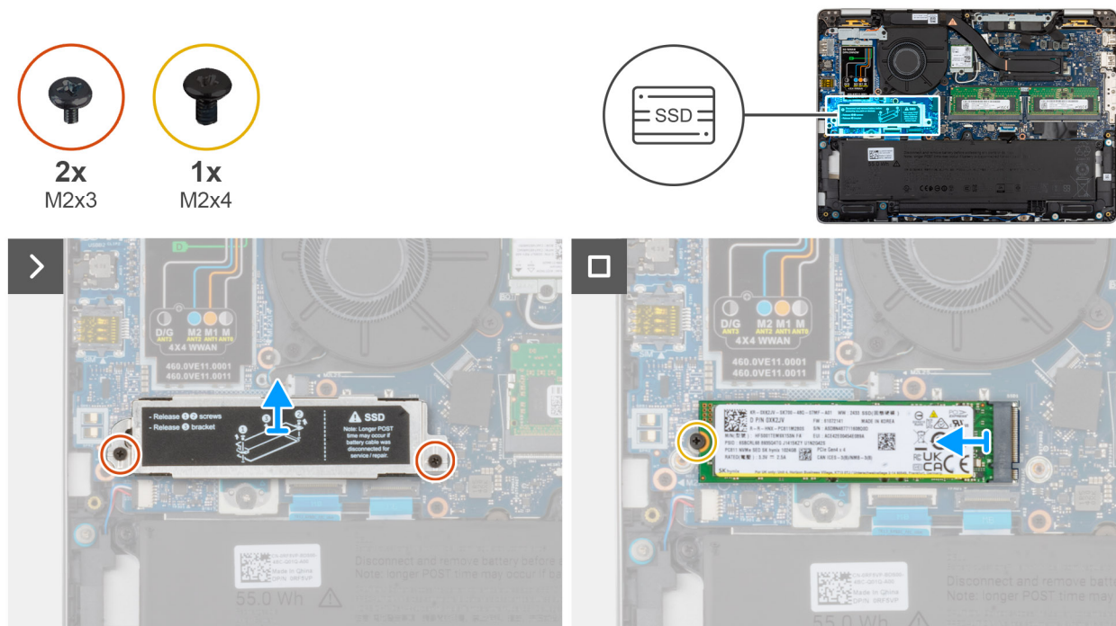
איור 37. הסרת ה-SSD מסוג M.2 2280
