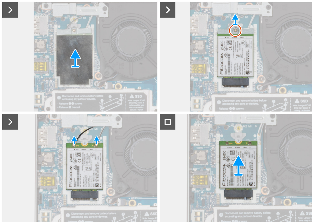
1x M1.6x3.2
