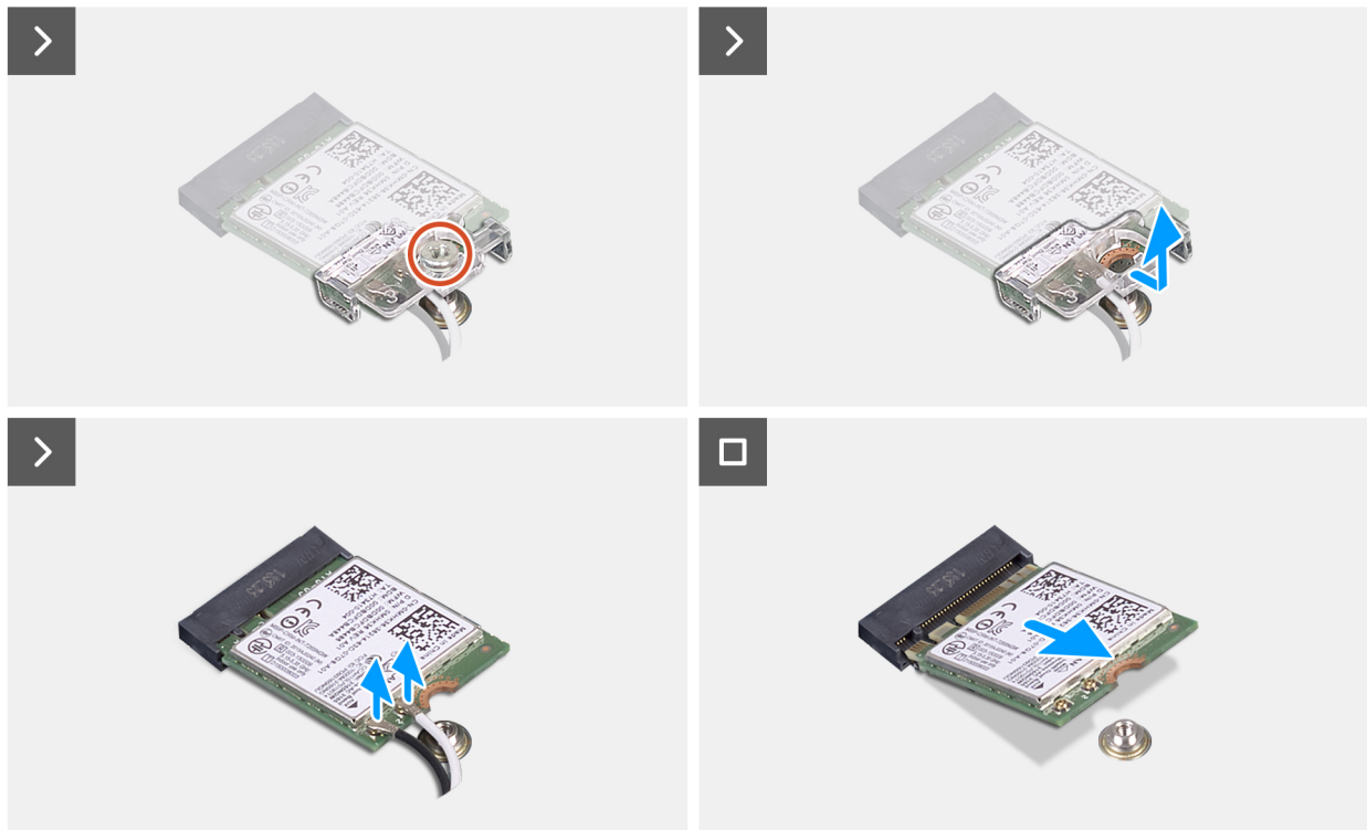
Ilustración 29. Extracción de la tarjeta inalámbrica
