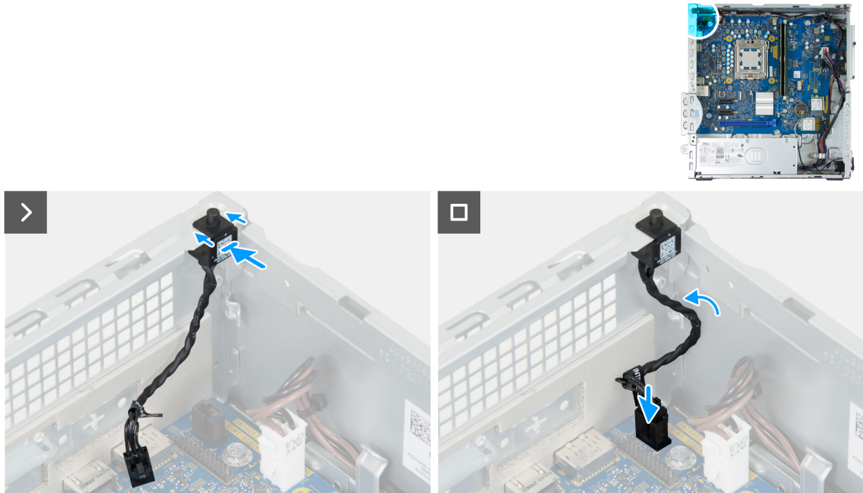
Ilustración 43. Instalación del switch de intrusión
