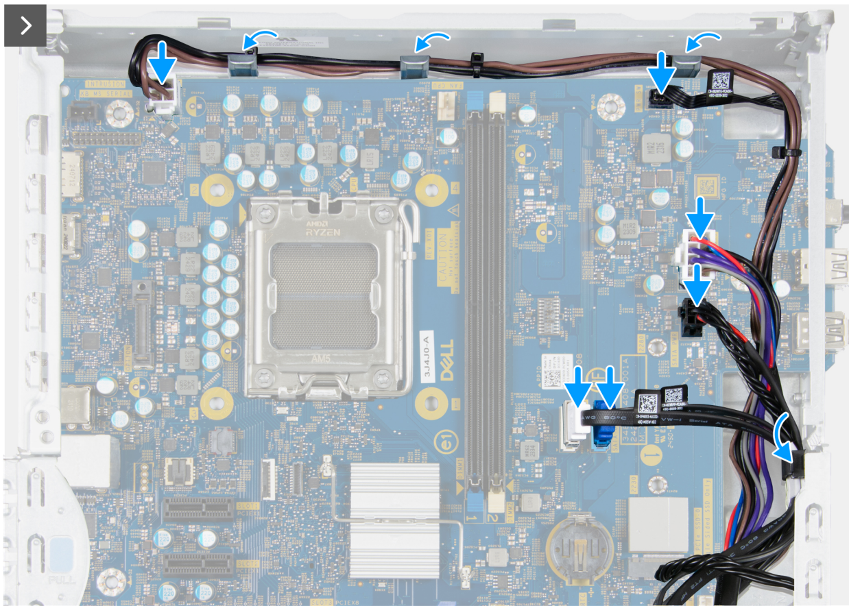
Ilustración 70. Instalación de la tarjeta madre
