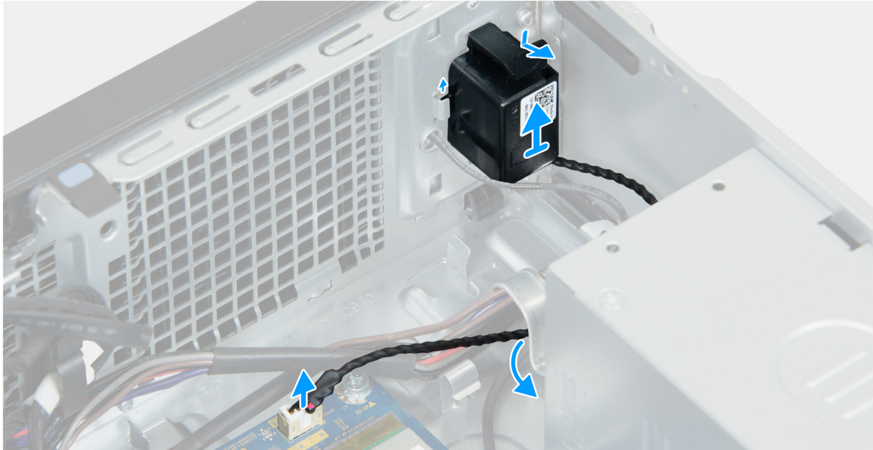
Ilustración 18. Extracción del altavoz interno
