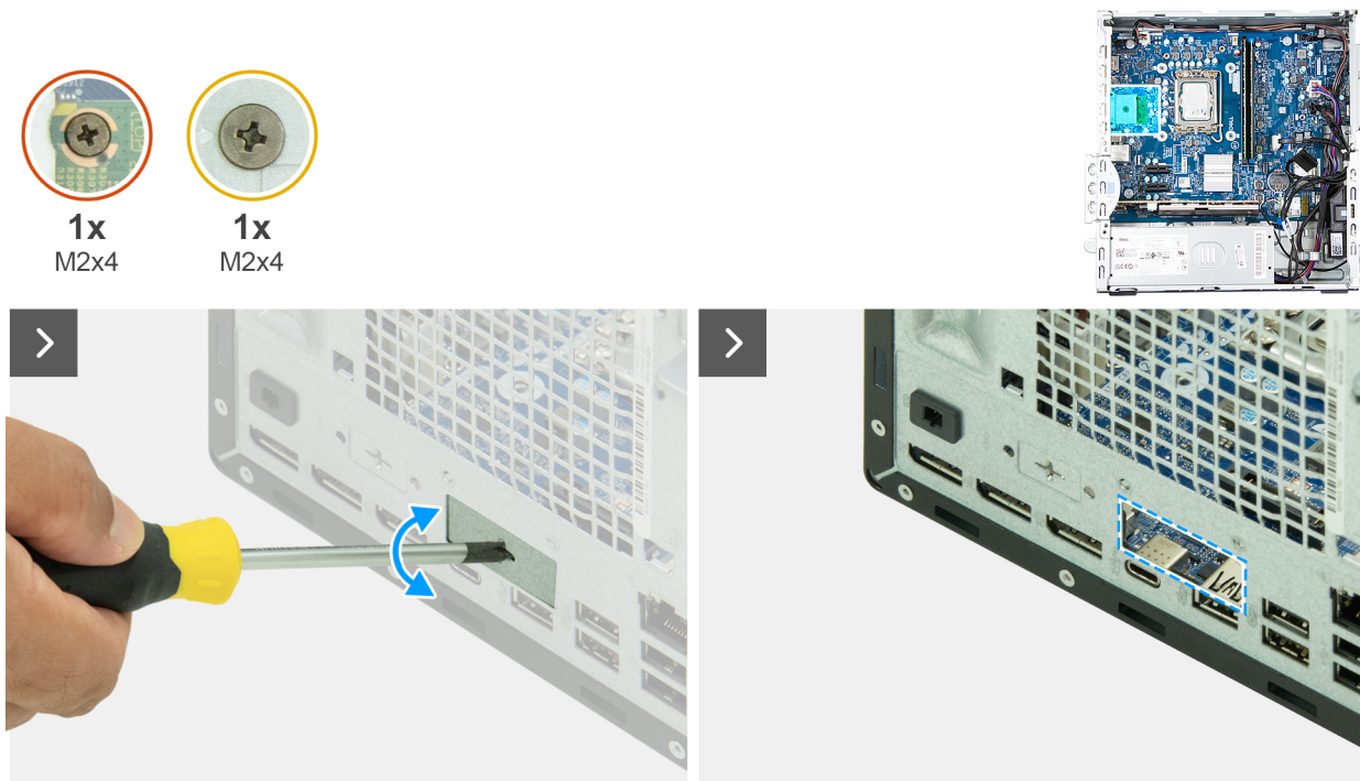
Ilustración 55. Instalación del módulo de puerto opcional
