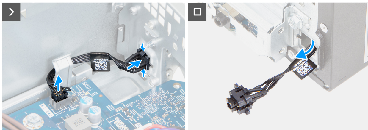
Ilustración 44. Extracción del botón de encendido
