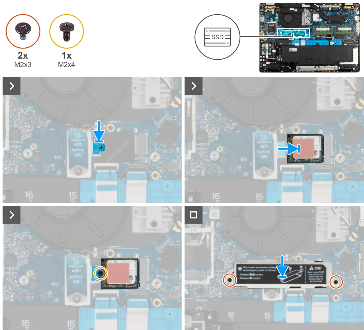
Abbildung 25. Einbauen des M.2-2280-SSD
