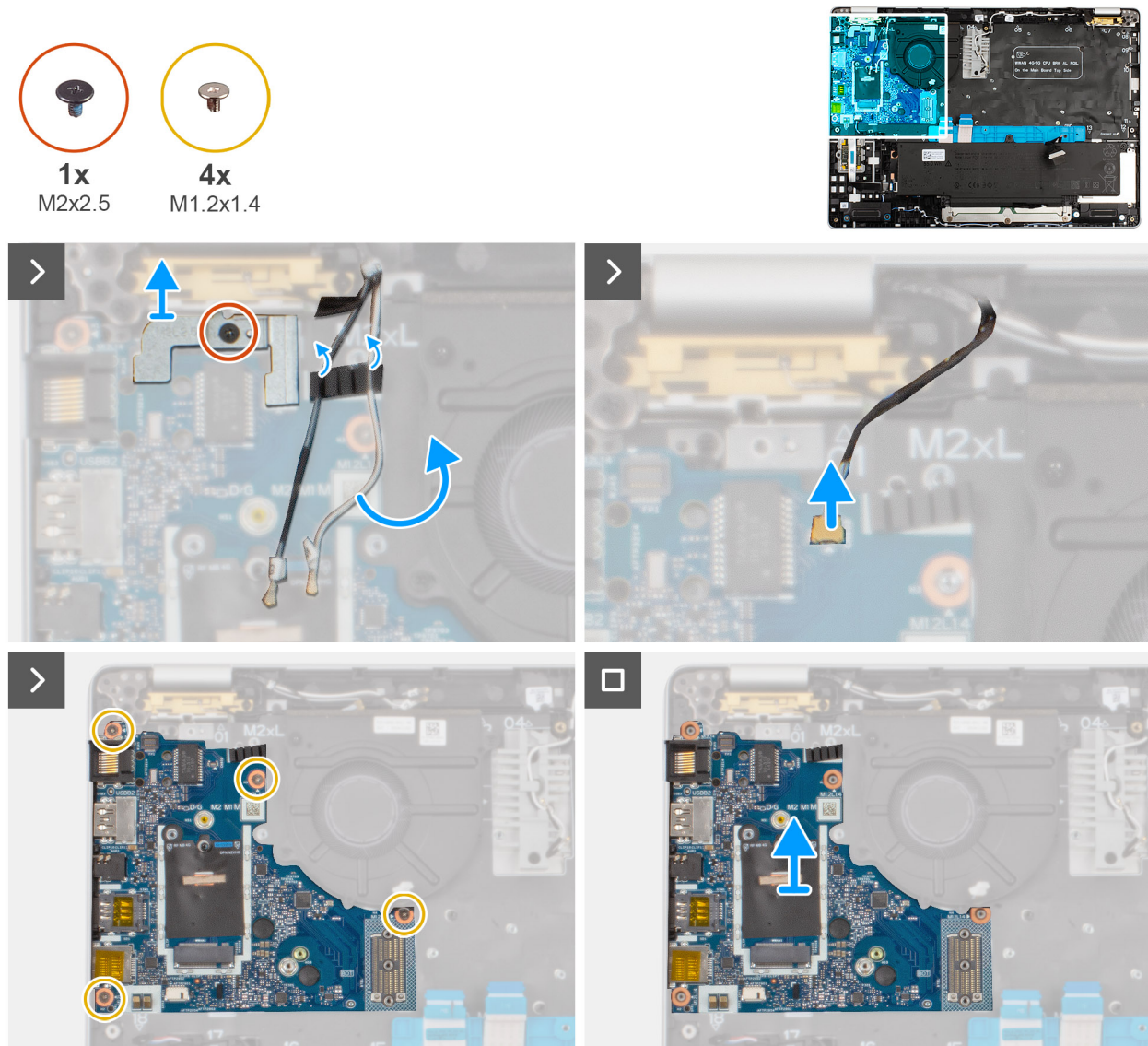
Abbildung 55. Entfernen der E/A-Platine
