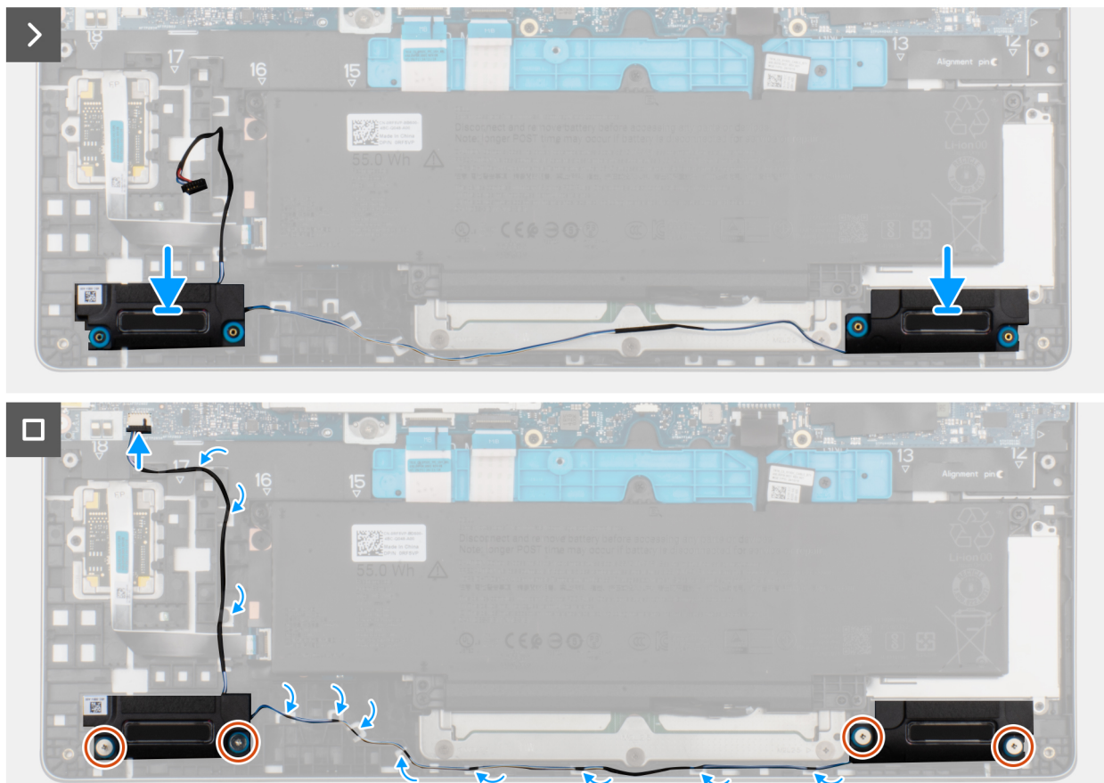
Abbildung 37. Installieren der Lautsprecher
