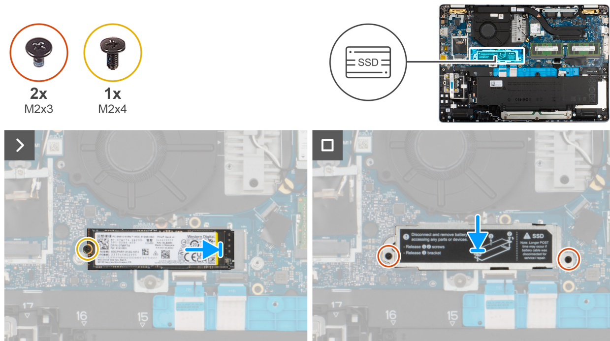
Abbildung 28. Einbauen der M.2230-SSD
