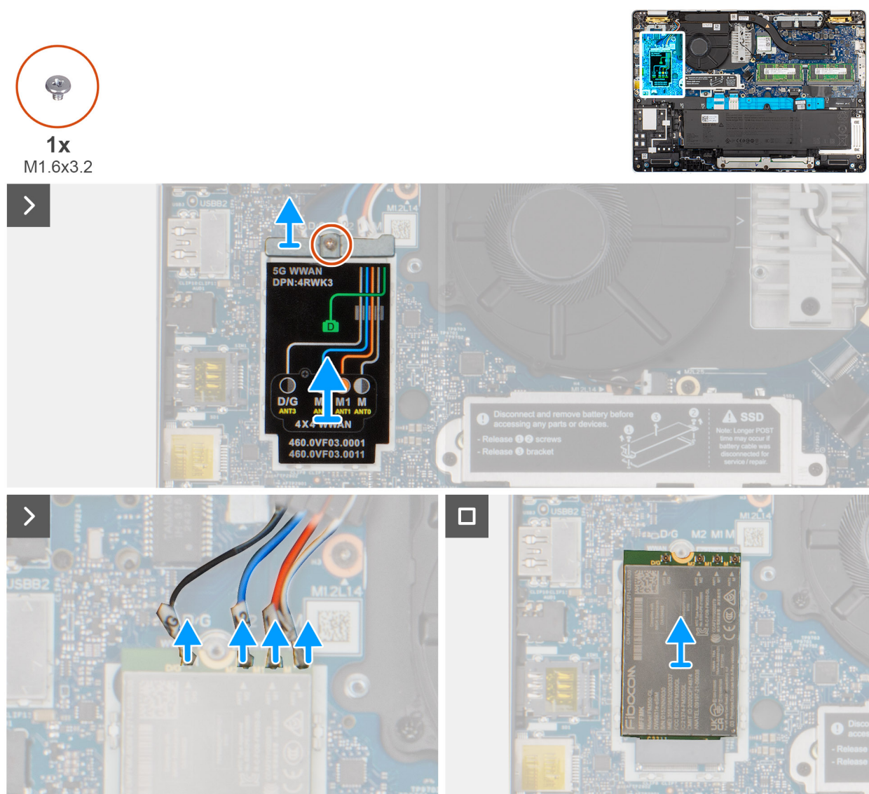
Abbildung 30. Entfernen der 5G-WWAN-Karte
