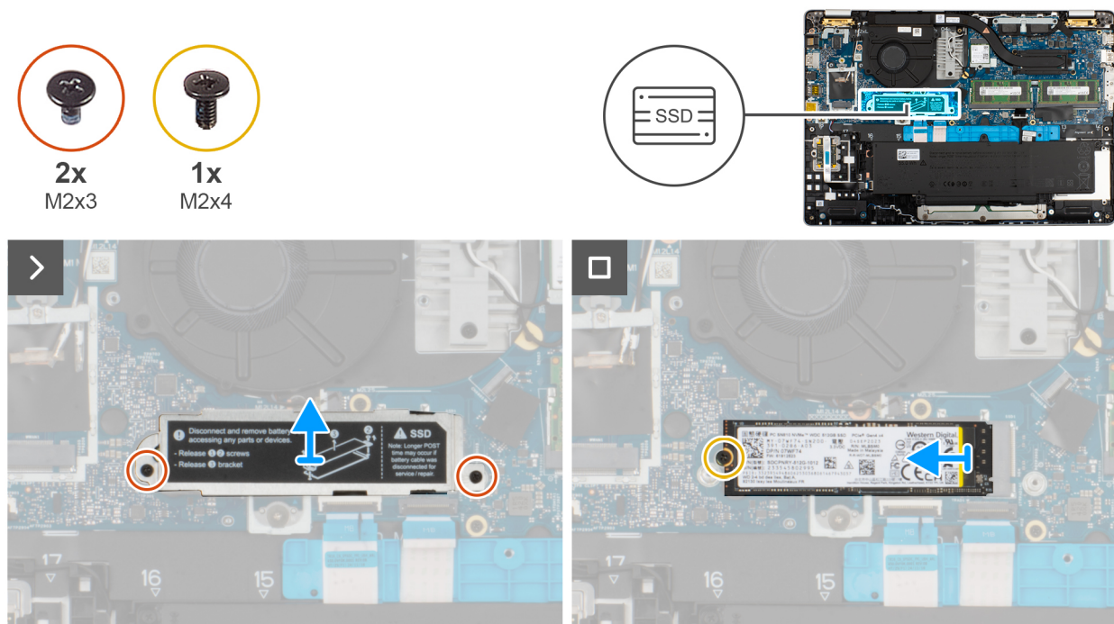
Abbildung 26. Entfernen des M.2-2280-SSD-Laufwerks
