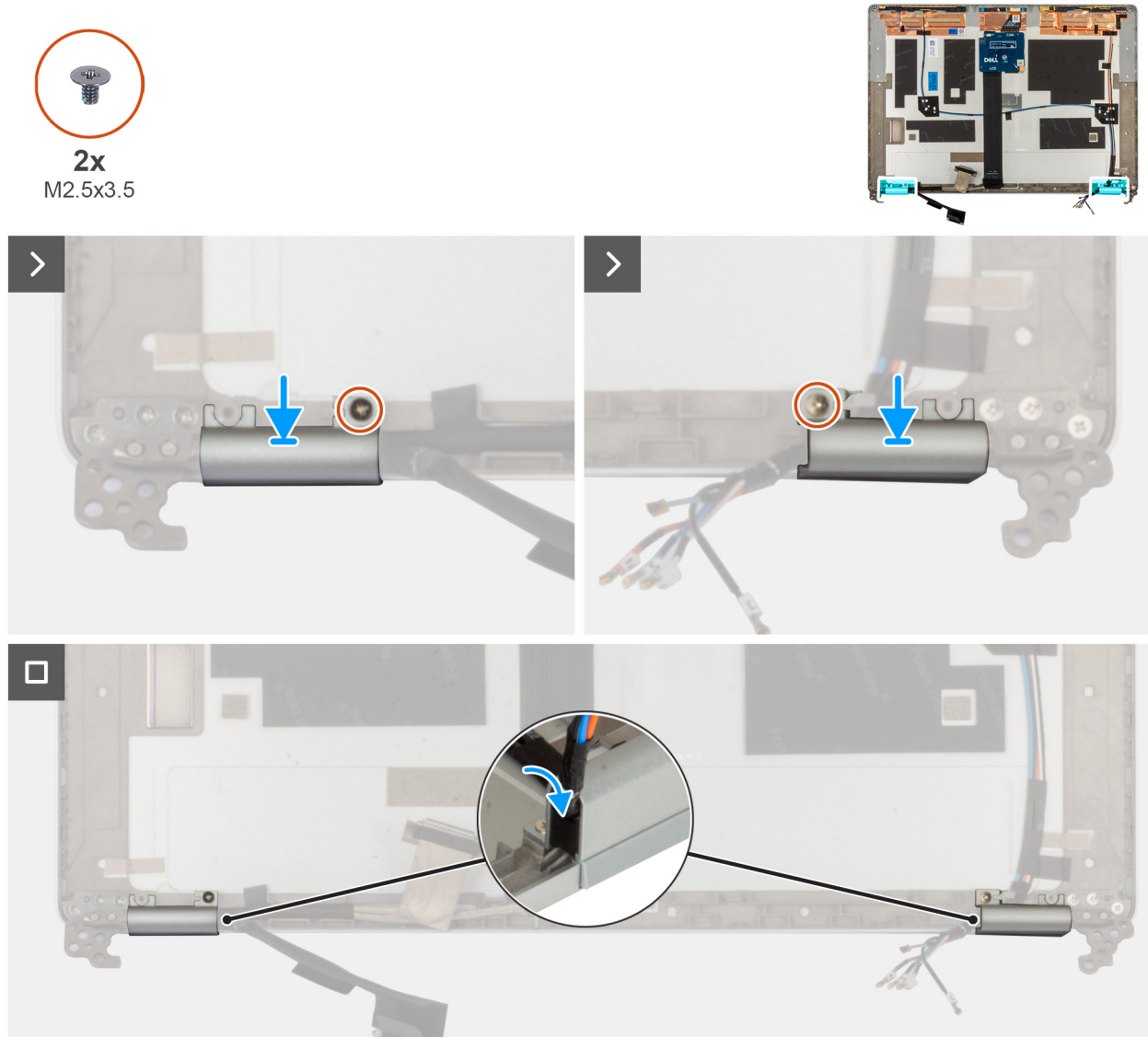
Abbildung 72. Einbauen der Bildschirmscharnierkappe
