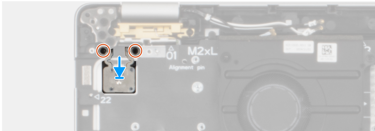
Abbildung 57. Installieren des Netzschalters mit optionalem Fingerabdruck-Lesegerät
