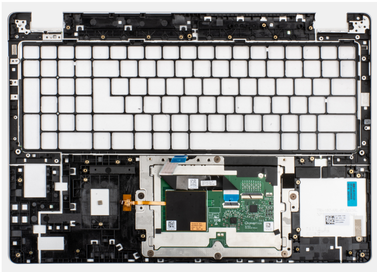
Abbildung 87. Entfernen der Handauflagenbaugruppe
