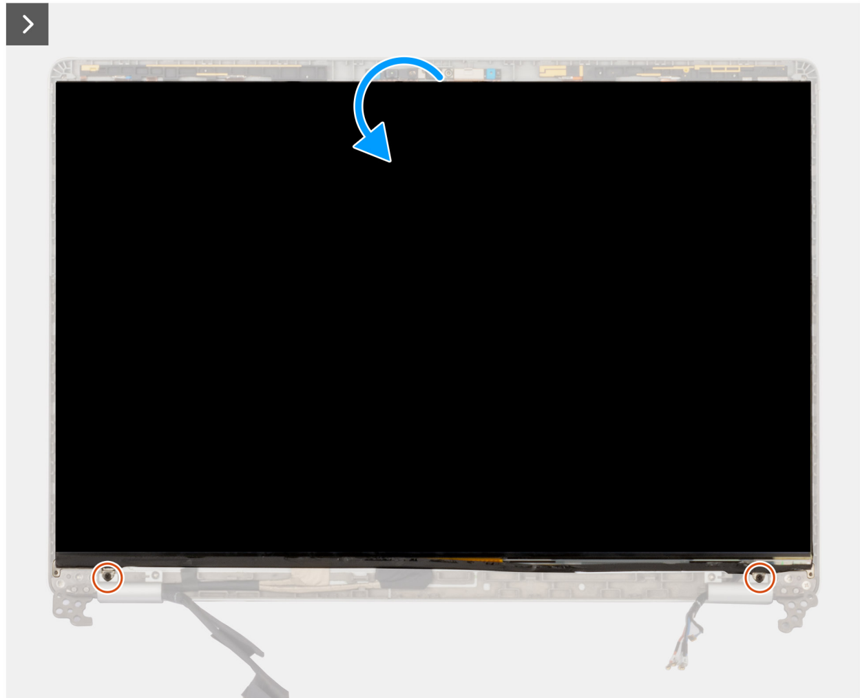
Abbildung 67. Entfernen des Bildschirms
