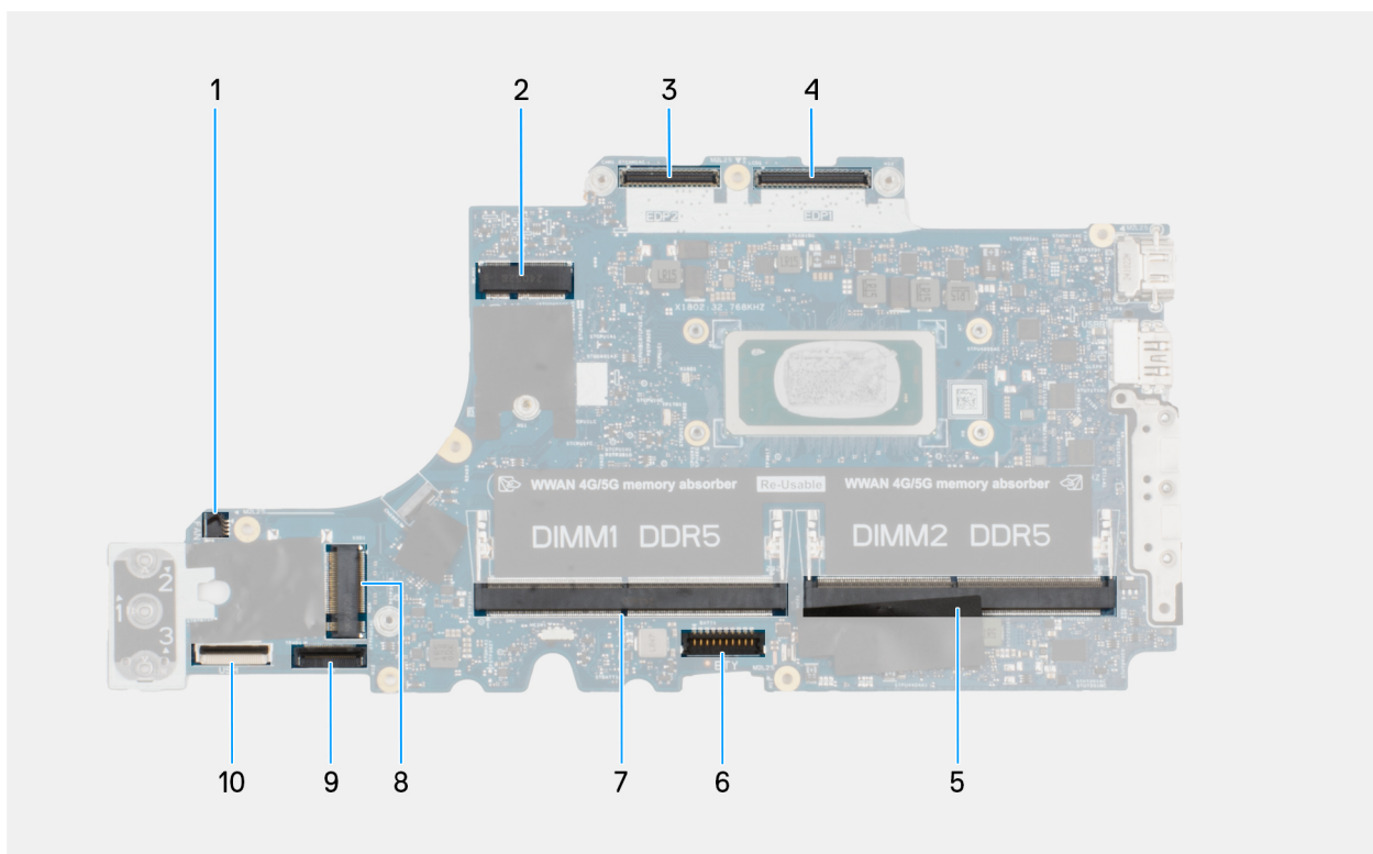
Abbildung 52. Hauptplattenanschluss
