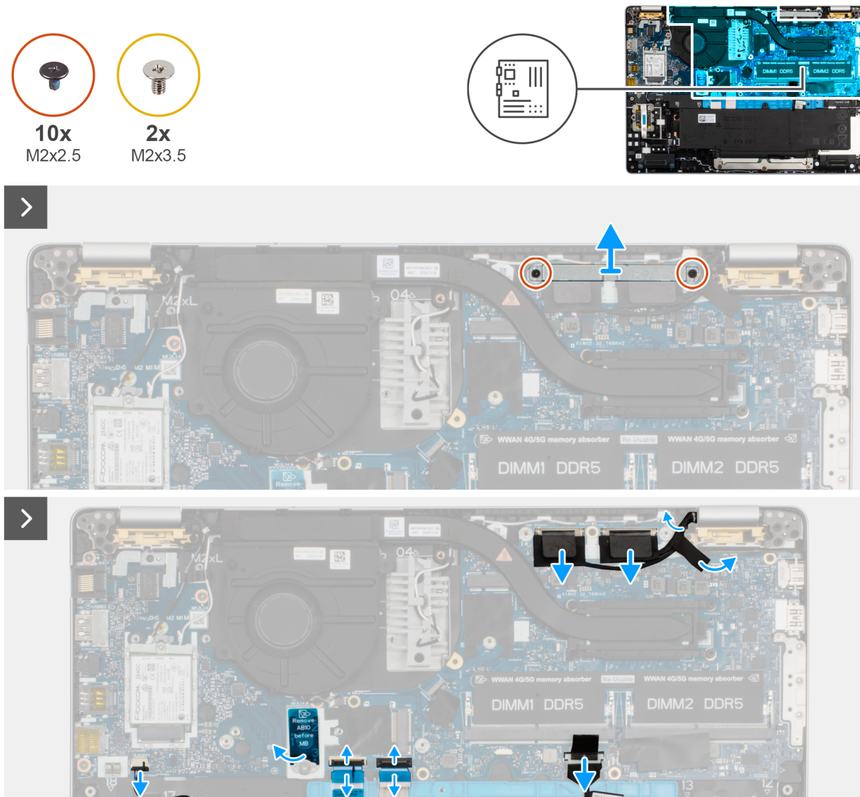
Abbildung 50. Entfernen der Hauptplatine
