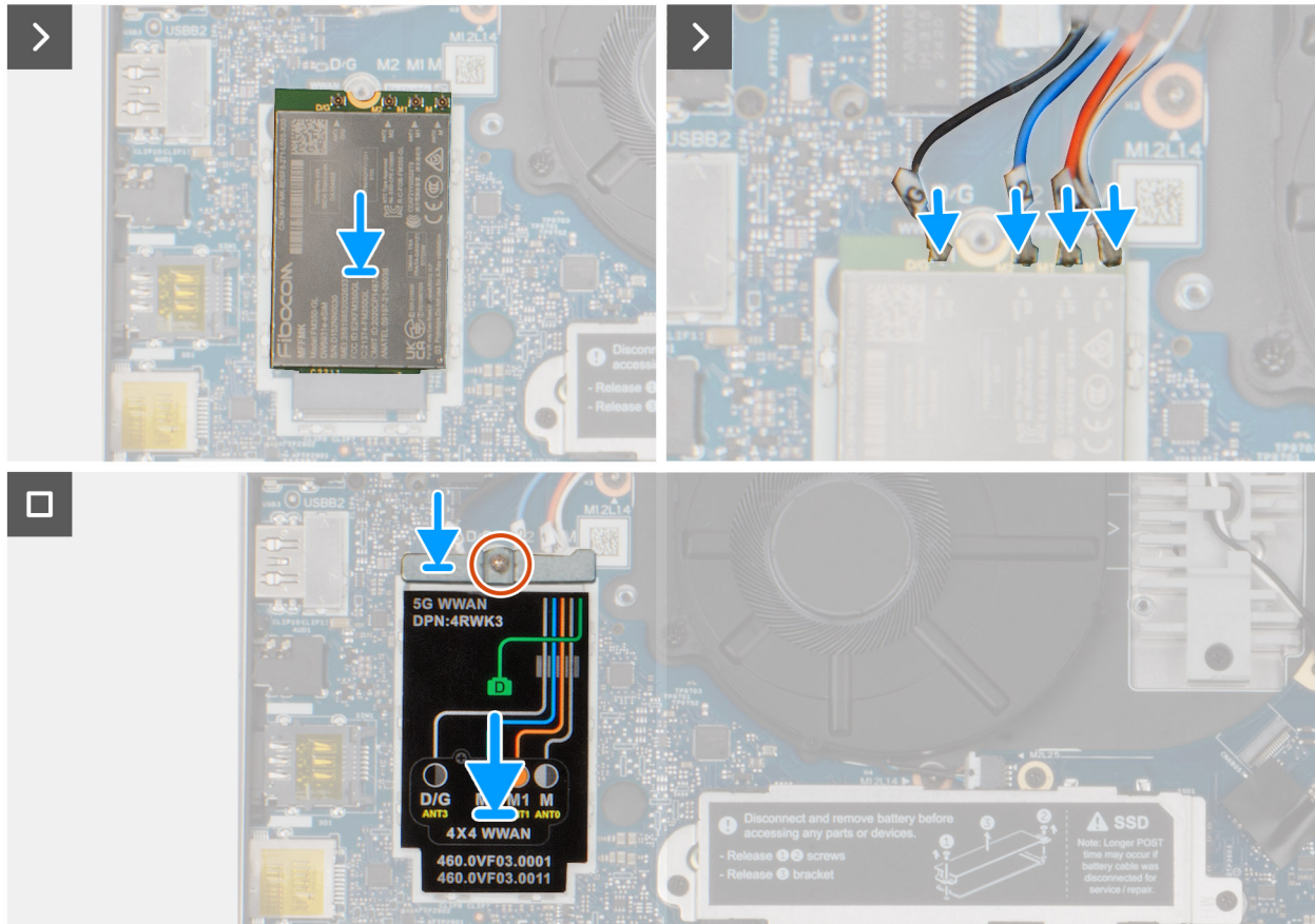
Abbildung 32. Einbauen der 5G-WWAN-Karte
