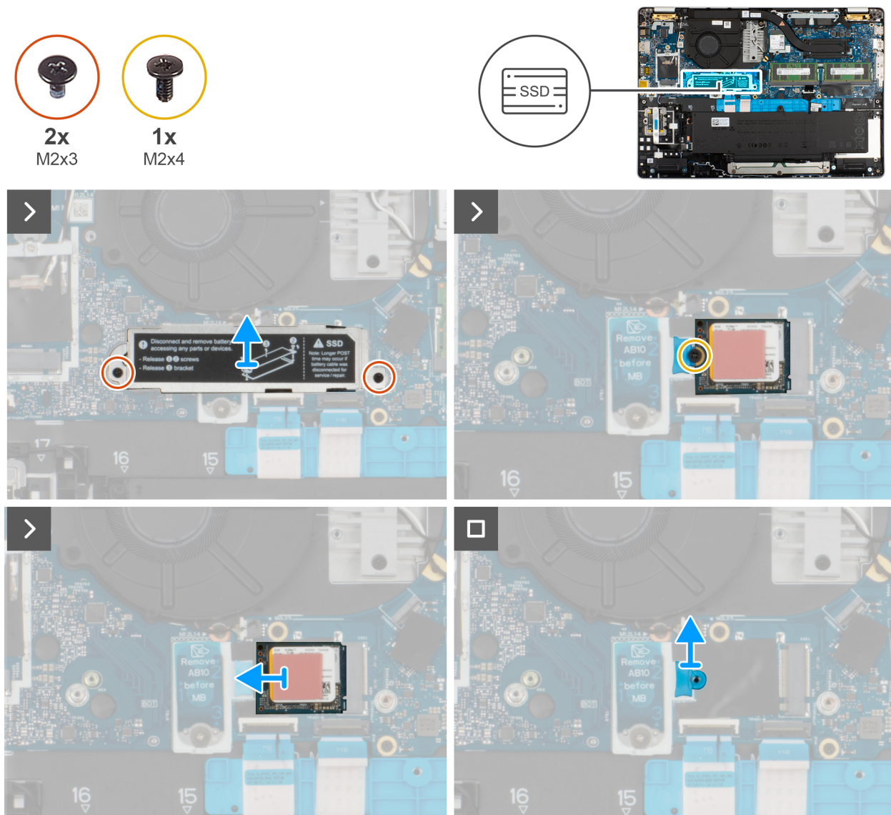
Abbildung 24. Entfernen des M.2-2230-Solid-State-Laufwerks
