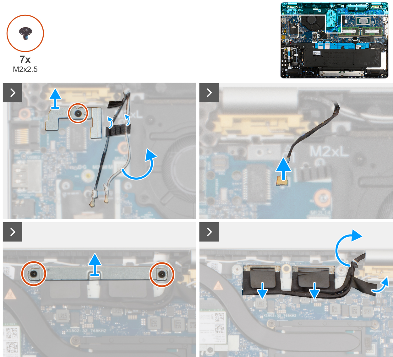
Abbildung 41. Entfernen der WLAN-Antenne
