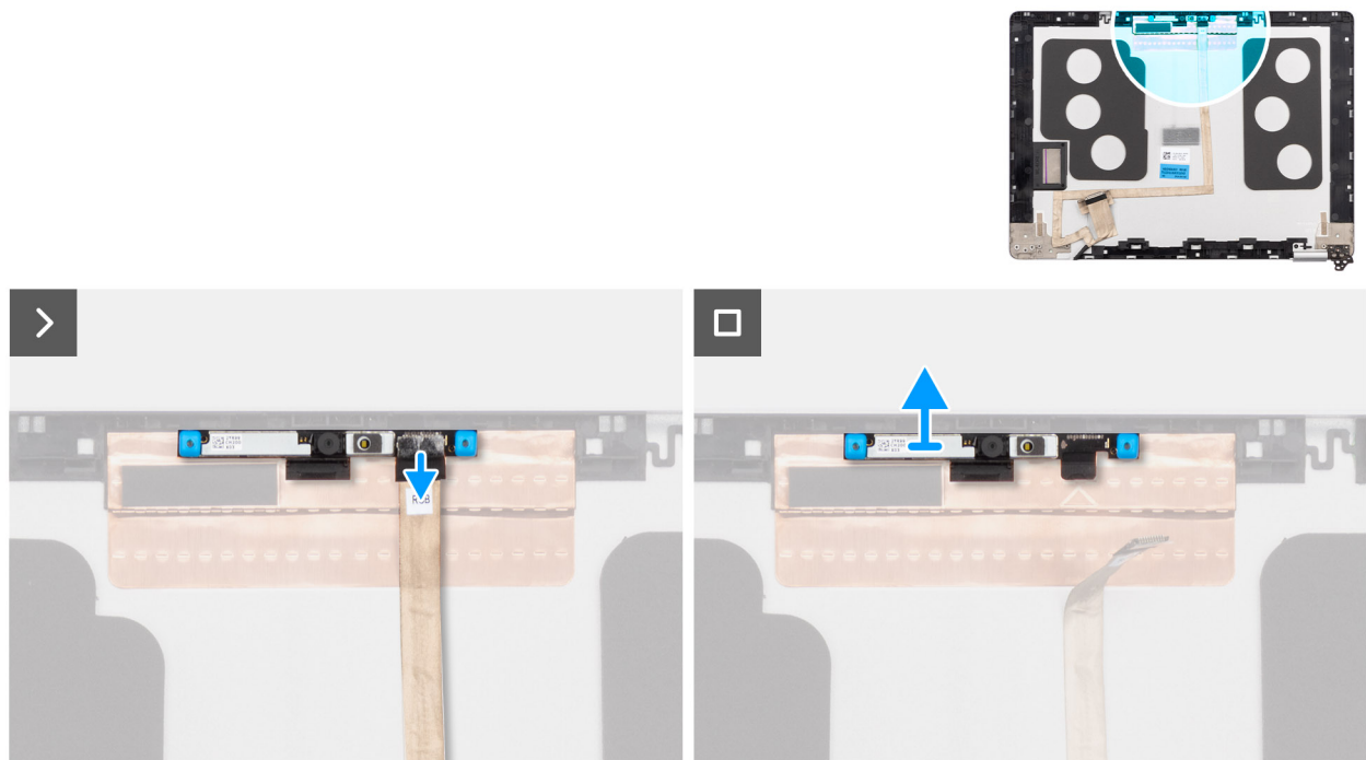
Abbildung 75. Entfernen des Kameramoduls
