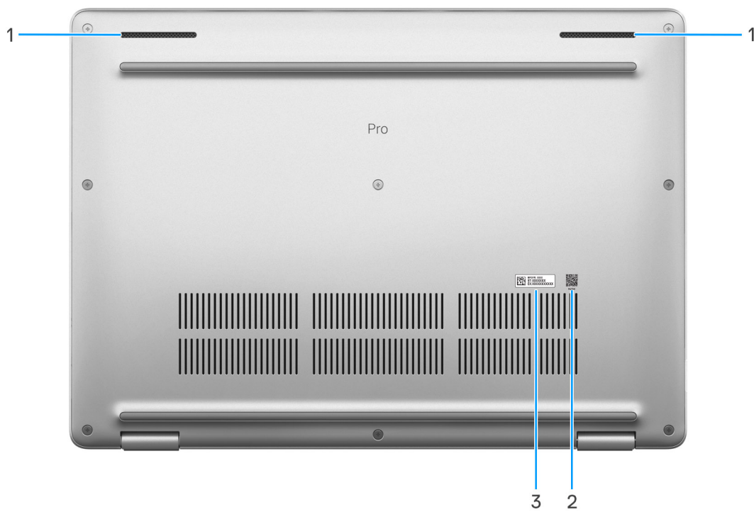
Abbildung 5. Untere Ansicht
