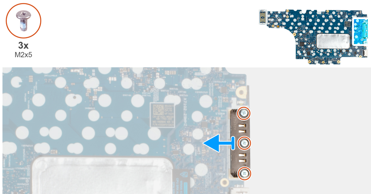
Abbildung 79. Entfernen des USB Type-C-Anschlussmoduls
