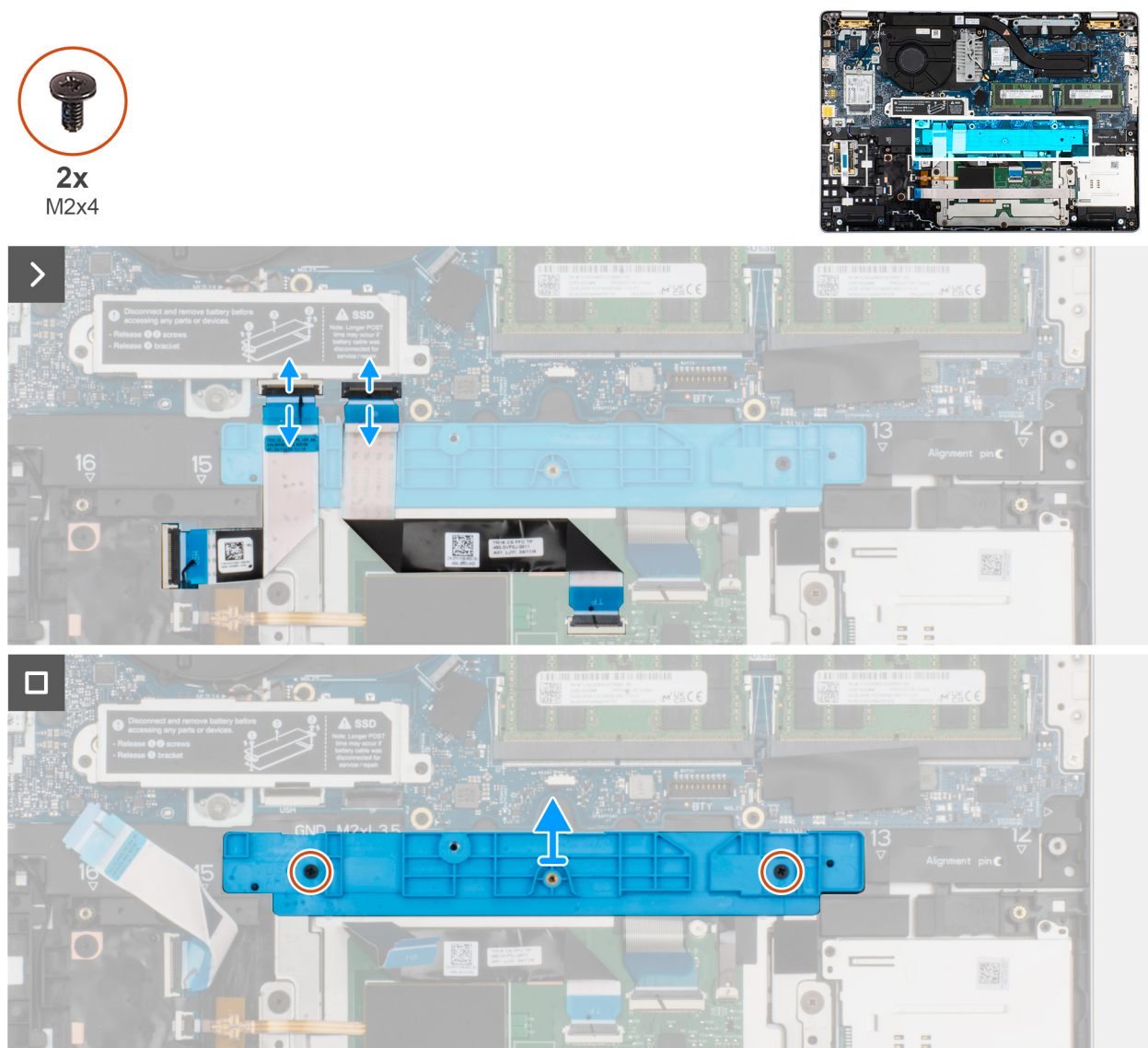
Abbildung 45. Entfernen der Akkuhalterung
