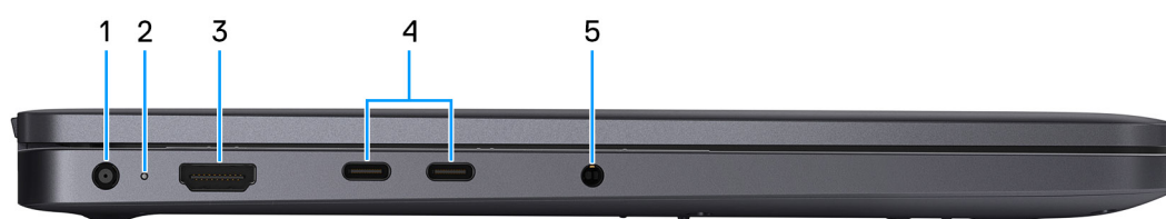
Abbildung 2. Linke Seitenansicht
