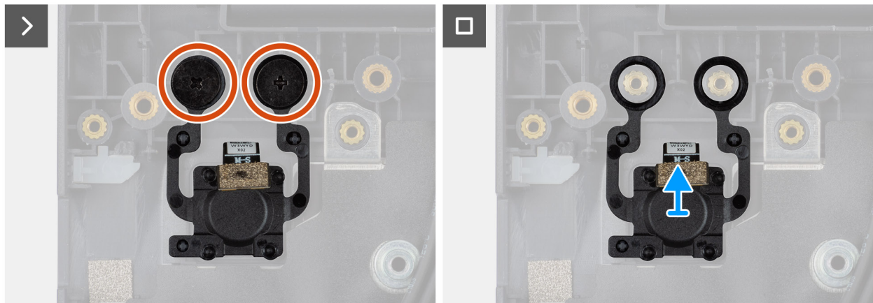
Abbildung 40. Entfernen des Netzschalters mit Fingerabdruck-Lesegerät
