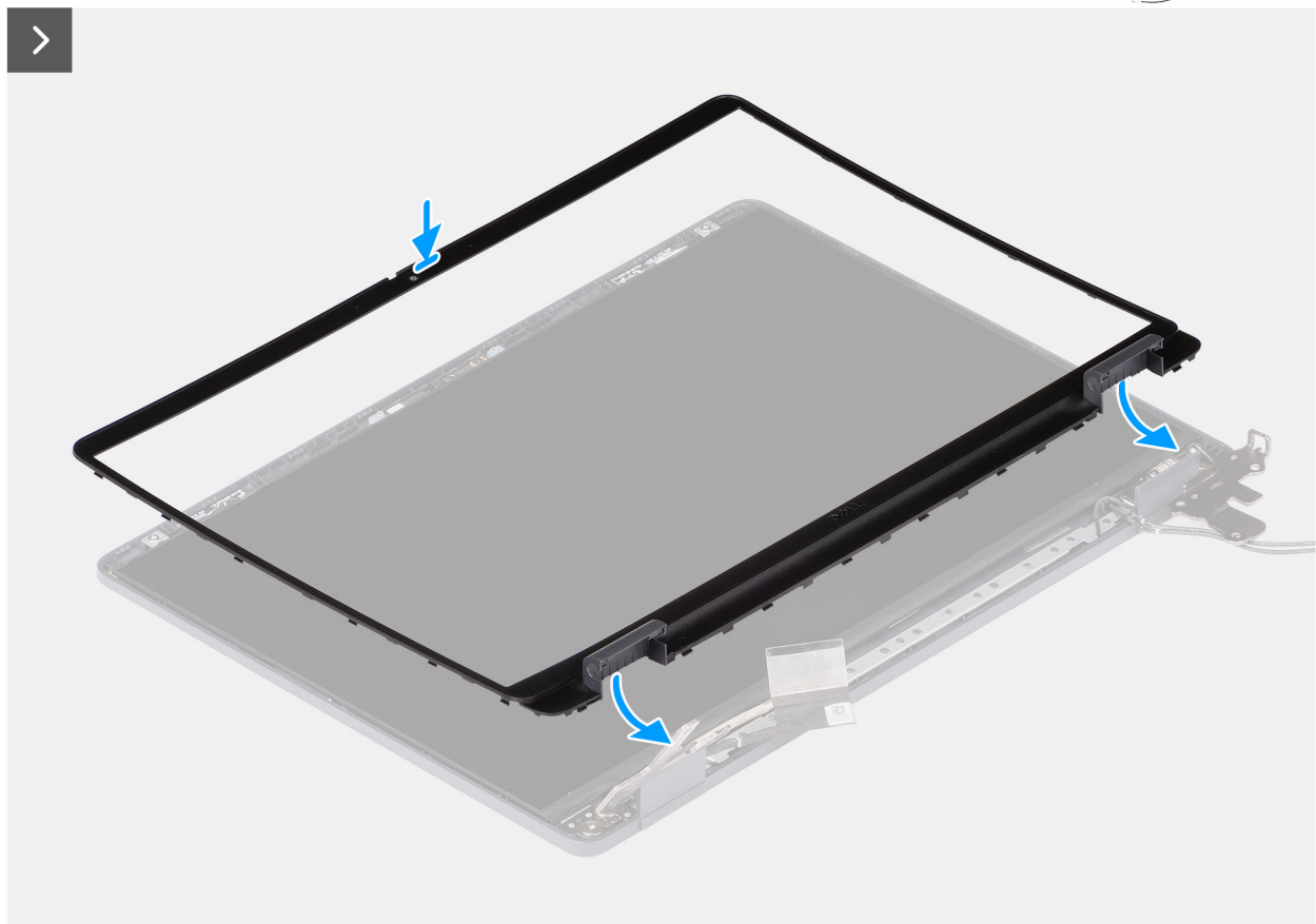
Abbildung 72. Einbauen der Bildschirmblende
