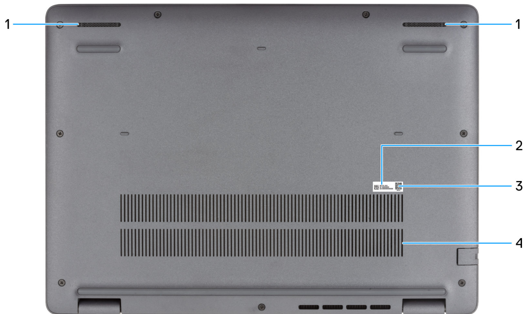
Abbildung 5. Untere Ansicht
