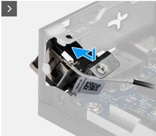
Figure 69. Installation du module d'antenne (câble blanc)
