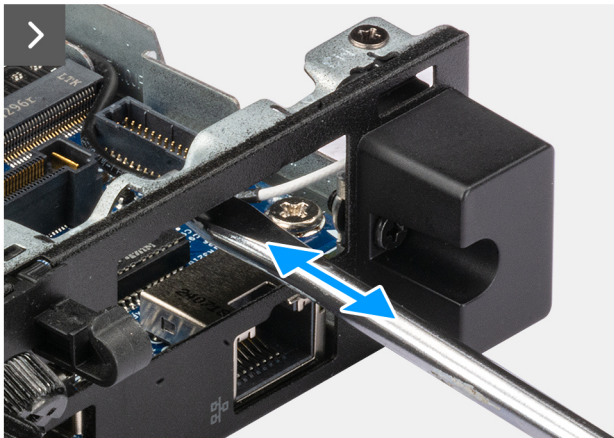
Figure 43. Installation du module de port USB-C
