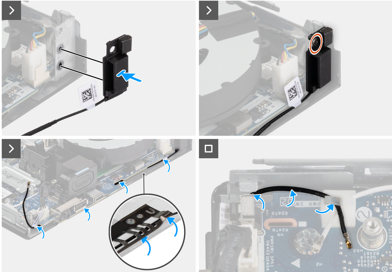
Figure 66. Installation du module d'antenne (câble noir)
