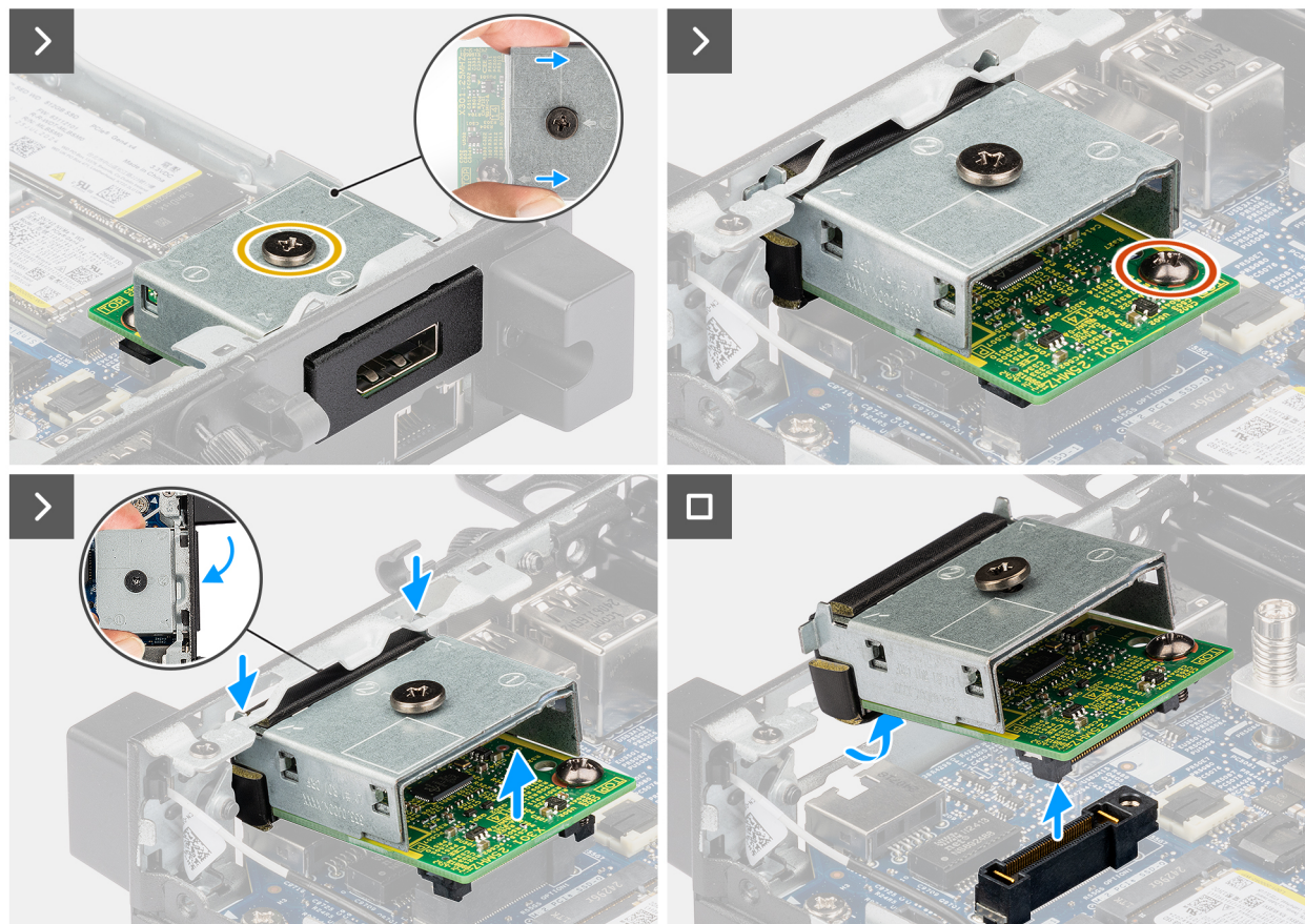
Figure 45. Retrait du module DisplayPort
