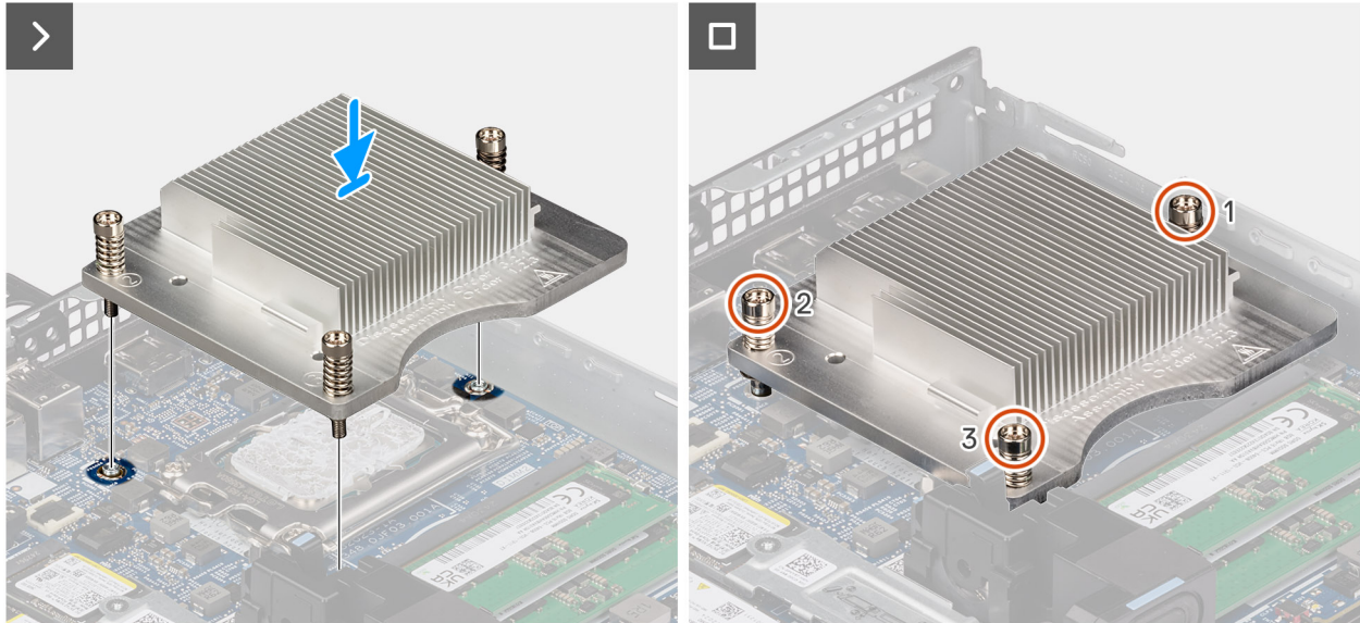
Figure 64. Installation du dissipateur de chaleur
