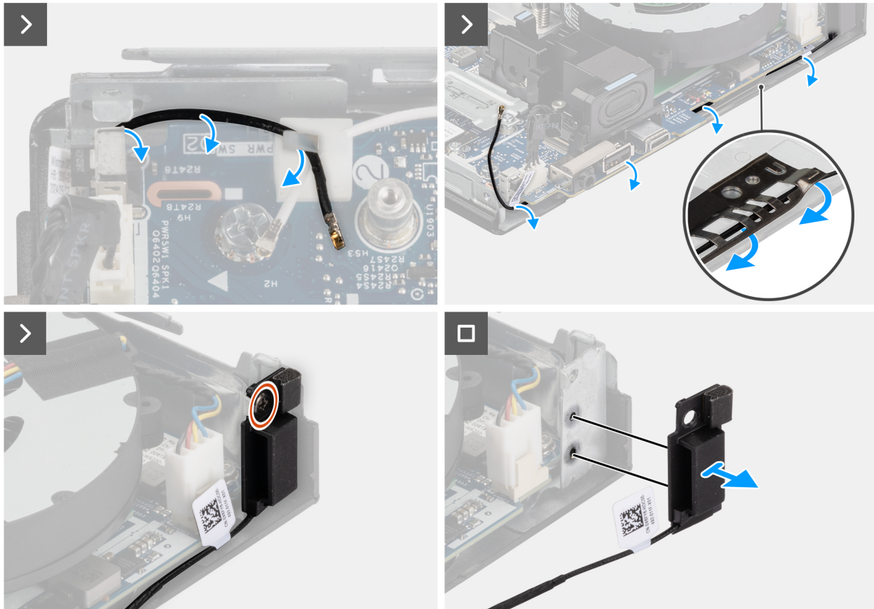
Figure 65. Retrait du module d'antenne (câble noir)
