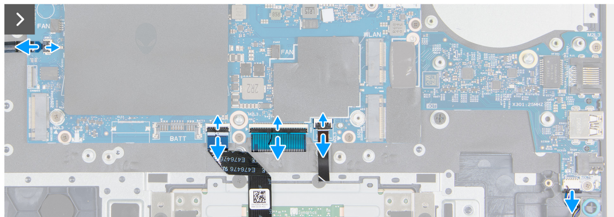
Rysunek 51. Wymontowywanie płyty głównej
