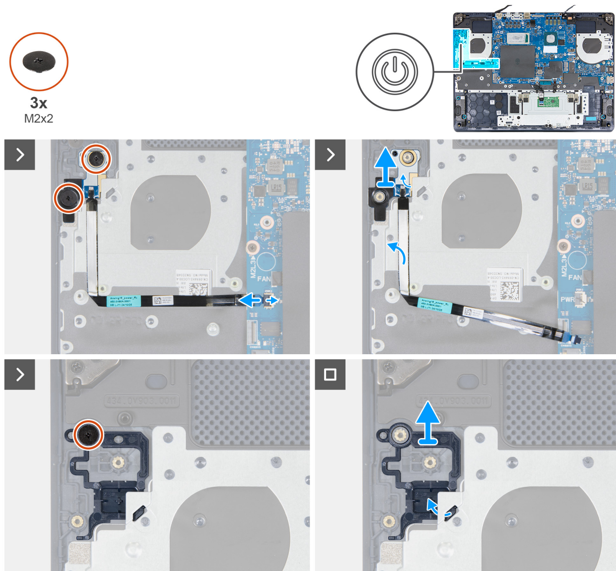
Rysunek 48. Wymontowywanie przycisku zasilania i płyty przycisku zasilania
