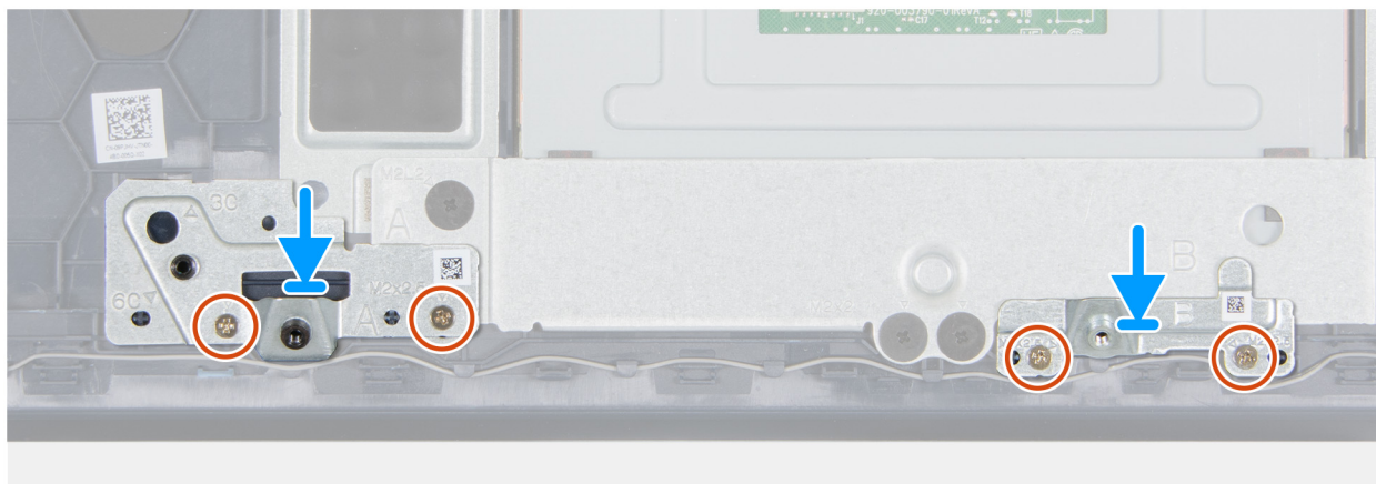
Rysunek 45. Instalacja klamer baterii 6-ogniowej
