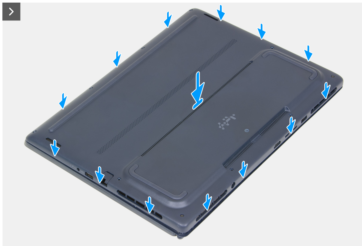
Rysunek 16. Instalowanie pokrywy dolnej
