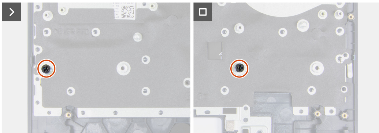
Rysunek 72. Wkręcanie uchwytów na śruby dysku SSD
