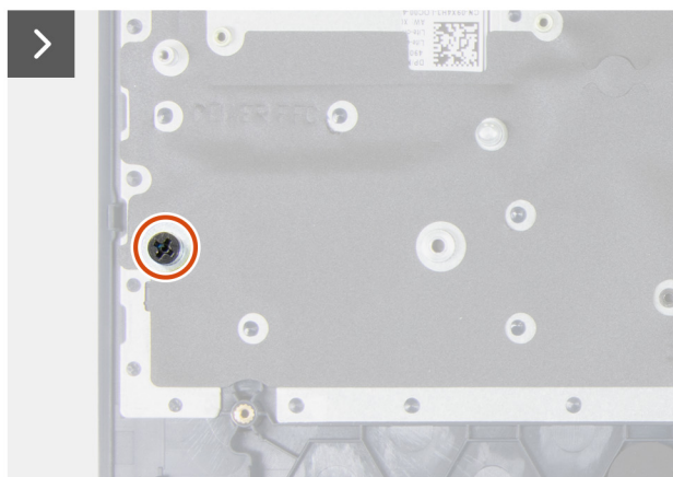
Rysunek 71. Wymontowywanie uchwytych na śruby dysku SSD
