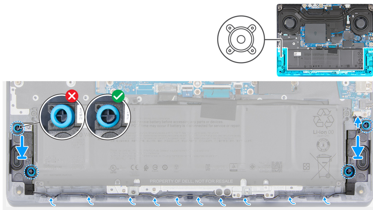
Rysunek 35. Instalowanie głośników
