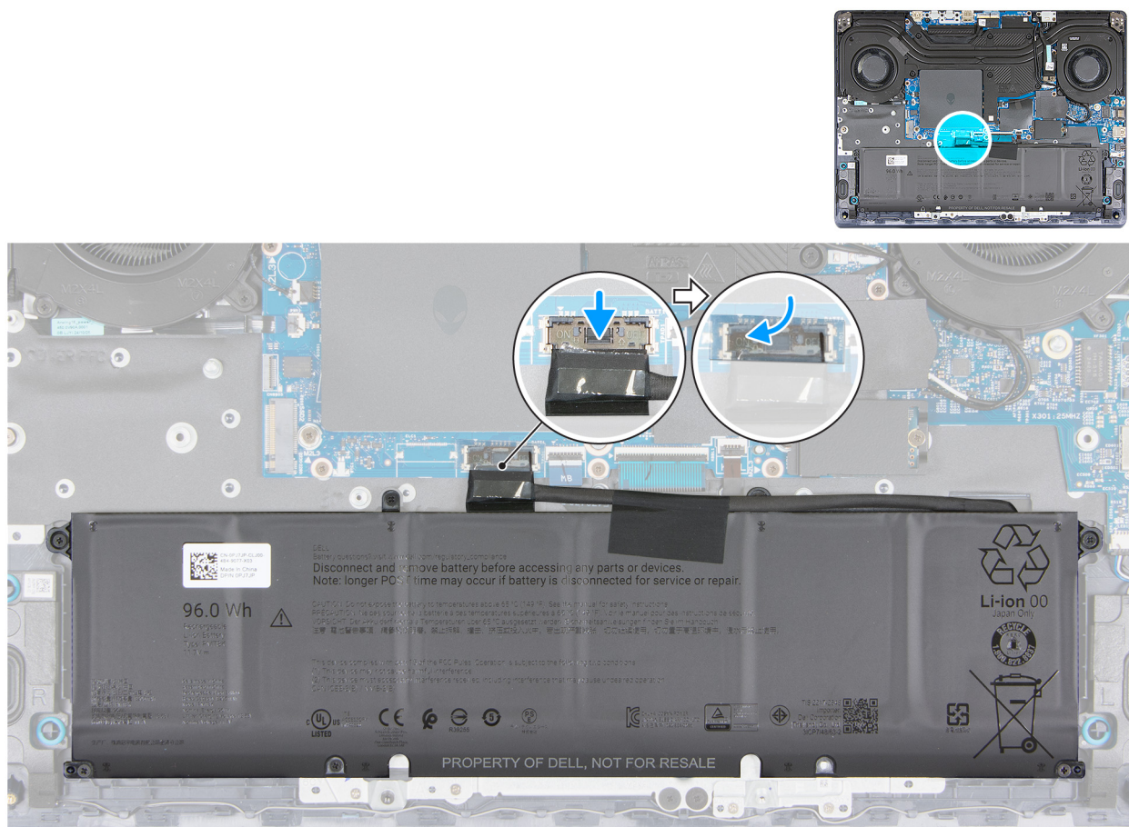
Rysunek 15. Podłączanie kabla baterii
