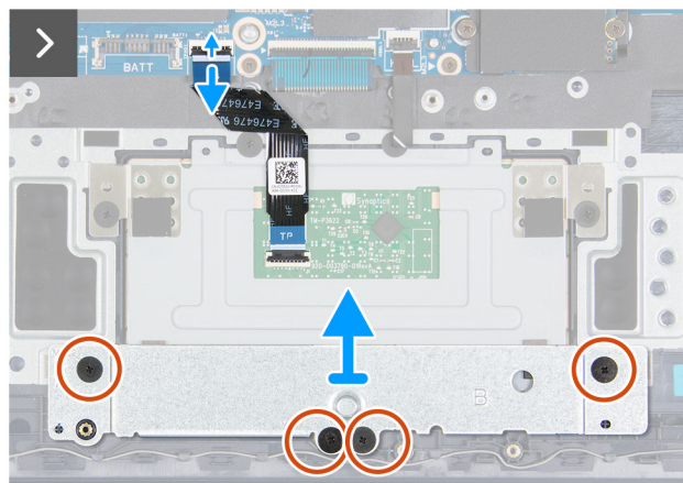
Rysunek 46. Wymontowywanie touchpada
