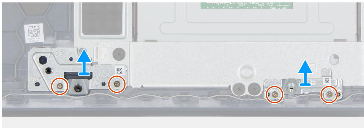
Rysunek 44. Wymontowywanie klamer baterii 6-ogniowej
