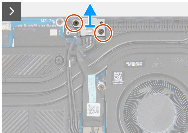
Rysunek 36. Wymontowywanie gniazda zasilacza
