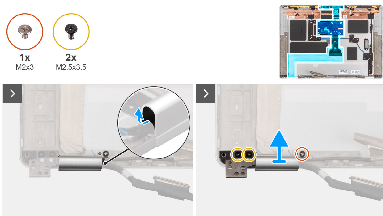
Figura 84. Rimozione del cavo del display
