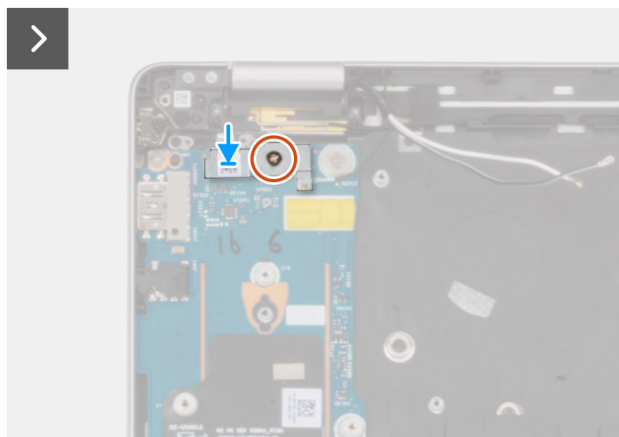
Figura 61. Installazione della scheda di I/O
