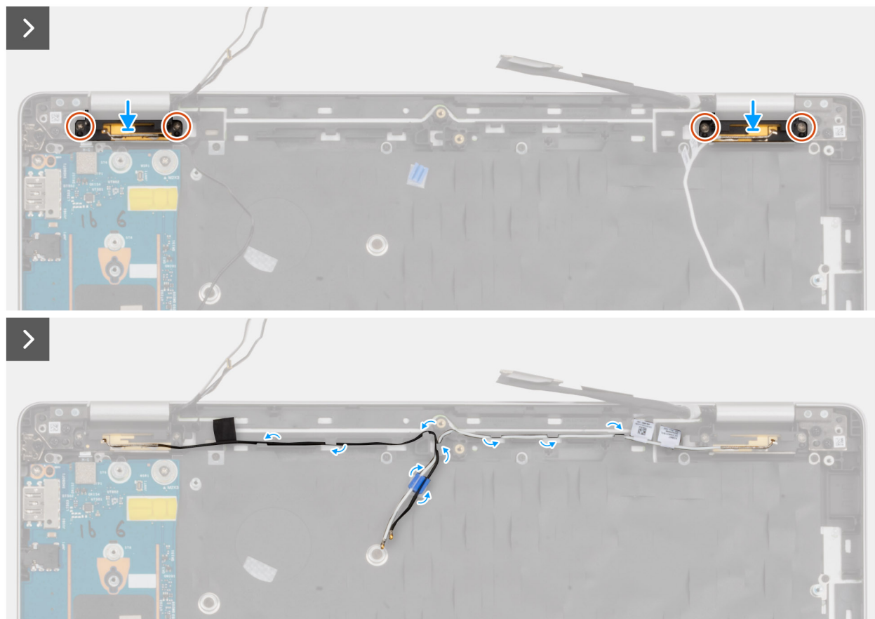
Figura 56. Installazione del modulo dell'antenna WLAN
