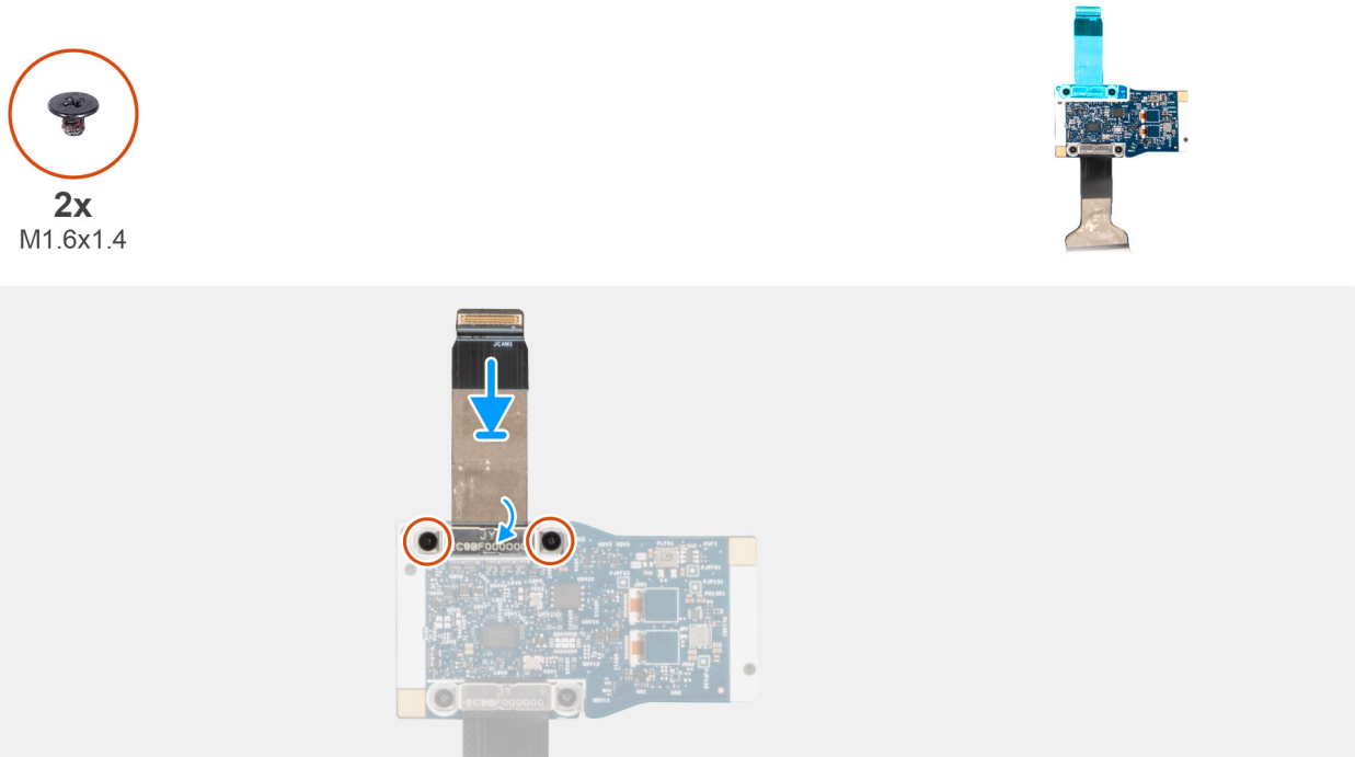
Figura 93. Installazione del cavo della scheda centrale
