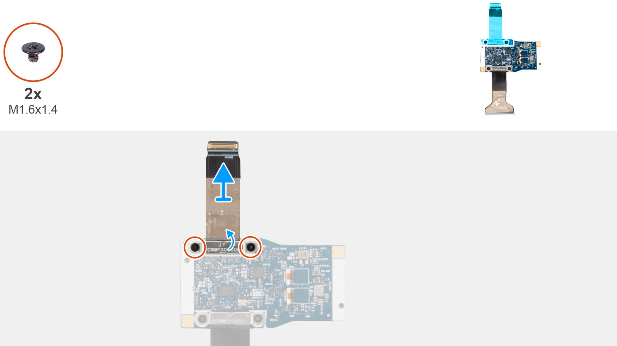
Figura 92. Rimozione del cavo della scheda centrale
