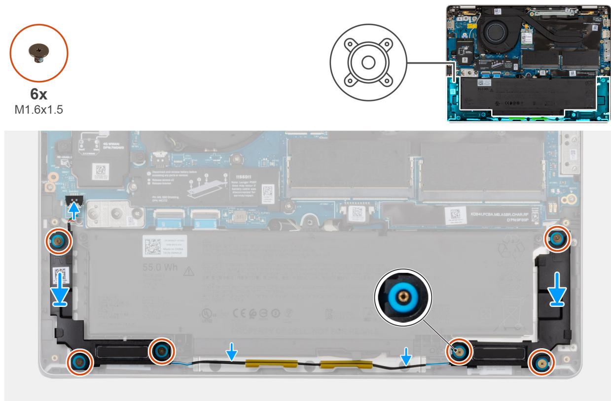
Figura 43. Installazione degli altoparlanti
