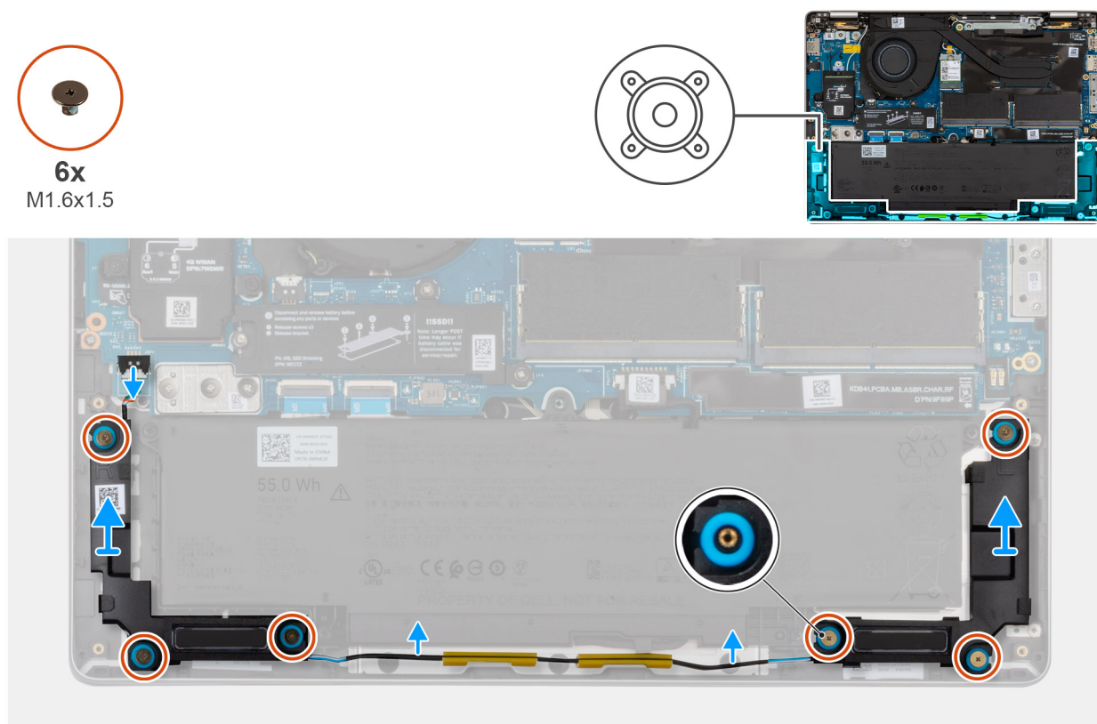
Figura 42. Rimozione degli altoparlanti
