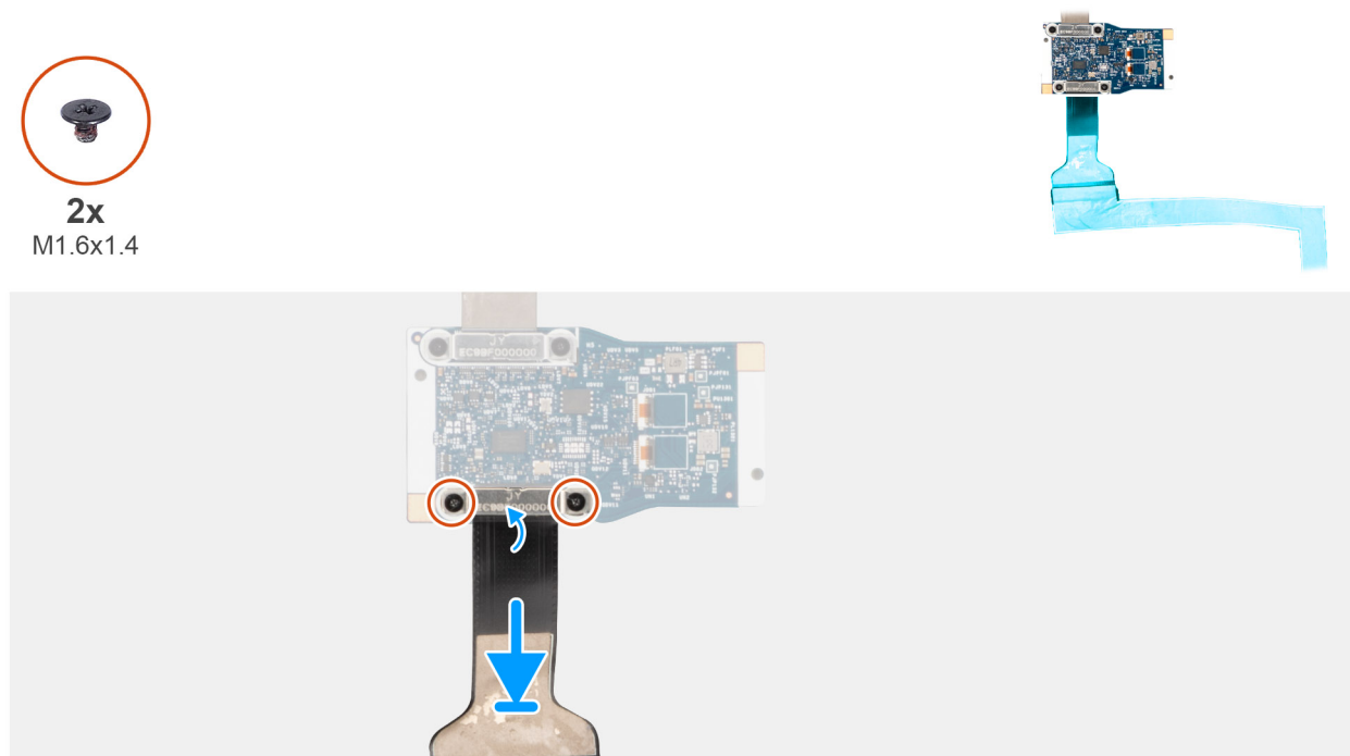
Figura 91. Installazione del cavo del display per fotocamera MIPI
