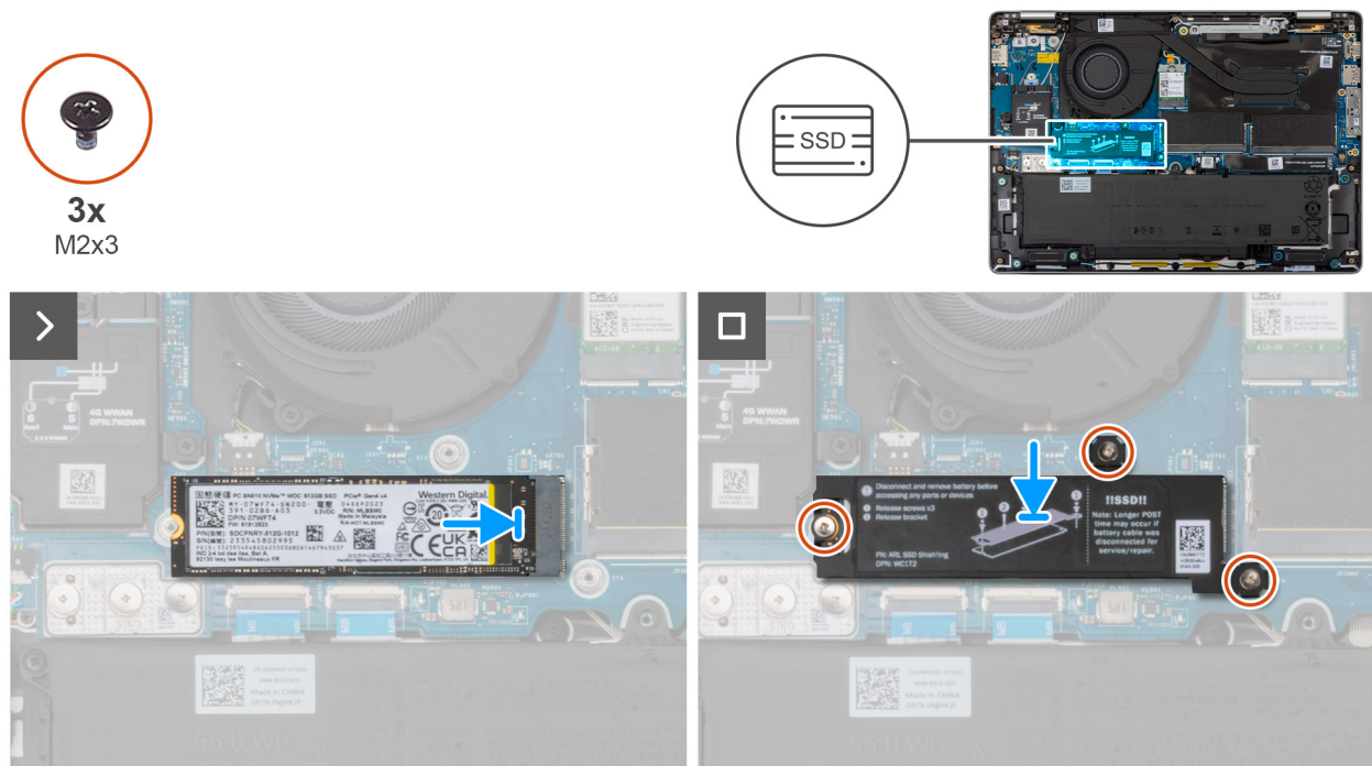
Figura 39. Installazione dell'SSD M.2 2280
