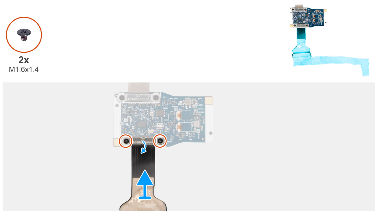
Figura 90. Rimozione del cavo del display per fotocamera MIPI
