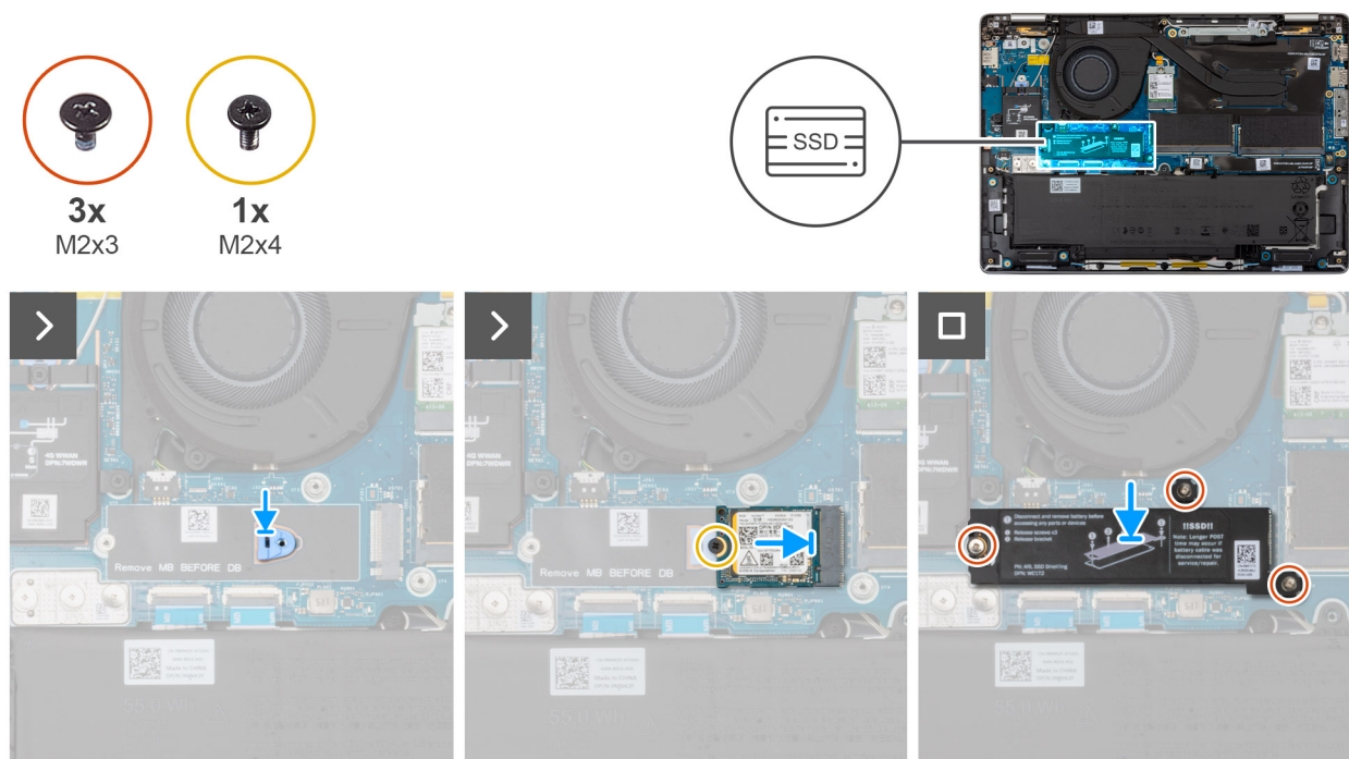
Figura 37. Installazione dell'SSD M.2 2230
