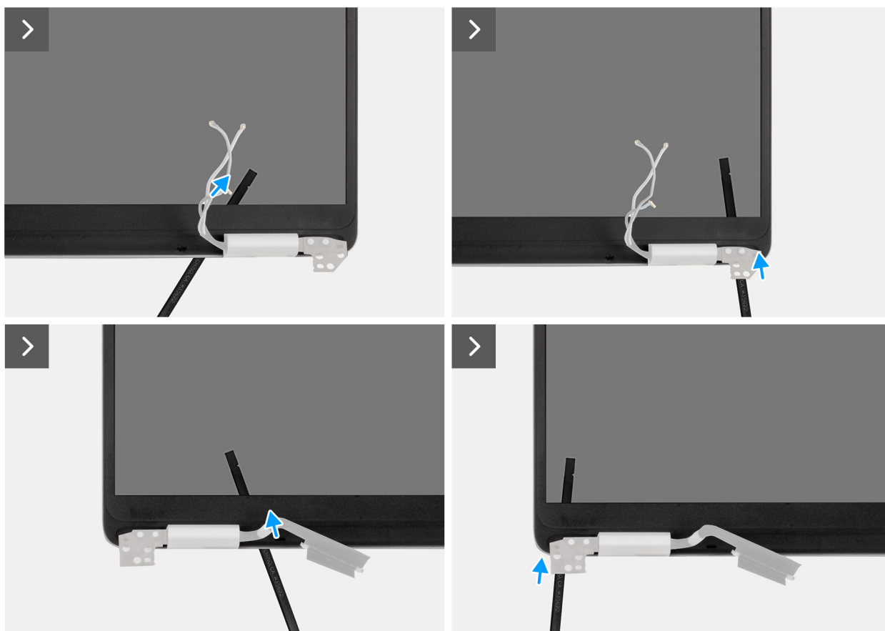
Figura 70. Rimozione della cornice del display
