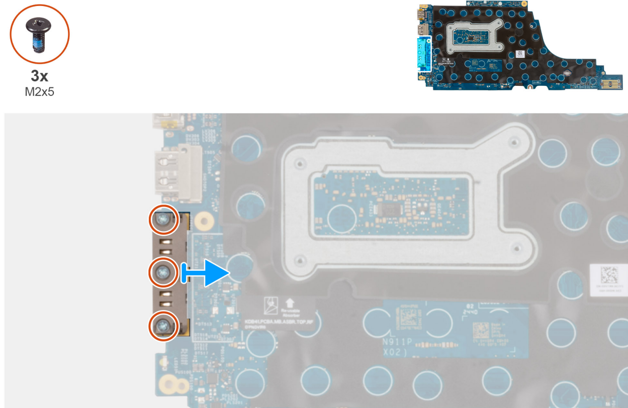
Figura 58. Rimozione del modulo del connettore USB Type-C
