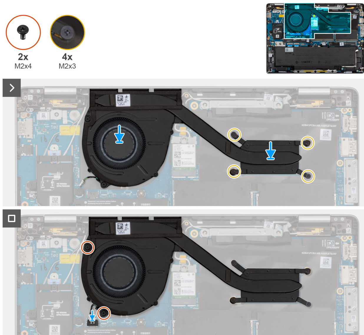
Figura 45. Installazione del gruppo ventola e dissipatore di calore
