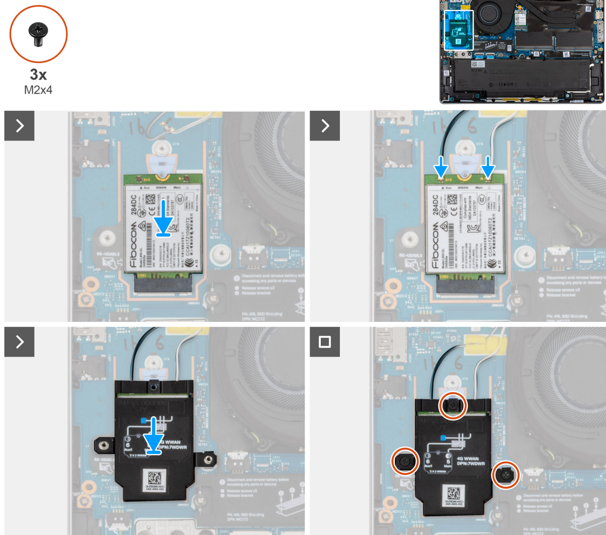
Figura 35. Installazione della scheda WWAN
