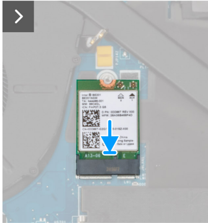
Figura 41. Installazione della scheda WLAN
