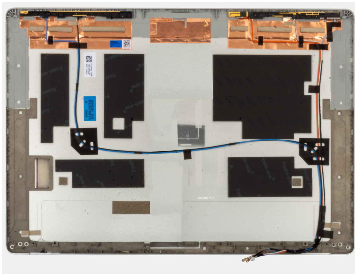
Figur 77. Ta bort bildskärmens baksida
