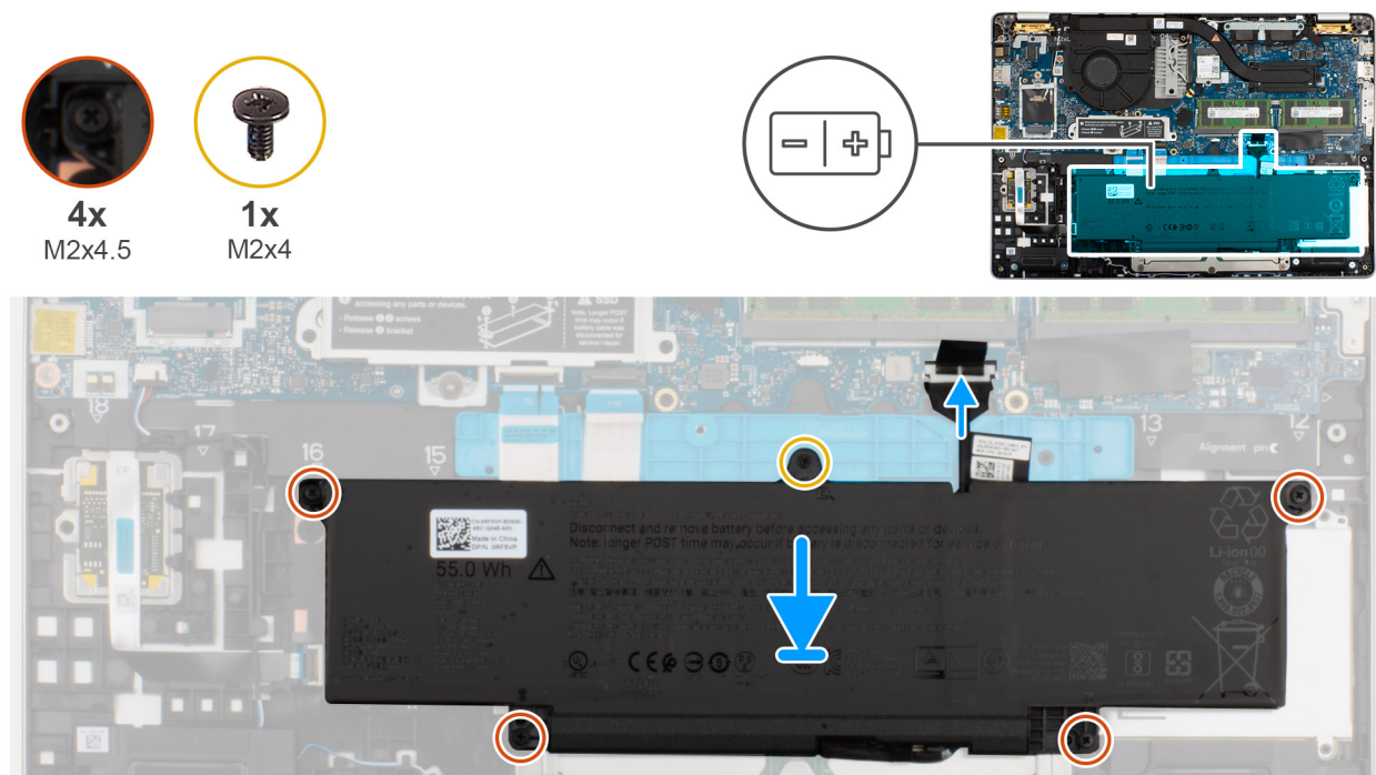
Figur 19. Installera batteriet
