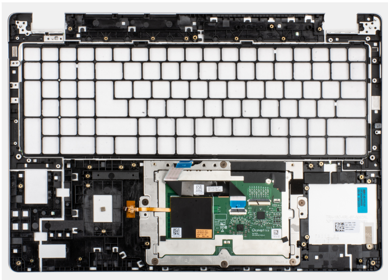
Figur 87. Ta bort handledsstödet
