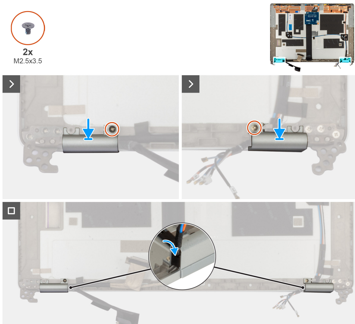
Figur 72. Installera locket för bildskärmsgångjärnen
