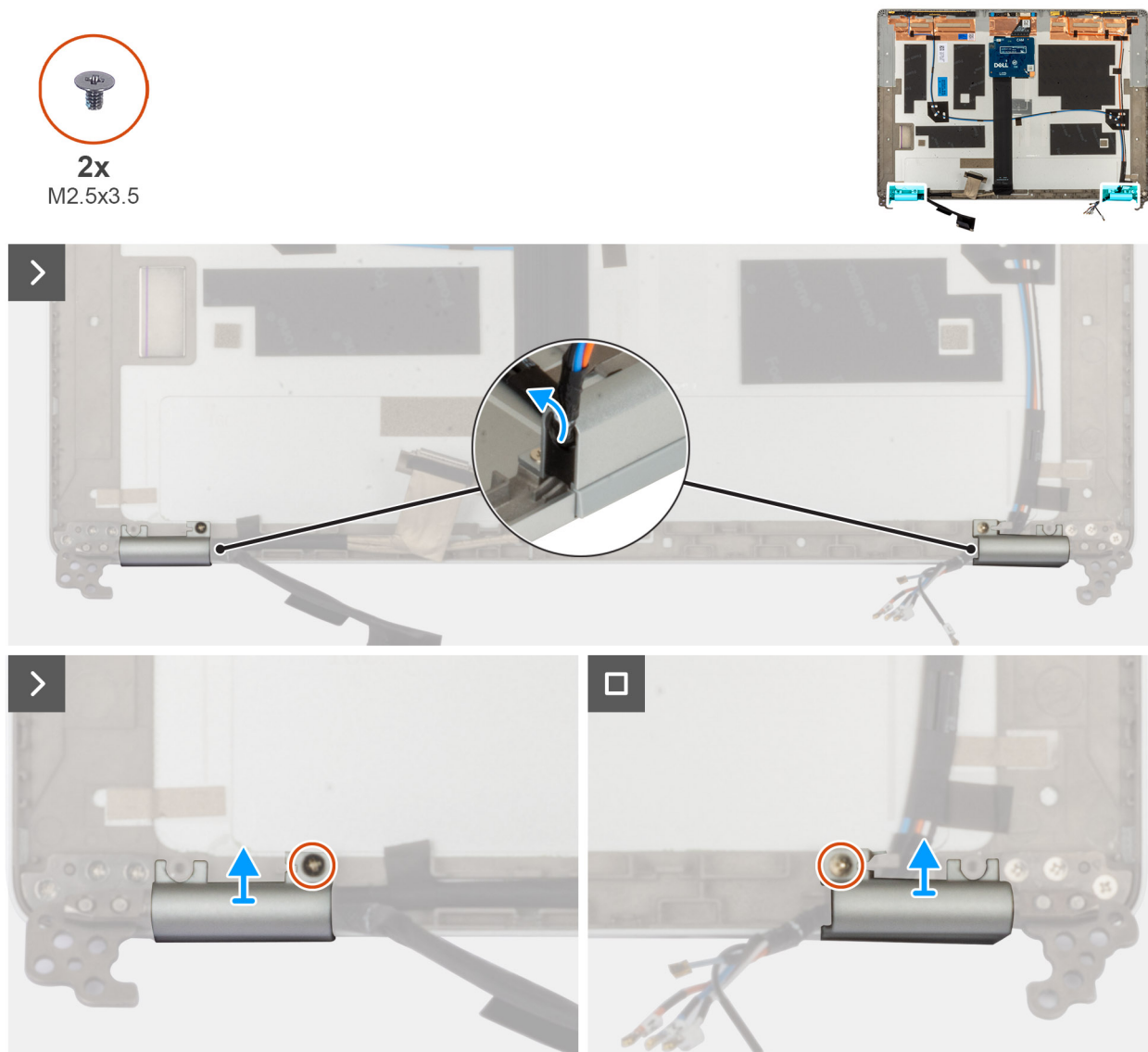
Figur 71. Ta bort locket för bildskärmsgångjärnen
