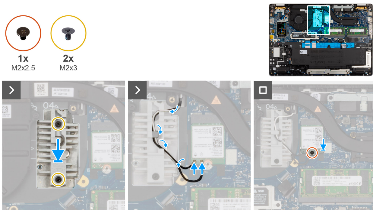
Figur 85. Installera tangentbordsutfyllnaden
