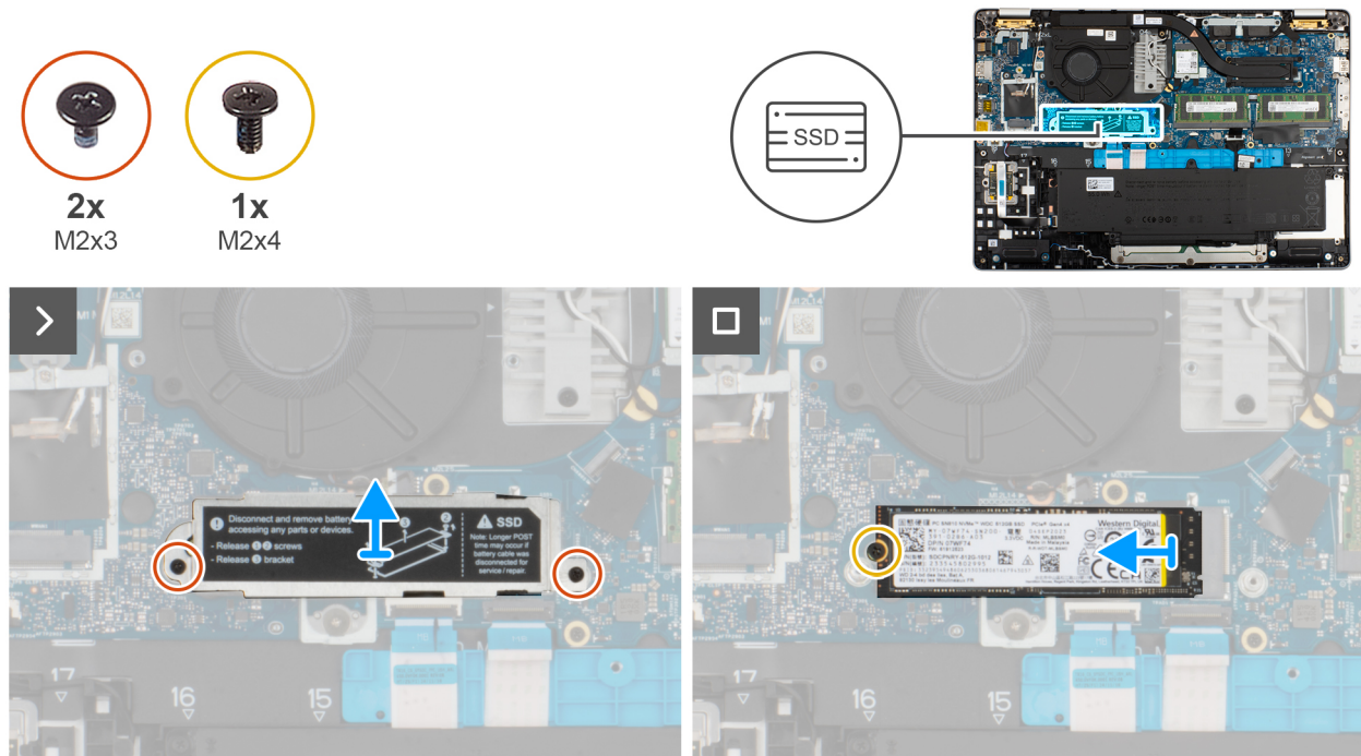
Figur 26. Ta bort M.2 2280 SSD
