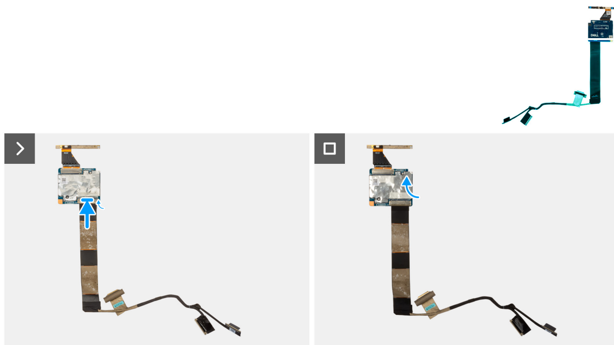
Figur 74. Installera bildskärmskabeln
