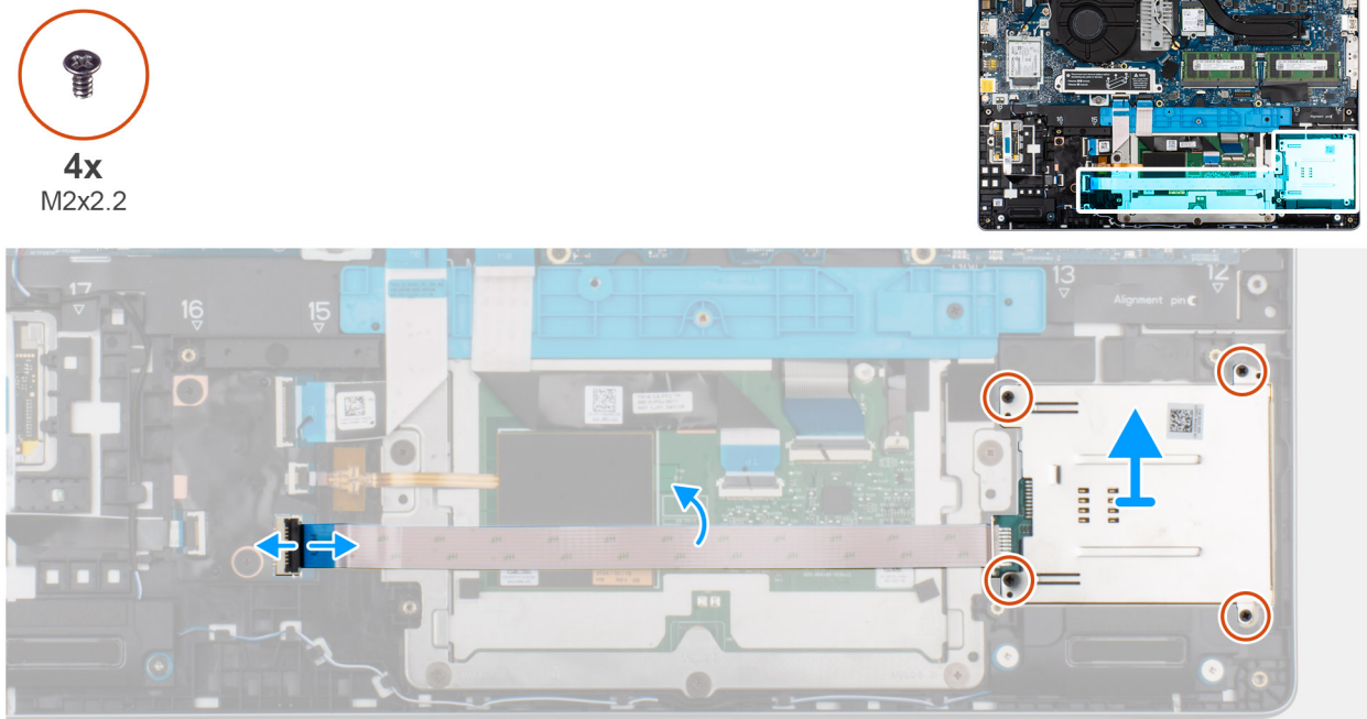
Figur 48. Ta bort smartkortläsaren
