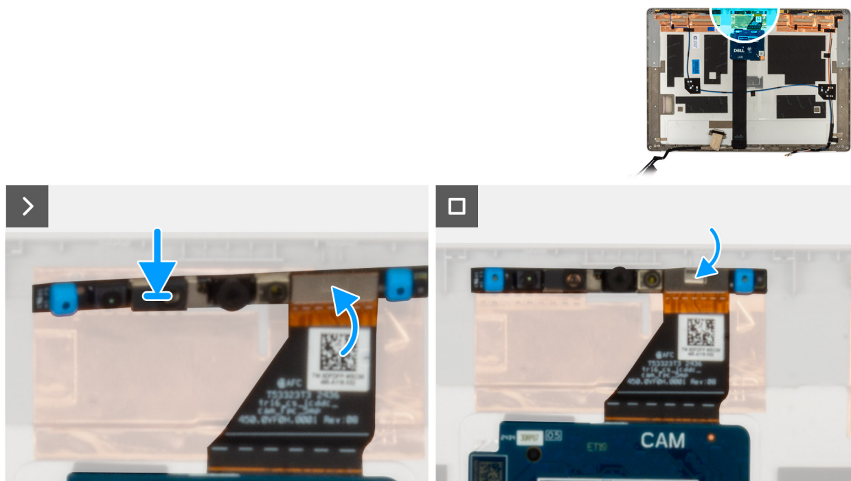
Figur 76. Installera kameramodulen
