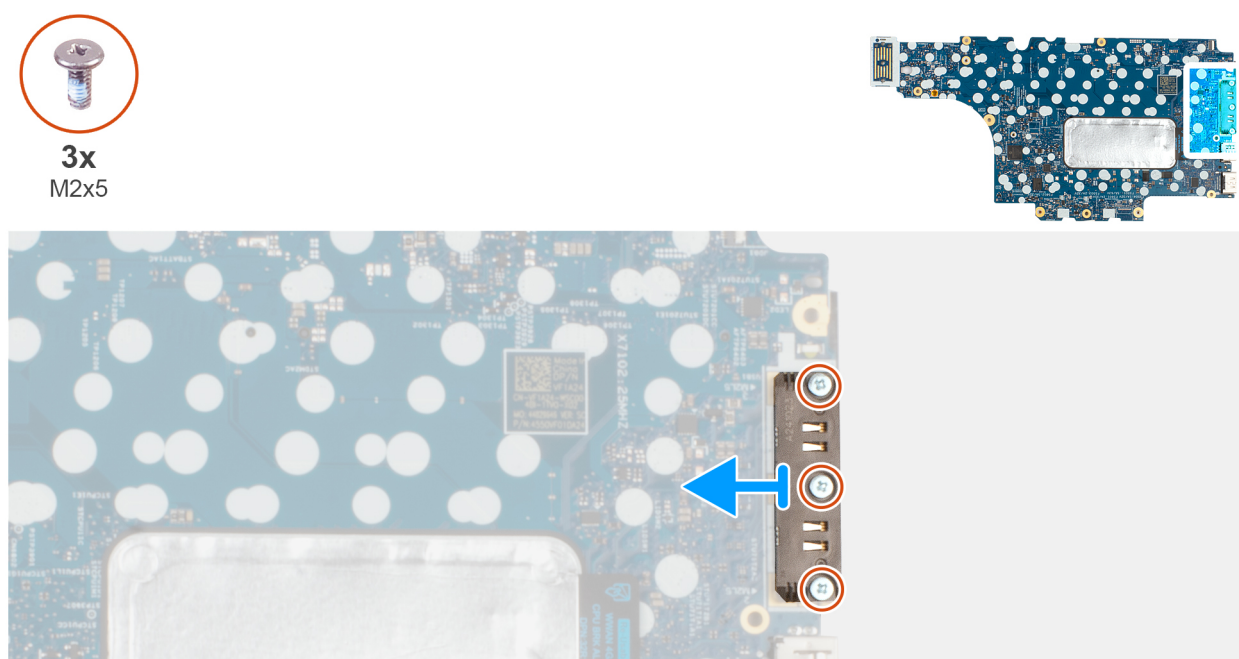
Figur 79. Ta bort USB typ-C-kontaktmodulen
