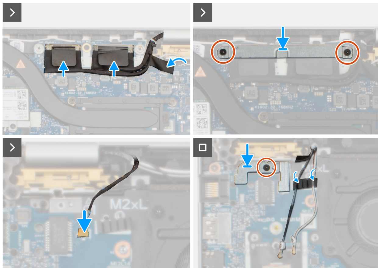
Figur 44. Installera WLAN-antennen
