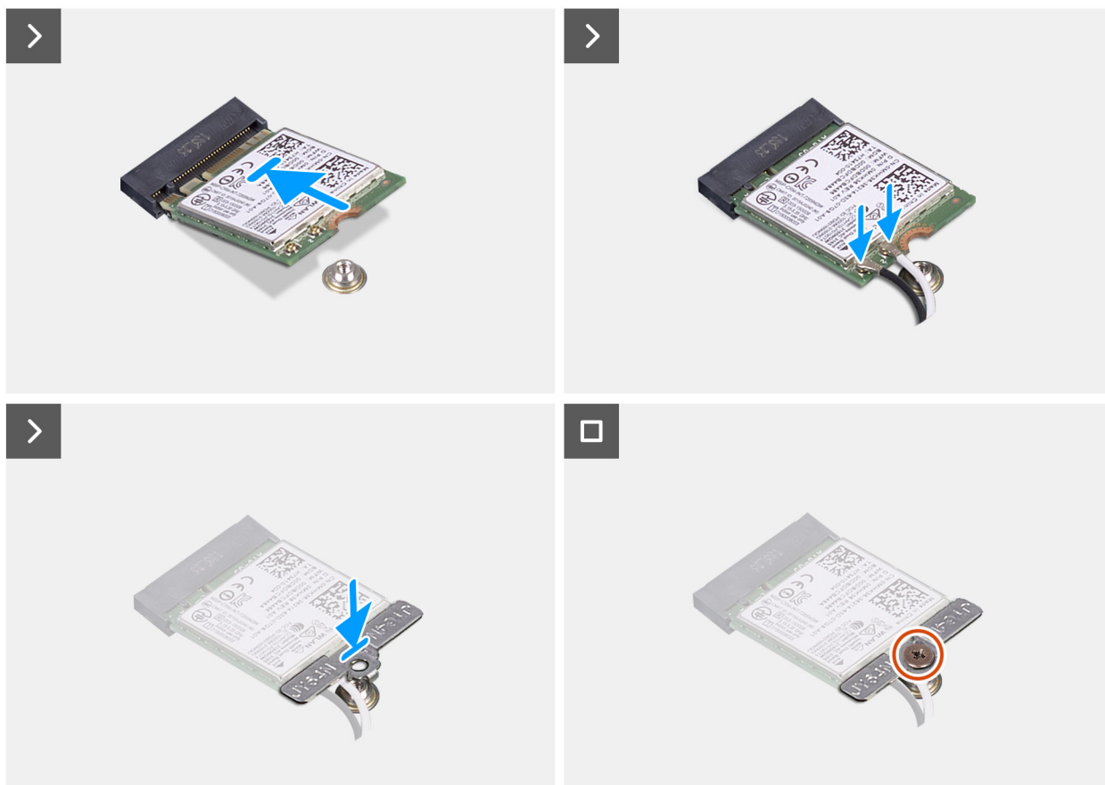
Figur 34. Installera WLAN-kortet
