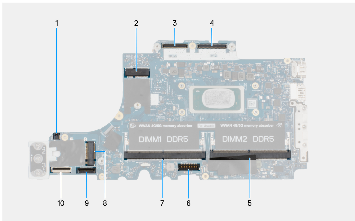
Figur 52. Kontakt på moderkortet
