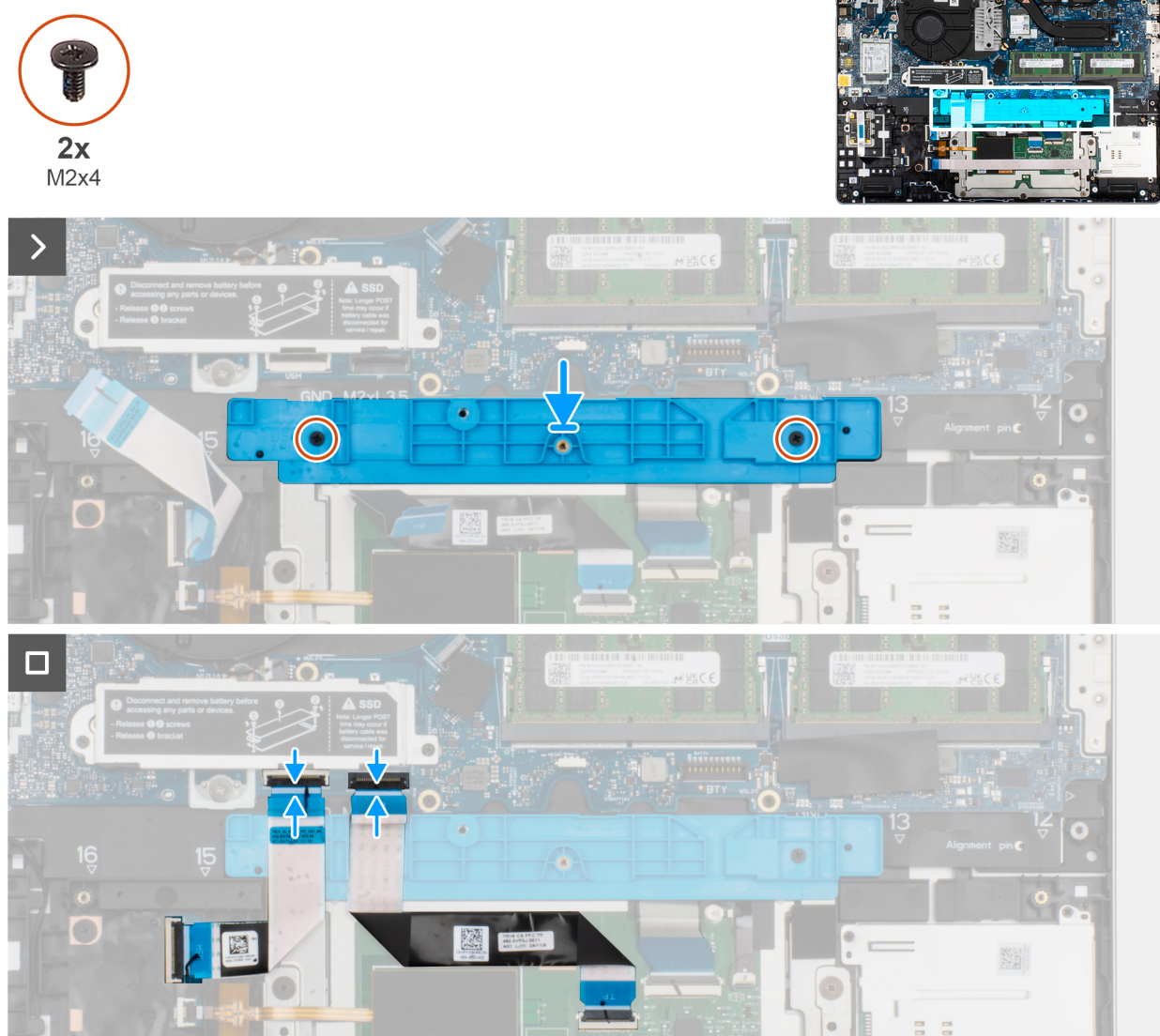
Figur 46. Installera batteristödkonsolen
