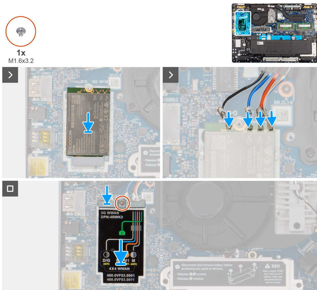
Figur 32. Installera 5G WWAN-kortet
