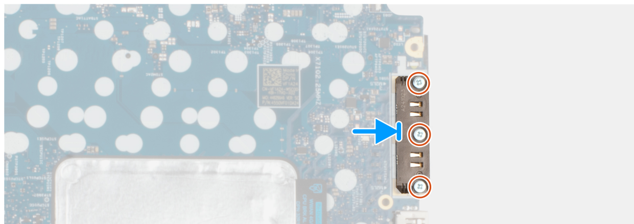
Figur 80. Installera USB typ-C-kontaktmodulen
