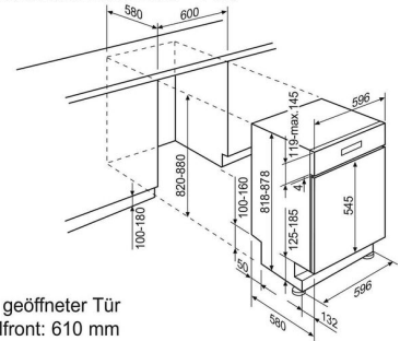
GA60SLIC/SLIS/GLIC/GLIS/LI + FI60
