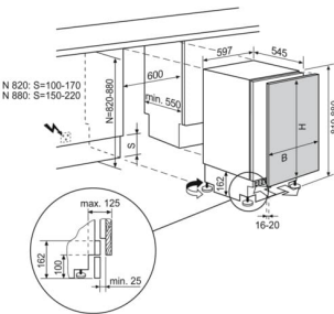
UK1205S / UG0985 (SMS) Möbelfront auf Gerätetür verschraubt
