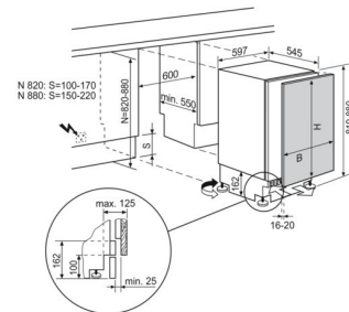
UK1205S / UG0985 (SMS) Möbelfront auf Gerätetür verschraubt
