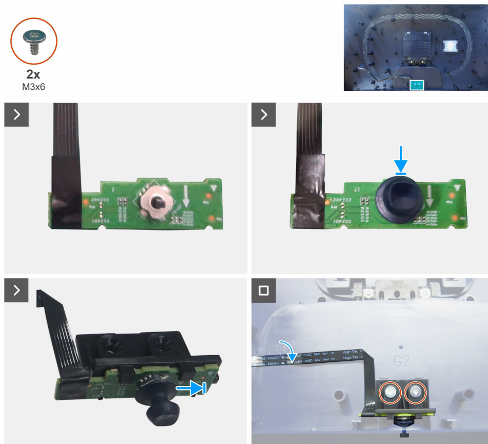
Obrázek 10. Instalace desky joysticku
