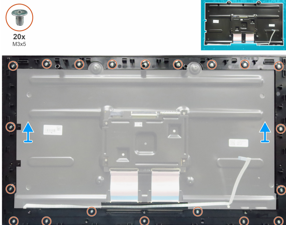
Obrázek 13. Demontáž středového rámečku
