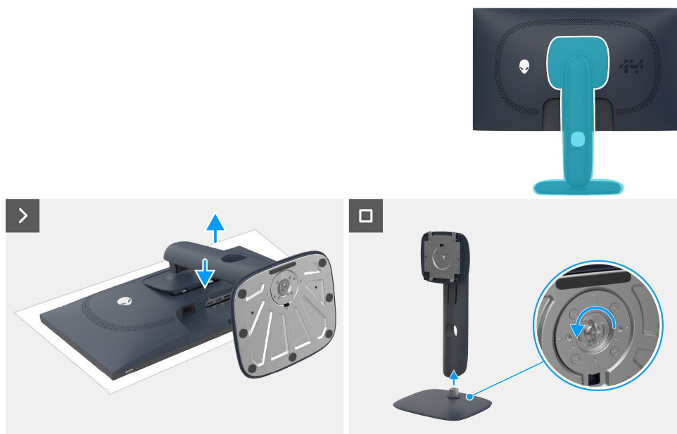
Obrázek 1. Demontáž stojanu
