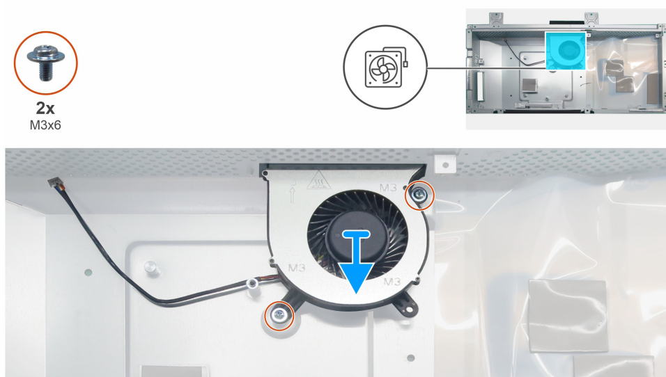
Obrázek 23. Demontáž ventilátoru
