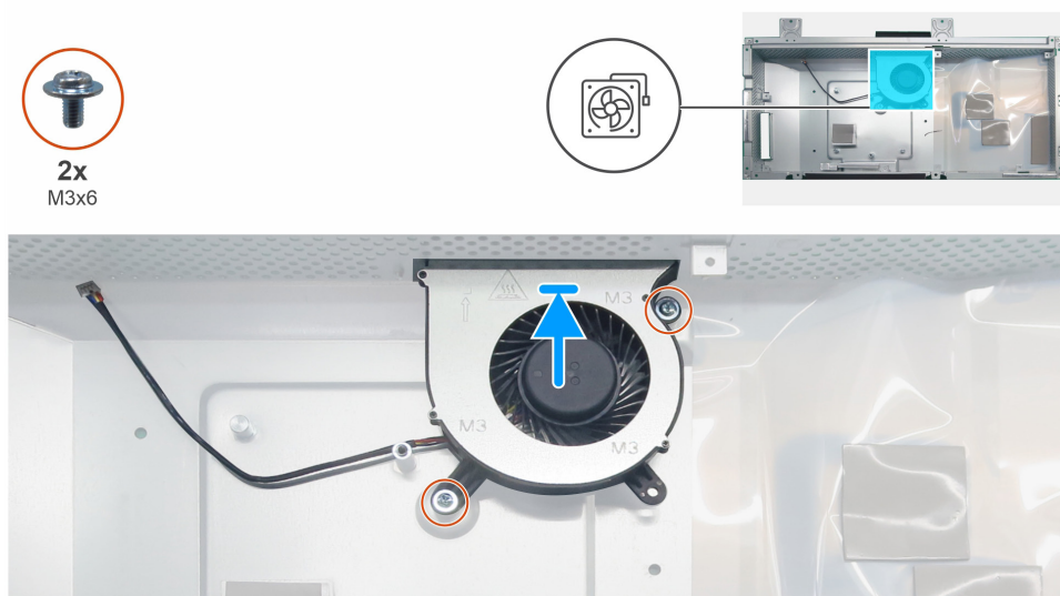
Obrázek 24. Instalace ventilátoru
