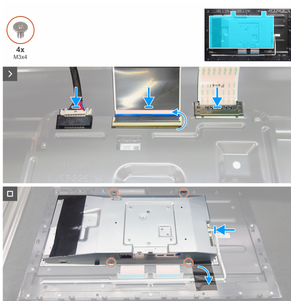
Obrázek 12. Instalace hlavního šasi
