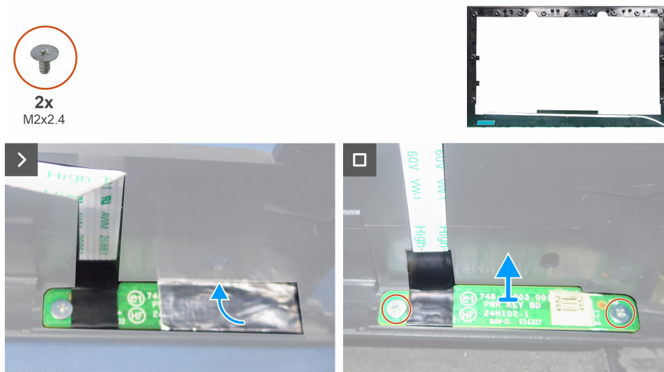
Obrázek 15. Demontáž desky klávesnice
