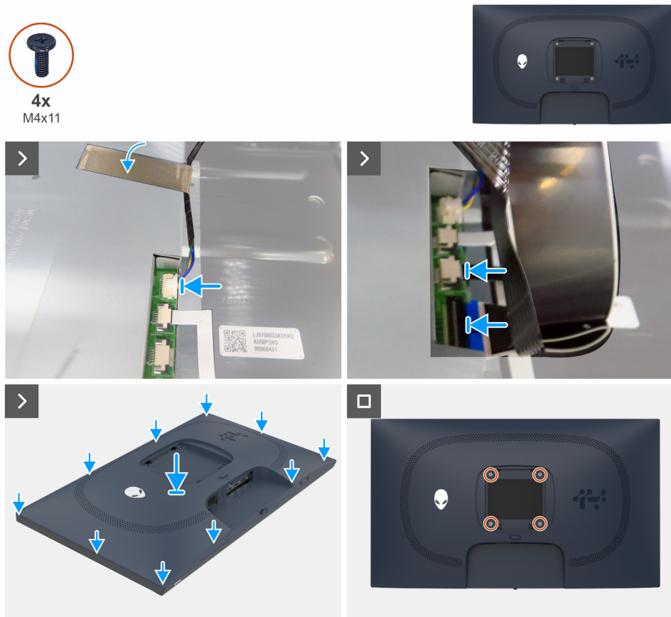
Obrázek 4. Instalace zadního krytu
