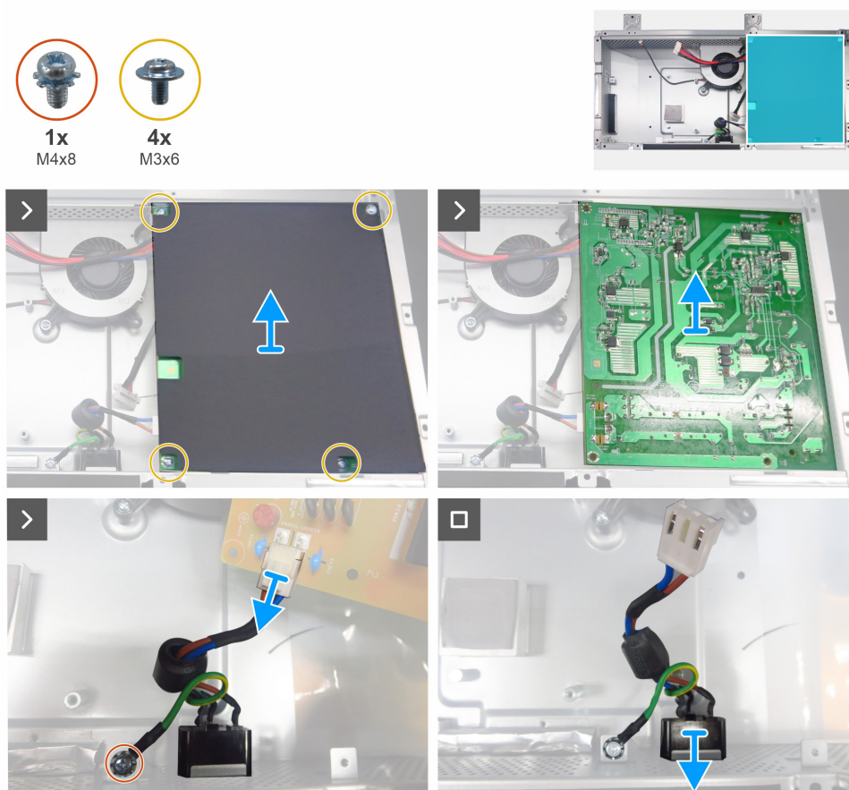
Obrázek 21. Demontáž napájecí desky
