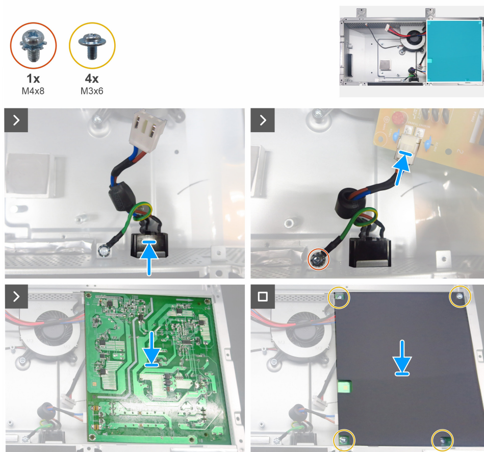
Obrázek 22. Instalace napájecí desky
