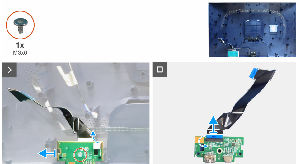
Obrázek 7. Demontáž USB desky
