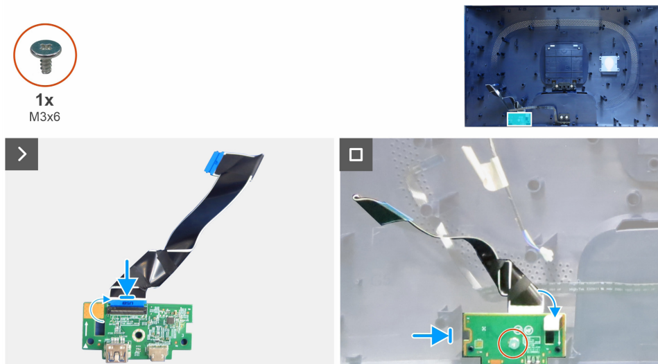
Obrázek 8. Instalace USB desky
