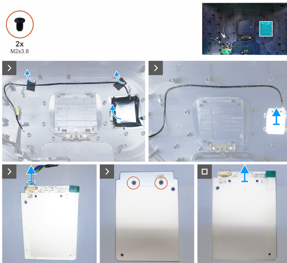
Obrázek 5. Demontáž modulu podsvícení
