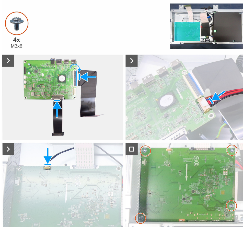
Obrázek 20. Instalace hlavní desky
