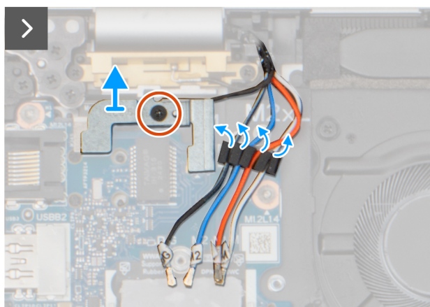
Afbeelding 61. De beeldschermeenheid verwijderen
