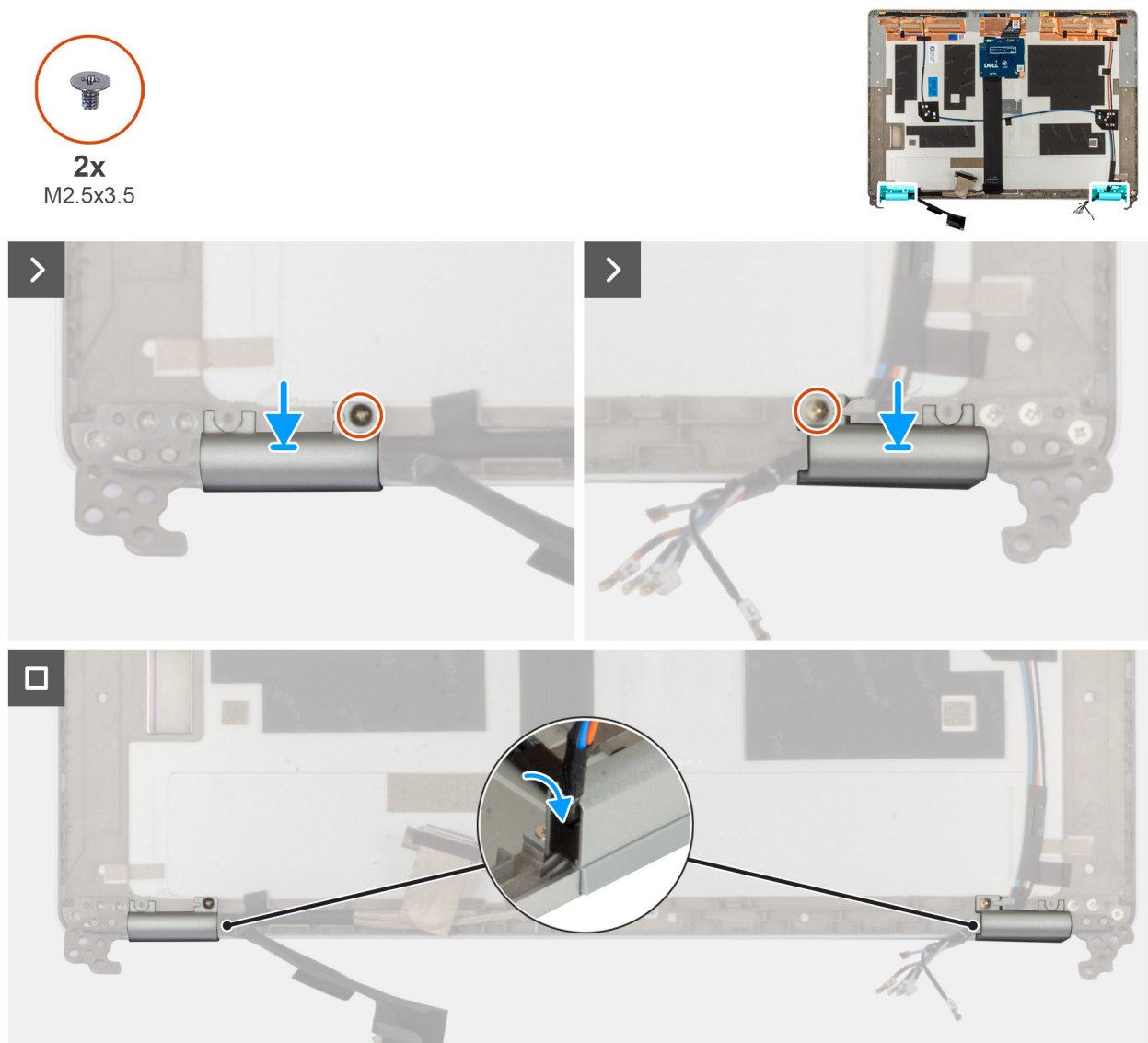
Afbeelding 75. De beeldschermcharnieraap installeren
