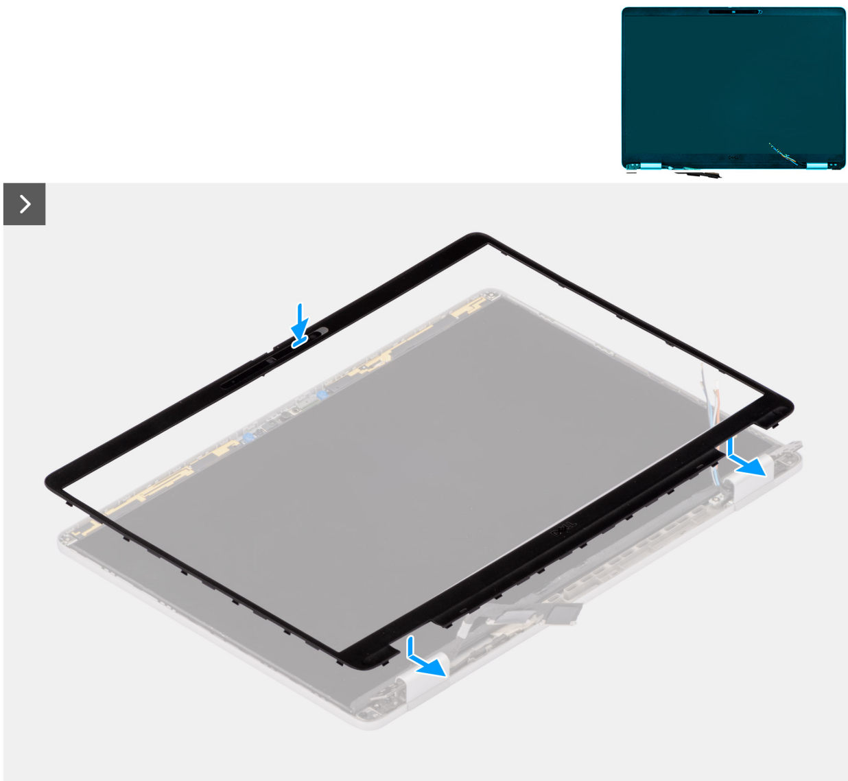
Afbeelding 69. De beeldschermbezel installeren
