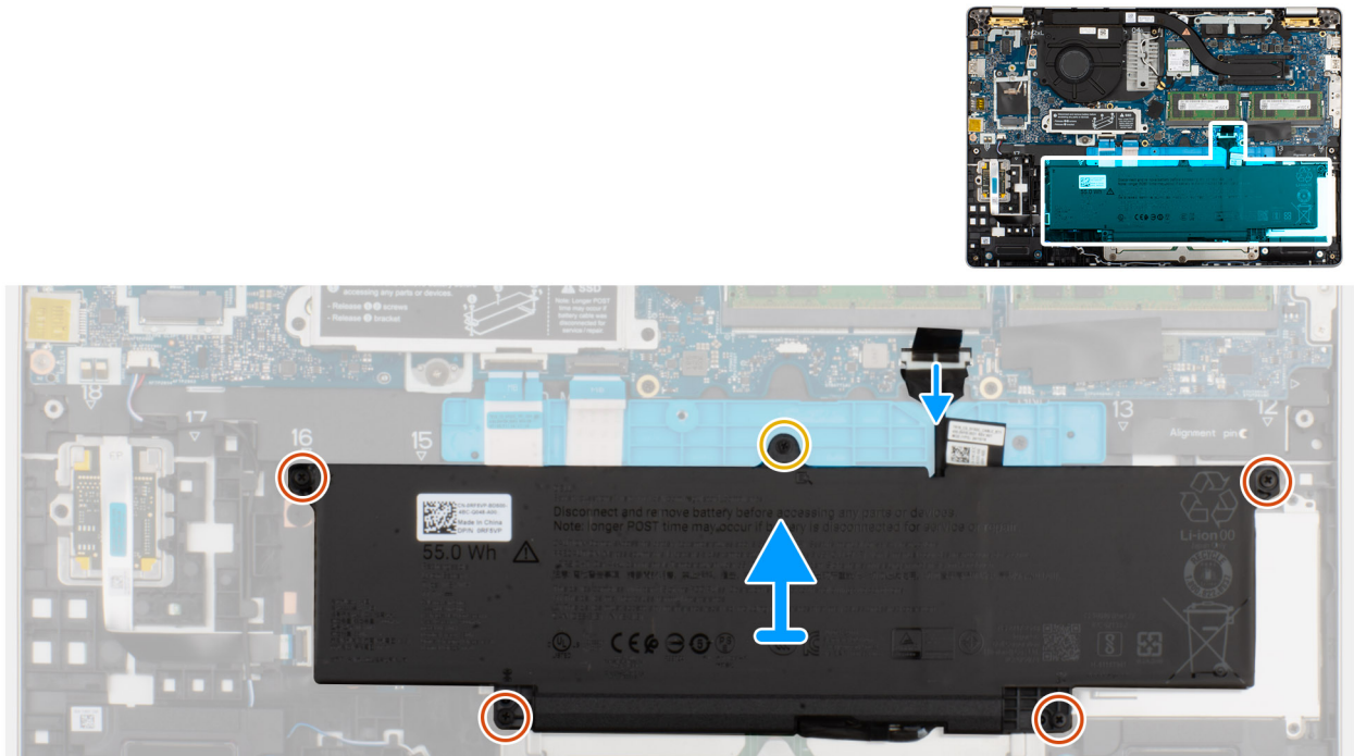
Afbeelding 15. De batterijkabel loskoppelen
