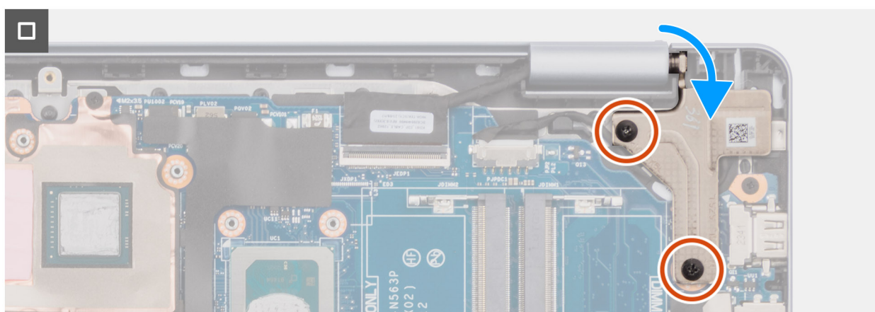
Abbildung 87. Einbau der Systemplatine
