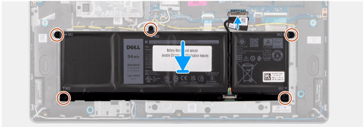
Abbildung 20. Installieren des 4-Zellen-Akkus
