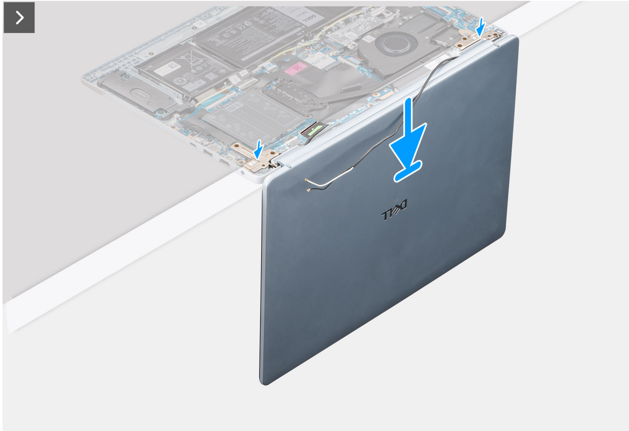
Abbildung 52. Einbauen der Bildschirmbaugruppe
