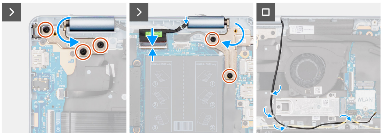
Abbildung 53. Einbauen der Bildschirmbaugruppe
