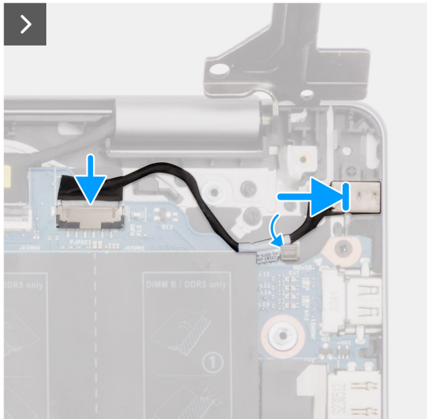
Abbildung 78. Einbauen des Netzadapteranschlusses
