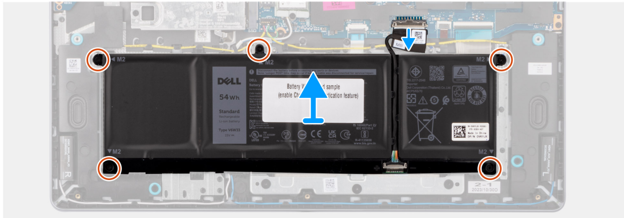
Abbildung 19. Entfernen des 4-Zellen-Akkus
