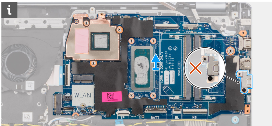
Abbildung 83. Systemplatine – USB-Typ-C-Halterung
