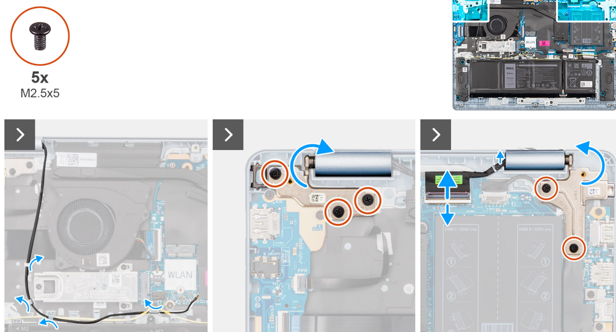
Abbildung 50. Entfernen der Bildschirmbaugruppe
