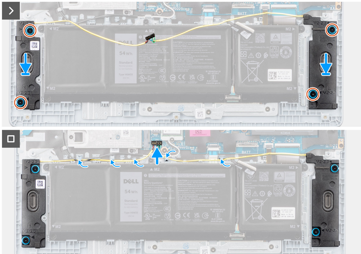
Abbildung 35. Installieren der Lautsprecher
