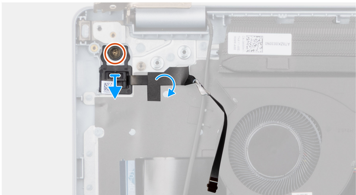
Abbildung 74. Entfernen des Netzschalters mit Fingerabdruck-Lesegerät
