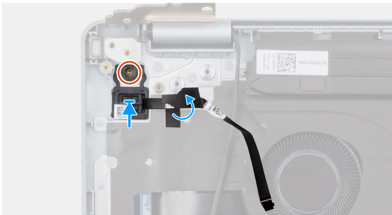
Abbildung 75. Einbauen des Netzschalters mit Fingerabdruck-Lesegerät
