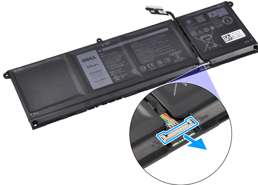
Abbildung 23. Lösen des Akkukabelanschlusses
