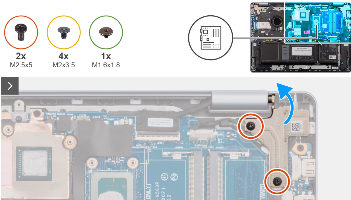
Abbildung 80. Entfernen der Systemplatine
