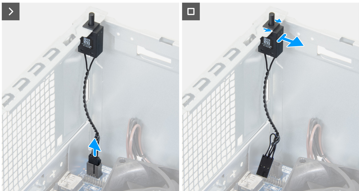
Abbildung 48. Entfernen des Eingriffsschalters
