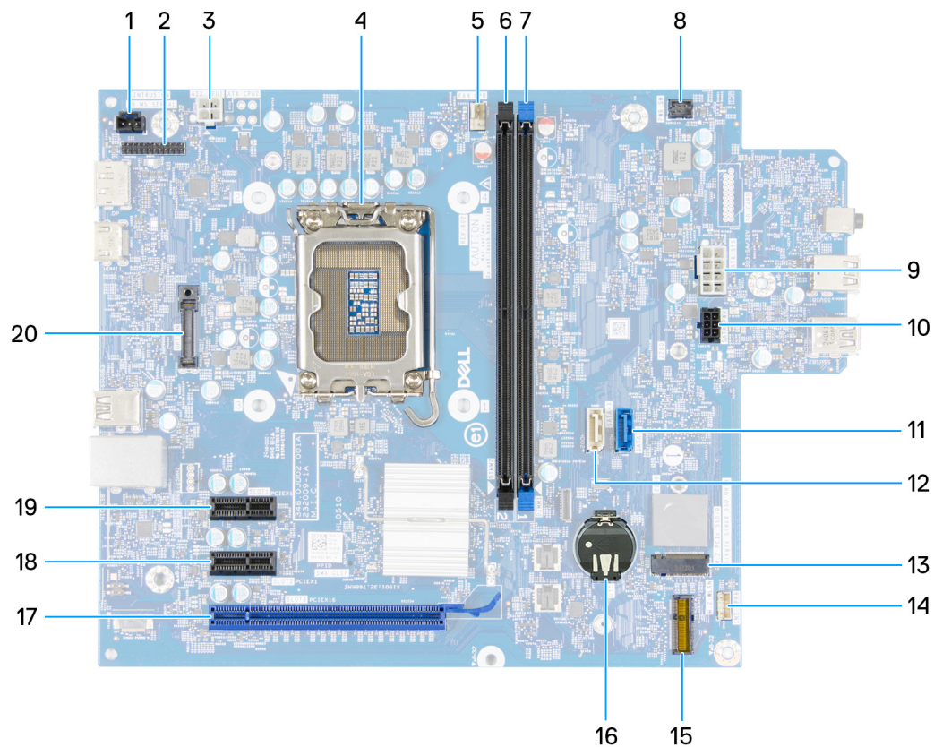
Abbildung 70. Systemplatinenbeschriftung
