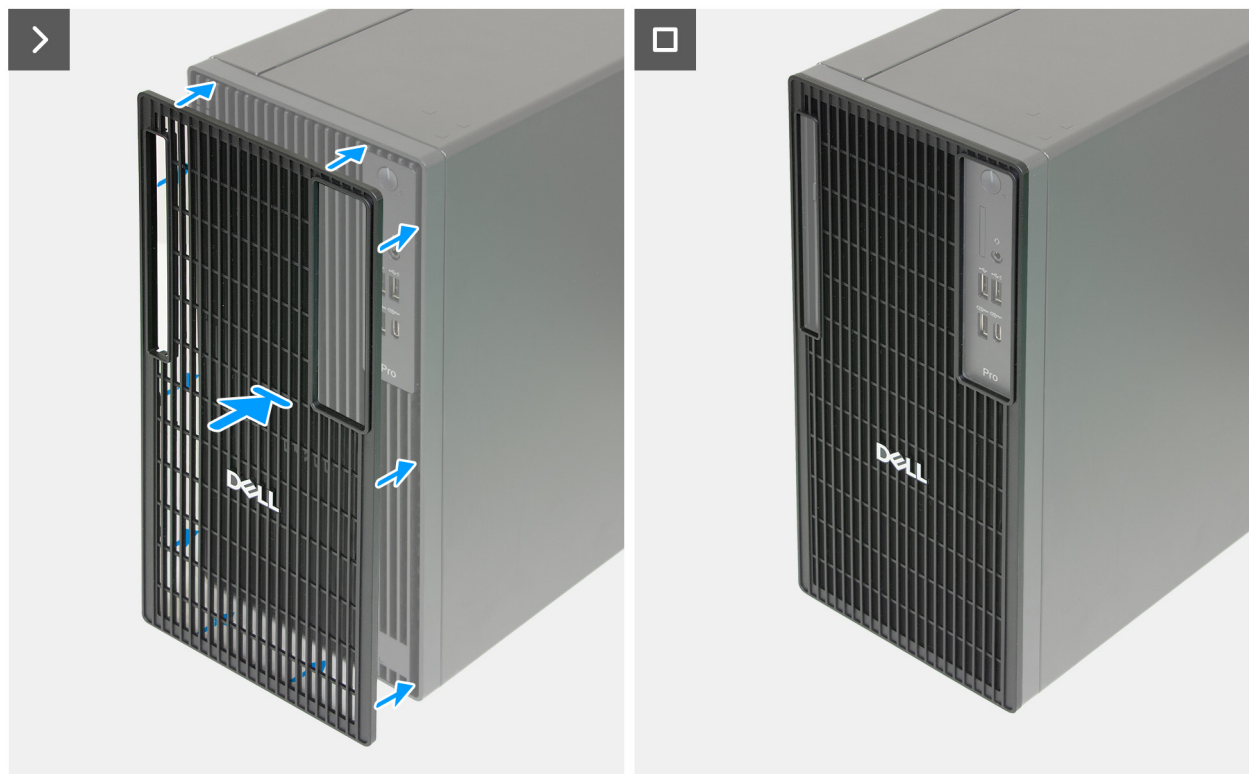
Abbildung 22. Installieren des Staubfilters
