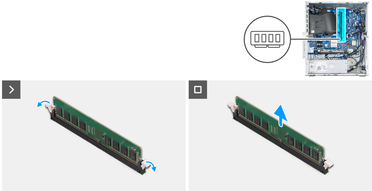
Abbildung 27. Entfernen des Speichers
