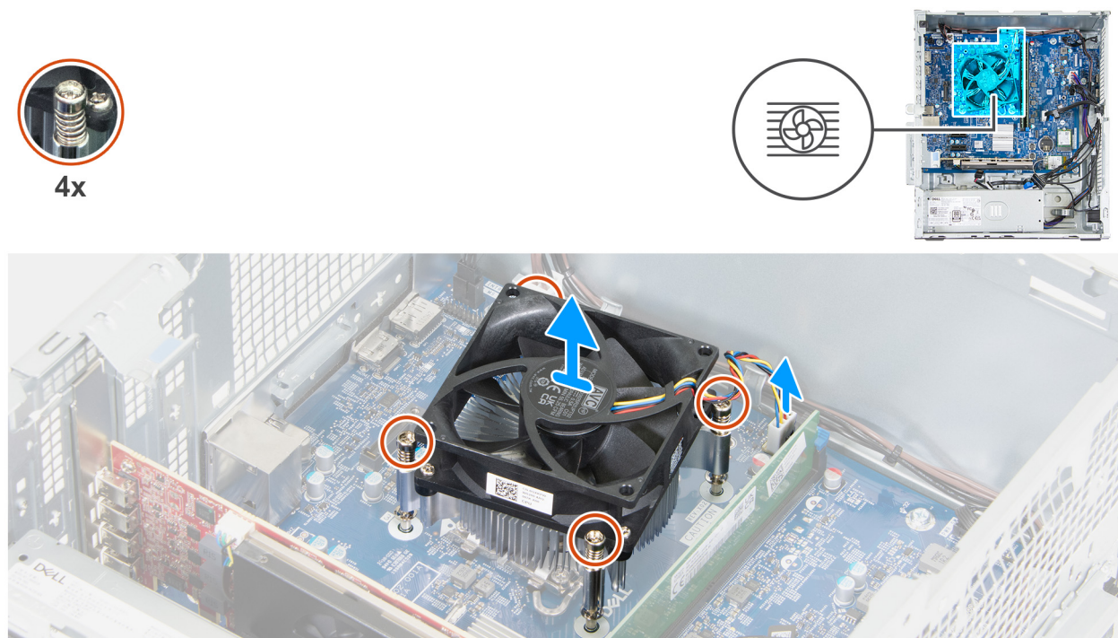
Abbildung 66. Entfernen des Prozessorlüfters und der Kühlkörperbaugruppe
