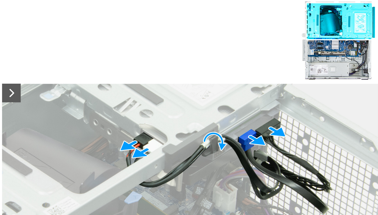
Abbildung 42. Entfernen des Laufwerksschachts
