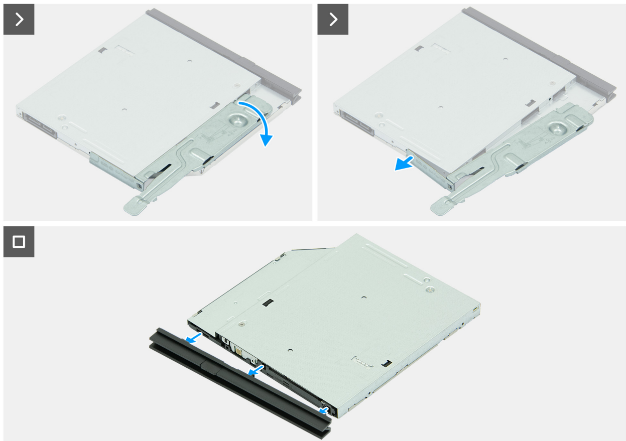
Abbildung 39. Entfernen des optischen Laufwerks
