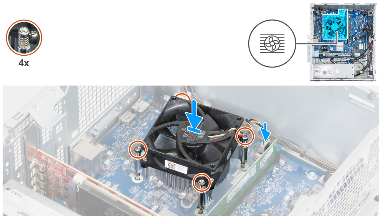
Abbildung 67. Installieren des Prozessorlüfters und der Kühlkörperbaugruppe
