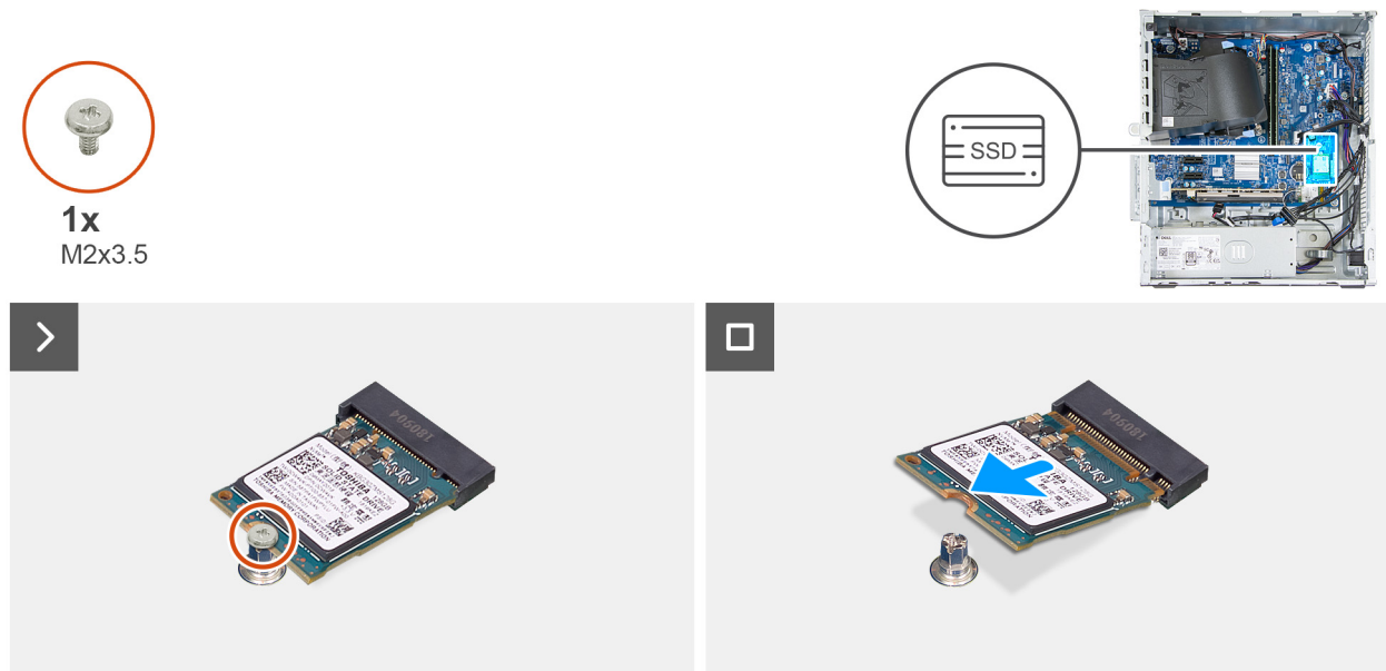
Abbildung 29. Entfernen des M.2-2230-Solid-State-Laufwerks
