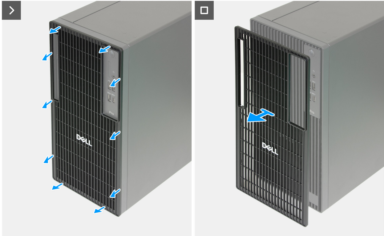
Abbildung 21. Staubfilter entfernen
