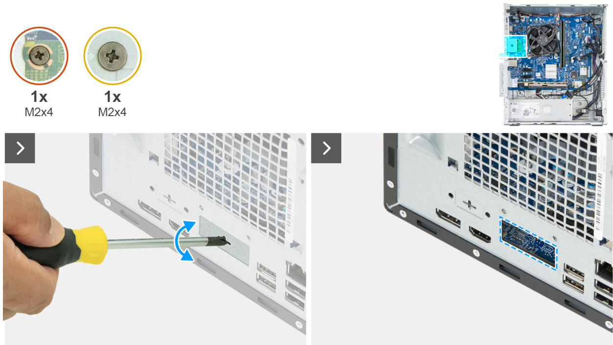
Abbildung 55. Installieren des optionalen Portmoduls
