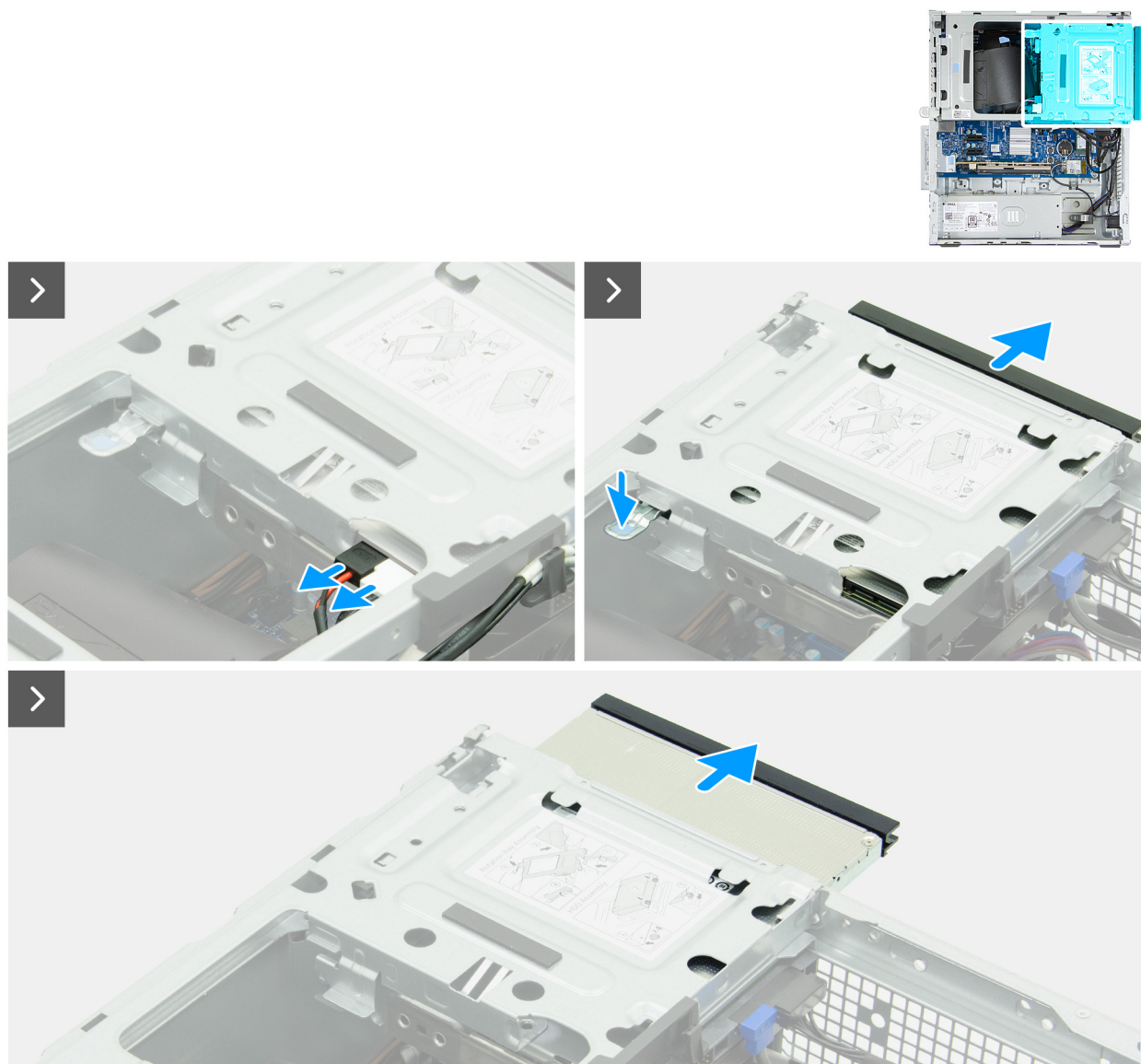
Abbildung 38. Entfernen des optischen Laufwerks
