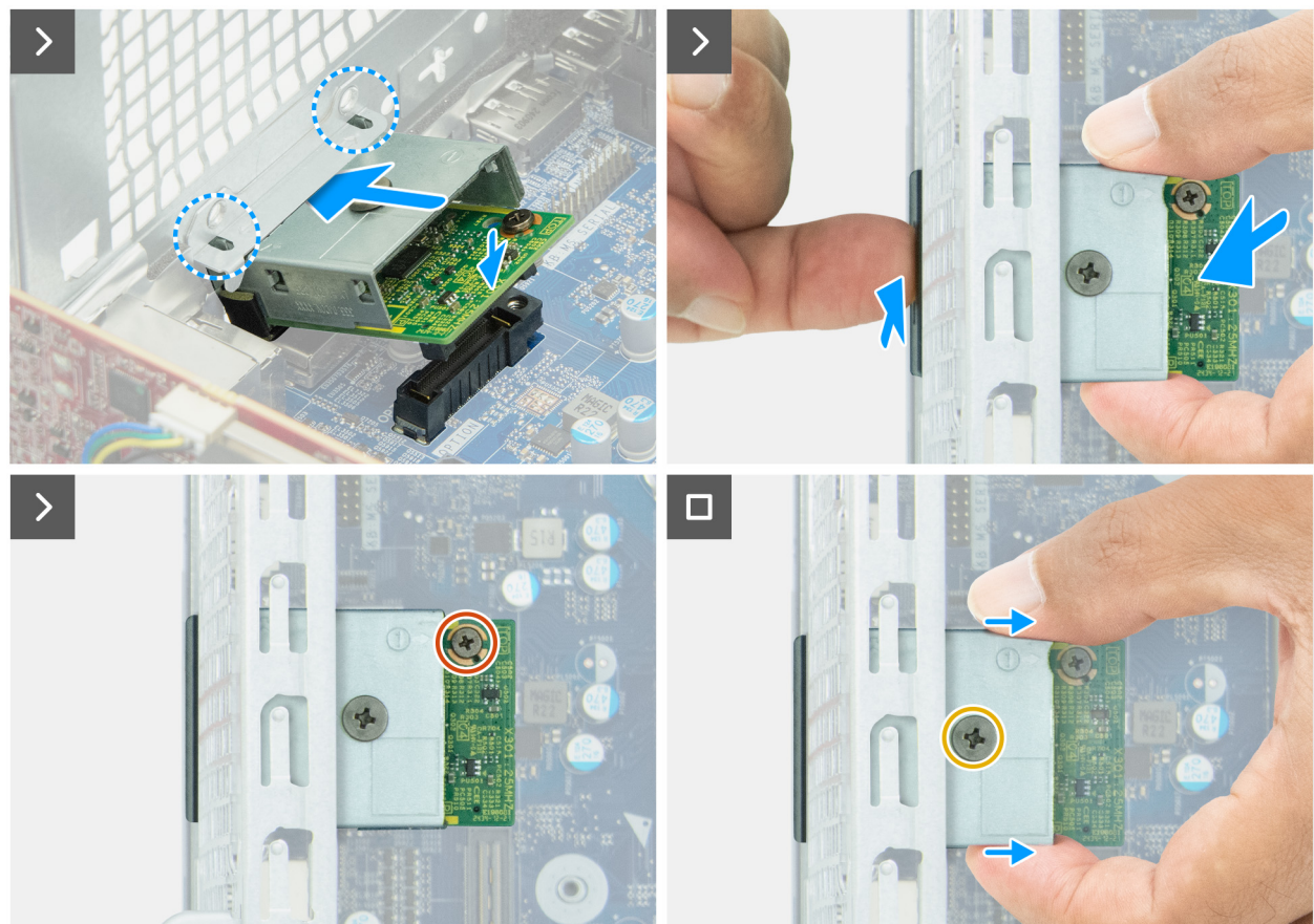
Abbildung 56. Installieren des optionalen Portmoduls
