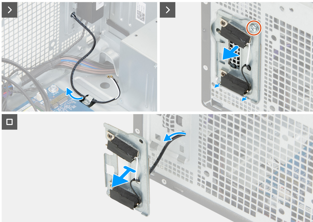
Abbildung 60. Entfernen der Antennenmodule
