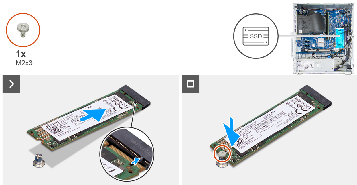
Abbildung 32. Einbauen des M.2-2280-Solid-State-Laufwerks
