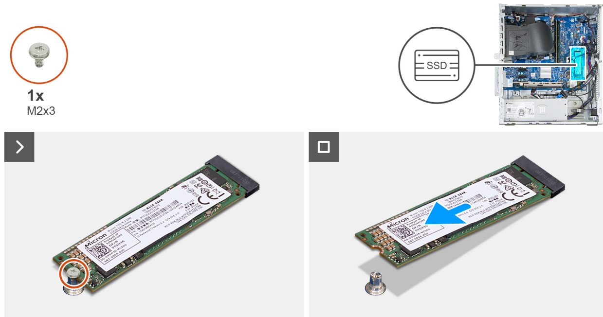
Abbildung 31. Entfernen des M.2-2280-Solid-State-Laufwerks
