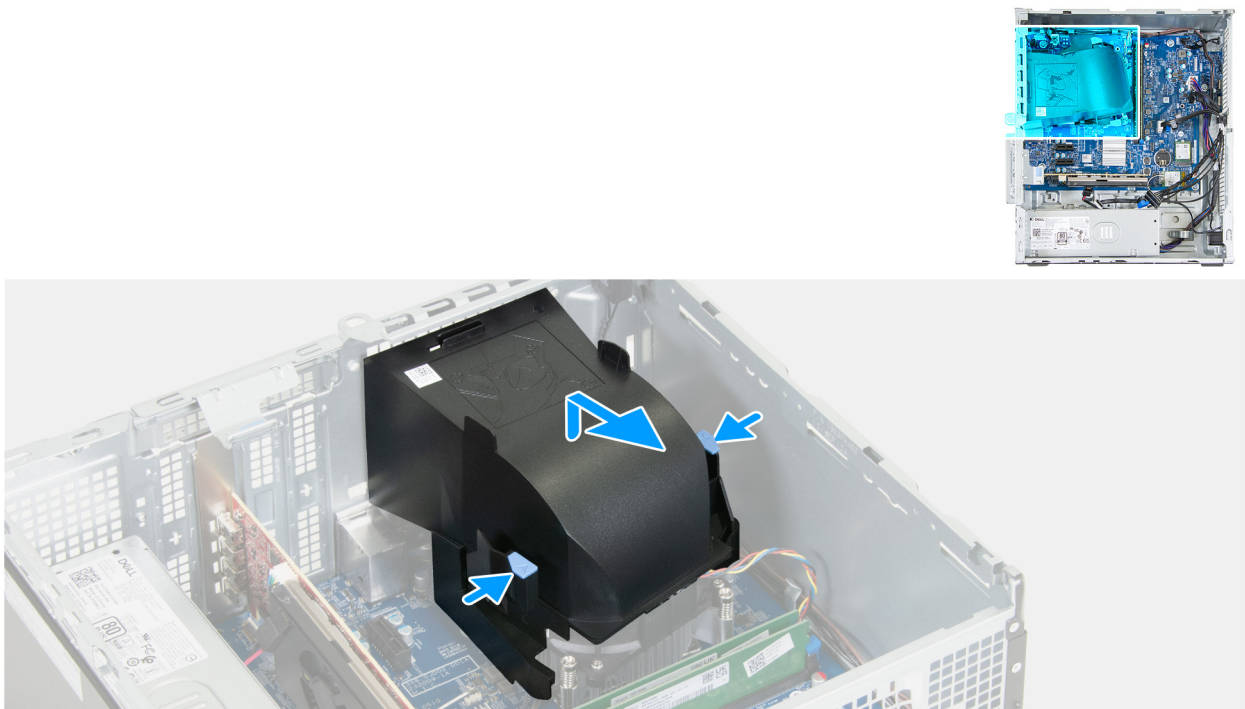
Abbildung 52. Abbildung: Entfernen der Lüfterverkleidung
