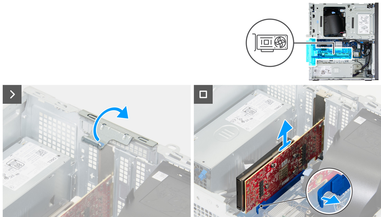
Abbildung 34. Entfernen der Grafikkarte
