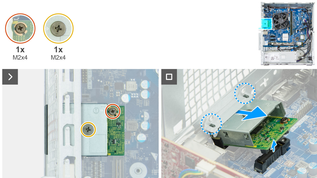
Abbildung 54. Entfernen des Moduls mit optionalem Anschluss
