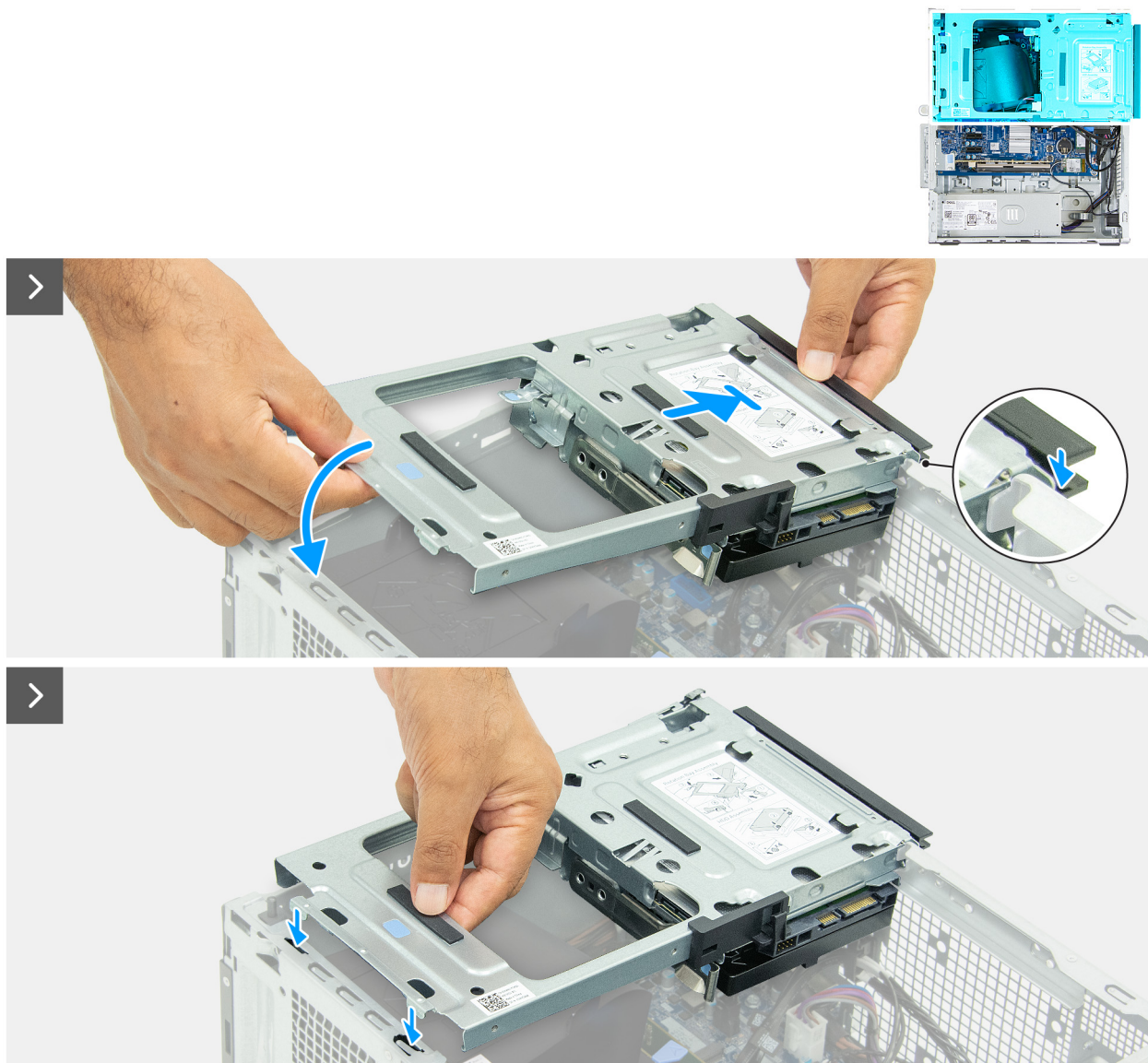
Abbildung 44. Einbauen des Laufwerkschachts
