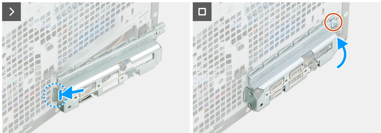
Abbildung 79. Einbau der Systemplatine
