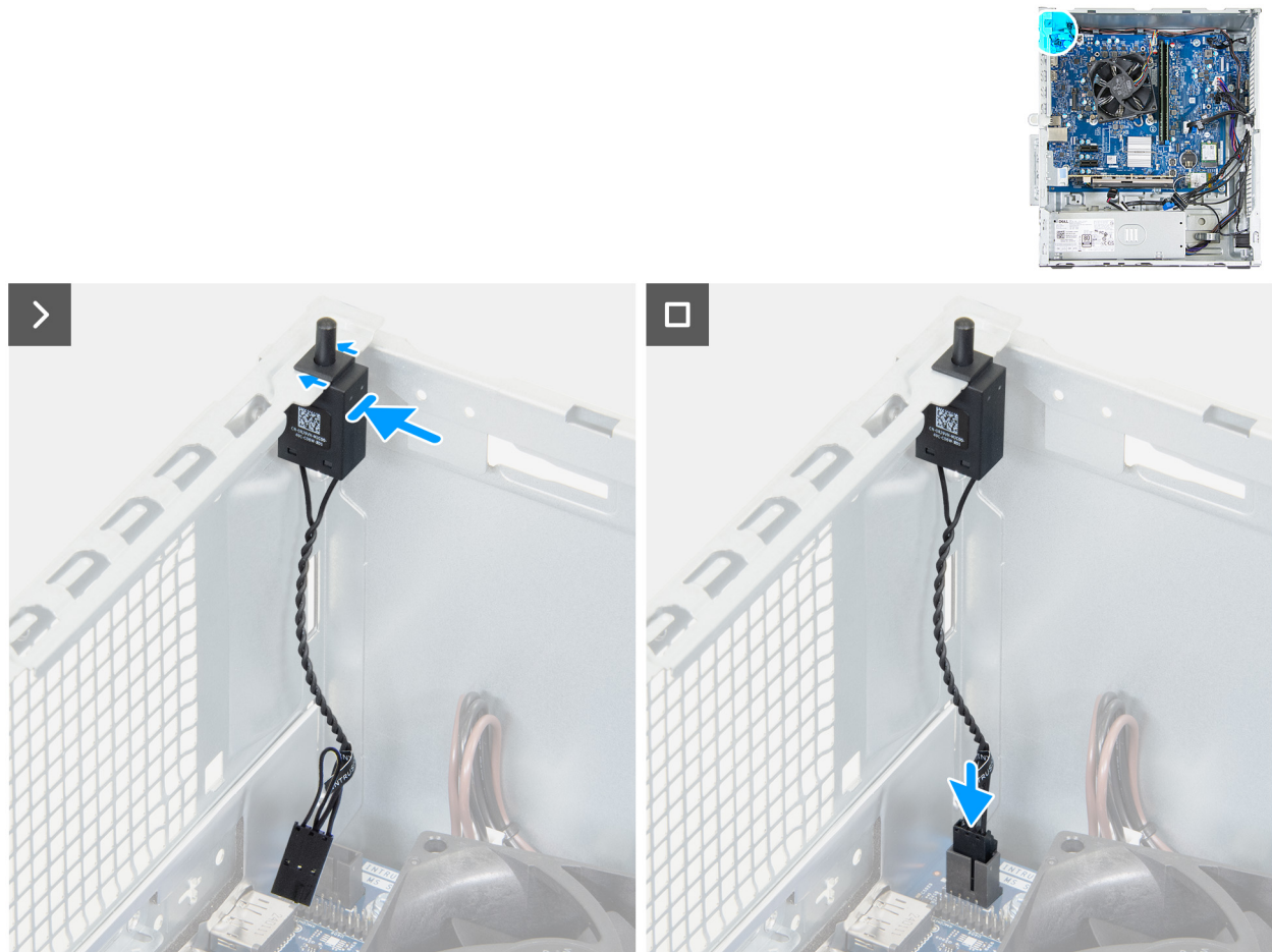
Abbildung 49. Installieren des Eingriffsschalters
