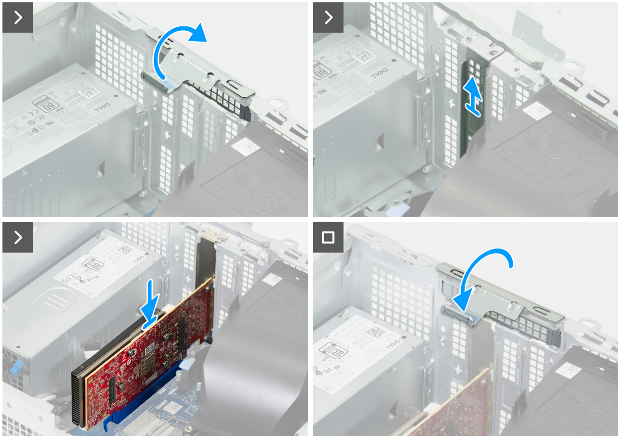
Abbildung 35. Installieren der Grafikkarte
