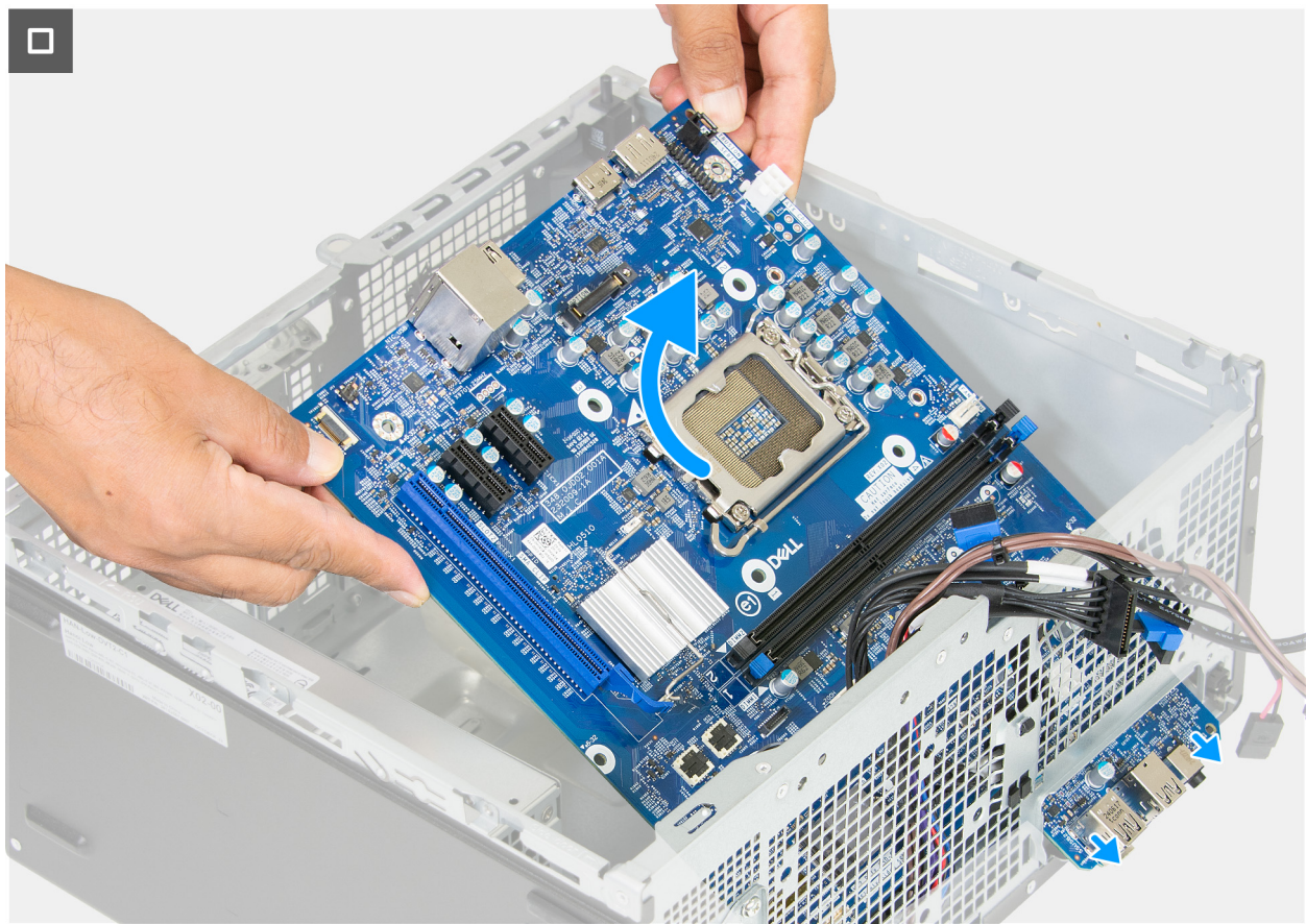
Abbildung 74. Entfernen der Systemplatine
