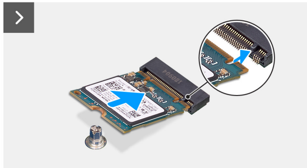
Abbildung 30. Installieren des M.2-2230-Solid-State-Laufwerks
