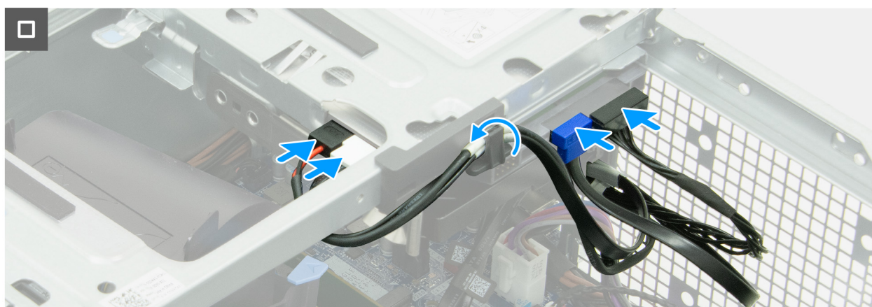
Abbildung 45. Einbauen des Laufwerkschachts
