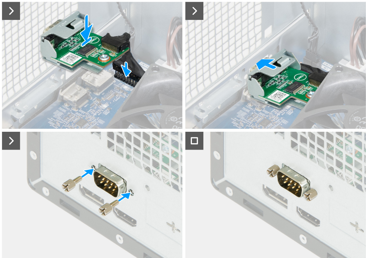
Abbildung 59. Installieren des seriellen Anschlussmoduls
