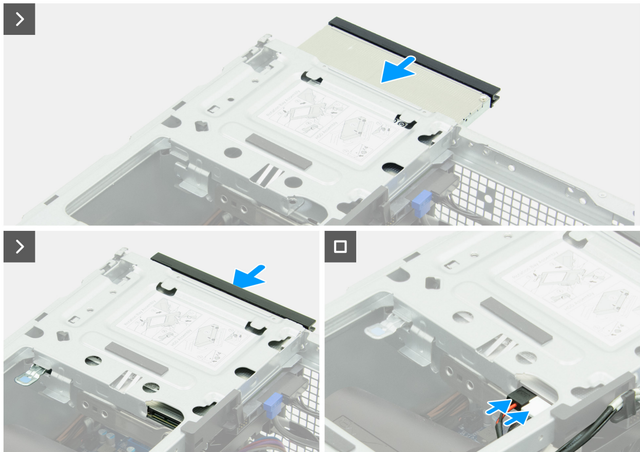
Abbildung 41. Installieren des optischen Laufwerks
