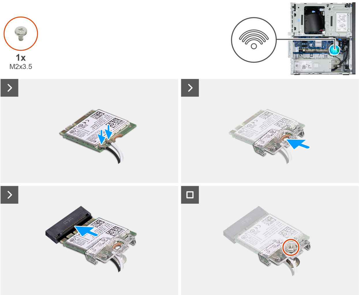
Abbildung 37. Installieren der Wireless-Karte
