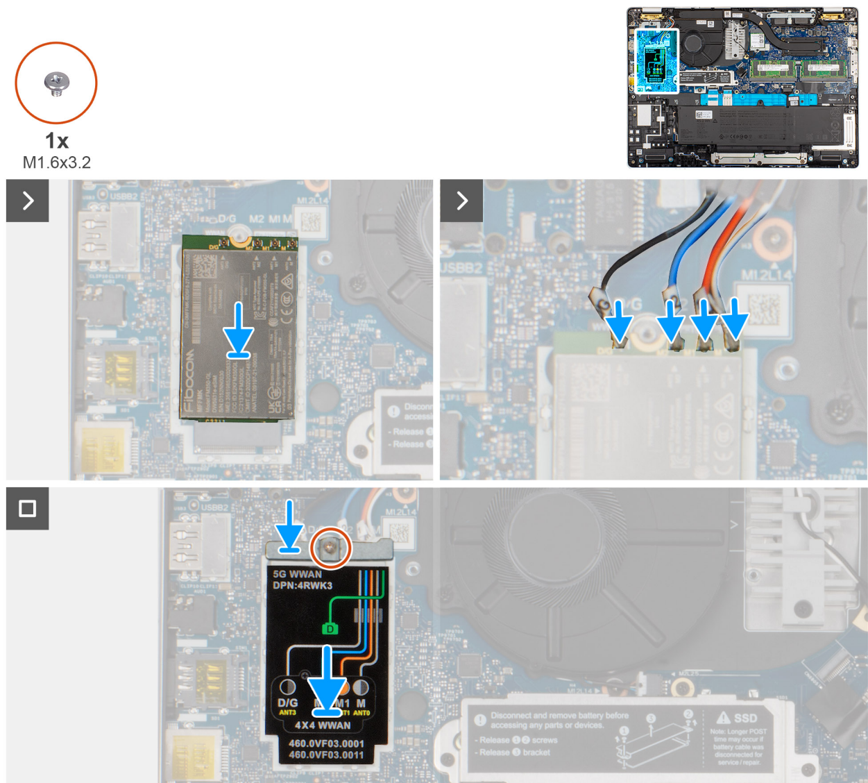
Figure 32. Installation de la carte WWAN 5G
