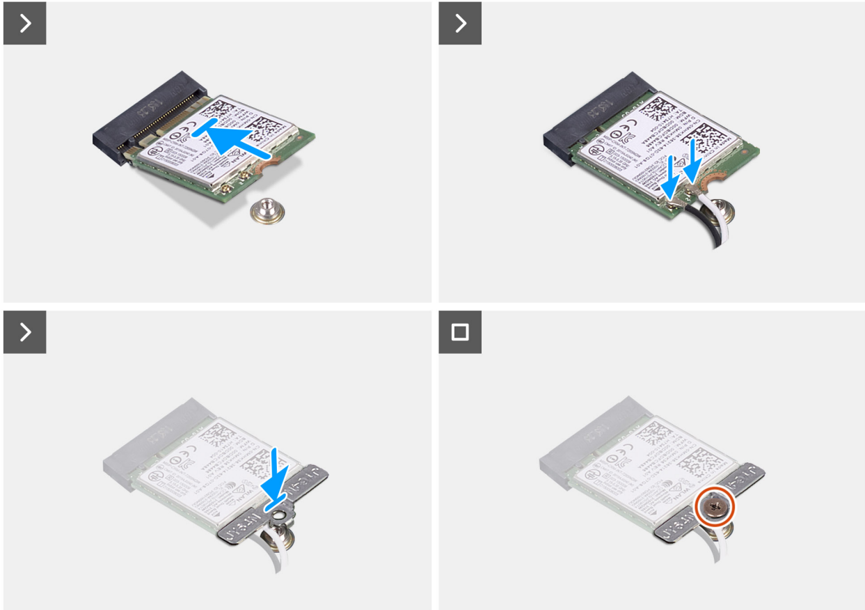
Figure 34. Installation de la carte WLAN
