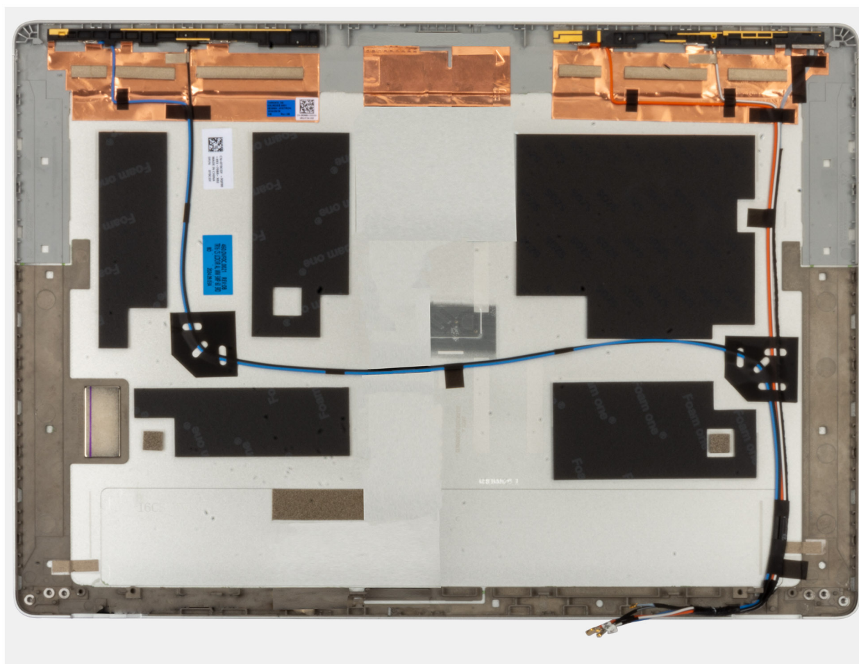
Figure 77. Retrait du capot arrière d'écran
