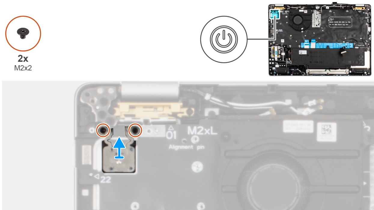
Figure 56. Installation du bouton d'alimentation avec lecteur d'empreintes digitales (en option)
