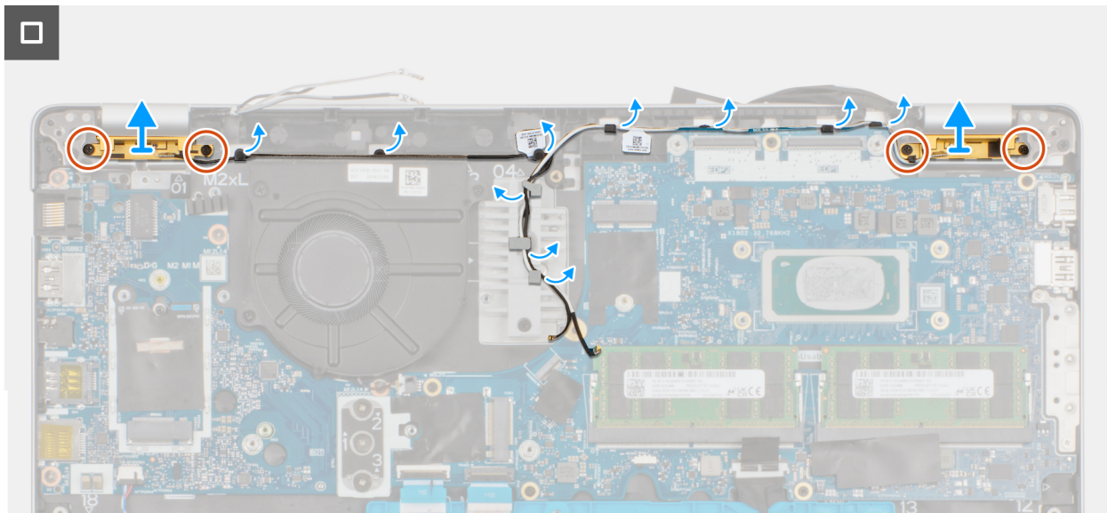
Figure 42. Retrait de l'antenne WLAN
