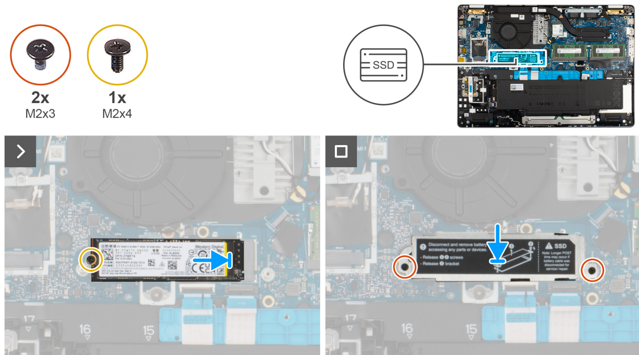
Figure 28. Installation du disque SSD M.2230
