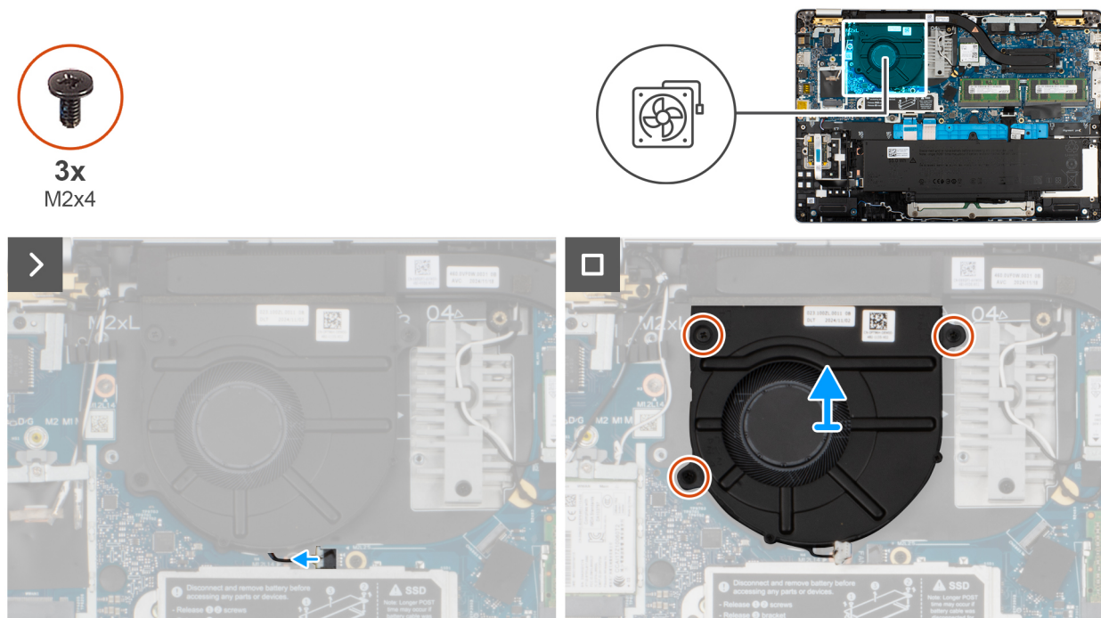
Figure 35. Retrait du ventilateur
