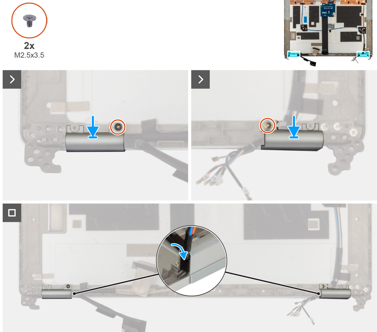
Figure 72. Installation du cache de la charnière d'écran
