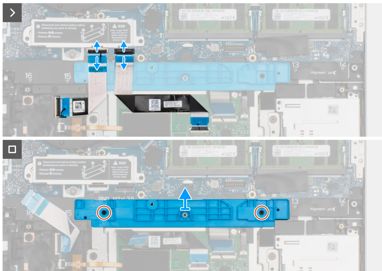
Figure 45. Retrait du support de la batterie
