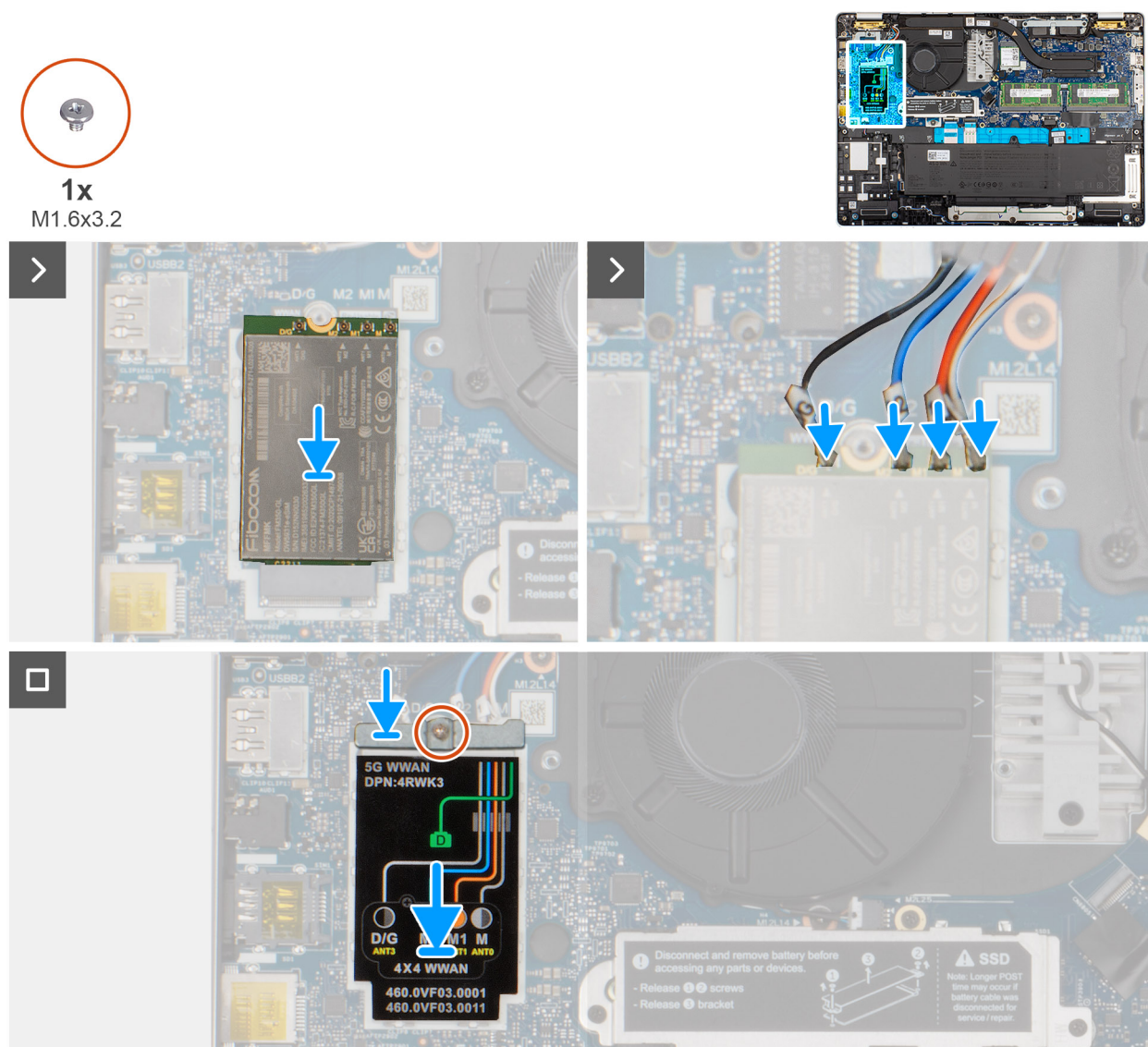
Afbeelding 32. De 5G WWAN-kaart installeren
