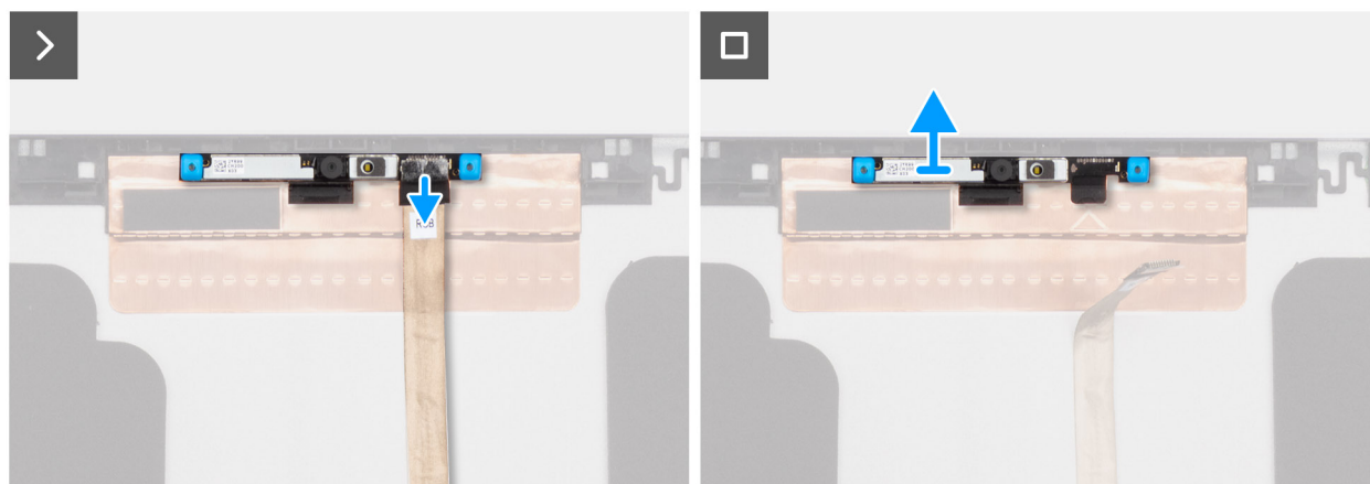
Afbeelding 75. De cameramodule verwijderen
