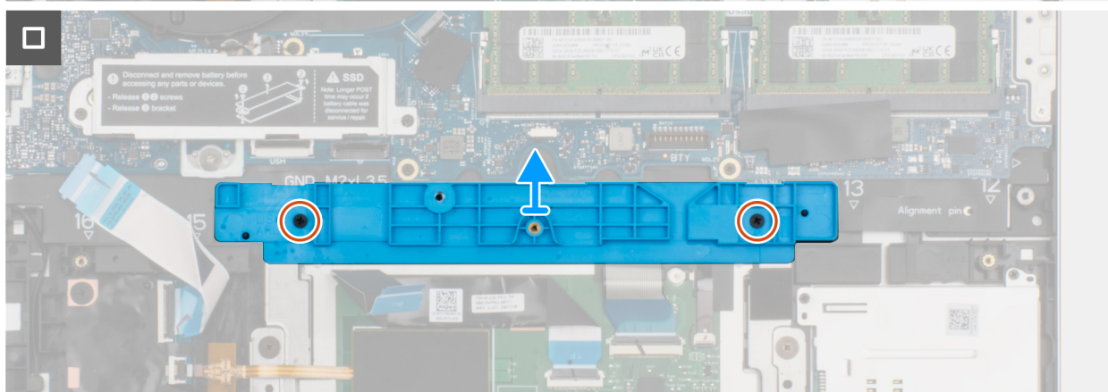
Afbeelding 45. De ondersteuningsbeugel van de batterij verwijderen
