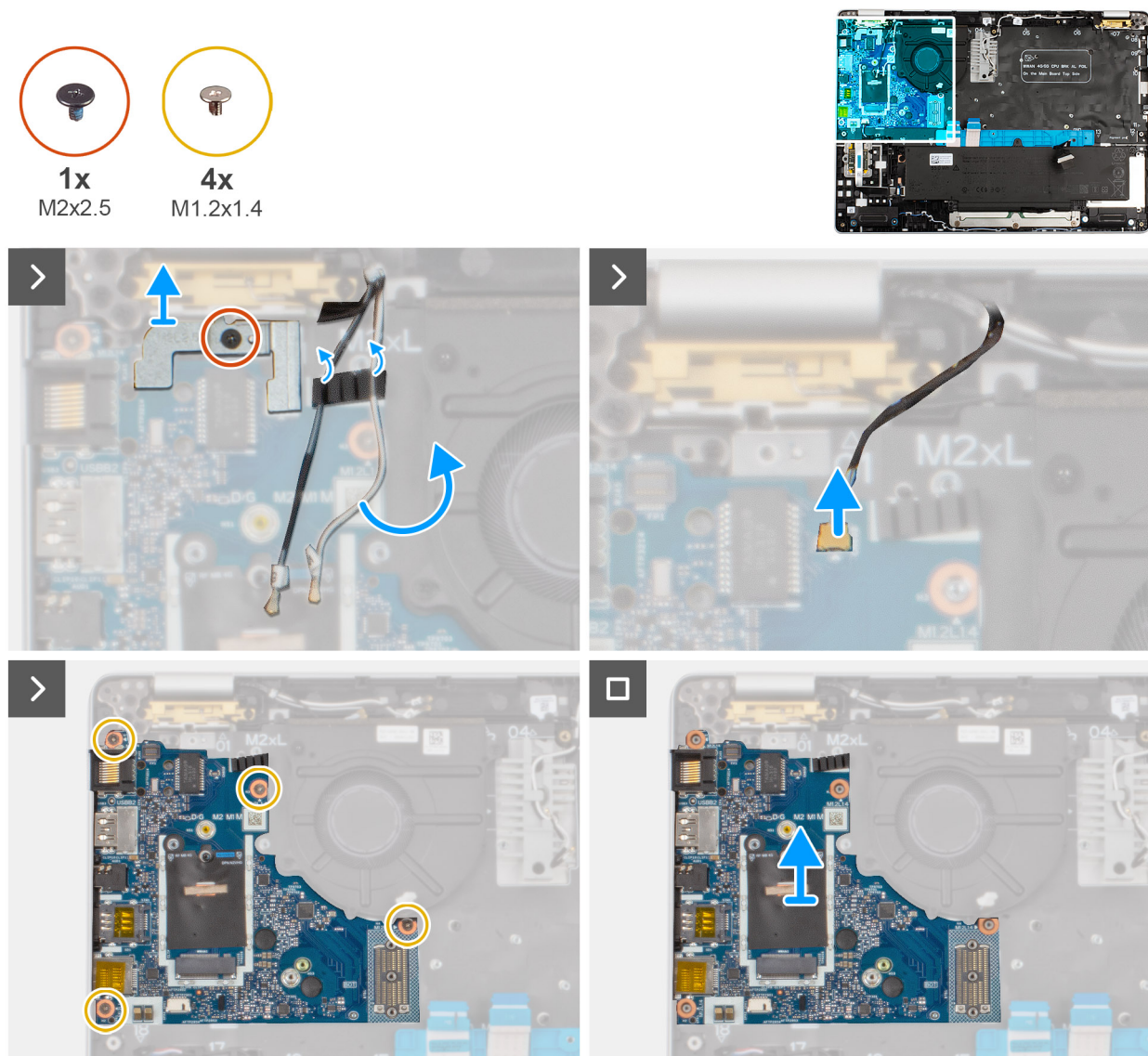
Afbeelding 55. De I/O-kaart verwijderen
