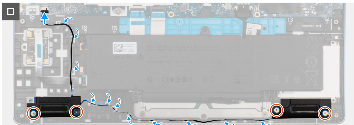
Afbeelding 37. De luidsprekers installeren
