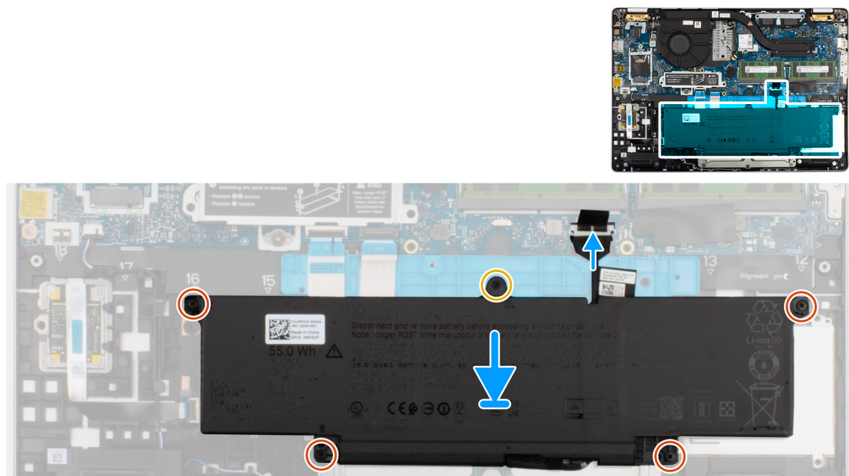
Afbeelding 16. De batterijkabel aansluiten
