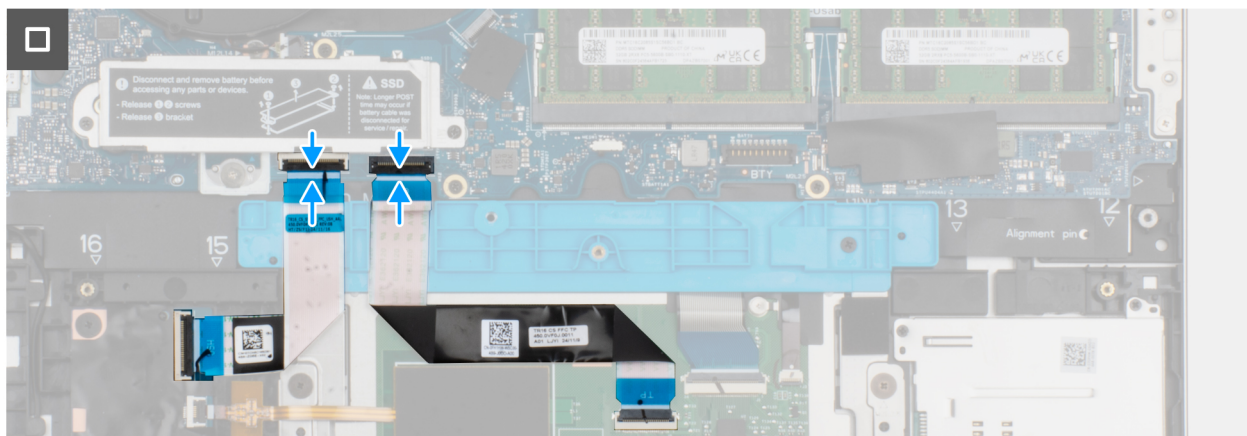
Afbeelding 46. De ondersteuningsbeugel van de batterij plaatsen
