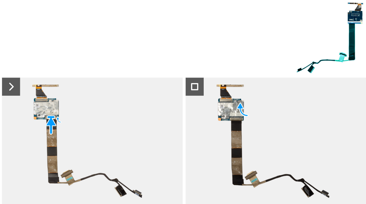
Afbeelding 74. De beeldschermkabel installeren
