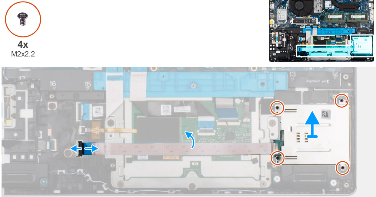
Afbeelding 48. De smartcardlezer verwijderen
