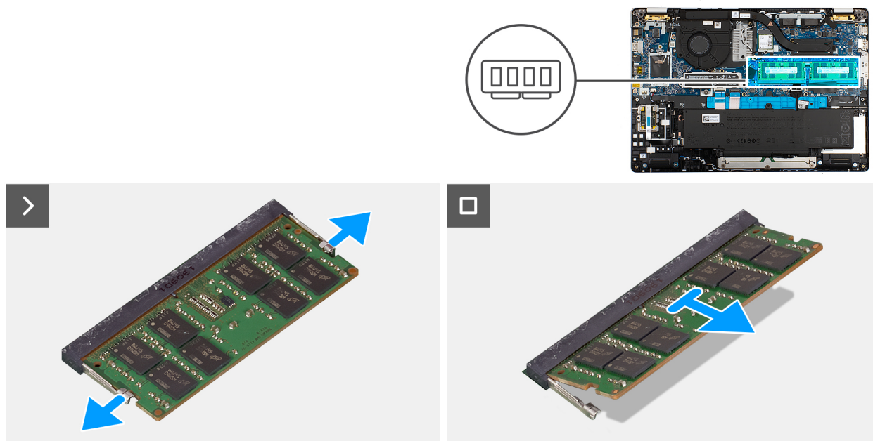
Afbeelding 22. De geheugenmodule verwijderen
