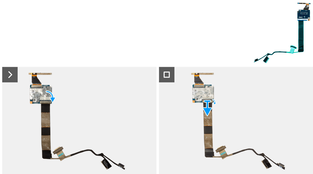
Afbeelding 73. De beeldschermkabel verwijderen
