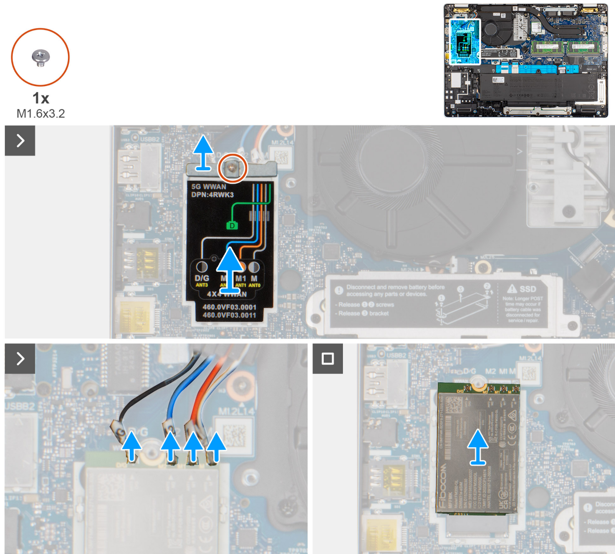
Afbeelding 30. De 5G WWAN-kaart verwijderen
