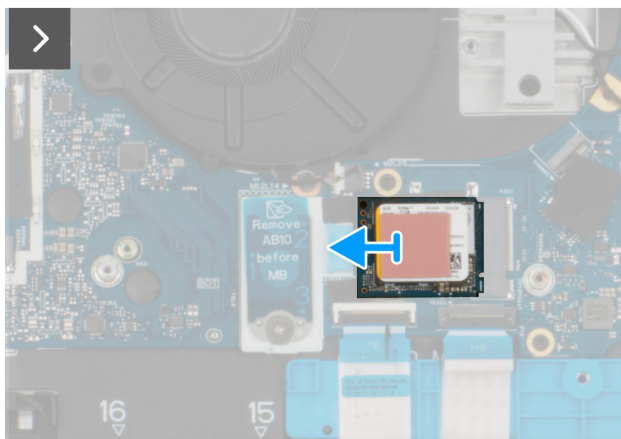
Afbeelding 24. De M.2 2230 SSD verwijderen
