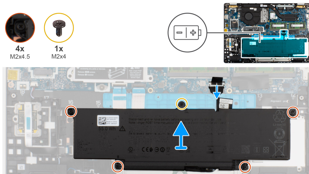
Afbeelding 18. De batterij verwijderen
