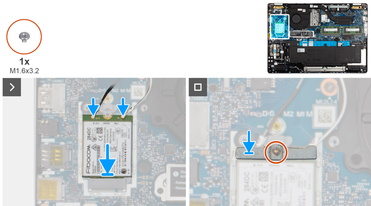
Figure 34. Installation de la carte WWAN 4G
