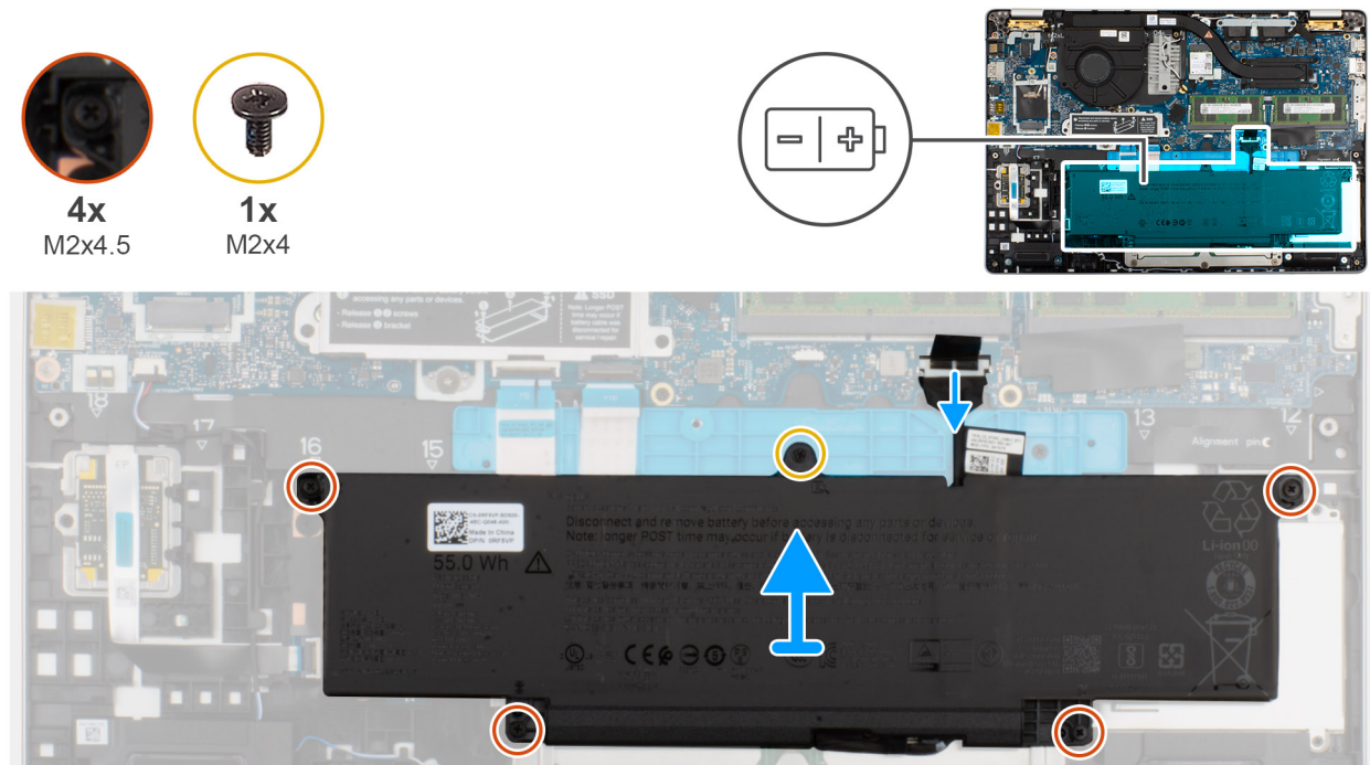
Figure 18. Retrait de la batterie
