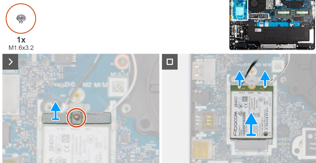
Figure 33. Retrait de la carte WWAN 4G
