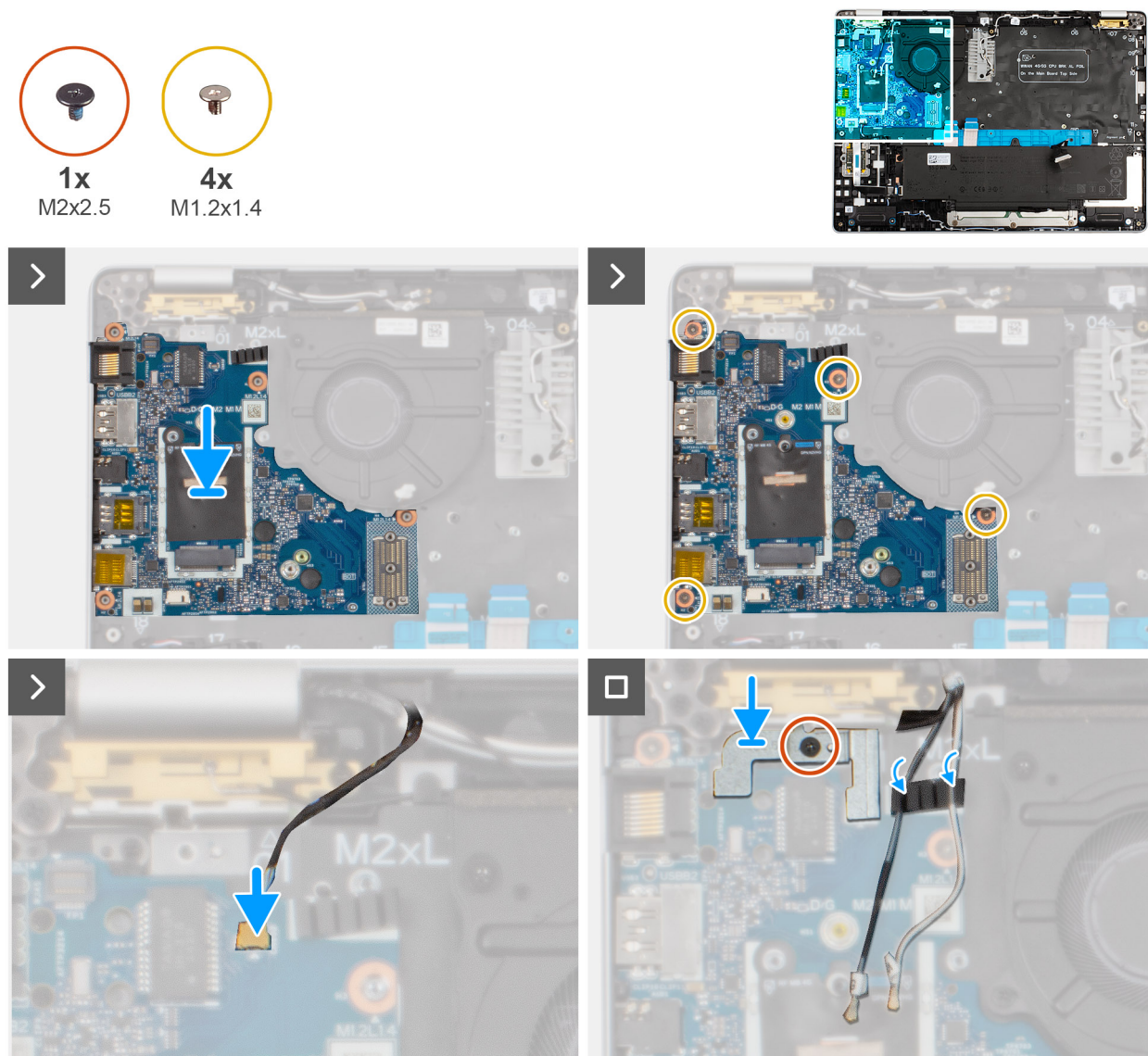
Figure 58. Retrait de la carte d'E/S
