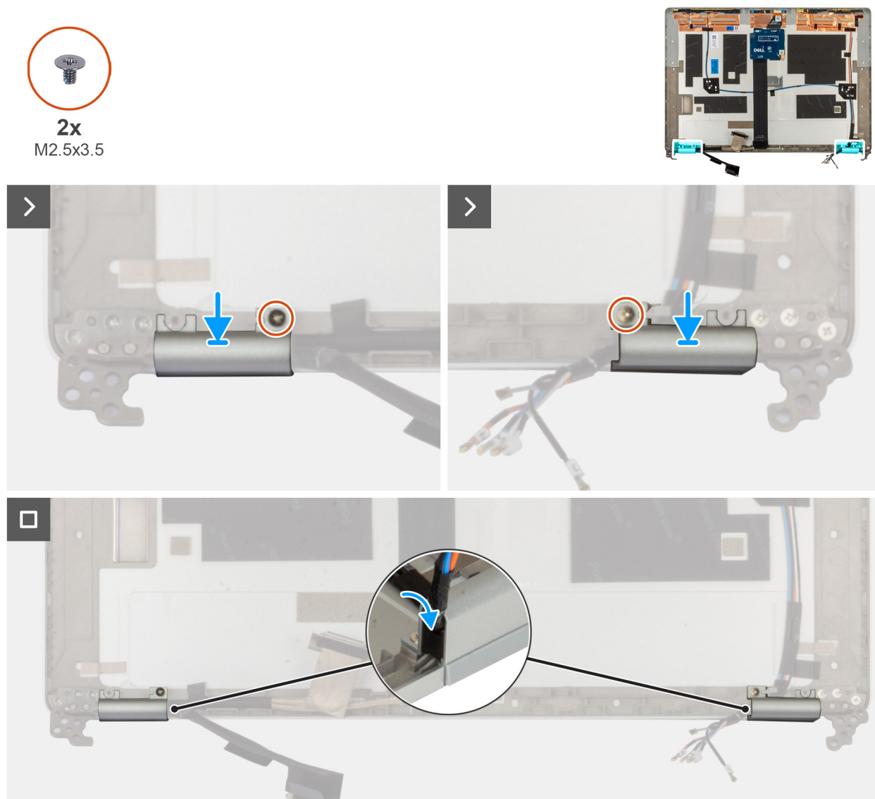
Figure 75. Installation du cache de la charnière d'écran
