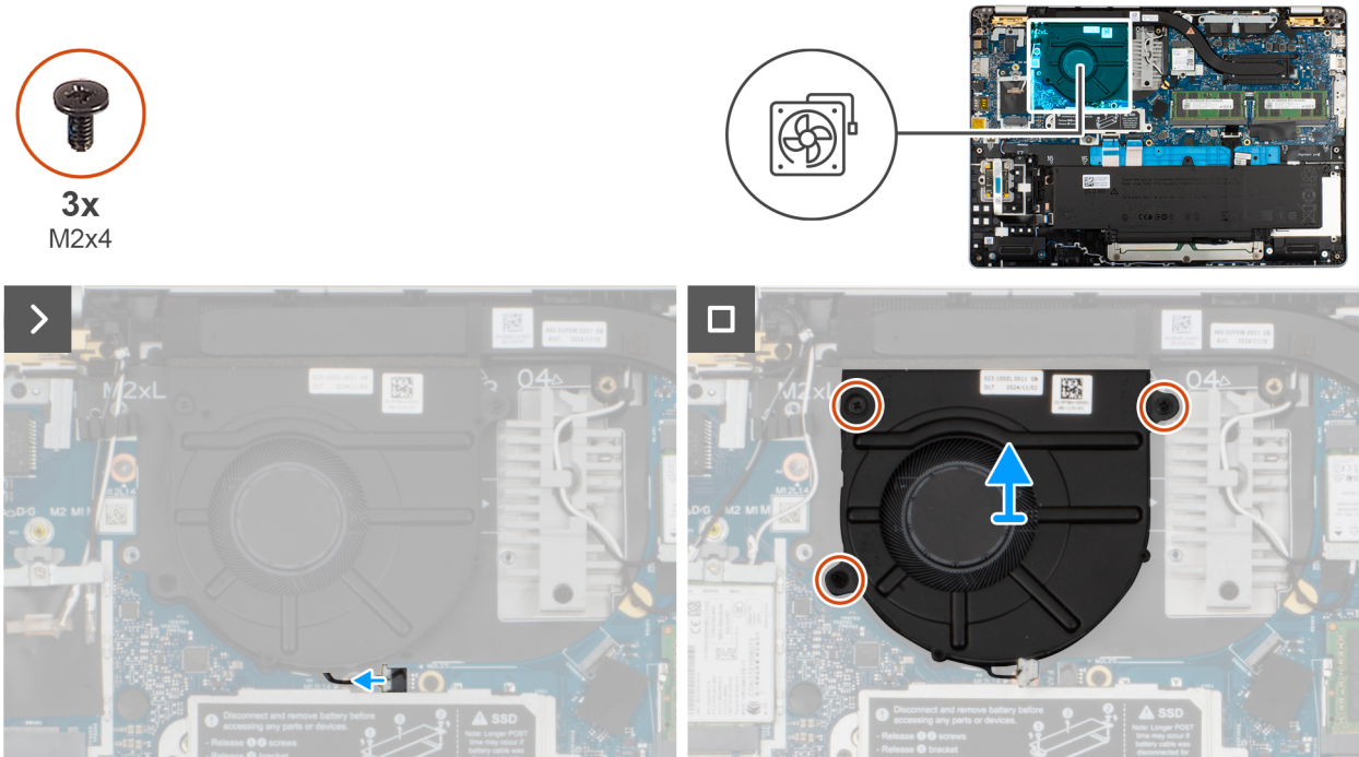
Figure 37. Retrait du ventilateur
