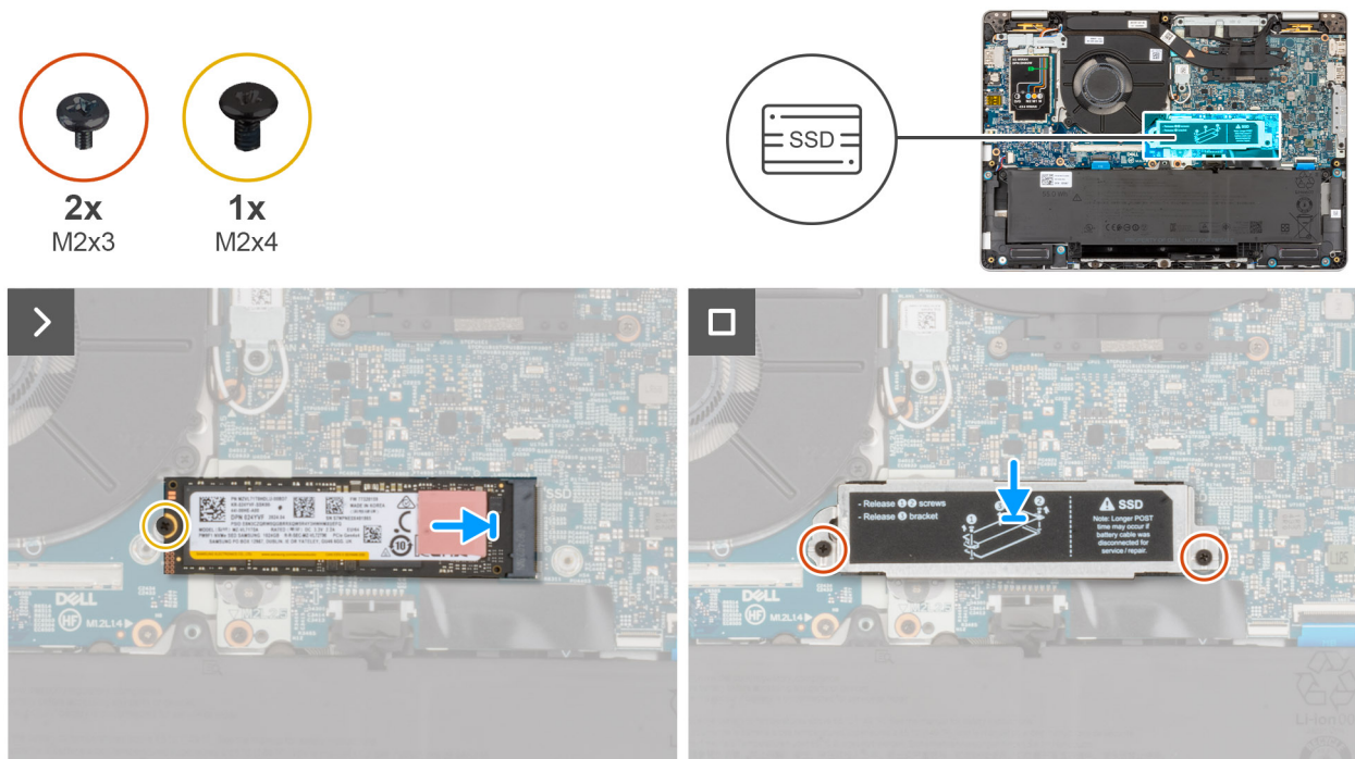
Figure 28. Installation du disque SSD M.2 2280
