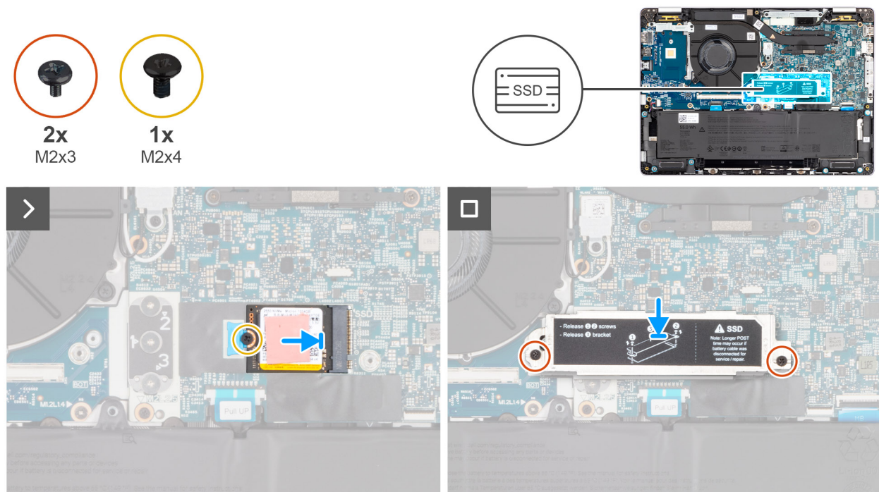
Figure 26. Installation du disque SSD M.2 2230
