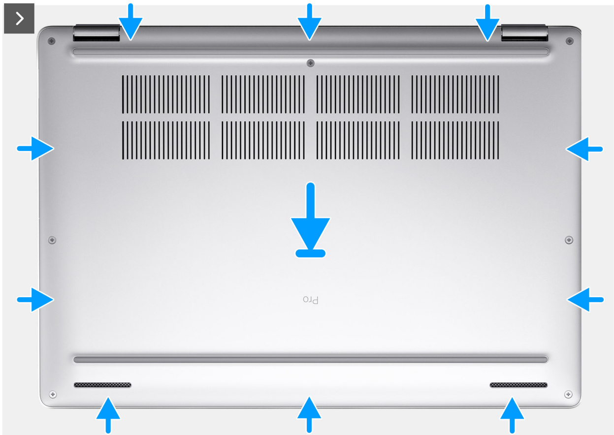
Figure 17. Installation du cache de fond
