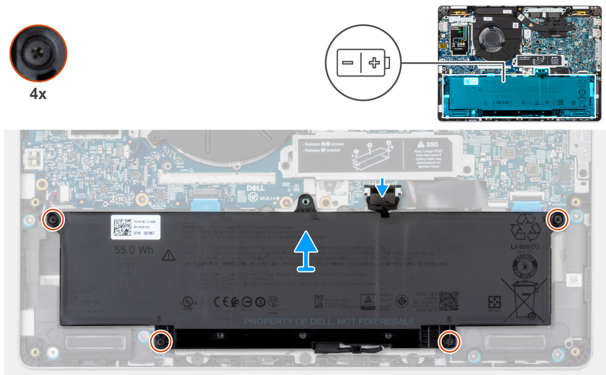
Figure 19. Retrait de la batterie
