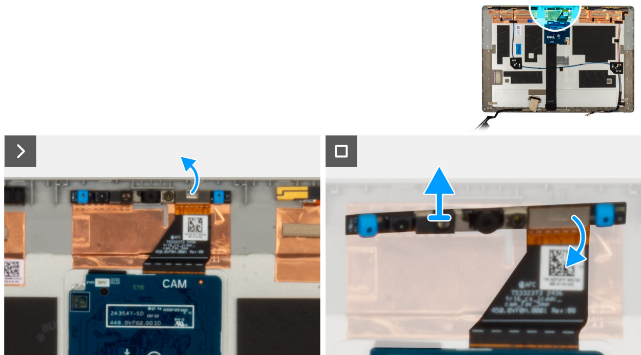
Afbeelding 69. De cameramodule verwijderen
