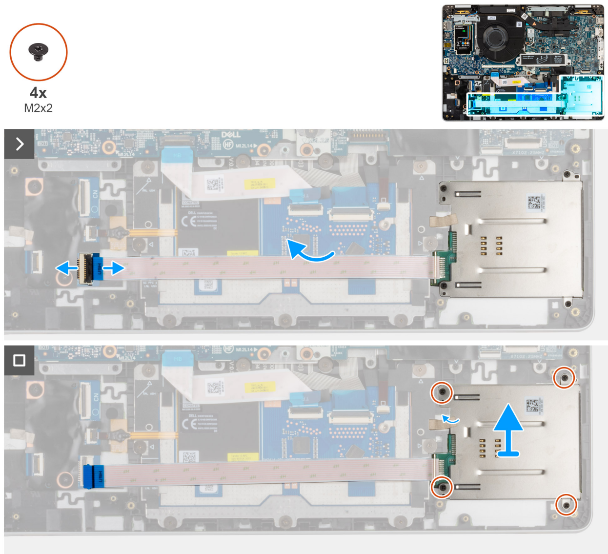
Afbeelding 36. De smartcardlezer verwijderen
