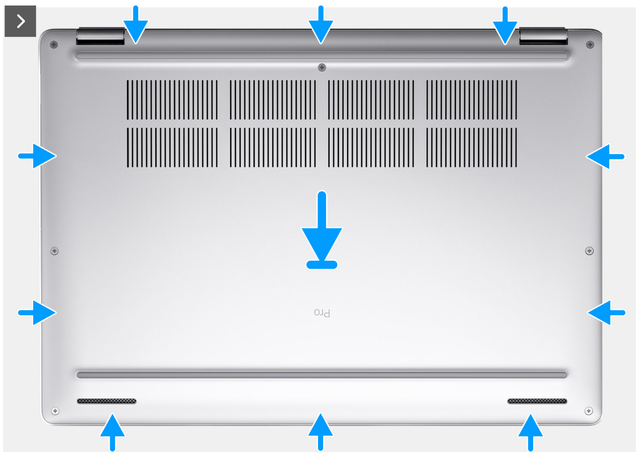
Afbeelding 17. De onderplaat installeren
