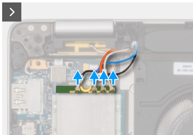
Afbeelding 23. De 5G WWAN-kaart verwijderen
