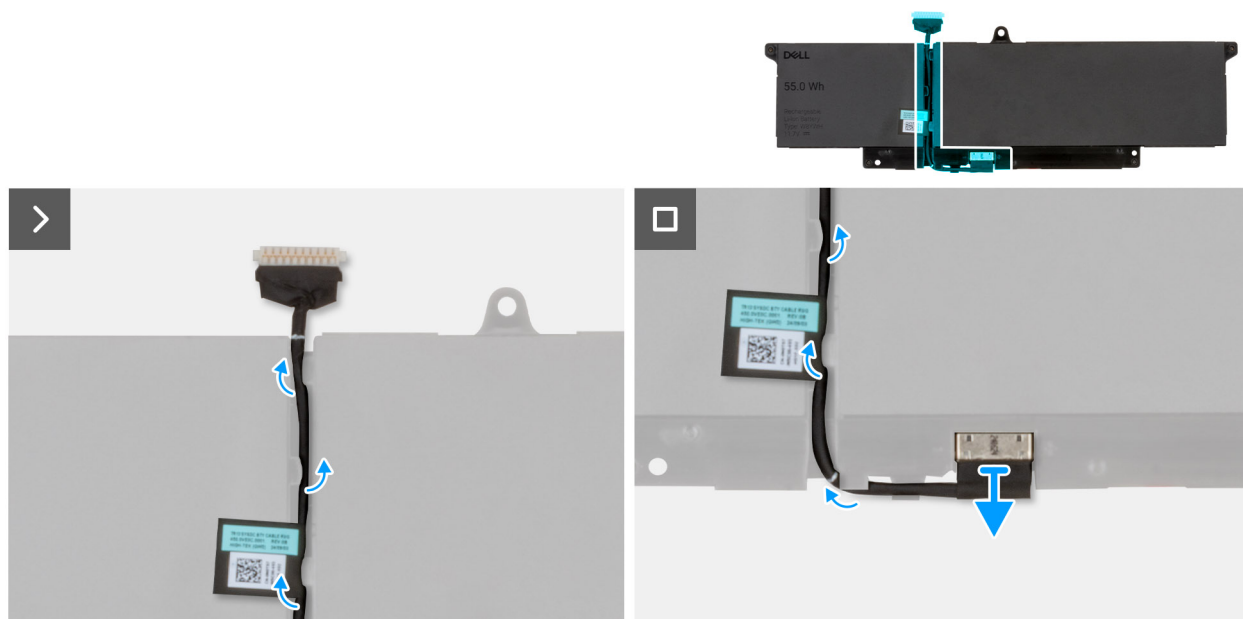
Afbeelding 21. De batterijkabel verwijderen
