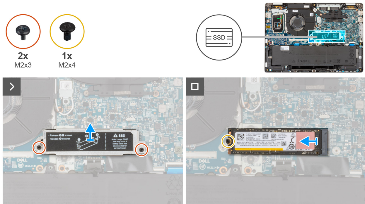
Afbeelding 27. De M.2 2280 SSD verwijderen
