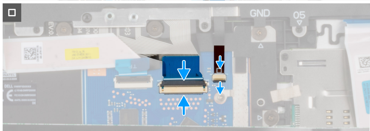
Afbeelding 60. Het toetsenbord plaatsen
