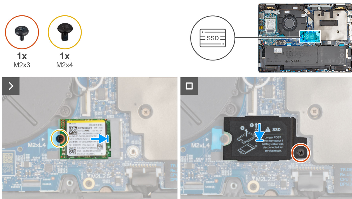
Obrázek 28. Montáž disku SSD M.2 2230
