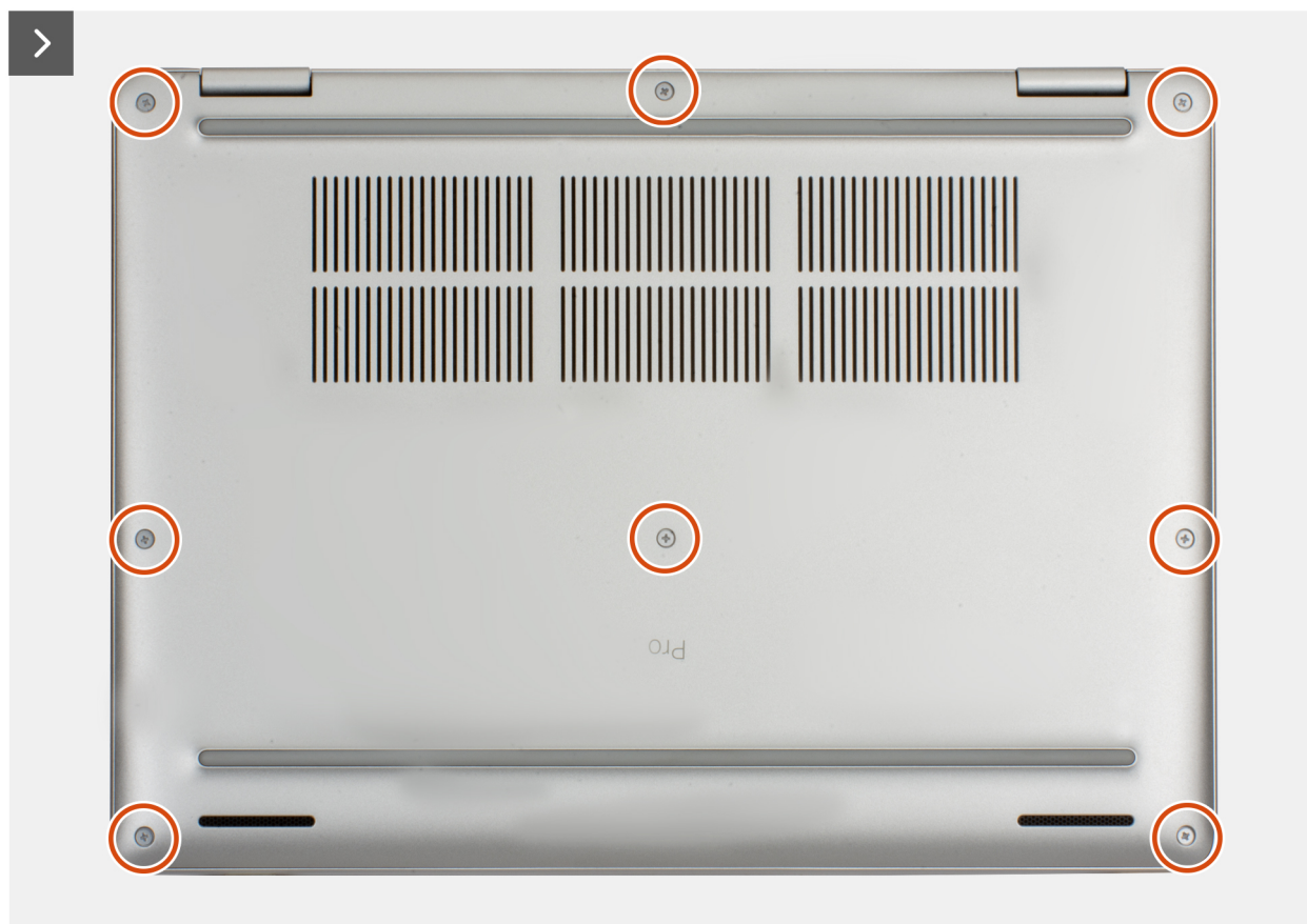
Obrázek 15. Sejmутí spodního krytu
