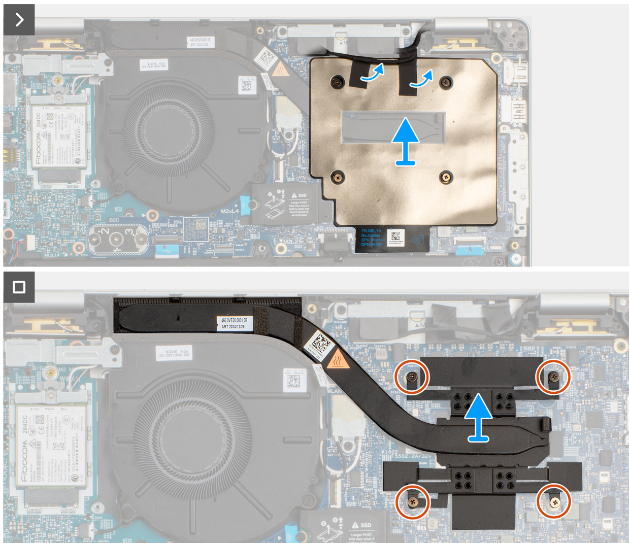
Obrázek 45. Demontáž chladiče
