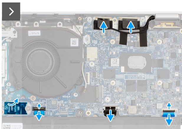
Obrázek 40. Demontáž základní desky
