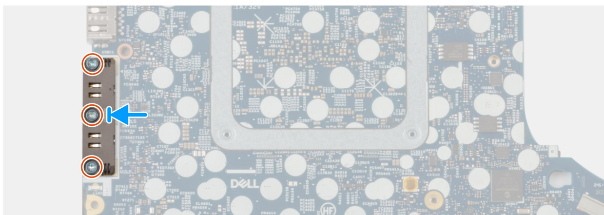
Obrázek 52. Montáž modulu konektoru USB Type-C
