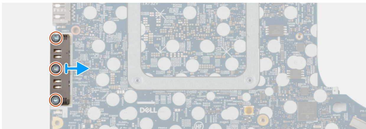
Obrázek 51. Demontáž modulu konektoru USB Type-C
