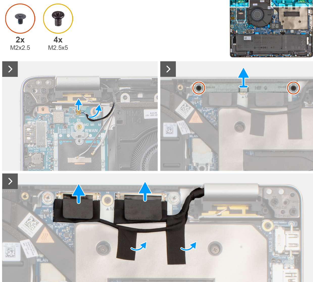
Obrázek 58. Demontáž sestavy displeje
