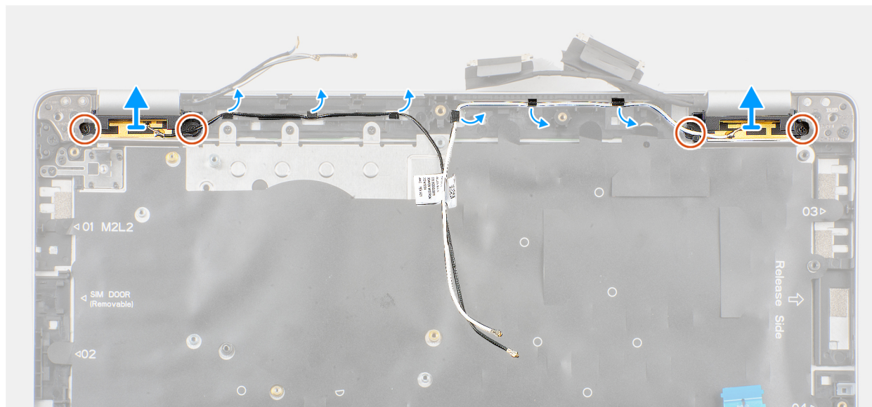
Obrazek 43. Demontáž anténního modulu WLAN
