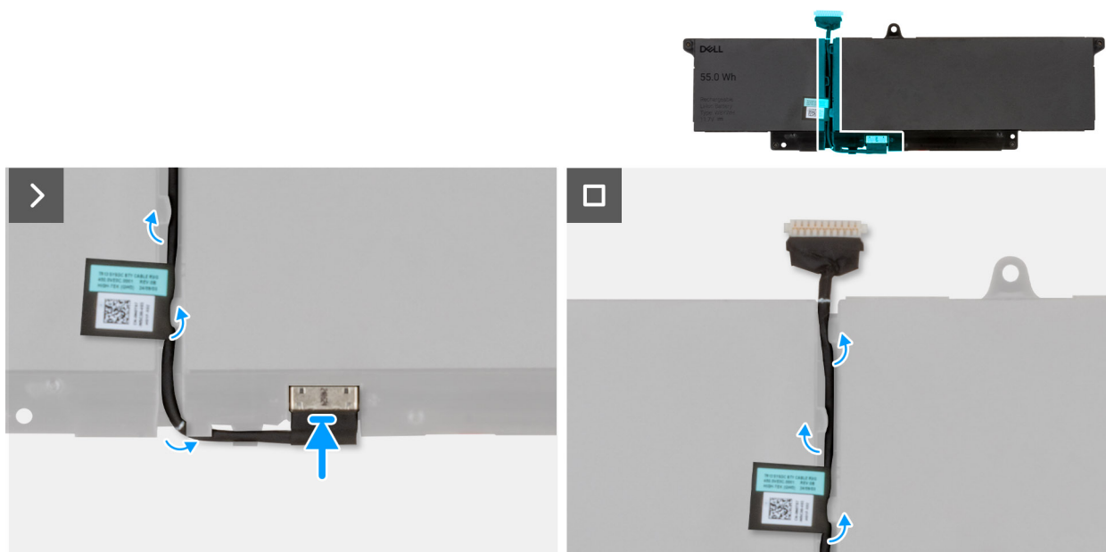
Obrázek 24. Montáž kabelu baterie
