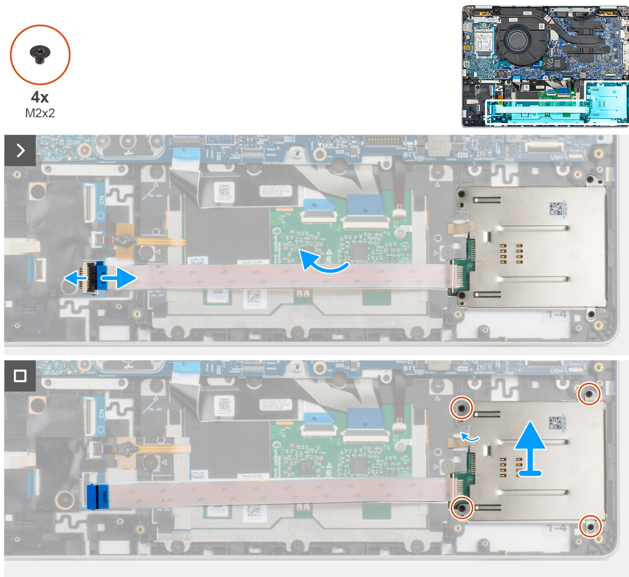
Obrázek 37. Demontáž čtečky čipových karet
