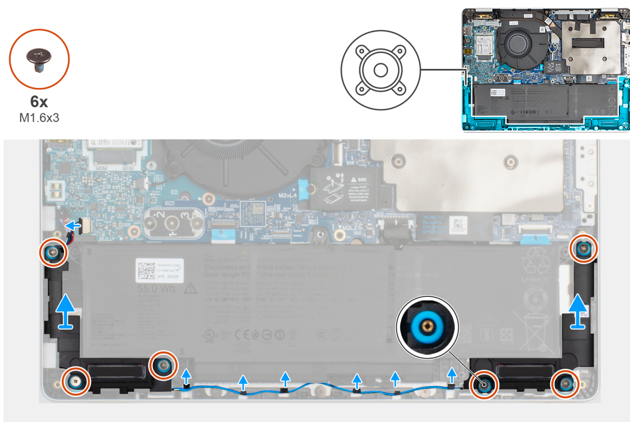
Obrázek 29. Demontáž reproduktorů
