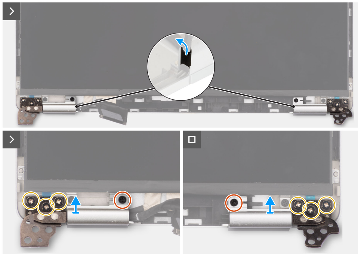
Obrázek 68. Demontáž pantů displeje
