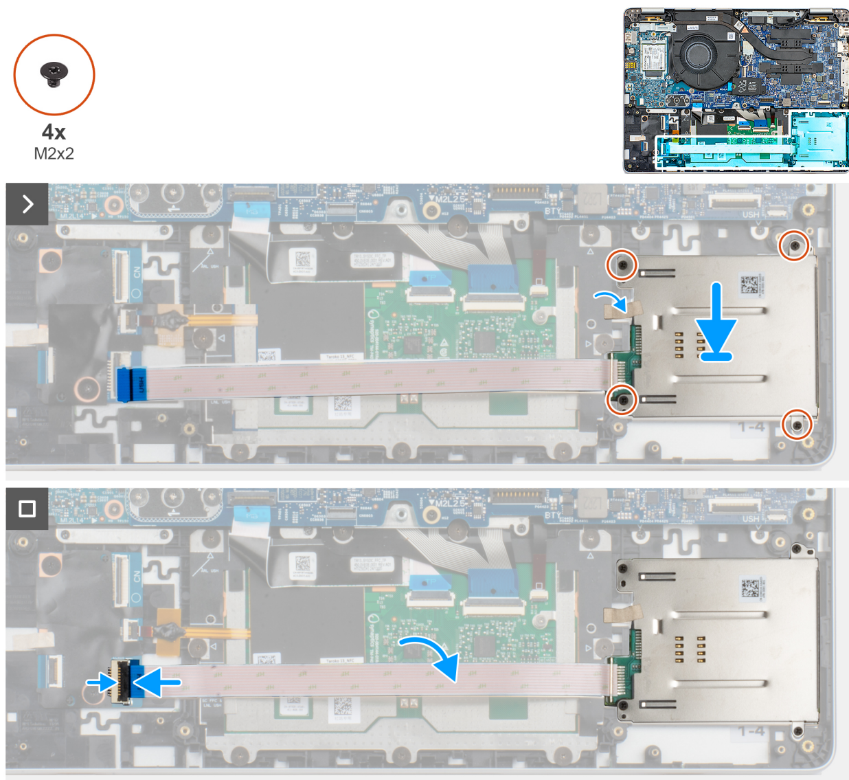
Obrázek 38. Montáž čtečky čipových karet
