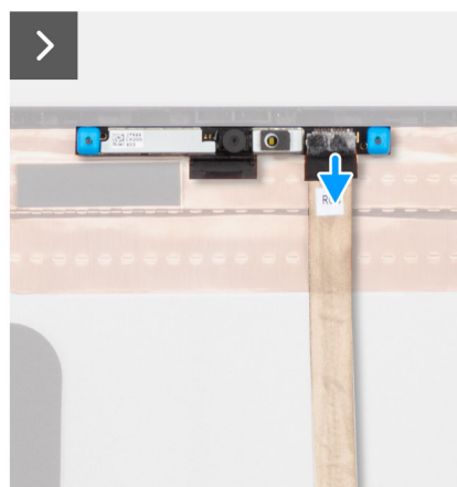
Obrázek 73. Vložení kabelu displeje
