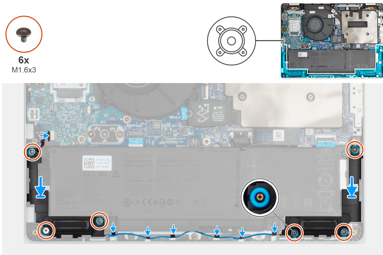
Obrázek 30. Montáž reproduktorů
