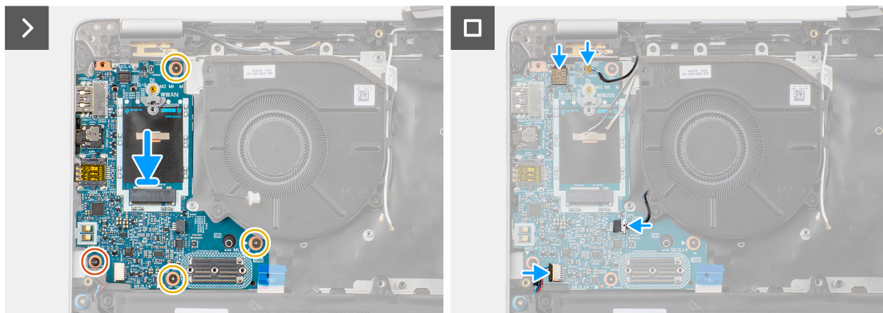
Obrázek 48. Vložení desky I/O
