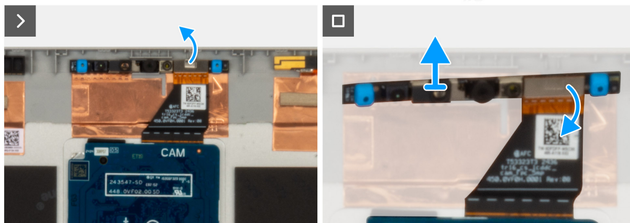
Obrázek 70. Demontáž modulu kamery
