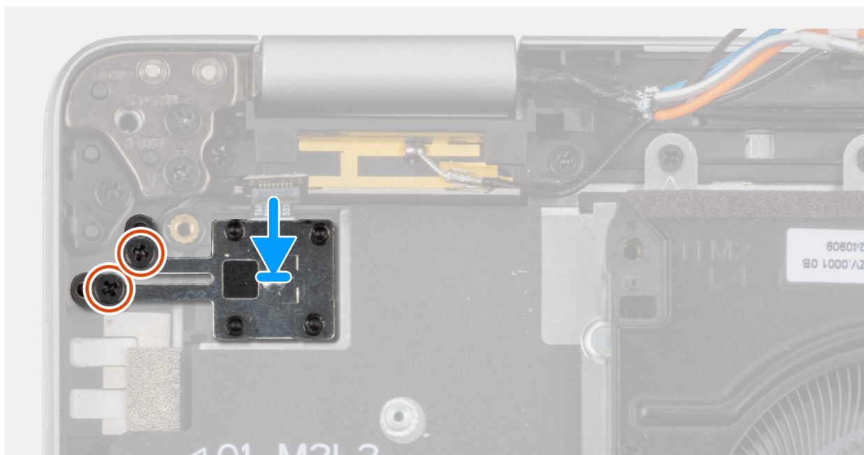
Obrázek 50. Montáž tlačítka napájení s volitelnou čtečkou otisků prstů
