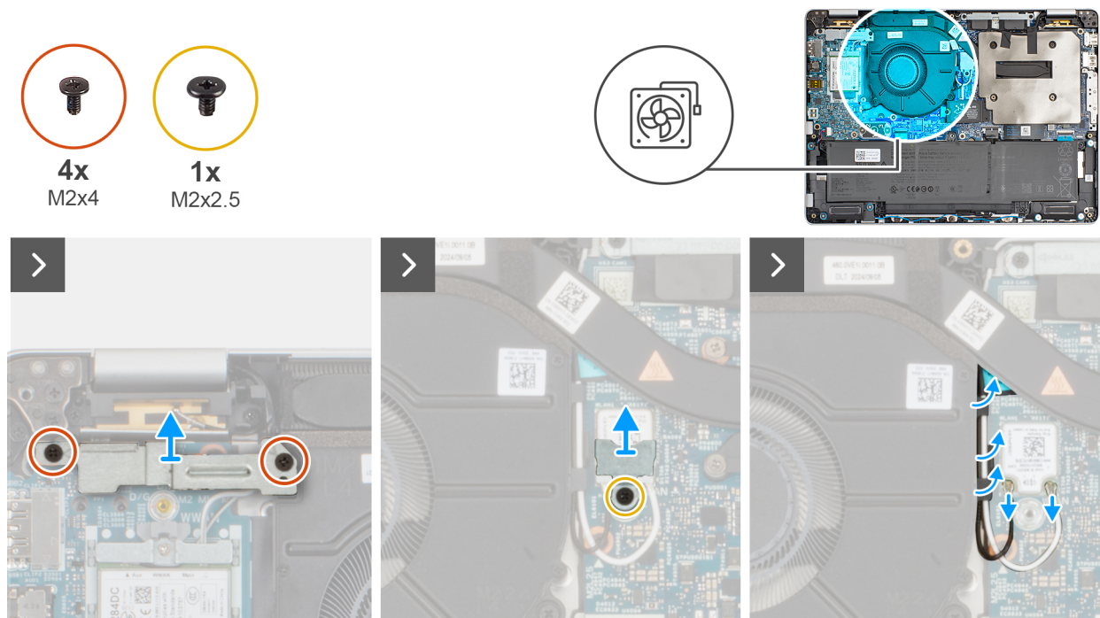
Obrázek 31. Demontáž ventilátoru
