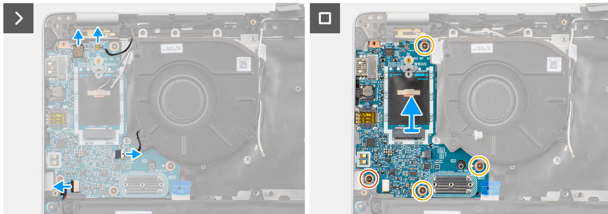
Obrázek 47. Demontáž desky I/O
