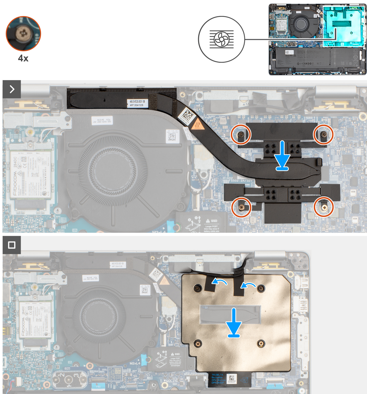
Obrázek 46. Montáž chladiče
