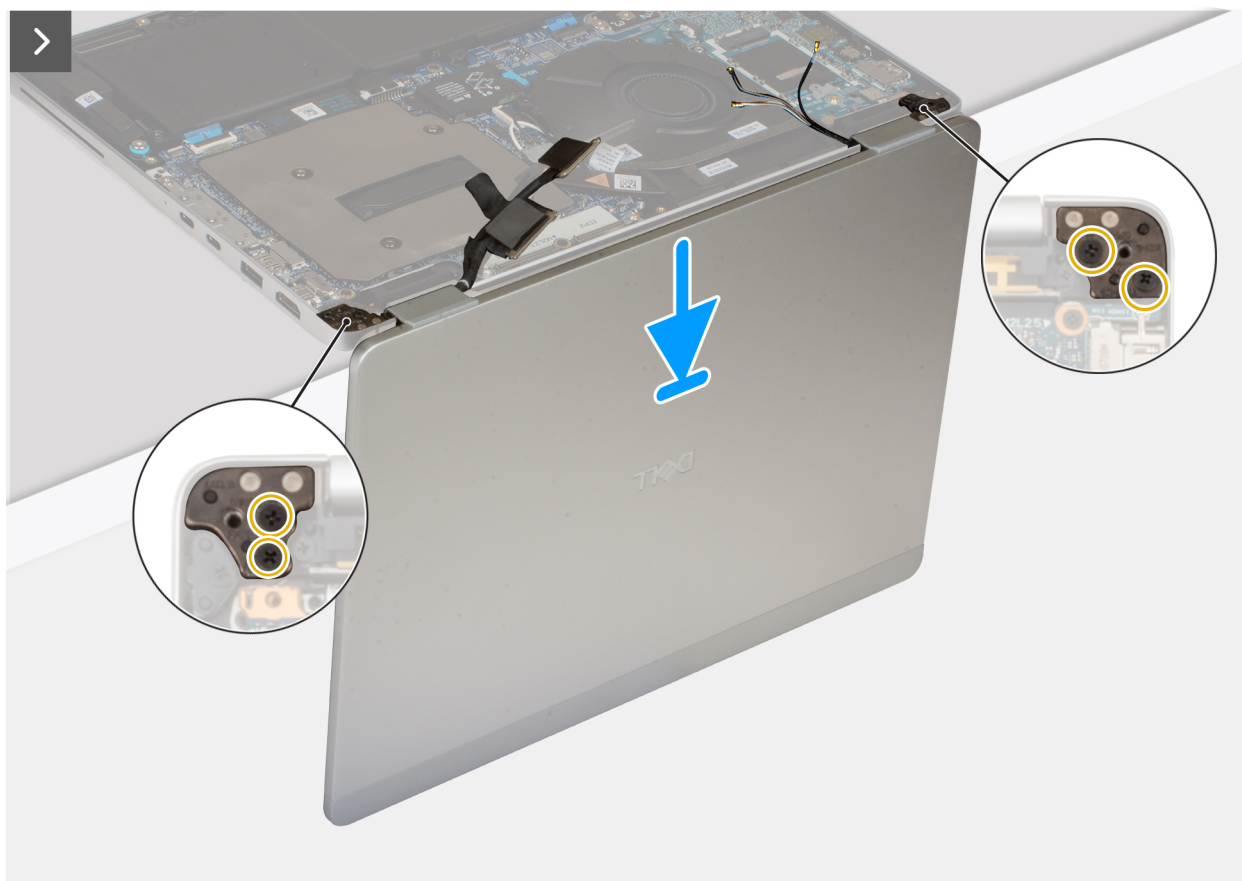
Obrázek 60. Montáž sestavy displeje
