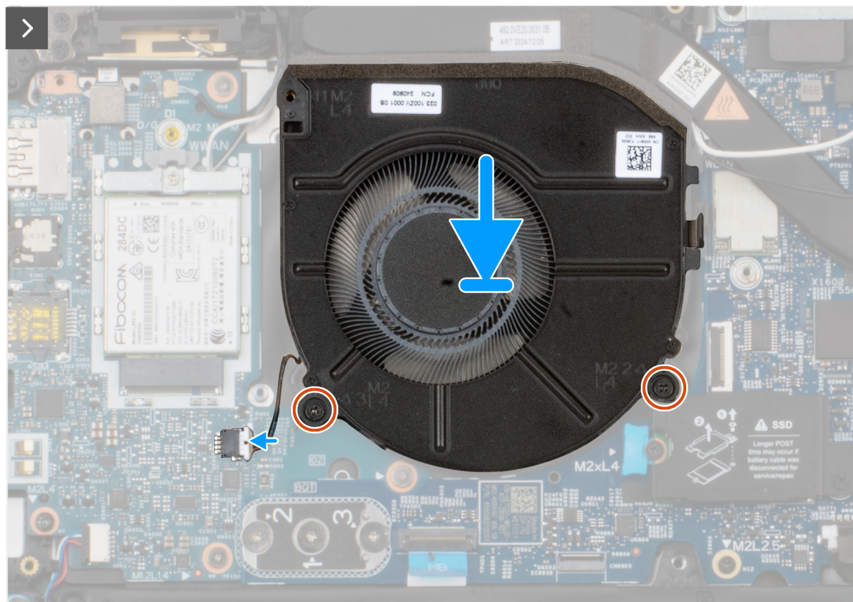
Obrázek 33. Montáž ventilátoru
