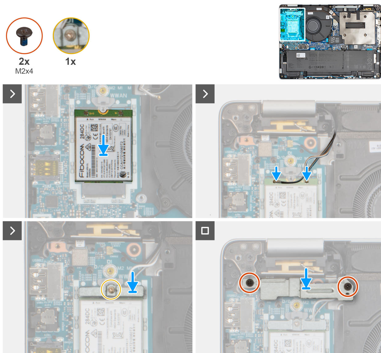
Obrázek 26. Montáž karty 4G WWAN
