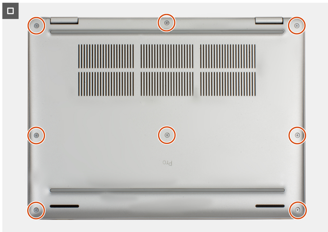
Obrázek 20. Nasazení spodního krytu
