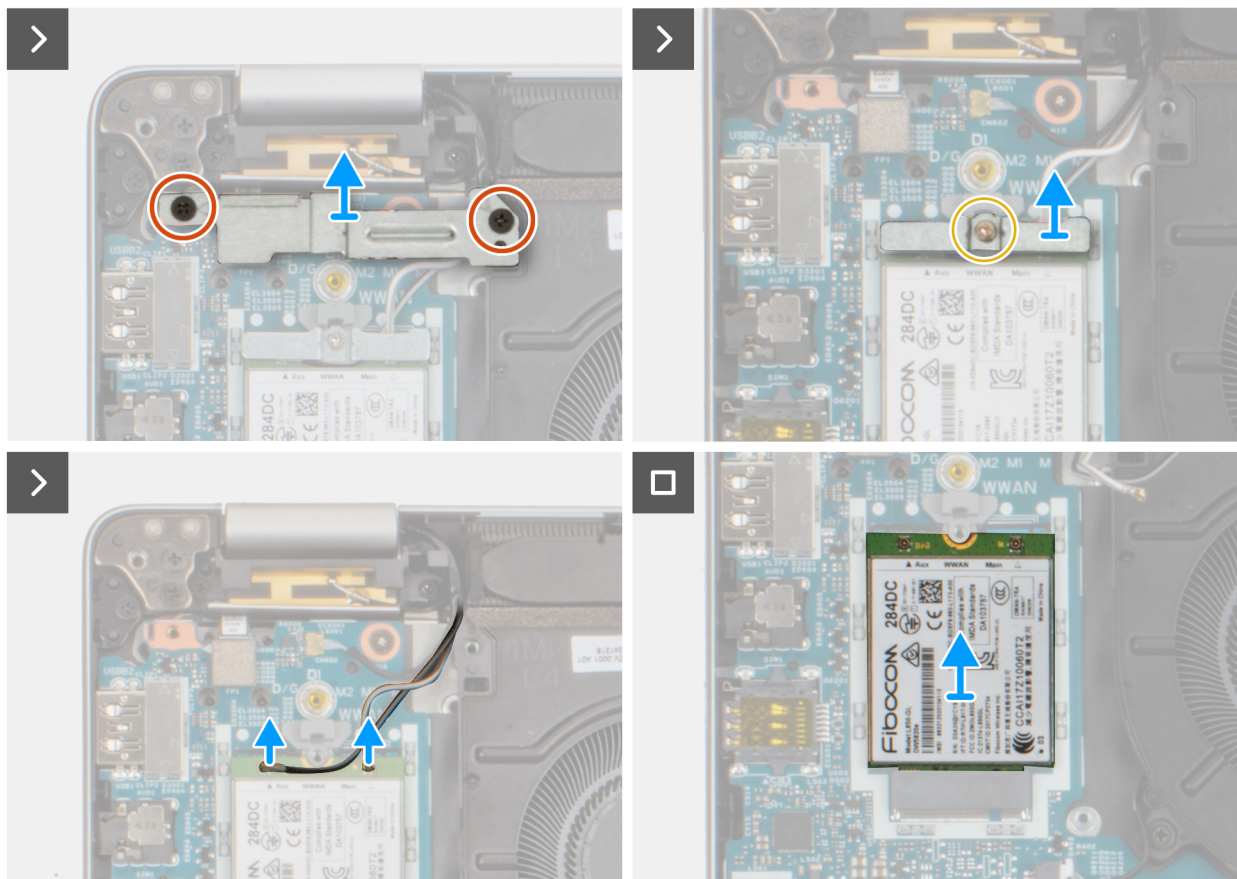
Obrázek 25. Vyjmutí karty 4G WWAN
