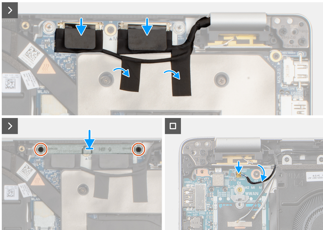
Obrázek 61. Montáž sestavy displeje
