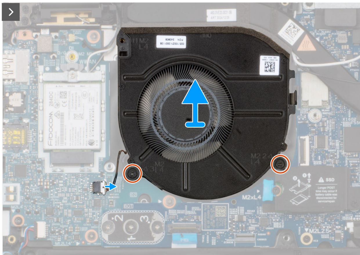
Obrázek 32. Demontáž ventilátoru
