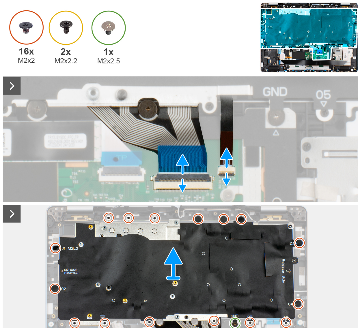
Obrázek 53. Demontáž klávesnice
