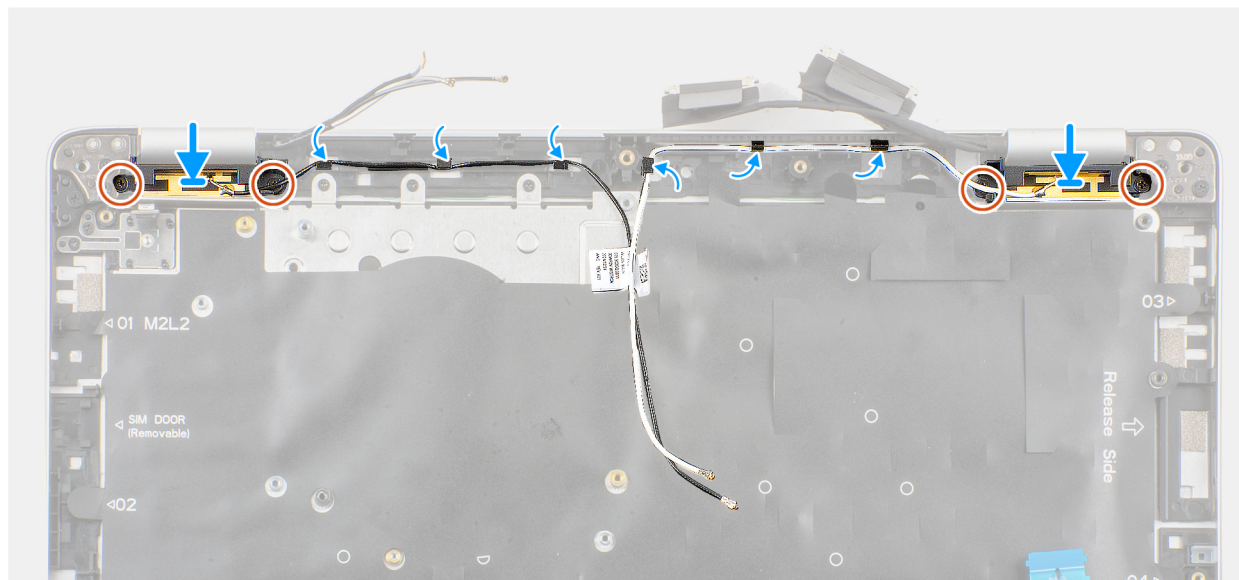
Obrázek 44. Montáž anténního modulu WLAN
